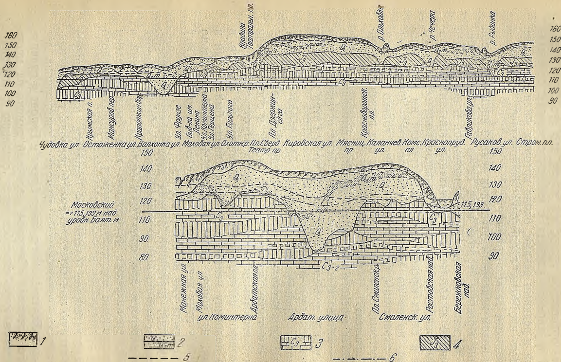
Рис. 20. Схематические геологические разрезы по линии московского метрополитена. Верхний рисунок — Кировско-Усачевская линия. Нижний рисунок — Арбатская линия.
