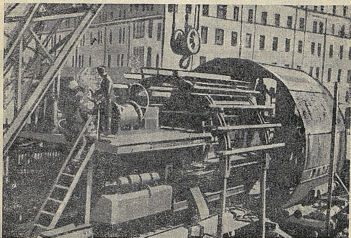
Рис. 14. Сборка щита.
