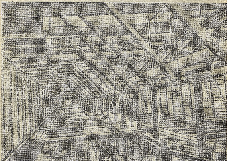
Рис. 13. Проходка открытым способом. Крепление котлована.
