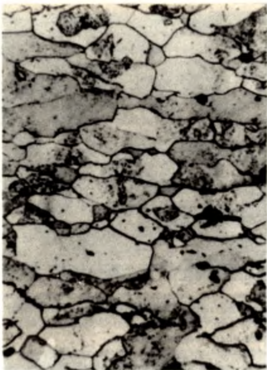
Рис. 48. Ориентированно-бластическая структура пиритовой руды. Полиров, шлиф, увел. 58.5. Хаутаваарское месторождение.
