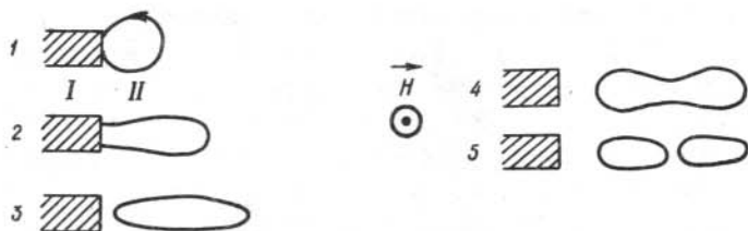
Рис.21. Пять стадий формирования длинного плазмоида по Бостикку /129/.
