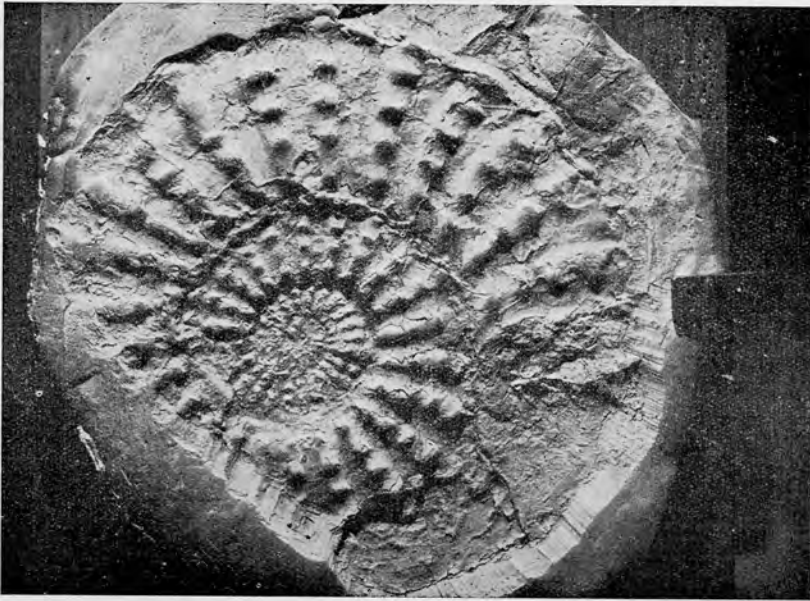
Abb. 93. Mortonicerias pseudo-texanum GROSS.
