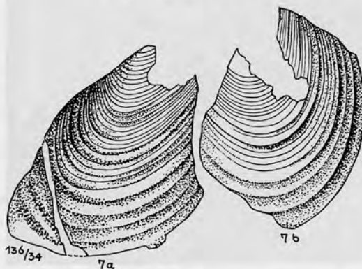
Abb. 7 a u. b. Inoceramus inconstans WOODS em. ANDERT, flach gedrückt a) Steinkern, b) Innenseite der Kalkschale. Oberes Mittelturon (klingender Inoceramenpläner), Hostin 1. Orig. Geol. Landesmus. (A No. 30.)
