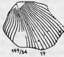
Abb. 19. Spondylus lamellatus NILSS. sp., Steinkern. Oberflächenzeichnung unter Benützung des Hohldruckes. Oberturon \alpha\beta , Waltersdorf 2. Orig. Geol. Landesmus. (A No. 126).
