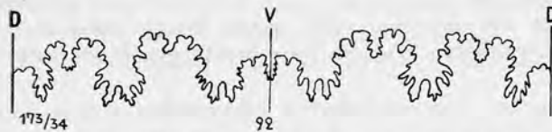
Abb. 92. Baculites bohemicus FRIC, Lobenlinie, vergr. 2:1. Emscher, Kieslingswalde. Orig. Geol. Landesmus. (A No. 605).
