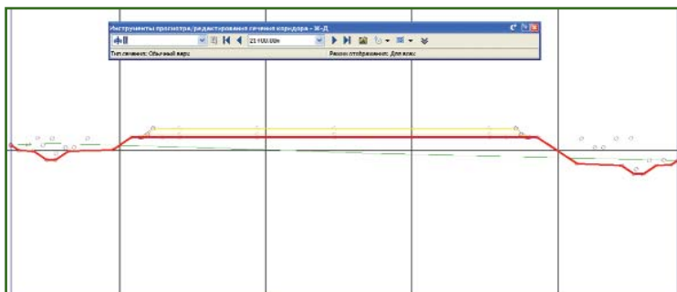
Рис. 7 Сечение коридора
