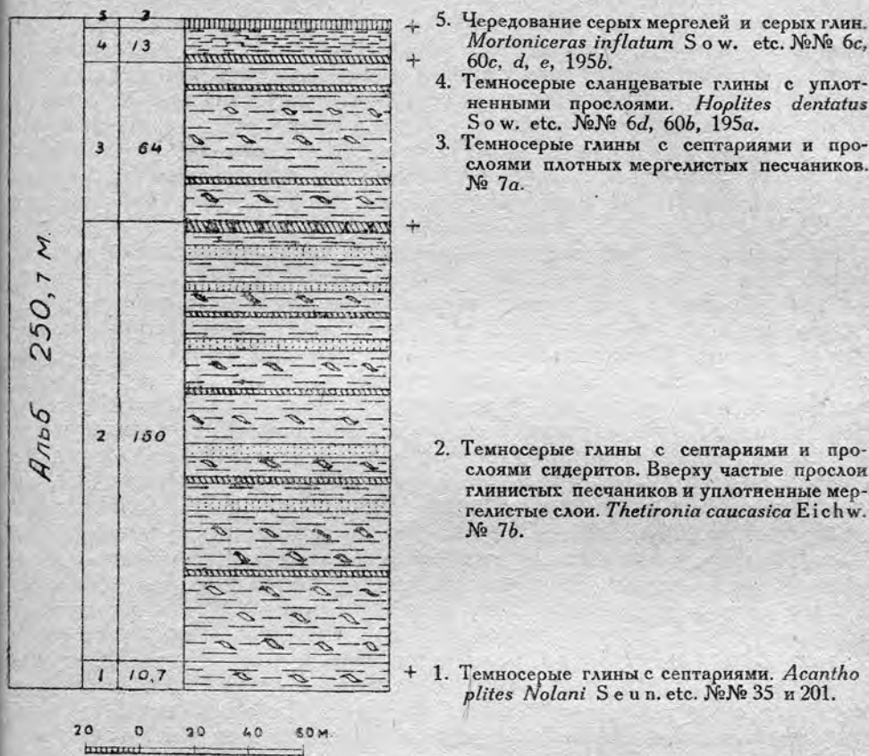
Рис. 8. Альбский ярус. Albian.
