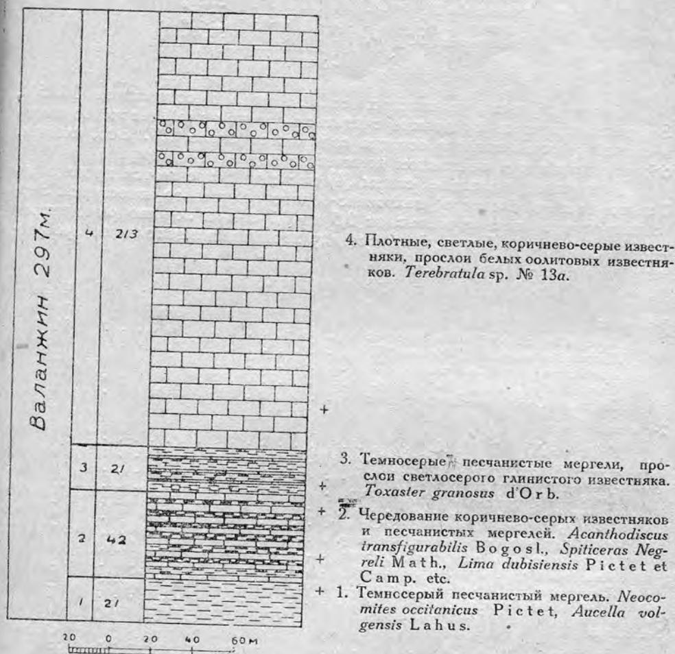
Рис. 4. Валанжинский ярус. Valanginian.
