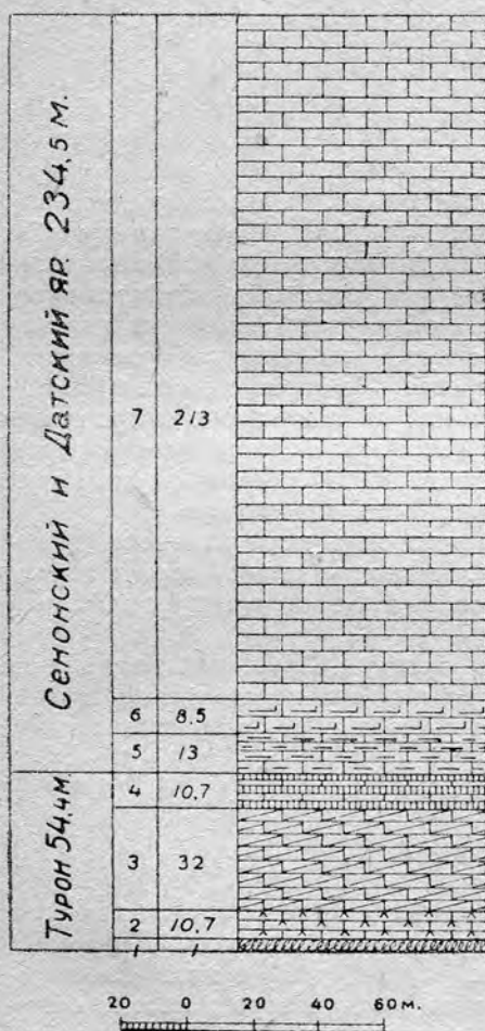
Рис. 9. Верхний мел. Upper Cretaceous.
