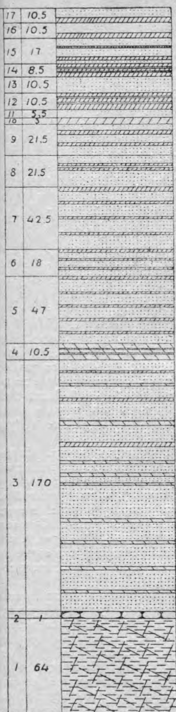
Рис. 5. Готеривский ярус. Hauterivian.
