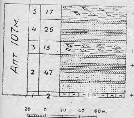
Рис. 7. Аптекий ярус. Aptian.
