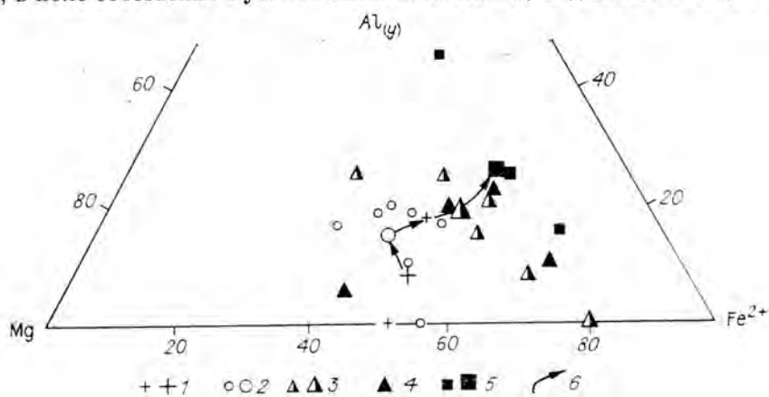
Рис. 7.4. Диаграмма Mg — Fe 2+ — Al(y) для турмалина.
