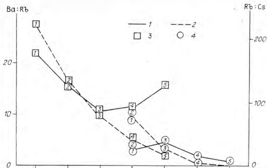
Рис. 7.1. Величины отношений Rb/Cs (1) и Ba/Rb (2) в последовательных генерациях калишпатов (3) и мусковитов (4) в двуполовошпатовых пегматитах Восточной Сибири. Номера точек соответствуют номерам средних величин в табл. 7.3 и 7.7.
