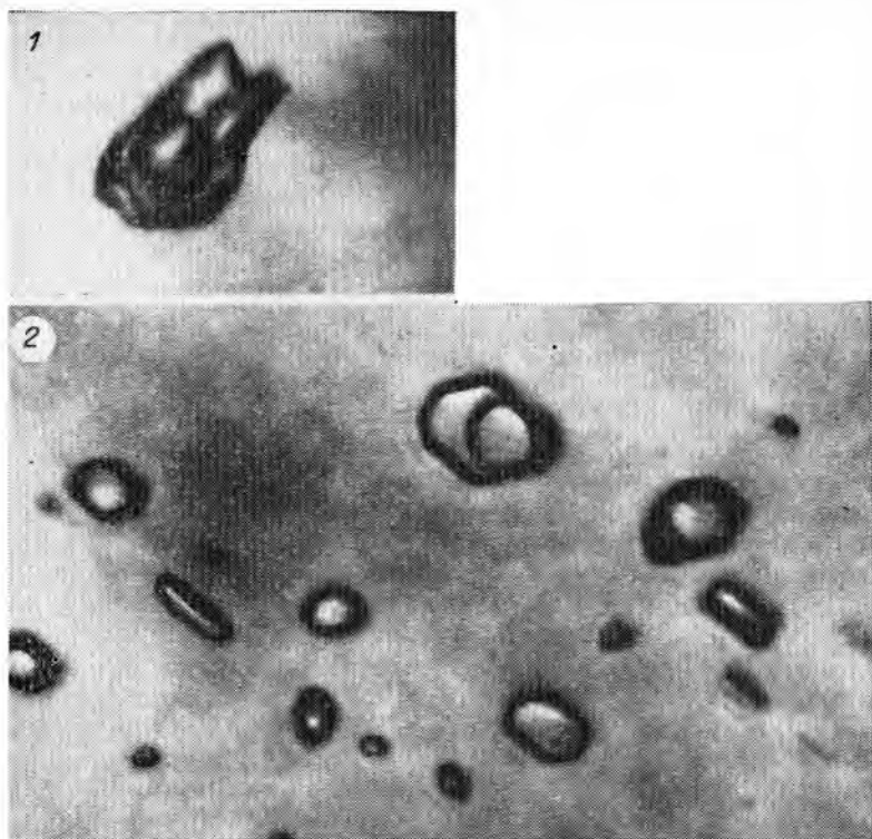
Рис. 6.4. Водно-углекислотные включения в минералах пегматитов 1 — кварц, 2 — мусковит.
