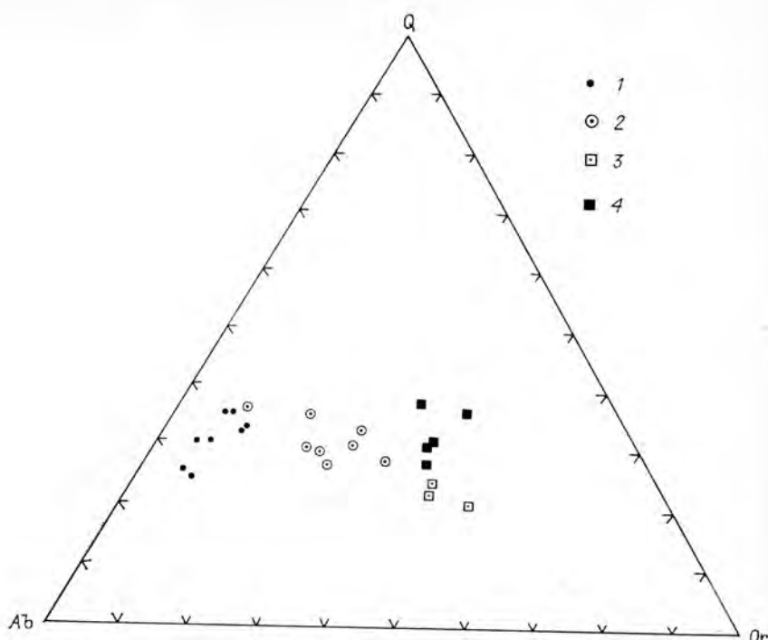
Рис. 3.5. Положение пегматоидных гранитов Мамского пояса на тройной диаграмме альбит (Ab)— ортоклаз (Or)— кварц (Q).
