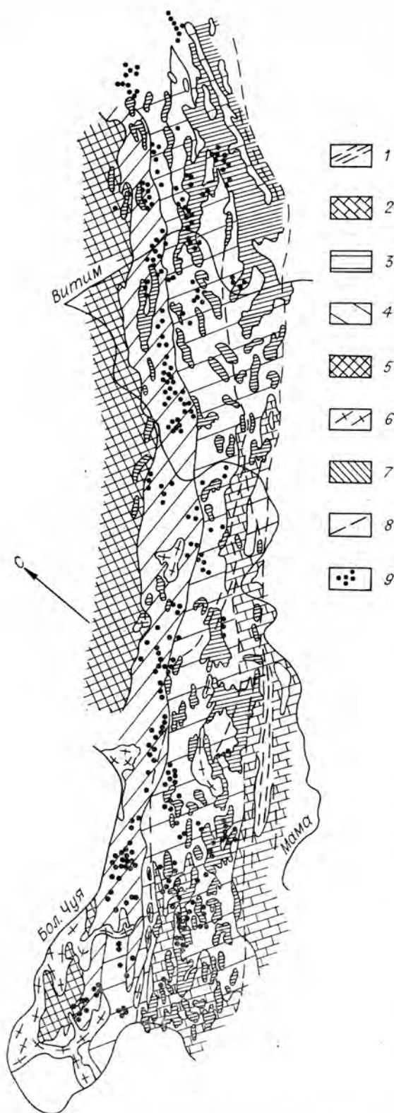
Рис. 3.1. Схематическая карта распространения пород в Мамском пегматитовом поясе, по В. Н. Чеснокову. [Геологические факторы..., 1972].
