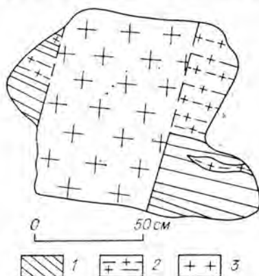
Рис. 3.3. Пересечение биотитового гнейса (1) и плагиоклазового гранита (2) двуполевошпатовым пегматоидным гранитом (3).
