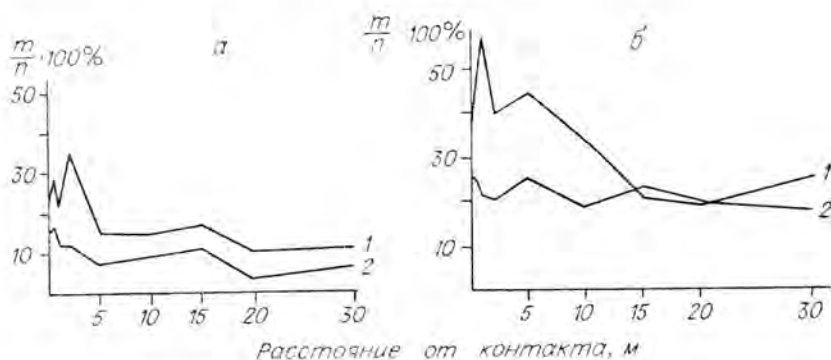
Рис. 9.6. Встречаемость мусковита, замещающего плагиоклаз (а) и «се-кущего» (б) в экзоконтактах пегматитов.
