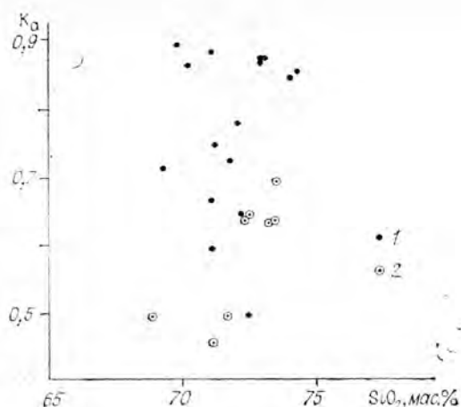
Рис. 3.4. Положение двуполевошпатовых (1) и плагиоклазовых (2) пегматоидных гранитов Мамского пояса на диаграмме коэффициент агнайтности K_a — кремнеземистость ( SiO_2 ).
