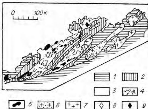
Рис. 2.28. Схема метаморфических и главнейших гранитоидных массивов Таймыра [Махлаев, 1987] и размещение пегматитовых проявлений.
