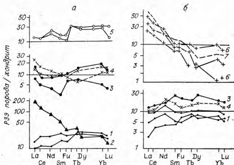
Рис. 2.22. Спектры редкоземельных элементов в толеитовой серии нюрн-дунских метабазитов и продуктах их гранитизации (а) и известково-щелочной серии (б).
