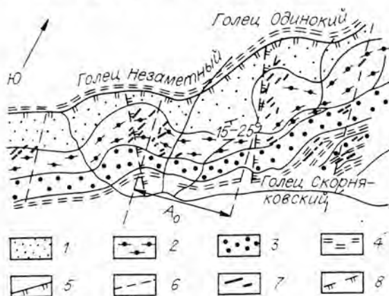
Рис. 4.7. Схема размещения мусковитовых пегматитов центральной части Согдиондонского месторождения. [Тарасов и др., 1975].
