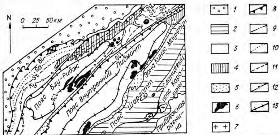
Рис. 2.4. Схема тектоники и геологического строения [по Lesure, 1968] и метаморфической зональности [по Butler, 1972] поясов Блу-Ридж и Пидмонт.
