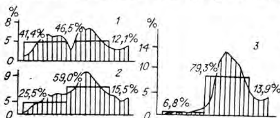
Рис. 10.2. Декрептограммы мусковитовых пегматитов Мамского пояса [Карский и др., 1974].
