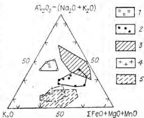
Рис. 2.7. Составы гранитов и вулканоплутонических кислых комплексов Кристаллических Аппалач [Rankin, 1975].
