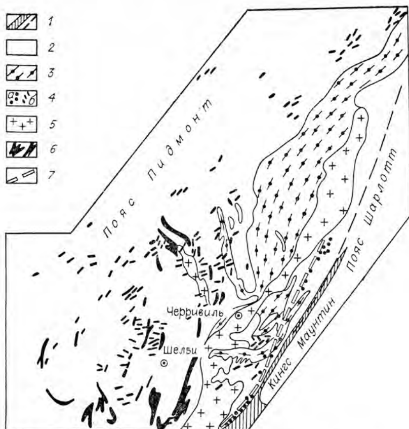
Рис. 2.8. Строение участка пояса Внутренний Пидмонт.
