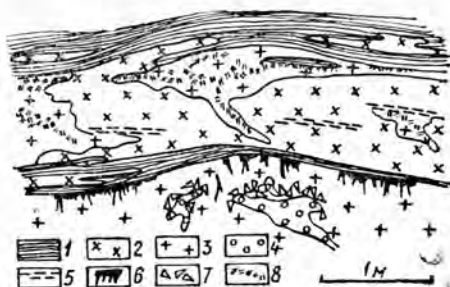
Рис. 4.4. Пологие зоны пегматита под «экранами» гнейсов. Жила 5 месторождения Большое Северное.
