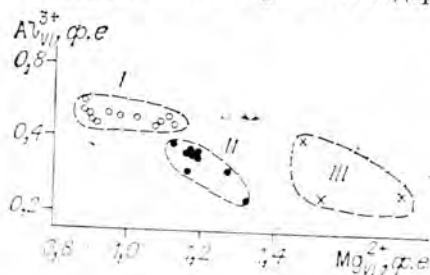
Рис. 7.2. Соотношение содержания магния и алюминия октаэдрической координации для биотитов [Слюдоносные пегматиты..., 1976].
