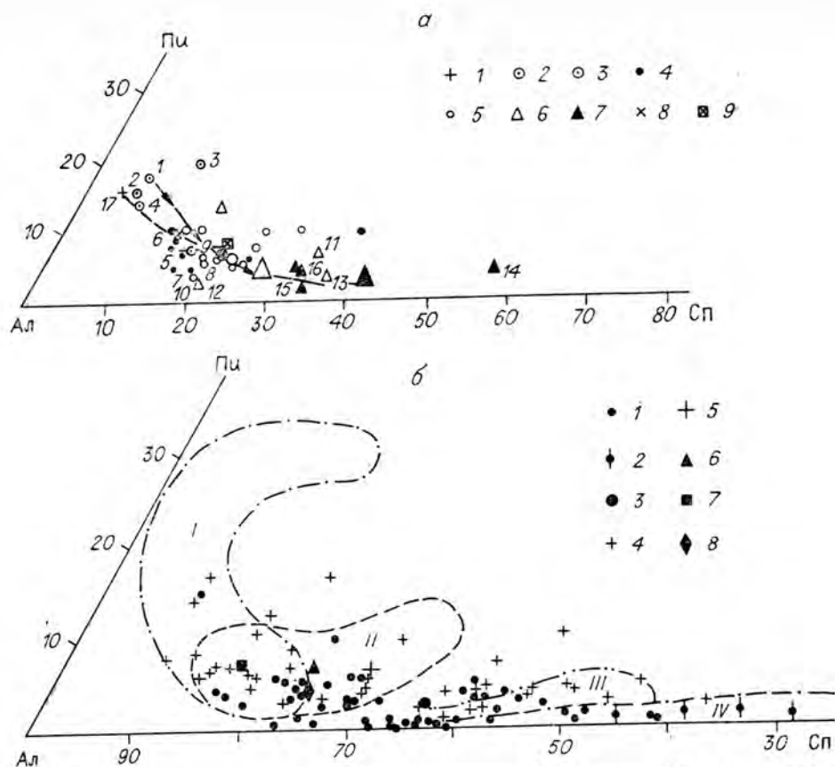
Рис. 7.3. Диаграммы альмандин (Ал)—спессартин (Сп)—пироп (Пи) для гранатов из слюдоносных пегматитов.
