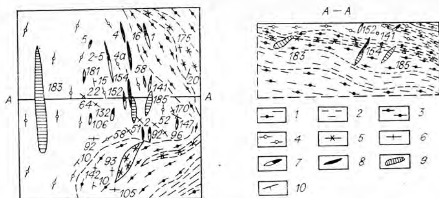
Рис. 4.8. Схема распределения различных типов слюдоносных пегматитов на южном участке месторождения Малиновая Варака [Слюдоносные пегматиты..., 1976.] 1—4 — гнейсы: 1 — гранат-биотитовые среднезернистые, 2 — биотитовые, 3 — кианит-гранат-биотитовые средне- и мелкозернистые, 4 — кианит-гранат-биотитовые грубозернистые; 5 — лейкократовые биотитовые гнейсы и аплиты; 6—9 типы пегматитов: 6—1, 7—2, 8—3, 9—4; 10 — элементы залегания. Цифрами указаны номера жил.
