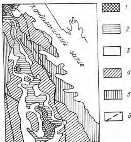
Рис. 2.15. Геологическое строение беломорского метаморфического комплекса [Беломорский комплекс..., 1962].
