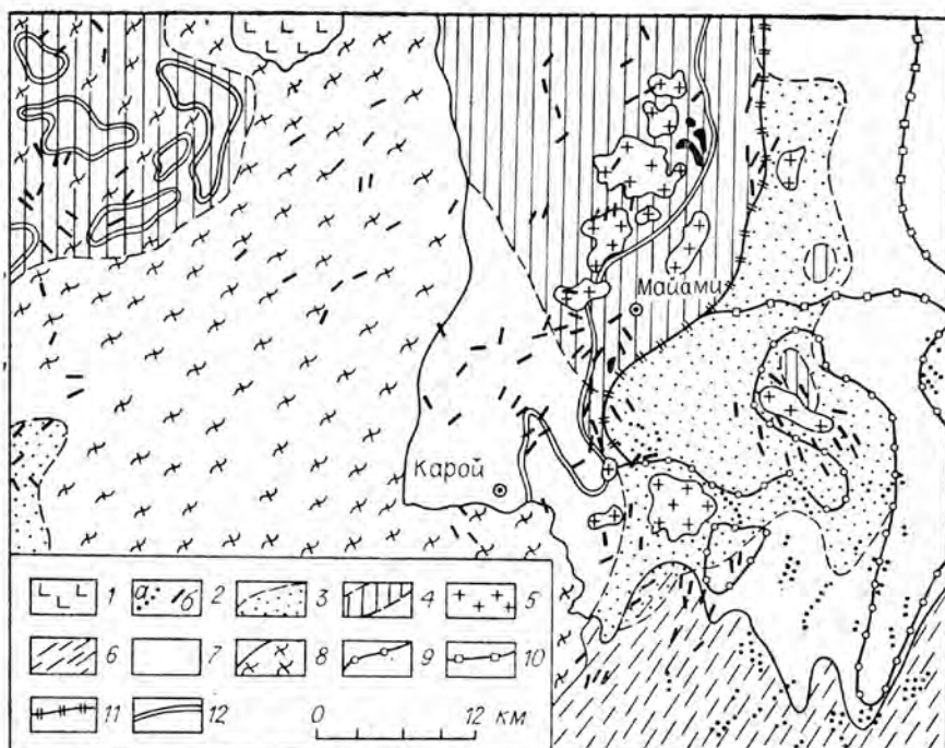
Рис. 2.27. Метаморфическая зональность и размещение мусковитовых пегматитов Майами, Урунге (Африка) [Wiles, 1961].
