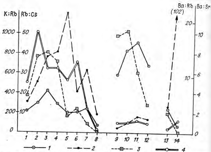
Рис. 8.3. Величины индикаторных отношений щелочных и щелочно-земельных элементов в последовательных структурных разновидностях двуполевошпатовых (1—8) и плагиоклазовых (9—14) пегматитов Мамского пояса. 1 — K/Rb; 2 — Rb/Cs; 3 — Ba/Rb; 4 — Ba/Sr. Номера разновидностей соответствуют номерам средних величин в табл. 8.1.
