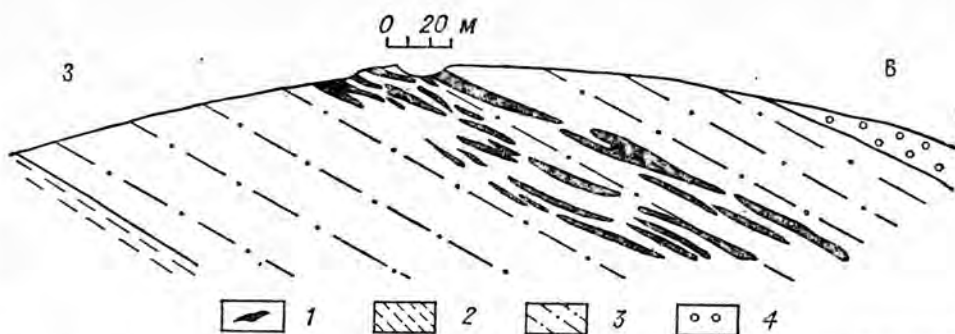
Рис. 4.5. Зона многочисленных плагиоклазовых пегматитовых линз участка Снежный месторождения Луговка.
