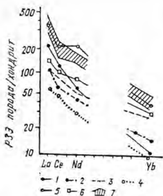
Рис. 2.3. Нормированные содержания главных лантаноидов в породах амфиболитовой фации, Мамско-Бодайбинский пояс, рудник Мал. Северный.
