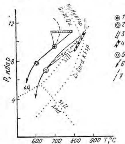
Рис. 2.17. Эволюция термодинамического режима метаморфизма беломорского комплекса по [Салье, Глебовицкий, 1976].
