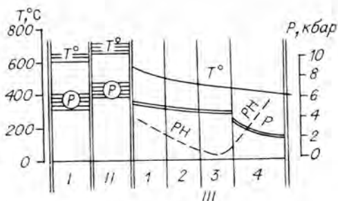
Рис. 6.5. Схема эволюции условий минералообразования в мусковитовых пегматитах на метаморфическом (I), магматическом (II) и послемагматическом (III) этапах.
