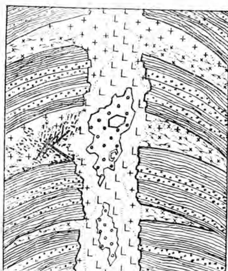
Рис. 4.1. Жила 15 рудника Согдиондон сложной морфологии.
