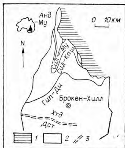
Рис. 2.26. Карта метаморфизма комплекса Уильям, Брокен-Хилл. По [Corbett, Phillips, 1981].
