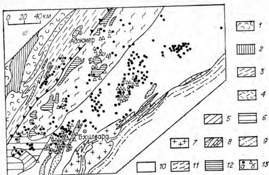
[Рис. 2.25. Геологическое строение и размещение пегматитов в Южной части пояса Раджастхан [Gupta и др., 1985].
