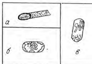
Рис. 6.3. Раскристаллизация стекловатой фазы во включениях.
