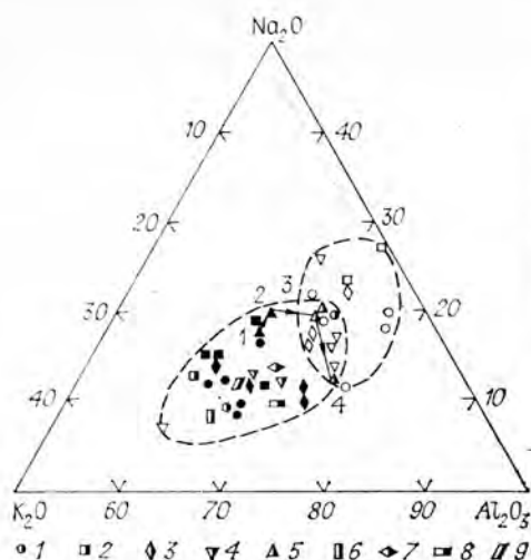
Рис. 8.2. Изменение соотношения алюминия и щелочей в составе двуполевошпатовых (залитые значки), плагиоклазовых (полые) и редкометалльно-мусковитовых (наполовину залитые) пегматитов разных поясов.
