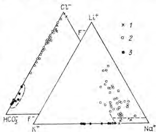
Рис. 10.1. Диаграмма состава водных вытяжек из кварца пегматитов различной специализации.
