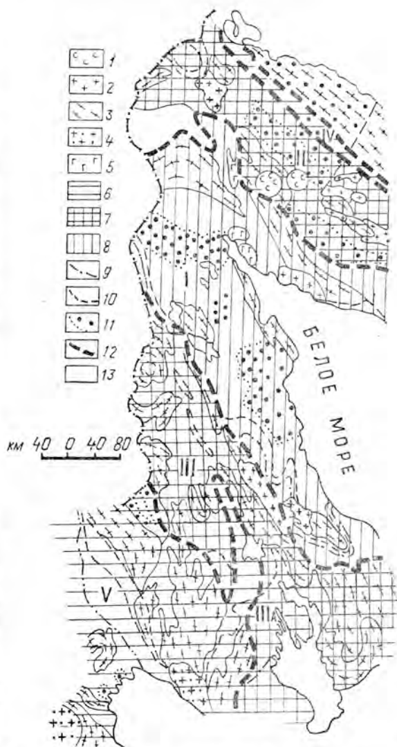
Рис. 2.14. Метаморфические пояса восточной части Балтийского щита по [Метаморфические пояса..., 1975] — с упрощениями.
