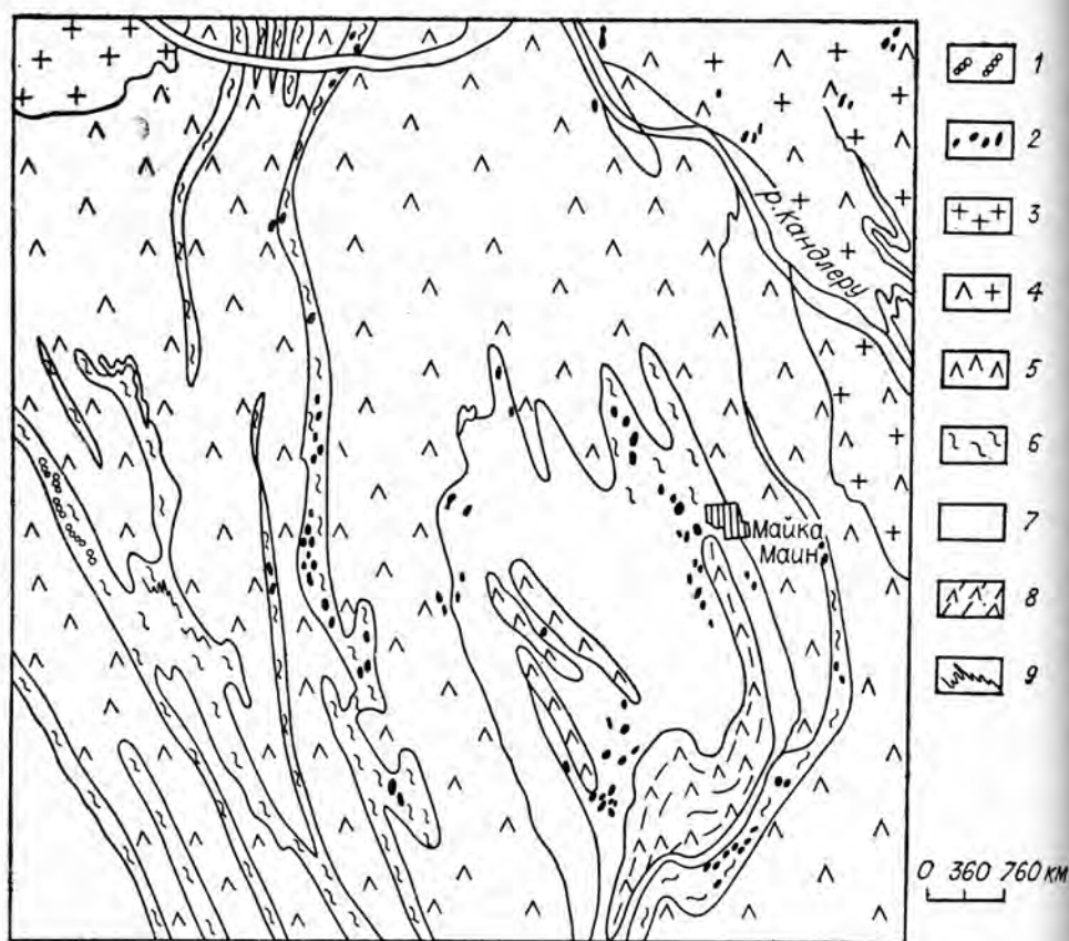
Рис. 2.23. Участок пояса Неллур [Ваву, 1970].
