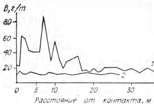
Рис. 9.4. Распределение бора в экзо-контактах двуполевошпатовых слюдоносных жил.
