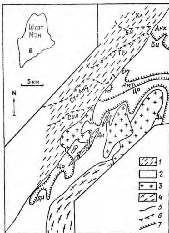
Рис. 2.10. Схема метаморфической зональности центральной части штата Мэн, США [по Ferry, 1982].
