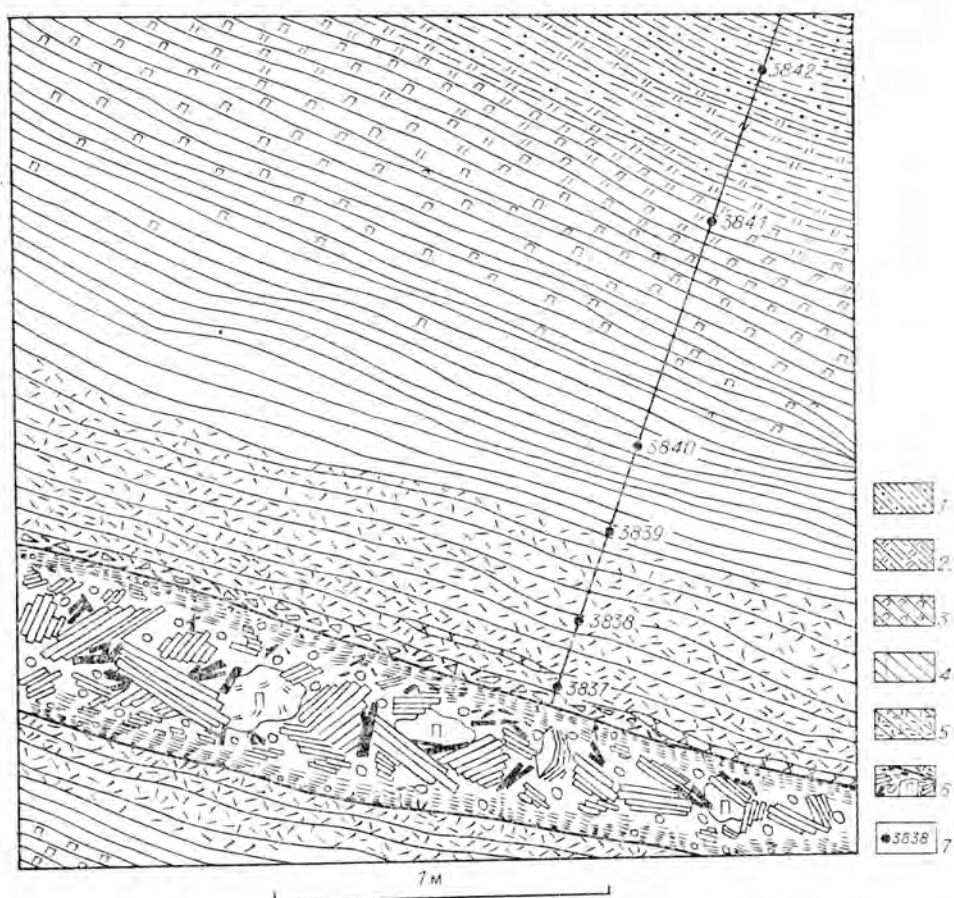
Рис. 9.1. Плагинклез-кварц-мусковитовая жила 99 месторождения Малое Северное [Шмакин, Макрыгина, 1969].
