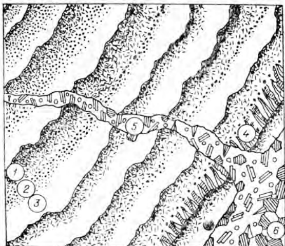
Рис. 4.3. Ритмические структуры в альбит-микроклиновом пегматите Хамардабанского пояса редкометалльно-мусковитовых пегматитов.
