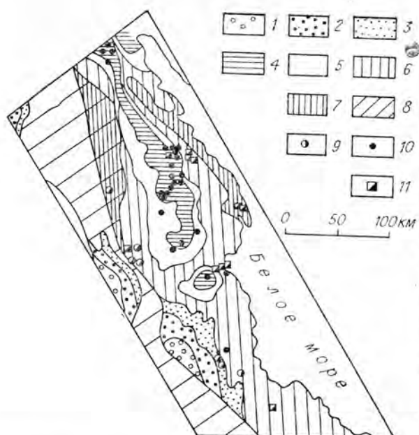
Рис. 2.16. Схема метаморфических фаций в Беломорском блоке и на сочленении его с Центрально-Карельской зоной [Геология..., 1985] и размещение пегматитов различной специализации.
