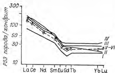
Рис. 2.13. Изменение уровня средних содержаний P3Э в метapelитах последовательных зон метаморфизма (I—IV) и мигматизации (V—VI) хамардабавского комплекса.
