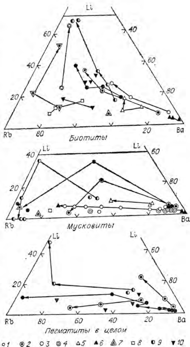
Рис. 8.4. Соотношение Li, Rb и Ba в пегматитах и слюдах различных пегматитовых поясов, последовательных генераций и типов жил.
