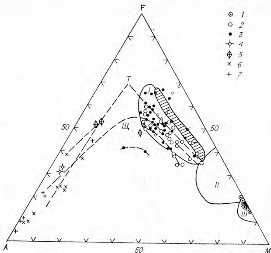
Рис. 2.21. Положение составов пород нюрундуканской серии по диаграмме AFM.
