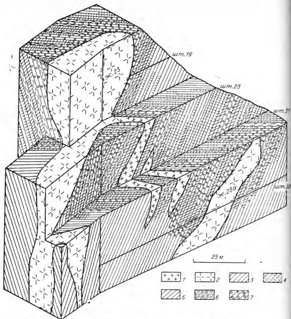
Рис. 9.2. Блок-диаграмма жил 23 и 23а месторождения Малое Северное с экзоконтактовыми ореолами [Шмакин, Макрыгина, 1969].
