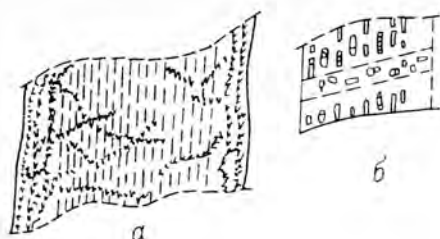
Рис. 6.1. Расположение первичных и первично-вторичных включений в кристалле берилла: а — общий вид расположения включений, б — система первичных включений (вертикальная) пересекается системой вторичных и первично-вторичных включений (горизонтальная).
