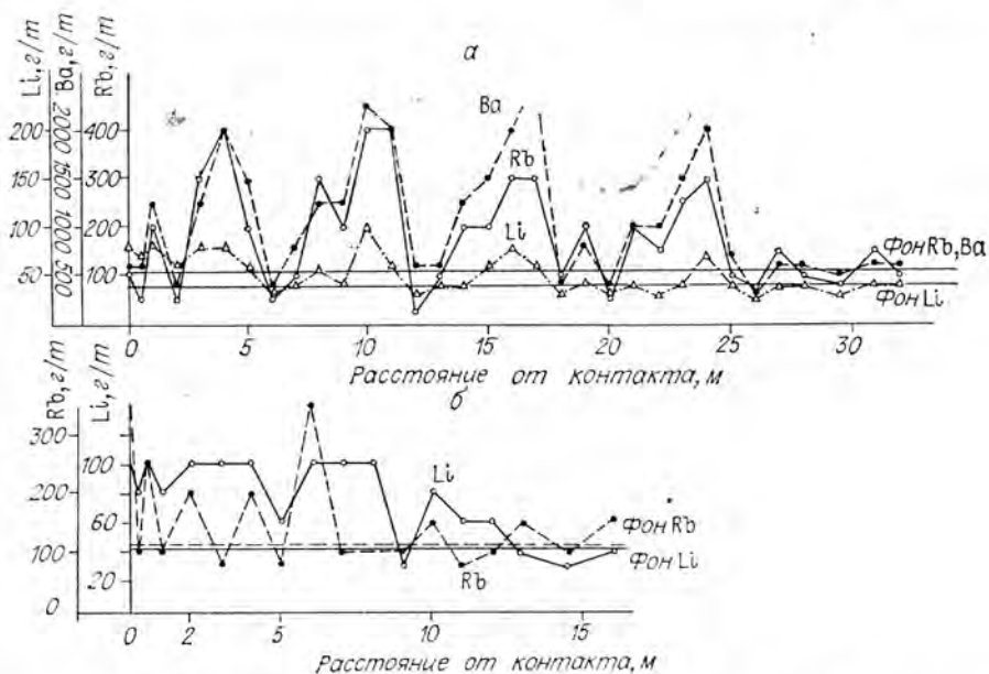
Рис. 9.3. Распределение Li, Rb и Ba в экзоконтакте жилы 16.
