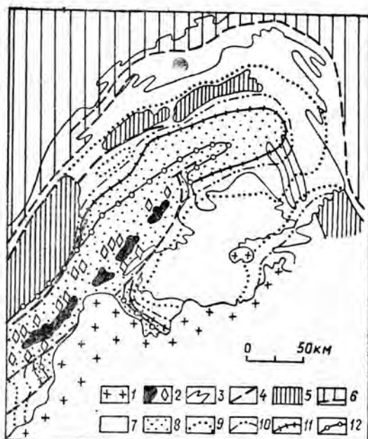
Рис. 2.1. Карта метаморфической зональности Патомского нагорья [по Б. В. Петрову, В. А. Макрыгиной, 1975 с дополнениями].
