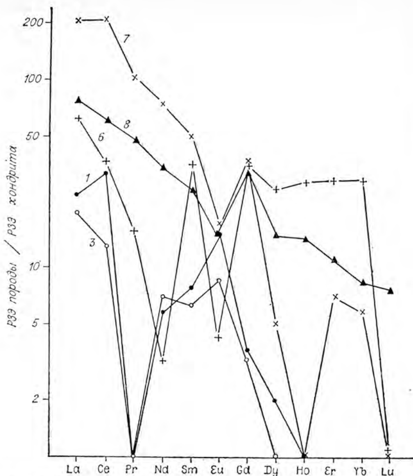
Рис. 3.6. Нормированное распределение редкоземельных элементов в гранитах. Номера на графике соответствуют номерам в табл. 3.6.
