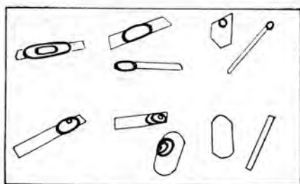
Рис. 6.2. Зарисовки различных соотношений фаз во включениях минералообразующей среды в берилле.
