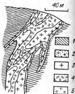
Рис. 4.2. Штокобразное пегматитовое тело. Жила 23, месторождение Малое Северное, Мамский пояс.
