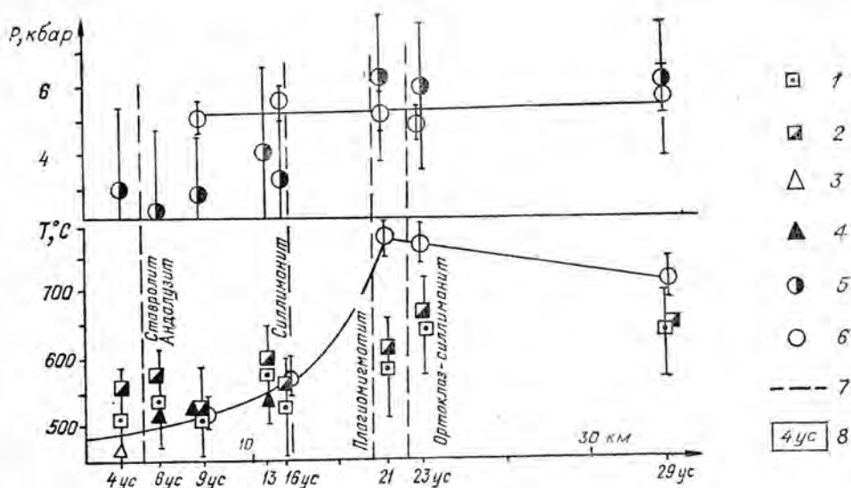
Рис. 2.12. Эволюция условий метаморфизма и гранитизации хамардабанского комплекса.
