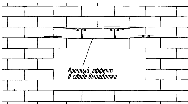
Рис. 8.9. Зашемление блоков в кровле выработки
