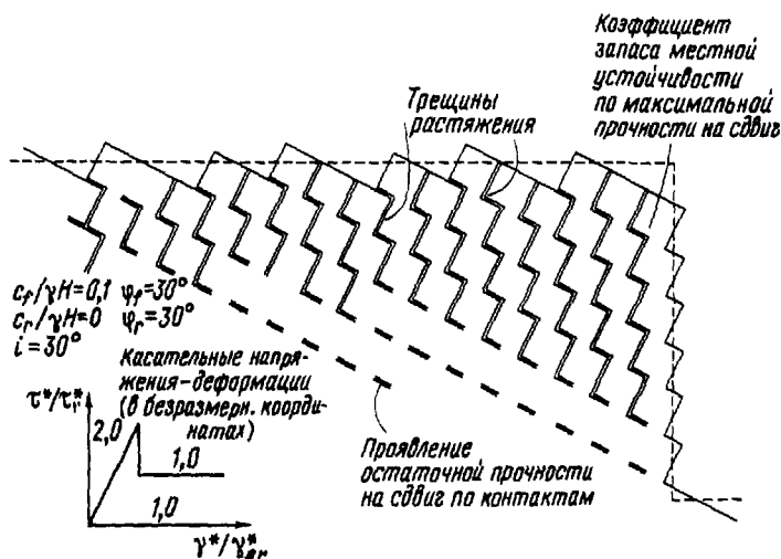
Рис. 12.22. Рисунок распределения трещины растяжения и мобилизация прочности на сдвиг хрупких трещин в откосе блоковой структуры.
