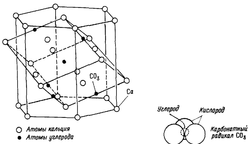
Рис. 1.16. Сложный карбонатиый ион и кристаллическая структура кальцита.
