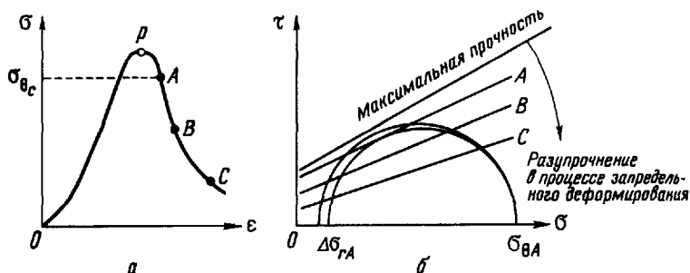
Рис. 14.7. Снижение прочности скальной породы в результате перераспределения усилий в массиве (подробнее см. в тексте). а — кривая напряжения — деформация; б — диаграмма Мора с несколькими огибающими, соответствующими различным фазам снижения прочности в процессе запредельного деформирования.
