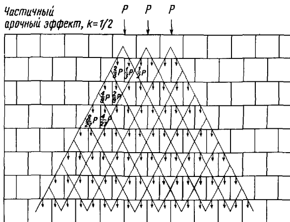
Рис. 15.13. Распределение напряжений в зернистой среде [10]
