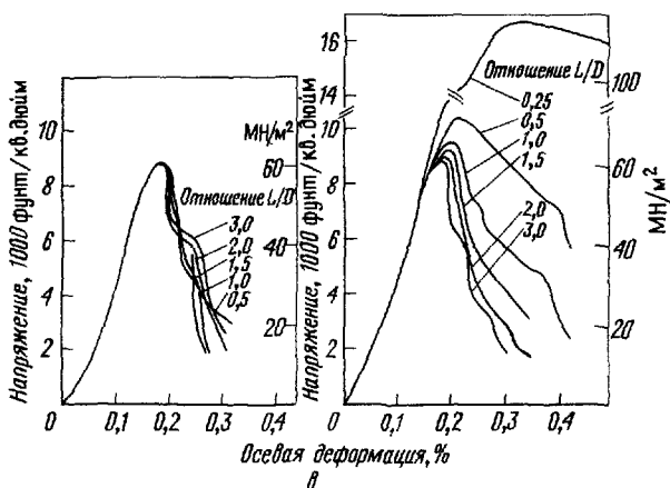
Рис. 5.10. Результаты испытаний мрамора на одноосное сжатие [7]. а — щеточные опорные плиты для испытания образцов диаметром 2 дюйма (51 мм) при нагрузке до 10 000 фунт/кв. дюйм (70 МН/м 2 ); б — изменение прочности на одноосное сжатие \sigma_c при изменении отношения L/D ; в — влияние отношения L/D на кривые напряжений — деформаций.
