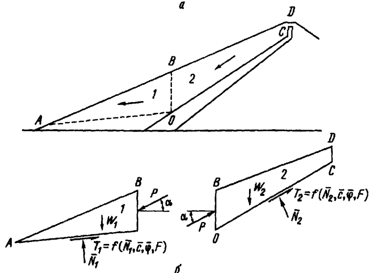
Рис. 12.19. Анализ устойчивости методом равновесия клиновых блоков. а — модель обрушения откоса плотны с глиняным ядром; б — блоки и действующие на них силы [17].
