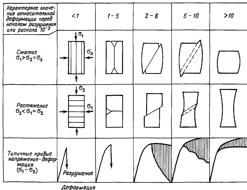
Рис. 4.13. Различные виды разрушения (переход от хрупкости к пластичности) при трехосиных испытаниях (схематизировано [8]).
