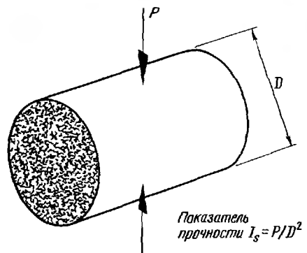
Рис. 9.6. Основные параметры в опыте с точечным приложением нагрузки.
