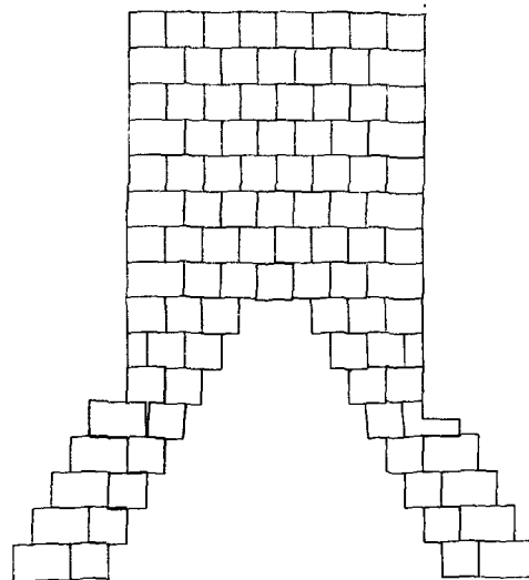
Рис. 15.7. Туннель в ступенчатой блочной структуре. Случай 1 — обрушение первоначального свода [5]
