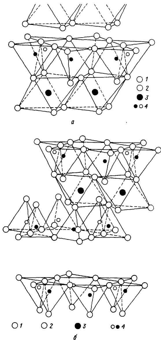
Рис. 1.21. Структура глинистых минералов. a — каолин: 1 — кислород, 2 — ион гидроксила, 3 — алюминий, 4 — кремний; б — монтмориллонит: 1 — кислород, 2 — ион гидроксила, 3 — алюминий, железо, магний, 4 — кремний, спорадически алюминий.
