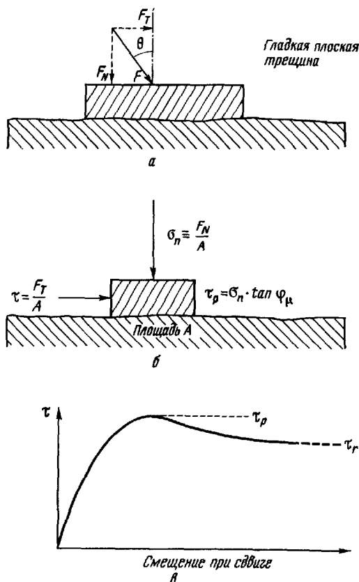
Рис. 7.5. Схема нагружения (а), аналитическое описание (б) и зависимость напряжения сдвига — деформация сдвига (в) для гладкой плоской трещины.
