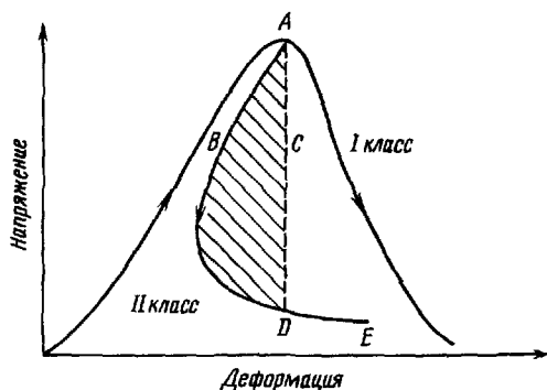
Рис. 6.20. Типы запредельного поведения скальных пород [31].
