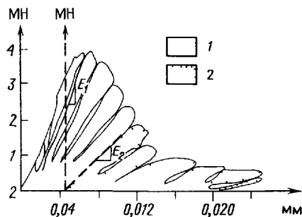
Рис. 4.21. Иллюстрация сходства поведения ненарушенной породы и скального массива на примере полной кривой нагрузка – деформация «ненарушенной» породы [20] 1 – ненарушенная порода, 2 – скальный массив
