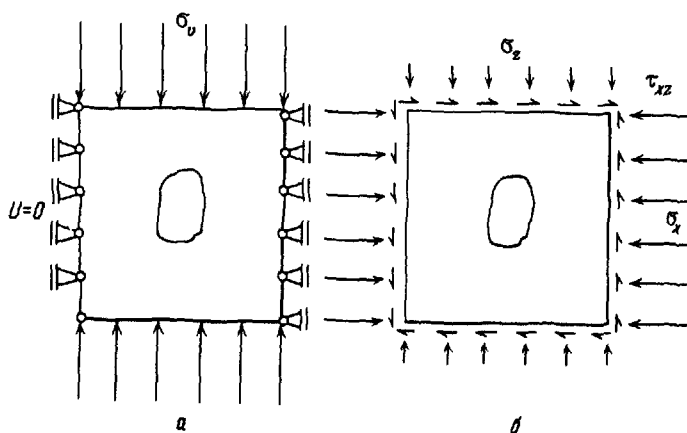
Рис. 2.3. Два взаимоисключающих вида граничных условий геомеханической модели подземной выработки. а – классическое решение с вертикальной нагрузкой и отсутствием возможности горизонтальных смещений; б – более прогрессивное решение с естественными напряжениями, действующими по всем граничным поверхностям модели.
