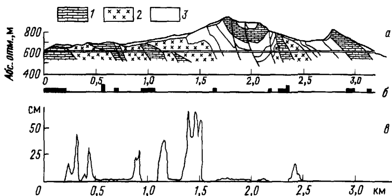
Рис. 9.1. Бельпенский туннель (Швейцарская Юра) а — продольный геологический профиль, б — водопритоки (в основном в известняках), в — пучение обратного свода (преимущественно в загипсованных породах) 1 — известняки, 2 — гипсоносные слои, 3 — другие литологические разности
