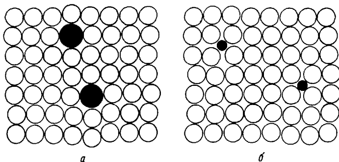
Рис. 1.22. Замещающие ( a ) и внедренные ( б ) атомы в твердых растворах.
