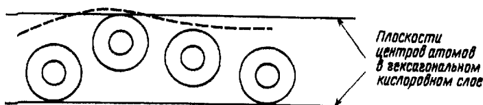
Рис. 1.24. Гипотетический механизм дислокаций в слюде.
