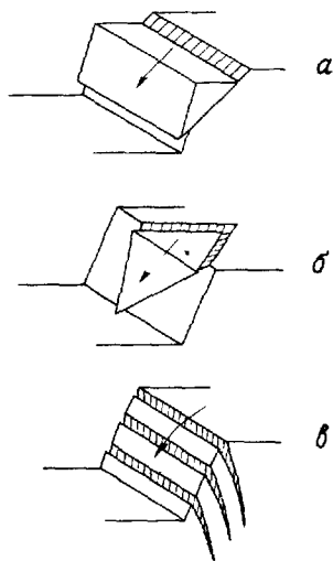
Рис 9 15. Основные типы разрушения скальных откосов по Хуку и др [15] а — плоский сдвиг в хорошо упорядоченных структурах как например кровельный сланец б — клиновидное разрушение по двум нарушениям сплошности, в — опрокидывание в твердых породах с крутопадающими нарушениями сплошности
