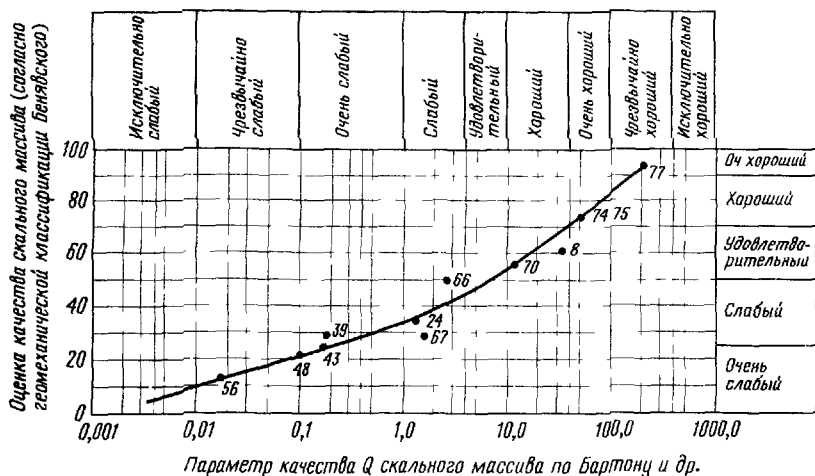
Рис. 9.13. Сопоставление качеств скальных массивов, определяемых по Бартону и др. и по Бенявскому соответственно (см. [25]) Цифры на кривой соответствуют нумерации в табл. 8 и 9 в работе Бартона и др. [3]
