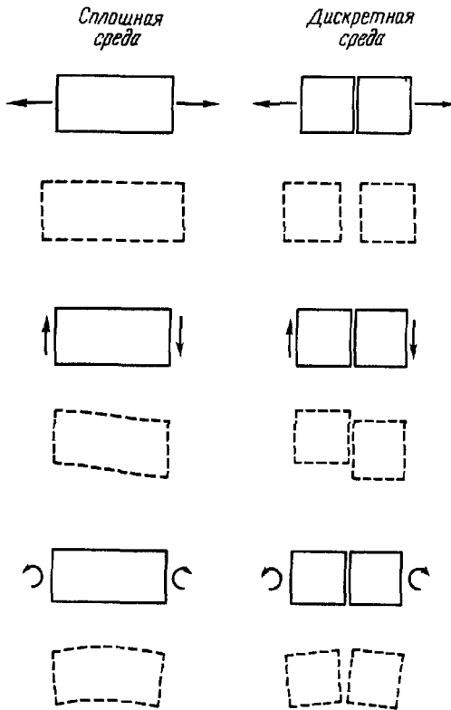
Рис. 12.1. Виды деформаций.
