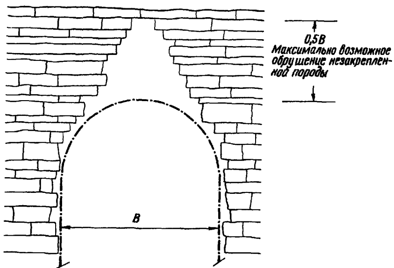
Рис. 15.2. Вывал в горизонтально-слоистом массиве [9].
