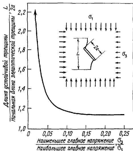
Рис. 5.2. Отношение длины устойчивой трещины к длине эллиптической трещины в зависимости от соотношения сжимающих напряжений.
