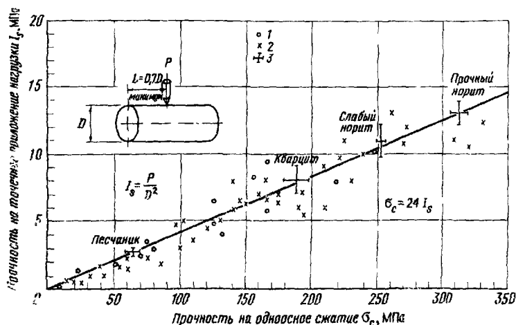
Рис. 9.7. Зависимость между показателем прочности на точечное приложение нагрузки I_s и прочностью на одноосное сжатие [5]. Источники данных: 1 — Broch and Franklin, 1972; 2 — D'Andrea et al., 1965; 3 — Беньявский [5].
