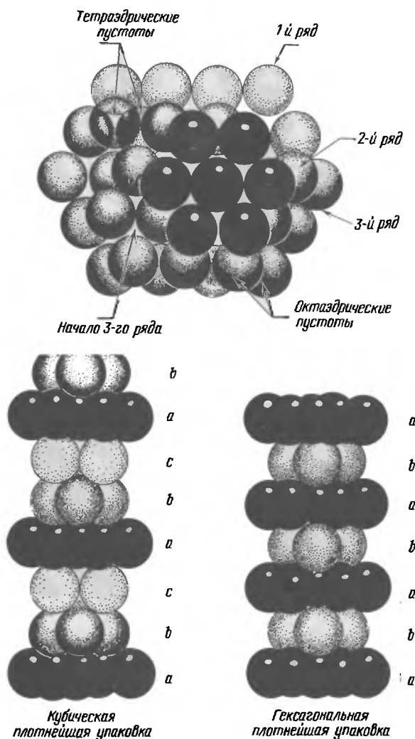
Рис. 1.7. Разновидности гексагональной плотнейшей упаковки.
