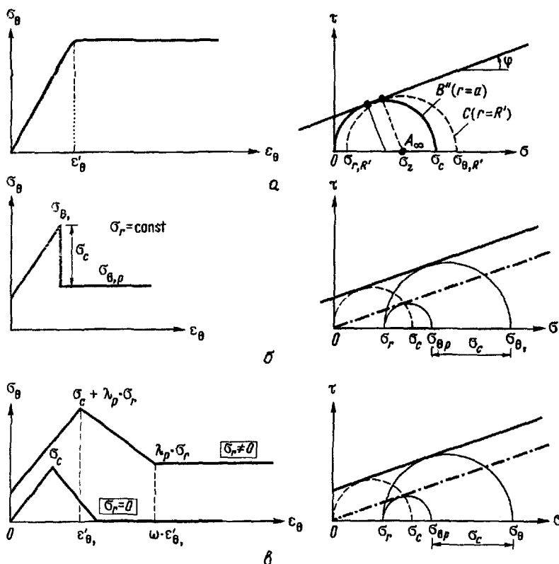
Рис. 14.2. Кривые напряжение – деформация (слева) и огнищающие Мога (справа), соответствующие трем случаям, рассмотренным в разд. 14.2–14.4. а – линейно-упругое идеально пластическое поведение; б – разупрочняющийся материал с бесконечной хрупкостью; в – материал с конечной ненулевой хрупкостью.
