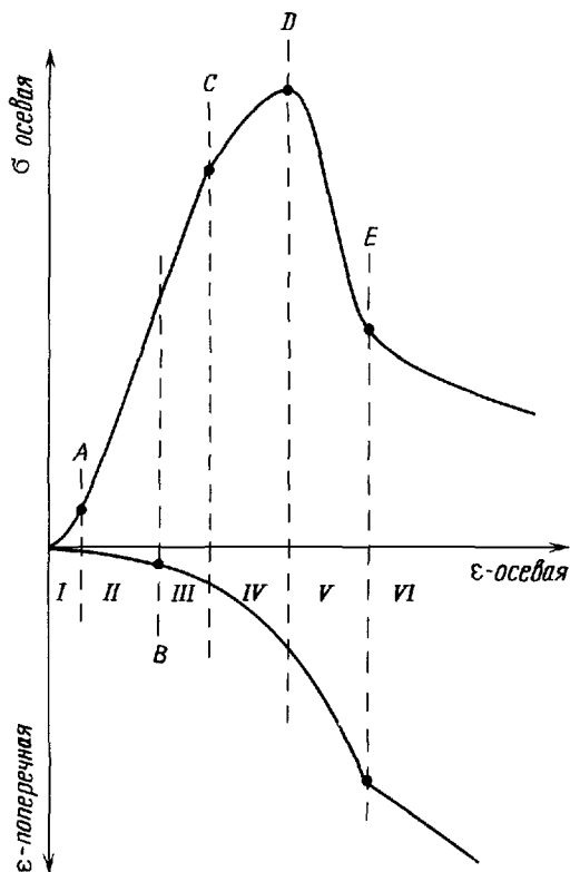
Рис. 4.8. Схематизированные кривые осевое напряжение — осевая деформация и осевая деформация — поперечная деформация с разделением на шесть участков типичных по характеру трещинообразования [10]
