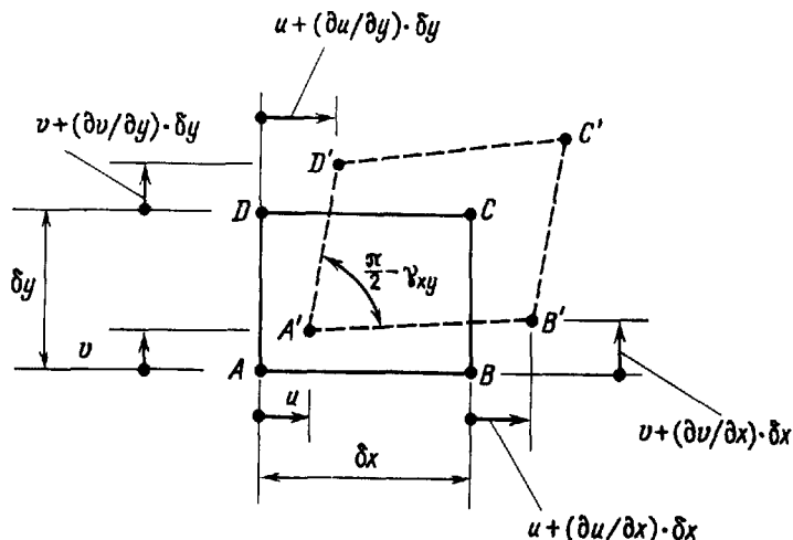
Рис. 3.2. Деформирование элемента.
