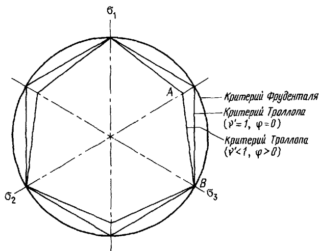
Рис. 5.7. Критерии Фруденталля и Троллопа в пространстве главных напряжений.
