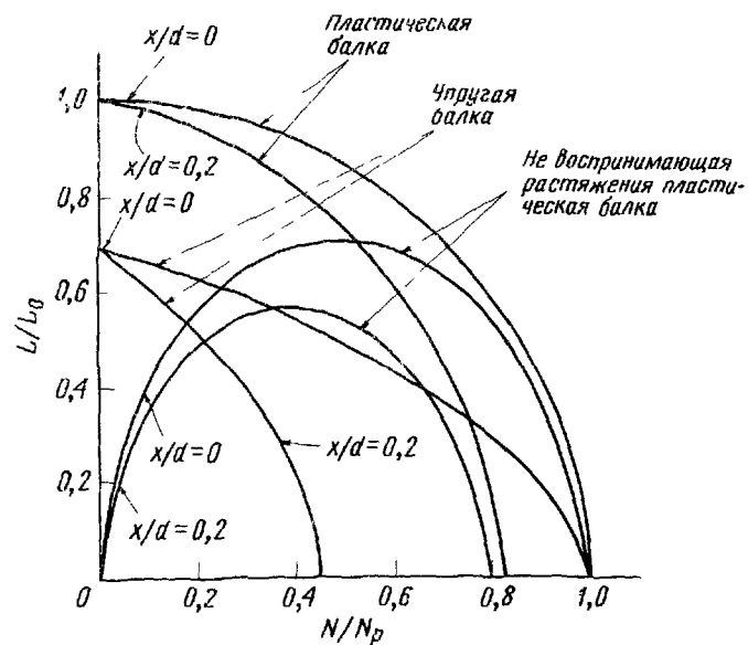
Рис. 15.6. Соотношение между величинами мгновенноустойчивого пролета и осевой нагрузкой для жесткопластической, упругой и не воспринимающей растяжения пластической балок [12]
