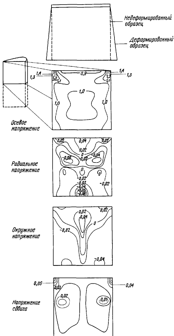
Рис. 6.12. Анализ напряженного состояния однооснонагруженного образца в условиях совершенного заземления торцевых поверхностей [25].
