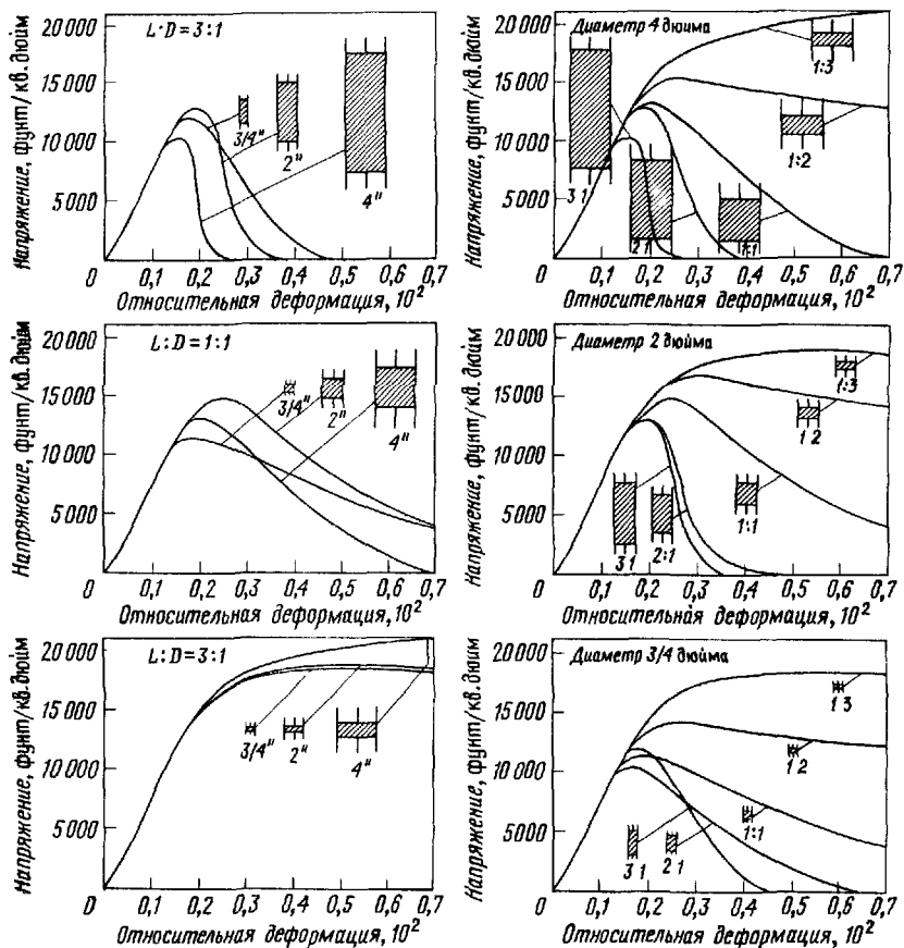
Рис. 6.10. Влияние размера и формы образца мрамора на характер кривой напряжение — деформация при одноосном сжатии [17]
