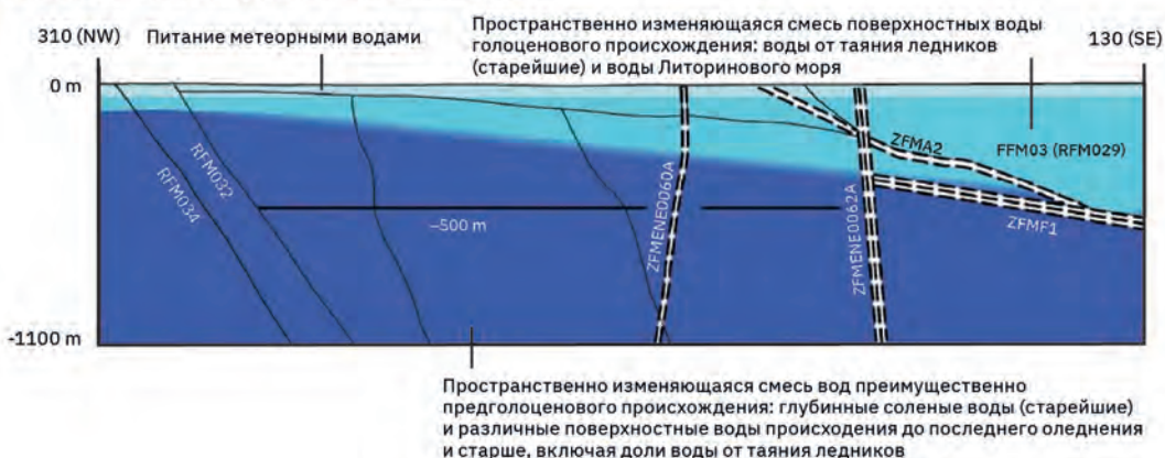
Рис. 2.9. Три концептуальные модели, используемые для оценки надежности подземного хранилища ОЯТ на участке Форсмарк [51]
