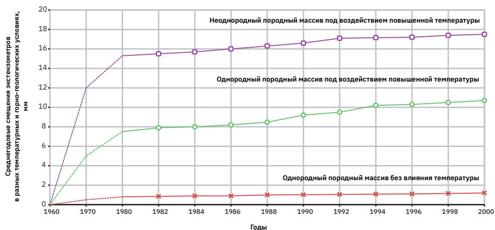
Рис. 4.28. Графики смещения контура выработок [t] в различных горно-геологических и температурных условиях за период 1980–2000 гг.
