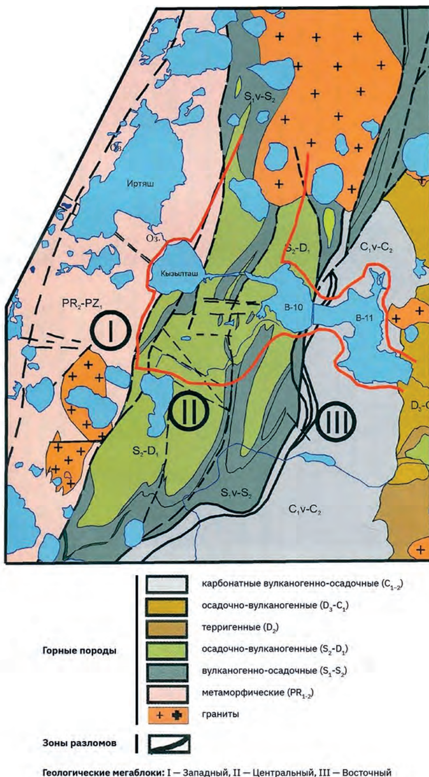
Рис. 3.5. Геологическое строение района ПО «Маяк» (исходный масштаб 1:100 000) [19]
