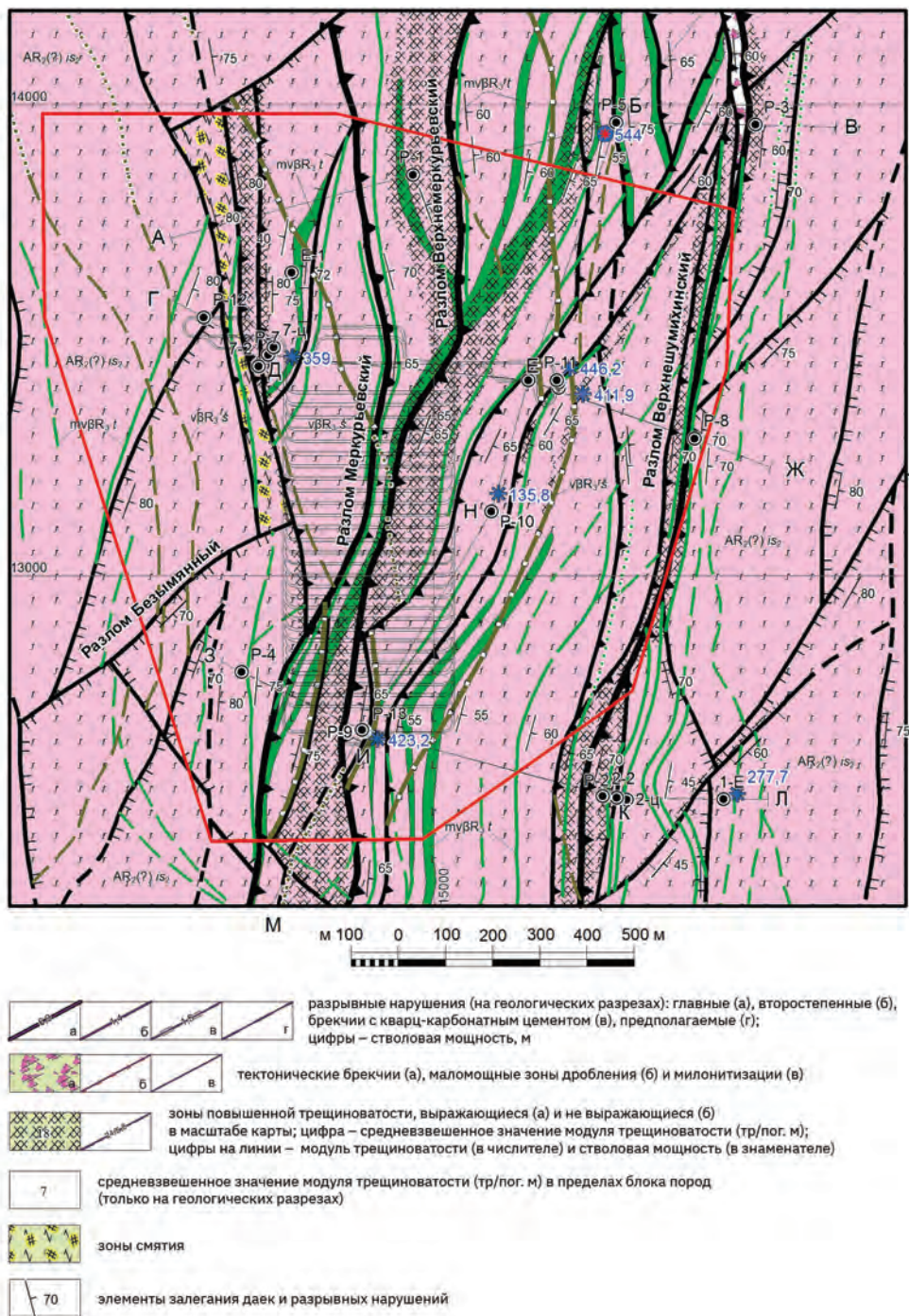
Рис. 5.19. Геологическая карта дочетвертичных образований участка (О. А. Морозов)
