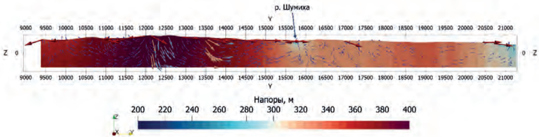
Рис. 5.42. Модельный разрез с юга на север через русло р. Шумихи
