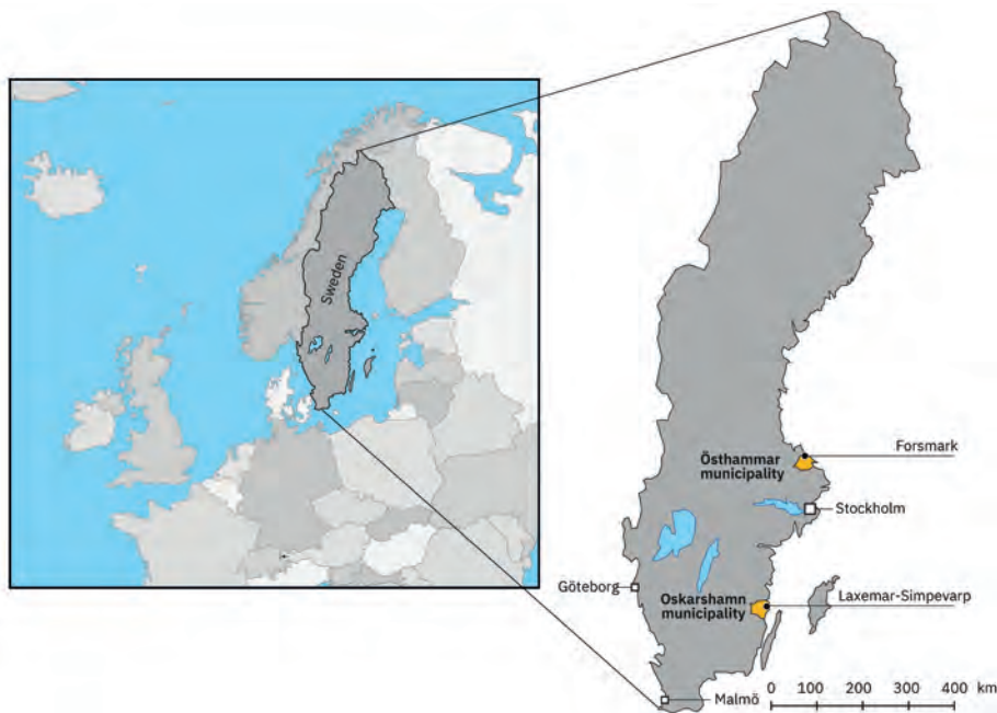
Рис. 2.5. Районы в Швеции, исследованные под окончательное хранилище ОЯТ (показаны желтым цветом). Место Форсмарк было в итоге признано предпочтительным вариантом [51, 86]
