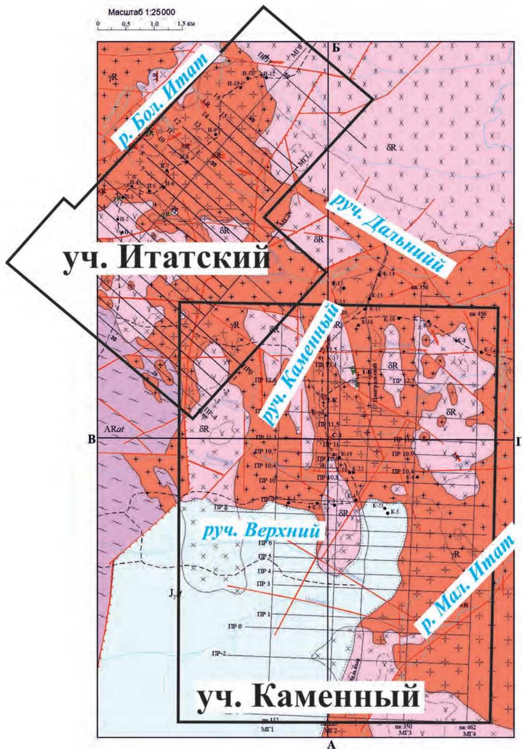
Рис. 4.6. Предварительная геологическая карта дочетвертичных образований участков Итатский и Каменный масштаба 1:25 000 (составили В. М. Даценко, В. А. Ключев и Э. Н. Линд, 2000 г.) [5]
