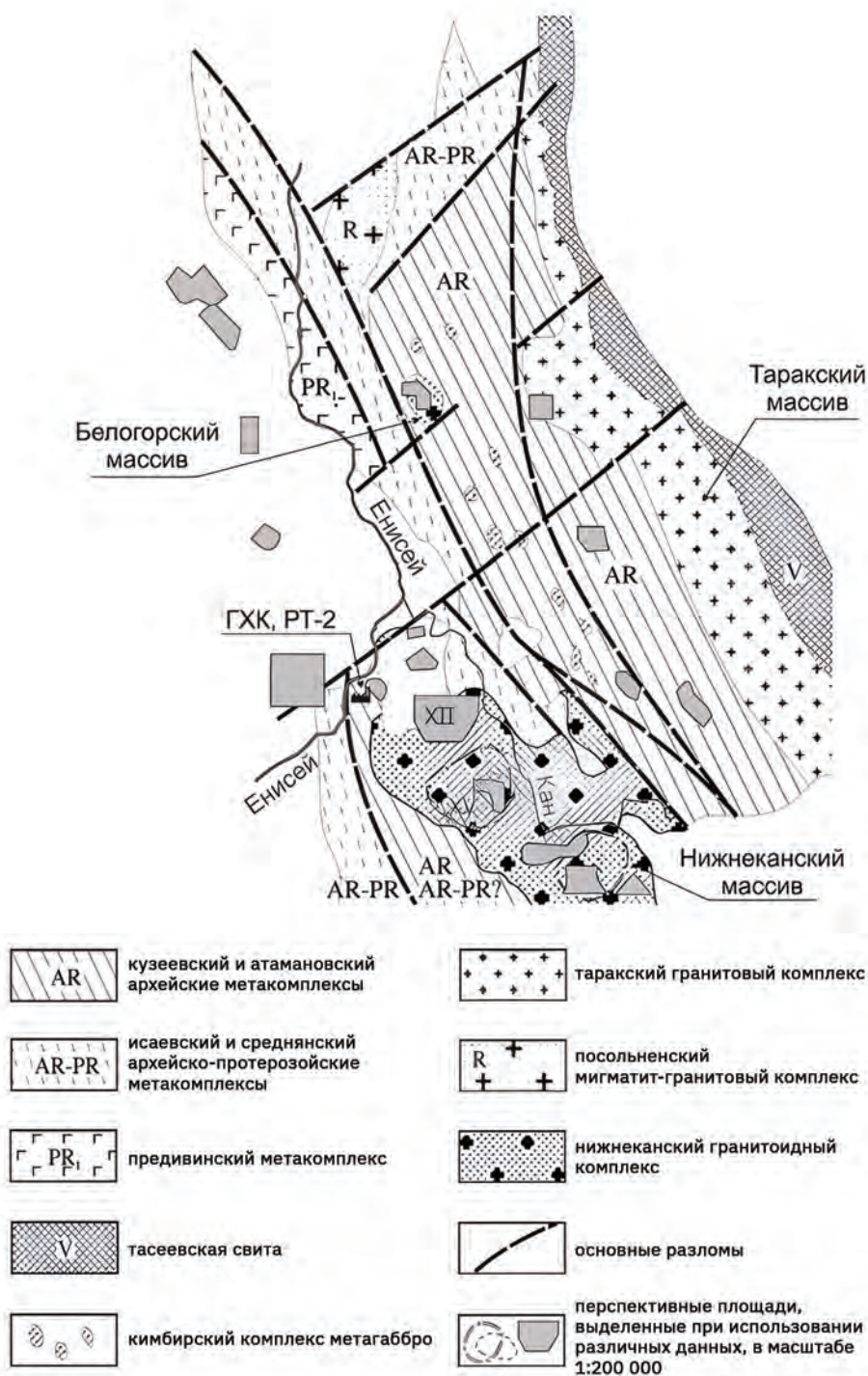
Рис. 4.2. Докембрийские формации южной части Енисейского кряжа. Масштаб 1:1 000 000 и предварительная (1993 г.) схема размещения перспективных площадей [2]
