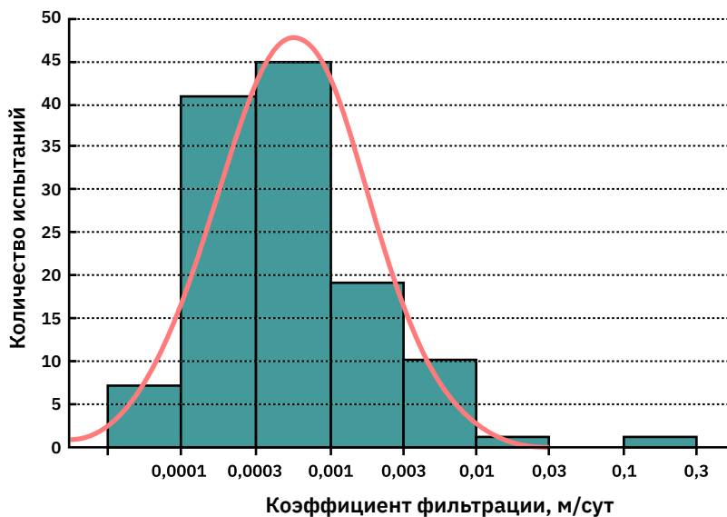
Рис. 5.28. Гистограмма распределения коэффициента фильтрации [31, 32]
