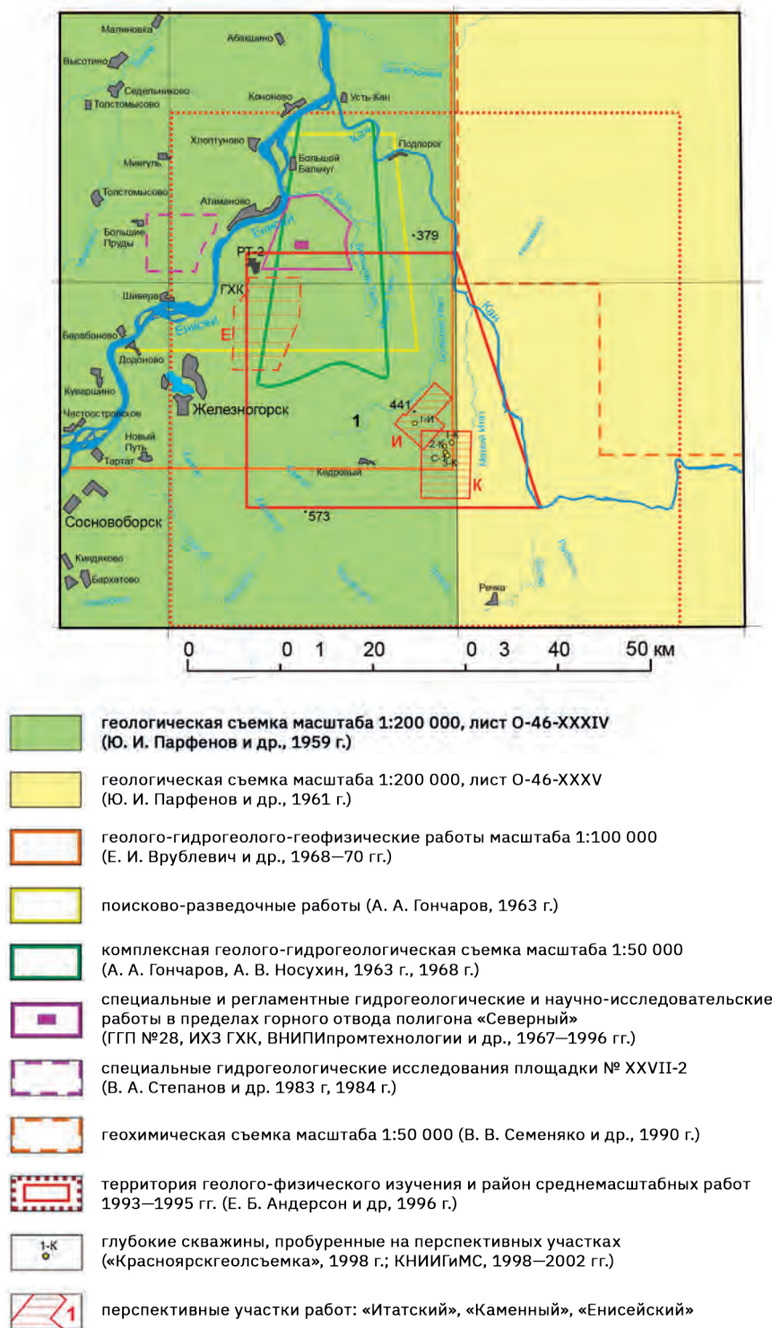
Рис. 4.7. Картограмма геолого-гидрогеологической изученности территорий, прилегающих к северу Нижнеканского массива гранитоидов. Масштаб 1:500 000 [о]
