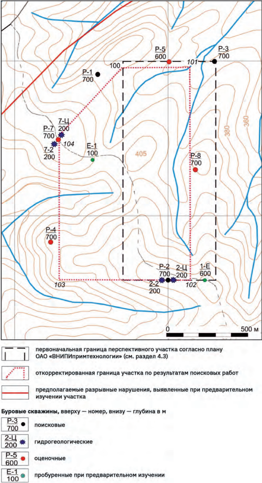
Рис. 5.2. Корректировка границ участка Енисейский по результатам поисковых работ
