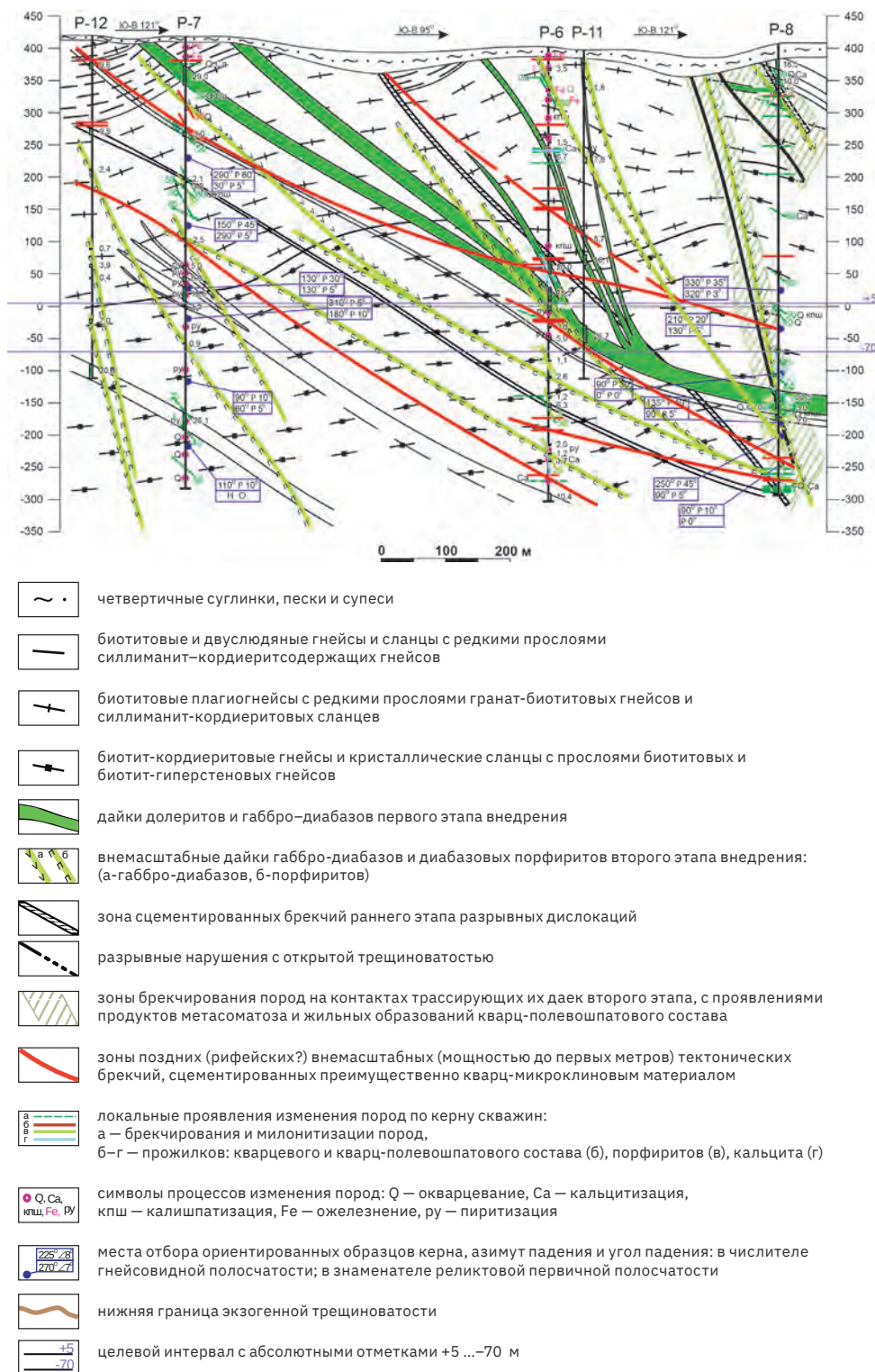
Рис. 5.7. Субширотный геологический разрез через Енисейский участок (составил К. А. Заблоцкий [14])
