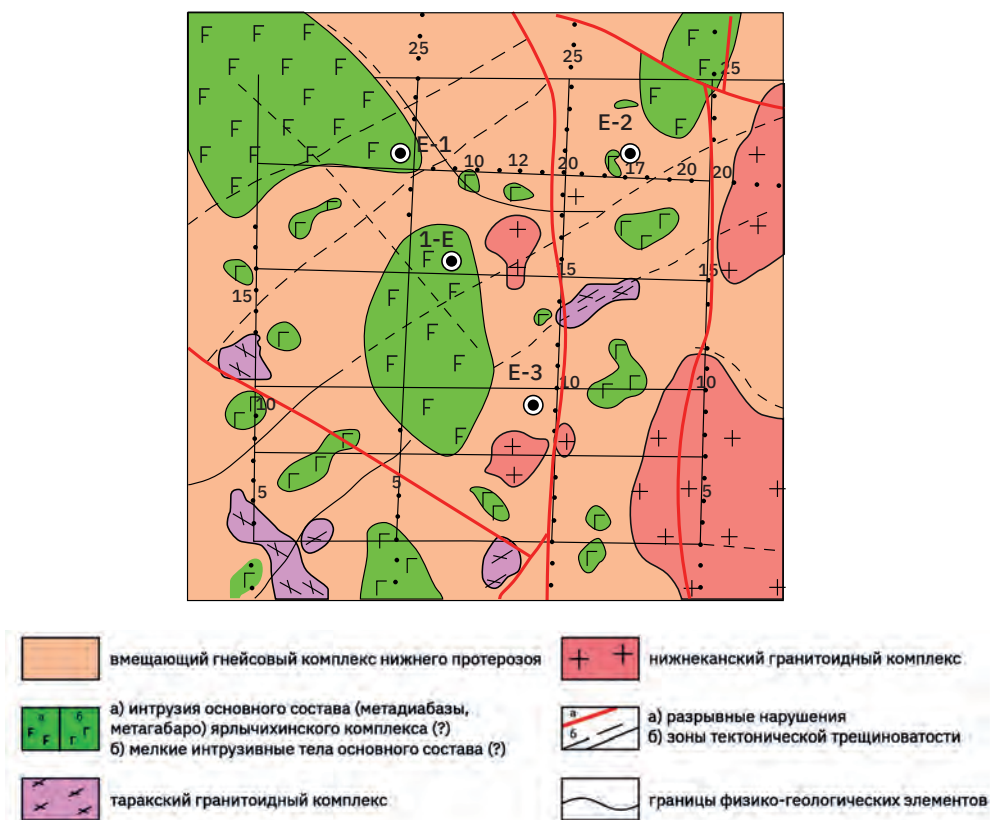
Рис. 4.19. Геологическая карта на срезе глубин 300–500 м
