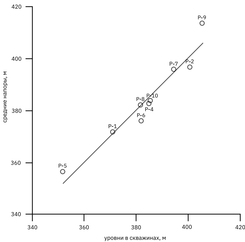
Рис. 5.32. Сопоставление абсолютных значений уровней в скважинах на 29.01.2013 со средними значениями напоров h_{cp} , полученных при пакерных исследованиях
