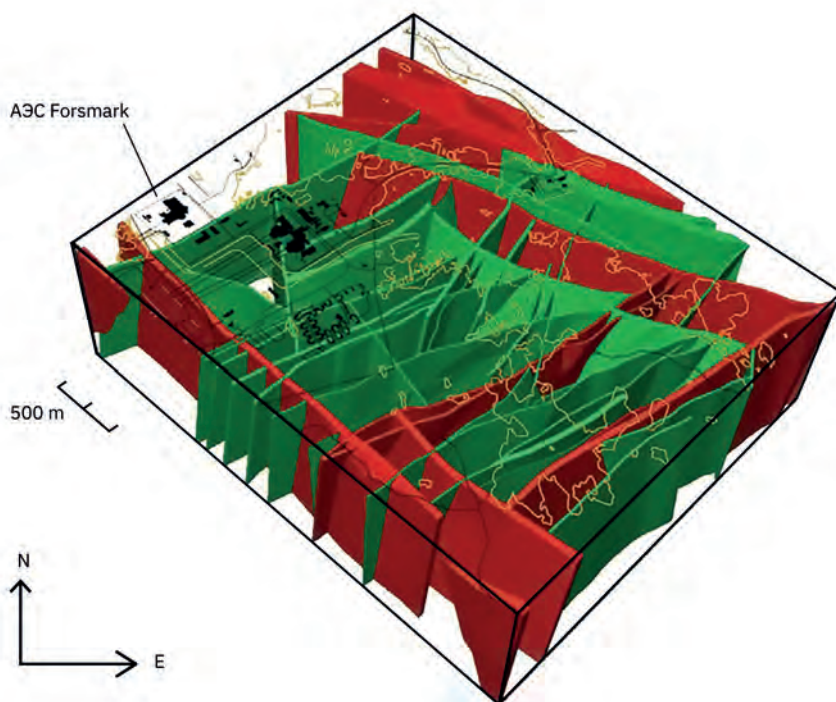
Рис. 2.10. Трехмерная модель, которая показывает все вертикальные и крутопадающие зоны в объеме локальной области [51, 86]
