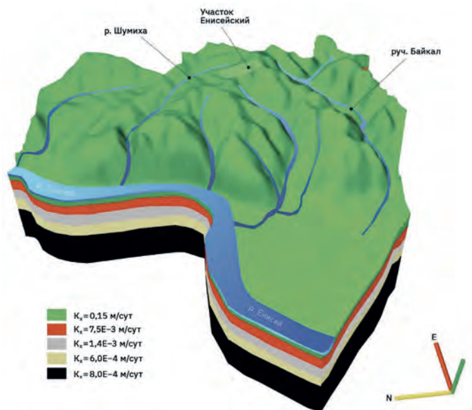
Рис. 5.53. 3D-представление модельной области
