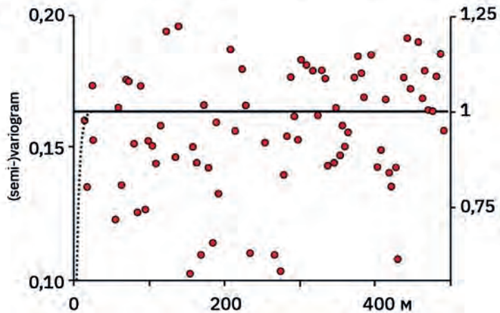
Рис. 5.47. Индикаторные вариограммы главной системы водопроводящих зон, построенные по трем направлениям
