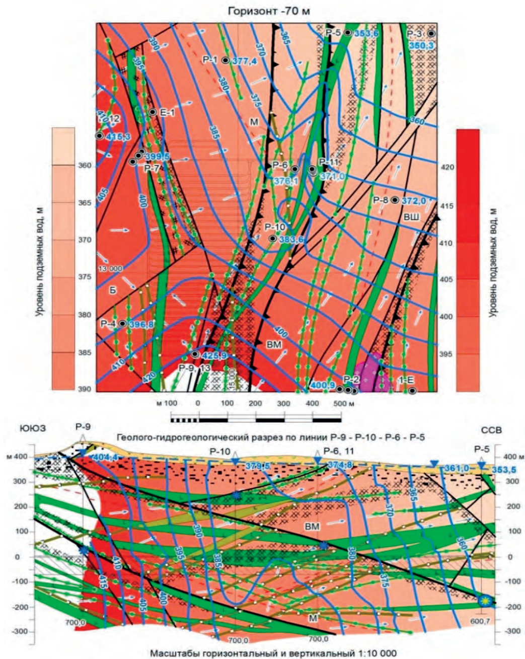
Рис. 5.33. Геолого-гидрогеологическая карта для горизонта -70 м и геолого-гидрогеологический разрез по линии скв. Р-9 – Р-10 – Р-6 – Р-5.
