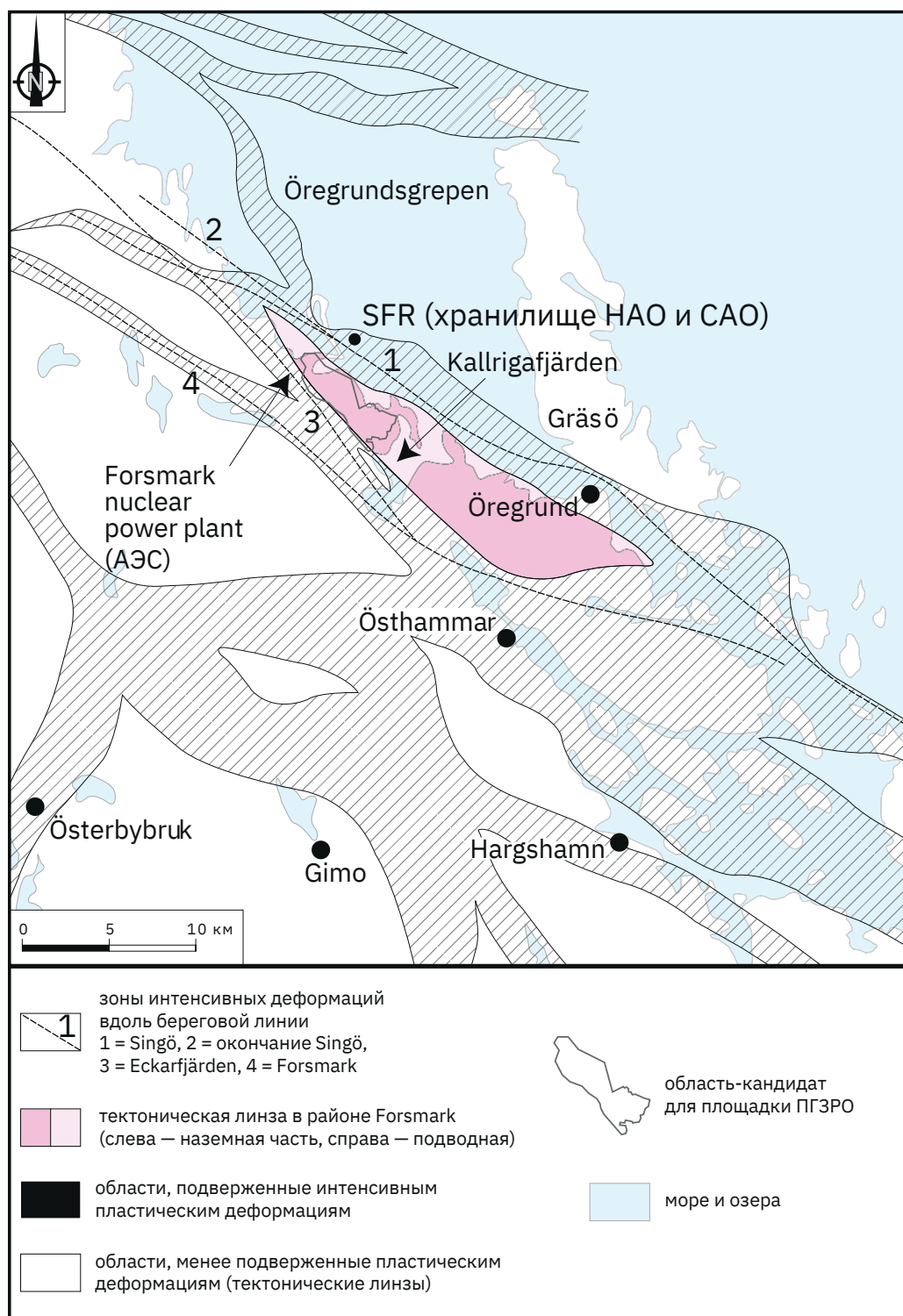
Рис. 2.6. Тектонически слабо деформированные линзы пород района Форсмарк и зоны, подверженные интенсивным пластическим деформациям [51, 86]
