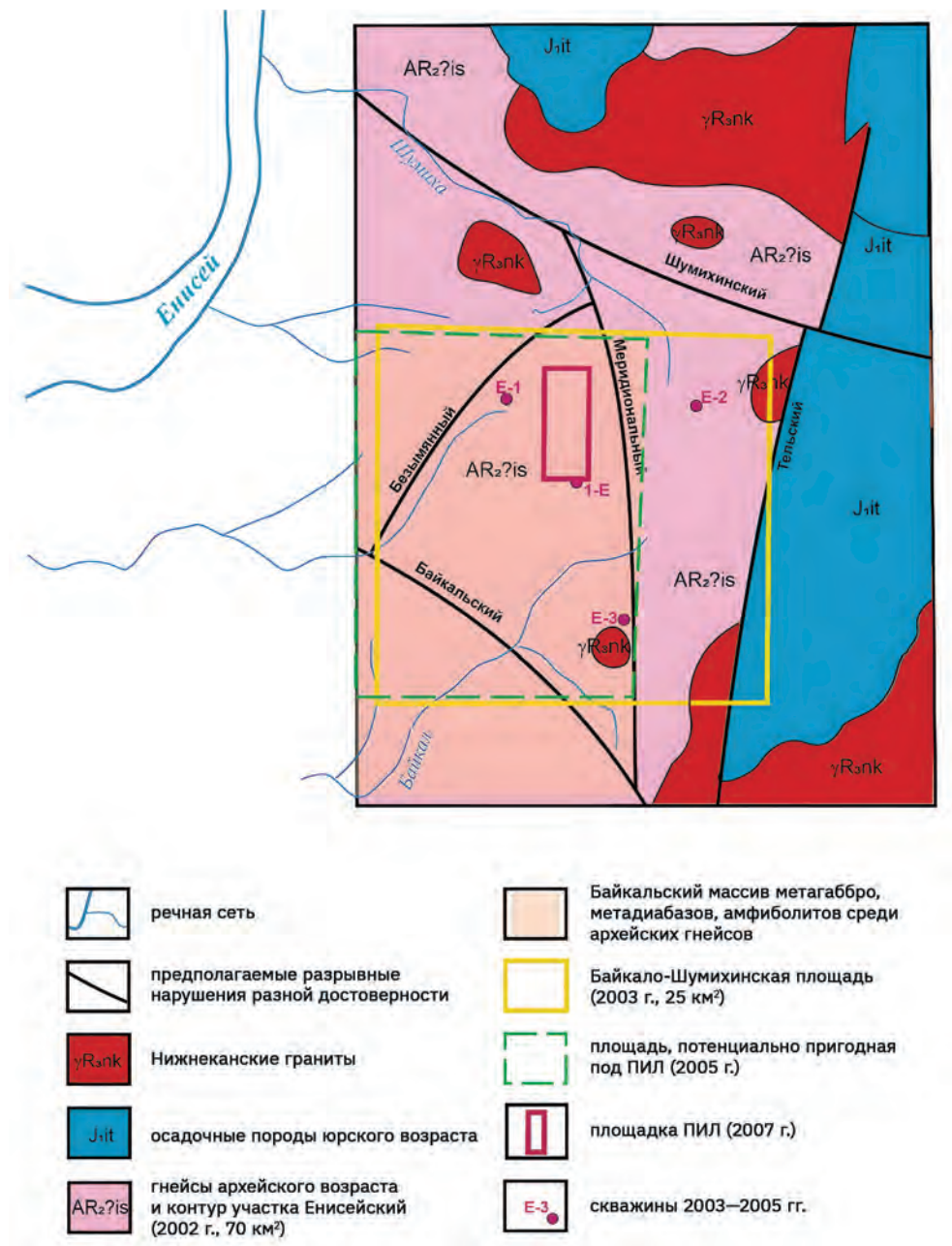
Рис. 4.4. Схема последовательного сокращения территории участка Енисейский в ходе предварительных исследований (по разным источникам)
