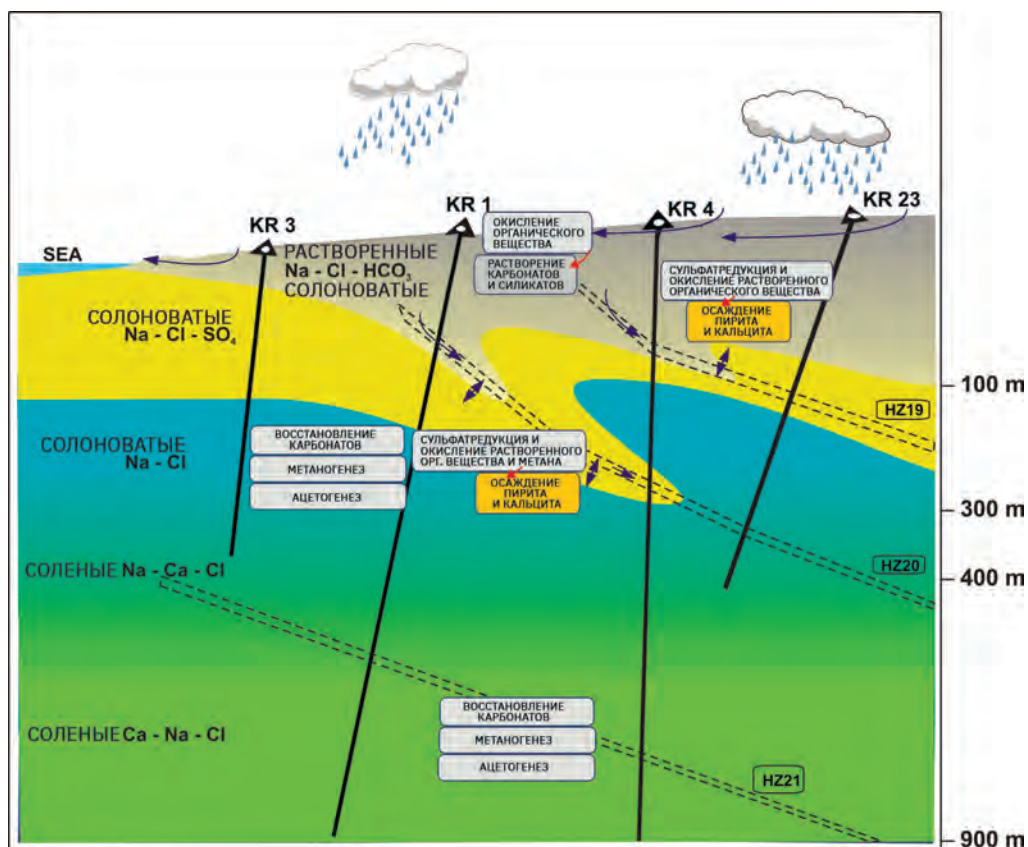
Рис. 2.17. Иллюстративная гидрогеохимическая модель участка Олкилуото в системе водопроводящих трещин (но не в матрице горных пород) [87] Изменения в цвете указывают на изменения водного типа. Тонкие стрелки представляют направления потока. Скругленные прямоугольники — основные источники и поглотители, влияющие на pH и окислительно-восстановительные условия
