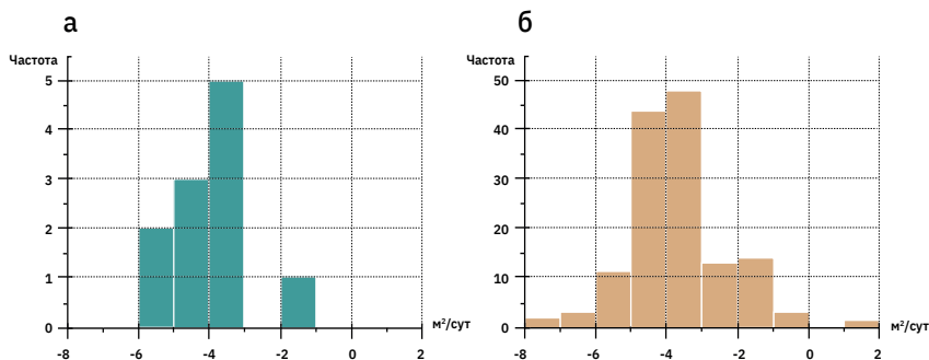
Рис. 5.45. Частотные диаграммы проводимостей 50-метровых интервалов: а — трассирующих разрывных нарушений ВШ, ВМ и М, выделенных по геологическим признакам; б — всех выполненных поинтервальных опытно-фильтрационных опробований
