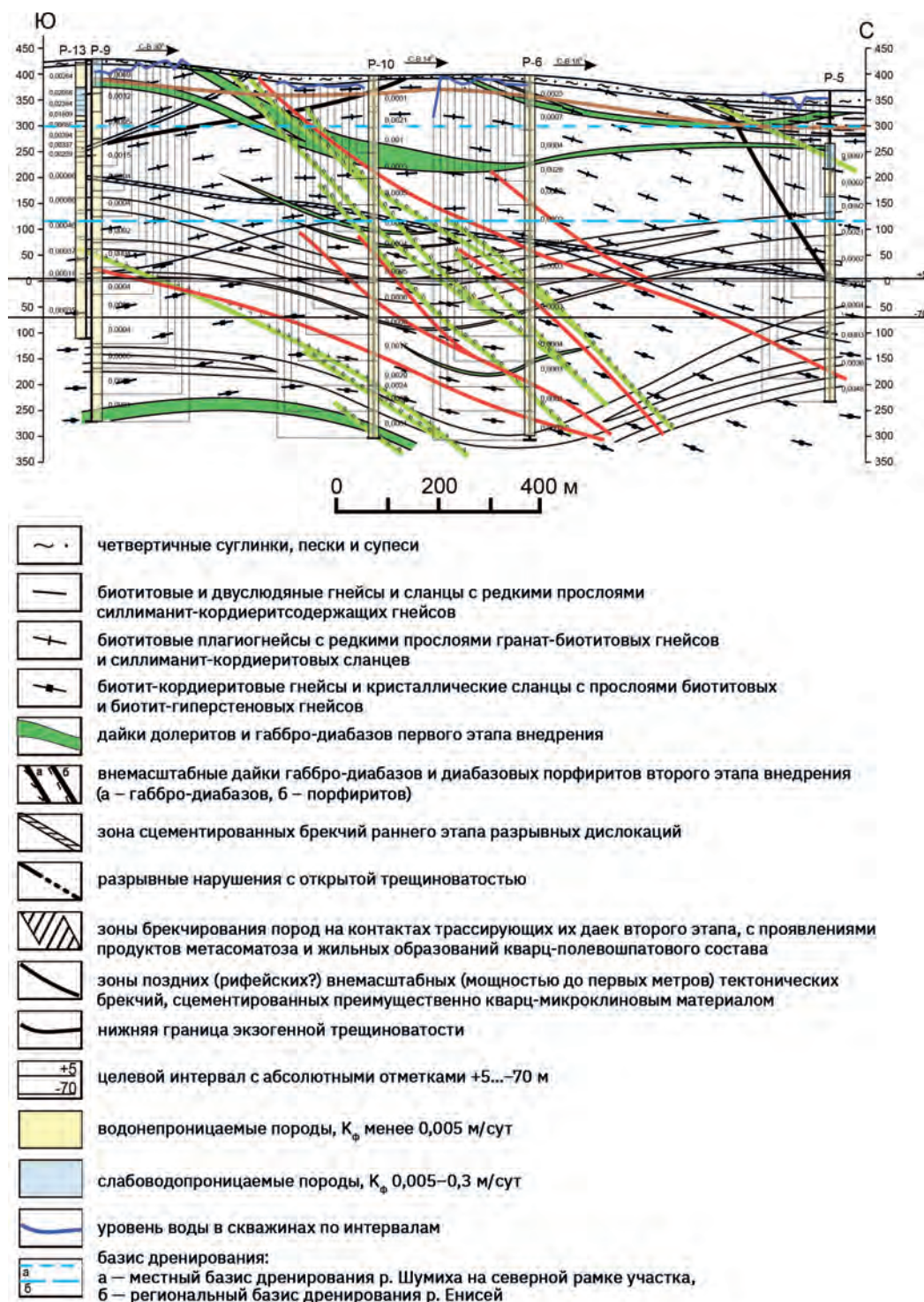
Рис. 5.30. Субмеридиональный гидрогеологический разрез (Караулов, Заблоцкий, 2015 [14])
