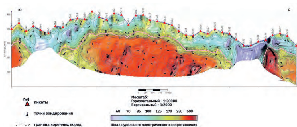
Рис. 4.13. Вертикальный разрез удельного электрического сопротивления по магистрали М-3. Метод переходных процессов (МПП) [а]
