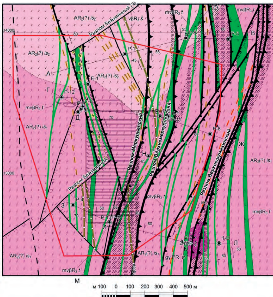
Рис. 5.21. Схема геологического строения на горизонте – 70 м (О. А. Морозов) Условные обозначения: см. рис. 5.19
