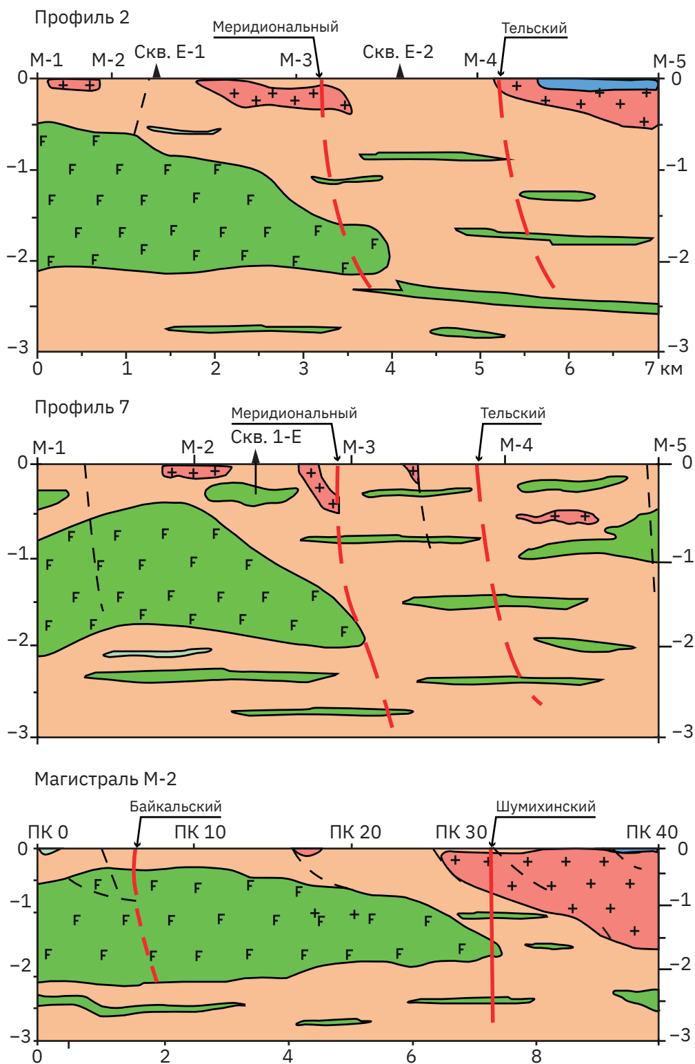
Рис. 4.21. Схематические геолого-геофизические разрезы к участку Енисейский [с] Условные обозначения: см. рис. 4.19
