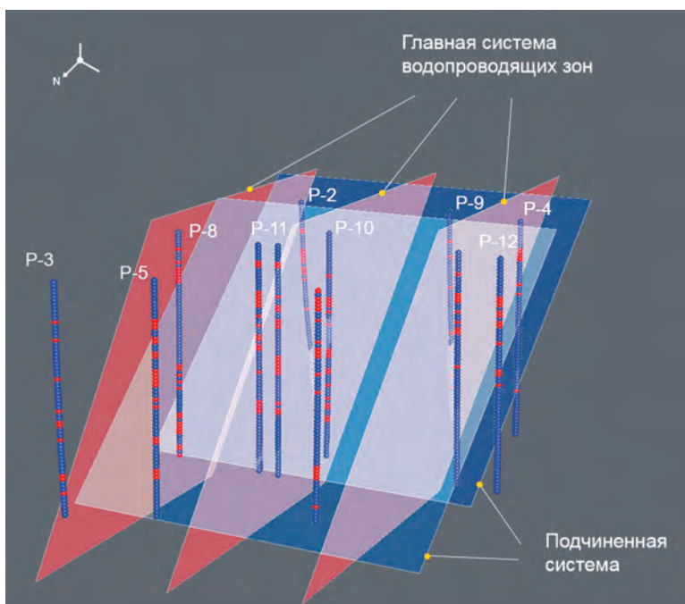
Рис. 5.46. Ориентация главной и подчиненной систем ориентировки зон дробления на участке Енисейский Красным отмечены зоны дробления; синим — вмещающий массив
