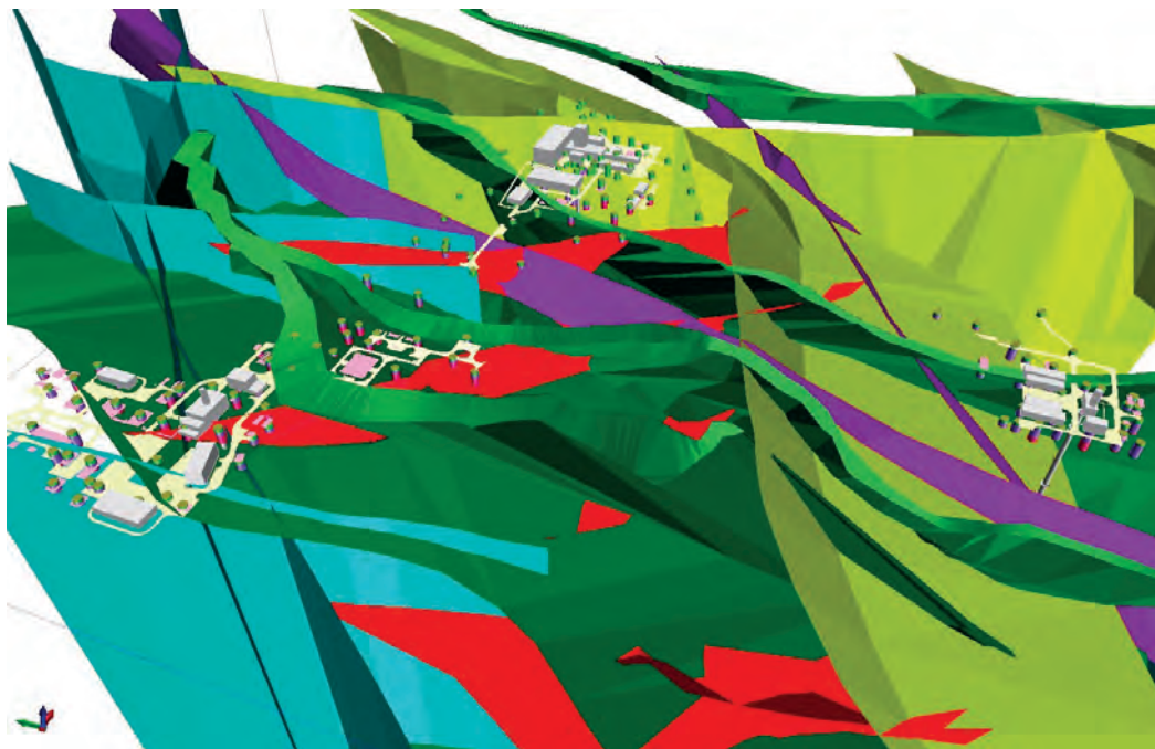
Рис. 5.18. Расположение проектируемых наземных сооружений относительно геологических тел Условные обозначения: см. рис. 5.14
