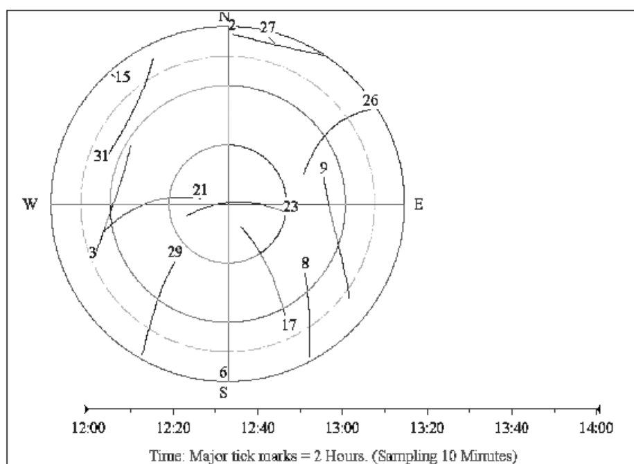
Рис. 10.6. Диаграмма небесной сферы (Skyplot) с траекториями спутников
