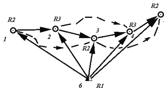
10.17. Базовый приемник R1 и два мобильных приемника R2 и R3
