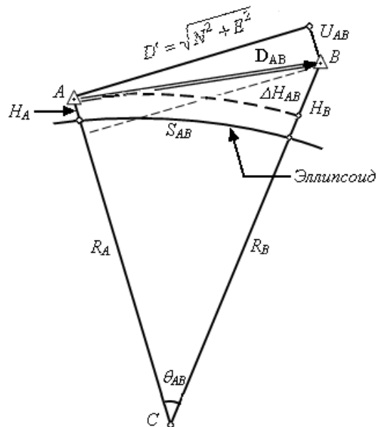
Рис. 11.6. Геометрия базовой линии
