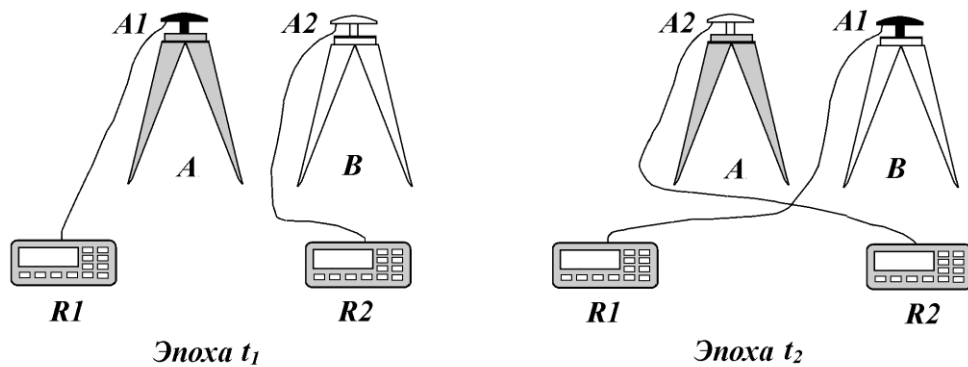
Рис. 8.11. Инициализация путем обмена позициями антенн приемников
