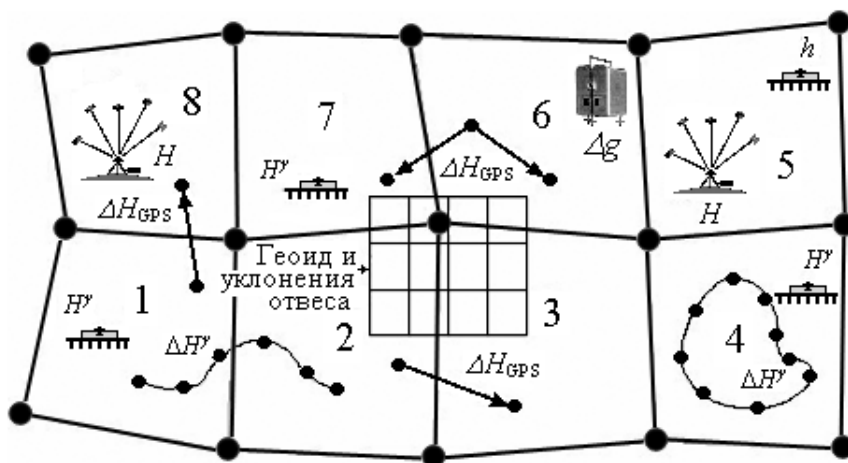
Рис. 11.10. Узловые точки и грани ячеек в модели высотной отсчетной поверхности, построенной по методу конечных элементов, и геодезические измерения (H, H', \Delta H, \Delta H') и опционально модель геоида \zeta , уклонения отвеса \xi, \eta и аномалии силы тяжести \Delta g как источники дополнительных данных)
