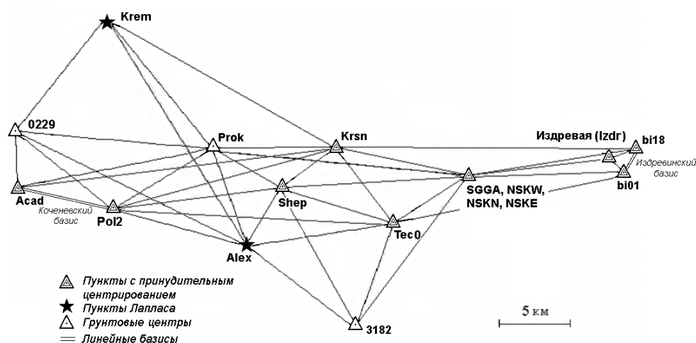
Рис. 10.19. Сеть эталонного метрологического полигона Сибирской государственной геодезической академии
