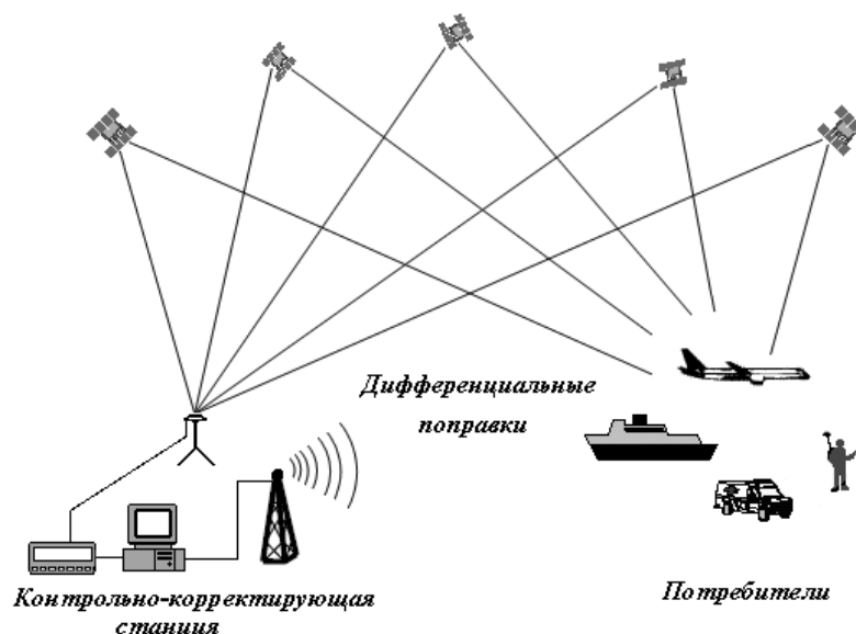
Рис. 8.4. Дифференциальный метод СРНС
