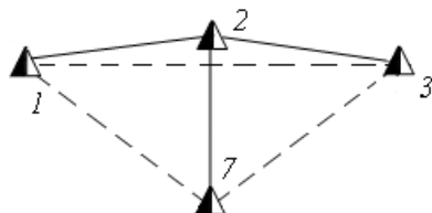
Рис. 10.3. Фрагмент сети, наблюдаемый четырьмя приемниками
