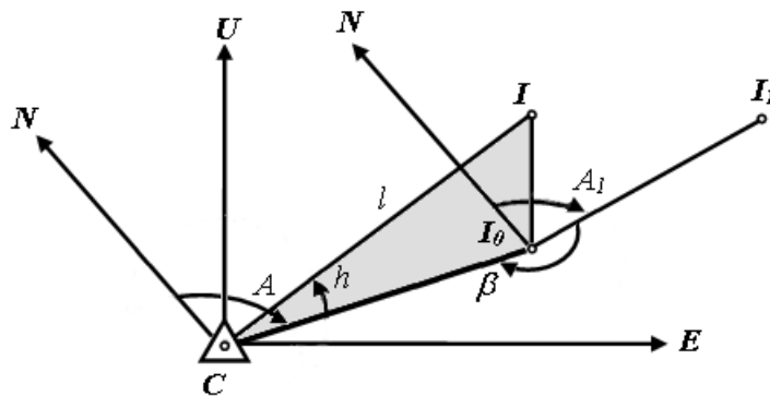
Рис. 10.11. Определение элементов приведения
