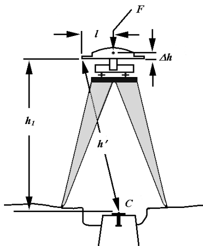
Рис. 10.9. Измерение высоты антенны
