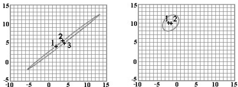
Рис. 11.5. Исходное и преобразованное пространства поиска неоднозначностей в методе LAMBDA [Joosten, Tiberius, 2000]
