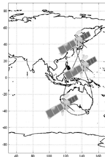
Рис. 12.3. Трасса спутников японской региональной навигационной системы QZSS при функционировании трех аппаратов [Takahashi, 2004]
