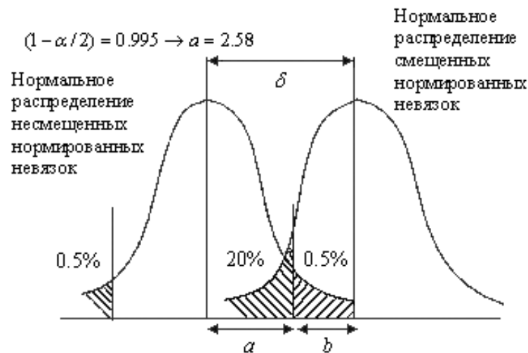
Рис. 11.7. Несмещённое и смещённое нормальное распределение остаточных невязок [Rizos, 1999]
