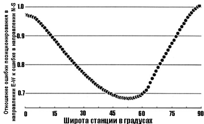
Рис. 9.6. Зависимость от широты станции отношения ошибки позиционирования в направлении E-W (восток-запад) к ошибке в направлении N-S (север-юг)
