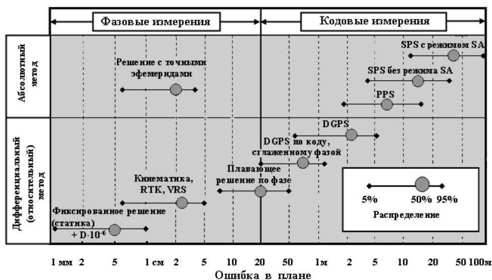
Рис. 10.1. Точность методов GPS/ГЛОНАСС измерений (по статье [Hein, 2000])
