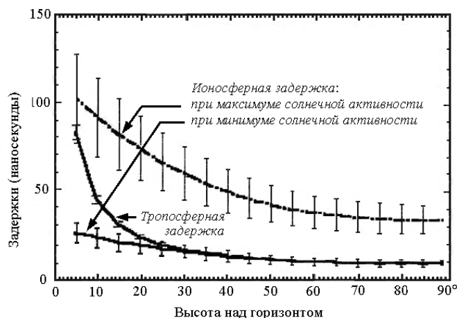
Рис. 9.1. Сравнение ионосферной и тропосферной задержек и их ошибок для средних широт и средних условий на разных высотах [Klobuchar, Kunches, 2003]
