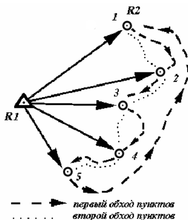
Рис. 10.8. Схема наблюдений в режиме реокупации
