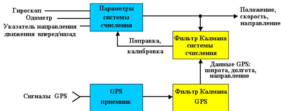
Рис. 8.14. Схема обработки данных в интегрированной системе GPS и системе счисления положений из одометра и гироскопа ( www.tycoelectronics.com/gps/deadreckoning.asp )
