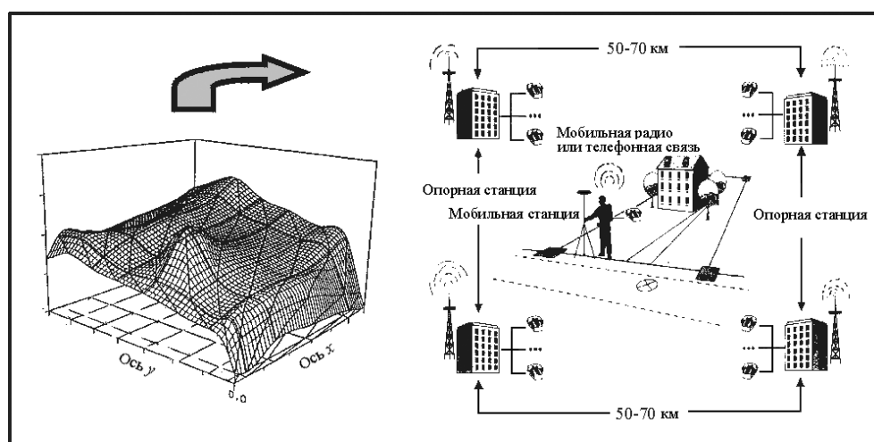
Рис. 11.11. Цифровая высотная поверхность DFHRS (слева) и использование ее базы данных DFHRS при определении высот в режиме online сетевым методом RTK (справа) [Jäger, 1999]
