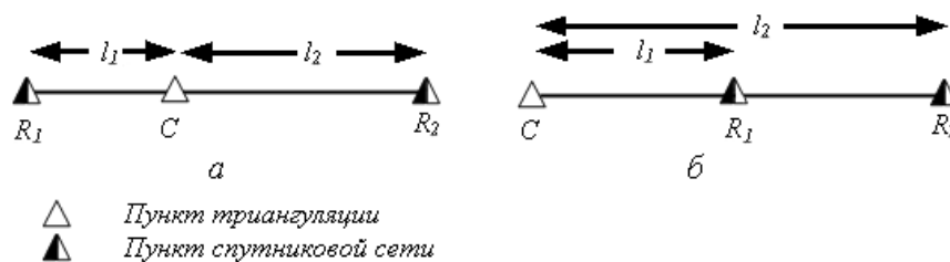
Рис. 10.12. Схема определения элементов приведения створным методом
