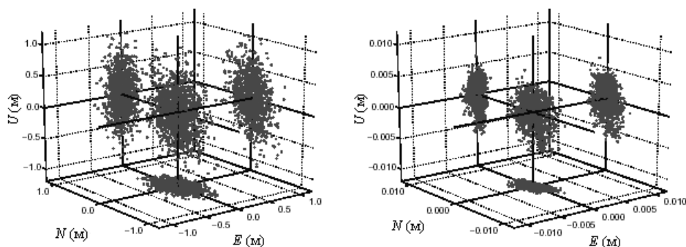
Рис. 11.2. Результаты обработки короткой базовой линии, представленные в системе координат E, N, U. Показано 1 200 одиночных решений для случая плавающих неоднозначностей (слева) и правильно разрешенных фиксированных неоднозначностей (справа). В плавающих решениях положение может иметь смещение на дециметр и более. При успешном разрешении неоднозначностей координаты имеют сантиметровый уровень точности [Joosten, Tiberius, 2000]
