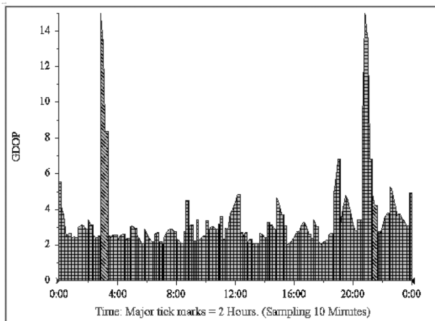
Рис. 10.5. Пример выдачи графика геометрического фактора GDOP
