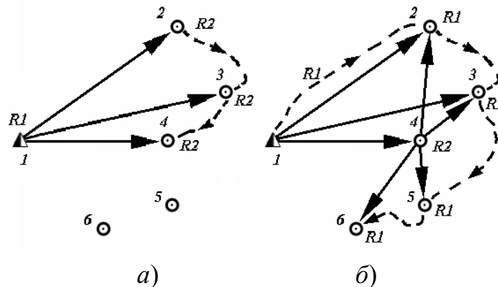
Рис. 10.14. Комбинация радиального и последовательного метода сбора данных
