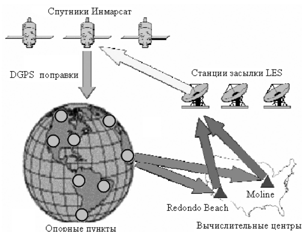
Рис. 8.7. Схема обмена данными в системе StarFire [Hatch et al., 2002]
