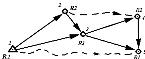
Рис. 10.18. Съёмка тремя мобильными приемниками
