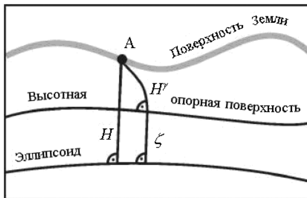
Рис. 11.8. Эллипсоидальная высота H , высота точки над ВОП H^\gamma и высота опорной поверхности \zeta над эллипсоидом при точке A(B, L) [Jäger, 1999]
