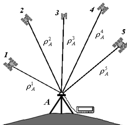
Рис. 8.1. Абсолютный метод спутниковых определений
