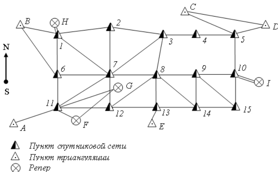
Рис. 10.2. Проект спутниковой геодезической сети
