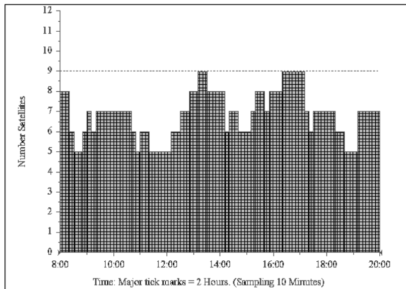
Рис. 10.4. График с указанием количества наблюдаемых спутников
