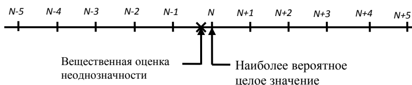
Рис. 11.4. Оценка вещественной неоднозначности и тестируемые кандидаты на целые значения
