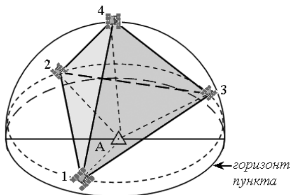
Рис. 8.3. Тетраэдр, вершины которого 1, 2, 3, 4 являются концами единичных векторов направлений на спутники с пункта А. Объем тетраэдра обратно пропорционален величине PDOP
