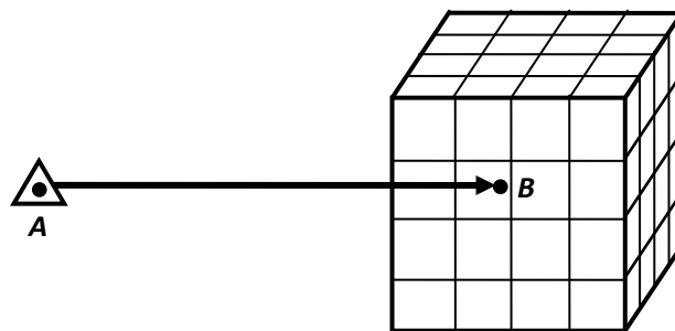
Рис. 8.12. Объем исследований неоднозначностей в виде куба
