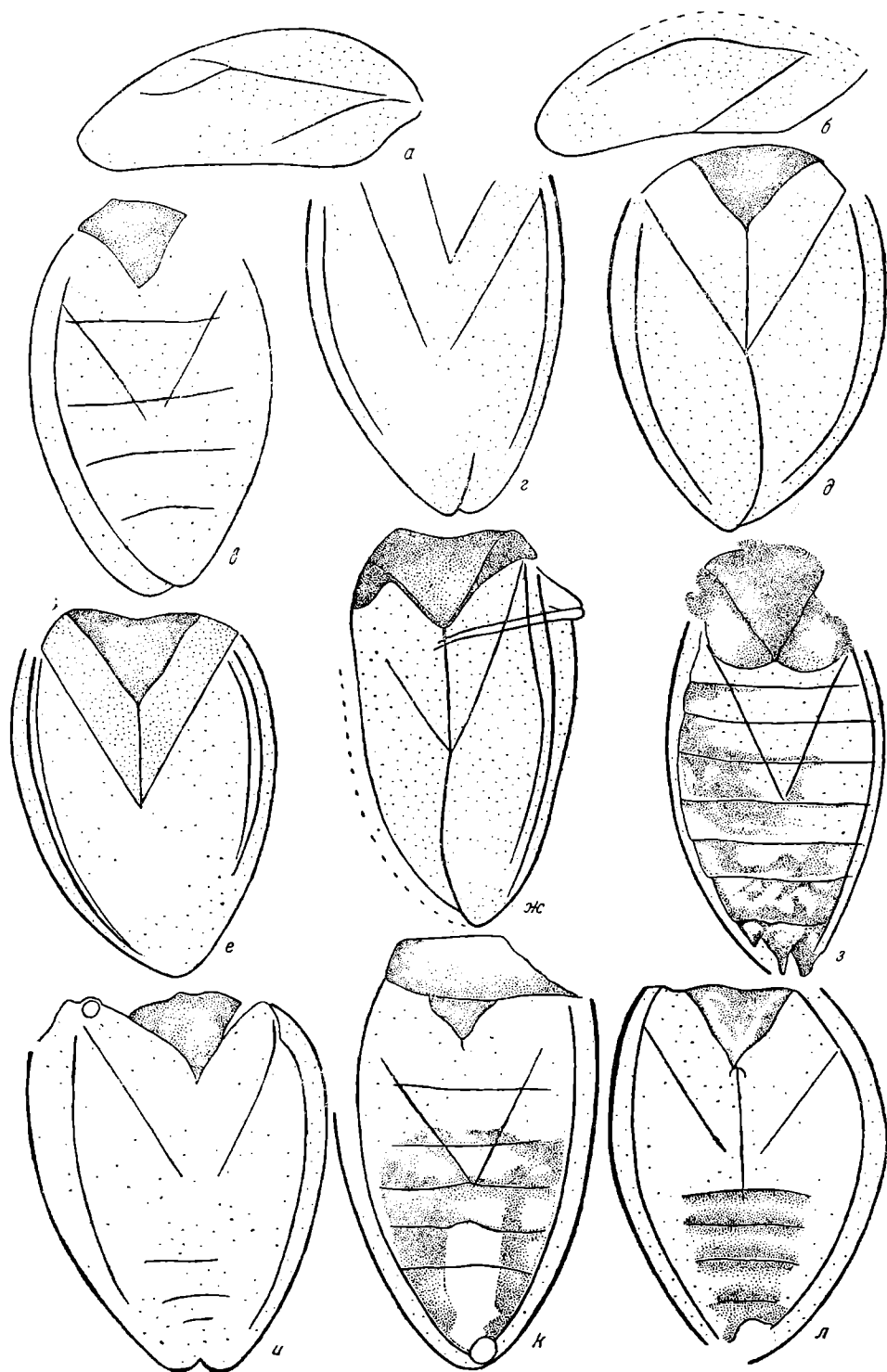
Рис. 23. Shurabella lepyroniopsis gen. n. sp. n. Остатки тел насекомых. Шураб III: а — № 459/108; б — № 459/72; в — № 459/71; г — № 459/144; д — № 459/59; е — № 459/80; ж — № 459/101 (см. продолжение рисунка на стр. 31).
