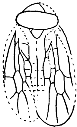
Рис. 20. Karabasia paucinervis Mart. Кара-Тай
