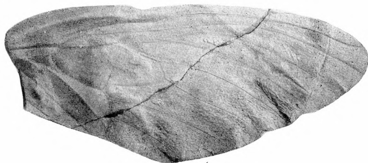
Фиг. 1. Cicadomorpha punctulata M a r t. Надкрылье. Карабас-Тау (Кара-Тау), № 2452/552
