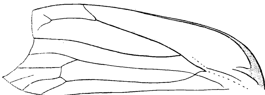
Рис. 29. Cycloscytina plachutai sp. n. Надкрылье. Шураб, № 459/150
