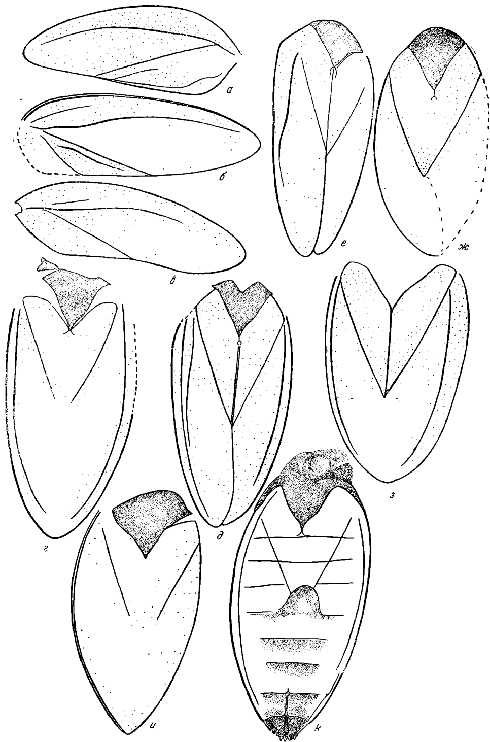
Рис. 24. Coleopteropsis dolichoptera gen. n. sp. n. Остатки тел насекомых. Шураб III: б — № 459/173; в — № 459/68; е — № 459/83в; д — № 459/83а; е — № 459/70; з — № 459/82; к — 459/189
