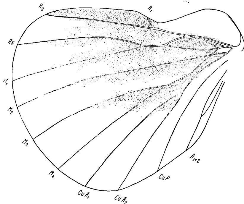
Рис. 6. Plachutella rotundata gen. n. sp. n. Заднее крыло (обратный отпечаток). Шураб III, № 459/22
