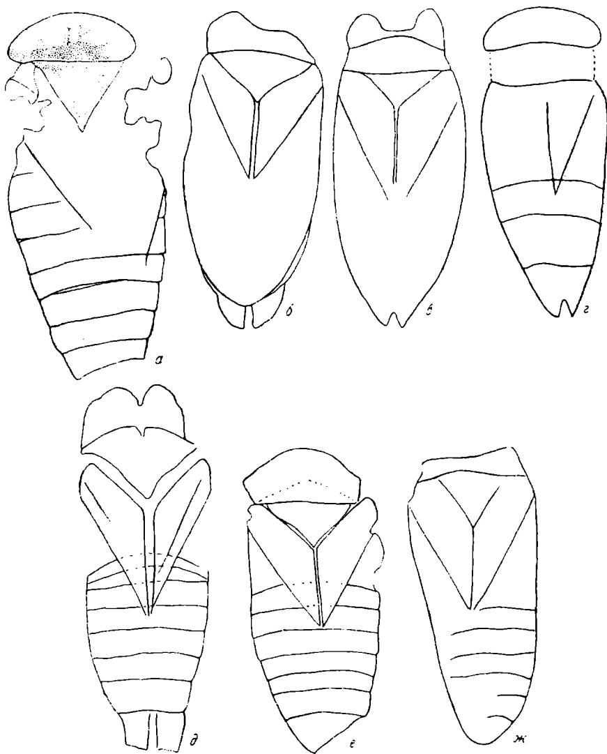
Рис. 22. Karataciella brachynota gen. n. sp. n. Остатки тела насекомого. Кара-Тай: а, в — № 61; б — № 2452/665а; г — № 55; д — № 63
