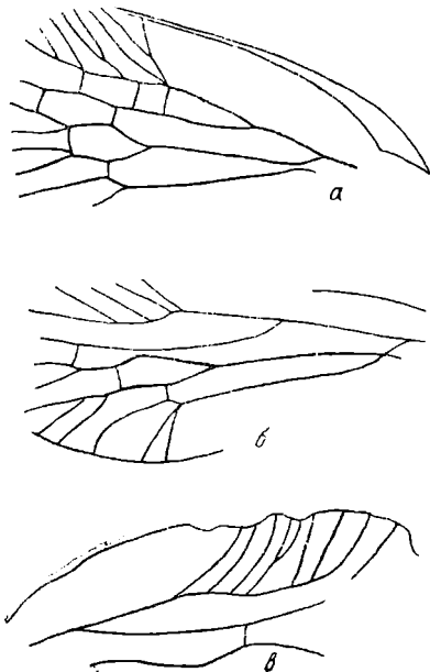
Рис. 30. Mesocixiella rohndendorfi sp. n. Индивидуальная изменчивость жилкования надкрылья. Фрагменты надкрылья. Кизил-Кия; а — № 166/52; б — № 166/49; в — № 166/55
