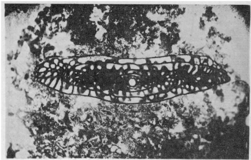
Рис. 2. Хорошо сохранившаяся раковина фузулины в известняке мячковского горизонта (увел. 30)
