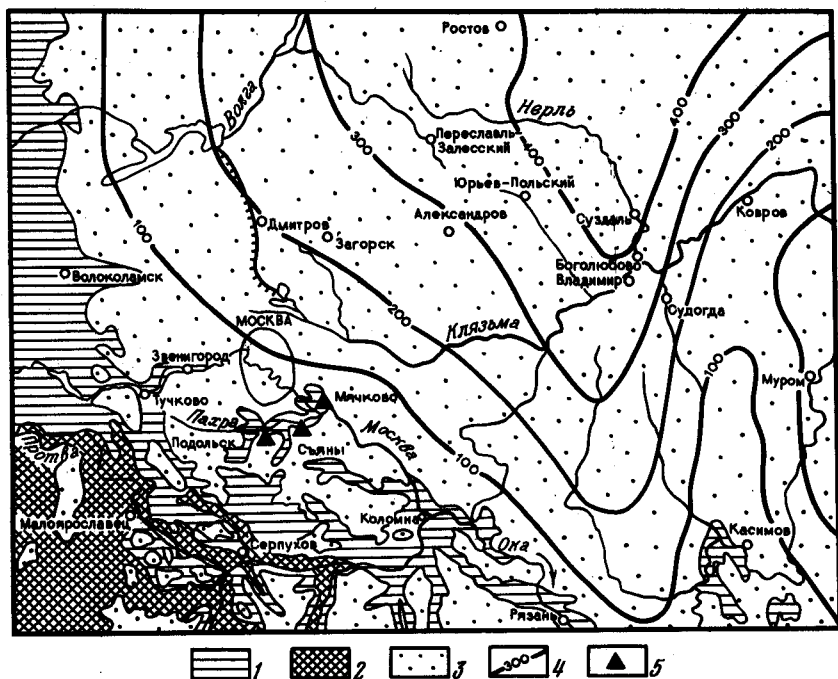
Рис. 1. Схема распространения среднекаменноугольных отложений в Подмоскowie и прилегающих областях (составлена с использованием материалов П. В. Флоренского и М. Н. Соловьевой):
