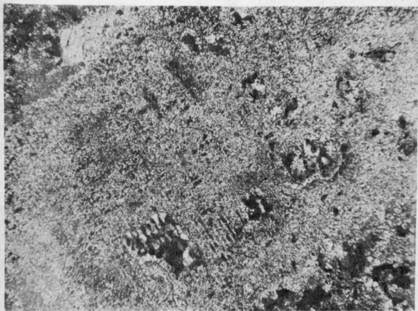
Рис. 37. Измененная порода — тонкозернистый гипс (основной фон) с отдельными участками известняка (пятнистые темные обособления)
