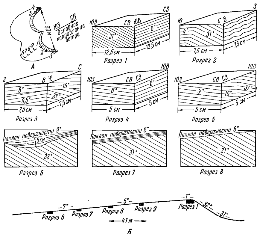
Фиг. 65. Слоистость бархана в Леуппе, Аризона (по Мак-Ки, 1953).
