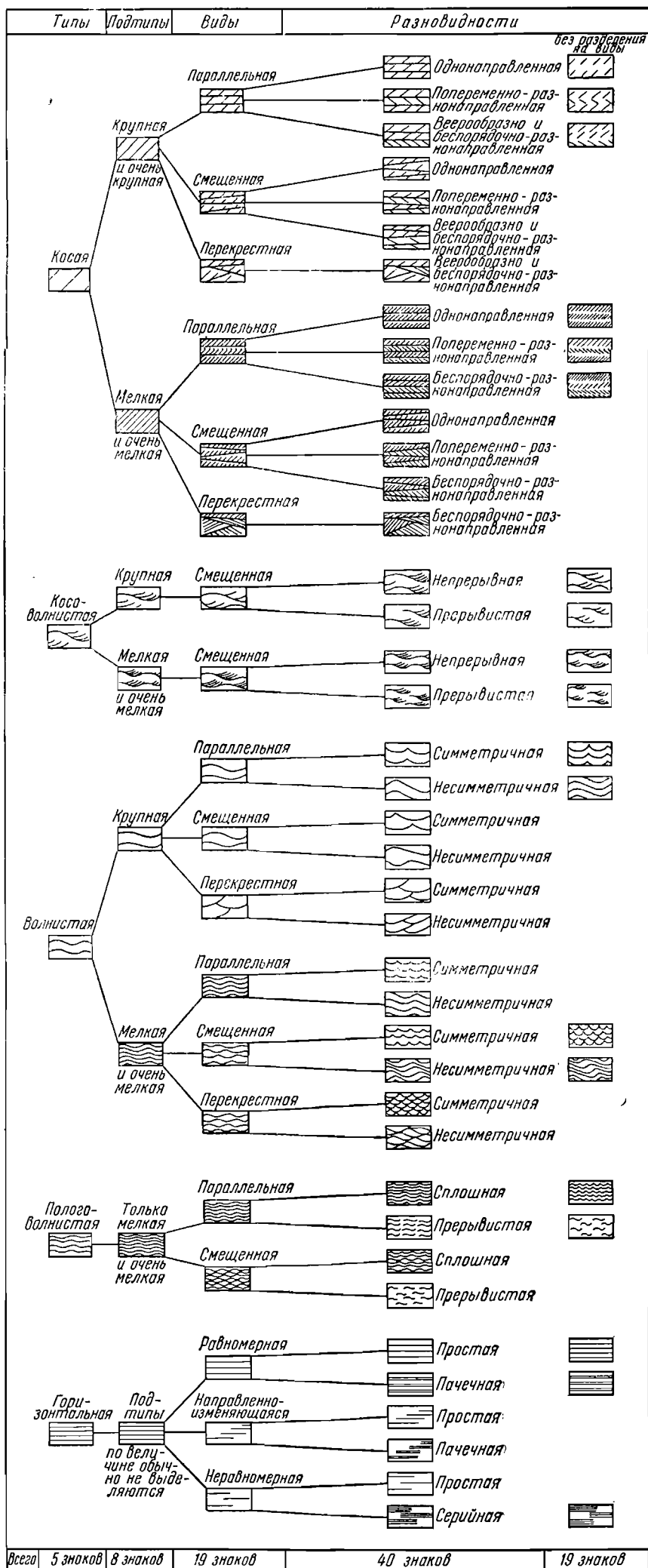
Фиг. 38. Условные обозначения, рекомендуемые для типов, подтипов, видов и некоторых разновидностей слоистости
