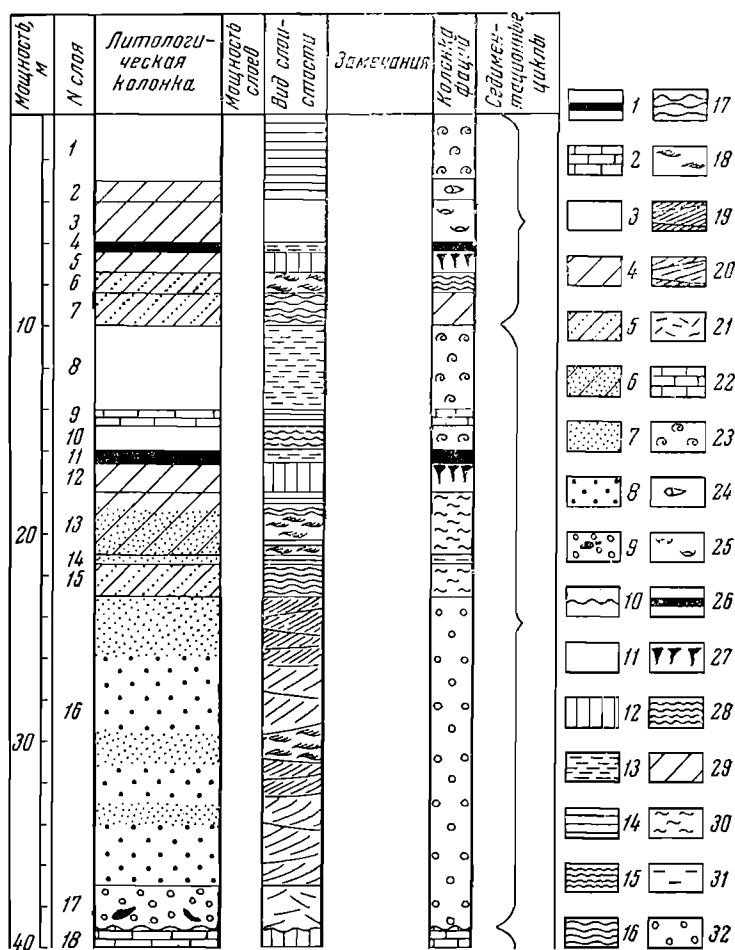
Фиг. 37. Пример колонки типов слоистости, параллельной основной литологической колонке.
