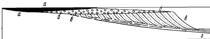
Фиг. 97. Схематическое изображение текстуры дельтовых отложений большой мощности и протяженности (отражающее лишь общий характер напластования).
