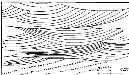
Фиг. 72. Косо-волнистая мульдобразная слоистость в мелкозернистом песке прирусловой отмели. Современные отложения р. Дон.
