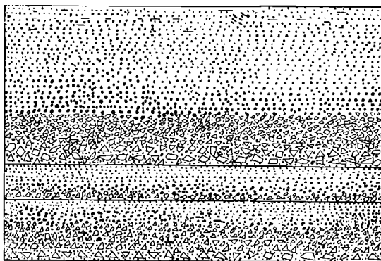
Фиг. 67. Ритмическая сортировка золовых пирокластических современных отложений в Мексике (по Шроку, 1950).
