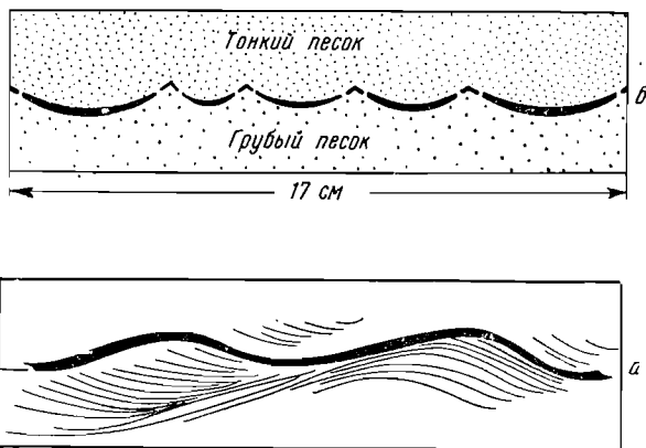
Фиг. 25. «Запечатывание» глинистым осадком валиков ряби.
