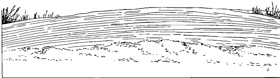
Фиг. 106. Слоистость берегового вала в поперечном разрезе. Правый берег устья р. Гаун (По Ульсту, 1957)
