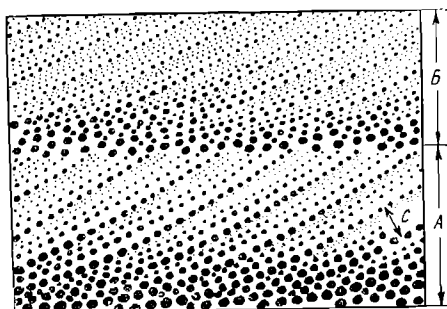
Фиг. 75. Многостепенная ритмическая сортировка, характерная для речных отложений.
