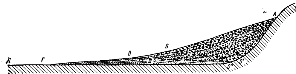
Фиг. 92. Вертикальный радиальный разрез наземной дельты, образованной у склона коренных пород (по К. В. Курдюкову, 1957).
