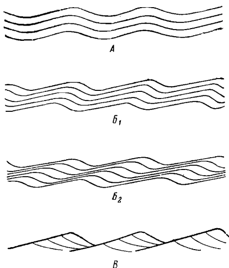
Фиг. 21. Постепенное видоизменение ряби течения и переход слоистости из одной разновидности в другую в результате последовательного изменения соотношения мощности слойков крутого и пологого склонов
