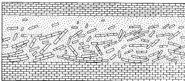
Фиг. 57. Текстуры растрескивания, взламывания и брекчиевидная.
