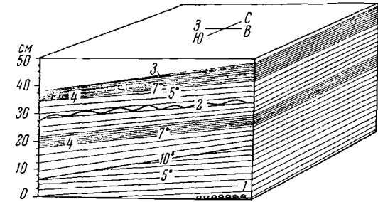
Фиг. 109. Косая слоистость отложений верхнего переднего пляжа. Калифорния. Океан слева (по Мак-Ки, 1953).
