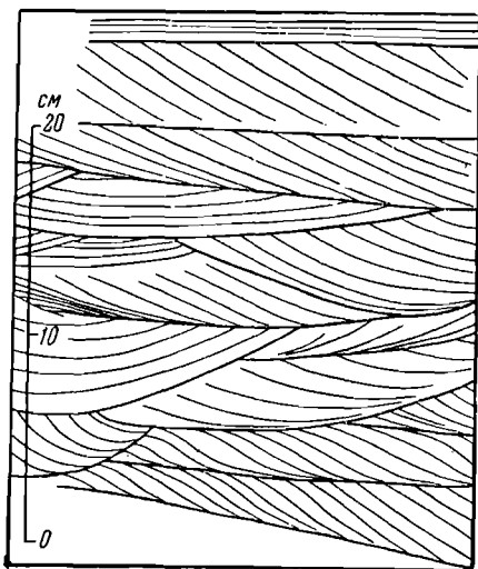
Фиг. 118. Мелкая косая и косо-волнистая слоистость в прибрежно-морских четвертичных отложениях около р. Маныч.
