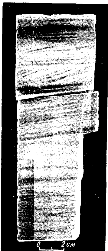
Фиг. 104. Слоистость баров или пересыпей в мелкозернистом песчанике.
