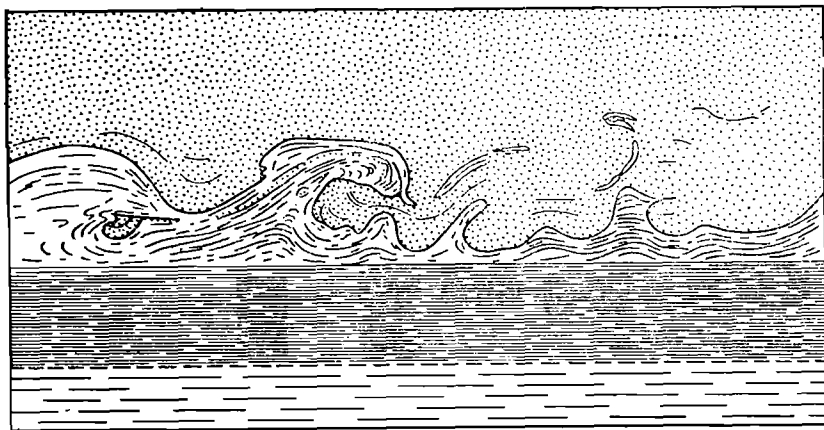
Фиг. 55. «Знаки нагрузки», образуемые в результате дифференциальной нагрузки на мягкий вязкий осадок. Отпечатки пластичного течения в слое тонкозернистого песка, отложившемся на полужидком глинистом осадке, слоистость которого деформирована (по Шроку, 1950)
