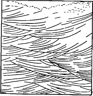
Фиг. 98. Характерная косая слоистость дельтовых третичных отложений (по Р. Шроку, 1950)
