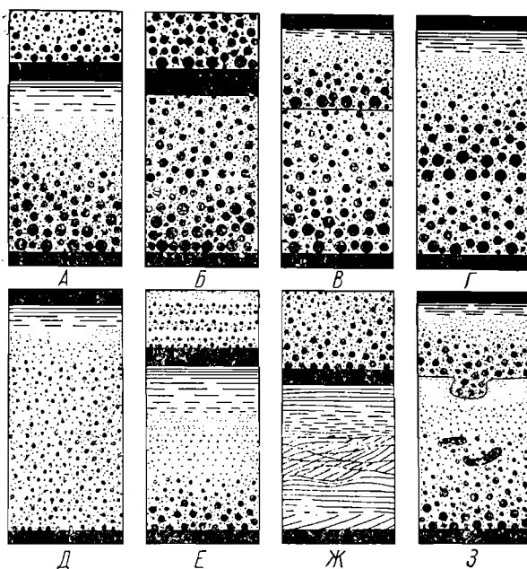
Фиг. 129. Различные типы сортированной слоистости (по Кюену, 1953). Черное — глубоководные тонкозернистые осадки («лютит»).
