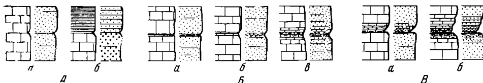
Фиг. 26. Типы переходов между слоями (по Ломбару, 1956, с изменением).
