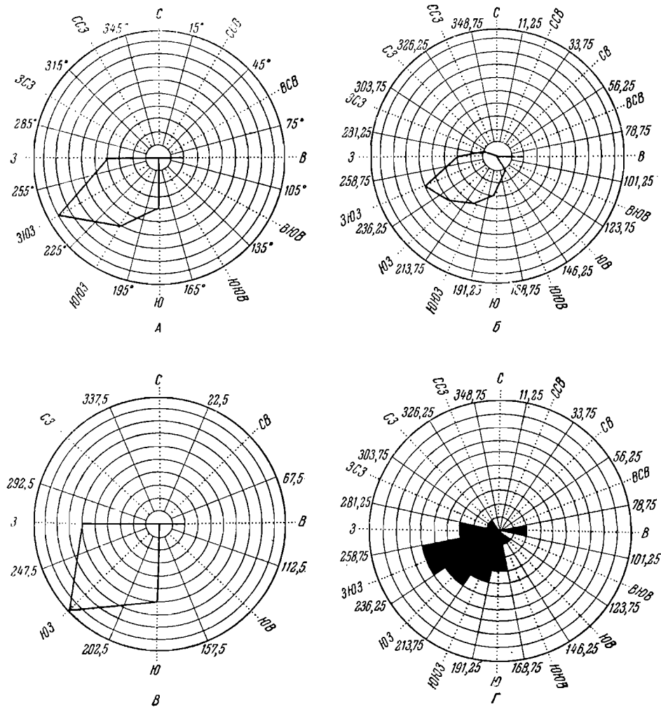
Фиг. 41. Диаграммы-розы направлений косых слоев, построенные для одних и тех же замеров, но при разбивке круга на секторы через различное количество градусов. А — на 12 секторов через 30°; Б — на 16 секторов через 22,5°; В — на 8 секторов через 45°; Г — то же, что и Б, но диаграмма дана с выделением всей площади сектора
