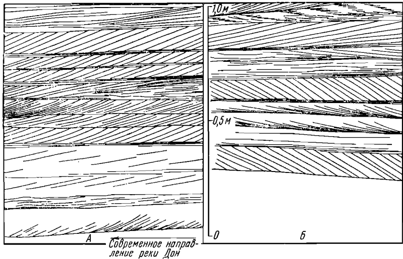
Фиг. 70. Параллельная однонаправленная косая слоистость русловых отложений (четвертичной террасы р. Дон). А — зарисовка в плоскости, параллельной современному течению р. Дон; Б — зарисовка в плоскости перпендикулярной
