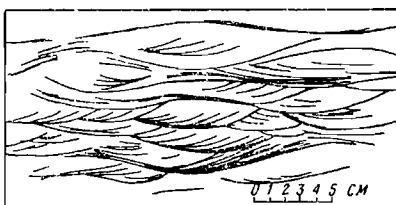
Фиг. 73. Косо-волнистая слоистость в отложениях верхней части прирусловой отмели р. Оки.
