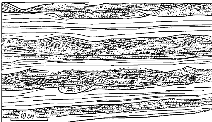
Фиг. 130. Прослой со слоистостью ряби течения в илистых песках между сланцами, отложенными мутевыми потоками, текшими в общем слева направо. Третичные отложения (по Кюнелю, 1953)
