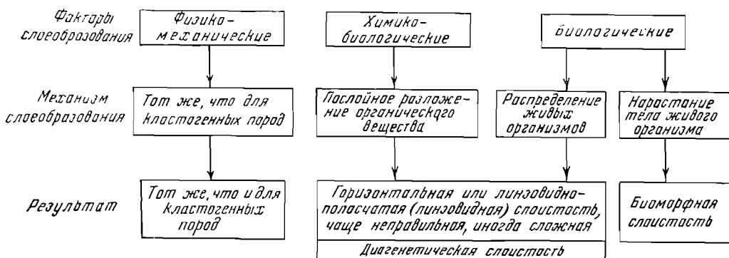
Фиг. 11. Схема зависимости текстуры органогенных отложений от механизма их образования
