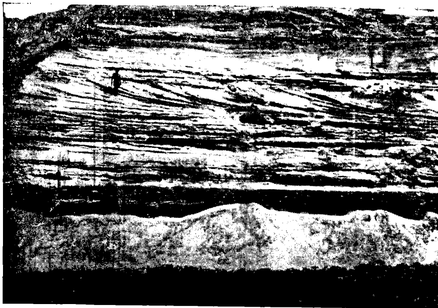
Фиг. 123. Очень крупная косая слоистость в морских мезозойских песках.
