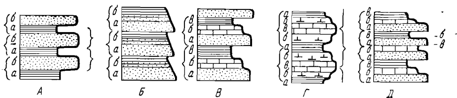
Фиг. 7. Типы ритмической слоистости.
