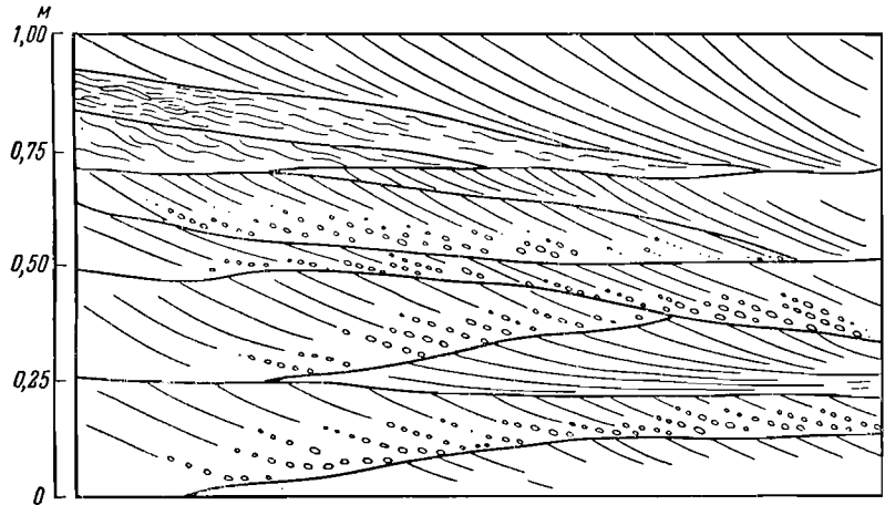
Фиг. 71. Косая однонаправленная слоистость речных отложений. Серии клиновидные (рис. Е. П. Брунс)
