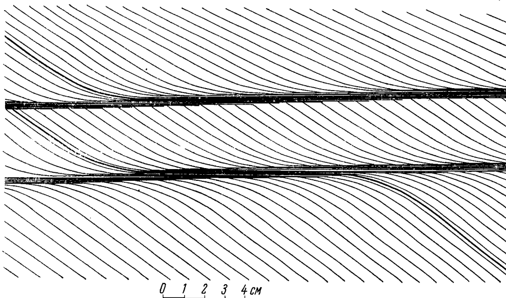
Фиг. 95. Тонкая асимметричная волнистая слоистость ряби течений во флювиогляциальном мелкозернистом песке.
