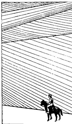
Фиг. 62. Очень крупная косая слоистость эоловых отложений в мезозойском песчанике (по Твенхофелу, 1932)
