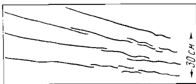
Фиг. 16. Усложнение волнением формы косых слойков у их основания в морских песчаных отложениях.
