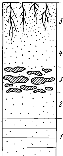
Фиг. 5. Условность выделения слоев.
