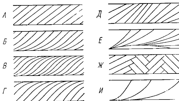
Фиг. 15. Форма слойков и их соотношение внутри одной серии.
