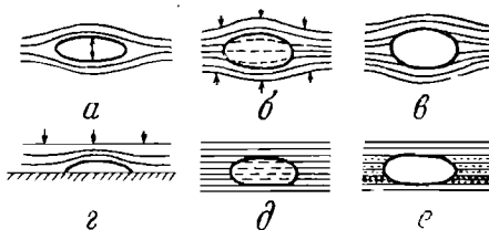
Фиг. 50. Соотношение слоистости с конкрециями.
