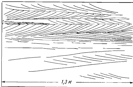
Фиг. 124. Попеременно-разнонаправленная (перистая) косая слоистость в морских песках.
