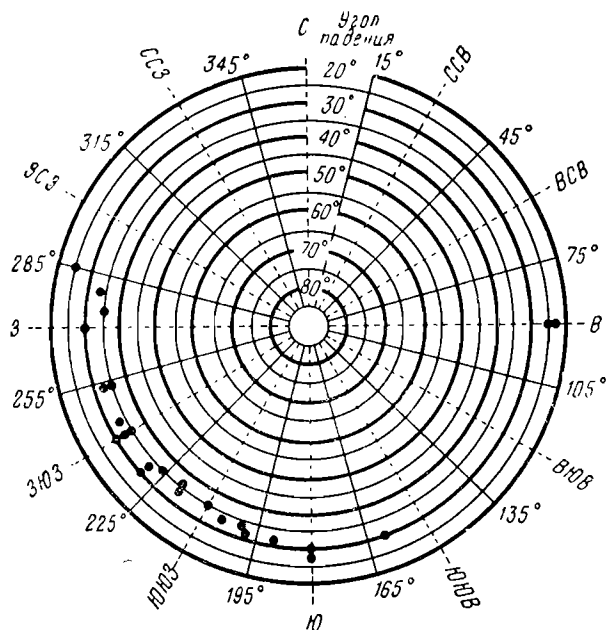
Фиг. 39. Круговая полярная диаграмма углов падения и азимутов косои слоистости
