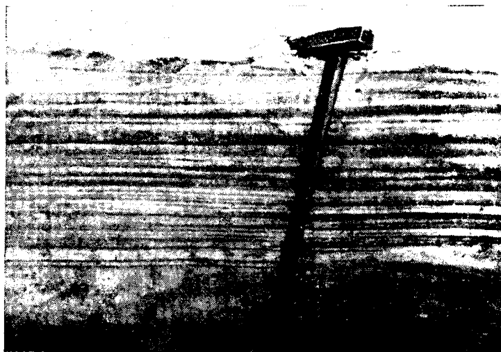
Фиг. 121. Правильная горизонтальная слоистость в морских песках. Слойки образуют пачки разных порядков. Карбон Подмосковского бассейна
