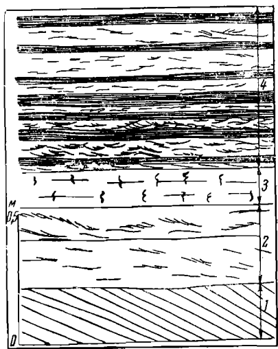
Фиг. 77. Комплекс пойменных отложений в карьере у ст. Хапры (верхний плиоцен).
