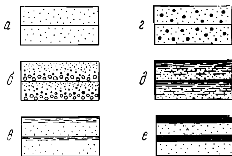
Фиг. 18. Типы строения слоев (а, б, в, г) и их пар (д, е).
