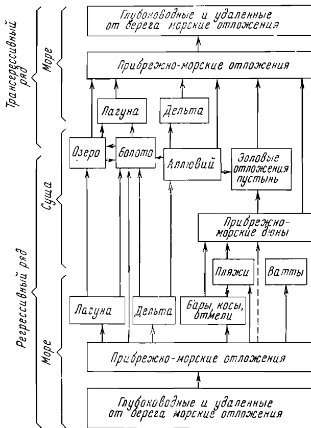
Фиг. 133. Схема возможных взаимных переходов отложений различных фаций при регрессивном и трансгрессивном их развитии
