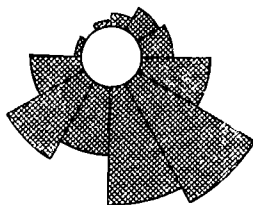
Фиг. 42. Диаграмма, в которой линии концентрических окружностей указывают процент замеров, попадающих в данный сектор. Рядом — пример такой диаграммы (построена Петтиджоном для кварцитов Барабу по 2833 замерам)
