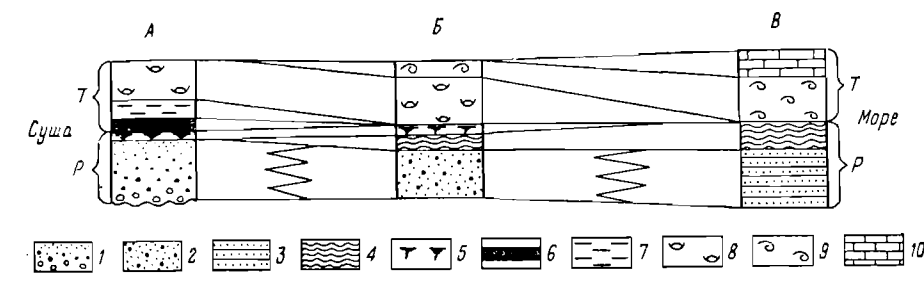
Фиг. 136. Изменение фациального состава цикла на площади по направлению от суши к морю.
