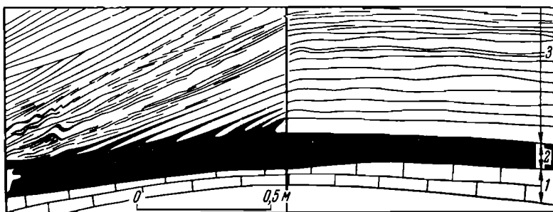
Фиг. 105. Слоистость песчаного берегового вала (четвертичные отложения). Местами, особенно внизу, косые слойки усложнены рябью.
