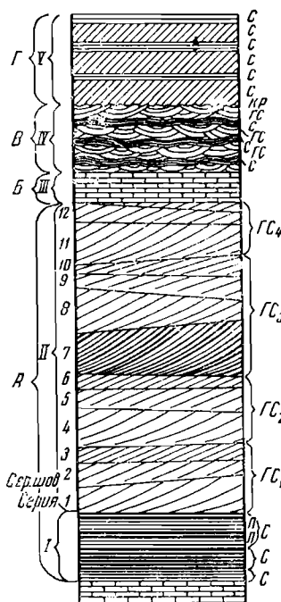
Фиг. 3. Основные слоевые элементы.
