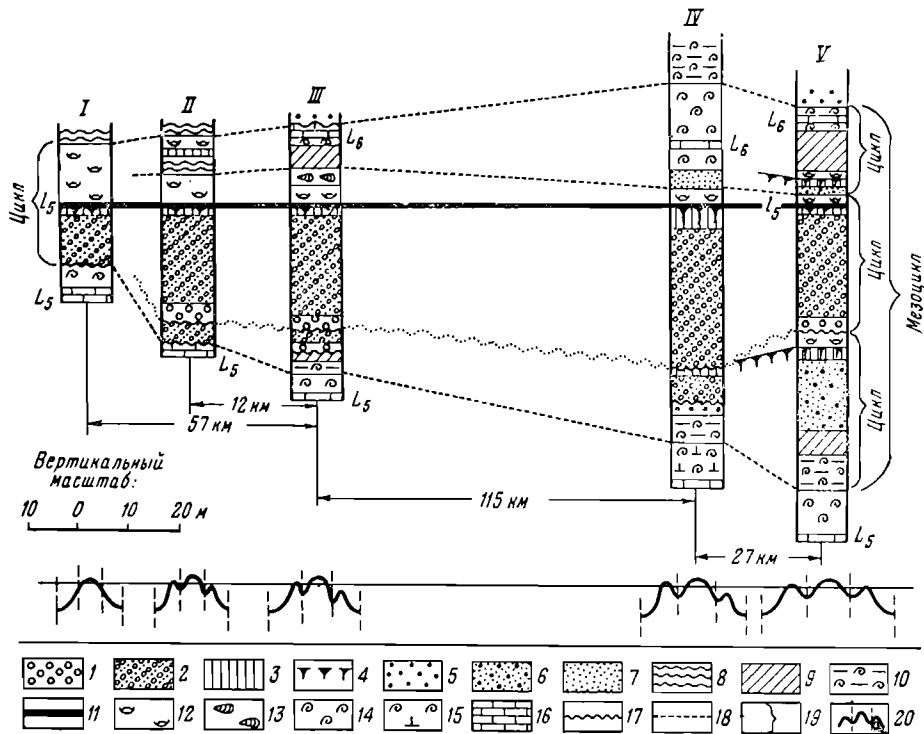
Фиг. 137. Расщепление элементарного цикла первого порядка и постепенное превращение его в мезоцикл (цикл второго порядка), состоящий из трех самостоятельных элементарных циклов. Внизу кривыми схематически показано постепенное усложнение строения данного разреза. Средний карбон Донецкого бассейна.
