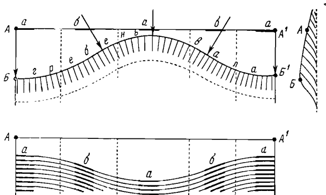
Фиг. 30. Кажущийся переход косой слоистости в горизонтальную, который виден в вертикальном разрезе в результате изогнутости песчаного вала.
