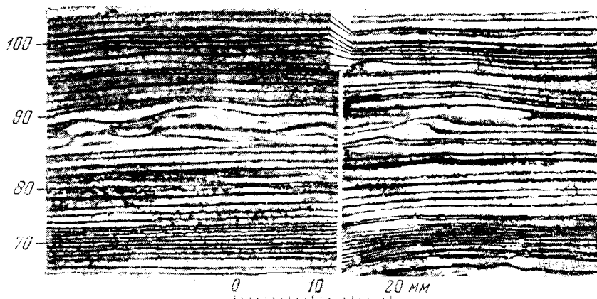
Фиг. 47. Сопоставление кернов из двух скважин, пройденных в горизонтально слоистом ангидрите. Видно одинаковое нарушение слоистости в интервале лент 85—88
