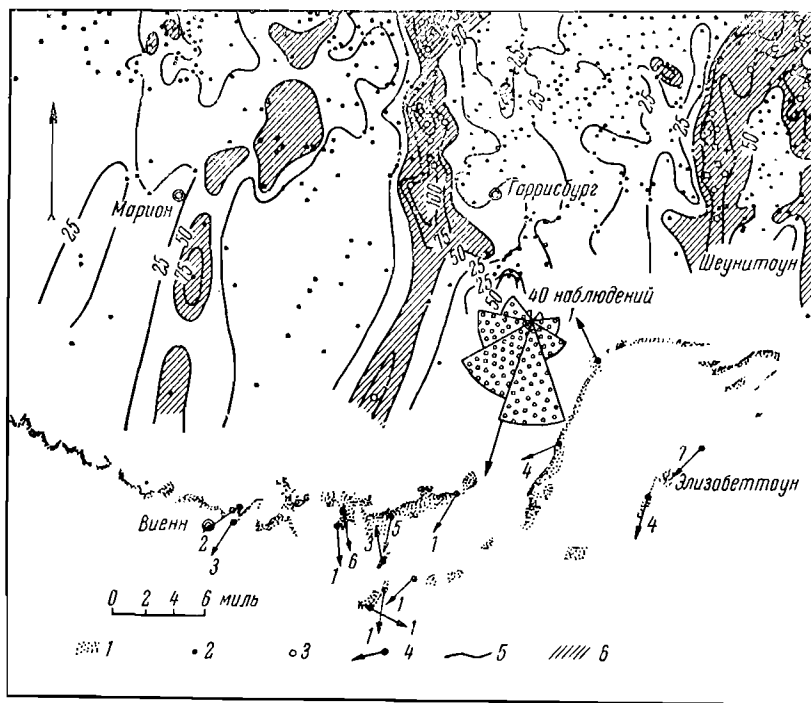
Фиг. 139. Диаграмма замеров кривой слоистости, нанесенная на карту распространения песчаников (по Поттеру, 1958).
