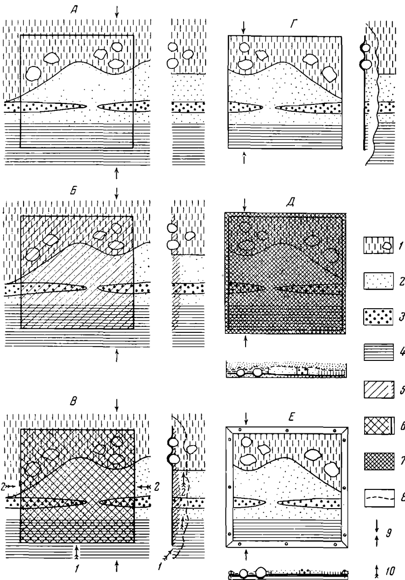
Фиг. 36. Отдельные этапы (А—Е) изготовления пленочного монолита (по К. К. Орвику, 1948).
