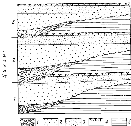
Фиг. 76. Сложное строение аллювиальной толщи. В левой части разреза видно многоярусное строение песчано-галечных отложений, обусловленное наложением речных отложений различных седиментационных циклов; это видно из сопоставления с правой частью разреза, где мощности аллювия каждого цикла уменьшаются.
