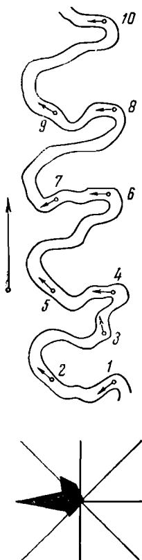
Фиг. 34. Возможность ошибочного определения направления меандрирующего потока при замерах азимутов падения косой слоистости.
