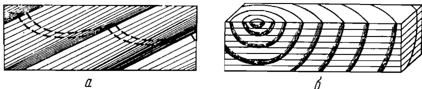
Фиг. 29. Вторичные полосы (типа колец Лизеганга), создающие ложное впечатление слоистости.
