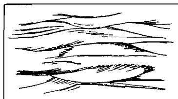
Фиг. 73. Косо-волнистая слоистость в отложениях верхней части прирусловой отмели р. Оки.
