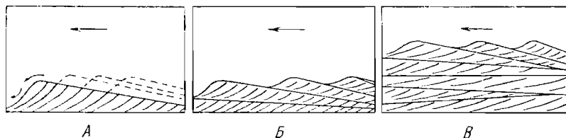
Фиг. 13. Образование косослоистых серий в осадке.
