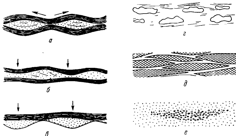
Фиг. 20. Линзовидная слоистость, обусловленная различным механизмом образования:
