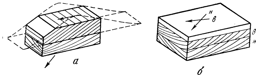
Фиг. 32. Изменение слоистости в зависимости от сечения.
