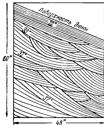
Фиг. 63. Перекрестная косая слоистость в разрезе поперечной высокой дюны, закрепленной растительностью (о-в Мустанг). Направление ветра слева направо (по Мак-Ки, 1953)
