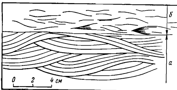
Фиг. 113. Деталь слоистости в прибрежно-морских песках (четвертичные отложения, берег Азовского моря).
