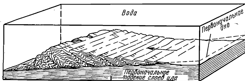
Фиг. 54. Текстура оползания или оплывания, образующаяся в осадке на слабо наклонном дне (по Р. Шроку, 1950)
