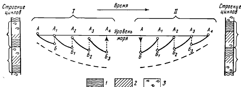
Фиг. 135. Неполные, резко асимметричные циклы, представленные лишь одним рядом фаций.
