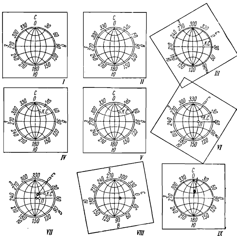
Фиг. 35. Техника редукции при помощи сетки Вульфа (по Вассоевичу и Гроссгейму, 1951).
