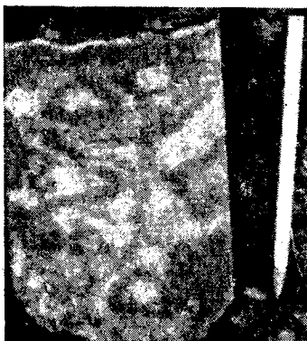
Фиг. 89. Ископаемая подпочва в пермских красноцветных отложениях Приуралья; сверху подпочва переходит в почву
