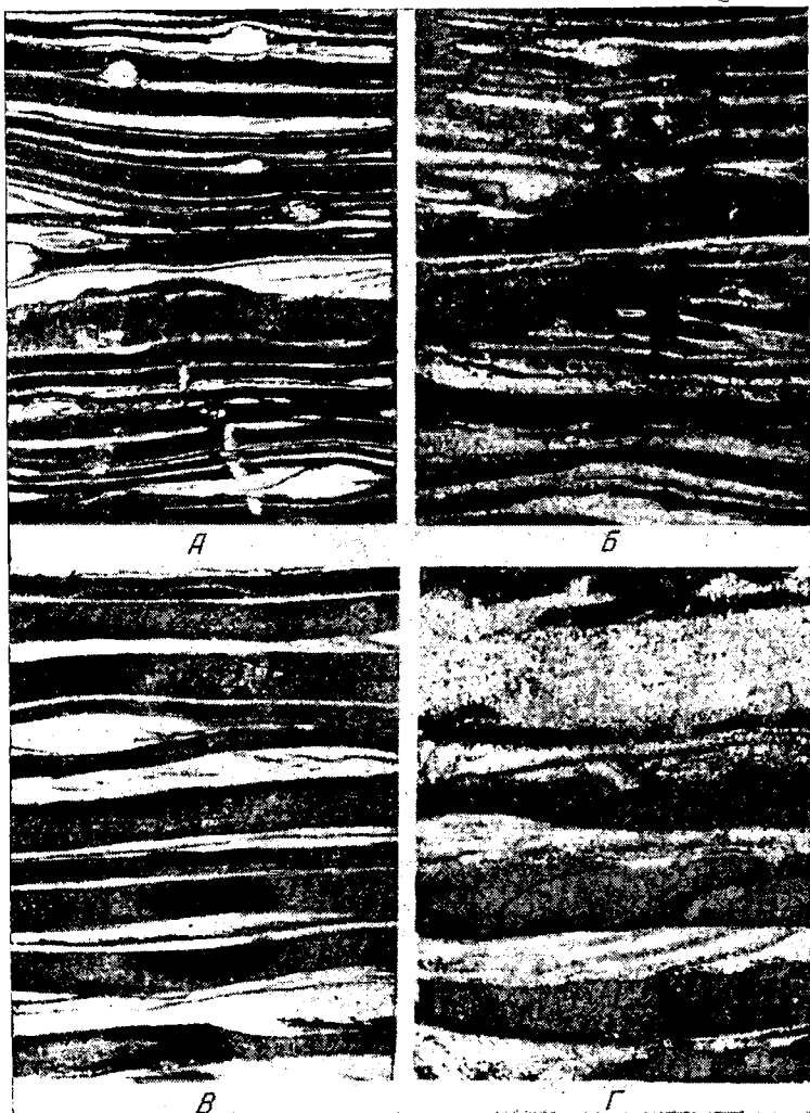
Фиг. 111. Сопоставление отложений современных ваттов (справа) и толщ переслаивания алевролитов в угленосных отложениях (слева) (по Поттеру и Глассу, 1958).
