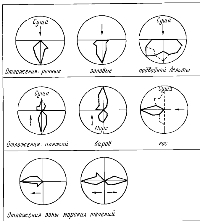
Фиг. 44. Диаграммы-розы для разных генетических типов косой слоистости. Стрелка показывает основное направление движения среды отложения
