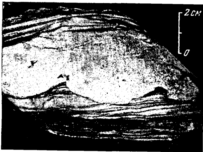
Фиг. 56. Размывы в основании песчаных прослоев, срезающие тонкую слоистость подстилающего алевролита на глубину 1—1,5 см. Отложения прибрежной зоны волнений и слабых течений лагун и заливов.
