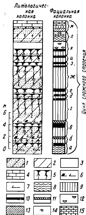
Фиг. 138. Сложное строение седиментационного цикла.
