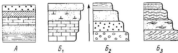
Фиг. 8. Различные типы чередования слоев в разрезе.
