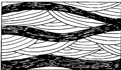
Фиг. 24. Сложная волнистая слоистость. Чередование материала более грубозернистого (светлое) и более тонкозернистого (темное). Границы их полого-волнистые. В более грубозернистом материале видна группа серий волнистой мульдобразной слоистости. Более тонкозернистый представлен одной серией с внутренней полого-волнистой слоистостью (неотчетливой)
