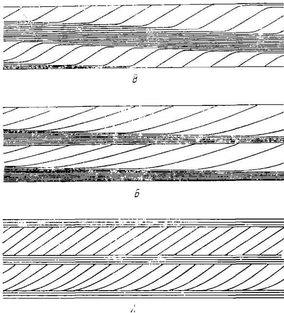
Фиг. 23. Различные способы образования чередования горизонтальных и косых слоев.
