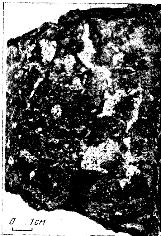
Фиг. 90. Ископаемая почва с большим количеством известковых конкреций, секущих слоистость (в красноцветах джезказганской свиты — карбон)
