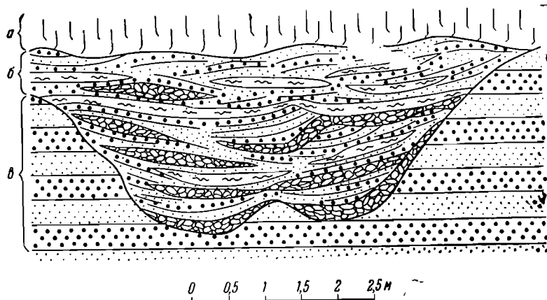
Фиг. 93. Овражный делювий (по А. С. Корженевской и О. Н. Бахваловой, 1940).
