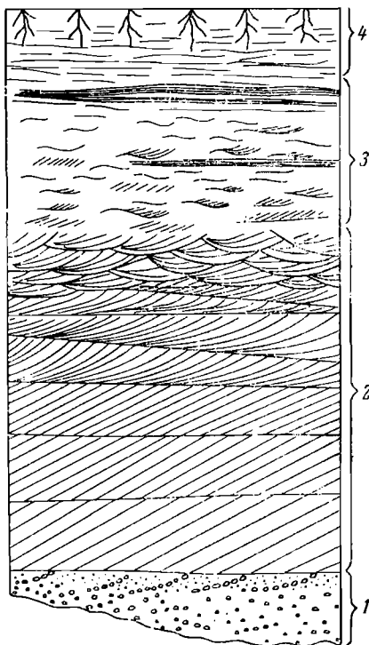
Фиг. 68. Схема смены типов слоистости в аллювиальной толще.
