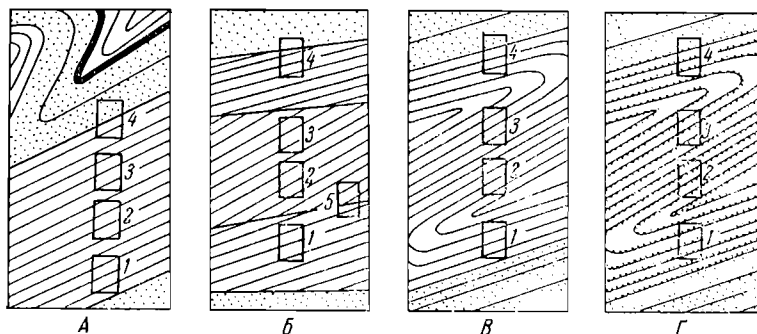
Фиг. 53. Определение элементов залегания по керну в косослоистой породе или в складчатой толще.
