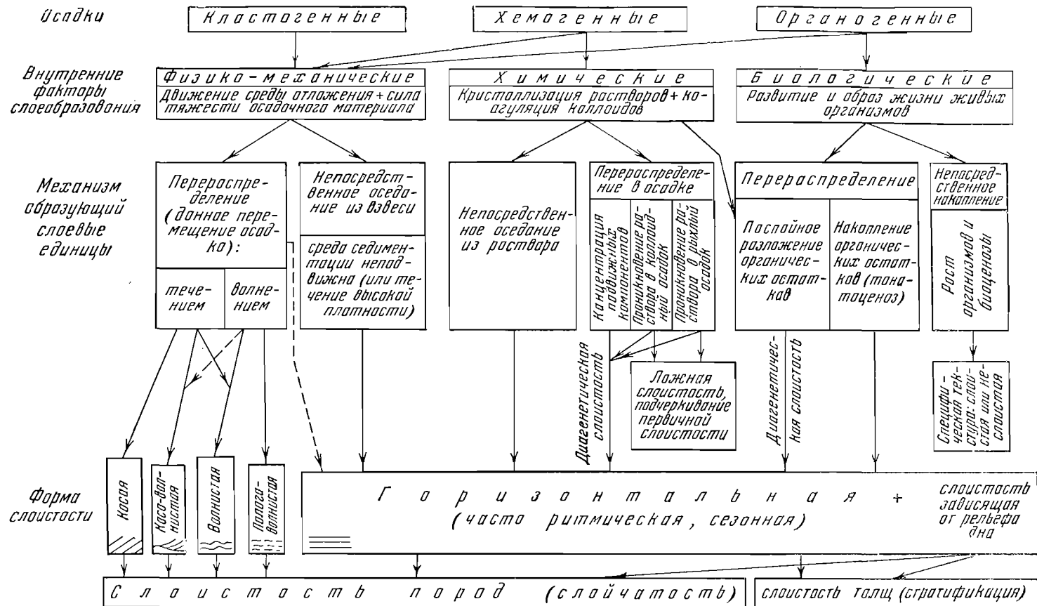
Фиг. 9. Схема зависимости морфологического типа слоистых текстур от различных внутренних факторов и механизма слоеобразования
