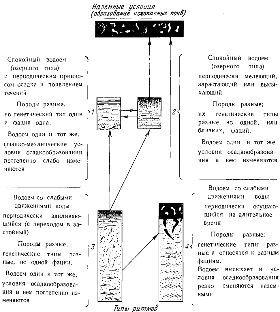
Фиг. 81. Ритмы, повторение которых характерно для разного типа водоемов, сменяющихся во времени
