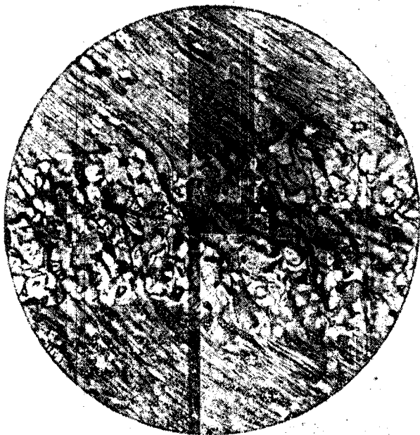
Фиг. 51. Соотношение слоистости и сланцеватости. Слоистость выявляется прослоем алевритовых зерен (кварц и полевой шпат) в глинистой породе. В последней видна сланцеватость, секущая слоистость под углом. Верхний девон Кузбасса (Атлас текстур и структур..., 1962)
