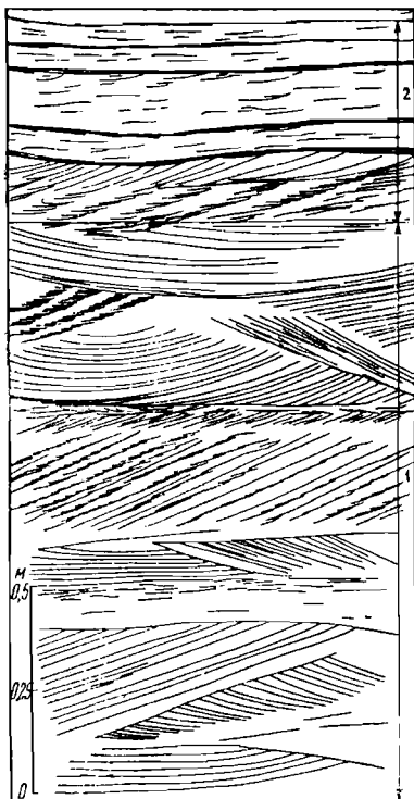
Фиг. 74. Слоистость в песчаных речных отложениях (левый берег р. Дон).
