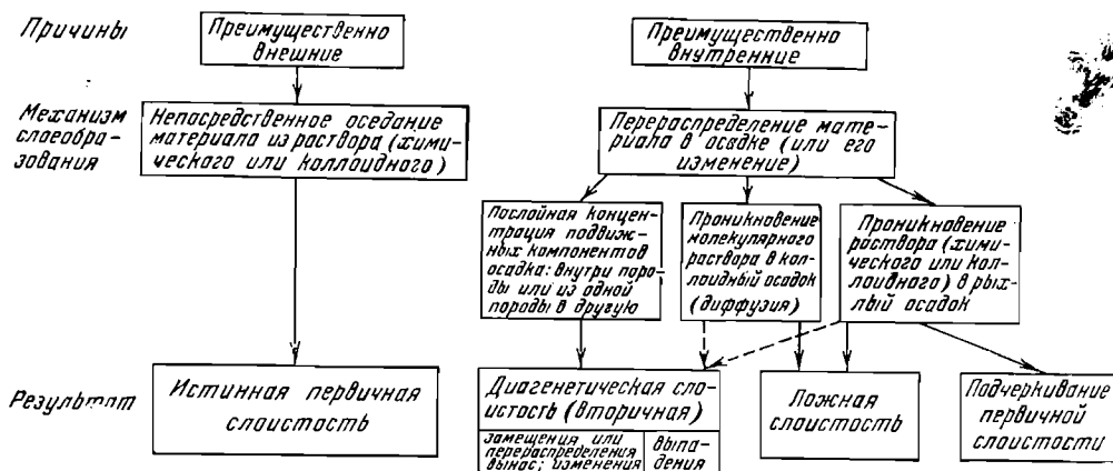
Фиг. 10. Схема зависимости текстуры хемогенных отложений от механизма их образования
