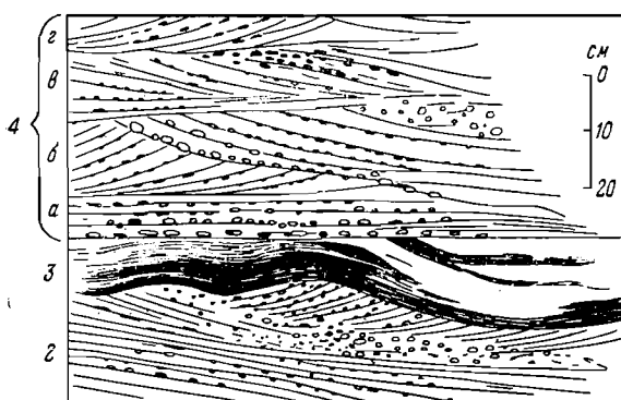
Фиг. 94. Разнонаправленная перекрестная косая слоистость флювиогляциальных песчано-гравийных отложений (2—4 слоя).
