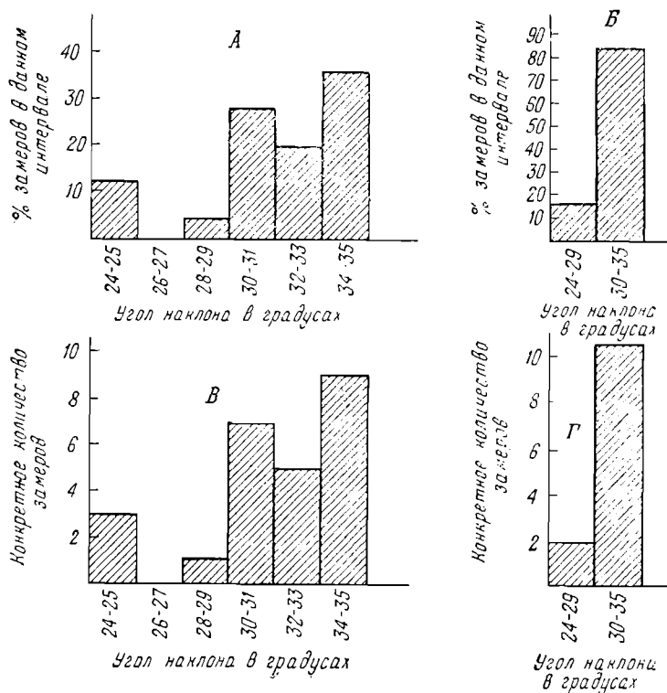
Фиг. 40. Диаграммы, характеризующие распределение слоистости по крутизне косых слойков.
