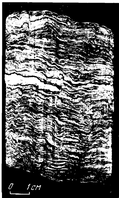
Фиг. 84. Плойчатая изогнутость слоев в листоватой известково-углистой породе, возникшая после седиментации (озерно-болотные отложения). Угленосная толща Донецкого бассейна
