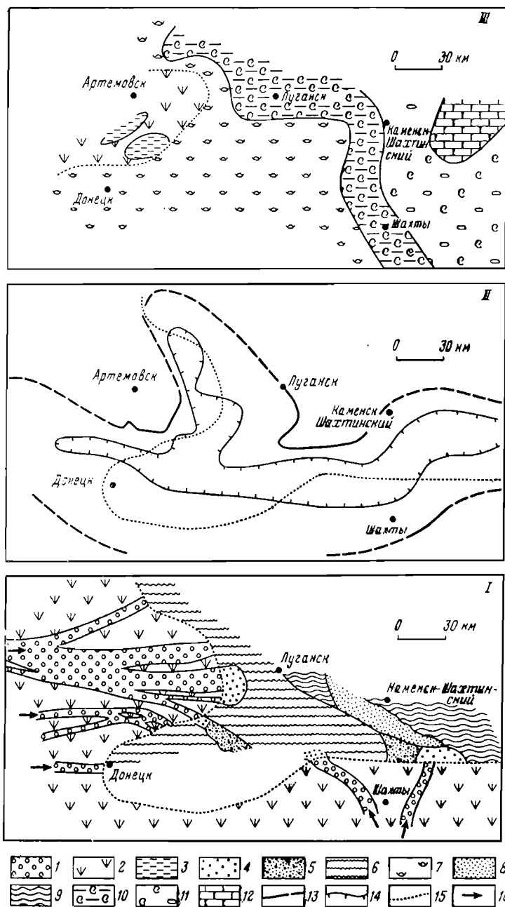
Фиг. 140. Детальные палеогеографические карты, построенные для трех частей угленосного цикла (с угольным пластом) из отложений среднего карбона Донецкого бассейна.
