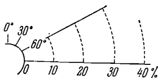
Фиг. 42. Диаграмма, в которой линии концентрических окружностей указывают процент замеров, попадающих в данный сектор. Рядом — пример такой диаграммы (построена Петтиджоном для кварцитов Барабу по 2833 замерам)
