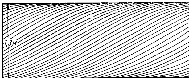
Фиг. 125. Схематическая зарисовка косослоистой серии морских песков.
