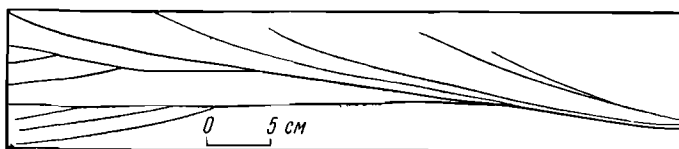
Фиг. 101. Пучковидный характер дельтовой слоистости
