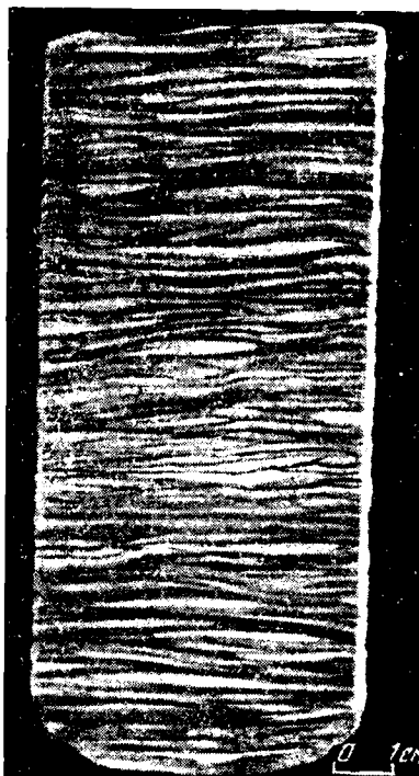
Фиг. 119. Правильная полого-волнистая слоистость; в результате смещения волн образуются линзовидные прослои.
