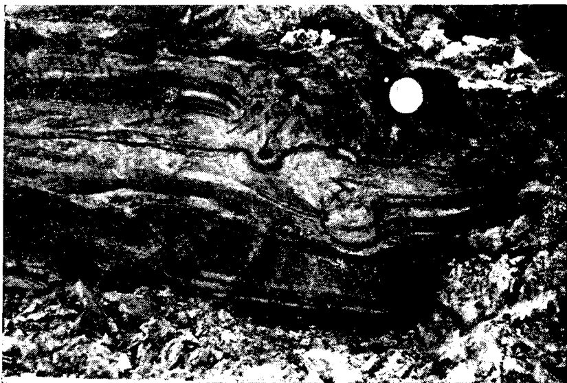
Фиг. 59. Текстура вытаптывания в отложениях современной поймы — субфация заиленной русловой отмели, переходящей в краевую часть старицы (фото А. А. Лазаренко)
