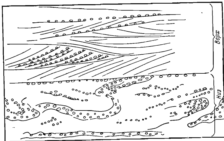
Фиг. 69. Слоистость в нижней части аллювиальных отложений.
