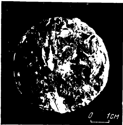
Фиг. 87. Отложения почвы с большим количеством корневых остатков — «кучерявчик» (ниже угольного пласта I 6 , Донецкий бассейн)
