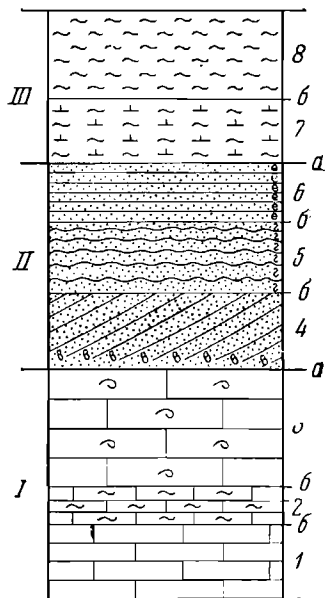
Фиг. 1. Соотношения пластов, слоев и слойков. Пласты обозначены римскими цифрами, слои — арабскими и слойки буквами в, г, е; а — границы пластов, б — границы слоев
