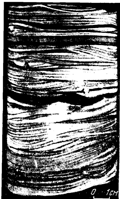
Фиг. 115. Сложная волнистая слоистость (полого-волнистая с мульдобразной) в отложениях зоны волнений. Угленосная толща Донецкого бассейна
