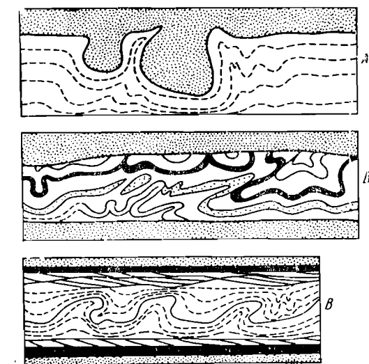
Фиг. 131. Схематическое изображение деформаций слоистости, встречаемых в отложениях мутевых течений (по Кюенену, 1953).
