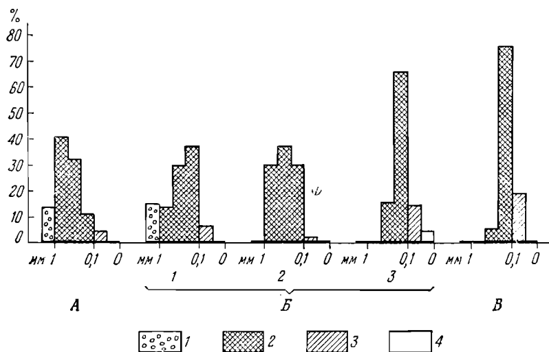
Фиг. 49. Диаграммы структуры осадков:
