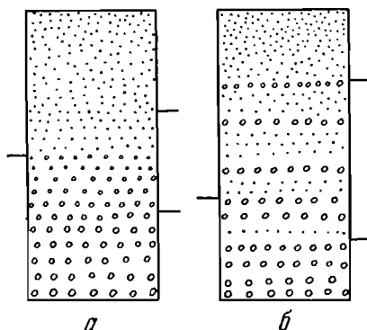
Фиг. 6. Типы постепенных переходов между слоями.
