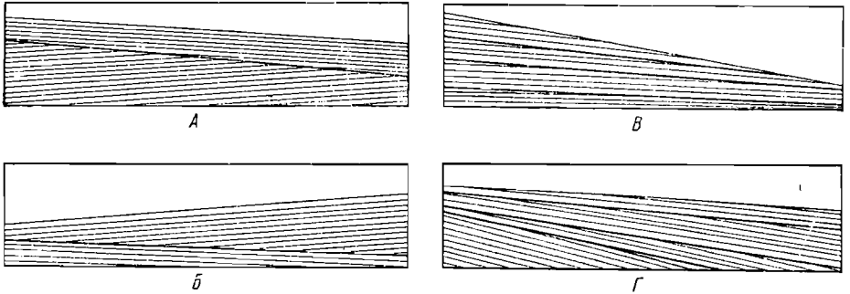
Фиг. 108. Типы косой слоистости бичей (по Томпсону, 1937). Для каждого рисунка море справа. А — Г — см. объяснение в тексте
