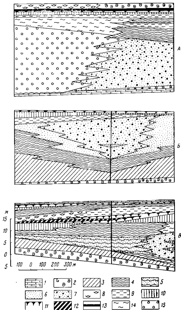
Фиг. 102. Ископаемые дельтовые отложения и их фациальный переход в смежные. Разрезы из угленосной толщи Донецкого бассейна (по Л. Н. Ботвинкиной, 1954 г.).
