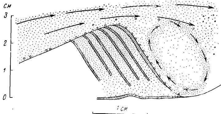
Фиг. 12. Образование косых слоев на переднем, крутом склоне песчаного вала (по А. А. Вейхеру, 1948)
