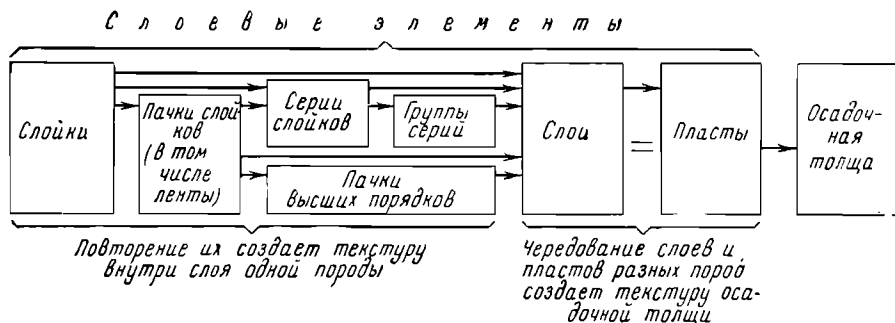
Фиг. 4. Схема соотношения и соподчинения различных элементов слоистой текстуры
