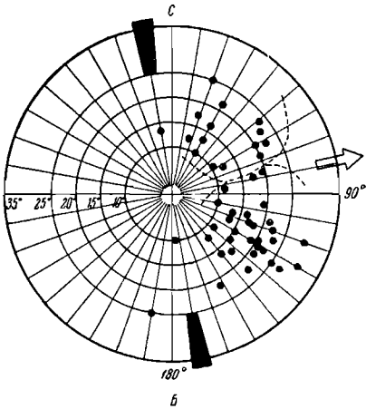
Фиг. 99. Косая слоистость в третичных дельтовых отложениях Японии (по Канэко Сиро, 1958).
