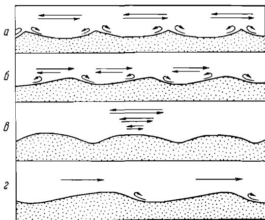
Фиг. 19. Механизм образования ряби (по Кюнелу, 1950).
