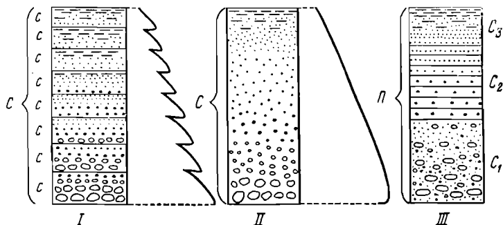
Фиг. 2. Сортировка в различных слоевых единицах.
