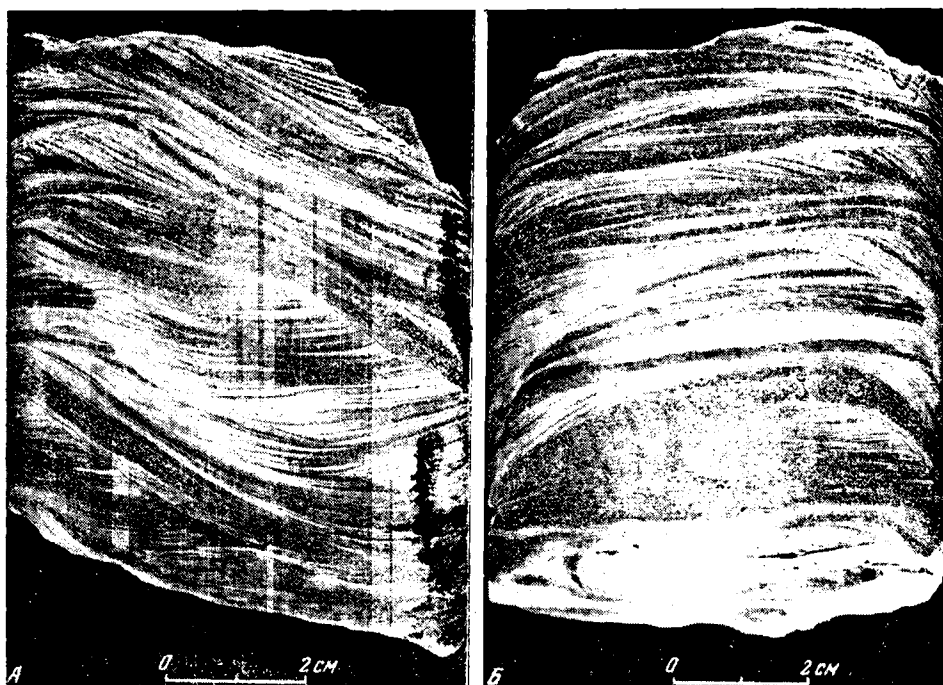
Фиг. 33. Однотипность текстуры в двух взаимно-перпендикулярных плоскостях керна. А — примерно по направлению течения; Б — в направлении, к нему перпендикулярном. Рисунок слоистости несколько отличается, но тип, подтип, вид и разновидности слоистости (косо-волнистая, мелкая, смещенная, однонаправленная, вогнуто-выпуклая) определяются одинаково в обоих срезах
