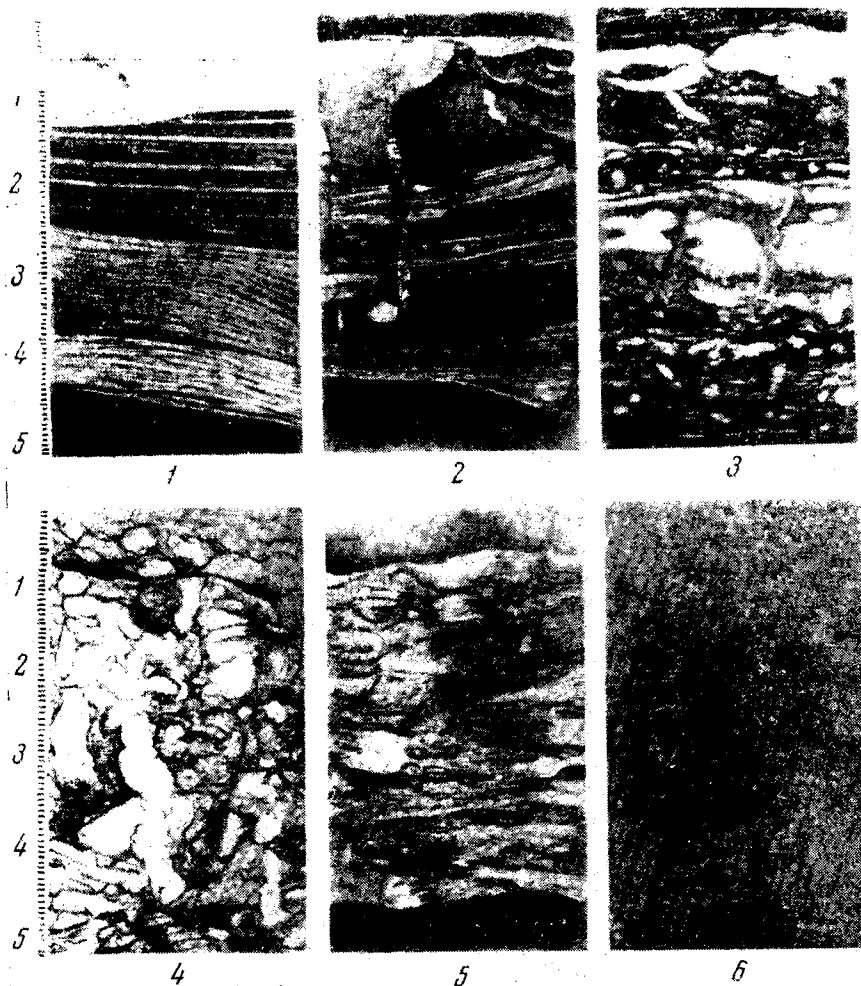
Фиг. 60. Различная степень нарушения слоистости в меловых отложениях Колорадо (по Моору и Скрутону, 1957).
