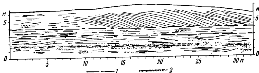
Фиг. 107. Слоистость подводной части литориновой пересыпи (внизу) и вала (по Ульсту, 1957).
