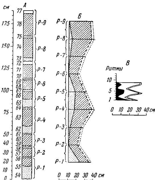
Фиг. 48. Построение ритмограммы для разрезов флишевых толщ и ленточнослоистых отложений (по Н. Б. Вассоевичу, 1948—1949).
