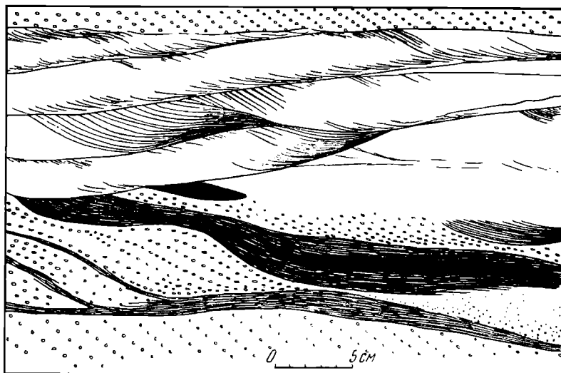
Фиг. 96. Независимость изменения структуры и текстуры во флювиогляциальных отложениях.
