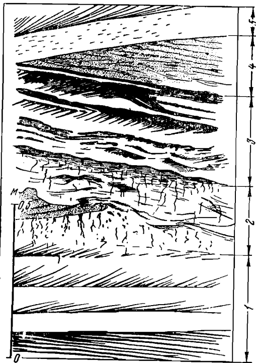
Фиг. 78. Прослои погребенной почвы в современных пойменных отложениях р. Дон.
