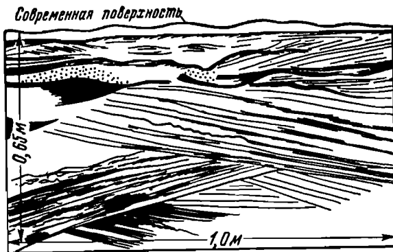
Фиг. 91. Косая разнонаправленная слоистость современных песчаных отложений, образованная временными потоками в крупном овраге. Слоистость подчеркивается глинистыми слойками (черное)
