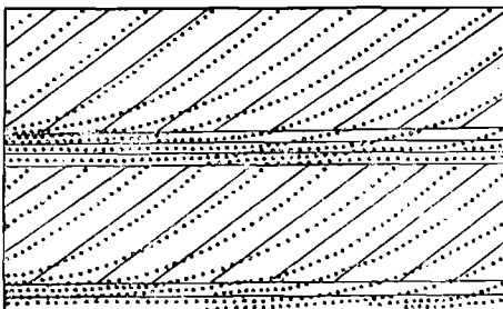
Фиг. 52. Чередование двух систем трещин, создающее на поверхности обнажения впечатление чередования косо- и горизонтальной слоистости в косо-слоистой породе.
