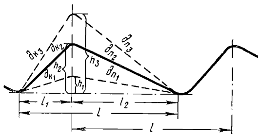
Фиг. 22. Величины, определяющие рябь
