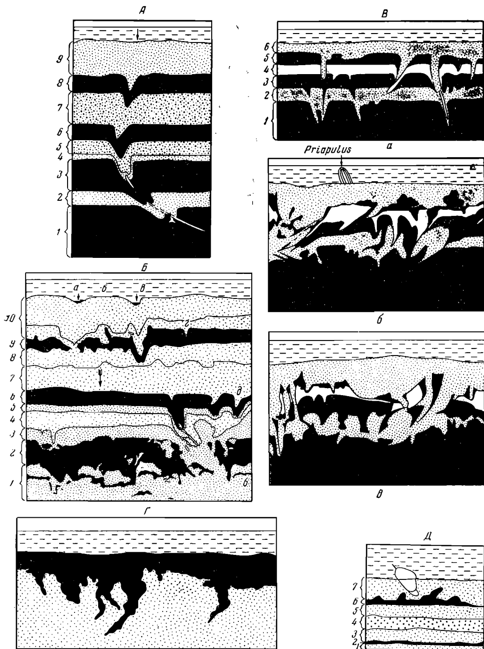
Фиг. 61. Опыты по нарушению слоистости зарывающимися животными (по И. К. Королук, 1958).
