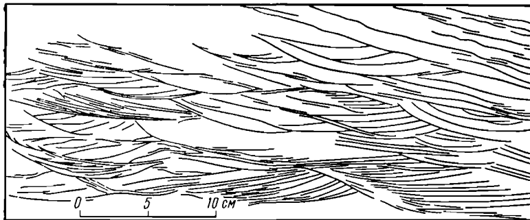
Фиг. 31. Точная копия слоистости, снятая на кальку прямо с поверхности обнажения и затем уменьшенная фотографированием. Слоистость волнистая, асимметричная и косо-волнистая в четвертичных прибрежно-морских отложениях у с. Маныч-Балабинский
