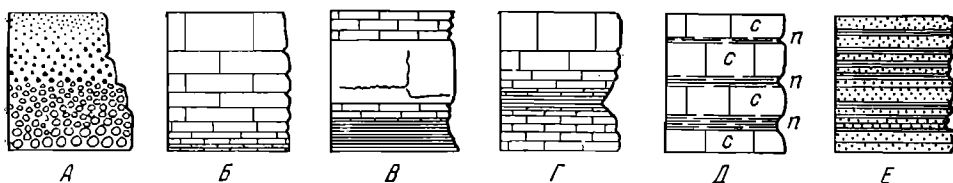
Фиг. 27. Различный характер изменения наложения.
