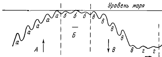
Фиг. 134. Кривая, отражающая цикличность разных порядков.
