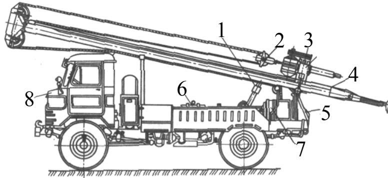
Рис. 2.11. Установка АВБ-2М: 1 – винтовой подъемник мачты; 2 – талевый блок; 3 – вибромолот; 4 – мачта; 5 – опора мачты; 6 – генератор; 7 – лебедка; 8 – автомобиль
