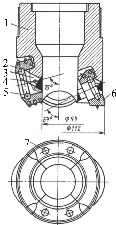
Рис. 3.32. Конструкция шарошечной коронки 6ДК 112К: 1 – корпус кольцевой формы; 2 – внутренняя шарошка (формирующая керн); 3 – замковый палец; 4 – штифт-фиксатор; 5 – замковый шариковый подшипник; 6 – наружная шарошка (формирующая ствол скважины); 7 циркуляционные каналы
