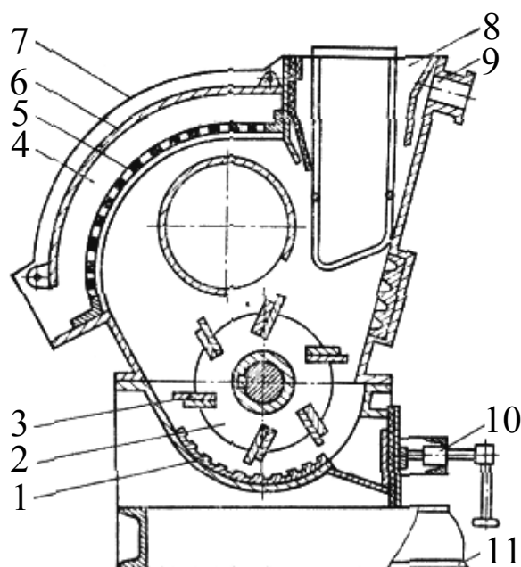
Рис. 4.5. Фрезерно-струйная мельница типа ФСМ: 1 – диспергирующая рифленая плита; 2 – лопастной ротор; 3 – лопасть; 4 – лоток; 5 – выходная решетка; 6 – отражательный щиток; 7 – борт; 8 – приемный бункер; 9 – патрубок для подачи воды; 10 – механизм открывания и закрывания крышки ловушки; 11 – рама
