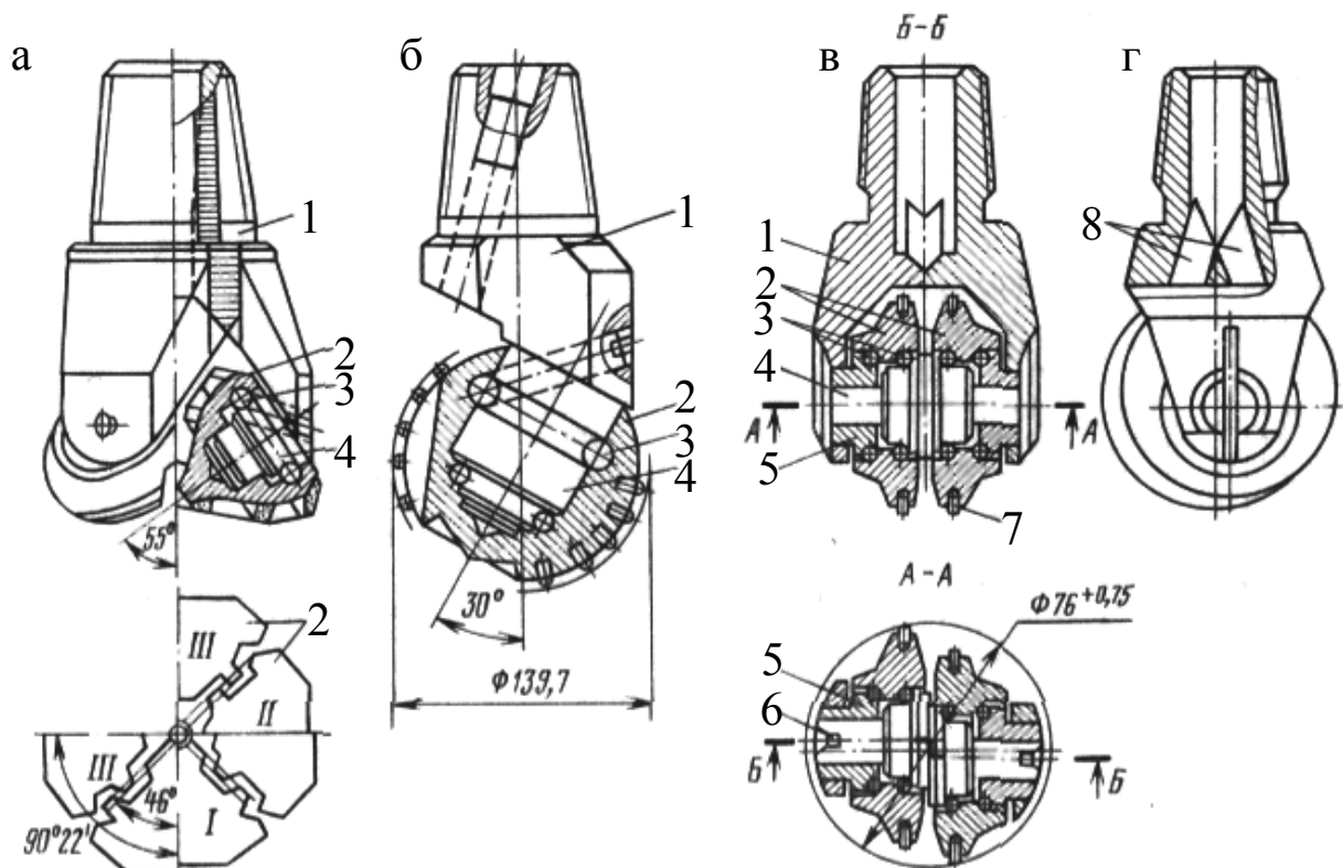
Рис. 3.30. Конструкции долот для бурения в породах средней твердости с шарошками конусной а, сферической б и дисковой в форм: 1 – корпус; 2 – шарашки; 3 – шариковые подшипники; 4 – цапфа; 5 – втулка; 6 – призматическая шпонка; 7 – твердосплавная вставка (штырь); 8 – промывочные каналы
