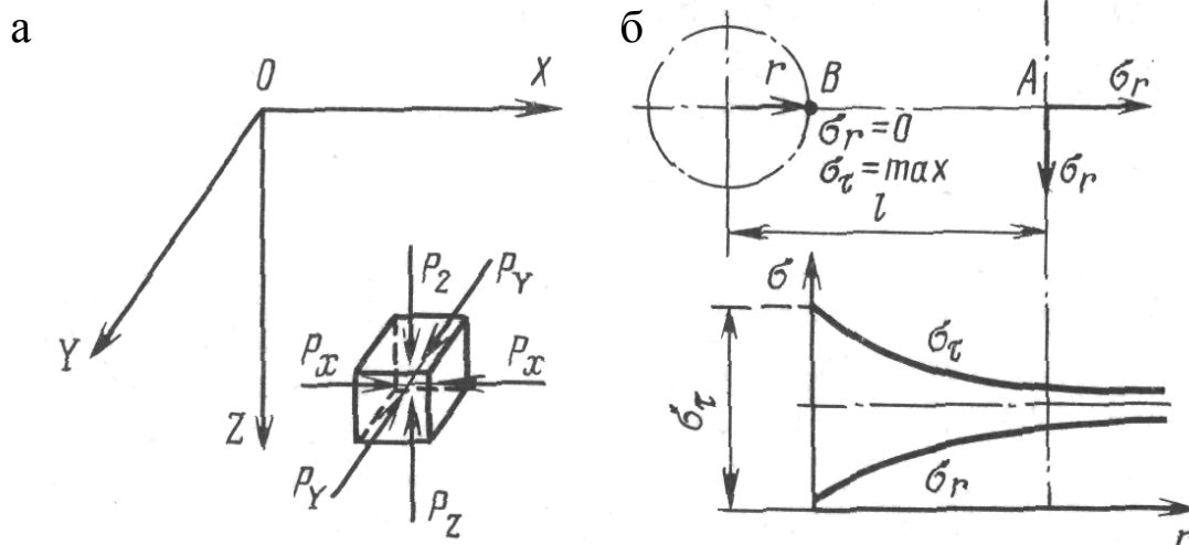
Рис. 1.10. Схемы к расчету устойчивости горных пород в стенках скважины
