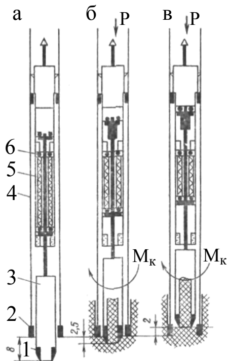
Рис. 2.24. Кинематическая схема работы кернаприемника «Конус»: а – в ненагруженном состоянии перед бурением угольного пласта, опережение штампа 8 мм; б – во время бурения пласта штампованием, опережение штампа 2,5 мм; в – при заклинивании керна, штамп отстает от алмазной коронки на 2 мм; 1 – штамп; 2 – алмазная коронка; 3 – контейнер; 4 – колонковый набор комплекса КССК-76; 5 – пружинный регулятор; 6 – подшипники; P – осевая нагрузка; M_k – крутящий момент
