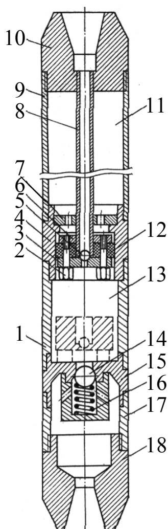
Рис. 4.8. Тампонажное устройство ТСТ-1ГВ: 1, 9 – корпуса смесительной камеры и устройства; 2 – болт; 3, 6 – шайба ниппеля и верхняя; 4, 17 – ниппели; 5 – шарик; 7 – дозатор; 8 – центральная труба; 10, 18 – переходники верхний и нижний; 11 – контейнер; 12 – уплотнительная манжета; 13 – смесительная камера; 14 – шарик; 15 – обойма обратного клапана; 16 – пружина
