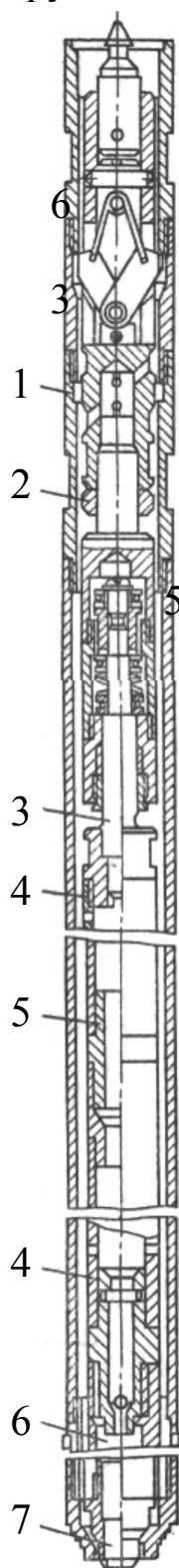
Рис. 2.23. Съемный керноприемника «Конус»: 1 – головка-фиксатор; 2 – гайка; 3 – регулятор; 4 – удлинитель; 5 – ниппель; 6 – контейнер; 7 – штамп
