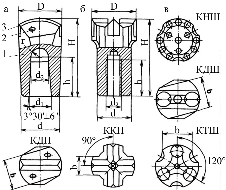
Рис. 3.11. Буровые коронки: а – с конусным отверстием; б – с резьбовым отверстием; в – вид с торца типов КПД; ККП; КНШ; КДШ; КТШ (размеры, мм: D – диаметр головки, d – диаметр корпуса, d_3 – диаметр резьбы, H – высота коронки, h_1 – длина резьбы, b – толщина лезвия)
