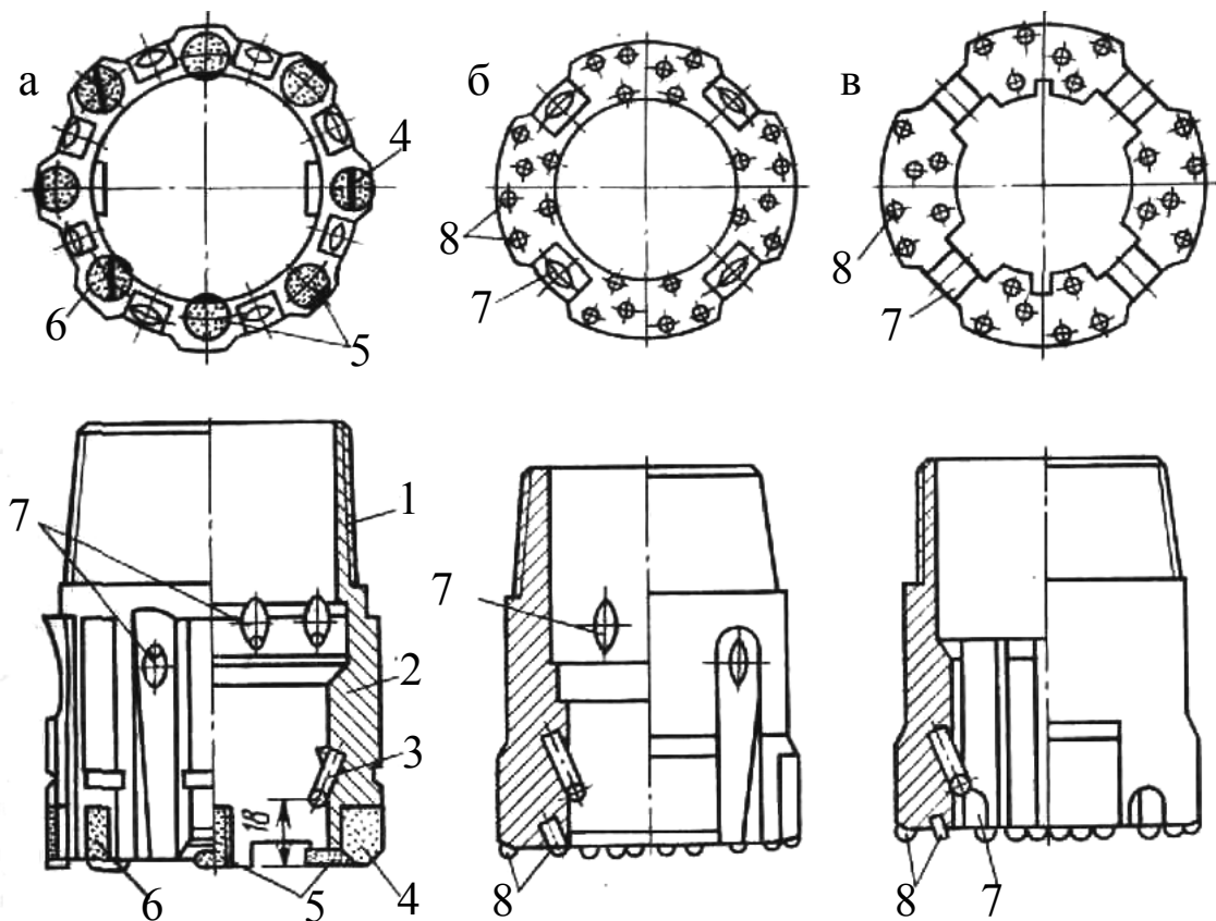
Рис. 3.6. Конструкции долот для ударно-вращательного бурения с пневмоударником: а – КДП; б – КДП-М; 1 – соединительная резьба; 2 – корончатое кольцо; 3 – скоба кернователя; 4, 5, 6, 8 – твердосплавные вставки различной формы; 7 – циркуляционные окна
