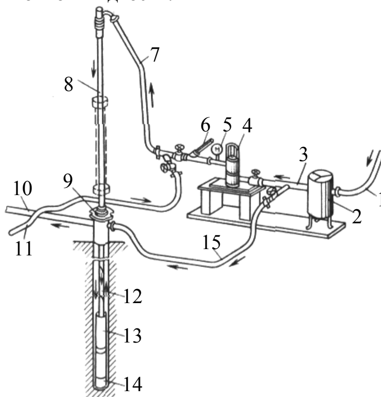
Рис. 4.3. Схема циркуляционной системы при бурении с продувкой скважины воздухом: 1,3,7,15 – нагнетательная линия (от компрессора); 2 – маслоотделитель; 4 – расходомер; 5 – манометр; 6 – термометр; 8 – буровые трубы; 9 – герметизирующее устройство; 10 – выкидная линия; 11 – водонапорная линия (от насоса); 12 – циркуляционный канал в буровых трубах; 13 – шламоулавливающая труба; 14 – коронка
