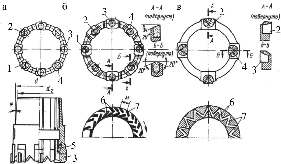
Рис. 3.5. Конструктивные элементы коронок для ударно-вращательного бурения с пневмоударником: 1, 2, 3, 4 – вставки; 5 – скоба кернорвателя; 6 – элементы породы скалываемые при ударе; 7 – линии контакта лезвия вставки с породой забоя
