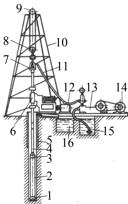
Рис. 2.1. Принципиальная схема колонкового бурения с прямой промывкой: 1 – породоразрушающий инструмент; 2 – колонковая труба; 3 – переходник; 4 – бурильные грубы; 5 – обсадные трубы; 6 – буровой станок; 7 – вертлюг-сальник; 8 – талевый блок; 9 – кронблок; 10 – вышка; 11 – напорный шланг; 12 – электродвигатель станка; 13 – насос; 14 – электродвигатель насоса; 15 – всасывающий шланг; 16 – отстойники
