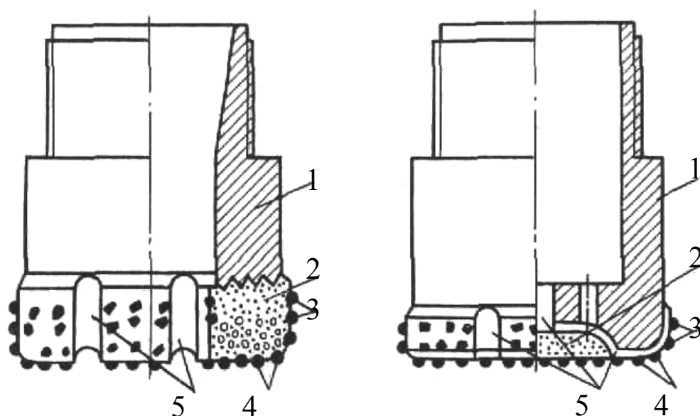
Рис. 3.33. Конструктивные элементы алмазных буровых инструментов: а – коронка; б – долото; 1 – корпус; 2 – матрица; 3 – подрезные резцы; 4 – торцовые резцы; 5 – циркуляционные каналы
