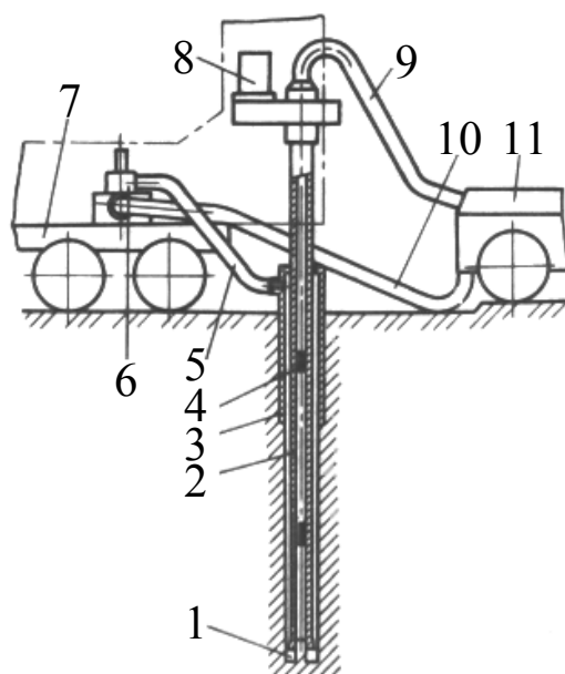
Рис. 2.2. Принципиальная схема колонкового бурения с гидротранспортом керна: 1 – породоразрушающий инструмент; 2 – буровые трубы; 3 – обсадные трубы (кондуктор); 4 – транспортируемый керн; 5 – нагнетательный циан; 6 – насос; 7 – буровая установка; 8 – врата геля; 9 – отводной шланг; 10 – всасывающий шланг; 11 – кернаприемное устройство с емкостью для промывочной жидкости
