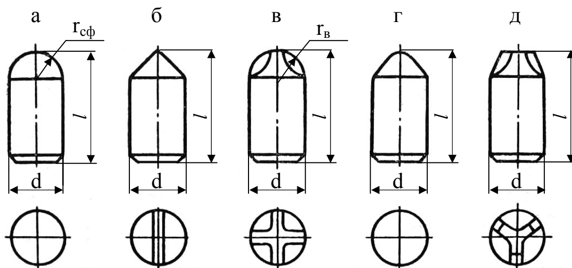
Рис. 3.24. Формы головок штырей: а – сферическая; б – клиновидная; в – лучевая; г – параболоидная; д – трехгранная
