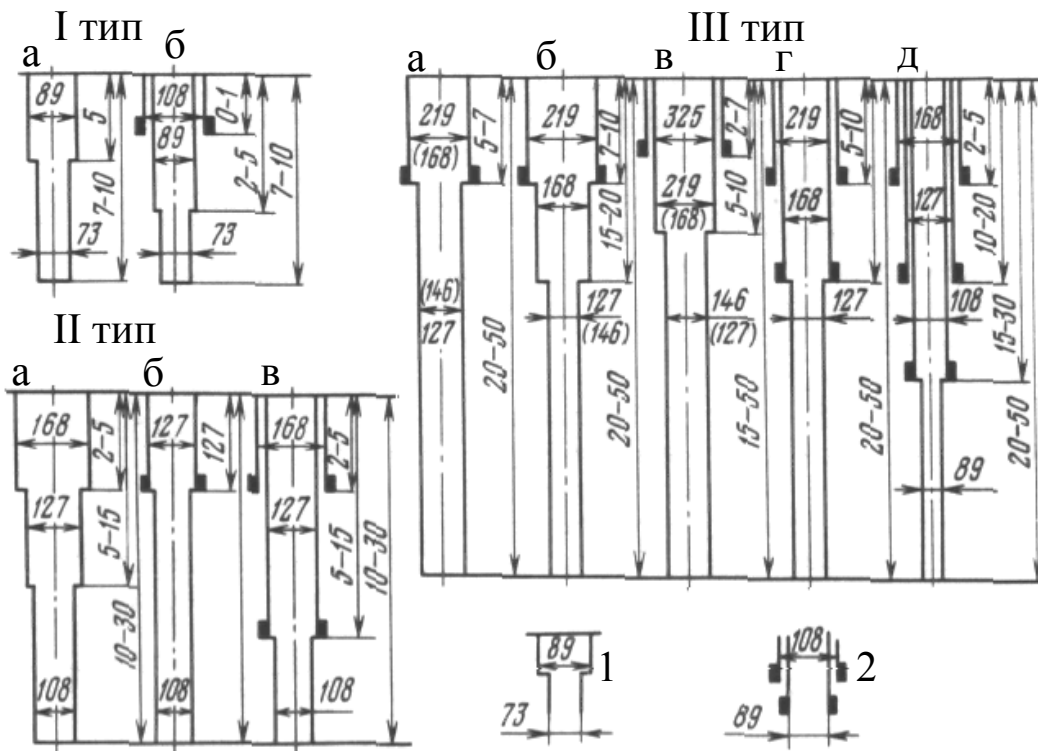
Рис. 1.7. Типовые конструкции инженерно-геологических скважин малого диаметра: а, б, в, г, д – группы скважин; 1 – скважины или части скважин, бурение которых осуществляется без крепления обсадными трубами; 2 – то же, с креплением обсадными трубами
