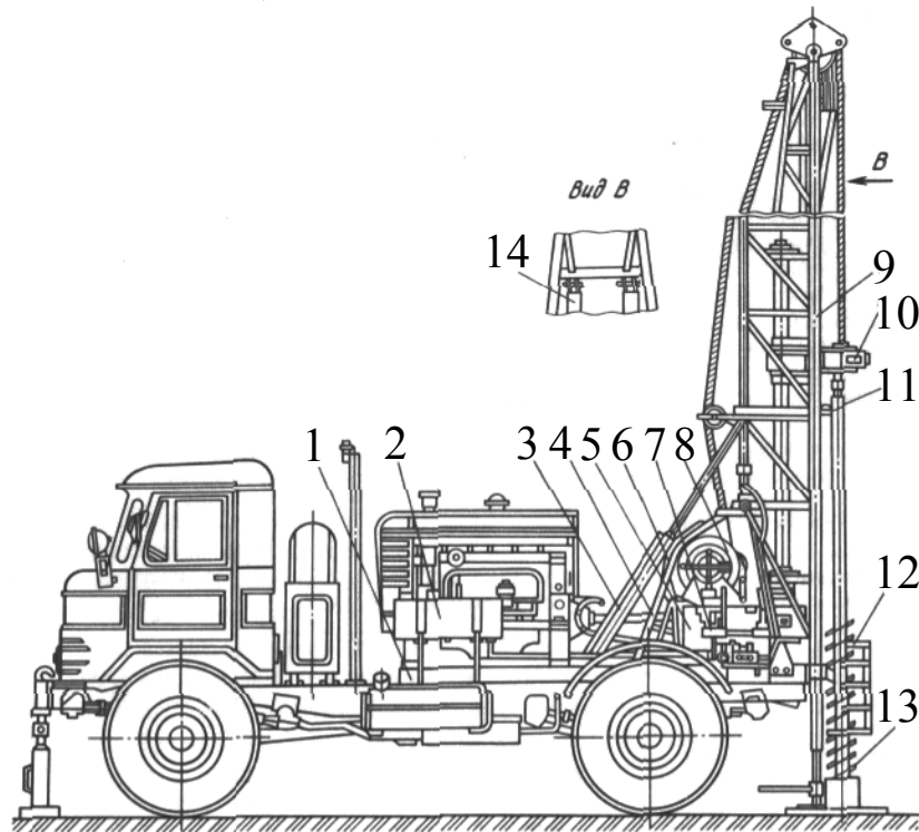
Рис. 2.14. Установка для гидрогеологического бурения УГБ-50М: 1 – рама; 2 – двигатель; 3 – гидродомкраты опускания и подъема мачты; 4 – ударный механизм; 5 – коробка передач; 6 – тормоза; 7 –
