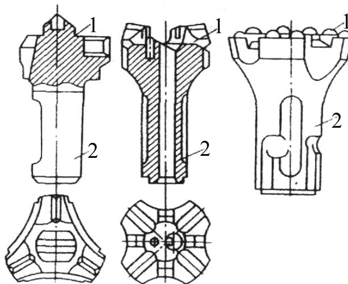
Рис. 3.10. Долота для ударно-вращательного бурения: а – К100В и БК-155; б – К105КА и К-130К; в – КНШ-110
