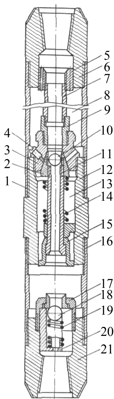
Рис. 4.7. Универсальный тампонажный снаряд УТС-2М
