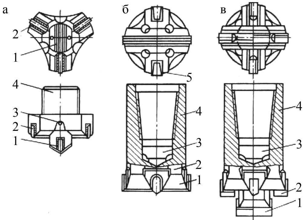
Рис. 3.7. Конструкции долот для ударно-вращательного бурения с гидроударниками: 1 – центральная вставка; 2 – боковые вставки; 3 – циркуляционные каналы; 4 – корпус; 5 – калибрующие вставки
