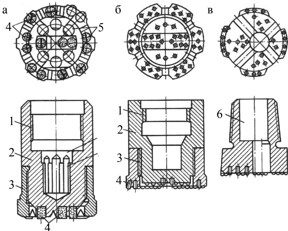
Рис. 3.8. Конструкции долот для ударно-вращательного бурения с пневмоударниками: 1 – присоединительная резьба; 2 – корпус долота; 3 – кольцо; 4 – вставки; 5, 6 – циркуляционные каналы
