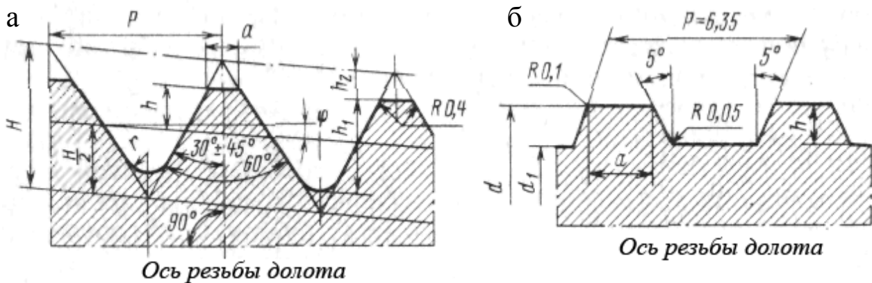
Рис. 3.26. Профили резьбы шарошечных долот: а – конической; б – трапецеидальной
