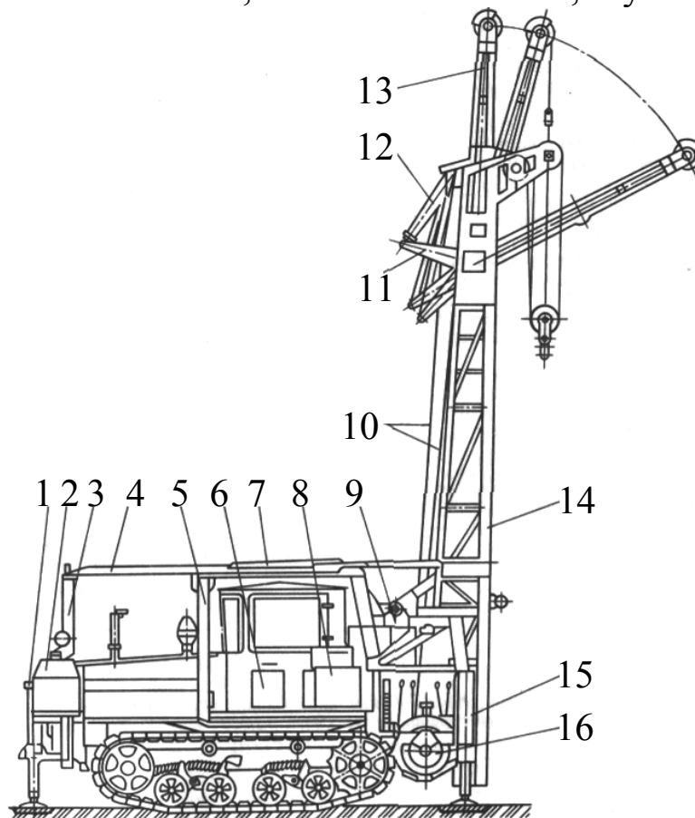
Рис. 2.15. Самоходная вибробуровая установка ВАС-75: 1 – передняя гидравлическая опора; 2 – топливный бак; 3 – передняя рама; 4 –
