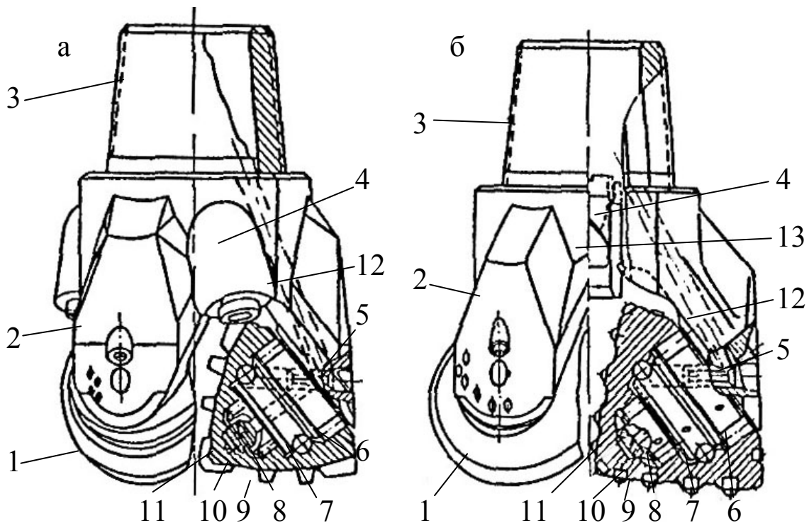
Рис. 3.17. Конструктивные схемы трехшарошечных долот: а – зубчатого с фрезерованным вооружением шарошек и периферийной
