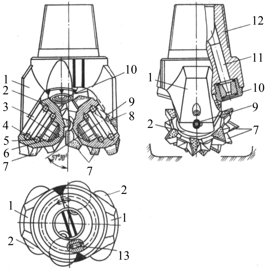
Рис. 3.29. Конструктивные элементы долота для бурения в мягких породах с гидромониторными насадками: 1 – лапа; 2 – шарошка; 3 – цапфа; 4 – шариковый замковый подшипник; 5 – шариковый промежуточный подшипник; 6 – роликовый концевой подшипник; 7 – зубья шарошки; 8 – штифт-фиксатор; 9 – замковый палец; 10 – гидромониторная насадка; 11 – промывочный канал; 12 – присоединительная резьба; 13 – ориентирующий штифт
