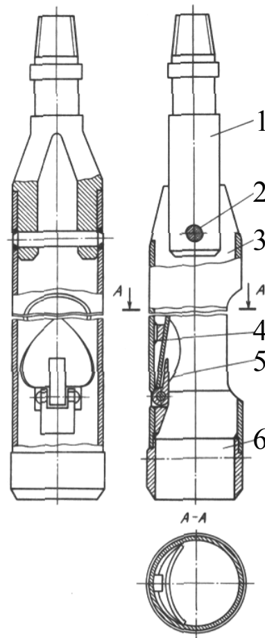
Рис. 3.1. Устройство вибронзонда с клапаном: 1 – переходник; 2 – палец; 3 – корпус; 4 – упор; 5 – клапан; 6 – рабочее кольцо
