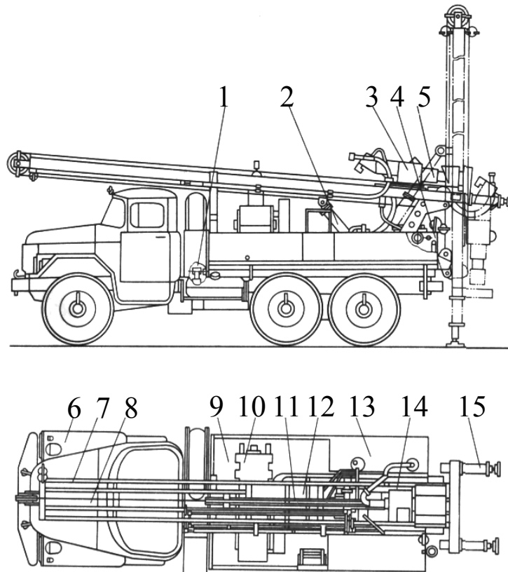
Рис. 2.16. Буровая установка УРБ-2А-2: а – вид сбоку; б – вид сверху; 1 – коробка отбора мощности; 2 – цилиндр подъема мачты; 3 – вращатель; 4 – пульт управления; 5 – элеватор для труб и патрон для шнеков; 6 – автомобиль; 7 – мачта; 8 – талевая система; 9 – рама;
