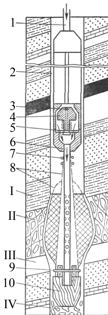
Рис. 4.9. Схема установки устройства перекрытия горных выработок УПГВ-1: I, III – соответственно кровля и почва горной выработки; II – горная выработка; IV – забой скважины; 1 – буровая труба; 2 – снаряд УТС-2М; 3 – шарик; 4 – клапан смесителя; 5 – смесительная камера; 6 – перфорированная труба; 7 – резиновое кольцо; 8 – эластичная оболочка; 9 – алюминиевая шпилька; 10 – пробка-центратор
