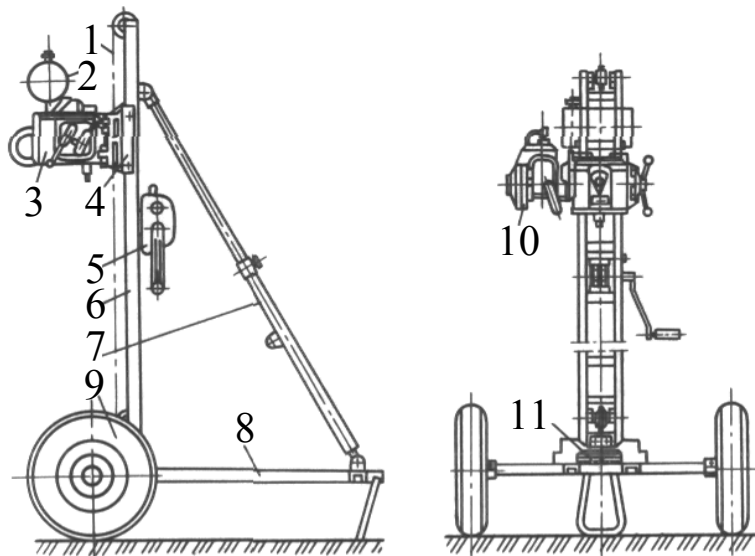
Рис. 2.8. Установка УКБ-12/25: а – вид сбоку; б – вид спереди; 1 – цепь; 2 – бензобак; 3 – вращатель; 4 – каретка; 5 – лебедка; 6 – стойка; 7 – подкос; 8 – рама; 9 – колеса; 10 – двигатель; 11 – центратор
