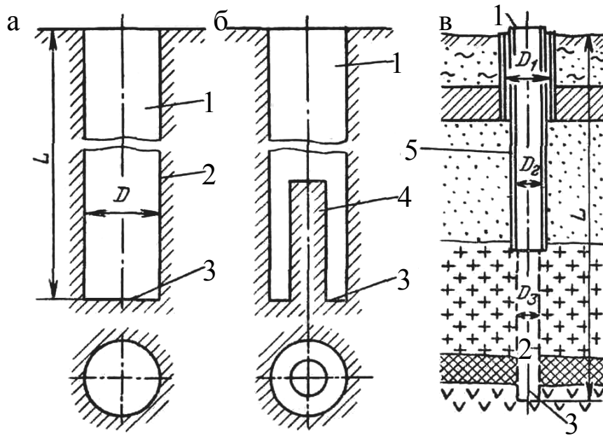
Рис. 1.6. Элементы буровой скважины: а – при бескерновом бурении; б – при колонковом бурении; в – элементы скважины; 1 – устье; 2 – стенки; 3 – забой; 4 – керн; 5 – стенки скважина, закрепленные обсадными трубами; L – длина скважины; D , D_1 , D_2 , D_3 – диаметры ствола скважины
