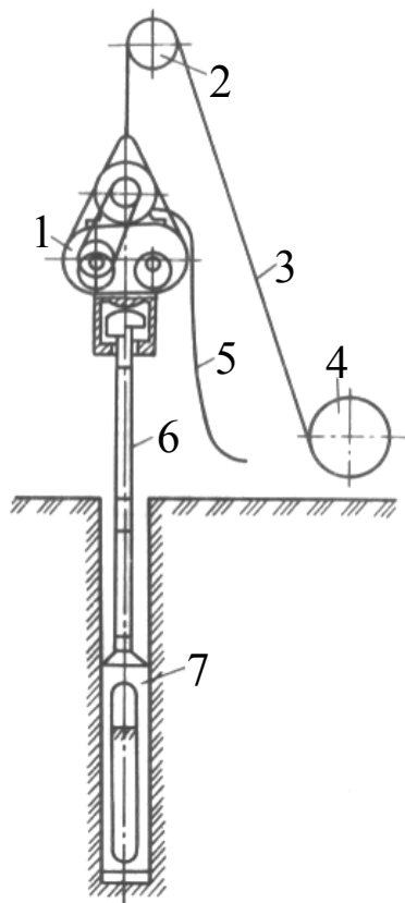
Рис. 2.4. Принципиальная схема ударно-вибрационного бурения: 1 – беспружинный вибромолот; 2 – блок мачты; 3 – канат; 4 – лебедка бурового агрегата; 5 – электрический кабель; 6 – буровые трубы (штанги); 7 – вибронзонд
