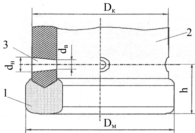
Рис. 3.39. Коронка с конусными промывочными каналами: 1 – матрица; 2 – корпус коронки; 3 – промывочный канал; D_M , D_K – наружные диаметры матрицы и коронки; d_H – наружный диаметр отверстия; d_B – внутренний диаметр отверстия; h – расстояние от торца матрицы до осевой линии промывочных каналов
