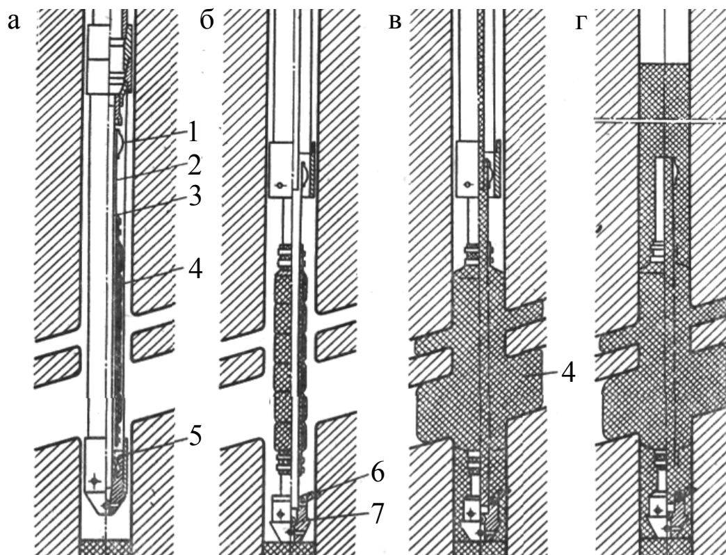
Рис. 4.10. Схема работы устройства перекрытия зон поглощений типа УПП: а – в транспортном положении в зоне выработки; б – закрепление устройства в стволе скважины и подъем его корпуса на высоту оболочки; в – закачивание наполнителей и тампонирующих смесей; г – освобождение бурильной колонны и корпуса УПП от устройства перекрытия; 1 – фонарь; 2, 3 – центральные трубы; 4 – высокопрочная ячеистая капроновая оболочка; 5 – предохранительный башмак; 6 – закрепляющее устройство; 7 – шар
