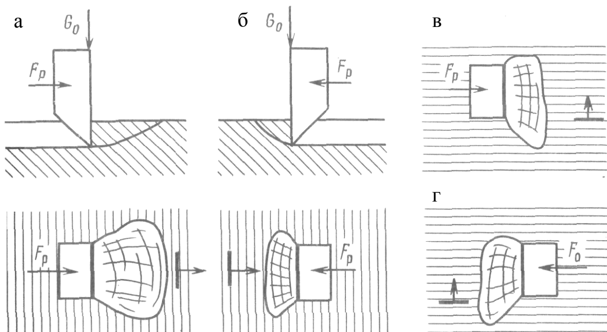
Рис. 1.9. Схемы разрушения анизотропной породы при введении резца
