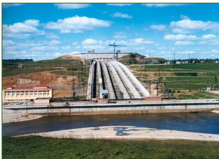
Рис. 1 Общий вид Загорской ГАЭС
