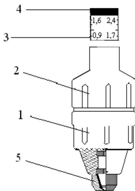
Рис. 2. Ареометр АБР-1:
