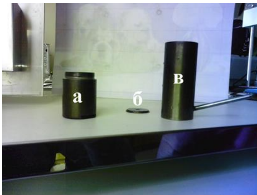
Рис. 8. Комплектация реторты: а) нижняя камера; б) крышка с отверстием для нижней камеры реторты; в) верхняя камера.
