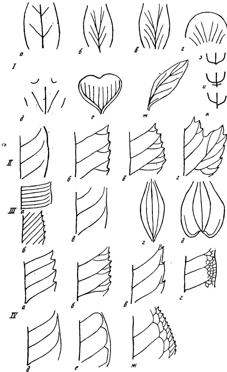
Рис. 2. Типы жилкования
