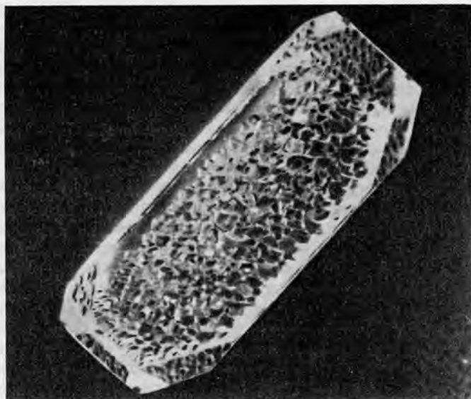
Рис. 3.2. Выращенный гидротермальным методом синтетический кристалл кварца с характерной бугристой поверхностью (похожей на галечную или булыжную мостовую), которая никогда не наблюдается у природного кварца.
