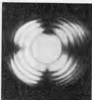
Рис. 8.1. Интерференционная фигура, наблюдаемая в полярископ с сильной собирающей линзой, введенной между верхним анализатором и образцом. Фигура характерна только для кварца.
