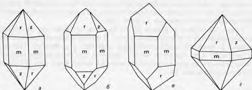
Рис. 2.1. Призматический габитус кристаллов кварца: r и z — грани ромбоэдров, m — грани призмы; a — гексагональный призматический кристалл, оканчивающийся развитыми в равной мере положительным и отрицательным ромбоэдрами; б — преобладает положительный ромбоэдр r ; в — развит только положительный ромбоэдр r ; г — одинаково развиты грани положительного и отрицательного ромбоэдров с коротким призматическим поясом (иногда призма вообще отсутствует).
