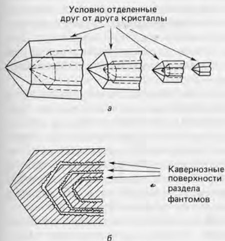
Рис. 7.1. Схематическое изображение серии «чашечных» кристаллов кварца, условно выдвинутых друг из друга (а). Поперечный разрез цельного «чашечного» кристалла, на котором видны поверхности раздела фантомов; по этим поверхностям кристалл можно разрезать на части (б).
