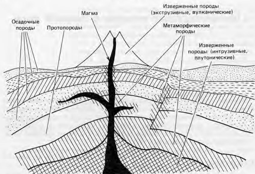
Рис. 1.1. Схема относительного расположения изверженных, осадочных и метаморфических пород. Кварц широко распространен в изверженных и метаморфических породах. Осадочные и изверженные породы рассекаются кварцосодержащими жилами.
