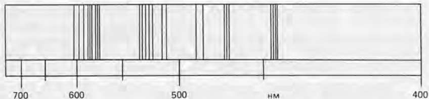
Рис. 8.3. Спектр редкоземельных элементов (дицима), наблюдающийся для желтого апатита.
