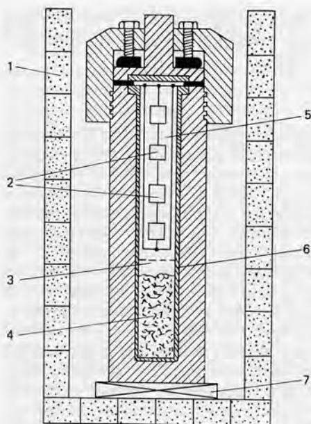
Рис. 3.1. Футерованный серебром автоклав, или «бомба», для гидротермального выращивания кварца. 1 – термоизоляция; 2 – затравочные пластинки; 3 – дырчатая перегородка; 4 – исходный материал (шихта); 5 – обогащенный кремнеземом водный раствор; 6 – серебряная футеровка; 7 – электрический нагреватель.
