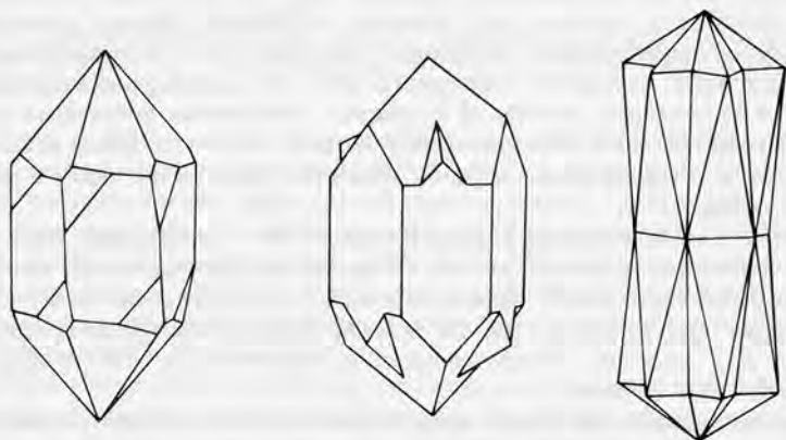
Рис. 2.6. Примеры двойникования по дофинейскому закону.
