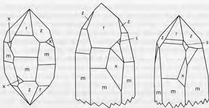
Рис. 2.3. Разновидности призматических кристаллов с развитыми зонами тригонального трапецоэдра и ромбоэдров: m – призма, r – положительный ромбоэдр, z – отрицательный ромбоэдр, x – тригональный трапецоэдр, s – тригональная пирамида.
