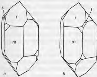
Рис. 2.2. Энантиоморфизм кристаллов кварца. В левостороннем кристалле (а) тригональная пирамида s примыкает к верхнему левому углу призматической грани m ниже грани положительного ромбоэдра r . В правостороннем кристалле (б) расположение граней зеркально-противоположное.
