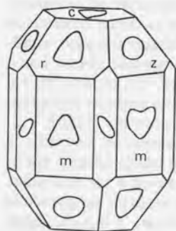
Рис. 4.1. Идеализированное изображение фигур удара, образующихся на различных гранях кристалла кварца.
