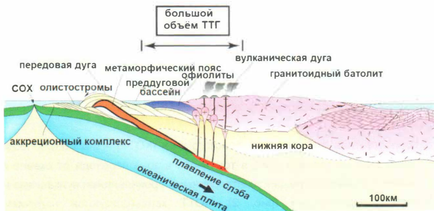
Рис. 2. Конвергентная окраина западно-тихоокеанского типа и ее основные элементы: зона субдукции, субдуктирующая океаническая плита, аккреционный комплекс, передовая дуга с преддуговым бассейном, вулканическая дуга, задуговой бассейн. Рисунок по работе Maruyama et al. (2011). На КОТТ восточной Пацифики отсутствует задуговой бассейн
