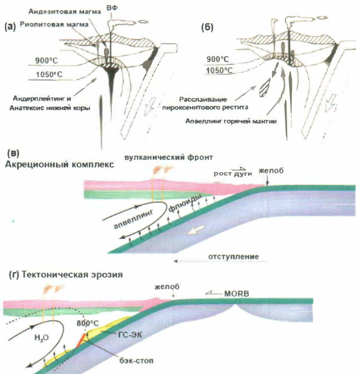
Рис. 14. Нужна ли деламинация мафической нижней коры для объяснения уменьшения ее мощности? Если островодужный андезит образуется при 20-30% частичном плавлении островодужного базальта, андерплетированного на глубину Мохо (а), рестит на границе Мохо должен деламинироваться и погружаться в мантию (б), из-за образования переутолщенной нижней коры в этом процессе (Nakajima and Arima, 1998; Tatsumi, 2000). Если интенсивная тектоническая эрозия обычна, как это видно сейчас вдоль сокращающихся плитных границ во всем мире, и как это было в прошлом Японских островов со времени 520 млн лет (в-г), в деламинации мафической нижней коры нет необходимости
