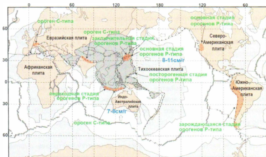
Рис. 9. Карта мира, показывающая районы продолжающейся орогении на разных стадиях вдоль основных конвергентных границ плит (по Maruyama et al., 2007, 2010). Показаны примеры складчатых поясов, сформированных на разных стадиях орогении тихоокеанского или Р-типа (Pacific). Орогены С-типа – коллизионные (collisional) – показаны для сравнения
