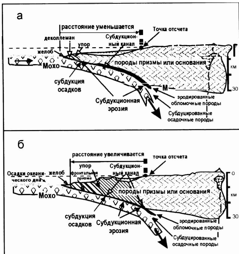
Рис. 17. Схема тектонической эрозии: аккрецирующие и эродирующие конвергентные окраины тихоокеанского типа (Scholl and van Huene, 2007). Деколлеман – поверхность срыва
