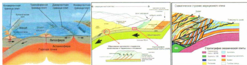
Рис. 3. Структурные элементы орогении тихоокеанского типа (слева), модель образования аккреционного комплекса (посередине) и строение аккреционного комплекса (справа), реконструированное для пояса Мино-Тамба, о. Хонсю, Япония, справа (Wakita, 2012). См. также рис. 25
