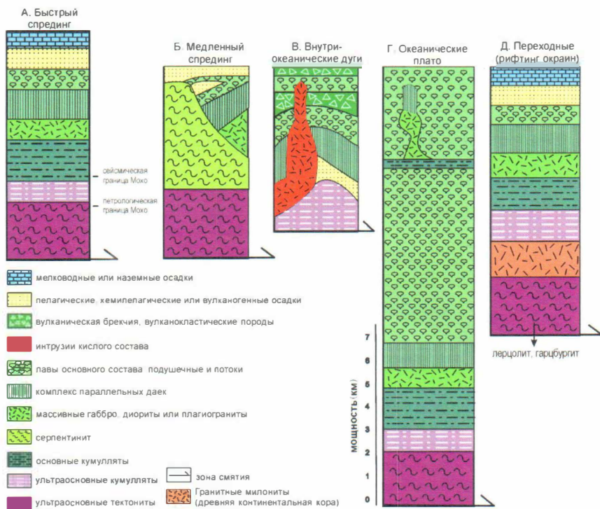
Рис. 22. Различные виды офиолитов (рисунок из Kusky et al., 2011, 2013). А – типичные офиолиты по определению Пенроуз (Колман, 1979), образованные в условиях быстрого спрединга; Б – офиолиты, образованные при медленном спрединге; В – офиолиты внутриокеанических дуг; Г – офиолиты океанических островов и плато; Д – офиолиты, образованные при рифтинге континентальных окраин
