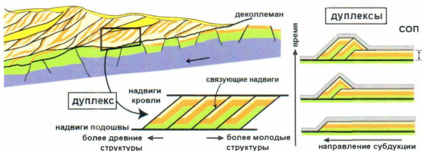
Рис. 26. При гравитационном оползании породы СОП могут образовывать олистостромы. Продолжающаяся аккреция приводит к образованию дуплекс структур (б), по направлению напластования которых можно определить направление древней субдукции (рисунок из Maruyama et al., 2010)
