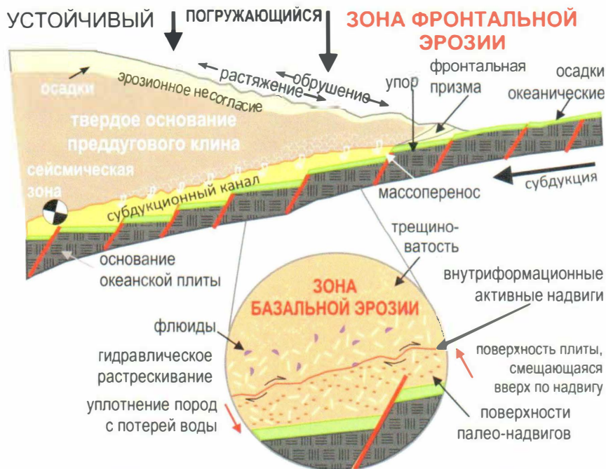
Рис. 19. Механизм тектонической эрозии, т.е. разрушение океанического слэба, островных дуг, аккреционной призмы и фронтальной дуги в результате надвигообразования, воздействия рельефа океанического дна и гидравлического растрескивания (von Huene et al., 2004)
