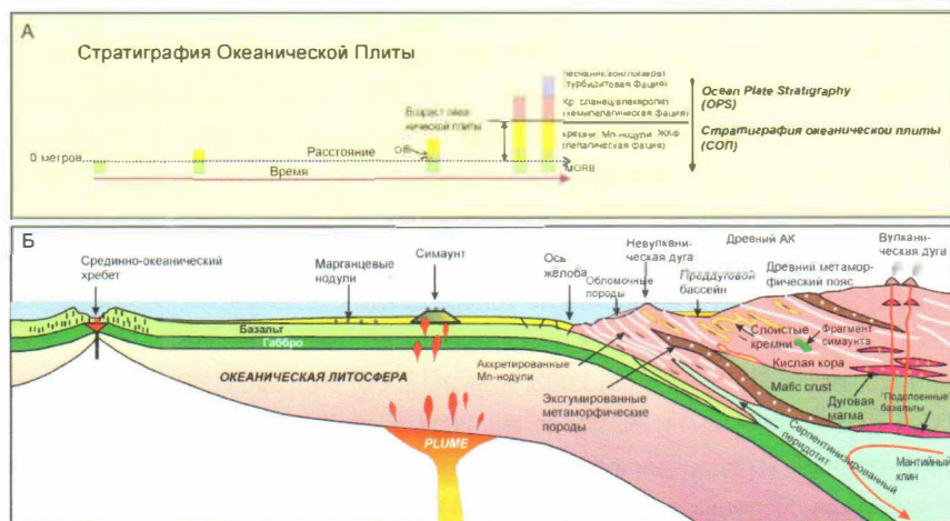
Рис. 21. Общая модель стратиграфии океанической плиты (СОП): от зарождения океанической коры в зоне срединно-океанического хребта до ее субдукции в зоне глубоководного желоба (Santosh, 2010)
