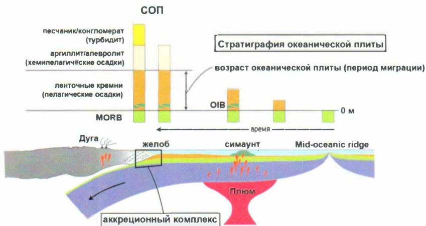
Рис. 23. Развитие СОП с ростом океанической коры и ее возрастом: океаническая плита слева от СОХ покрывается глубоководными ленточными кремнями, затем проходит над горячей точкой с образованием над ней симаунтов. С возрастом океаническая кора покрывается все более мощными пелагическими кремнями и затем, ближе к глубоководному желобу, хемипелагическими осадками (алевролит, аргиллит, сланец). В зоне желоба отложения СОП «запечатываются» турбидитами
