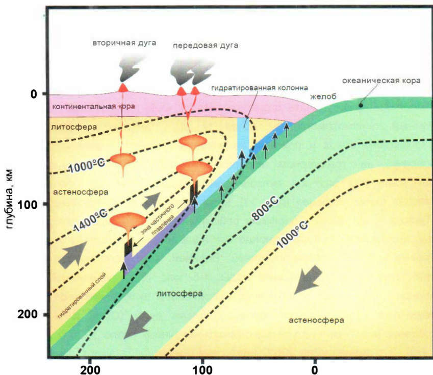
Рис. 10. Петрологическая модель островодужного вулканизма, разработанная Т. Тацуми, на примере северо-восточной Японии (Tatsumi et al., 1983). Дегидратация погружающегося водонасыщенного океанического слэба происходит на глубине 50-60 км с высвобождением водного флюида, который гидратируют мантийный клин, конвекция в котором идет синхронно с субдукцией. В свою очередь, синхронно идет дегидратация слэба на двух уровнях -100 и 180 км с образованием амфибола и флогопита. Распад амфибола и флогопита на первом и втором вулканических фронтах обеспечивает генерацию разнообразных островодужных магм. Особое значение имеет наличие двух вертикальных колонн водосодержащей магмы; и присутствие под вулканическим фронтом мантии с высокими температурами в (около 1400°C), т.е. на 50°C выше, чем температура магмогенерации в срединно-океаническом хребте
