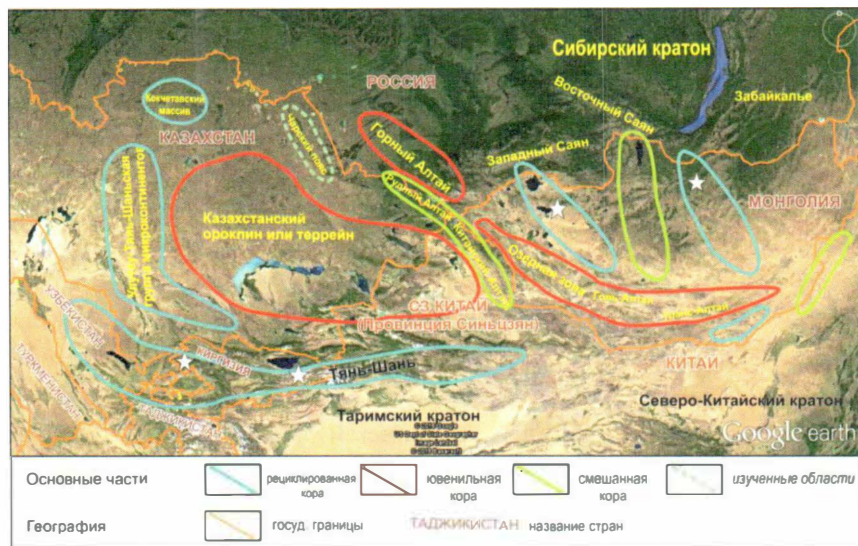
Рис. 20. Сегменты Центрально-Азиатского складчатого пояса, имеющие изотопные характеристики типичные для ювенильной (красный контур) или рециклированной (синий контур) коры и коры смешанного типа (зеленый контур) (рисунок из Safonova, 2017 на основе Kröner et al., 2014). Белыми звездами показано приблизительное расположение областей вероятно тектонической эрозии. Это - аккреционные комплексы с СОП, включая океанические поднятия (базальты типа OIB), голубыми сланцами по базальтам типа OIB и MORB и внутриокеаническими дугами. Это комплексы образовались в областях ювенильного корообразования, но сейчас находятся в пределах сегментов с «рециклированными» характеристиками
