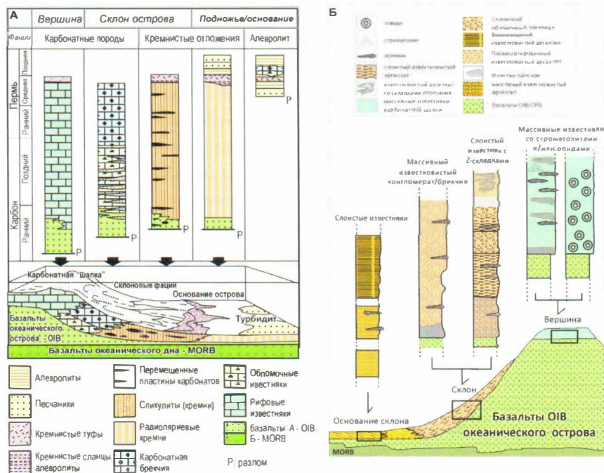
Рис. 27. Схематические реконструкции и литостратиграфические колонки древних океанических островов, сделанные по двум наиболее хорошо изученным типовым объектам западной Пацифики (А – симаунт Акиоши, юго-западная Япония; карбон-пермь; рисунок из Kanmera, Sano, 1991) и Центрально-Азиатского складчатого пояса (Б – Курайский симаунт, Горный Алтай; поздний неопротерозой (рисунок из Uchio et al., 2004)
