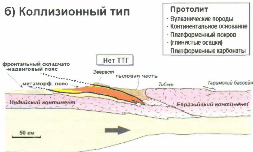
Рис. 4. Орогенные пояса тихоокеанского (а) и коллизионного (б) типа (Maruyama et al., 2011)
