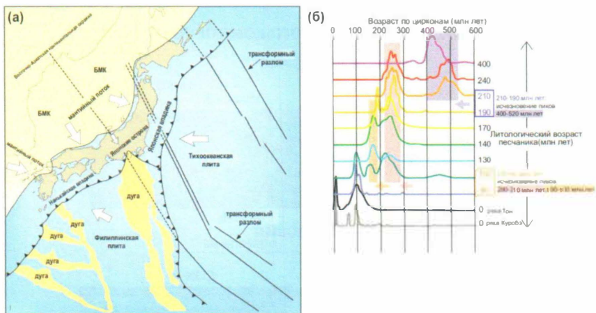
Рис. 16. (а) Внутриокеанические дуги на Филиппинской плите, субдуцирующие в желоб Нанкай. При этом аккреции не происходит (рисунок из Yamamoto et al., 2009). (б) спектры U-Pb возрастов детритовых цирконов из среднепалеозойских, мезозойских и современных песчаников Японии; видна смена типа области сноса (рисунок из Isozaki et al., 2010). Четко видны три главных периода в более чем 500 млн летней геологической истории Японских островов: до позднего триаса (> 200 млн лет), юра – поздний мел (200-90 млн лет) и пост-поздний мел (< 90 млн лет), что свидетельствует о резкой смене типа области сноса терригенных пород (песчаников) в прото-Японии
