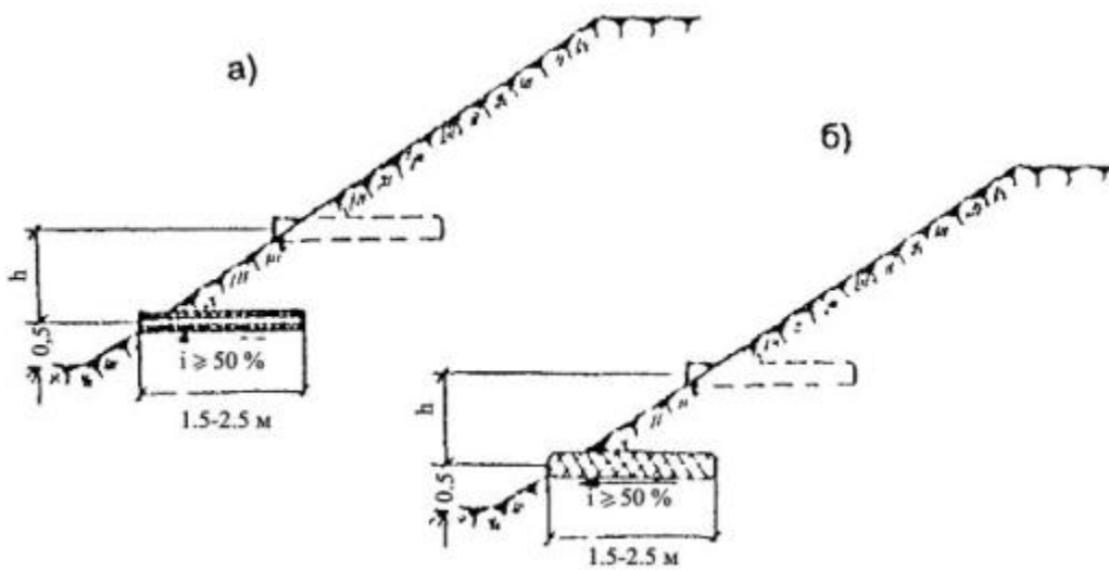
Рис. 5.9. Осушение откосов:
