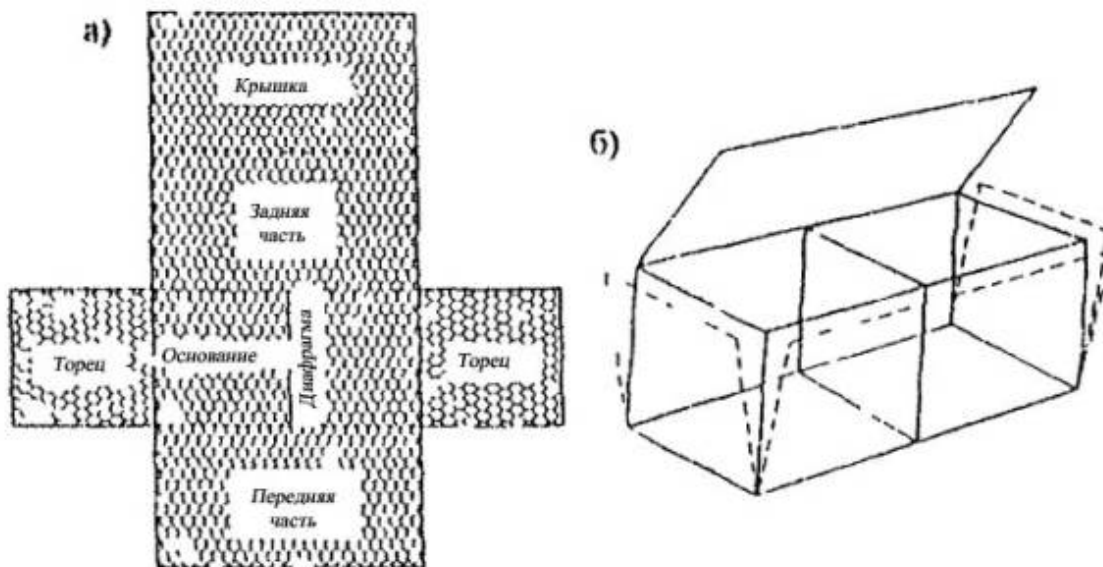
Рис. 2.5. Сетчатая развертка коробчатого габиона с диффрагмой:
