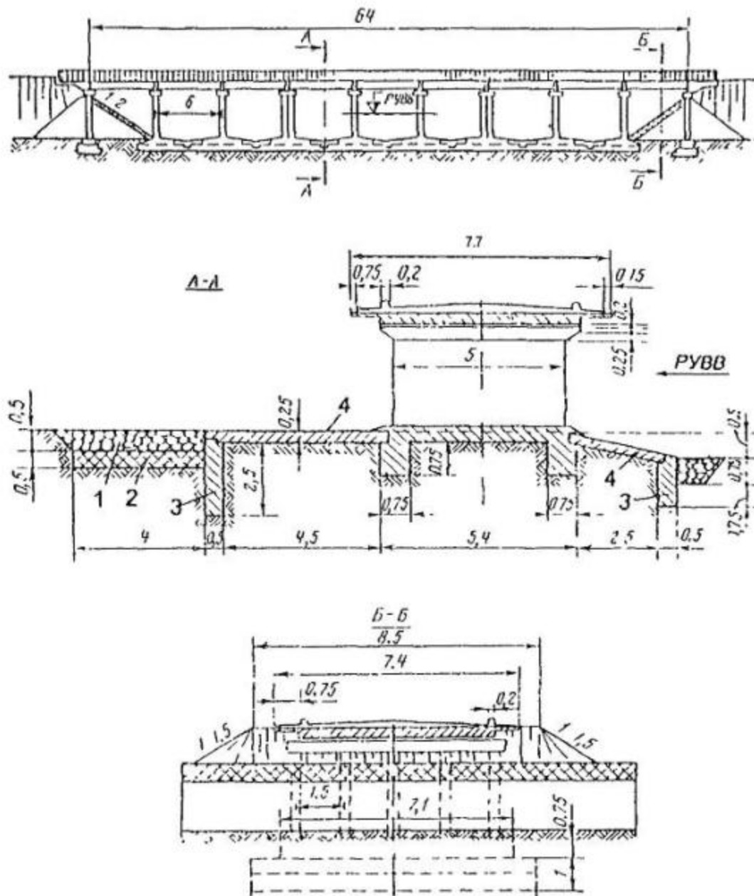
Рис. 4.13. Конструктивная схема моста с укрепленным руслом не предгорной реки:
