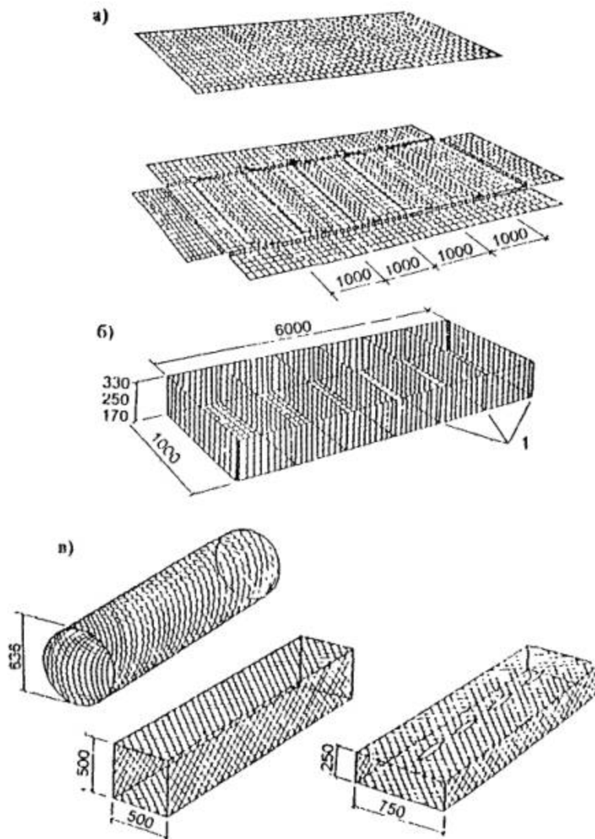
Рис. 2.27. Каркасы габионов:
