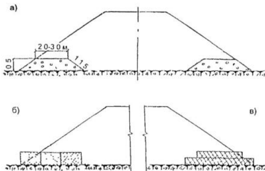
Рис. 5.6. Подошвенные слои:
