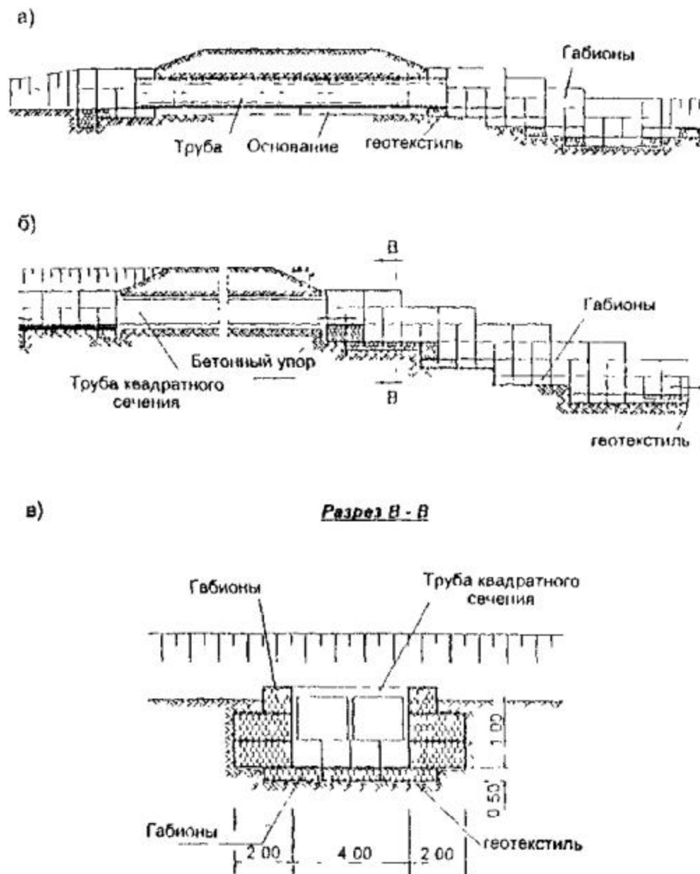
Рис. 6.13. Схемы возможных габбионных укреплений входных и выходных участков водопропускных труб с водобойными устройствами.
