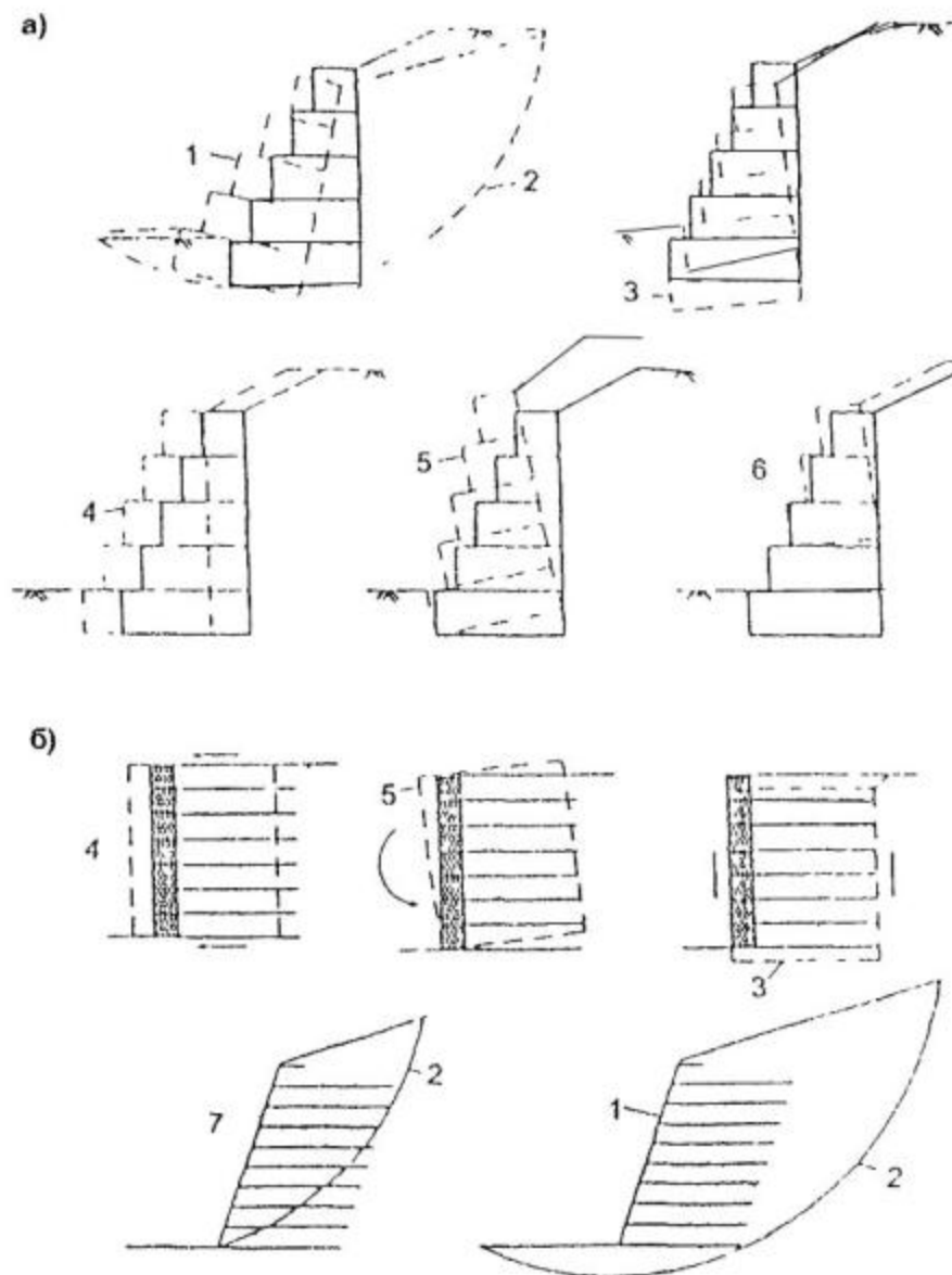
Рис. 5.11. Возможные схемы разрушения габионных стен:
