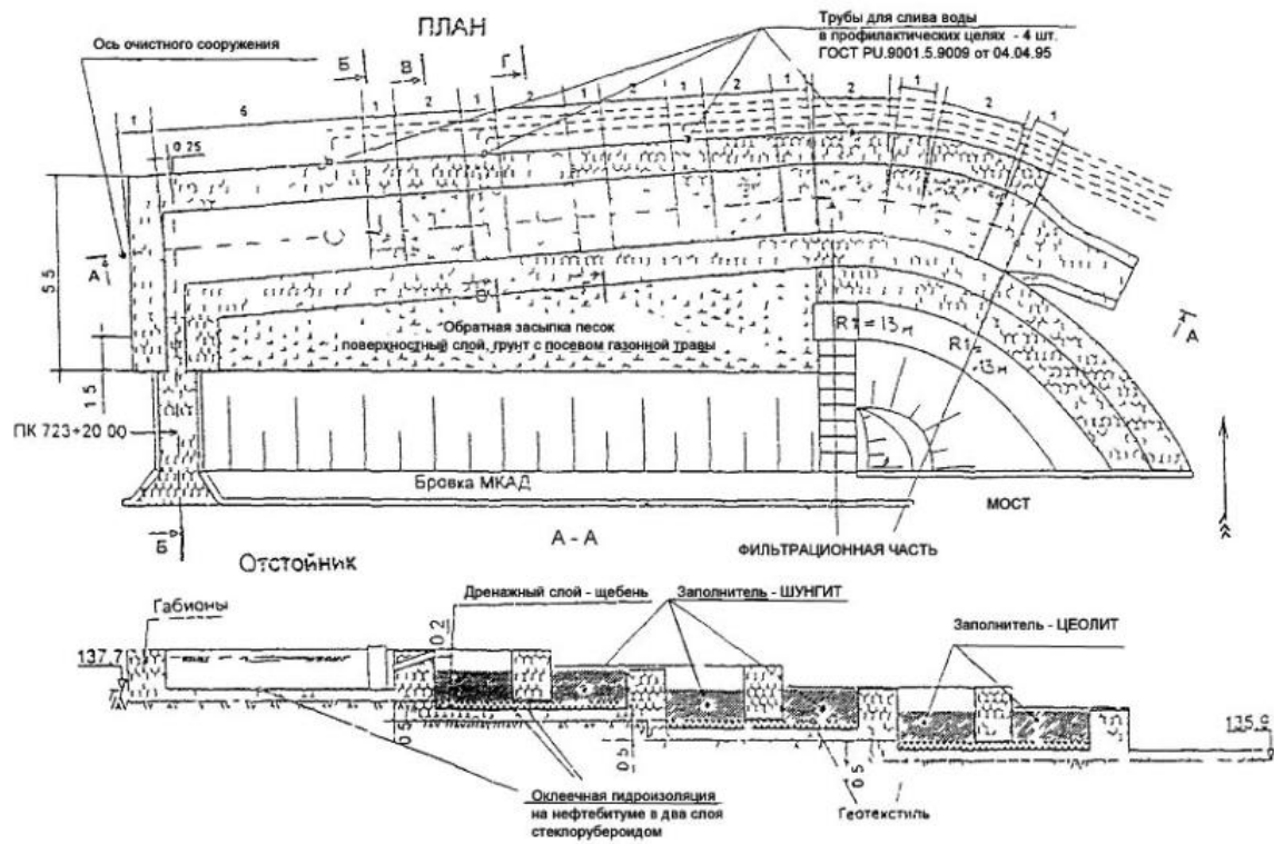
Рис. 6.26. Габрионное очистное сооружение.
