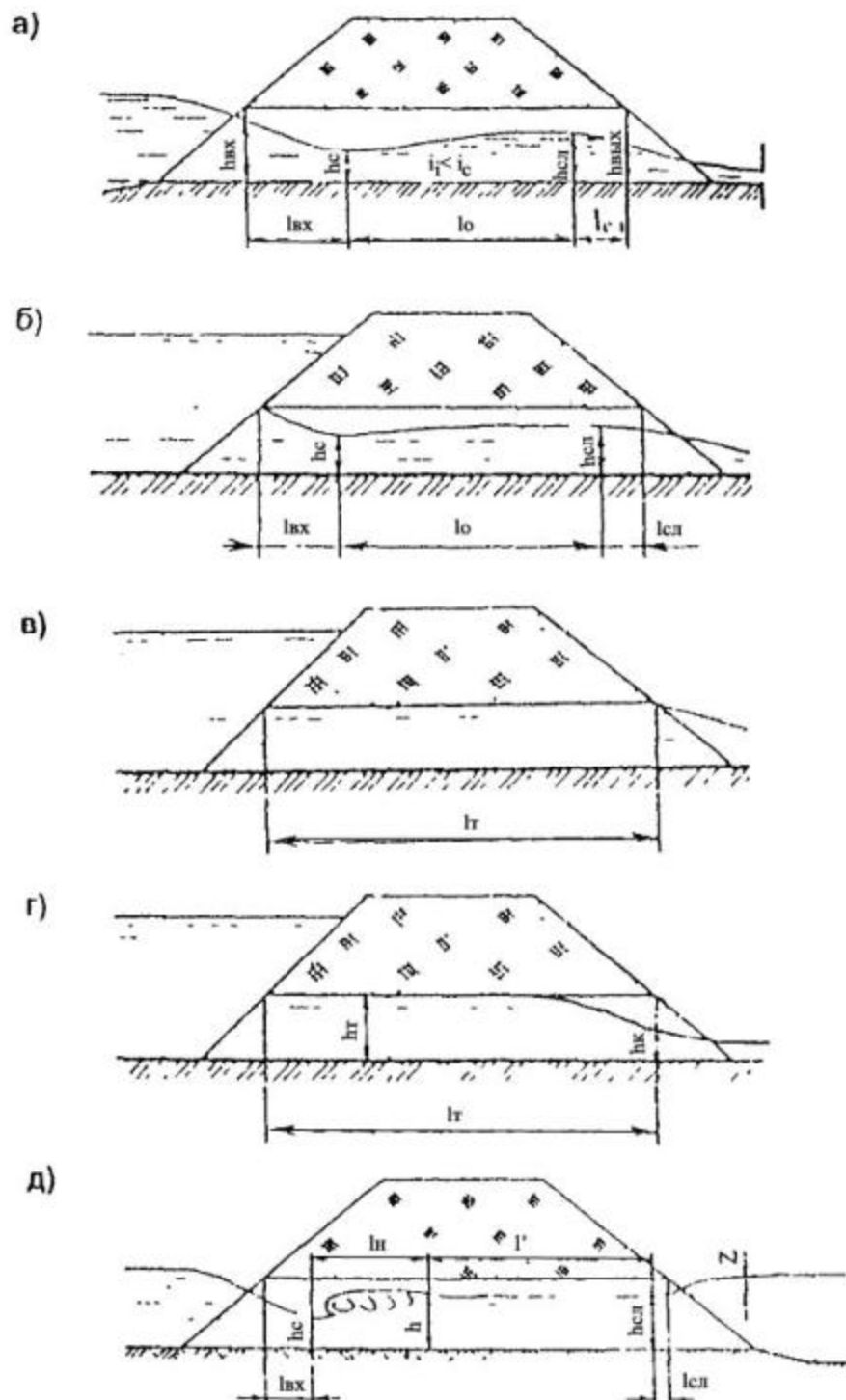
Рис. 6.1. Схемы уровня поверхности воды в водопропускных трубах при режимах протекания:
