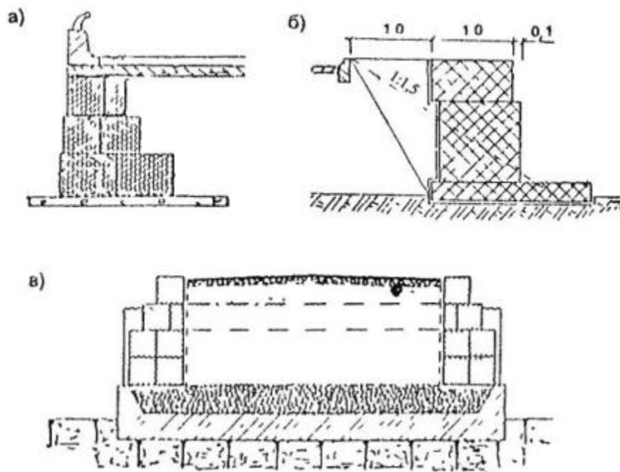
Рис. 5.3. Схемы конструктивных решений по замене откосных частей земляного полотна габионными подпорно-удерживающими сооружениями.
