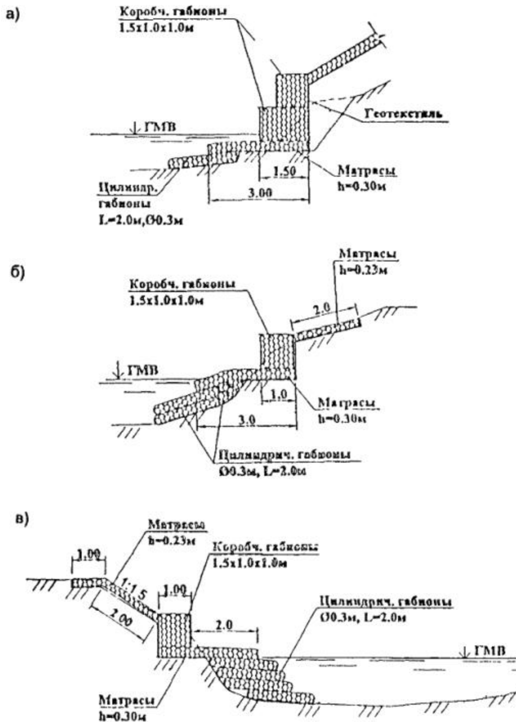
Рис. 3.17. Схемы габионных укреплений для защиты нижней части подтопляемых откосов от подмыва при наличии меженных вод с применением матрасных, коробчатых и цилиндрических габионов.
