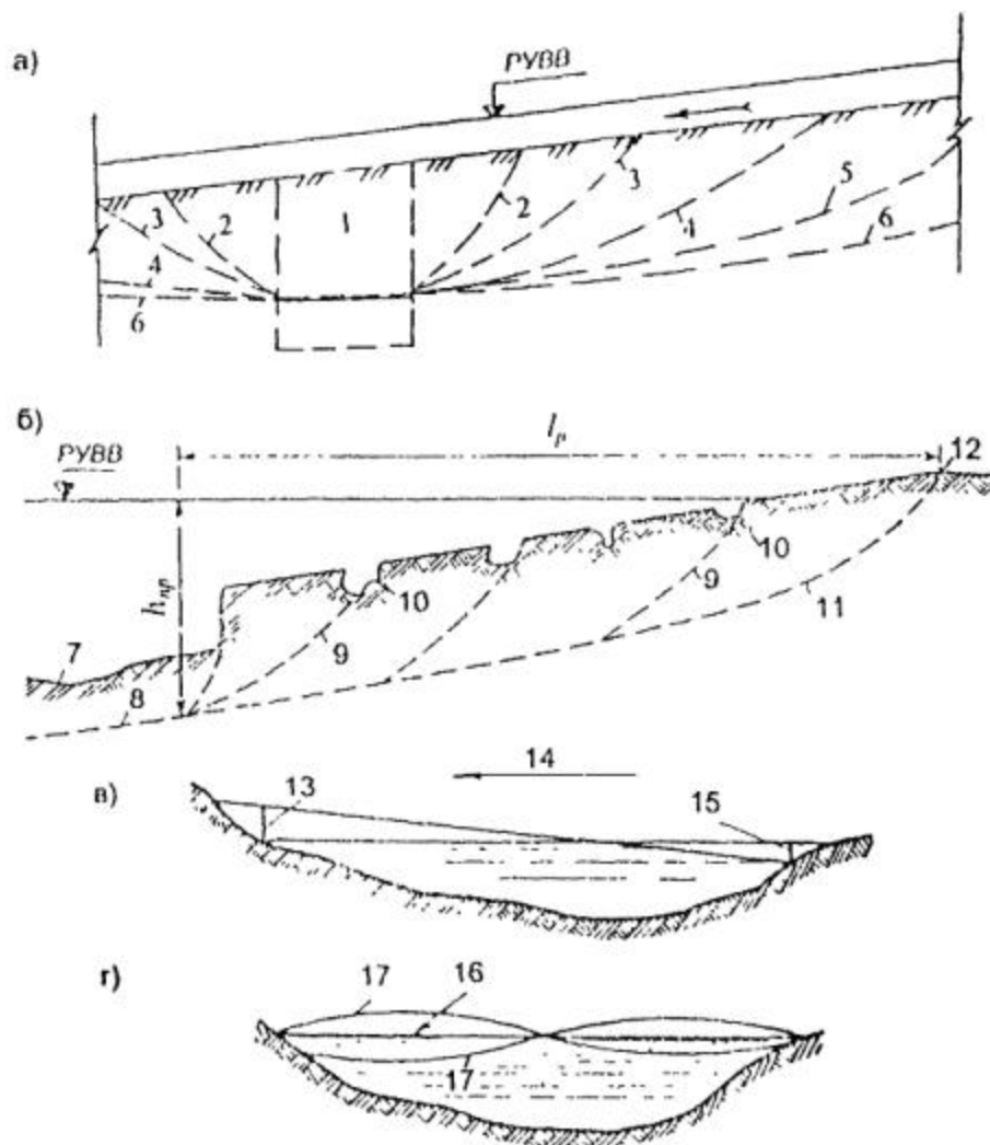
Рис. 3.12. Схемы развития попятного размыва и изменения уровенных поверхностей:
