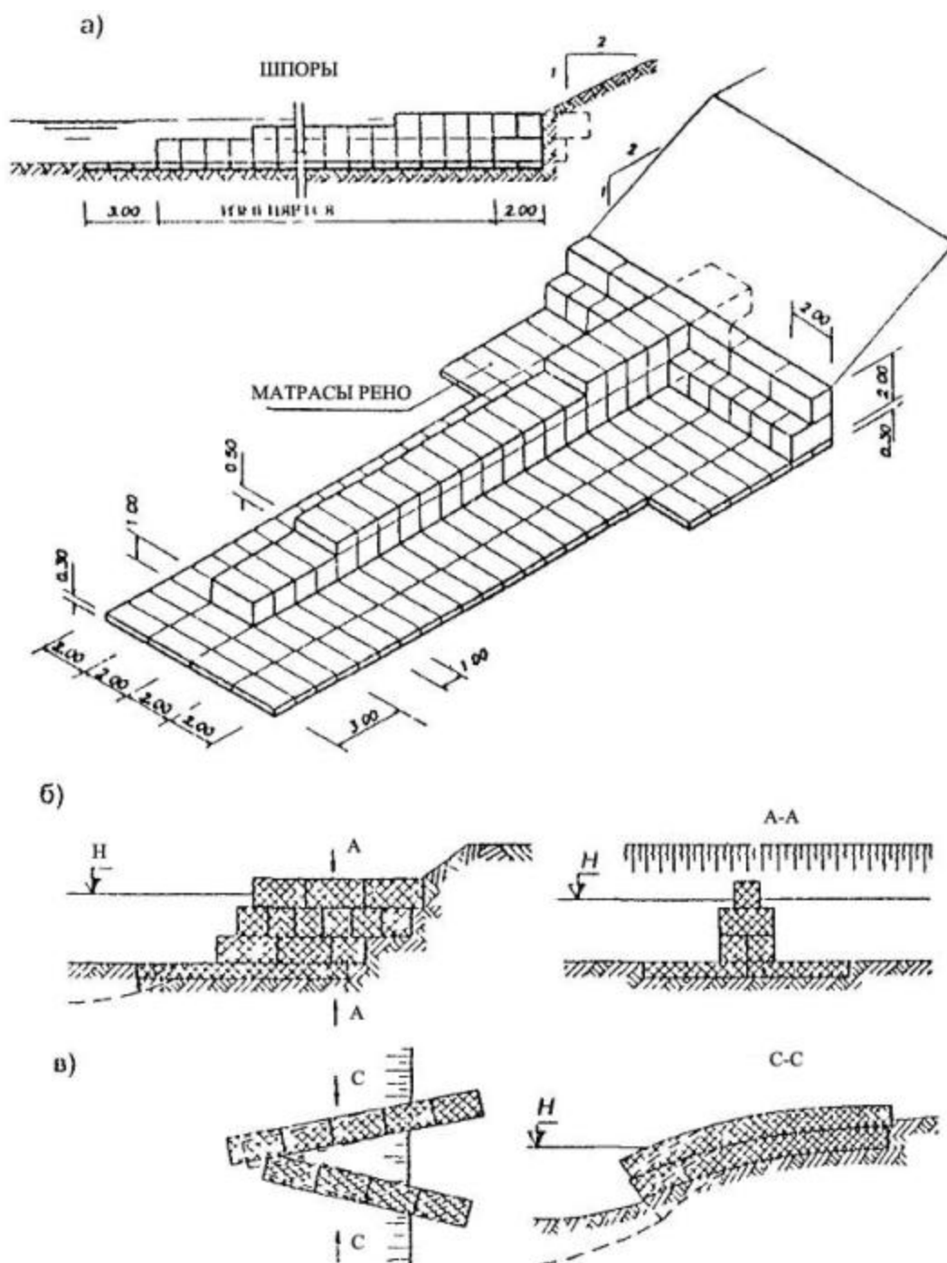
Рис. 4.25. Схемы конструкций и габионных укреплений шпор:
