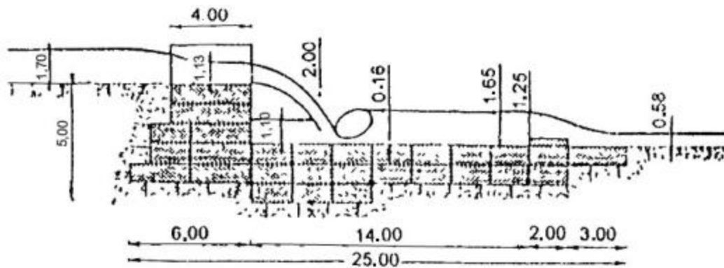
Рис. 7.4. Схема габионного плотинного порога-водослива для защиты опор мостов от попятного размыва.
