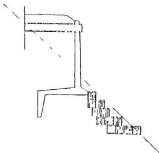
Рис. 5.2. Схема габионной конструкции для защиты фундаментов галлерей.
