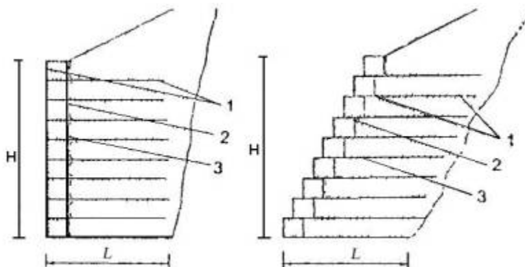
Рис. 2.16. Конструкции системы Террамеш в виде вертикальной и наклонной стен:
