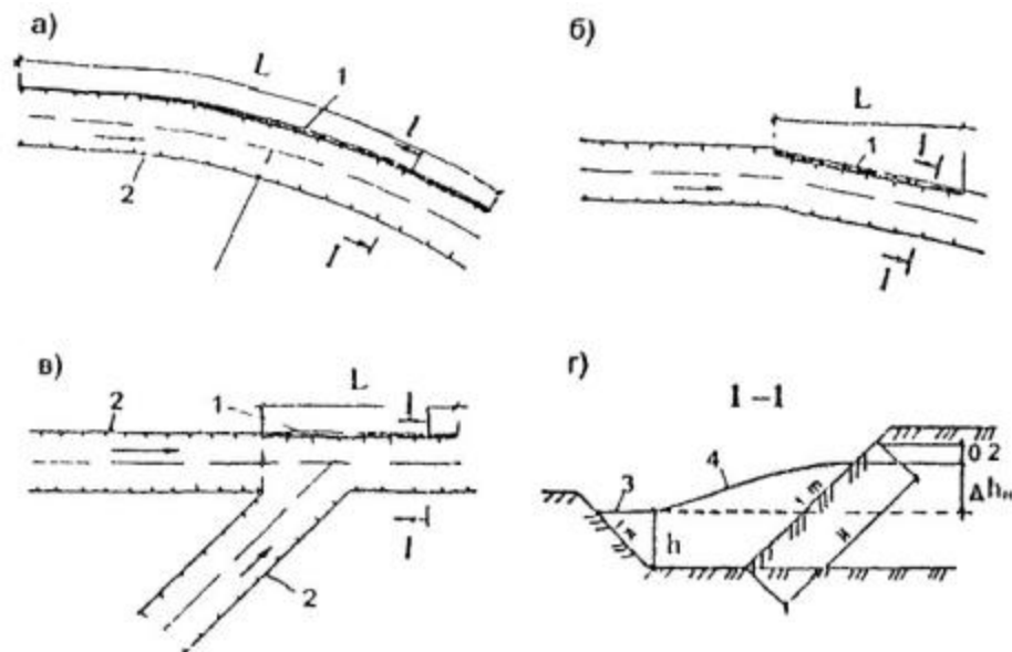
Рис. 6.22. Схемы к определению плано-высотных границ габионных укреплений водоотводных канав при искривлении движения водных потоков:
