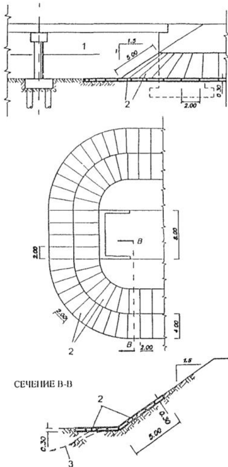
Рис. 4.3. Схема габионного укрепления подмостовых конусов, свободно размещаемых в пролетах мостов с размываемыми руслами:
