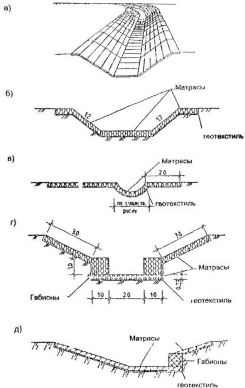
Рис. 6.21. Схемы габионных укреплений водоотводных канав, резервов и кюветов.
