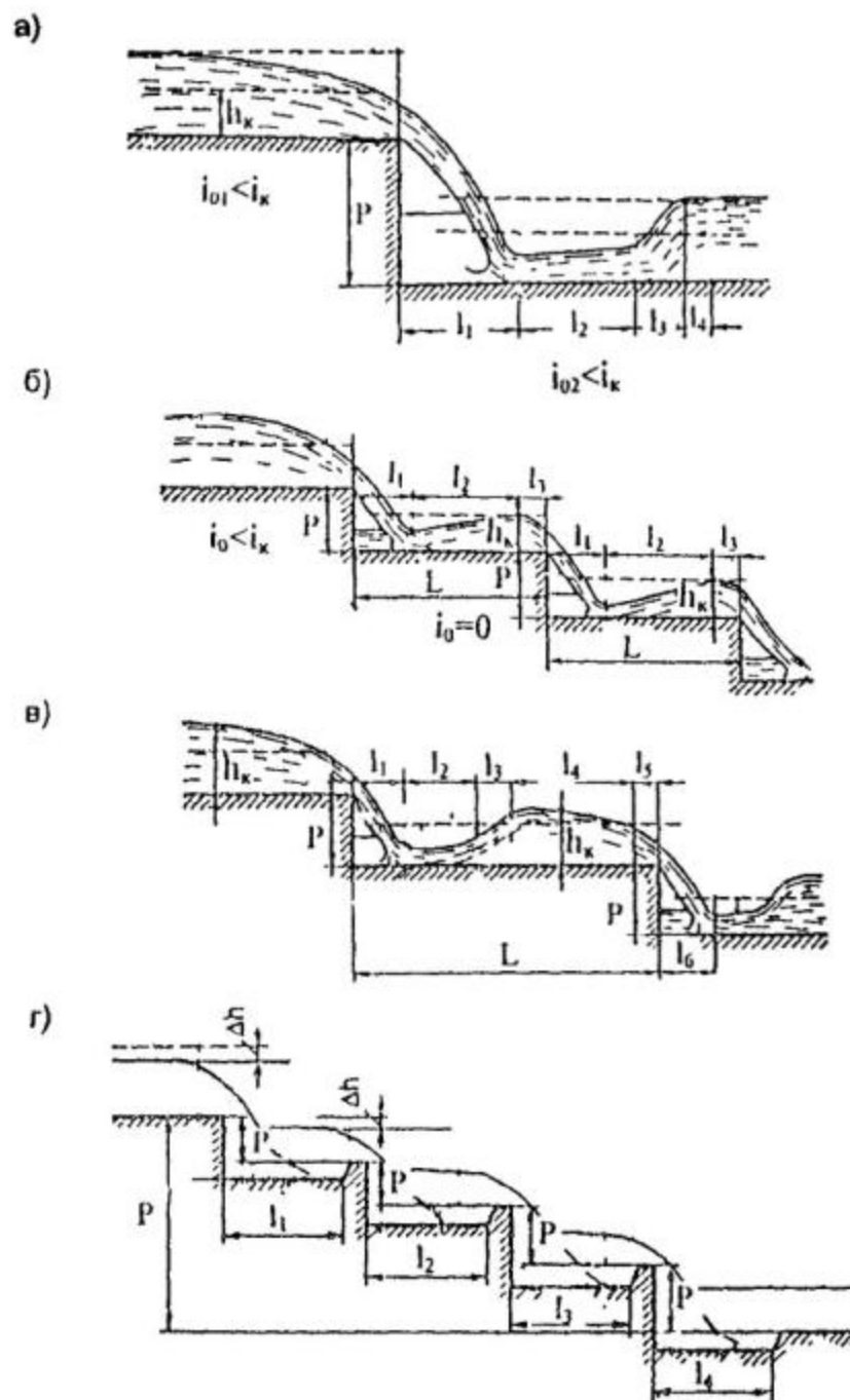
Рис. 6.19. Формы кривых свободной поверхности в перепадах:
