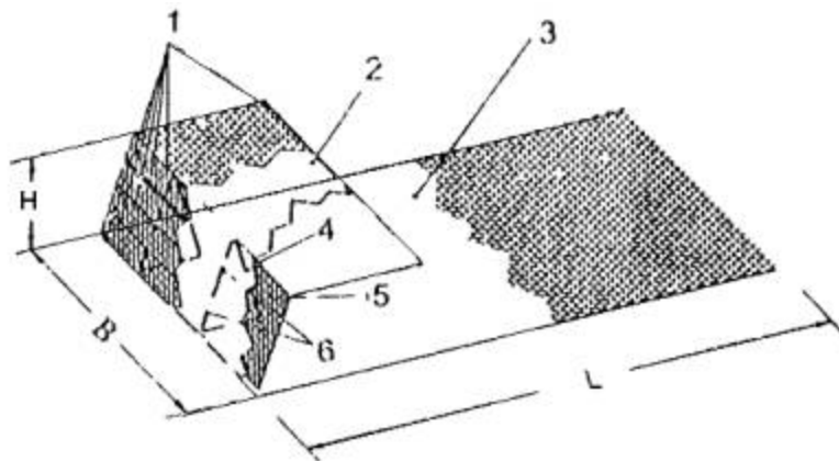
Рис. 2.19. Конструктивные элементы системы зеленый Террашеш:
