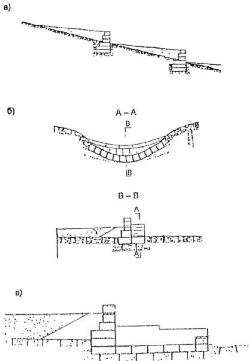
Рис. 7.11. Схемы габрионных селезадерживающих сооружений.
