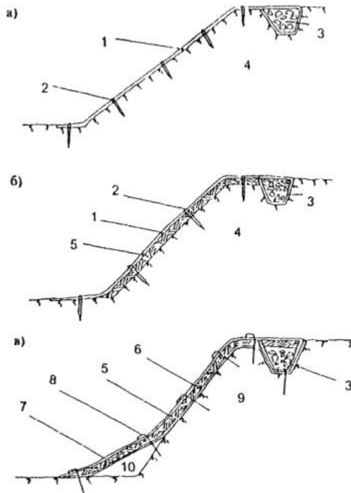
Рис. 3.2. Схемы защиты откосов с помощью биоматов:
