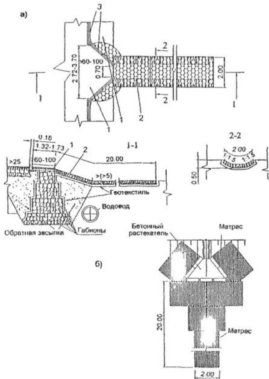
Рис. 6.25. Габрионные откосные лотки (а) и укрепления на выходных участках традиционных телескопических лотков (б):
