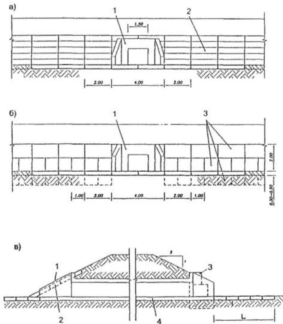
Рис. 6.5. Схемы возможных габионных укреплений верхнего и нижнего бьефов прямоугольных водопропускных труб:
