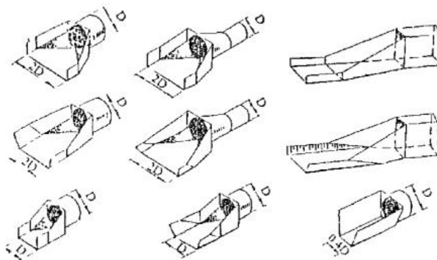
Рис. 6.11. Схемы протекания воды в косогорных трубах.
