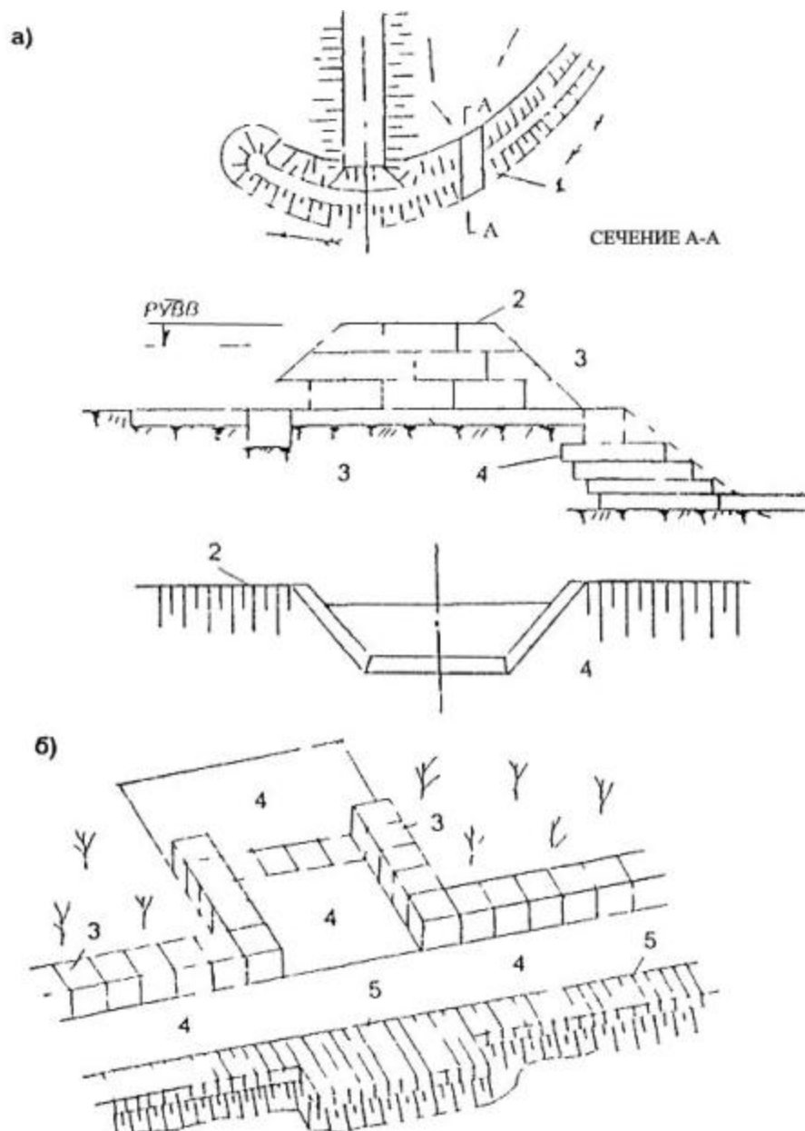
Рис. 4.28. Противоэрозионные габионные водосливы:
