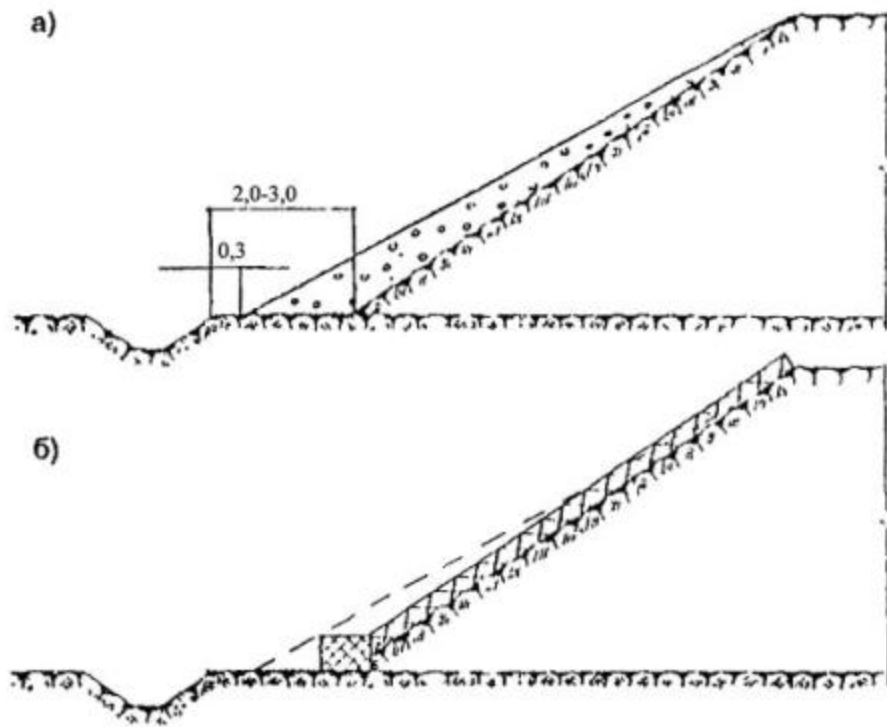
Рис. 5.8. Дренажирование откоса:
