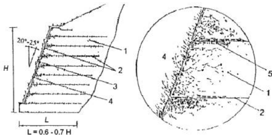
Рис. 2.20. Конструкция системы зеленый Террашеш:
