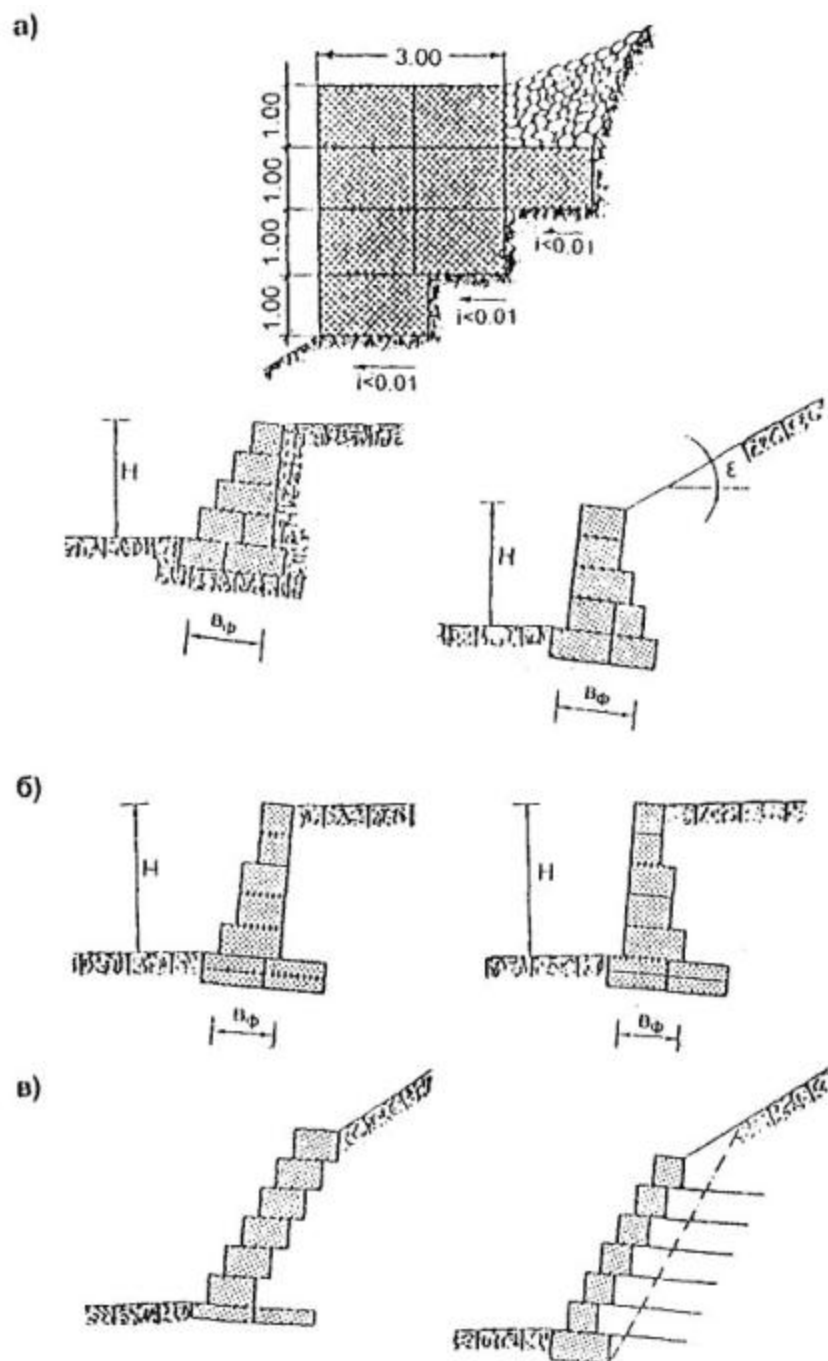
Рис. 5.10. Схемы основных разновидностей габионных стен:
