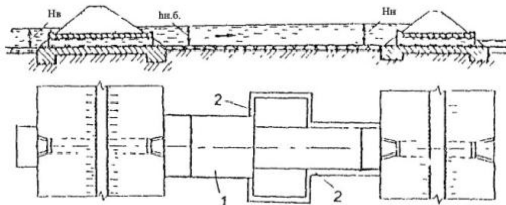
Рис. 6.10. Схема противоэрозионного сопряжения пространства между водопропускными трубами, расположенными на близлежащих дорогах или на раздельном дорожном полотне:
