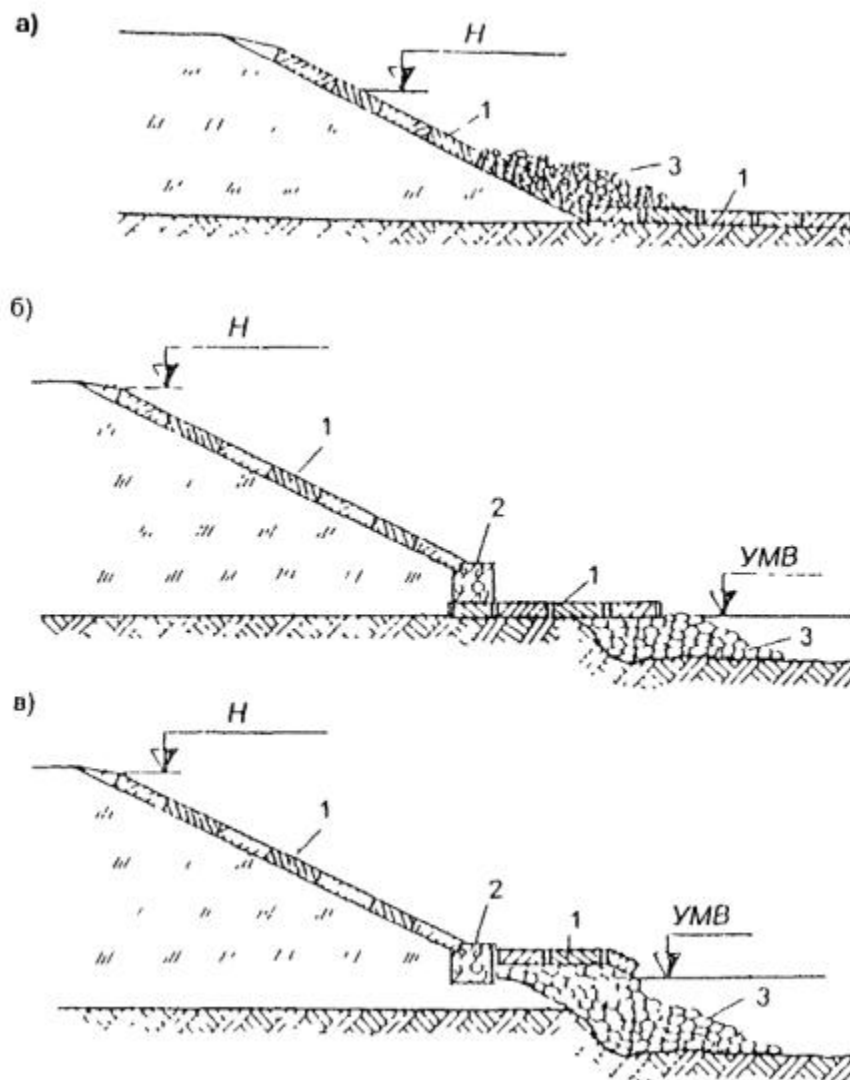
Рис. 3.16. Схемы габионных укреплений для защиты нижней части подтопляемых откосов от подмыва:
