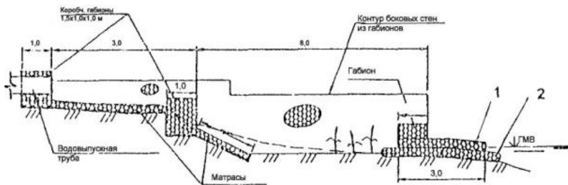
Рис. 6.23. Принципиальная схема конструкции прибрежного очистного сооружения на выходе из водопропускной трубы:
