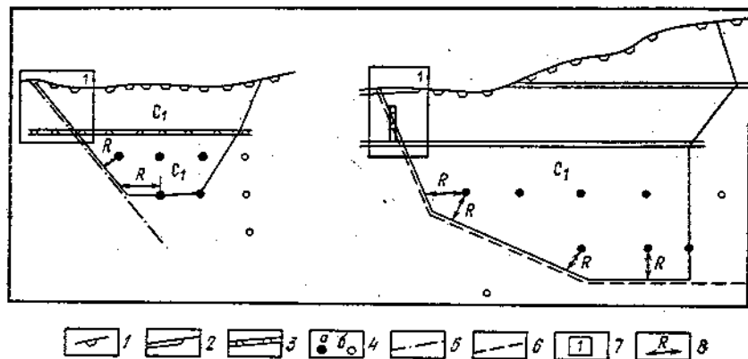
Рис. 71. Неограниченная экстраполяция запасов категории C_1 к скважинам. Справа тела большой мощности ( >2,5 м); слева тела жильного типа малой мощности (до 2,5 м). 1 — каналы; 2 — траншеи; 3 — подземные горные выработки; 4 — скважины ( \alpha — балансовое сечение, \beta — забалансовое сечение); 5 — разрывное нарушение, ограничивающее рудное тело по простиранию; 6 — линия сочленения с другим рудным телом; 7 — участок, где доказано распространение промышленного оруденения до естественных ограничений; 8 — расстояние экстраполяции
