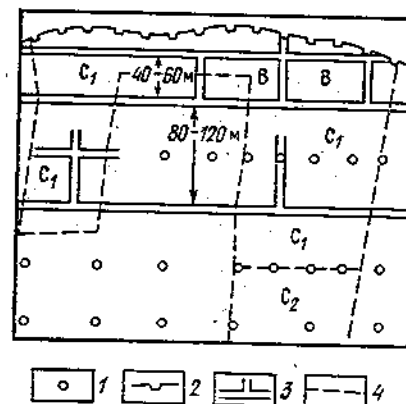
Рис. 3. Схема разведки жилы скважинами и штреками из восстающих с промежуточного горизонта.
