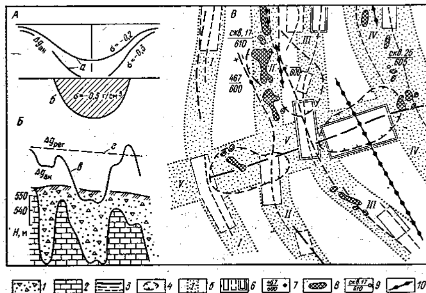
Рис. 55. Выделение рудоносных карстовых депрессий на золоторудном поле по данным гравиразведки.
