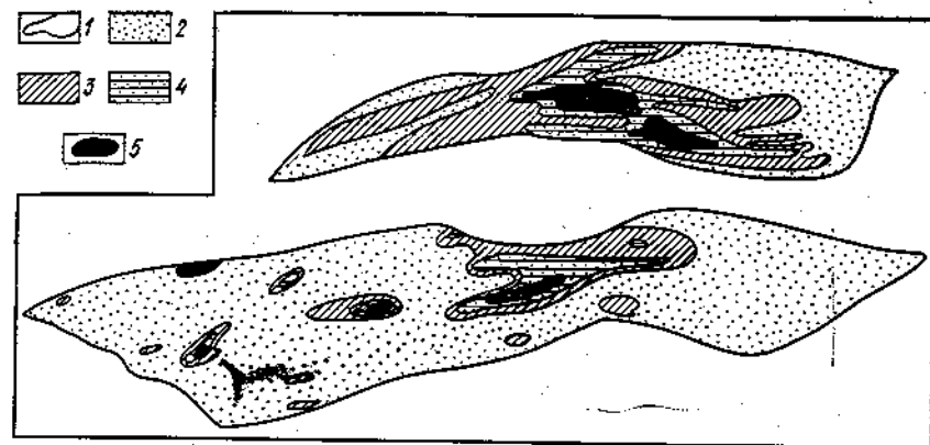
Рис. 51. Аксонометрическая проекция трубообразного рудного тела (Месторождение 11).
