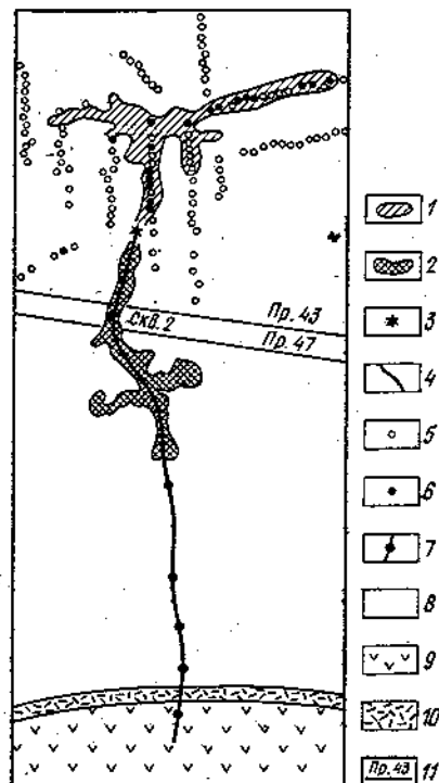
Рис. 56. Прослеживание золотосульфидной залежи методом заряда на переменном токе с измерением магнитного поля.
