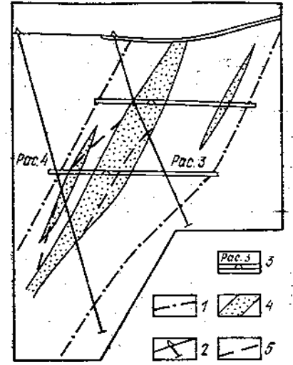
Рис. 74. Формальный подход к оконтуриванию и увязке рудных тел по их падению на месторождениях типа жильных и минерализованных зон.
