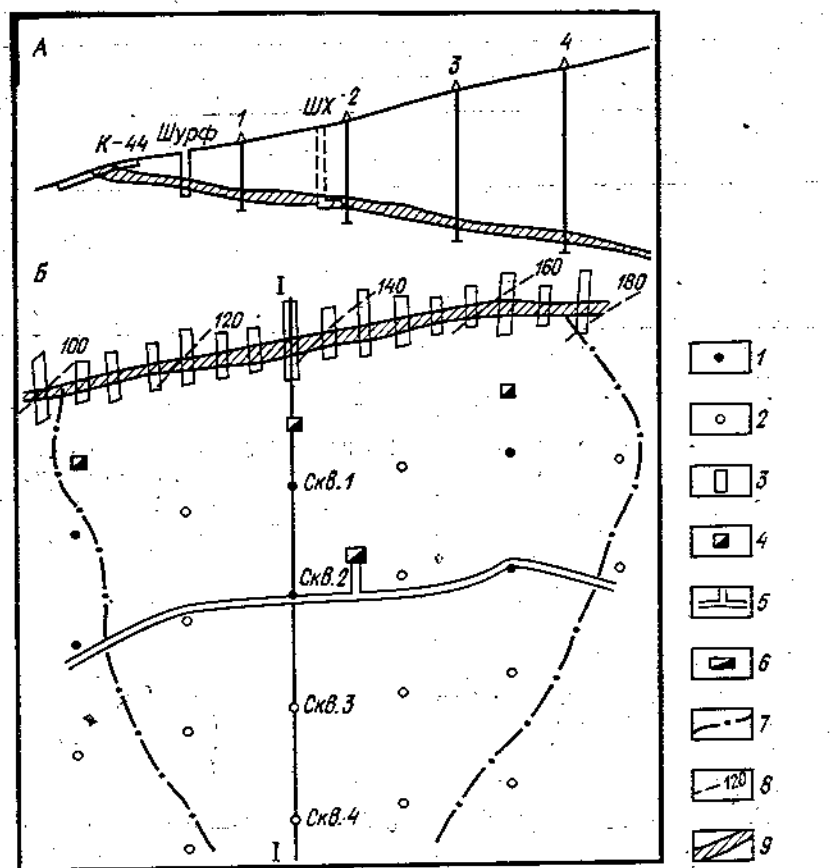
Рис. 8. Схема разведки пологозалегающей жилы.
