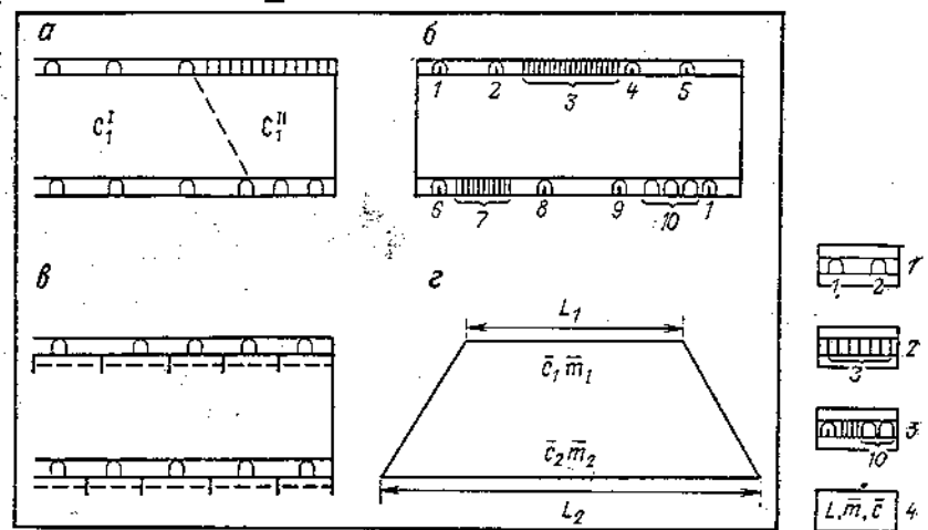
Рис. 75. Особенности определения средних параметров подсчета запасов при неравномерной сети разведочных пересечений.
