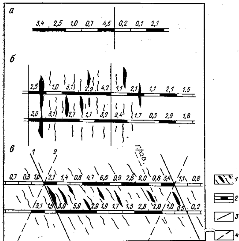
Рис 69. Оконтуривание промышленных руд по мощности при отсутствии четких геологических границ.
