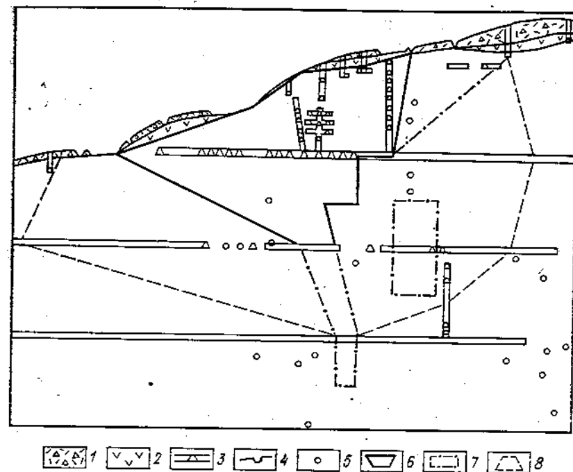
Рис. 16. Система разведки и оконтуривание запасов рудного тела жильного типа (Месторождение 2).
