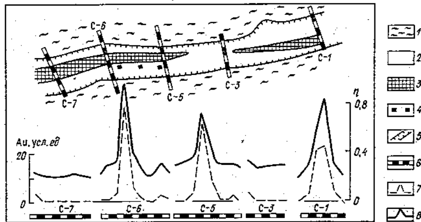
Рис. 59. Выделение золоторудных интервалов по расчистке на одном из месторождений Западного Узбекистана с помощью рентгенорадиометрического метода.
