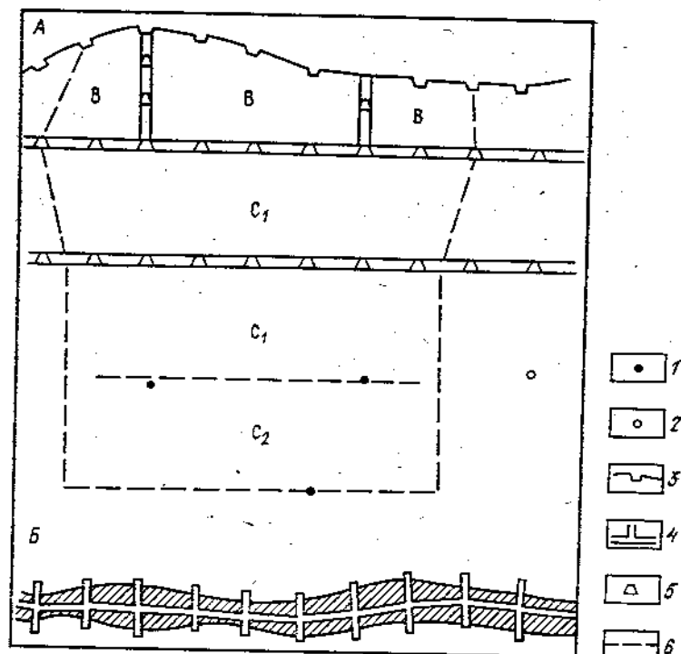
Рис. 2. Схема разведки мощной жилы.
