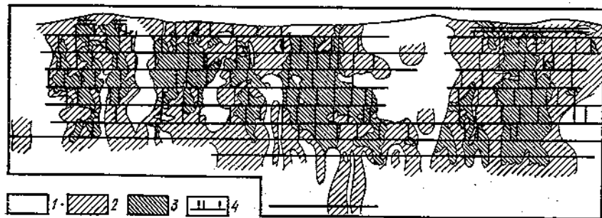
Рис. 10. Система разведки жилы с вертикальными рудными столбами (Месторождение 1).
