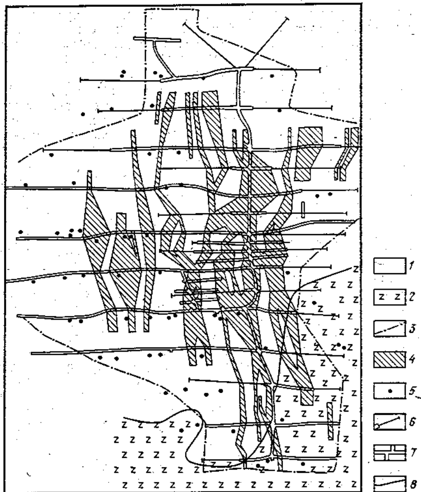
Рис. 36. Геологоразведочный план горизонта месторождения штокверкового типа (Месторождение 7).
