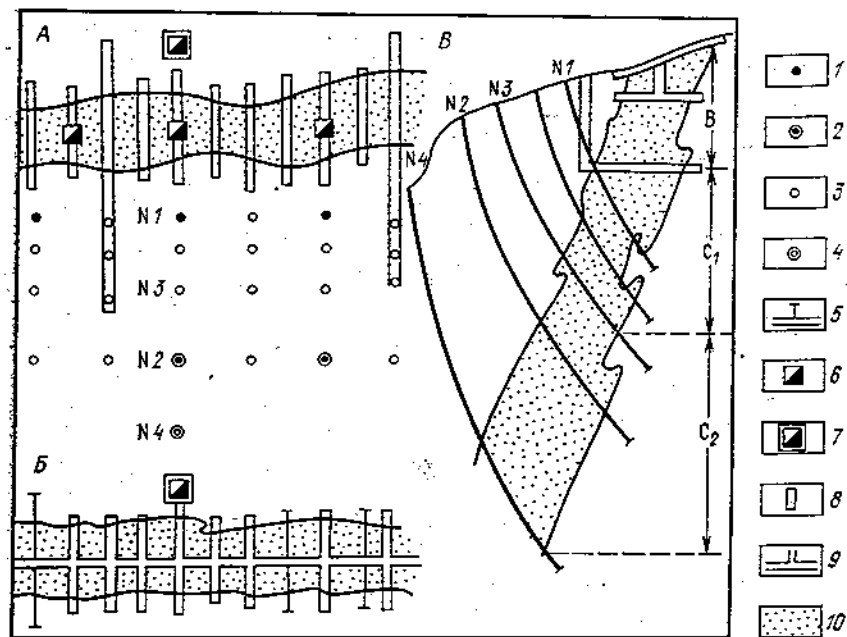
Рис. 4. Схема разведки жильных и минерализованных зон.
