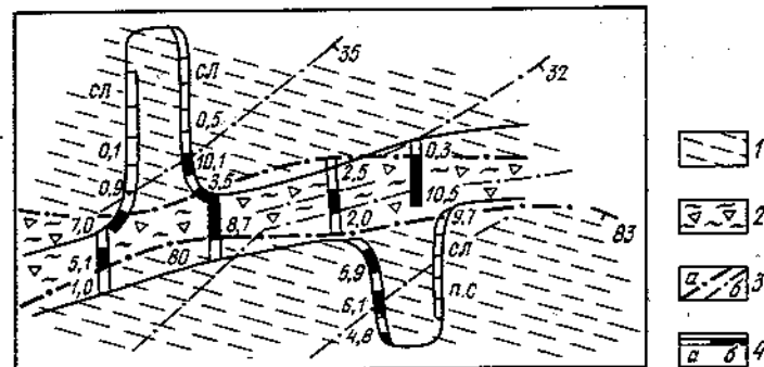
Рис. 68 Схема определения границ рудного тела в условиях редкой оперяющей трещиноватости.
