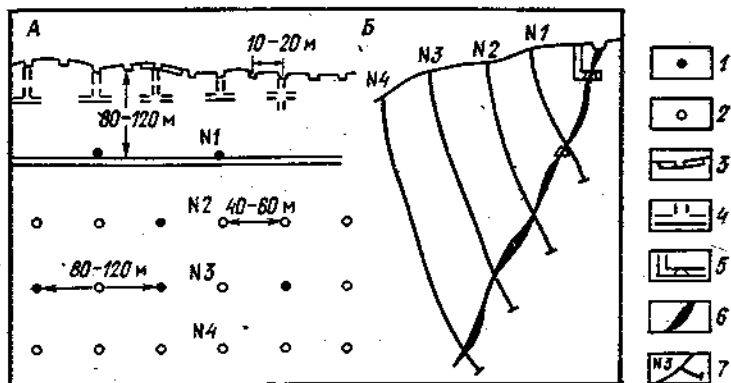
Рис. 1. Схема разведки маломощной жилы.
