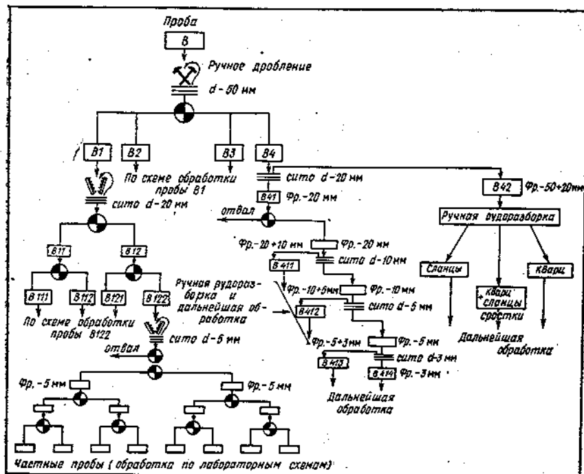
Рис. 53. Принципиальная схема обработки валовых проб при экспериментальных исследованиях (на примере месторождения с прожилково-вкрапленным оруденением)
