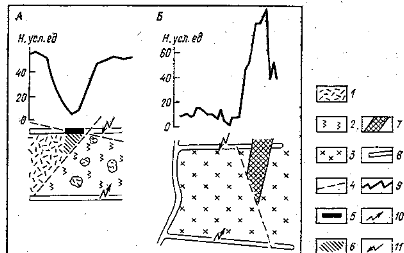
Рис. 60. Результаты радиоволновых измерений при частоте 10 МГц на золоторудных месторождениях, сложенных рудными телами существенно сульфидного (А) и кварцевого состава (Б).
