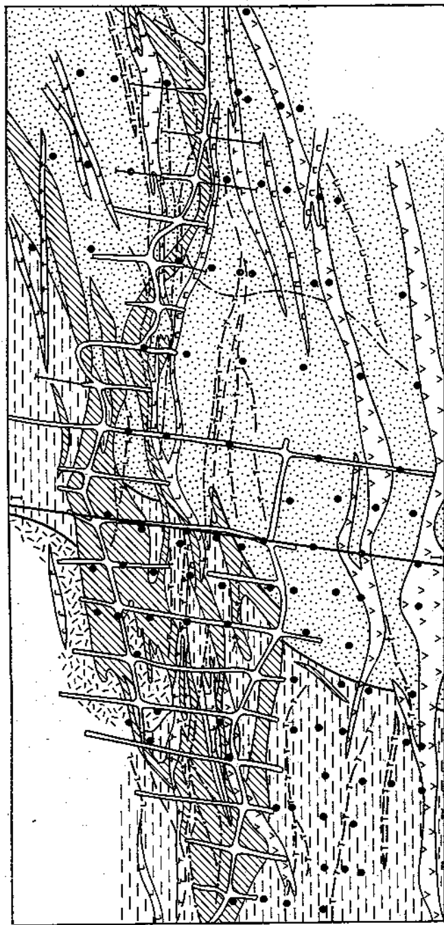
Рис. 42. Геологоразведочный план горизонта месторождения типа минерализованных зон (Месторождение 9).
