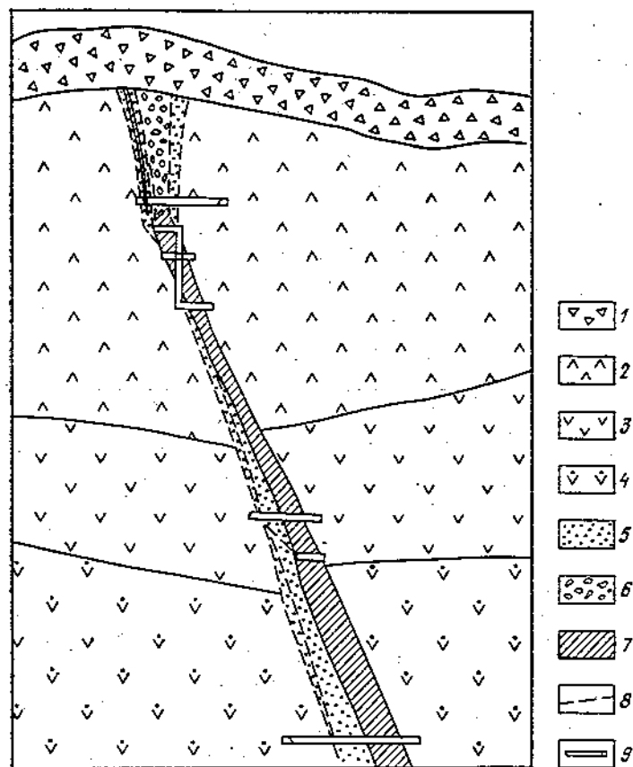
Рис. 52. Геологоразведочный разрез месторождения с трубообразными рудными телами (Месторождение И).
