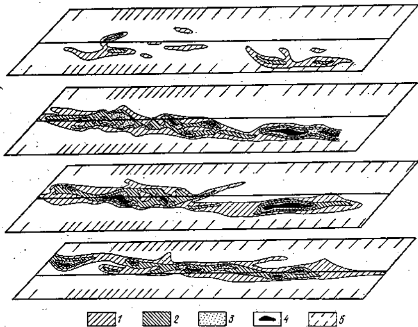
Рис. 32. Распределение полезного компонента по горизонтам (Месторождение 6).
