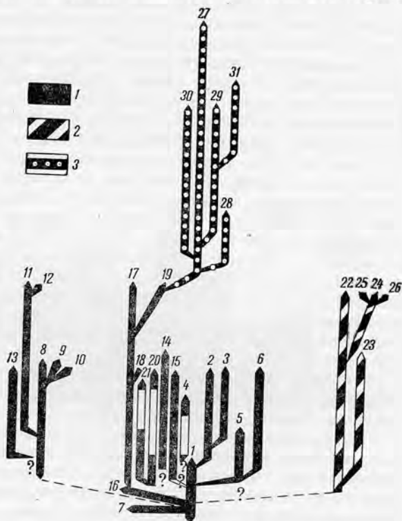
Рис. 2. Схема филогенетических отношений семейств в отряде Nautilida;
