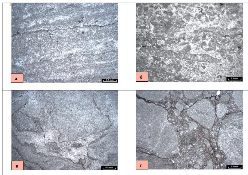
Рисунок 3. а-доломит строматолитовый, x 25, н //; б,в,г-доломиты обломочные, x 25, н //.
