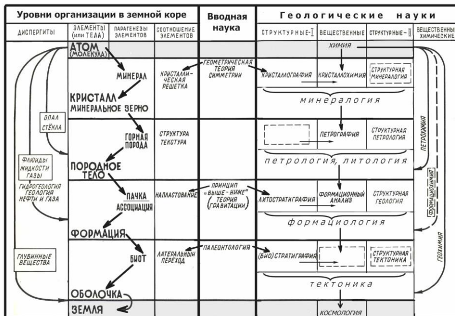
Рисунок 1. Иерархия объектов геологии и система геологических наук (в штриховых рамках потенциальные геологические дисциплины).
