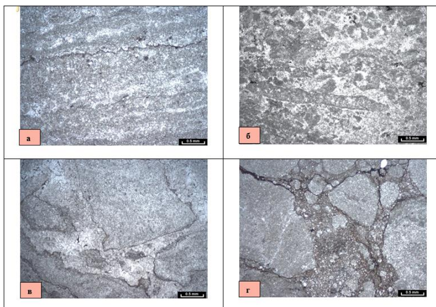
Рисунок 7. а-доломит строматолитовый, x 25, н //; б,в,г-доломиты обломочные, x 25, н //.
