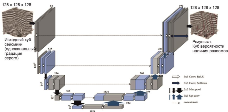
Рисунок1. Архитектура нейронной сети.
