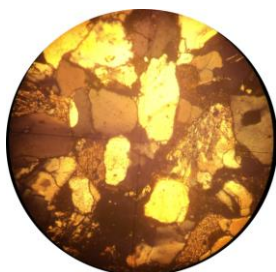
Рисунок 2. Песчаник крупно – среднезернистый, п/ш-кварцевый, с обломками глинисто-глинистых пород, кварцитов. Кушаб, скв. 1П. Ник. +, ув. 9x15.
