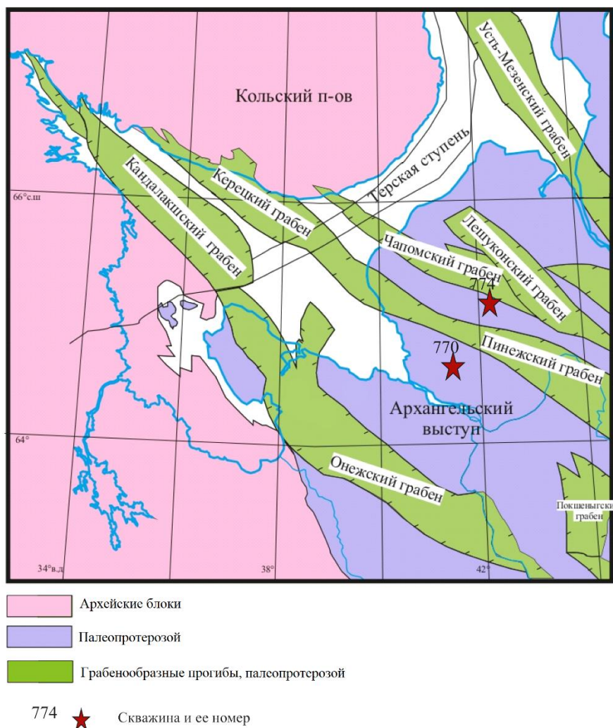
Рисунок 1. Схематическая тектоническая карта северной части Восточно-Европейской платформы и Фенноскандинавского щита [5]
