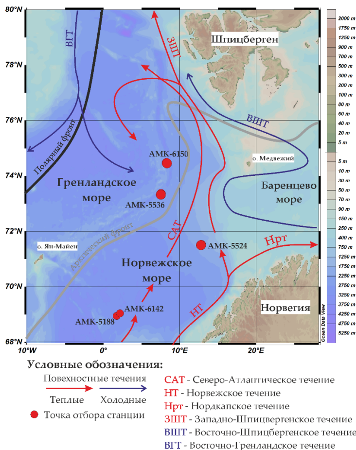
Рисунок 3. Карта Норвежско-Гренландского бассейна, показывающая основные направления поверхностных течений, распределение водных масс и расположения исследуемых колонок на станциях (Vauch et al, 2001; Klitgaard-Kristensen et al, 2002; Hoff et al, 2016).
