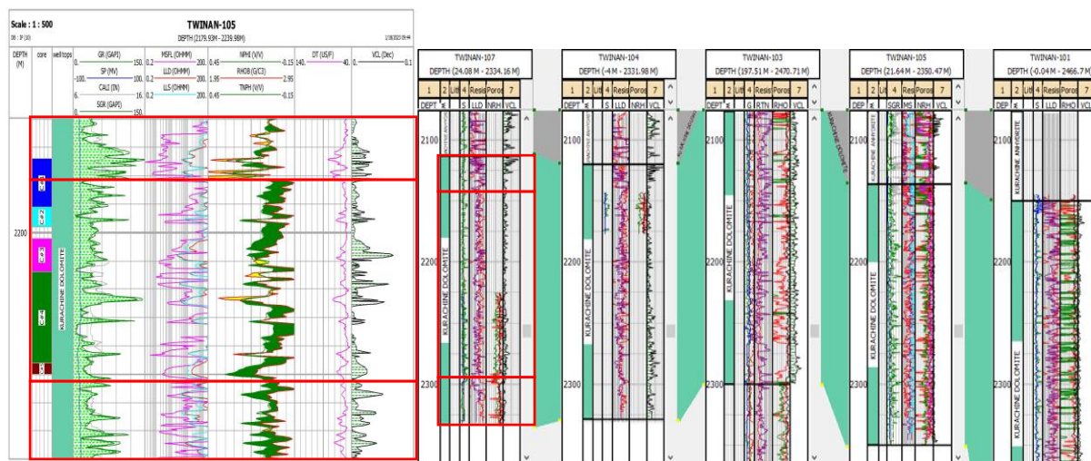
Рисунок 2. Каротажная характеристика курачинской доломитовой свиты в скважине "Твинан_105" и корреляция с другими скважинами.
