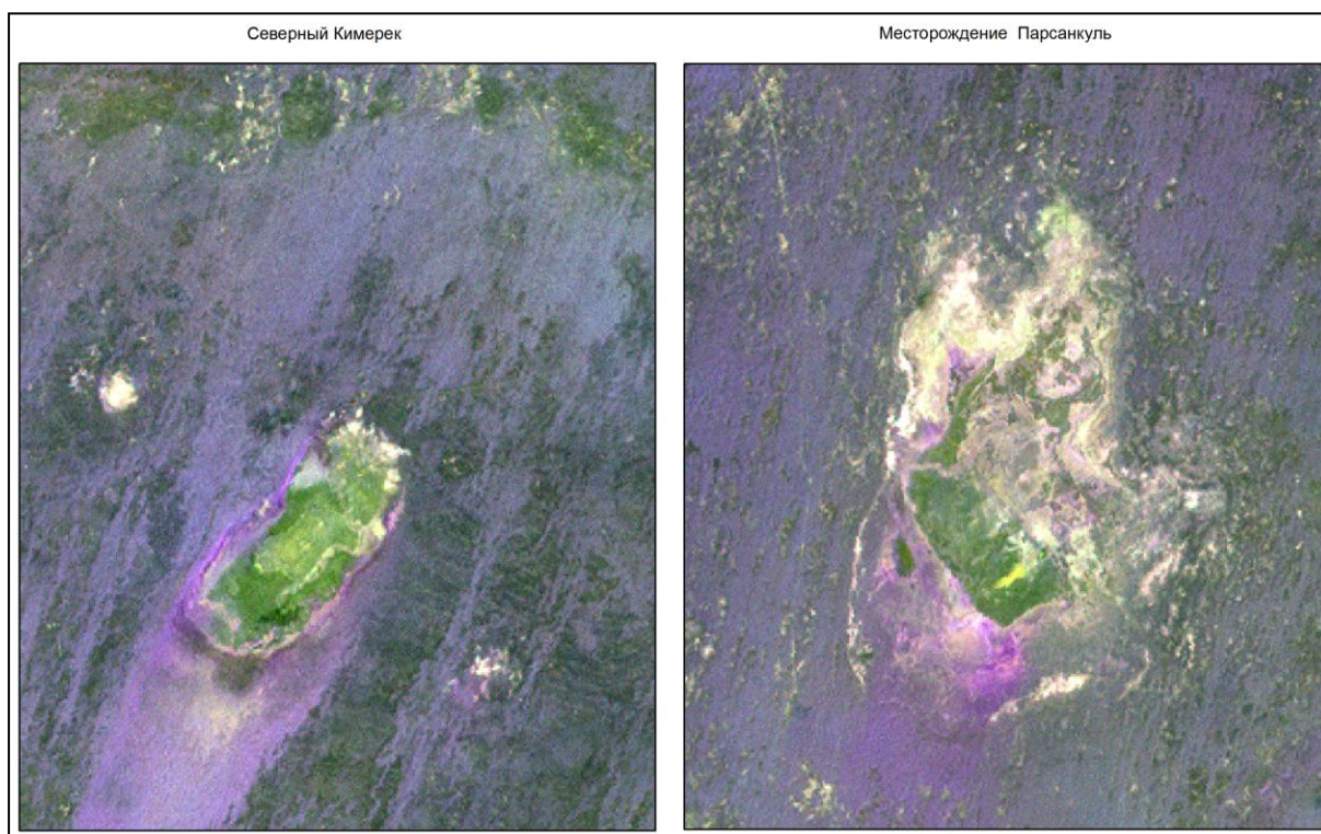
Рисунок 1. Спектрональный космический снимок Landsat 7 ETM+
