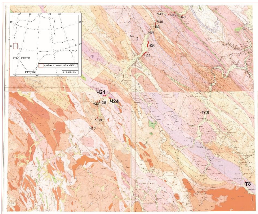
Рисунок 1. Карта района работ
