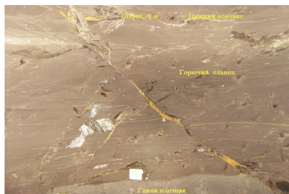
Рисунок 2. Разлом в горючих сланцах и глинах (штолок № 1)
