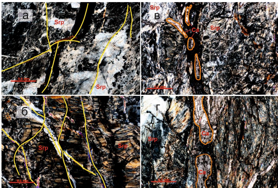
Рисунок 2. а и б – системы трещин со смещением (выделены желтым); в и г – кальцит подвергшийся будинажу (зерна выделены оранжевым). Srp – серпентин, Ca – кальцит. Нх, увел.5.
