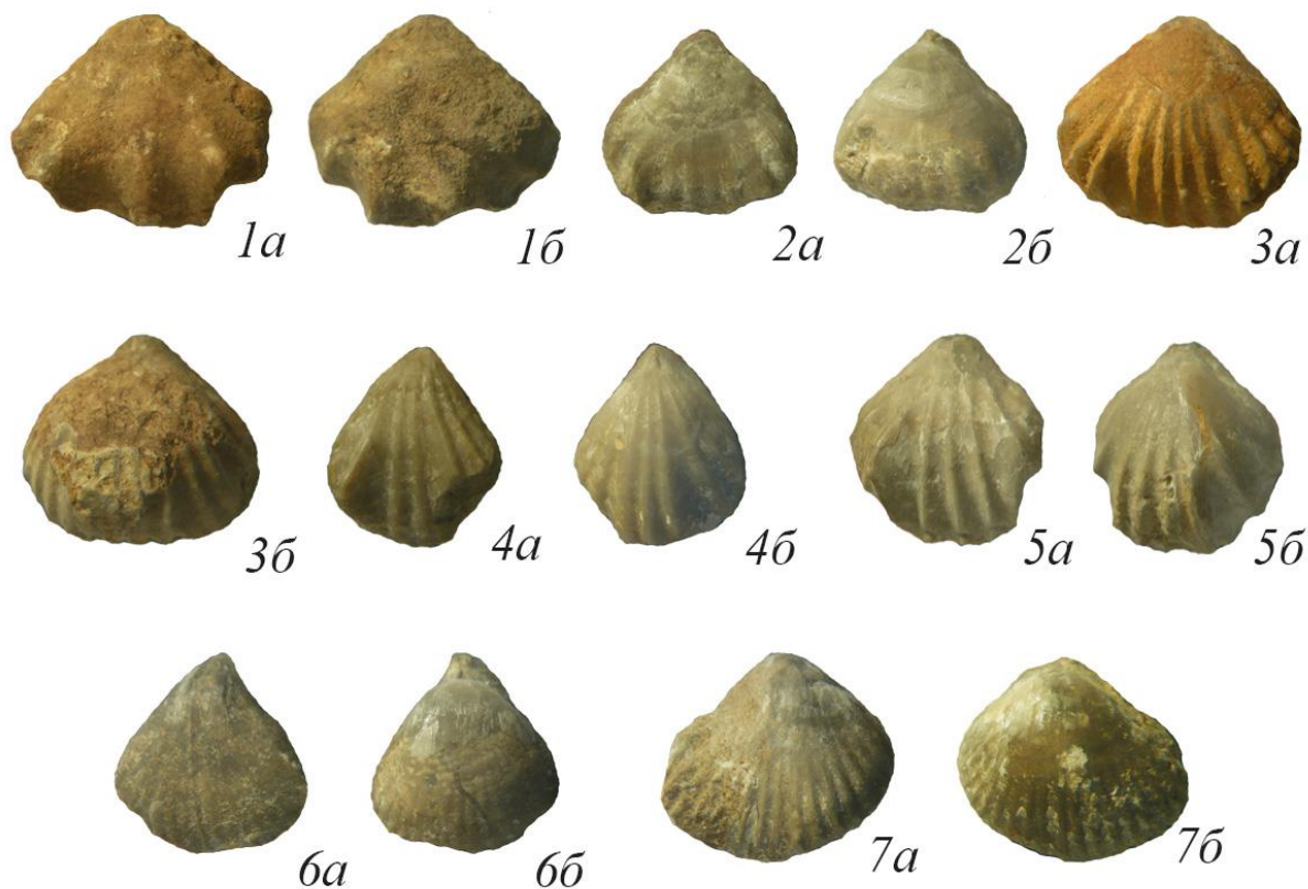
Рисунок 1. Нижнеюрские ринхонеллиды эскиординской свиты: 1 – Bodrakella bodrakensis Mois., экз. № 3/359; 2 – Cuneirhynchia persinuata (Rau), экз. № 3/360; 3 – Gibbirhynchia curviceps (Quenst.), экз. № 3/361; 4 – Piarorhynchia variabilis var fronto Quenst., экз. № 3/362; 5 – Piarorhynchia variabilis var squamiplex (Quenst.), экз. № 3/361; 6 – Septaliphoria aff. subcostellata (Gemm.), экз. № 3/362; 7 – Septaliphoria pontica (Mois.), экз. № 3/363. Длина масштабной линейки 1 см.
