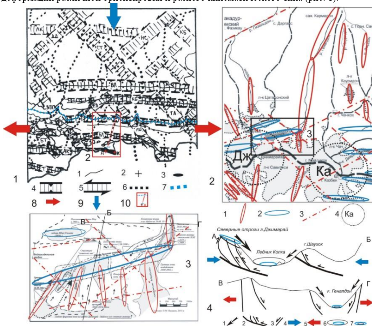
Рисунок 1. Схема 1. Структурно-кинематическая схема с элементами тектодинамики листа К-38-IX [9]. 1 – геологические границы; 2 – доальпийское основание; 3 – неоинтрузии; 4–6 – зоны концентрации деформаций: 4 – сжатия; 5 – сдвига (правого и левого); 6 – растяжения; 7 – эскарп Скалистого хребта; 8–9 – тектодинамические оси регионального растяжения (8) и сжатия (9); 10 – район Кармадонской катастрофы (область схемы 2). Схема 2. Район Кармадонской катастрофы (основа по [1]) 1 – долины по зонам растяжения, 2 – долины по зонам сжатия, 3 – линейменты по сдвиговым зонам, 4 – Казбекский и Джимарайский магматические центры. Прямоугольник – область схемы 3. Схема 3. Северный склон Джимарай-Казбекского горного узла (основа по [1]). Условные обозначения на схеме 2. Рис. 4. Схематические разрезы по линиям АВ и ВГ на схеме 3. 1 – направления тектоно-гравитационных потоков на склонах; 2 – система взбросо-надвигов, ретронадвигов и сбросов в висячих крыльях региональных широтных надвигов; 3 – системы меридиональных сбросов и диагональных сдвигов; 4–5 – оси напряжений: 4 – растяжения, 5 – сжатия; 6 – гравитационный и ледовый материал в зоне накопления (долины "сжатия"); 7 – гравитационный и ледовый материал в зонах активного выноса материала (долины "растяжения").
