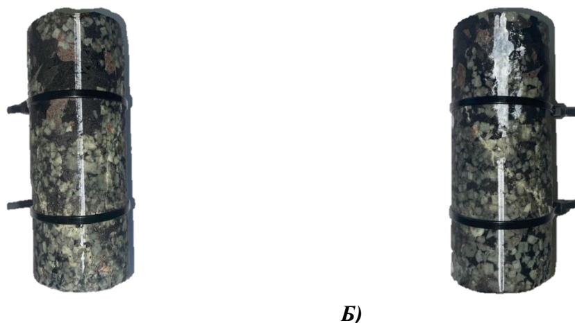
Рисунок 1. Образец массивного уртита в двух проекциях: А) – Южная проекция, Б) - Восточная проекция.
