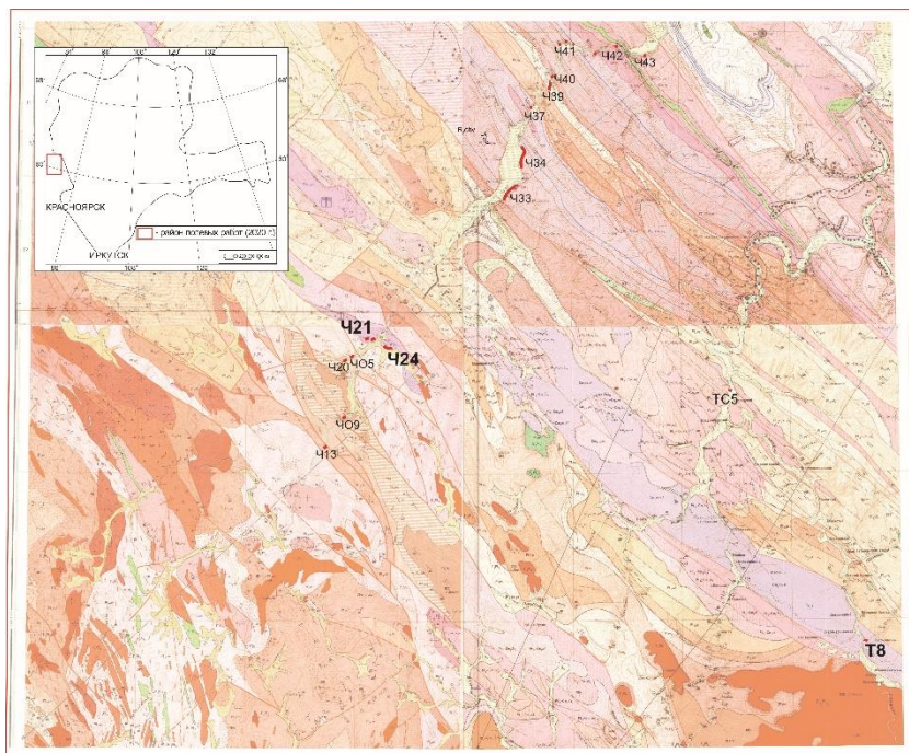
Рисунок 5. Карта района работ
