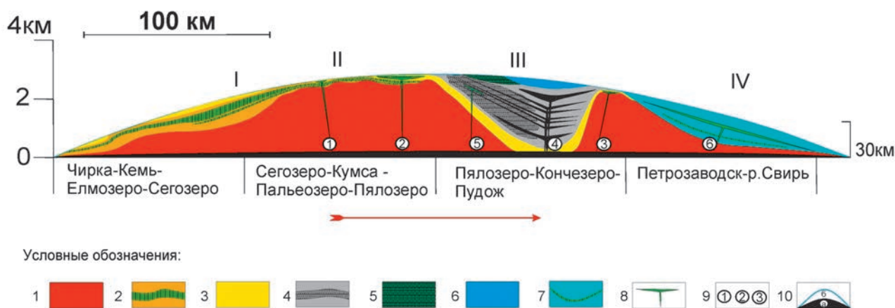
Рис. 2.19. Модель, отражающая характер проявления процессов силлогенеза в тектонической эволюции палеопротерозойской ОС на ятулийско-вепсийском этапах развития структуры (Сост. А.В. Полещук с использованием математических расчетов [Дэллмес, 1961; Косыгин, Магницкий, 1948; Робертс, 1972] и геологических материалов [Галдобина, 1982; Галдобина и др., 1972; Кайряк, 1973; Куликов и др., 1999; Полеховский, Голубев, 1989; Сацук и др., 1988; Светов, 1972, 1979; Соколов и др., 1970; Харитонов, 1966 и мн. др.], а также собственных наблюдений автора):
