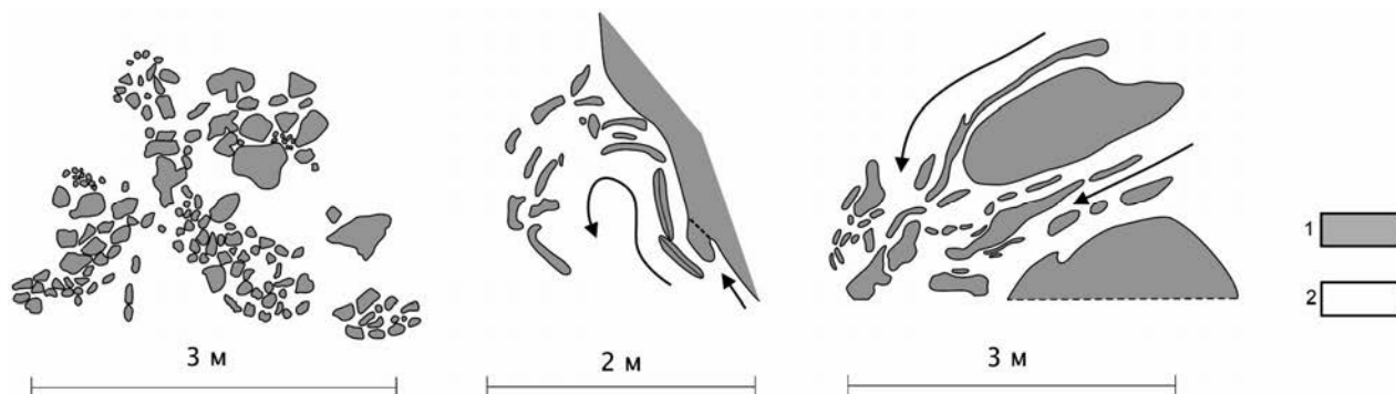
Рис. 2.14. Иллюстрация пластичных взаимоотношений шунгитонесущих пород и габбродолеритов и основные типы пеперитов в шунгитонесущих породах [Полещук, 2007]:
