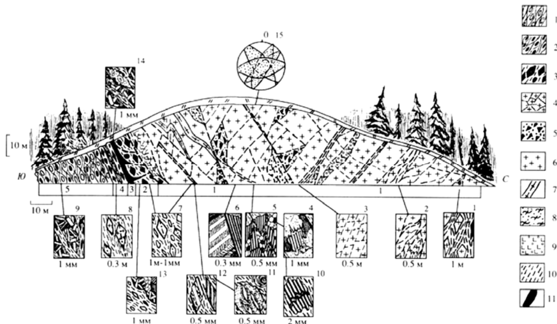
Рис. 2.6. Строение Кумсинского купола [Леонов и др., 1996]:
