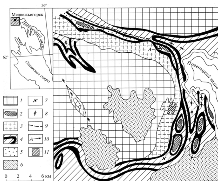
Рис. 2.5. Схема геологического строения северо-западного Прионежья и положение гранитных куполов:
