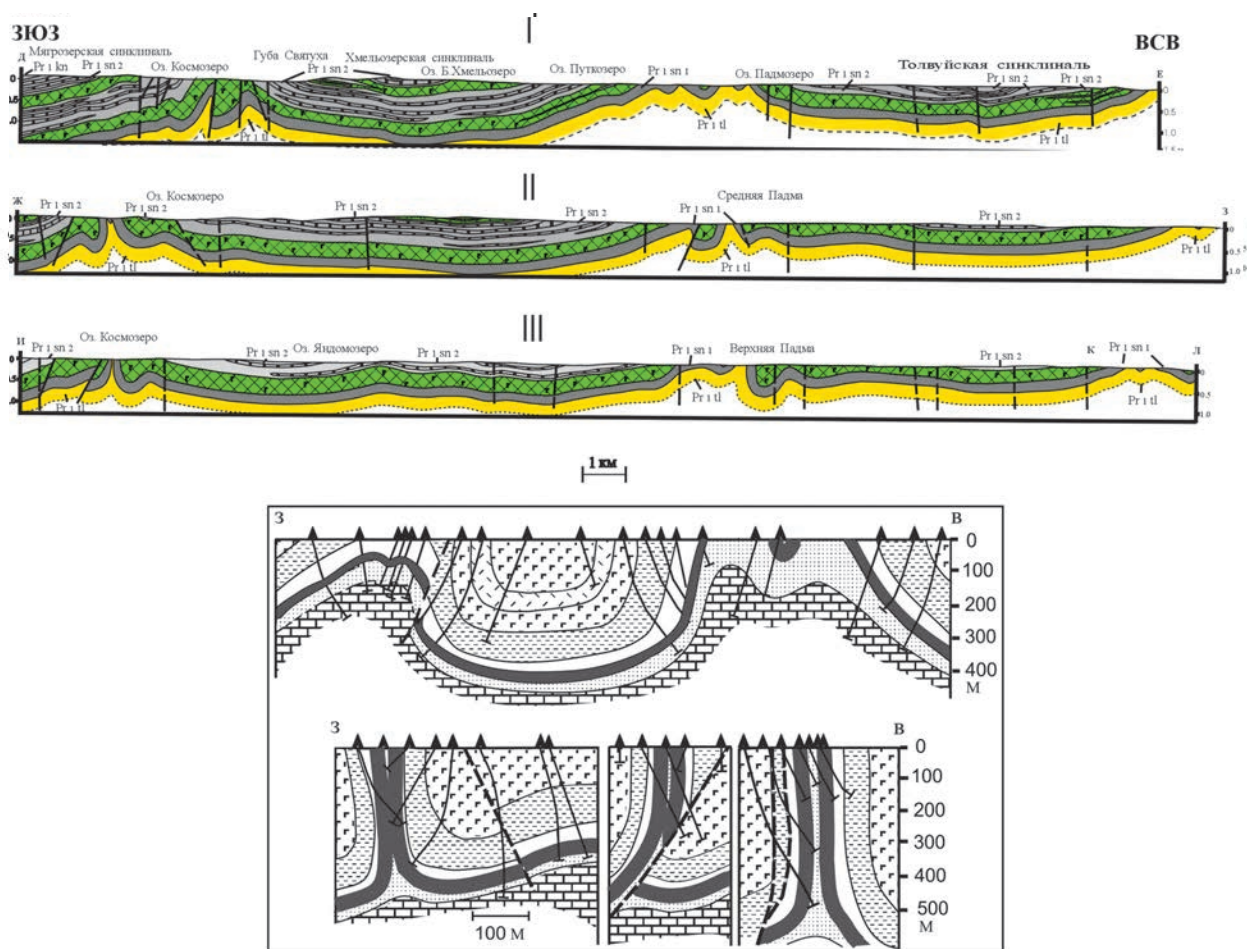
Рис. 2.2. Поперечные профили через псевдодиапировые антиклинальные структуры Северо-Онежского синклинория (по данным Отчета Карельской геологической экспедиции..., 1991):
