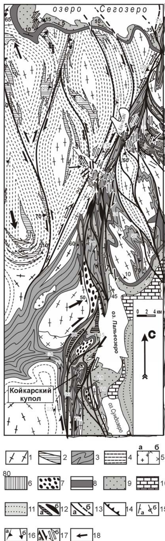
Рис. 2.7. Структурно-геологическая схема Койкарско-Сегозерской зоны концентрированной деформации (Сост. С.Ю. Колодяжный [2006] с использованием материалов ПГО «Севзапгеология» и [Войтович, 1971; Колодяжный, 1999; Сыстра, 1991]:
