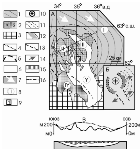
Рис. 2.11. Схема Онежской структуры с элементами новейшей структуры и геокинематической интерпретации (Сост. Д.С. Зыков):
