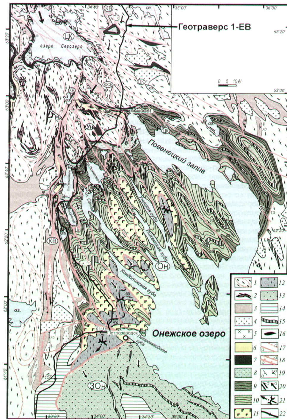
Рис. 2.1. Структурно-геологическая схема ОС (Сост. С.Ю. Колодяжный [2006] с использованием данных [Войтович, 1971; Новикова, Чахмахчев, 1967; Сыстра, 1991], фондовых материалов и личных наблюдений:
