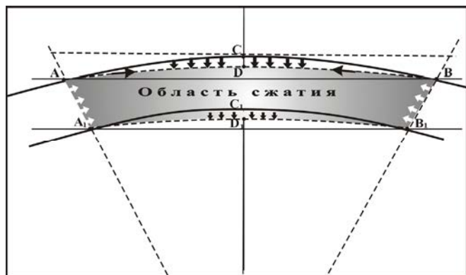
Рис. 2.18. Схема формирования первичного динамического бассейна (по: [Дэллмес, 1961]):
