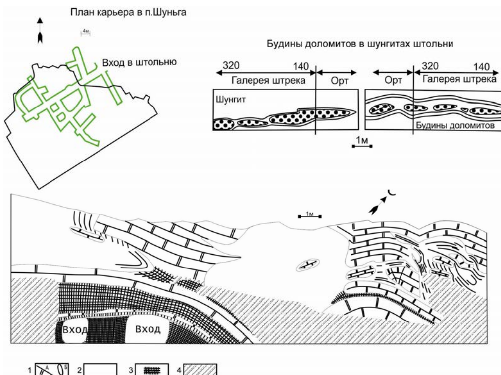
Рис. 2.13. Иллюстрация пластичных взаимоотношений пород шунгит-доломит-лигитового комплекса в карьере в п. Шуньга (над входом в штольню стенки карьера) [Полещук, 2006].
