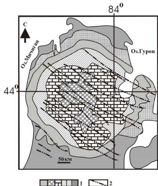
Рис. 2.17. Схема Мичиганского бассейна, отражающая соотношение центрально-симметричного строения и внутрибассейновой линейной складчатой структуры (по: [Бакиров, 1959]):
