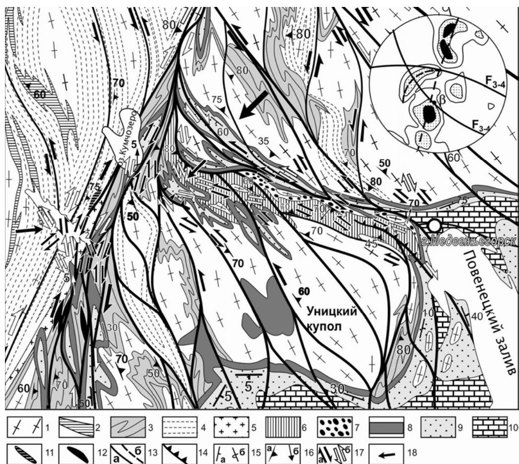
Рис. 2.10. Структурно-кинематическая схема Кумсинской сдвиговой зоны (Сост. С.Ю. Колодзяжный). Диаграмма – стереографическая проекция полюсов слоистости сумийско-ятулийских пород Кумсинской структуры: 141 замер, изолинии 1–4–8 %. Буквенные обозначения: F_{3-4} – осевые плоскости складок третьей – четвертой генерации, \beta – ось складчатости:
