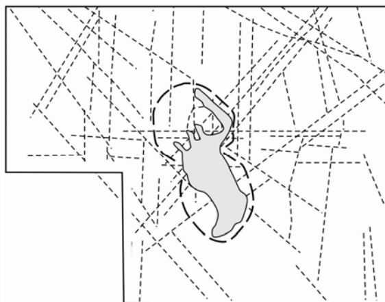
Рис. 2.12. Наложение новейшей Онежской депрессии (жирный пунктир) на сетку новейших разломных структур и линеаментов (тонкий пунктир) (по: [Кочнева и др., 2002])
