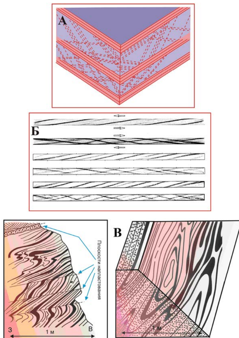
Рис. 2.3. А – структура кварцитопесчаников петрозаводской свиты (окрестности с. Соломенное); Б – формирование полос дислокации при сдвиге на границе слоев; В – межслоевые зоны проскальзывания.
