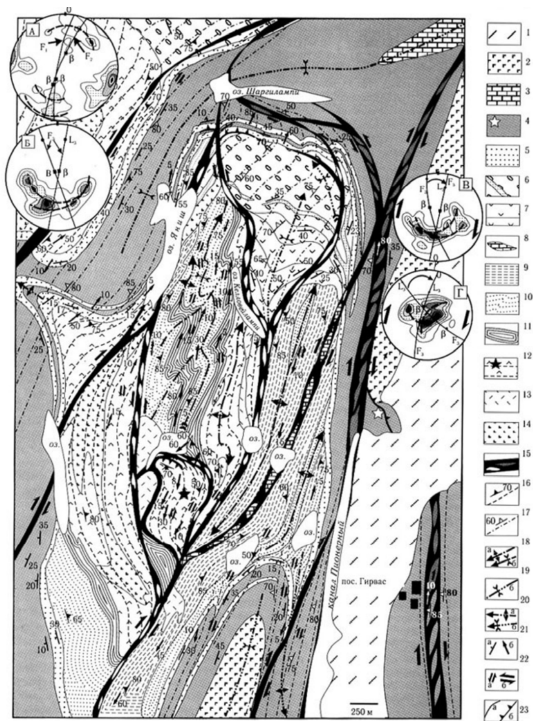
Рис. 2.8. Схема строения Койкарской антиклинали (Сост. С.Ю. Колодяжный [2006]):
