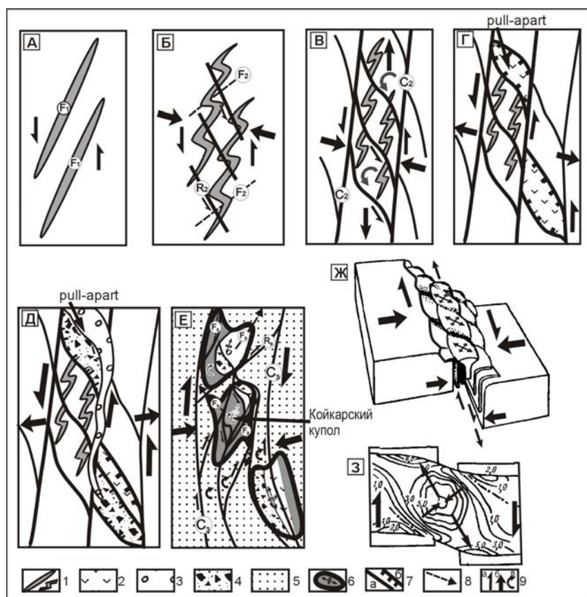
Рис. 2.9. Схема структурно-кинематической эволюции Койкарской зоны (Сост. С.Ю. Колодяжный [Леонов, Колодяжный, 2002]):
