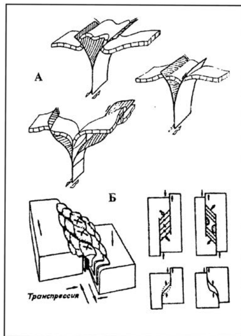
Рис. 2.4. Структуры цветка (пальмового дерева). А – по: [Alvarez, Maurin, 1991]. Б – по: [Морозов, Гептнер, 1997]
