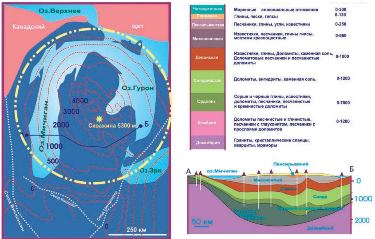
Рис. 2.16. Схема строения Мичиганского бассейна (по: [Кохи, Лэндс, 1961; Pirtle, 1932; Sleep, Sloss, 1978]). Объяснения в тексте
