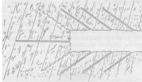
Рис. 158. Передовые гидрогеологические скважины (по Д. И. Щеголеву)
