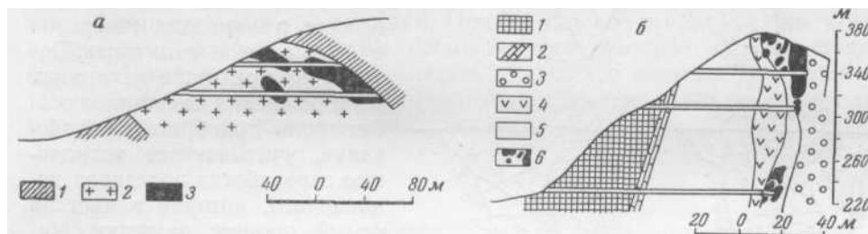
Рис. 92. Схема разведки слюдяных месторождений а — «жила» № 16 Мамского месторождения (по М. Ф. Маркову): / — кристаллические сланцы; 2 — мелкозернистый пегматит; 3 — пегматит с мусковитом б — рудник № 2 Слюдянского месторождения; / — гнейсы; 2 — мраморы; 3 — сиениты; 4 — пироксениты; 5 — гнейсы с пегматитовыми телами; 6 — ослюденные пегматиты
