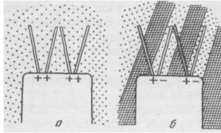
Рис. 96. Порядок отбора материала при шпуровом способе опробования
