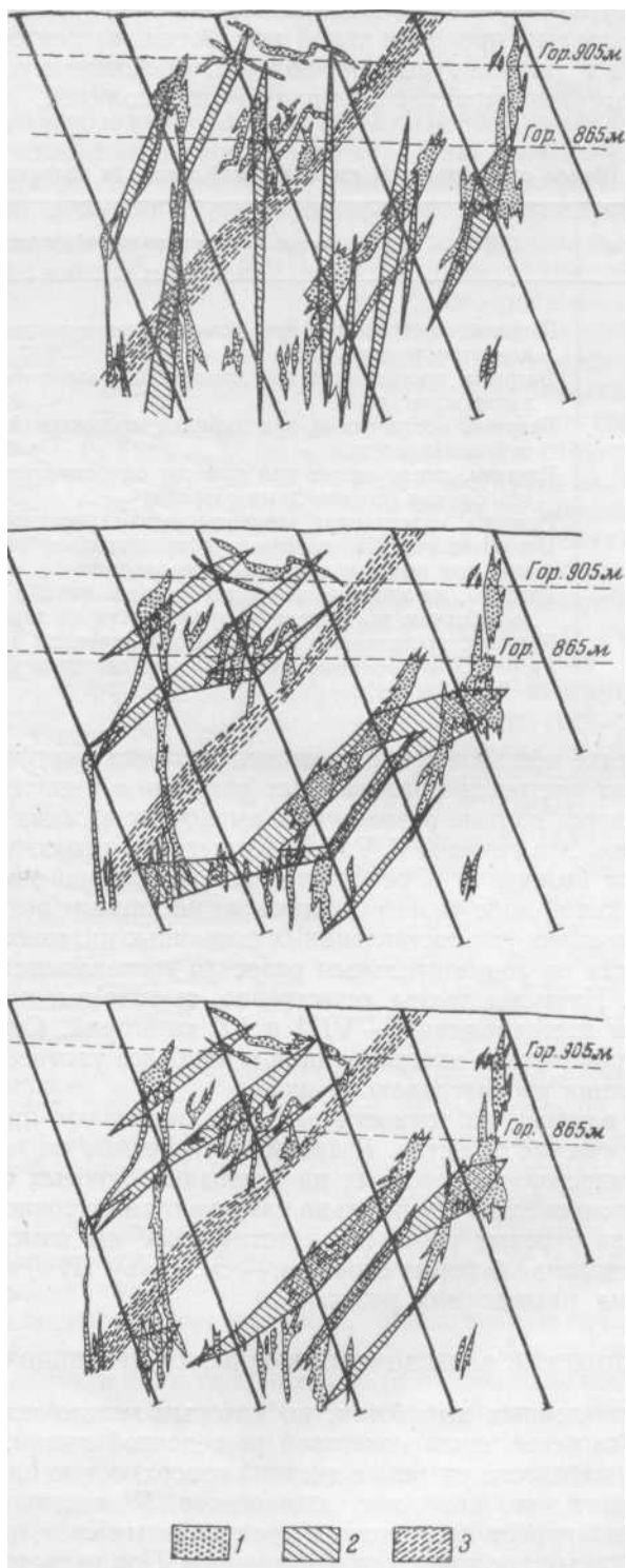
Рис. 17. Возможные варианты построения контуров морфологически сложных рудных тел по одним и тем же разведочным данным (по Д. А. Зенкову) 1 — истинные сечения рудных тел; 2 — сечения рудных тел, полученные путем интерполяции; 3 — зоны нарушений
