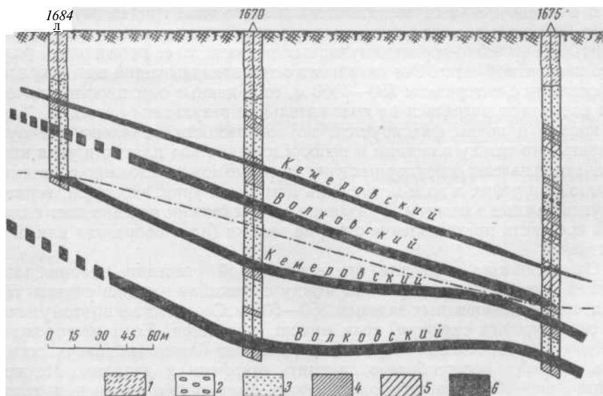
Рис. 77. Геологические разрезы по IV разведочной линии Петровского участка в Кузбассе (по Н. П. Гречишникову)
