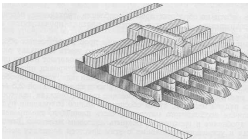
Рис. 111. Прибор С. М. Коломейченко для сокращения проб
