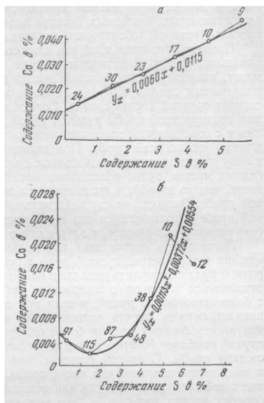
Рис. 108. Характер связи между содержанием Co и S в пиритизированных магнетитовых рудах (по Б. И. Галкину) а — прямая, б — криволинейная связь. Цифры около точек указывают на количество анализов, по которым вычислено среднее содержание Co и S в данной точке
