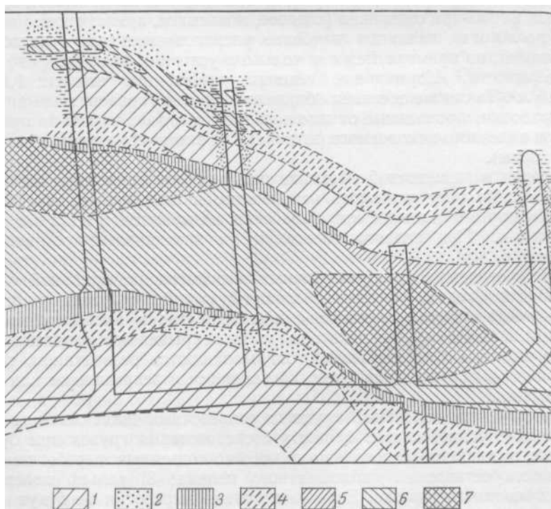
Рис. 28. Штрек с ортами, пересекающими параллельные рудные тела (по Ю. Г. Гершойгу)
