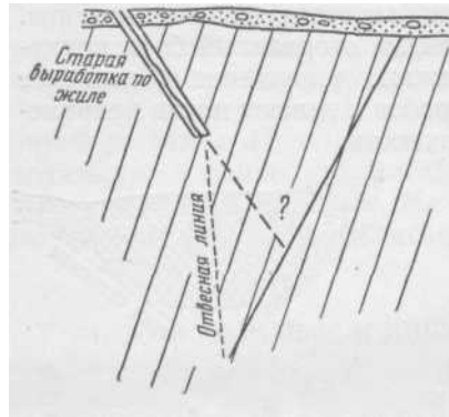
Рис. 82. Схема бурения разведочной скважины «до вертикали»*
