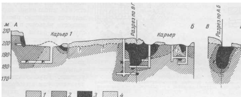
Рис. 37. Система шурфов с рассечками на месторождении Семиз-Бугу (по П. М. Татаринovu)
