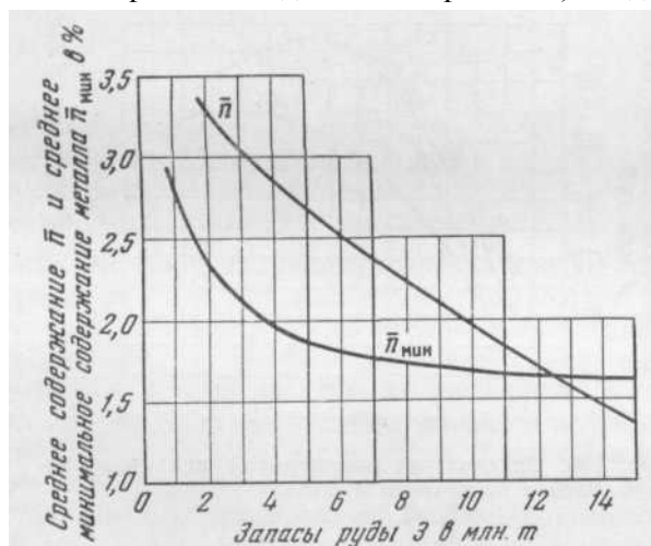
Рис. 134. Зависимость средних и средних минимальных содержаний металла от переменных запасов (по В. В. Померанцеву)
