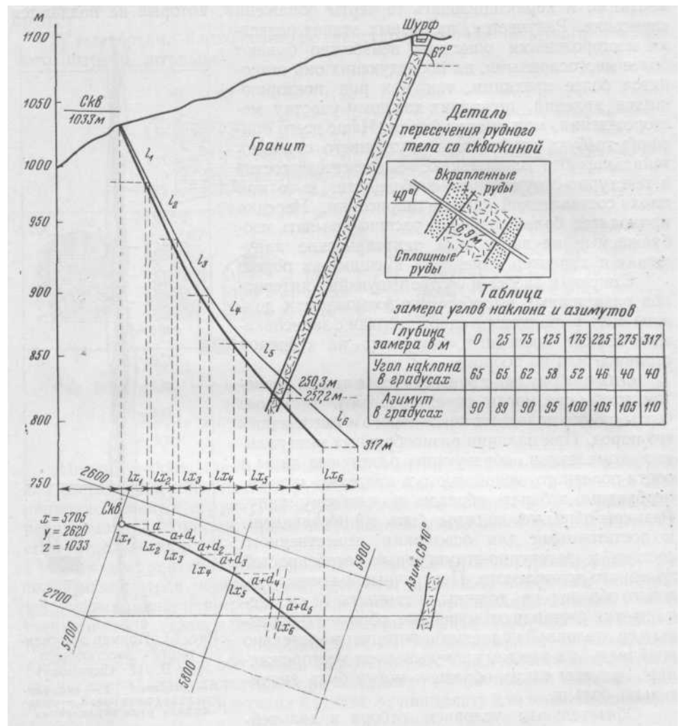
Рис 62. Построение скважины по данным измерений зенитных и азимутальных искривлений
