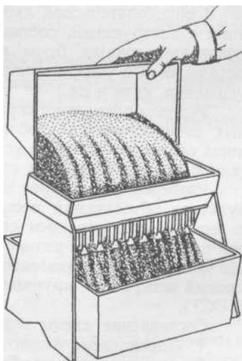
Рис. 112. Сокращение пробы делителем Джонса
