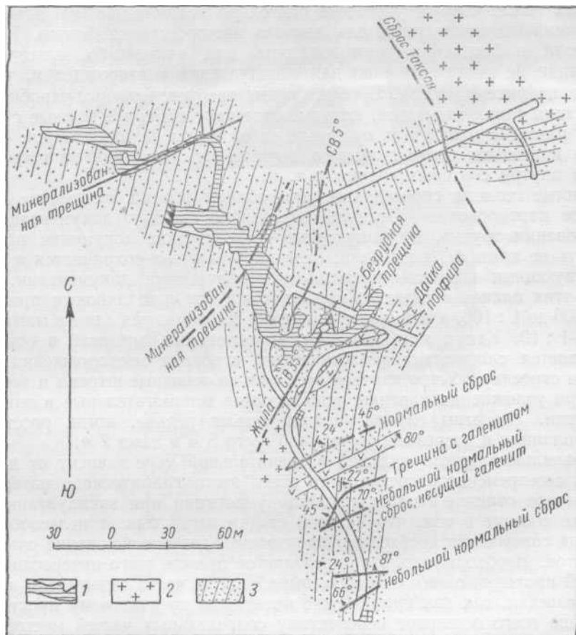
Рис. 154. Подземное картирование на руднике Таксон / — рудное тело; 2 — докембрийские граниты; 3 — кембрийские кварциты
