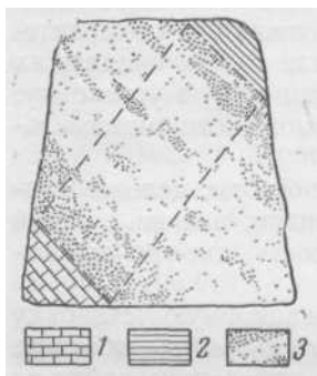
Рис. 103. Схема отбора проб при полосчатом распределении ценного компонента в рудном теле (по Б. И. Галкину)
