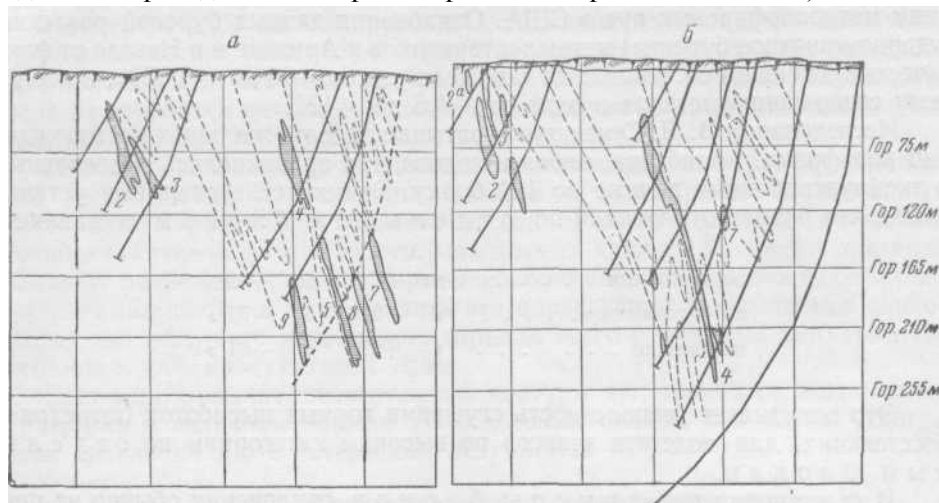
Рис. 47. Сопоставление контуров колчеданных линз, проведенных по данным бурения (а) и по результатам отработки (б) на разрезах вкрест простирания (по А. Б. Генбому)
