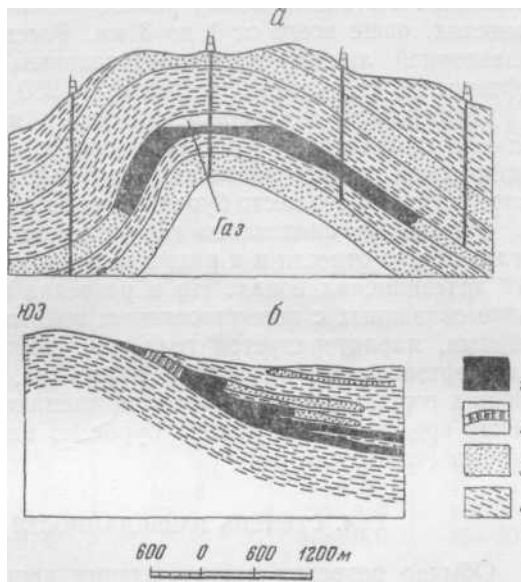
Рис. 54. Схема заложения разведочных скважин с учетом особенностей строения нефтяных месторождений
