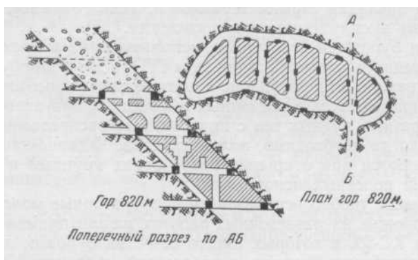
Рис. 140. Схема горных выработок, проходящих при разработке крутопадающей линзы (по А. В. Бричкину)
