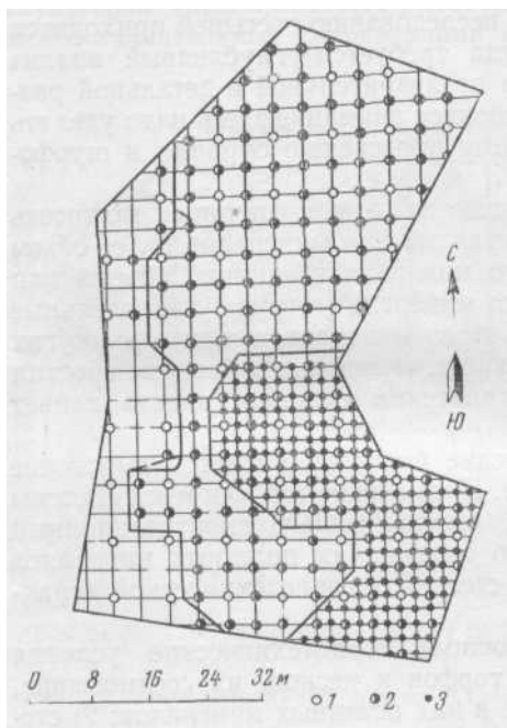
Рис. 73. Схема разведки оловянной россыпи (по Лэйку)
