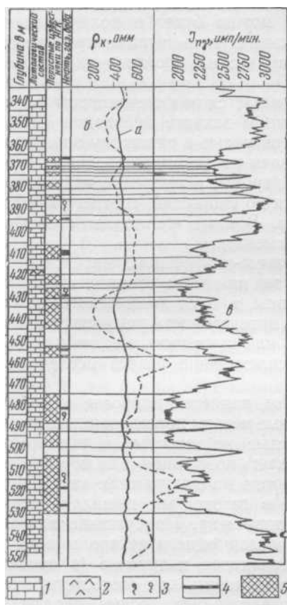
Рис. 33. Выделение нефтеносных и водоносных известняков нейтронным гамма-методом (по В. Н. Дахнову) а — кривая кажущегося сопротивления; б — то же в крупном масштабе; в — кривая интенсивности гамма-излучения / — известняки; 2 — ангидрит; 3 — газопроявления; 4 — нефтепроявления; 5 — пористые зоны
