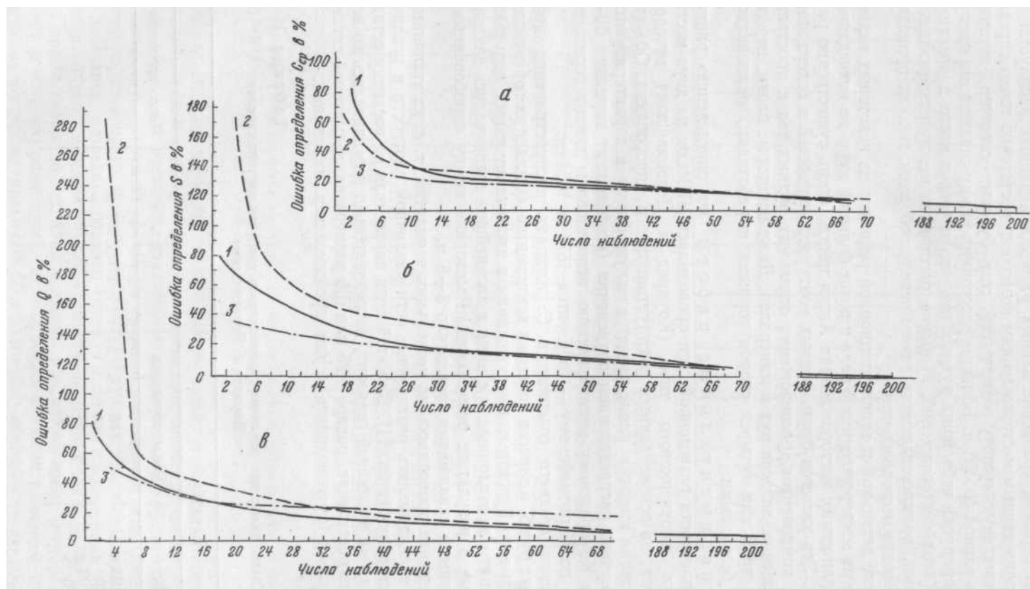
Рис. 48. Зависимость ошибок определения среднего содержания (а), площади оруденения (б) и запасов (в) от количества скважин (наблюдений) 1 — кривые максимальных ошибок определения C_{\text{ср}} , S и Q Для месторождения Коунрад; 2 — то же для горизонта 1674 м Первомайского месторождения; 3 — то же для горизонта 1664 м Первомайского месторождения
