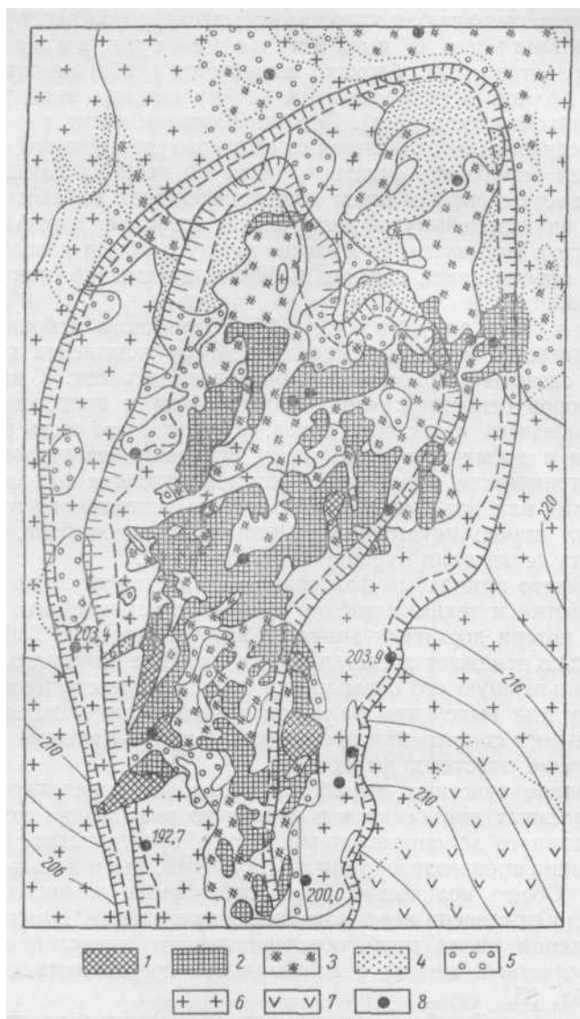
Рис. 157. План карьера на железорудном месторождении (по М. Н. Альбову)
