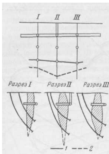
Рис. 21. Проведение внешнего контура по способу разрезов (по В. И. Смирнову) / — внутренний контур; 2 — внешний контур
