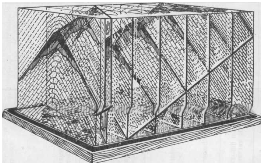
Рис. 71, Прозрачная модель месторождения
