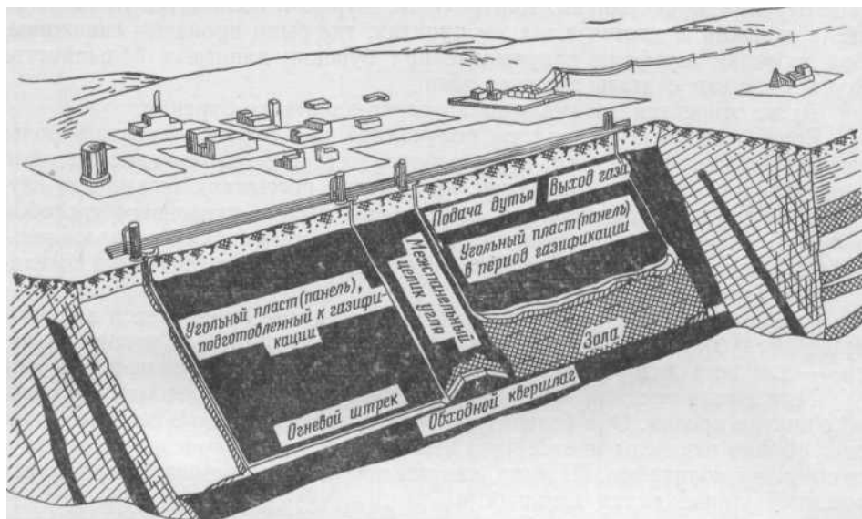
Рис. 76. Схема подземной газификации углей (по И. Ефременко и Н. Талызину)
