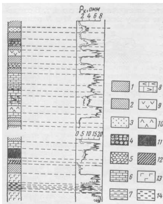
Рис. 32. Кривые кажущегося сопротивления, зарегистрированные микрозондом малого размера (точечная) и микрозондом большого размера (сплошная) (по В. Н. Дахнову)
