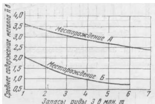
Рис. 129. Зависимость среднего содержания металла от переменных запасов вкрапленных руд двух месторождений (по В. В. Померанцеву)
