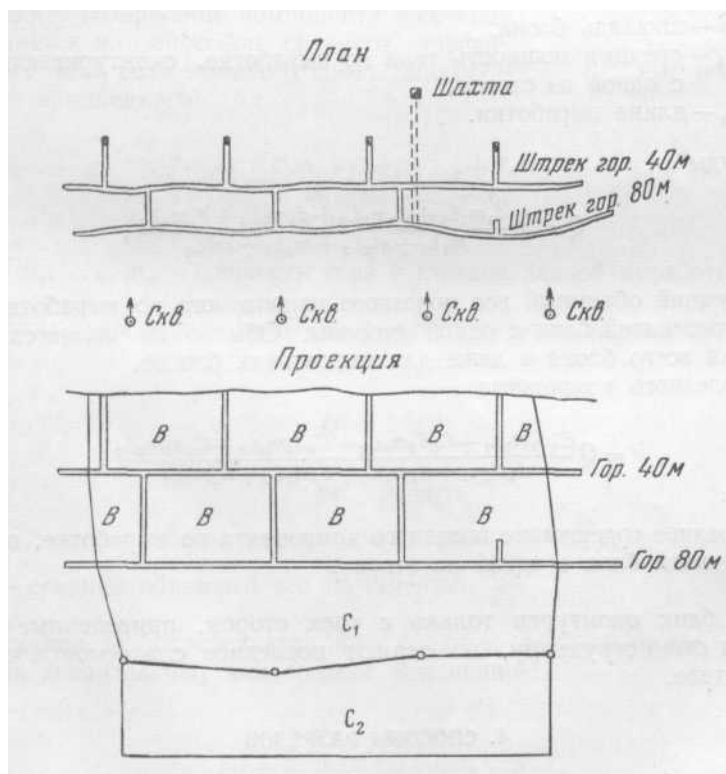
Рис. 121. План горных выработок по золоторудной жиле и проекция ее на вертикальную плоскость с построением блоков подсчета запасов
