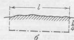
Рис. 23. Проведение внешнего контура в зависимости от длины тела по простиранию а — по правилу треугольника; б — по прямоугольному полотну
