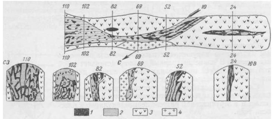
Рис. 60. Пример документации штольни при крутом падении тела полезного ископаемого (по Г. Д. Ажгирею)
