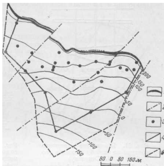
Рис. 20. Проведение внешнего контура по тектоническому нарушению на восточном фланге месторождения (по В. И. Смирнову, с видоизменениями) 1 — выход пласта; 2 — линии тектонических нарушений; 3 — буровые скважины, пересекающие рудное тело; 4 — линия внутреннего контура; 5 — линия внешнего контура
