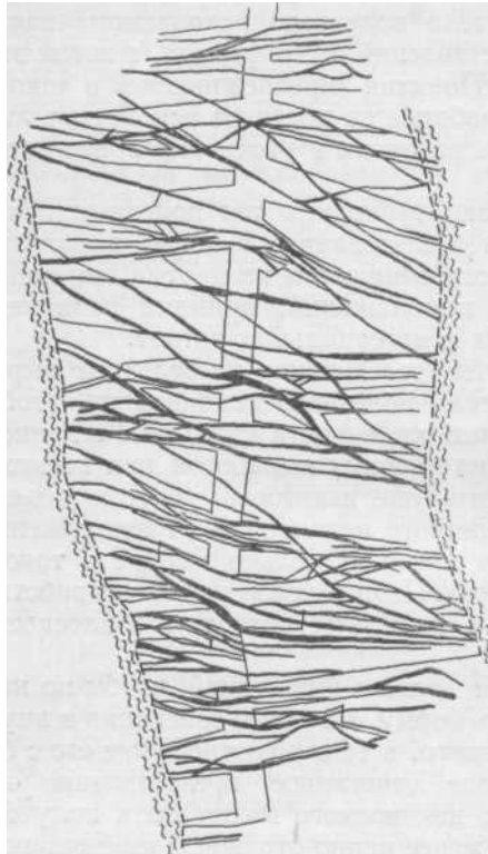
Рис. 16. Участок Березовской золоторудной дайки
