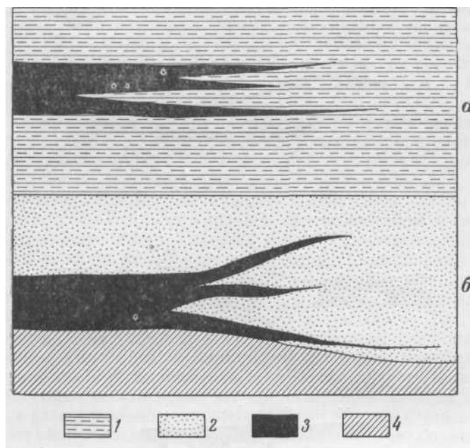
Рис. 150. Виды выклинивания угольных пластов в глинистых породах и песчаниках (по П. В. Васильеву) /— глины; 2 — песчаники; 3 — уголь; 4 — глинистые сланцы
