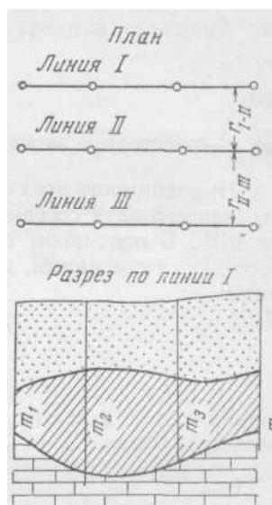
Рис. 122. Схема к подсчету запасов способом параллельных сечений
