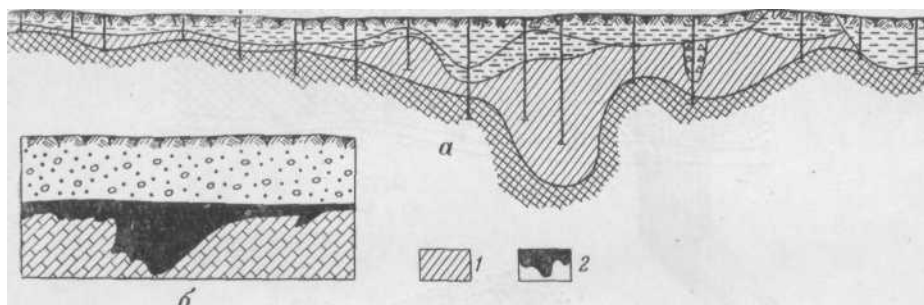
Рис. 12. «Карманы» экзогенных месторождений
