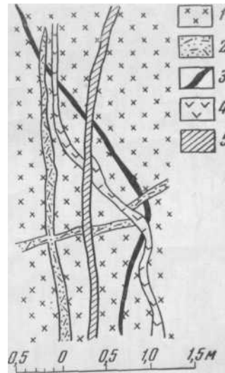
Рис. 148. Пересечение рудной жилы дайками (по Н. И. Бородаевскому) 1 — гранит; 2 — пегматит; 3 — золотоносная кварцевая жила; 4 — лампрофир; 5 — аплит
