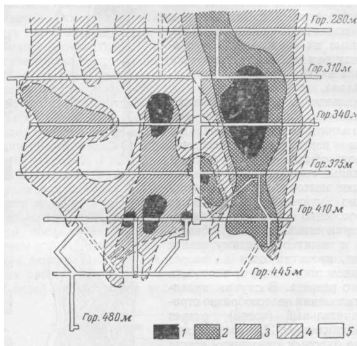
Рис. 67. Проекция изолиний содержания металла на осевую плоскость рудного тела
