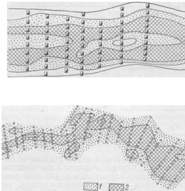
Рис. 11. Обогащенные «струи» в россыпях (по Купер-Конину)
