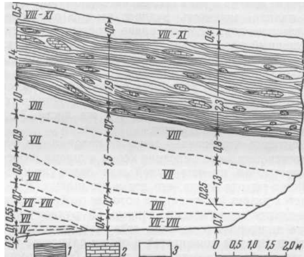
Рис. 106. Пример геологической документации на медном руднике по естественным типам руд (визуальное опробование)
