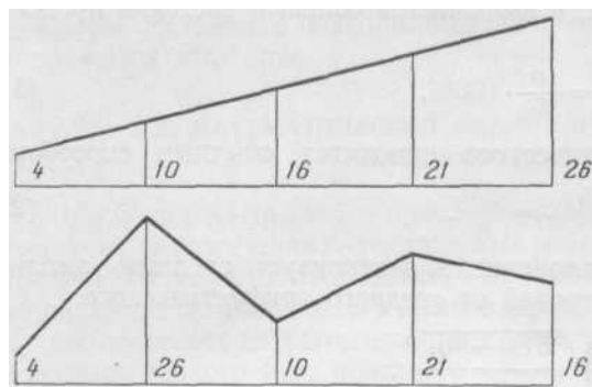
Рис. 1. Различный характер изменчивости при одинаковой степени изменчивости
