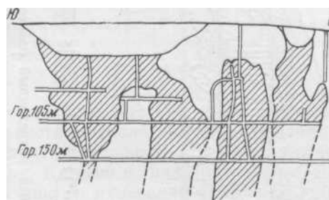
Рис. 65. Проекция общих контуров рудных тел на вертикальную плоскость
