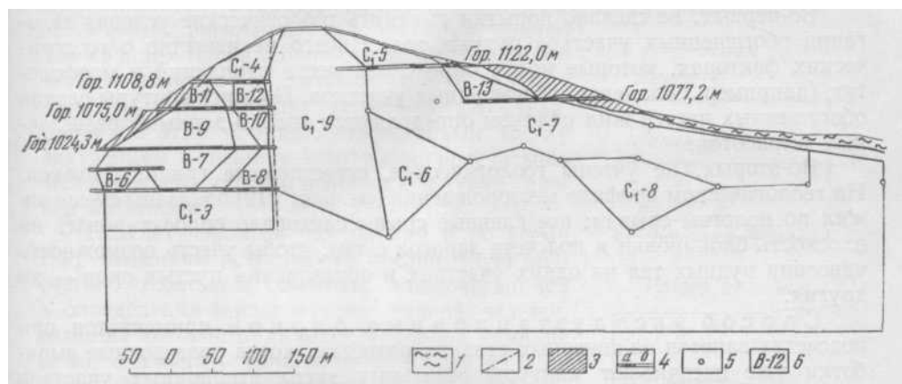
Рис. 120. Проекция на вертикальную плоскость полиметаллической жилы с построением блоков подсчета запасов / — четвертичные отложения; 2 — дизъюнктивные нарушения; 3 — отработанные участки жилы; 4 — интервалы штолен с кондиционным (а) и некондиционным (б) содержанием свинца и цинка; 5 — точки пересечения жилы скважинами колонкового бурения; 6 — категории запасов и номера подсчетных блоков
