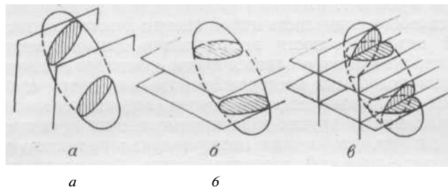
Рис. 15. Основные виды разведочных разрезов а — схема вертикальных разрезов; б — схема горизонтальных разрезов; в — схема вертикальных и горизонтальных разрезов
