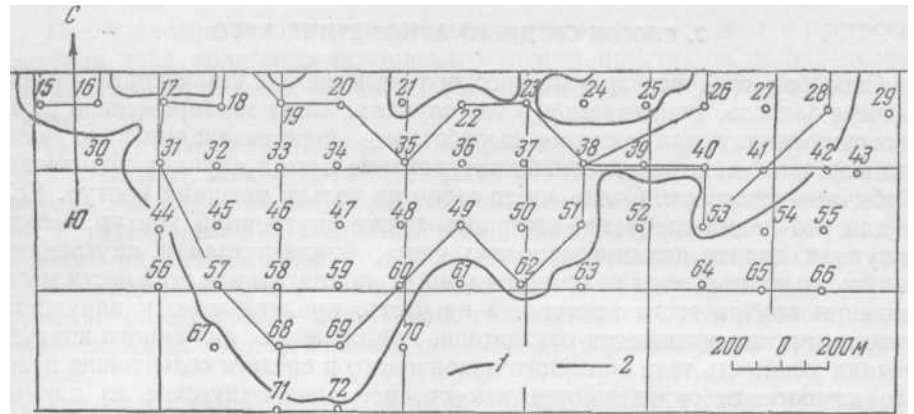
Рис. 118. Схема подсчета запасов способом среднего арифметического в поле шахты № 13 Подмосковского угольного бассейна (по Г. Г. Денисову)
