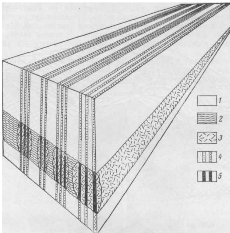
Рис. 69. Блок-диаграмма перспективная 1 — метаморфические сланцы; 2 — амфиболиты; 3 — оруденелые амфиболиты; 4 — кварцево-сульфидные жилы; 5 — участки кварцевых жил с повышенной концентрацией оруденения
