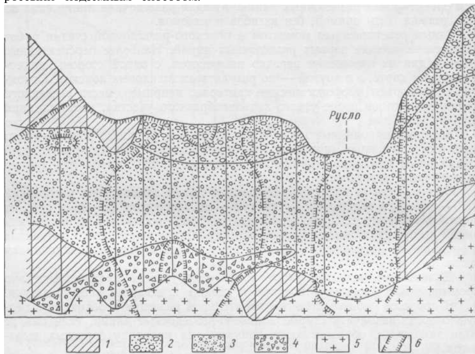
Рис. 75. Разрез по разведочной линии через россыпь р. Куронах / — глина; 2 — крупновалунный слой; 3 — речник; 4 — щебенка с песком; 5 — плотик; «—» — границы многолетней мерзлоты
