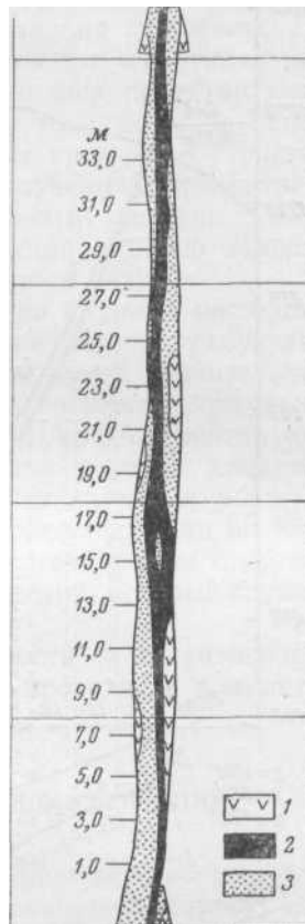
Рис. 61. Пример документации восстающего (по В. И. Смирнову) / — диориты; 2 — сульфидная руда сплошная; 3 — сульфидная руда вкрапленная
