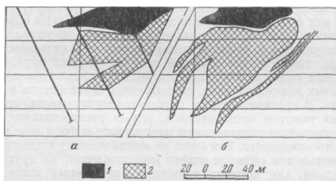
Рис. 46. Контуры Полиметаллического рудного тела (по П. С. Бернштейну)
