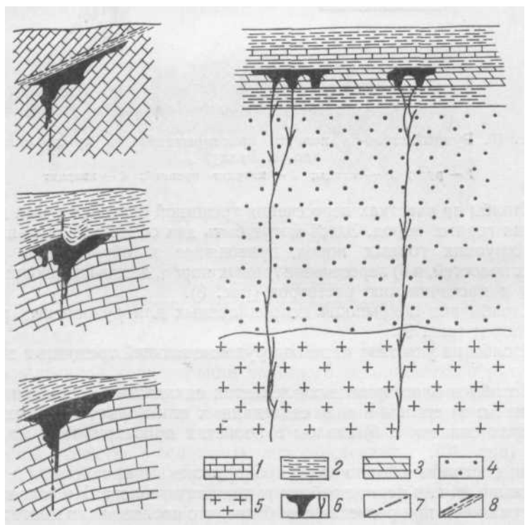
Рис. 9. Рудные столбы под покрывкой непроницаемых горных пород
