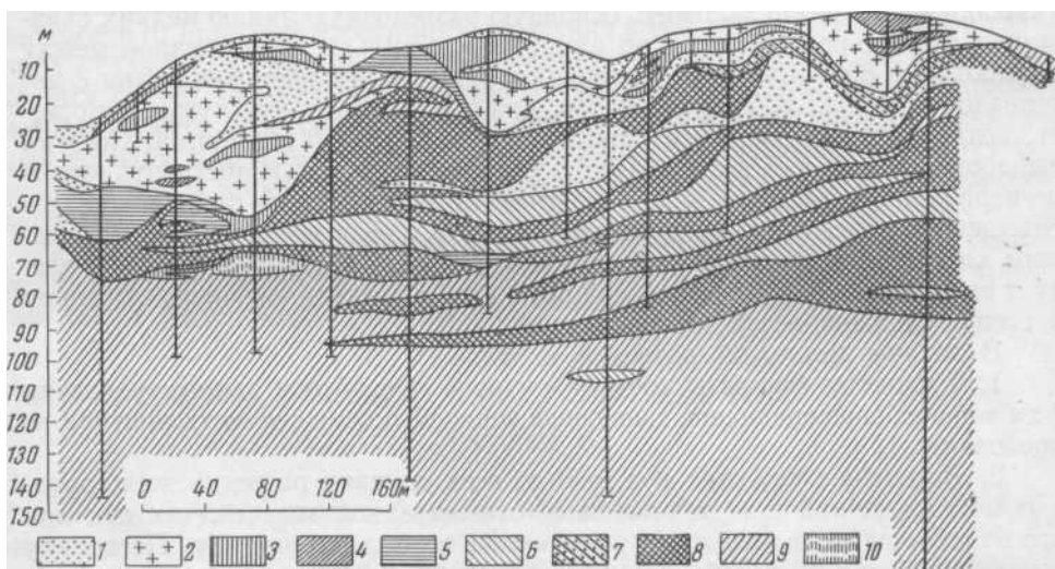
Рис. 72. Меридиональный разрез Аккермановского месторождения по участку № 2 (по К. Н. Трубину)
