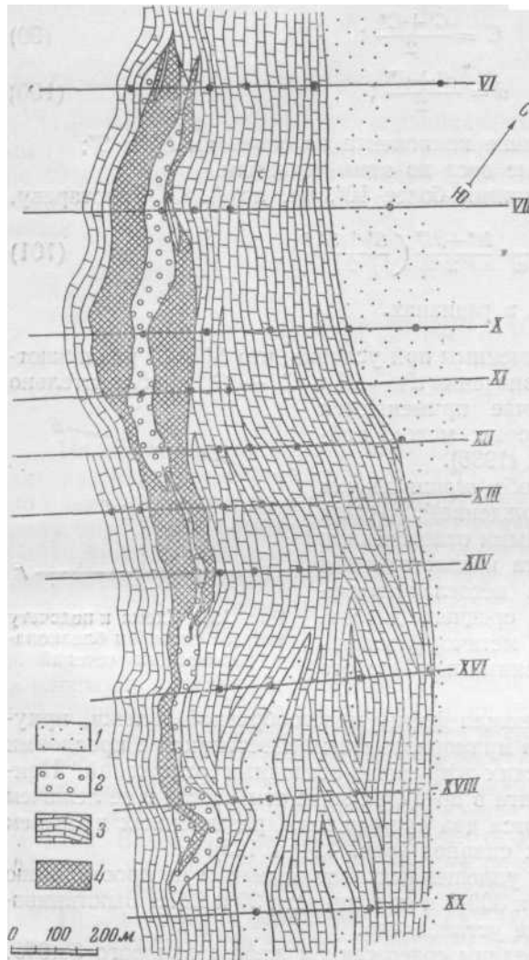
Рис. 124. Геологический план Белорецкого месторождения
