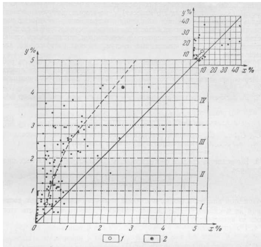
Рис. 116. Диаграмма сопоставления данных точечного ( y ) и бороздового ( x ) опробования / — средние значения по классам; 2 — среднее значение по серии
