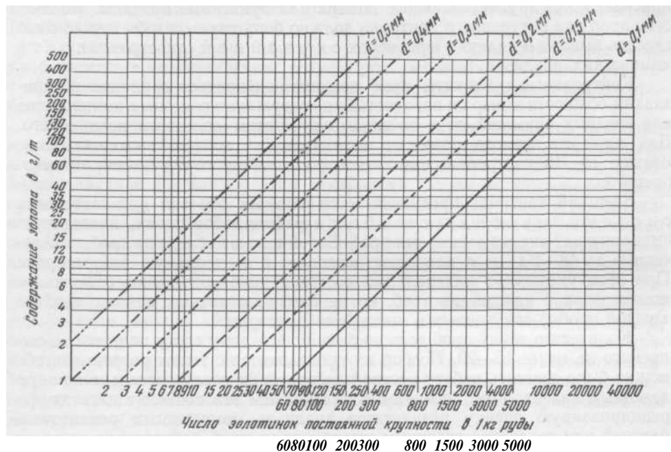
Рис. 114. Диаграмма ориентировочной зависимости между числом золотинок кубической формы в килограммовой пробе руды и содержанием в ней золота с тщательным сохранением хвостов. Предел измельчения зависит от крупности золота и колеблется приблизительно от — 1 до — 0,4 мм. Особое внимание обращается на тщательное сохранение хвостов. Для предотвращения потерь промывка производится на лотке в специальном железном баке, на дно которого осаждаются хвосты.
