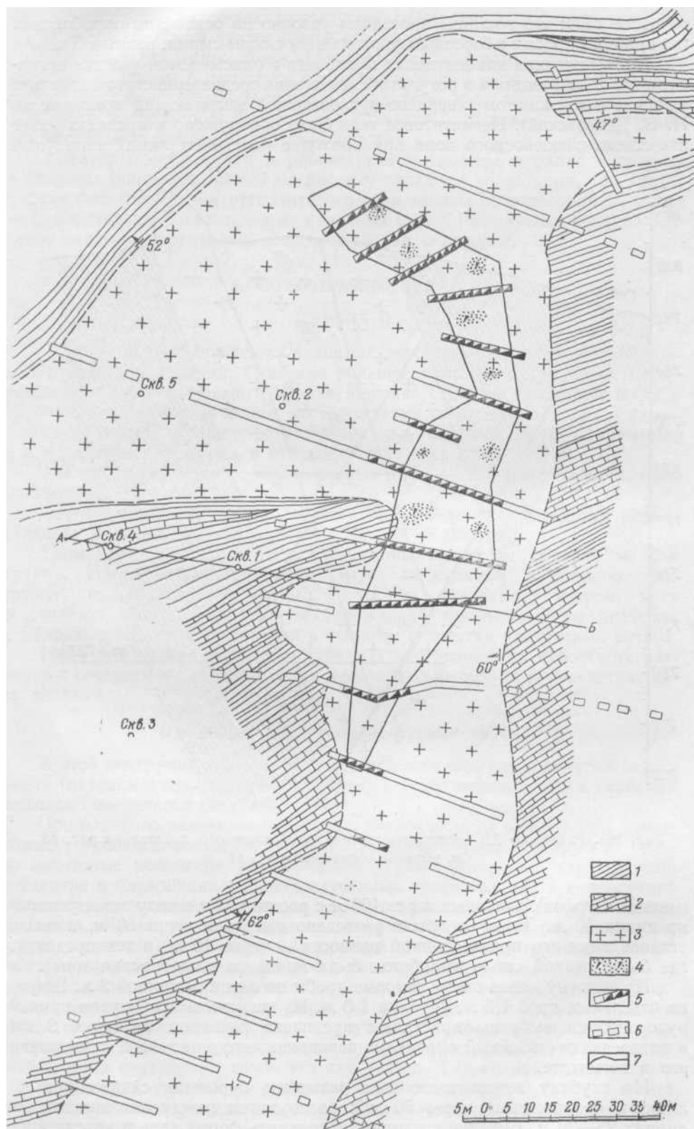
Рис. 88. Схема разведки одного из пегматитовых тел
