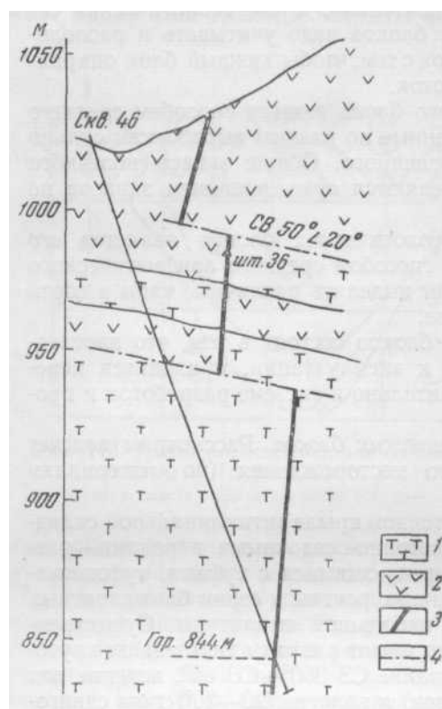
Рис. 119. Геологический разрез через одну из жил полиметаллического месторождения
