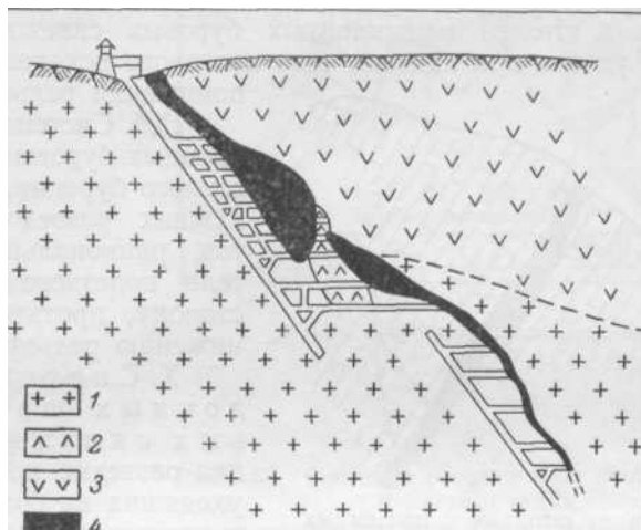
Рис. 42. Система разведки наклонной шахтой с квершлагами (рудник Крейтон, Сёдбери) 1 — граниты; 2 — зеленокаменные породы; 3 — нориты; 4 — сульфидные руды
