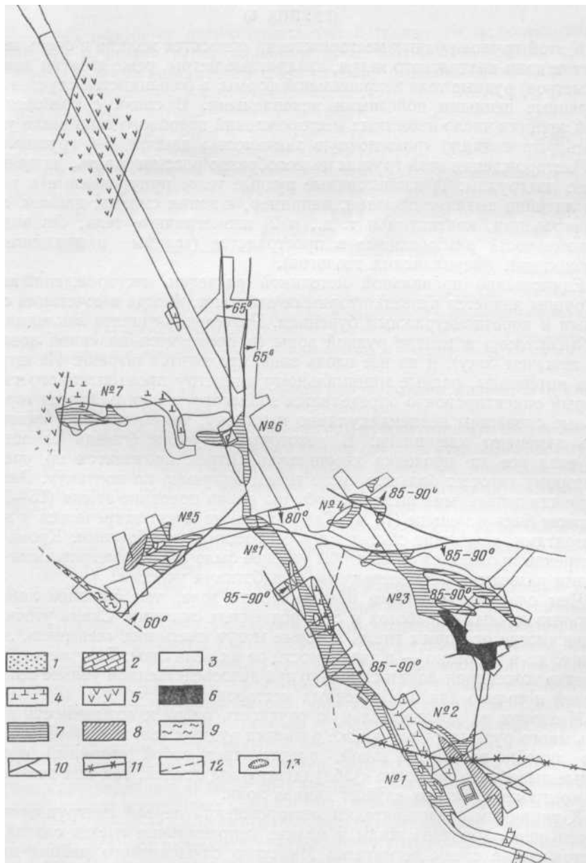
вого горизонта (б) рудника Курусай (по Ф. И. Вольфсону) ровзтые мраморы и мраморизованные известняки; 4 — микродиориты; 5 — кварцевые 9 — зоны брекчирования; 10 — тектонические трещины лорудные; // — тектониче- 13 — древние выработки. Цифрами на рисунке указаны номера рудных тел
