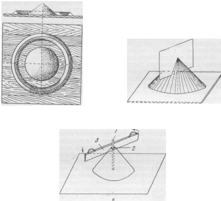
Рис. 110. Перемешивание способом кольца и конуса
