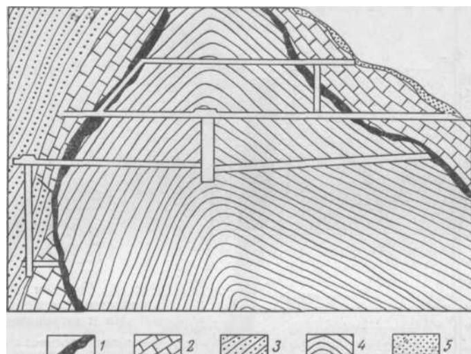
Рис. 39 Система разведки штольнями со слепыми шахтами (по П. М. Татарину)
