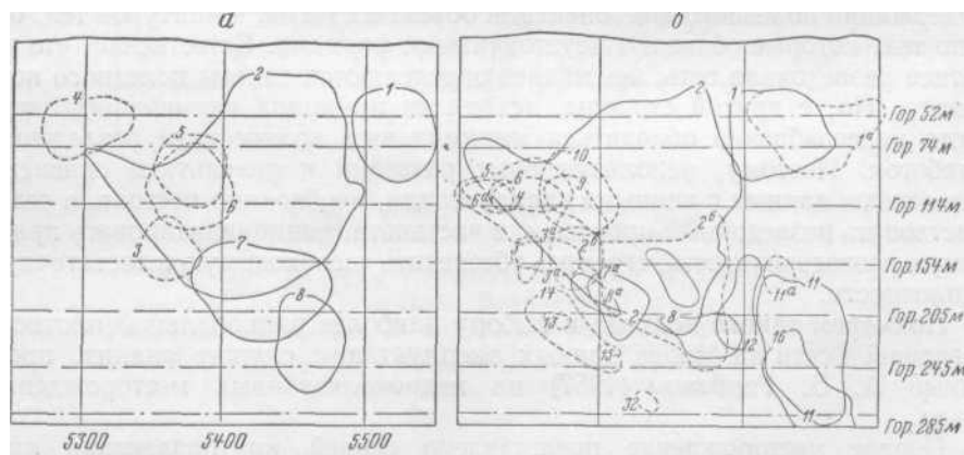
Рис. 47а. Сопоставление контуров колчеданных линз, проведенных по данным бурения (а) и по результатам отработки (б) в продольной проекции на вертикальную плоскость (по А. Б. Генбому)
