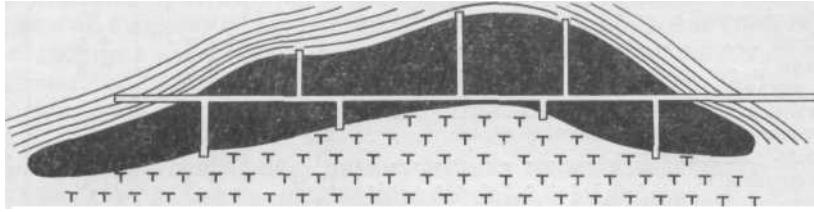
Рис. 29. Восстающие и гезенки, пройденные из горизонтальной выработки для пересечения пологой рудной залежи
