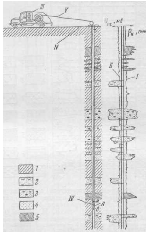
Рис. 31. Схема электрометрии скважины методом сопротивления и потенциалов собственной поляризации пород (по В. Н. Дахнову)
