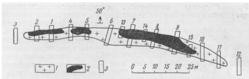
Рис. 91. Разведка пегматитовой жилы канавами / — пегматит; 2 — промышленные скопления мусковита; 3 — канавы (цифры указывают порядок их заложения)
