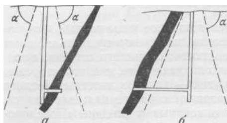
Рис. 27. Соотношения контуров рудных тел и околошахтных охранных целиков ( 70^\circ < \alpha < 80^\circ )
