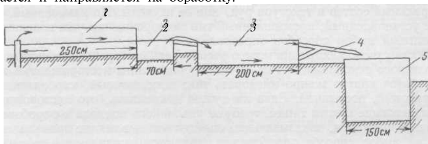
Рис. 105. Установка для сбора шлама
