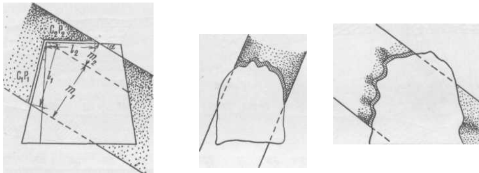
Рис. 99. Примеры взятия бороздовых проб при неравномерном распределении полезного компонента (по Б. И. Галкину)
