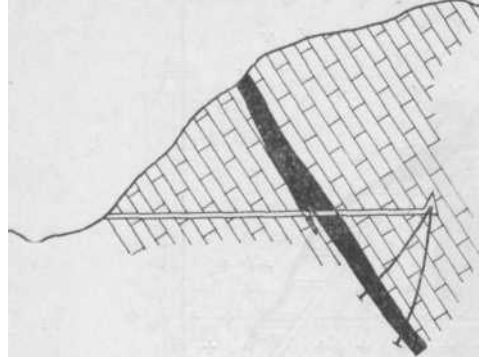
Рис. 43. Сочетание штольни и подземных буровых скважин
