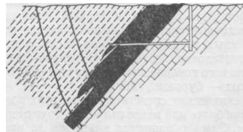
Рис. 44. Сочетание разведочной шахты с буровыми скважинами
