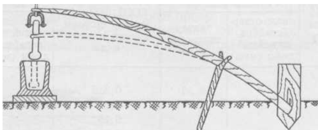
Рис. 109. Дробление пробы пестом с баланси́ром
