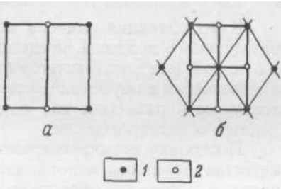
Рис. 52. Сгущение с изменением вида сети а — превращение квадратной сети в прямоугольную; б — превращение ромбической сети в прямоугольную / — выработки первой очереди; 2 — выработки второй очереди
