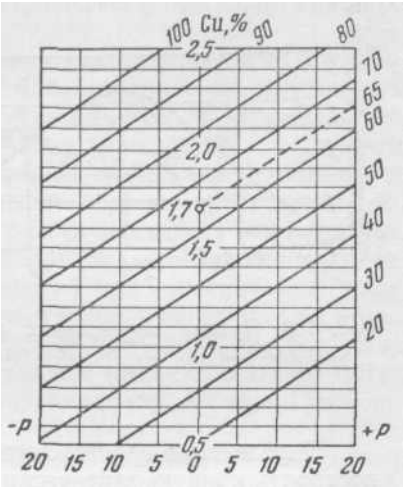
Рис. 137. Номограмма для определения минимального среднего содержания меди в монометаллической руде (по В. В. Померанцеву)
