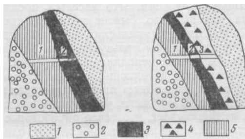
Рис. 102. Секционное опробование на месторождении Ni-Co-руд
