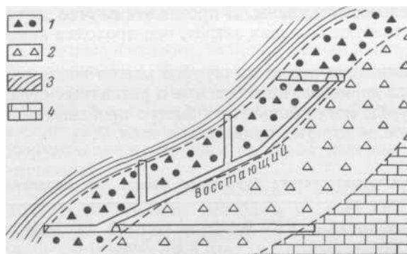
Рис. 30. Наклонный восстающий по рудному телу (по А. К- Полякову)
