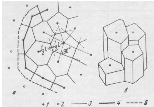
Рис. 128. Подсчет запасов по способу ближайшего района
