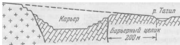
Рис. 160. Барьерный целик, ограждающий известняковый карьер (по М. П. Альбову)
