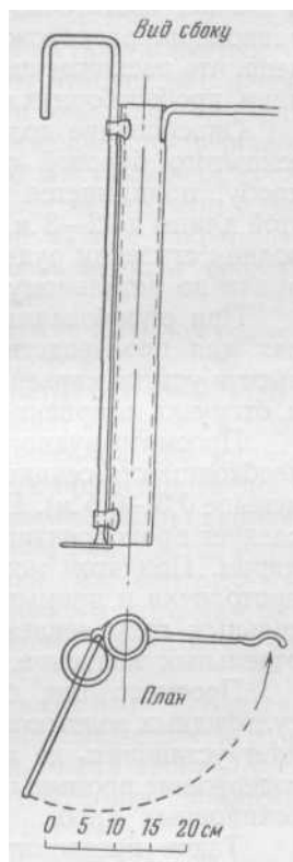
Рис. 104. Ручной пробоотборник системы Тихомирова и Коломейченко
