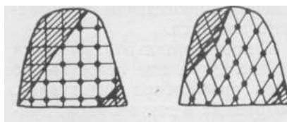
Рис. 94. Схемы отбора проб точечным способом
