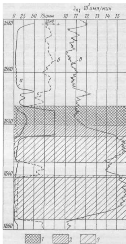
Рис. 34. Определение положения водонефтяного контакта нейтронным гамма-методом а — кривая кажущегося сопротивления; б — кривая потенциалов собственной поляризации; в — кривая интенсивности нейтронного гамма-излучения / — нефтеносная часть пласта; 2 — переходная зона; 3 — водоносная часть пласта
