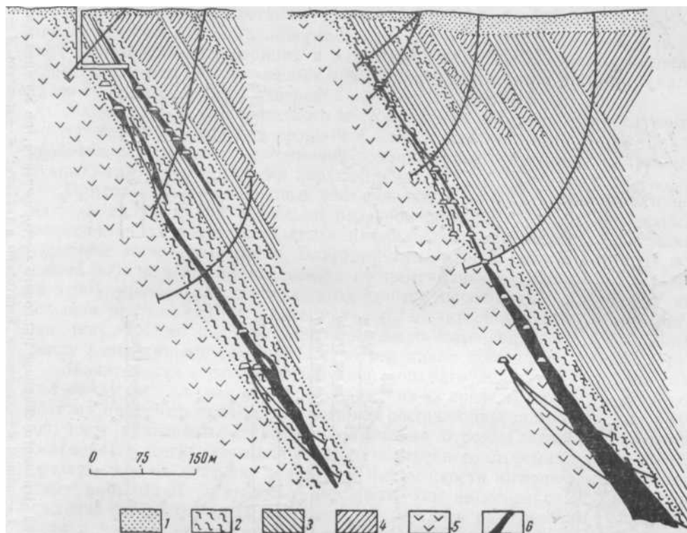
Рис. 84. Схема разведки медноколчеданного месторождения, представленного несколькими жиллообразными залежами (по материалам ГРП) / — наносы; 2 — кварцево-серицитовые и кварцево-хлорито-серицитовые сланцы; 3 — кварцево-хлоритовые, эпидото-хлоритовые сланцы, частично порфиритоиды; 4 — кремнистые и хлоритоглинистые сланцы; 5 — зеленокаменные породы; 6 — медистый колчедан
