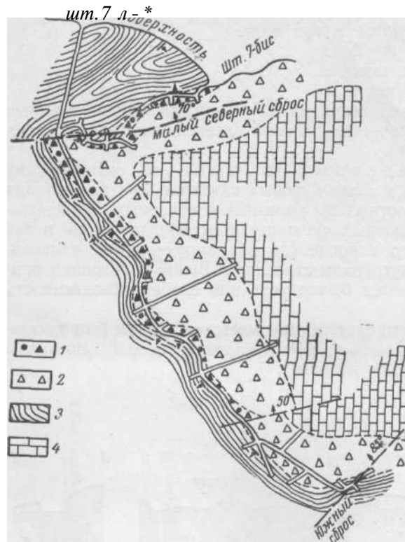
Рис. 38. Разведка штольней с рассечками (по А. К. Полякову) — оруденелая брекчия промышленная; 2 — оруденелая брекчия непромышленная; 3 — сланцы; 4 — известняки
