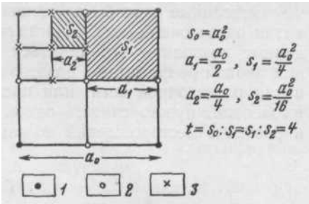
Рис. 50. Сгущение разведочной сети уменьшением расстояния между выработками вдвое 1 — выработки первой очереди; 2 — выработки второй очереди; 3 — выработки третьей очереди
