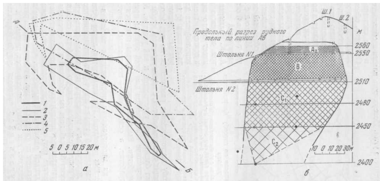
Рис. 127. Схема к подсчету запасов по полиметаллическому месторождению
