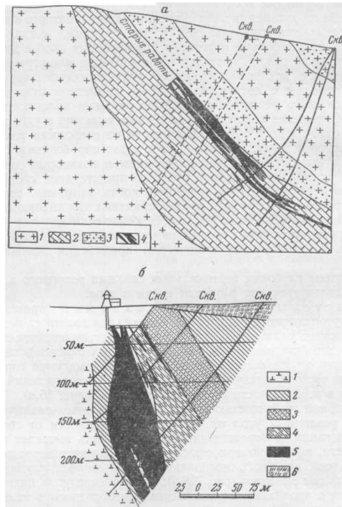
Рис. 36. Система наклонных буровых скважин а — система доразведки жил Савинского месторождения: / — кварцевые диориты; 2 — известняки; ^ — сланцы и кварциты; 4 — рудные тела б — система разведки медистых колчеданов: / — альбитофиры; 2 — сланцы; 3 — сланцы окварцованные; 4 — сланцы пиритизированные; 5 — колчедан; 6 — бурые глины
