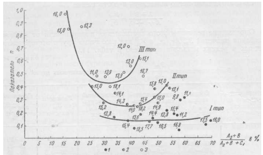
Рис. 56. Кривые соотношений разведки и метража буровых скважин по Прокопьевско-Киселевскому району Кузбасса (по В. Я. Каудельному) / — данные по участкам простого геологического строения; 2 — данные по участкам сложного геологического строения; 3 — данные по участкам очень сложного геологического строения. Цифры возле точек показывают рабочую угленосность толщи
