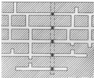
Рис. 141. Система подготовительных выработок, используемых для эксплуатационной разведки (продольная проекция жилы на вертикальную плоскость) (по А. В. Бричкину)
