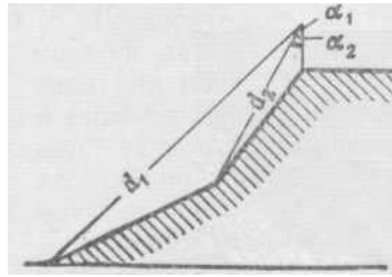
Рис. 156. Съемка профиля уступа (по М. Н. Альбову)
