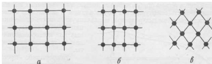
Рис. 18. Правильные разведочные сети а — квадратная; б — прямоугольная; в — ромбическая
