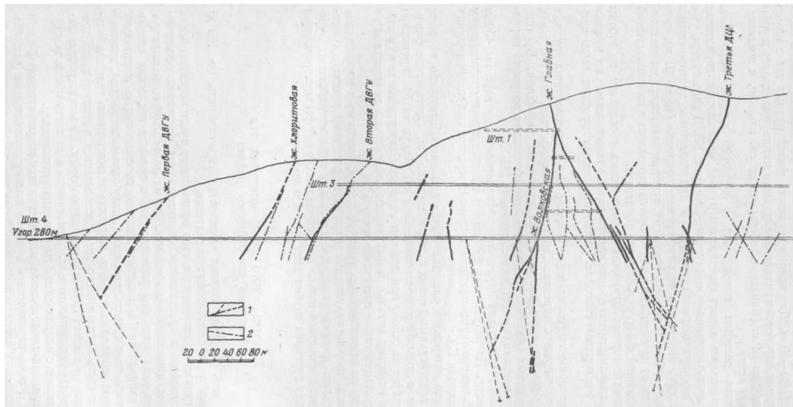
Рис. 87. Разрез по оси штольни № 4 на Хрустальном месторождении (по В. П. Полохову) / — рудные жилы; 2 — тектонические нарушения
