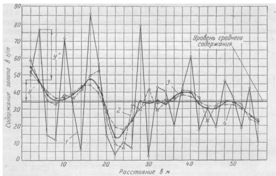
Рис. 3. Построение кривой регрессии (по П. Л. Каллистову)
