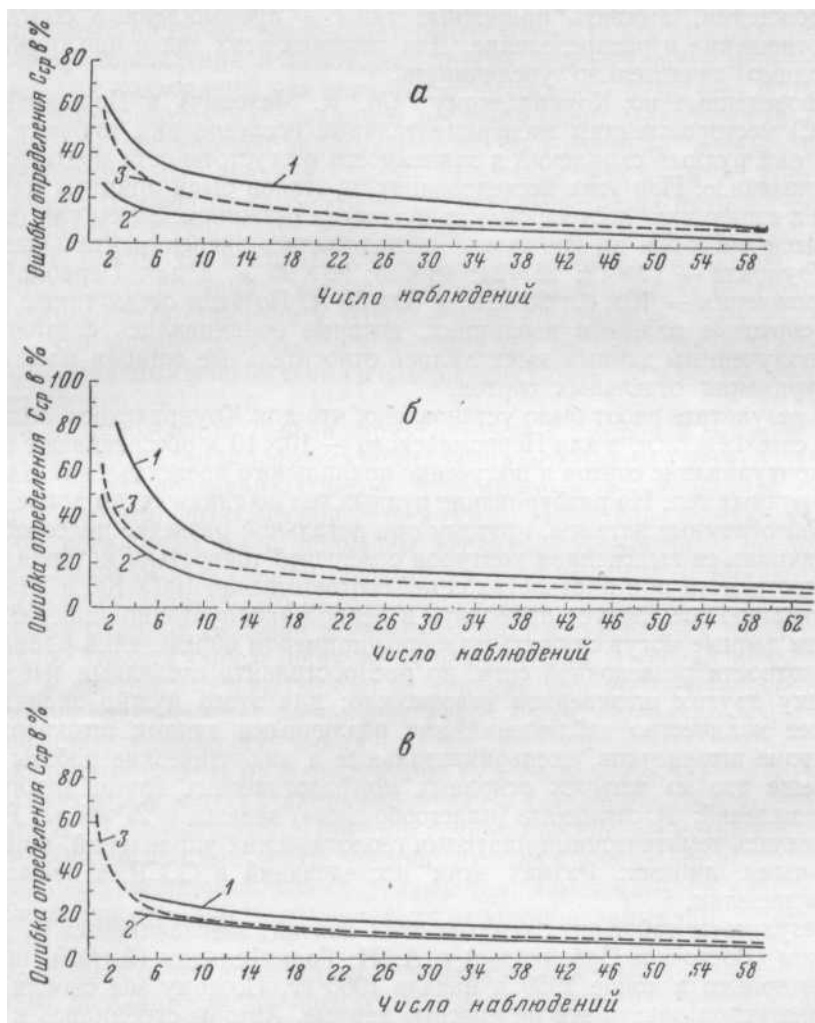
Рис. 49. Кривые ошибок определения C_{ср} в зависимости от числа наблюдений а — для месторождения Коунрад; б — для горизонта 1674 м Первомайского месторождения; в — для горизонта 1664 м Первомайского месторождения 1 и 2 — кривые максимальных и средних значений ошибок, полученных экспериментальным путем; 3 — кривые ошибок, вычисленные по формуле n = \frac{1}{\sigma^2}
