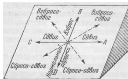
Рис. 58. Классификация дизъюнктивов (по И. А. Молчанову)
