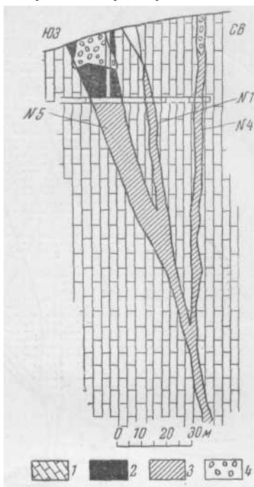
Рис. 89. Разрез месторождения Курусай (по Ф. И. Вольфсону)
