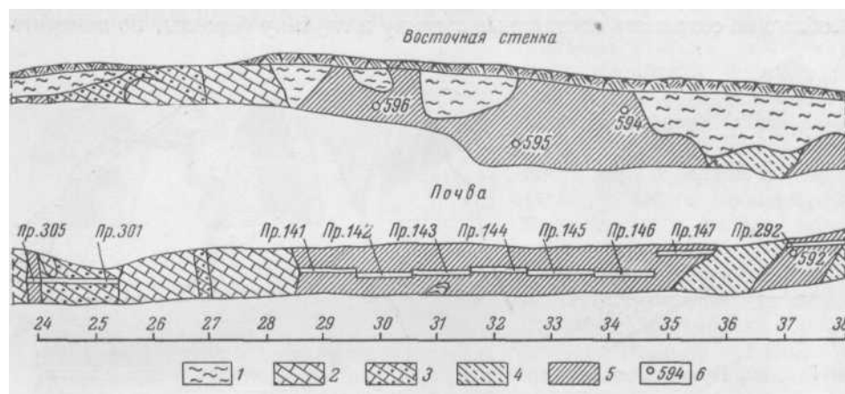
Рис. 101. Зарисовка части канавы на Курганском полиметаллическом месторождении / — дельвий; 2 — известняки; 3 — оруденные известняки; 4 — сланцы; 5 — окисленные руды; 6 — места взятия образцов
