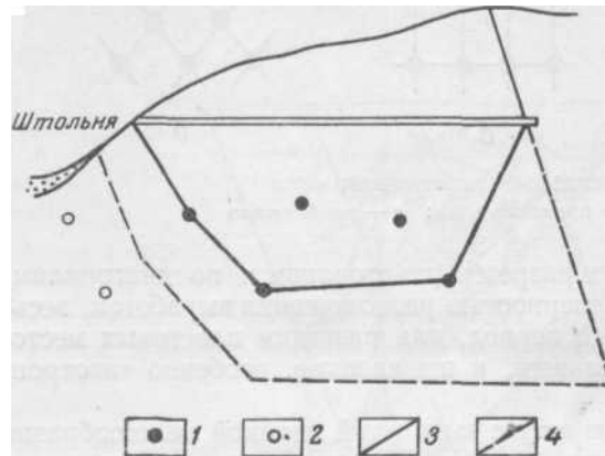
Рис. 19. Оконтуривание крутопадающего тела полезного ископаемого в проекции на вертикальную плоскость
