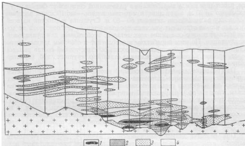
Рис. 74. Обогащенные прослойки россыпи Содержание металла (в г/м 2 ): 1—более 1; 2—от 1 до 0,2; 3 — от 0,2 до 0,03; 4—меньше 0,03
