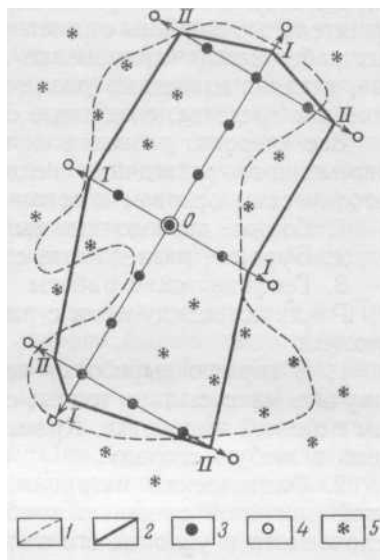
Рис. 26. Векторный способ оконтуривания тел полезных ископаемых (по Д. А. Зенкову, с видоизменениями) I — векторы первой очереди; II — векторы второй очереди / — истинный контур тела; 2 — контур, проведенный по данным векторных ходов; 1 — продуктивные разведочные выработки; 4 — пустые разведочные выработки; 5 — пункты будущей сети детальной разведки месторождения
