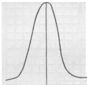
Рис. 4. Кривая нормального распределения
