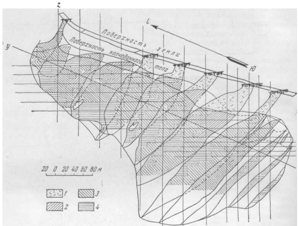
Рис. 126. Схема к подсчету запасов по месторождению медистого колчедана / — железная шляпа. Содержание меди (в %): 2 — больше 2,5; 3 — меньше 2,5; 4 — меньше 1,0
