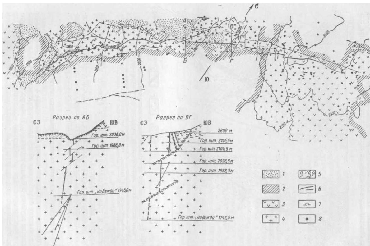
Рис. 85. Схематический план и разрезы участка Згидского свинцово-цинкового месторождения (по материалам ГРП) / — аллювиально-делювиальные и моренные отложения; 2 — сланцы; 3 — покровные кератофиры и туффиты; 4 — граниты; 5 — тектонические нарушения (а — прослеженные, б — предполагаемые); * — рудные жилы; 7 — устья штолен; 8 — буровые скважины
