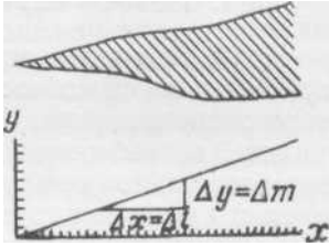
Рис. 13. Математическое выражение закономерной изменчивости формы
