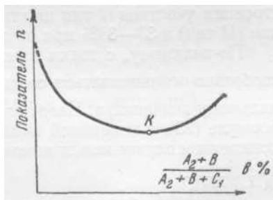
Рис. 55. Соотношение метража разведочных выработок, затраченного на разведку 1000 m запасов полезного ископаемого по высоким категориям (показатель n ), и степени разведанности участка
