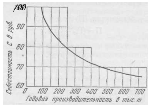
Рис. 131. Зависимость себестоимости добычи и переработки руды от годовой производительности рудника (по В. В. Померанцеву)
