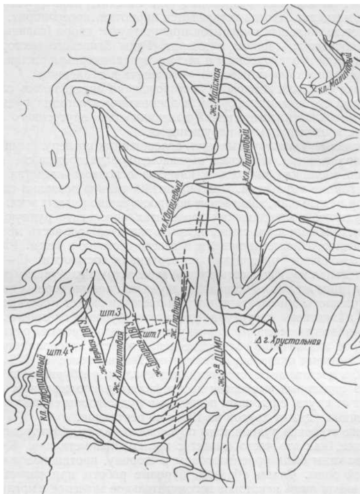
Рис. 86. План Хрустального месторождения (по В. П. Полохову)
