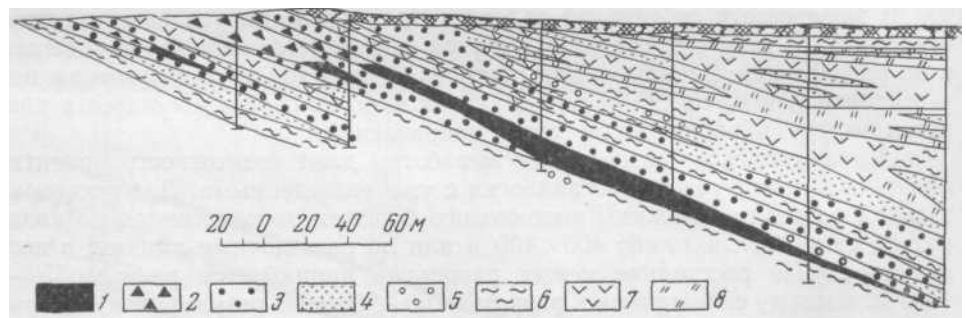
Рис. 78. Разрез одного из участков Джезказганского медного месторождения / — руда сульфидная; 2 — руда окисленная; 3 — серые песчаники с вкрапленниками медных минералов; 4 — серые песчаники безрудные; 5 — конгломераты; 6 — красные сланцы; 7 — красные песчаники; 8 — зеленовато-серые сланцы
