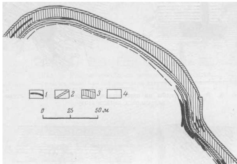
Рис. 10. Рудный столб в полости приоткрывания на крыле складки (по А. Бэлли) / — руда; 2 — сланцы; 3 — кварцит крепкий; 4 — кварцит
