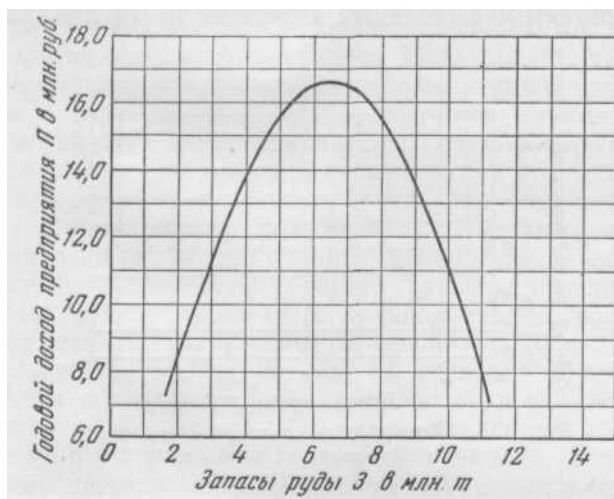
Рис. 133. Зависимость дохода от переменных запасов руды (по В. В. Померанцеву)
