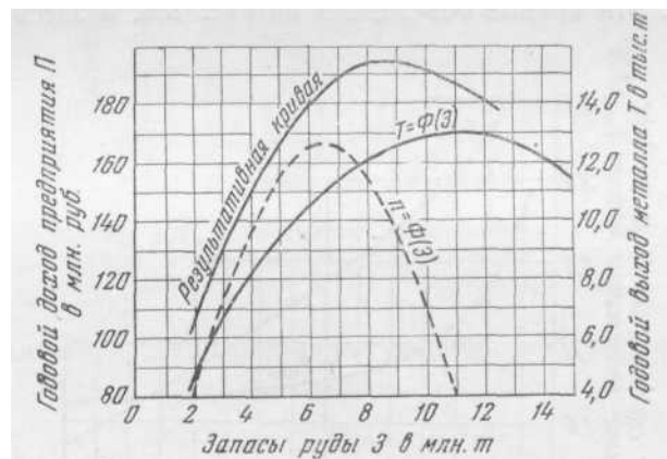
Рис. 136. Определение оптимальной величины запасов по кривым P = \Phi(Z) и T = \Phi(Z) (по В. В. Померанцеву)
