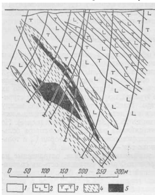
Рис. 83. Геологический разрез через месторождение, представленное серией линзообразных рудных тел (по А. Г. Белову)
