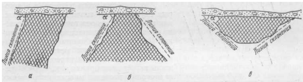
Рис. 81. Виды склонения рудных жил (проекции на вертикальную плоскость) а — параллельное; б — «трапецеидальное»; в — «треугольное».
