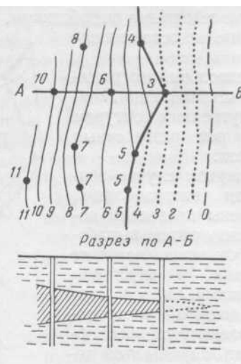
Рис. 22. Проведение внешнего контура по способу изолиний мощности (по В. И. Смирнову) Цифры около скважин показывают вскрытую мощность полезного ископаемого
