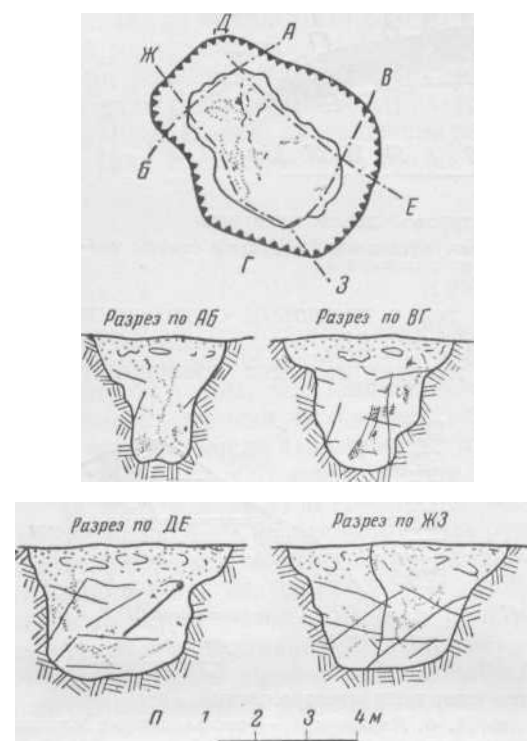
Рис. 93. Платиноносное гнездо хромита в дунитах (по А. Г. Бетехтину). Точками и прожилками показаны скопления платиноидов
