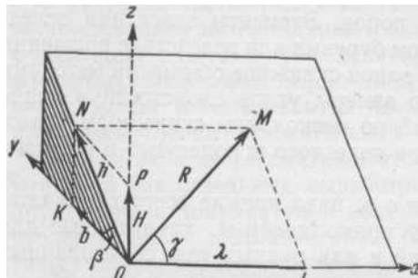
Рис. 57. Разложение вектора перемещения (по И. А. Молчанову)
