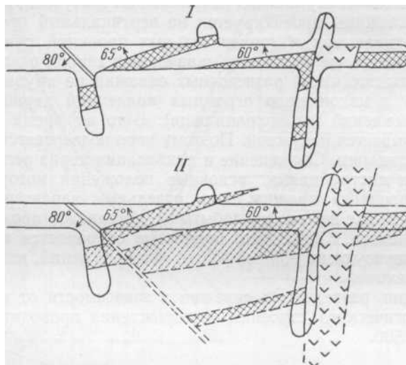
Рис. 63. Этапы составления погоризонтного плана / — нанесение данных первичной геологической документации на сводный маркшейдерский план; // — увязка данных между отдельными выработками
