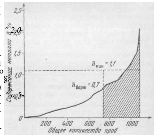
Рис. 139. График зависимости между содержанием полезного компонента в пробах и количеством проб (по А. П. Прокофьеву)
