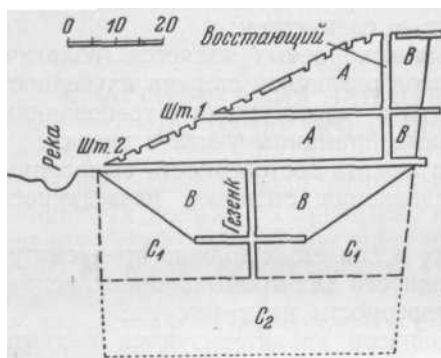
Рис. 53. Схема категоризации запасов крутопадающей рудной жилы (продольная проекция на вертикальную плоскость)
