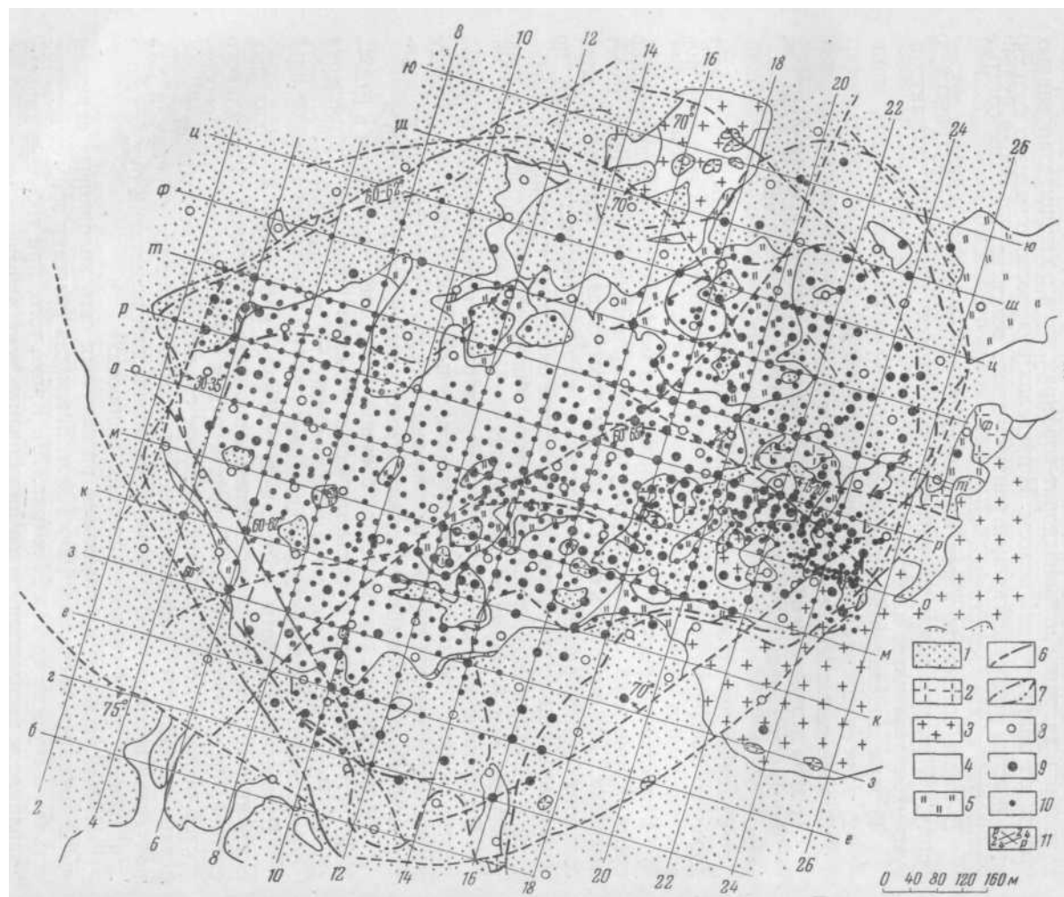
Рис. 79. План разведки отработанной части Коунрадского месторождения / — вторичные кварциты по эффузивам; 2 — неизменные гранодиорит-порфиры и кварцевые диорит-порфиры; 3 — каолинизированные гранодиорит-порфиры и кварцевые диорит-порфиры; 4 — вторичные кварциты по гранодиорит-порфирам; 5 — интенсивно каолинизированные вторичные кварциты; 6 — дизъюнктивные нарушения; 7 — контуры распространения халькозиновых и окисленных руд; 8 — скважины колонкового бурения 1929—1934 гг.; 9 — скважины бурения 1938—1939 гг., пройденные глубже горизонта 620 м; 10 — мелкие скважины, остановленные выше горизонта 620 м; 11 — линии разрезов
