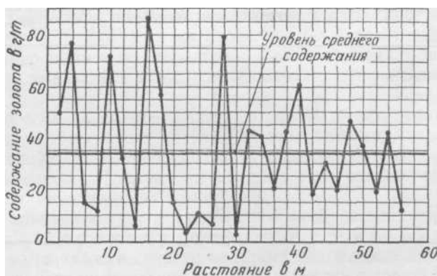
Рис. 2. Беспорядочные колебания содержаний полезного компонента (по П. Л. Каллистову)
