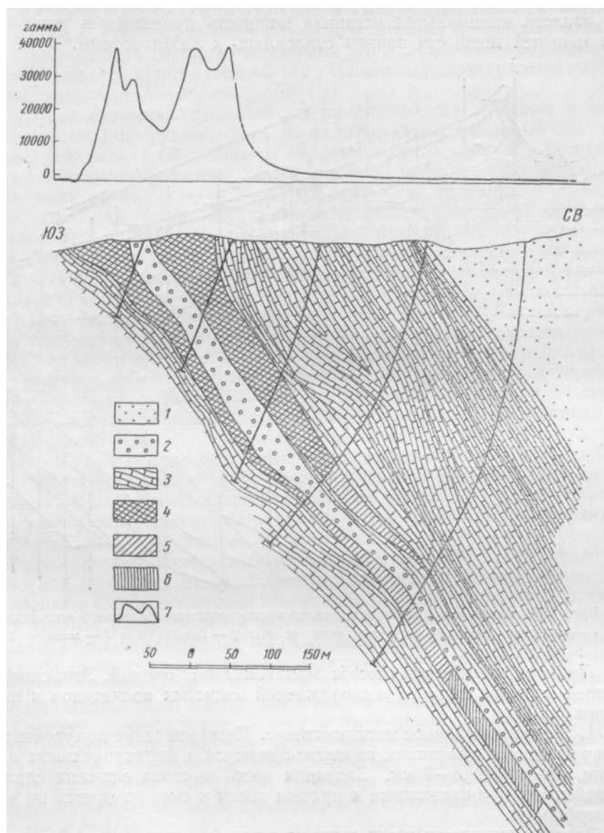
Рис. 125. Геологический разрез по линии X Белорусского месторождения 1 — ороговикованные песчаники и роговики; 2 — скалы; 3 — мраморизованные известняки с прослоями роговиков; 4 — магнетитовые руды в сечениях блоков категории В; 5 — то же категории C_1 ; 6 — то же категории C_2 ; 7 — кривая магнитометрической съемки по линии разреза
