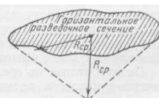
Рис. 24. Проведение внешнего контура по поверхности конуса
