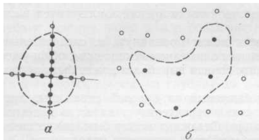
Рис. 25. Универсальные способы оконтуривания тел полезных ископаемых — а — оконтуривание «крестом»; б — оконтуривание сетью разведочных выработок
