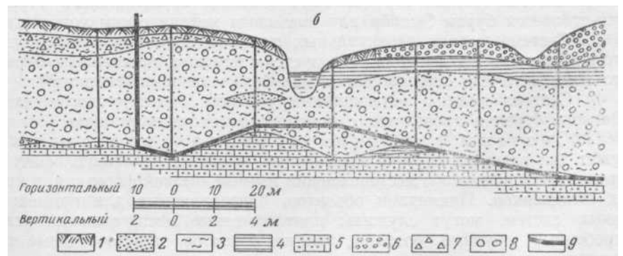
Рис. 35. Система разведки россыпи мелкими вертикальными скважинами (по В. И. Смирнову)
