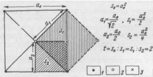
Рис. 51. Сгущение разведочной сети способом конверта / — выработки первой очереди; 2 — выработки второй очереди; 3 — выработки третьей очереди
