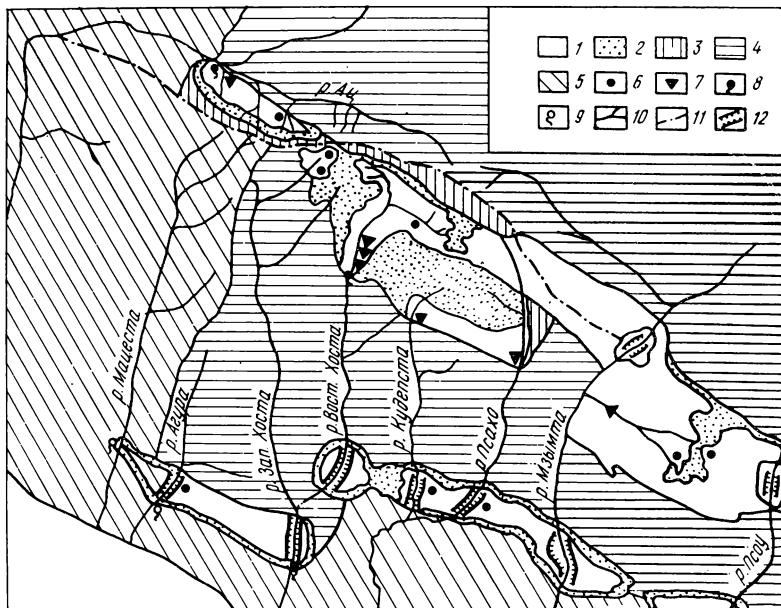
Рис.7. Карстолого-гидрогеологическая схема района Большого Сочи
