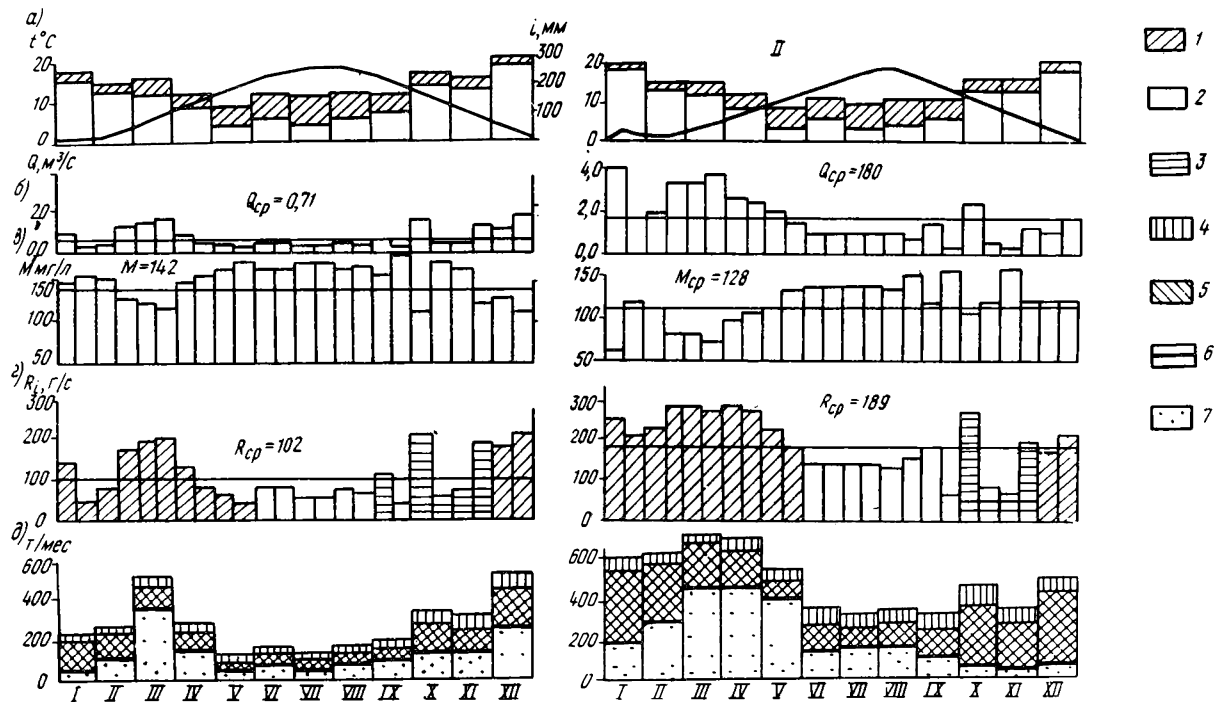
Рис.5. Годовой ход температуры воздуха, ^\circ\text{C} ; атмосферных осадков и испарения, мм (а); расхода, \text{м}^3/\text{с} (б); минерализации, \text{мг}/\text{л} (в); ионного стока, \text{г}/\text{с} (г) и \text{т}/\text{мес} (д), на массивах Алек (I) и Ахцу (II). Типы питания: 1 – снеговое; 2 – конденсационно-дождевое; 3 – дождевое. Составляющие ионного стока: 4 – атмосферные осадки; 5 – инфильтрация и инфлюация; 6 – конденсация; 7 – подземный сток
