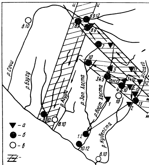
Рис.3. Схема проведения индикаторных опытов на массивах Алек и Ахчу а — место запуска индикатора; б — место выхода индикатора; в — источники, где индикатор не получен (цифры и знаки — номера опытов); 2 — направления движения подземных вод вдоль разломных зон: К — Кепшинской; М — Монастырской; Ц — Ципинской
