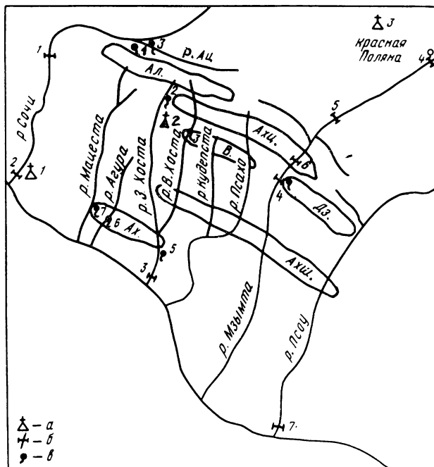
Рис.1. Схема Сочинского курортного района – ключевого опорного карстового района Северо-Западного Кавказа Карстовые массивы Ал.–Алек, Ахц.–Ахцу, В.–Воронцовский, Дз.–Дзыхра, Ахш.–Ахштырь, Ах.–Ахун; а – метеостанции и метеопосты: 1 – г.Сочи; 2 – Калиновое озеро; 3 – Ачишхо; б – гидрологические посты: 1 – р.Сочи (Пластунка); 2 – р.Сочи (Город); 3 – р.Хоста (Город); 4 – р.Мзымта (Красная поляна); 5 – р.Мзымта (Греческое устье); 6 – р.Мзымта (уш.Ахцу); 7 – р.Псоу (пос.Леселидзе); в – крупнейшие карстовые источники: 1 – в устье р.Ац; 2 – под Шалашом; 3 – "Котел"; 4 – Глубокий яр; 5 – Нижнехостинский; 6 – Агура (пресный и минеральный); 7 – Машеста (минеральный)
