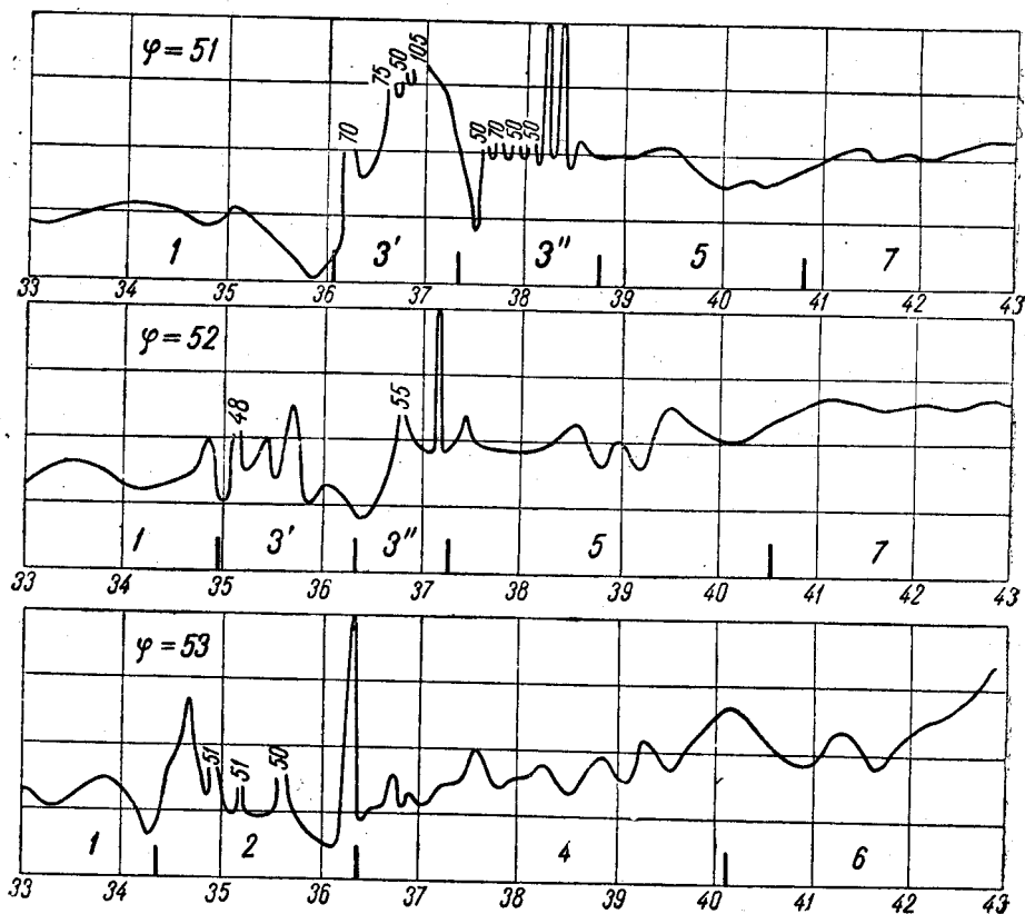
Рис. 40. Кривые изменения Z_a по широтным профилям: 4=51^\circ по 51^\circ с. ш.; \varphi=52^\circ по 52^\circ с. ш. и \varphi=53^\circ с. ш.
