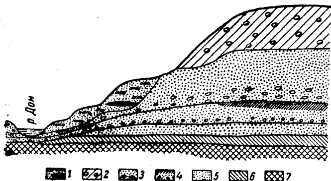
Рис. 27. Схема залегания вулканических пеплов рис-жюрмского возраста в окрестностях г. Павловска у с. Дуванка
