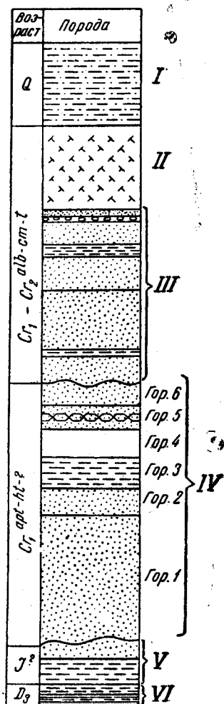
Рис. 19. Схематический разрез района Латвиевского месторождения (по литературным данным)
