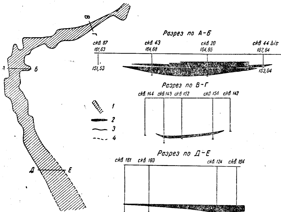
Рис. 11. Пасековские буроугольные месторождения (Воронежской обл.) 1—угольная залежь (на плане); 2—угольная залежь (на разрезах); 3—контур угольной залежи, установленный детальными разведками; 4—открытый контур угольной залежи
