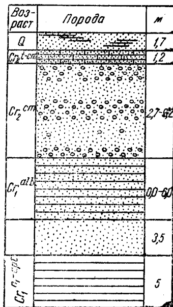
Рис. 14. Геологический разрез Полпинского месторождения фосфоритов
