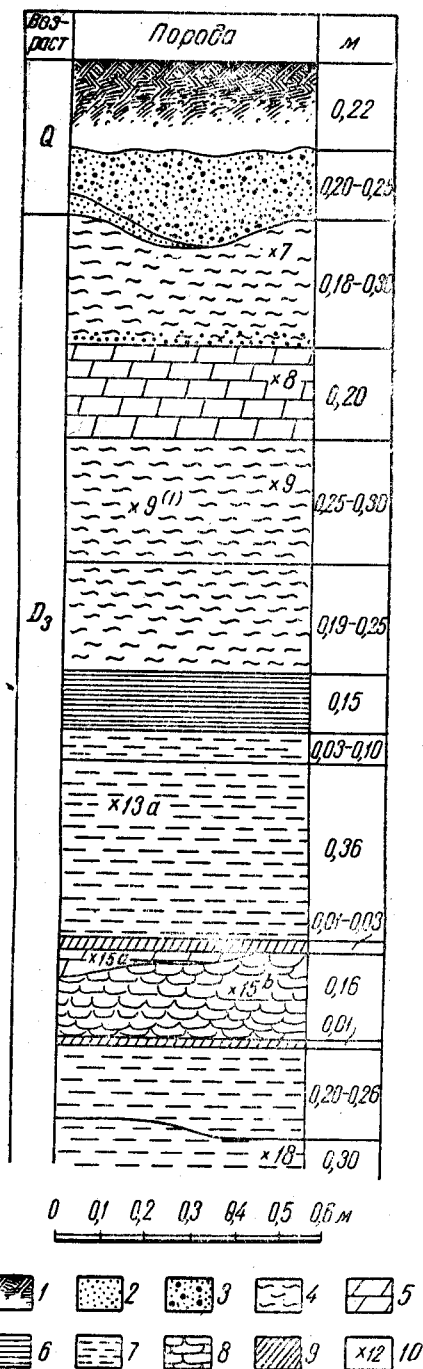
Рис. 4. Обнажение по левому берегу р. Дон у села Верхний Мамонт
