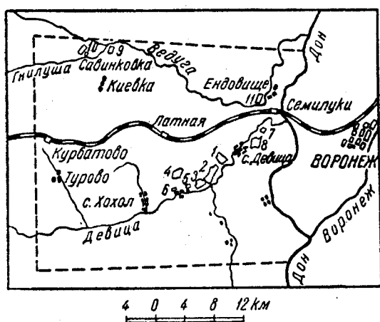
Рис. 18. Обзорная карта Латненского месторождения (по литературным данным)
