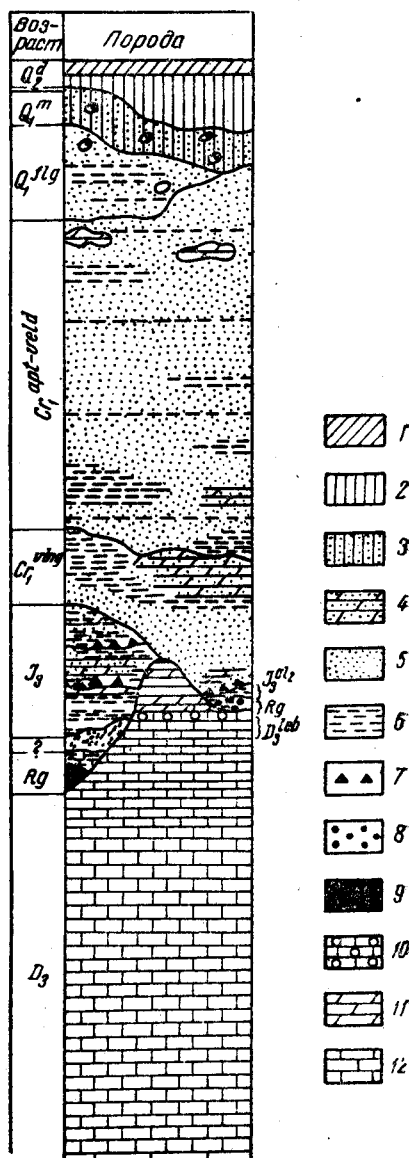
Рис. 6. Схематический сводный разрез отложений Липецкого района (по Т. Н. Давыдовой) 1—почва; 2—суглинки; 3—супеси; 4—песчаники; 5—пески; 6—глины; 7—фосфоритовые гальки; 8—вкрапленные руды; 9—сплошные руды; 10—доломитизированные известняки; 11—мергели; 12—известняки
