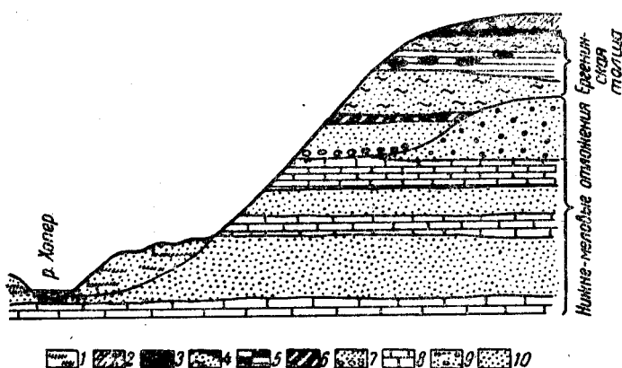
Рис. 29. Схематический разрез месторождения вулканических пеплов ергенинской толщи неогена у с. Горелки
