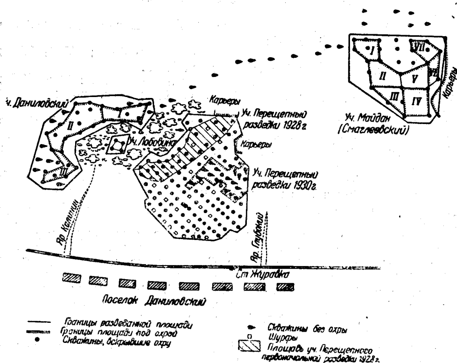
Рис. 33. Эскизный план площади, разведанной при поисках охры в Смаглеевском и Журавском районах
