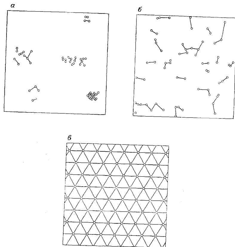
Рис. 5.14. Значения статистик метода ближайшего соседа R для различных схем расположения точек на картах (по Р. А. Ома, 1984): а — точки сгруппированы в пять групп, R=0,34 ; б — точки рассеяны случайно, R=0,91 ; в — точки размещены по шестиугольной сети, R=2,15 . Плотность точек \lambda одинакова для всех схем
