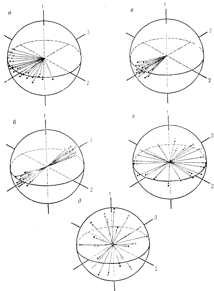
Рис. 5.31. Схемы векторов на единичной сфере:
