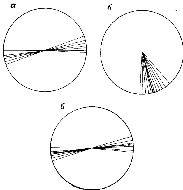
Рис. 5.23. Удвоение угла с целью вычисления средней ориентации:
