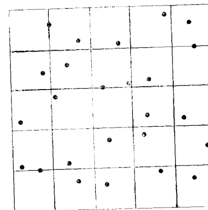
Рис. 5.9. Случайное расположение, полученное случайным выбором точки в пределах регулярной схемы ячеек.
