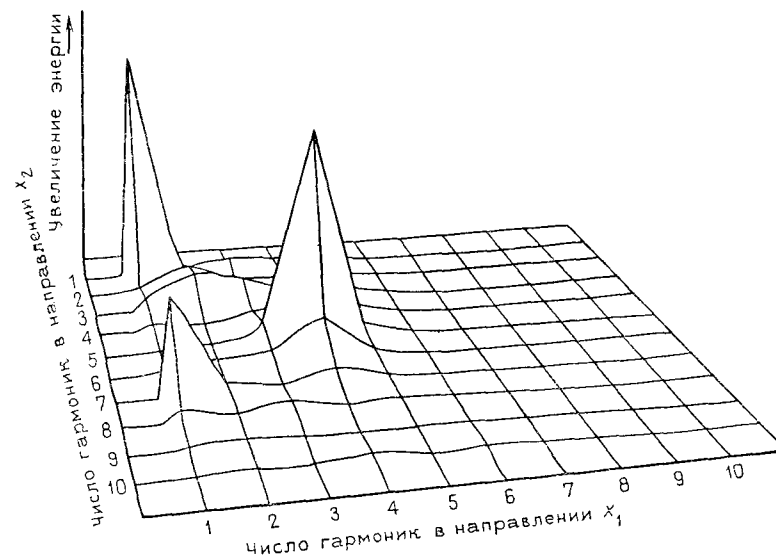
Рис. 5.94. Двумерный спектр волноприбойных знаков.
