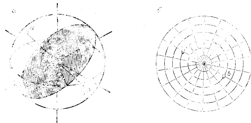
Рис. 5.34. Проектирование полюсов на плоскости: a — плоскость и ее полюсы на единичной сфере; b — полюсы плоскости, спроектированные на равноплощадную диаграмму. Точка a — проекция на верхнюю полусферу, точка b — проекция на нижнюю полусферу
