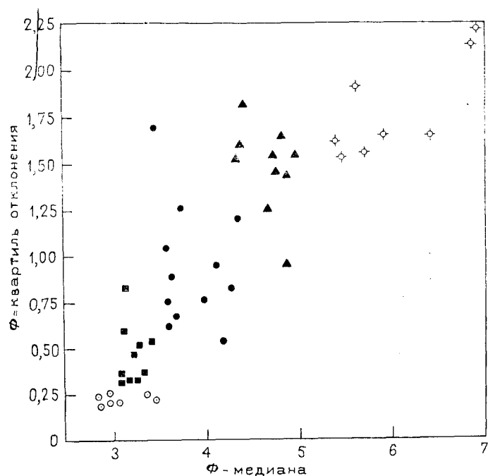
Рис. 6.31. Диаграмма зависимости кватиль от медианы в осадках залива Баратария в \phi -единицах. Символы те же, что и на рис. 6.30
