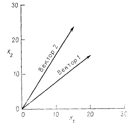
Рис. 6.19. Векторное представление дисперсий и ковариаций в виде матрицы порядка 2 \times 2 .
