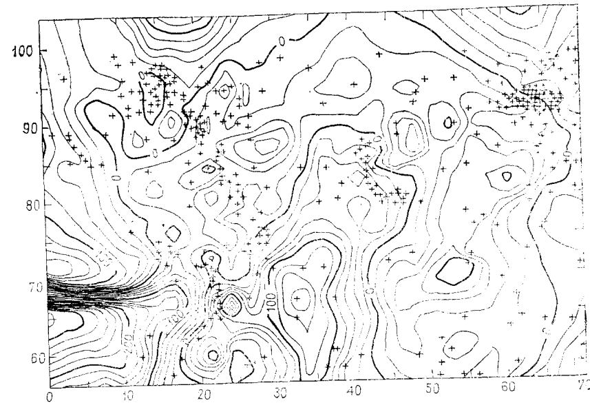
Рис. 5.79. Карта разностей значений структурной карты скал Бейзил-Фиш (см. рис. 5.78) и тренда второй степени (см. рис. 5.75).
