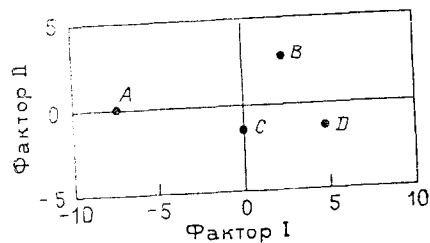
Рис. 6.14. Факторные метки R -метода для четырех видов аммоноидей
