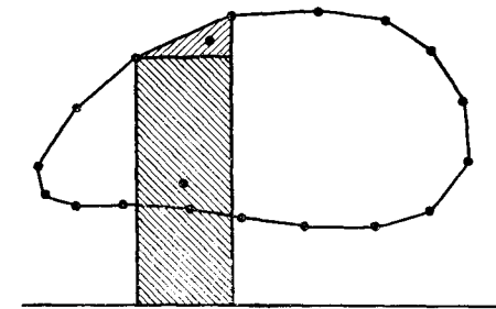
Рис. 5.36. Определение центроида трапециевидной аппроксимации.
