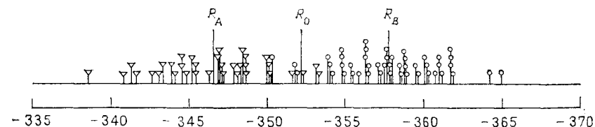
Рис. 6.4. Проекция выборок, представленных в табл. 6.5, на дискриминантную прямую, изображенную на рис. 6.3:
