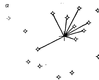
Рис. 5.57. (а) Метод поиска, локализирующий n ближайших соседей вокруг оцениваемого узла сети. На радиальное распределение контрольных точек не накладывается никаких ограничений. (б) Схема поиска по квадратам, используемая для установления истинного распределения контрольных точек вокруг оцениваемых узлов сети. (в) Октантный вариант схемы поиска вокруг оцениваемых узлов сети
