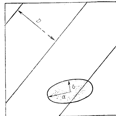
рис. 5.1. Поиск эллиптического объекта с помощью параллельных линий: a — большая полуось; b — малая полуось; D — расстояние между линиями
