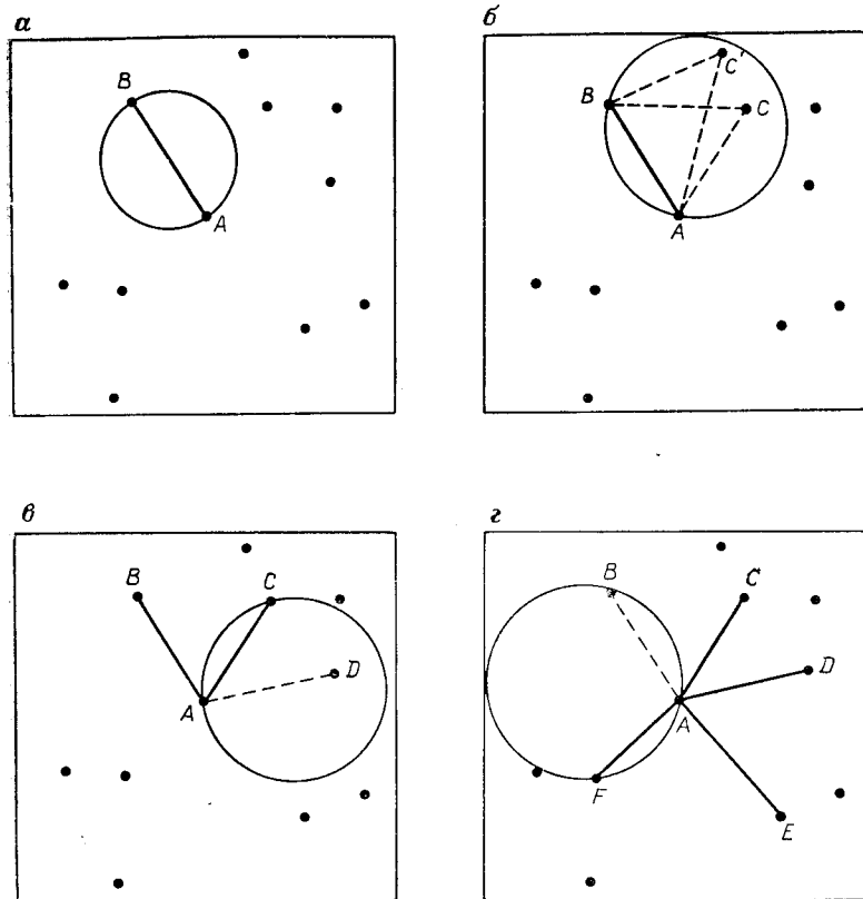
Рис. 5.47. Определение Тиссеновских соседей точки A:
