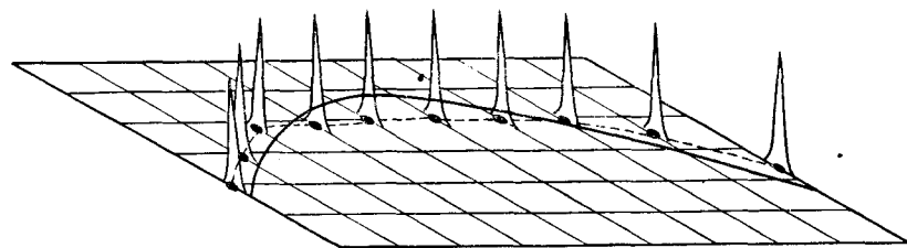
Рис. 5.85. Распределение случайной компоненты относительно наблюдаемой поверхности, соответствующей структурной модели поверхности тренда. Отклонения в повторениях точек концентрируются около средних значений, а не около линии, определенной полиномиальной моделью
