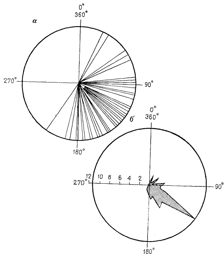
Рис. 5.19. Направления штриховки ледника, изображенные на рис. 5.18: а — направления, представленные как единичные векторы; б — направления, представленные как роза-диаграмма, на которой указаны числа векторов внутри последовательных 10-градусных интервалов
