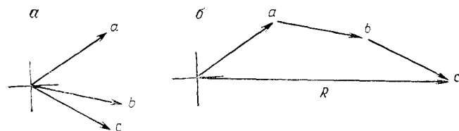
Рис. 5.20. Определение среднего направления множества единичных векторов: а — три вектора, взятые с рис. 5.18; б — вектор R , полученный комбинацией трех единичных векторов. Порядок комбинации несуществен
