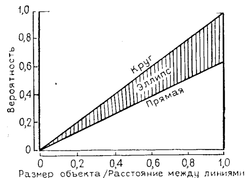
Рис. 5.3. Вероятность обнаружения объекта с помощью схемы поиска параллельными линиями.
