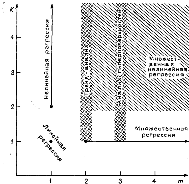
Рис. 5.89. Соотношение между нелинейной регрессией, анализом поверхностей тренда, четырехмерными поверхностями тренда и множественной регрессией: k — степень уравнения регрессии; m — число независимых переменных (размерность пространства)
