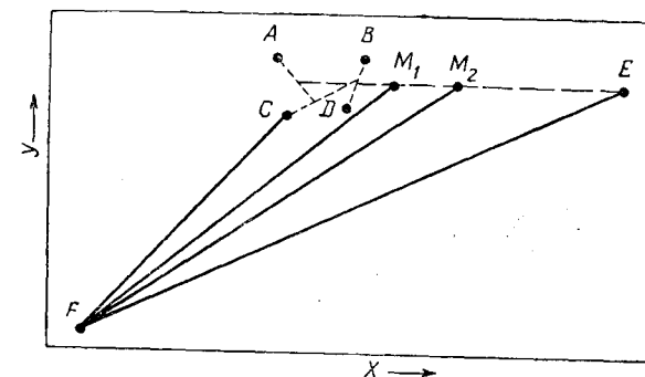
Рис. 6.12. Диаграмма, которая показывает, как объекты, характеризуемые двумя переменными X и Y , входят в группу.
