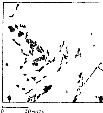
Рис. 5.82. Расположение основных нефтегазовых полей в центральном Кавказе
