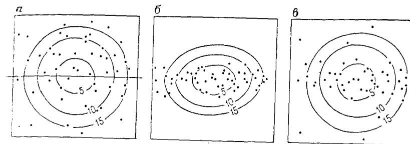
Рис. 5.86. Влияние распределения контрольных точек на поверхность тренда: а — исходная поверхность со случайным расположением контрольных точек; б — возмущенный тренд, полученный путем опробования исходной изучаемой поверхности в узкой полоске; в — почти правильный тренд, полученный путем добавления нескольких дополнительных точек за пределами узкой полосы наблюдений
