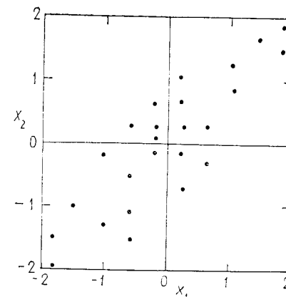
Рис. 6.34. Данные рис. 6.33 после стандартизации.
