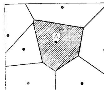
Рис. 5.45. Многоугольник Тиссена (заштрихован) вокруг точки A.
