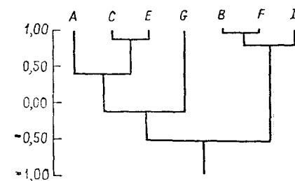
Рис. 6.11. Дендрограмма корреляционной матрицы, приведенной в табл. 6.15. Группы построены на основании невзвешенного усреднения. Кофенетический коэффициент корреляции равен 0,72
