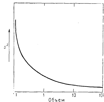
Рис. 5.61. Теоретическое изменение дисперсии содержаний полезного компонента в зависимости от измененного объема пробы или разрабатываемого блока
