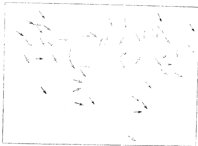
Рис. 5.18. Карта, представляющая направления штриховки ледника в южной части Финляндии (51 измерение) на площади 35 км 2
