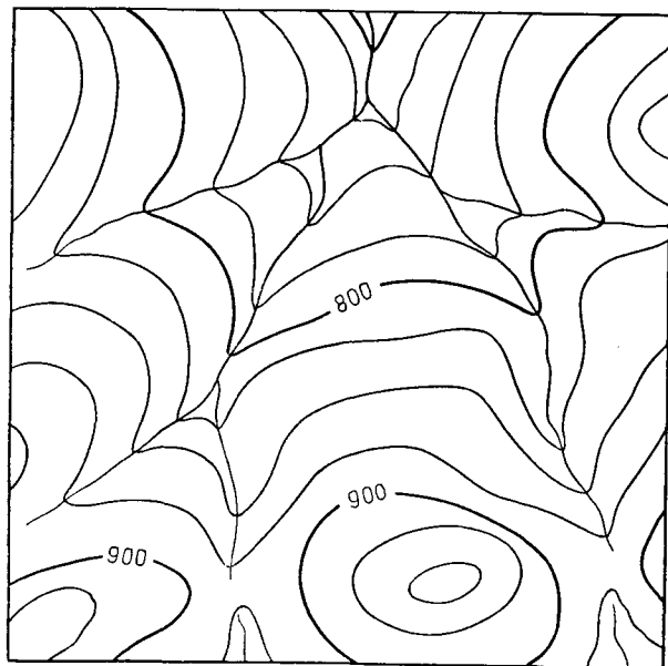
Рис. 5.59. Карта в изолиниях, построенная по топографическим данным вручную. Огметим увеличение влияния русел на форму изолиний
