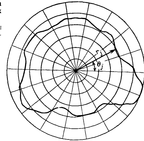
Рис. 5.35. Проекция контура зерна песка, выраженная в полярных координатах.
