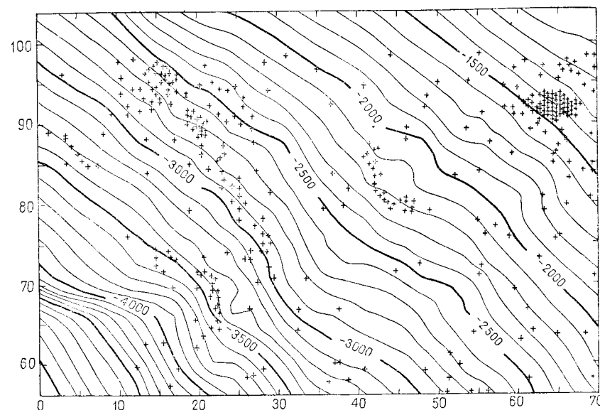
Рис. 5.76. Структурная карта вершины скал Бейзил-Фиш, бассейн Альберта. Изолинии указаны в футах ниже уровня моря. Крестики — контрольные скважины
