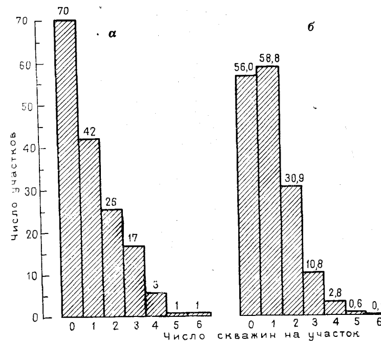
Рис. 5.12. Гистограммы, показывающие наблюдаемые числа скважин на участок на площади пермского бассейна (а) и ожидаемые числа, если поля распределены случайно в соответствии с пуассоновской моделью (б)
