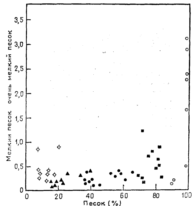
Рис. 6.32. Диаграмма зависимости содержания песка от отношения содержания тонкозернистого песка к очень тонкозернистому в осадках залива Баратария.
