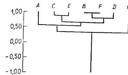
Рис. 6.10. Дендрограмма корреляционной матрицы, приведенной в табл. 6.15. Группы построены по методу прямой связи. Кофенетический коэффициент корреляции равен 0,71
