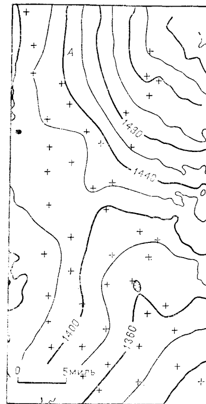
Рис. 5.67. Карта уровней воды в Экус Бедз, большом водонесном слое в южной части Центрального Канзаса.
