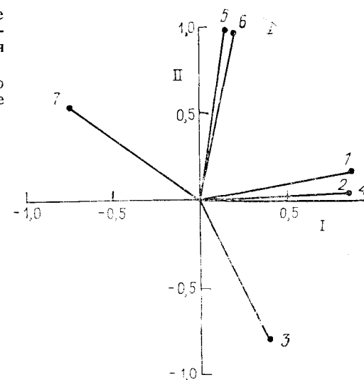
Рис. 6.37. Графическое представление тех же нагрузок после вращения по методу варимакс.
