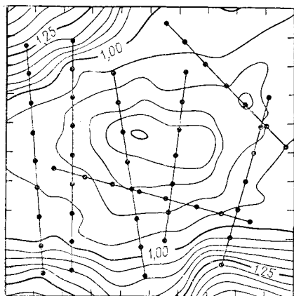
Рис. 5.99. Структурная конфигурация отражающей поверхности, определенная с помощью времени возвращения сейсмических сигналов.
