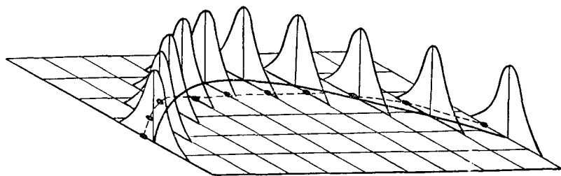
Рис. 5.84. Распределение случайной компоненты относительно линии регрессии в полиномиальной модели.
