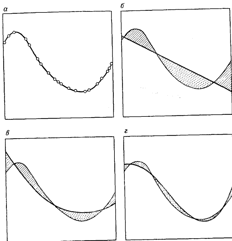
Рис. 5.72. Двумерная иллюстрация понятия тренда:
