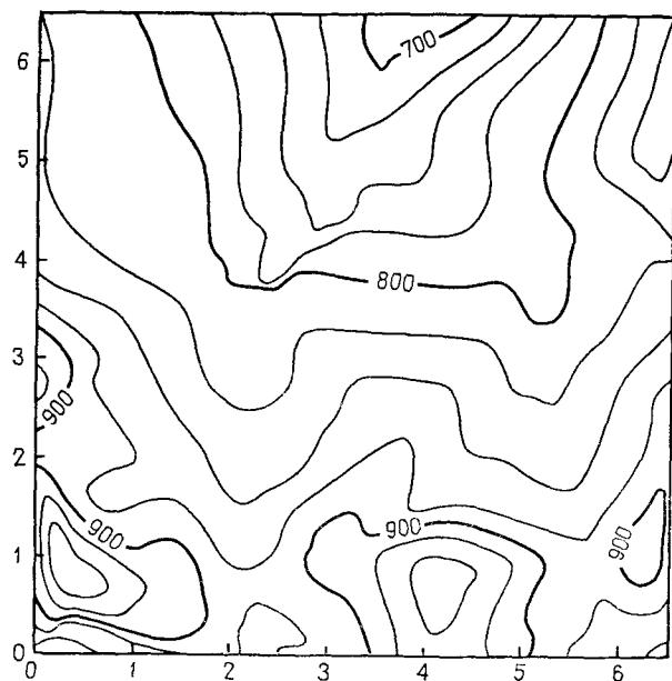
Рис. 5.51. Топографическая карта в изолиниях, полученная по программе, в которой в качестве математической модели поверхности использована треугольная сеть. Интервал между изолиниями — 25 футов (0,3 м)
