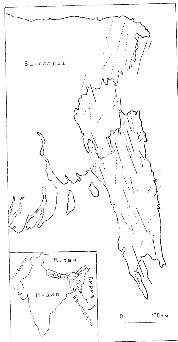
Рис. 5.25. Карта Восточного Бангладеш, на которой указаны осевые плоскости больших антиклиналей (жирные линии) и обширные линеаменты, полученные со спутников (пунктир).
