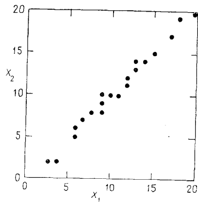
Рис. 6.23. Данные табл. 6.19 ранжированы и нанесены на график
