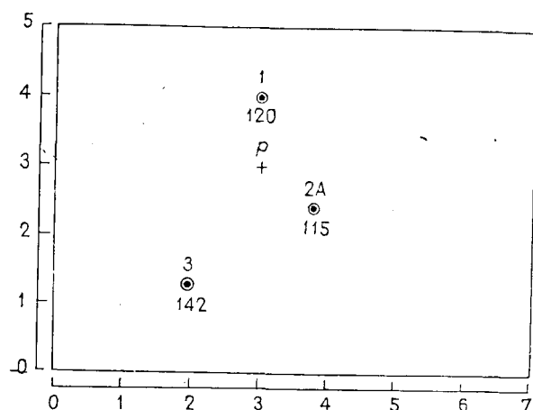
Рис. 5.65. Карта, показывающая уровни воды (в м) в трех наблюдательных скважинах. Скважина 2А ближе к оцениваемой точке p , чем скважина 2 на рис. 5.63
