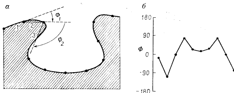
Рис. 5.42. Преобразование цифровых координат в угловые отклонения:
