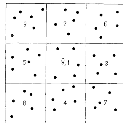
Рис. 5.62. Схема скользящего среднего для оценки содержаний полезного компонента в центре блока \hat{Y} по средним для буровых скважин в блоках 1—9
