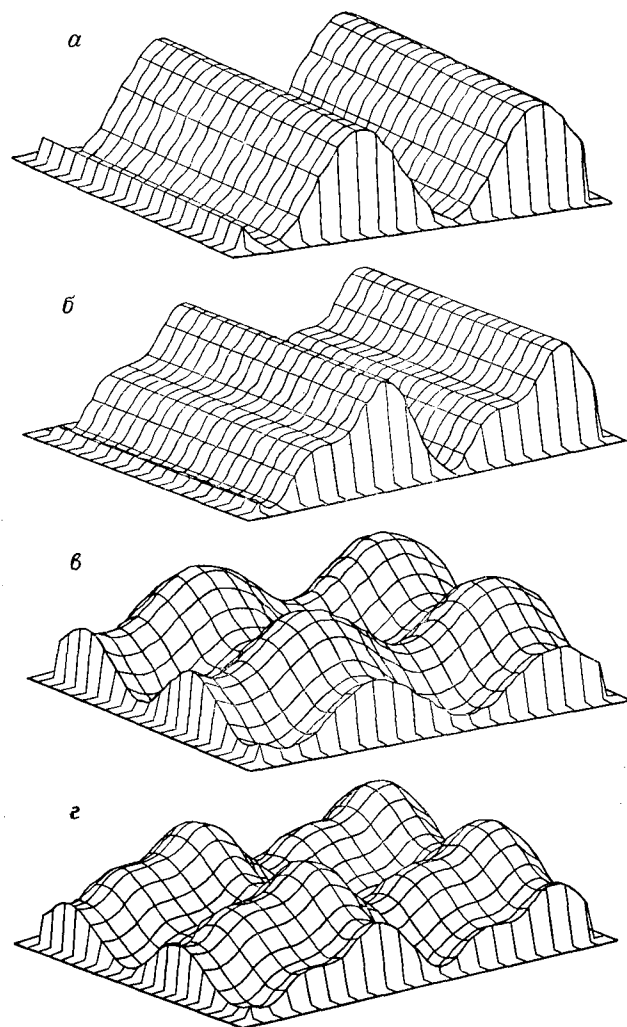
Рис. 5.91. Двумерные синусоидальные волны:
