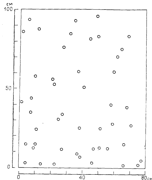
Рис. 5.15. Схематическое представление полированной плиты анортозита, на которой показано расположение кристаллов магнетита
