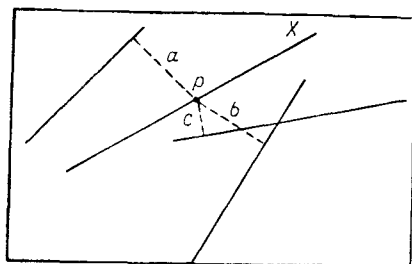
Рис. 5.16. Вычисление расстояний между линиями по методу ближайшего соседа.
