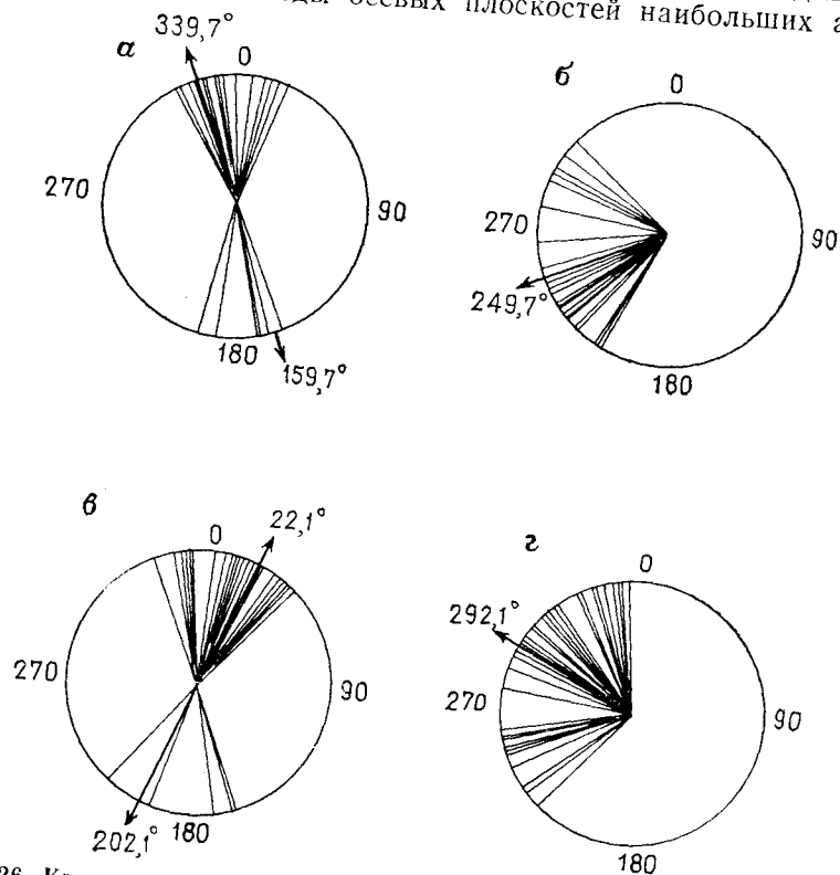
Рис. 5.26. Круговое представление ориентации по данным Восточного Бангладеш. Указана средняя ориентация.
