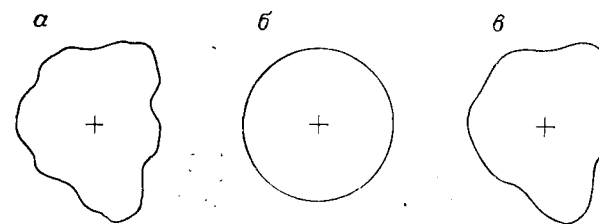
Рис. 5.39. Сравнение оцифрованного контура песчинки (а) с нулевой гармоникой или окружностью среднего радиуса (б) и с контуром, построенным по шести гармоникам (в)
