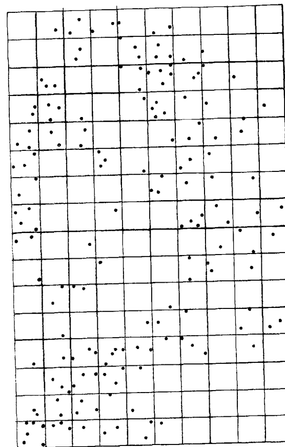
Рис. 5.11. Расположение нефтяных поисковых скважин в восточной части шельфа пермского бассейна, графства Фишер и Ноланд, Техас
