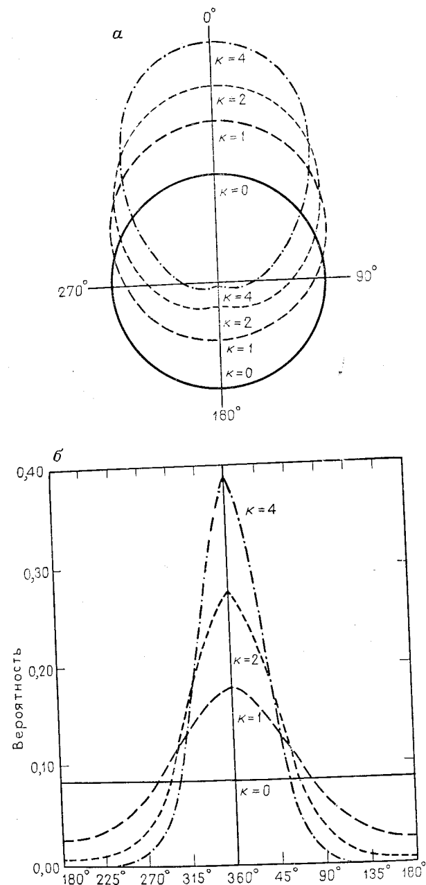
Рис. 5.24. Распределения фон Мизеса, имеющие различные параметры концентрации [33]:
