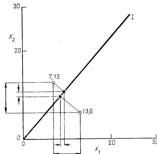
Рис. 6.21. Проекция точечных данных табл. 6.19 на главные компоненты. Дисперсия по компоненте I равна 37,9, а дисперсия по компоненте II — 6,5
