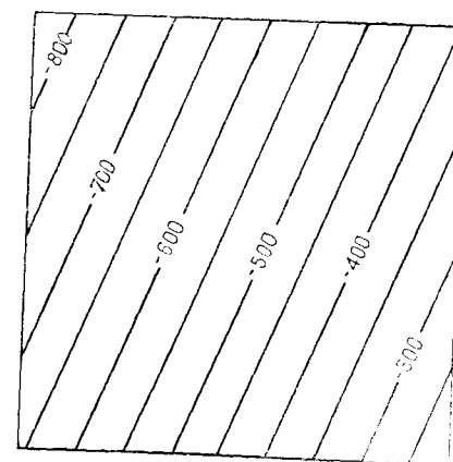
Рис. 5.74 Карта поверхности тренда по скважинам рис. 5.73. Интервал между изолиниями равен 50 м
