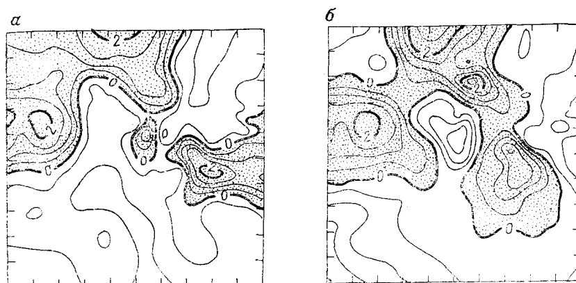
Рис. 5.103. Изменчивость стандартизованных параметров размера частиц донных осадков, собранных на побережье Северной Каролины (карты исходных параметров представлены на рис. 5.97):
