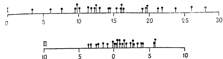
Рис. 6.21. Проекция точечных данных табл. 6.19 на главные компоненты. Дисперсия по компоненте I равна 37,9, а дисперсия по компоненте II — 6,5
