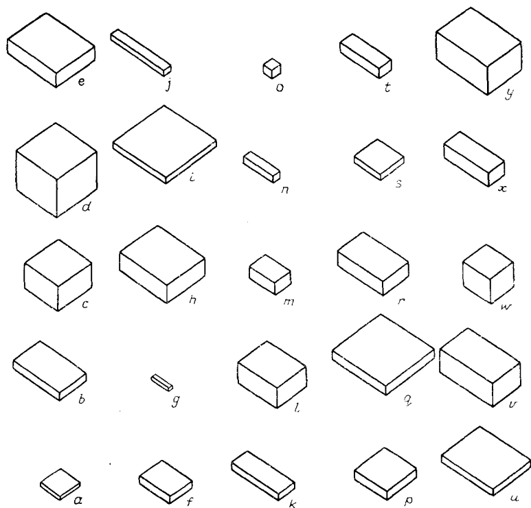
Рис. 6.16. Двадцать пять блоков со случайными значениями длины, ширины и высоты.
