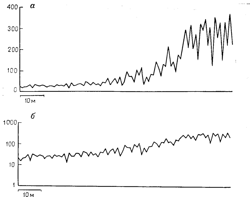
Рис. 5.60. Изменчивость содержаний серебра вдоль штольни рудника в Мексике:
