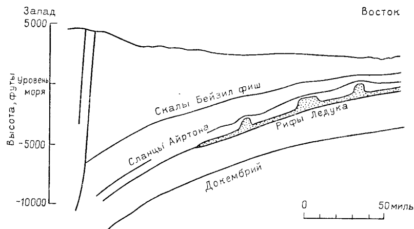
Рис. 5.75. Изображение разреза западного поля бассейна Альберта в виде диаграммы.
