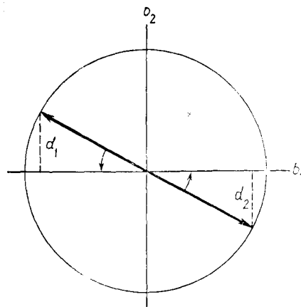
Рис. 5.30. Проекция двух диаметрально противоположных векторов на собственный вектор b_1 .
