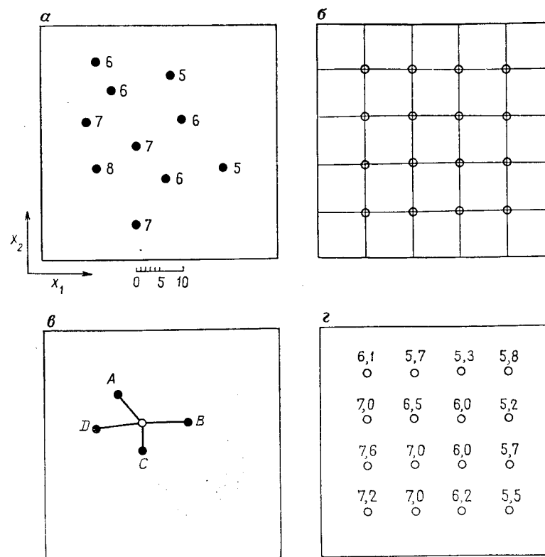
Рис. 5.53. Последовательность вычислений для построения изолиний при нахождении значений в узлах сети:
