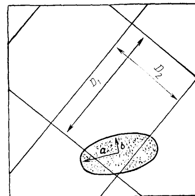
Рис. 5.2. Поиск эллиптического объекта с помощью сети, характеризуемой интервалом D_1 в одном направлении и интервалом D_2 в другом:
