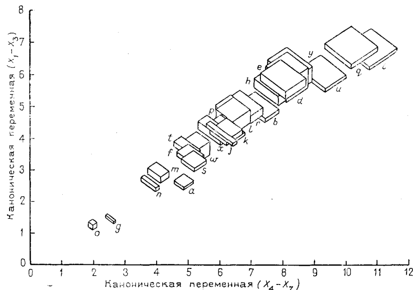
Рис. 6.52. Совместное представление первой пары канонических переменных для данных по случайным блокам.
