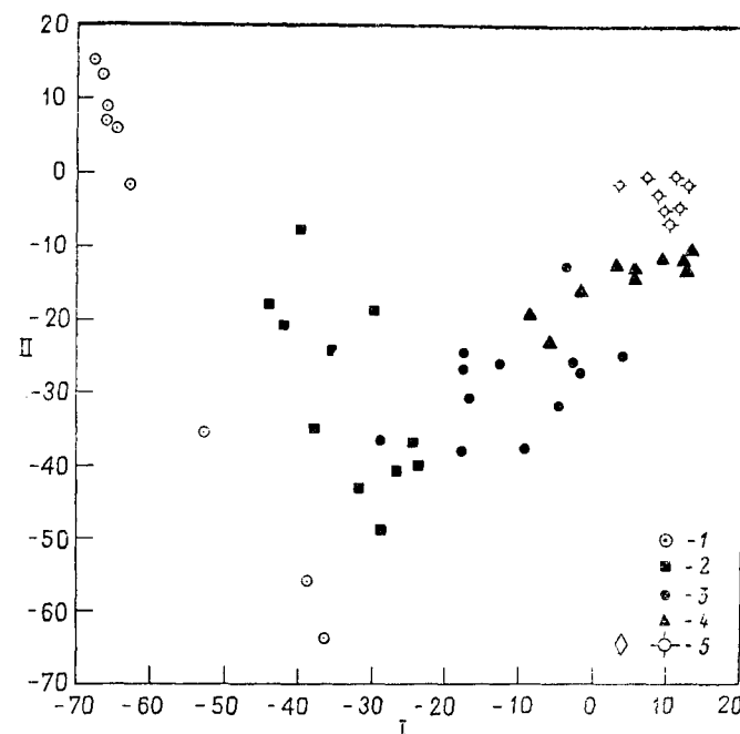
Рис. 6.30. Проекция анализов осадков залива Баратария на плоскость первых двух главных компонент. Различные символы соответствуют пяти различным типам осадочных пород [37]:
