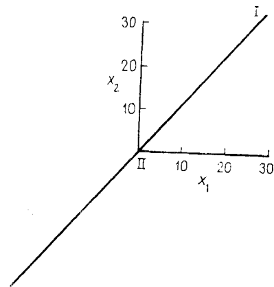
Рис. 6.24. Эллипс, определенный векторами дисперсий и ковариаций ранжированных данных рис. 6.23. Главная компонента I чрезвычайно вытянутого эллипса соответствует 99% общей дисперсии
