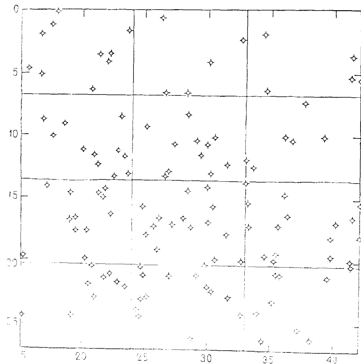
Рис. 5.10. Расположение 123 скважин, пробуренных в верхних слоях осадочных отложений в Центральном Канзасе. Карта разделена на 12 ячеек одинакового размера
