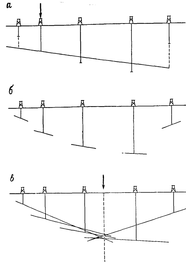
Рис. 5.55. Интерполяция для равномерно расположенных точек сети с помощью метода проектирования падения, который требует вычисления локального падения в каждой данной точке (изображено в разрезе) [69]:
