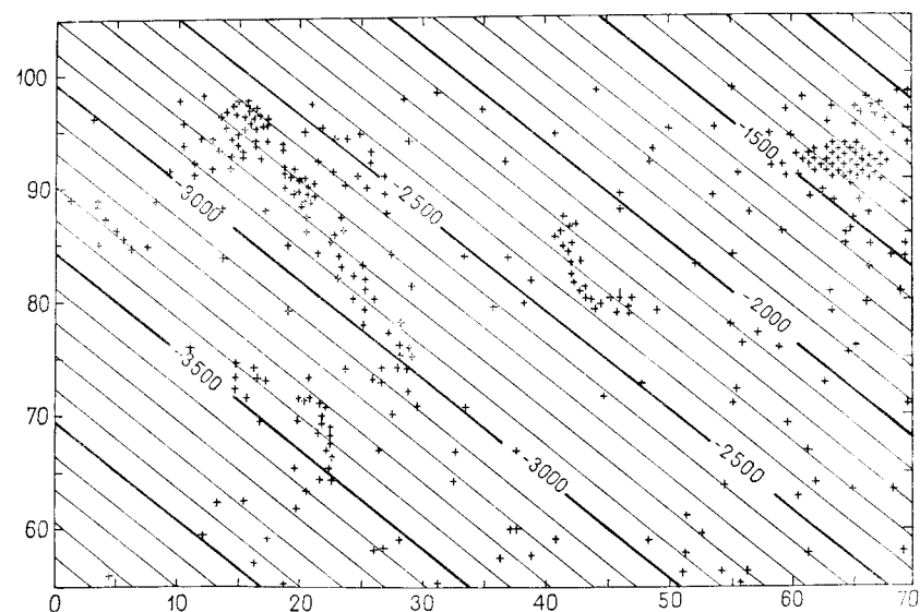
Рис. 5.77. Поверхность тренда первой степени, построенная для скал Бейзил-Фиш.
