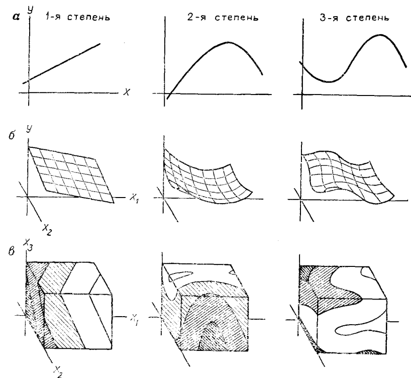
Рис. 5.90. Тренды от одной (а), двух (б) и трех (в) независимых переменных, полученные по полиномиальным уравнениям первой, второй и третьей степеней [37]
