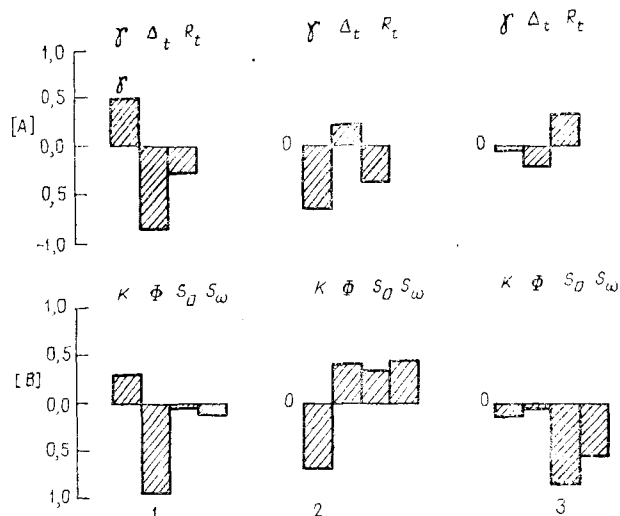
Рис. 6.54. Каноническое преобразование векторов [A] и [B], вычисленное по данным каротажа скважин и измерениям керна в скважине Северо-Западного Канзаса.
