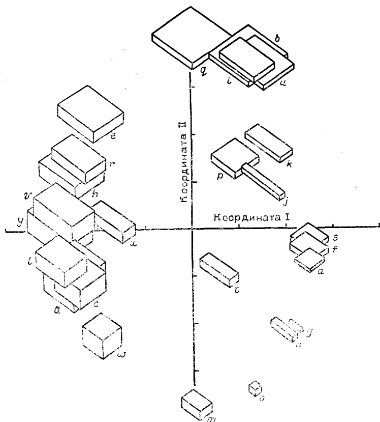
Рис. 6.43. Представление двух главных координат для данных по случайным блокам.
