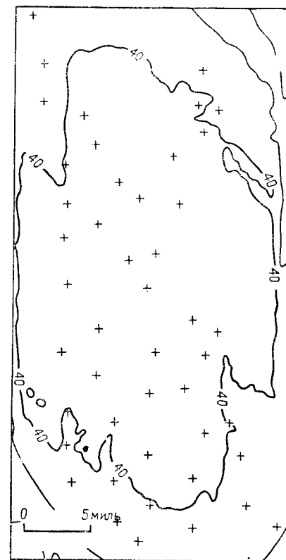
Рис. 5.70. Карта представляет стандартную ошибку дрифта первого порядка уровней воды в Экус Бедз.
