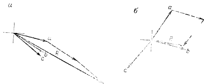
Рис. 5.21. Использование длины вектора R для выражения дисперсии некоторого набора единичных векторов:
