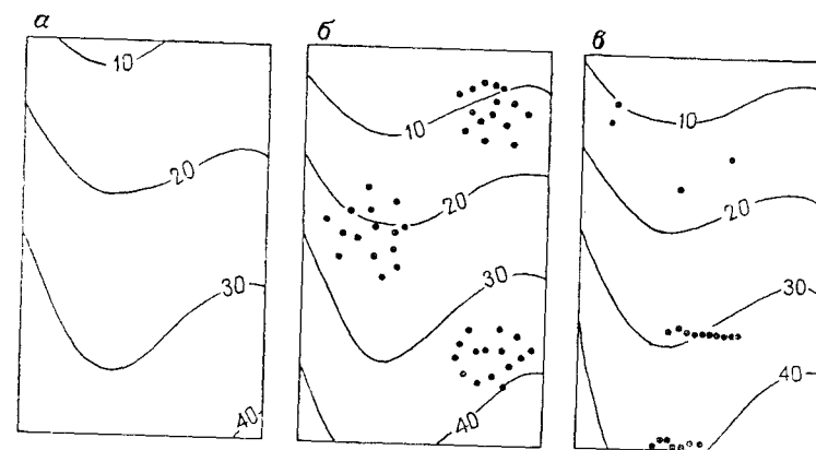
Рис. 5.87. Влияние группировки контрольных точек на поверхности тренда: а — исходная поверхность тренда третьей степени; б — поверхность тренда, полученная по контрольным точкам, расположенным группами; в — поверхность тренда, полученная по контрольным точкам, расположенным по частичным пересечениям проверяемой поверхности
