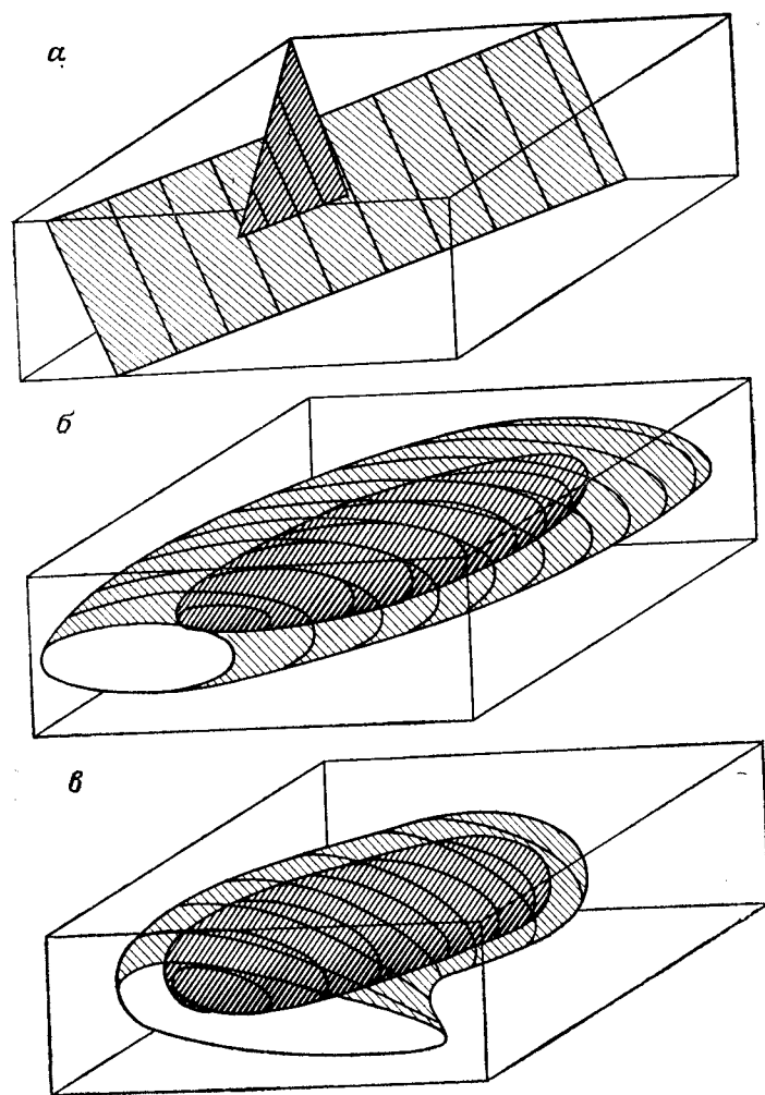
Рис. 5.88. Четырехмерные полиномиальные поверхности тренда для содержания урана.
