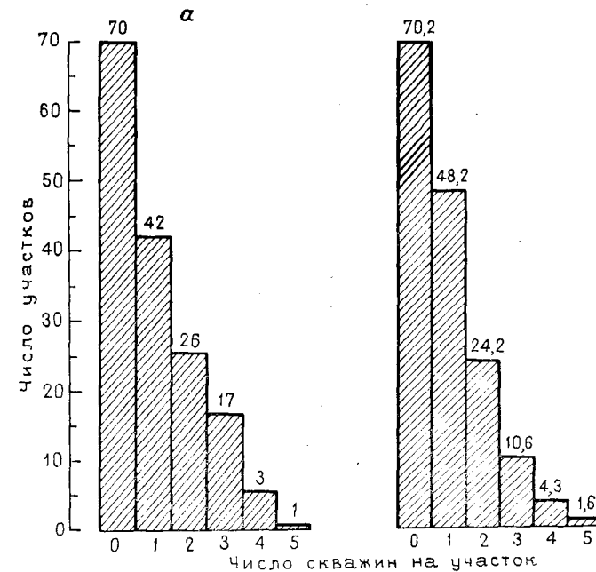
Рис. 5.13. Гистограммы, показывающие наблюдаемые числа разведочных скважин на участок на одной из площадей пермского бассейна (а) и ожидаемые числа в отрицательной биномиальной модели (б)
