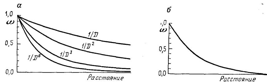
Рис. 5.56. Примеры взвешивающих функций от расстояния, используемых в программах построения карт в изолиниях:
