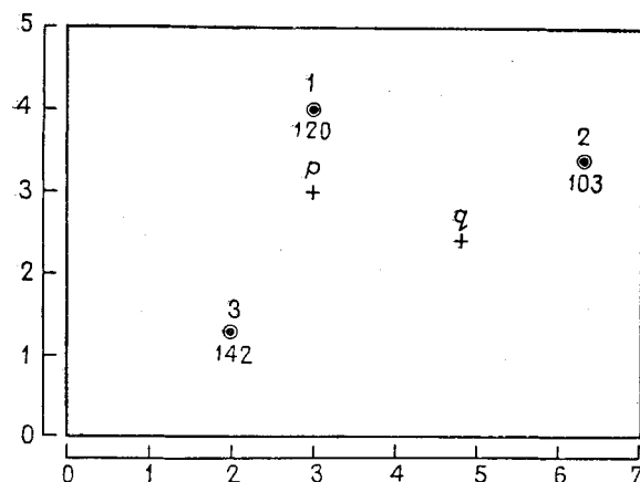
Рис. 5.63. Карта уровней воды (в м) в трех наблюдательных скважинах. Оценки уровня воды сделаны в точках p и q . Координаты указаны (в км) для произвольного начала
