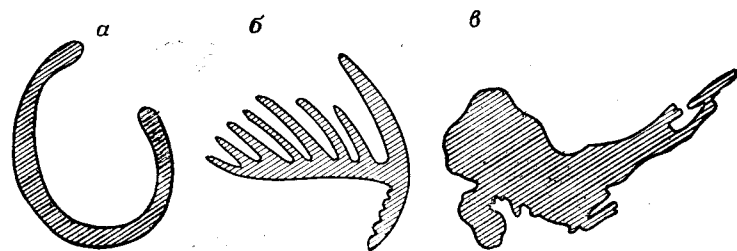
Рис. 5.41. Примеры форм, которые нельзя анализировать с помощью полярного метода Фурье из-за наличия двузначных радиусов:
