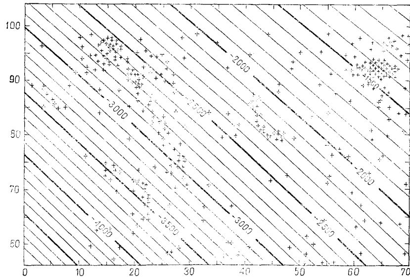
Рис. 5.78. Поверхность тренда второй степени, построенная для скал Бейзил-Фиш.
