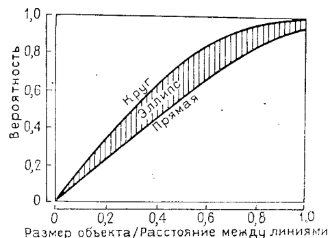
Рис. 5.4. Вероятность обнаружения объекта квадратной сетью поиска.
