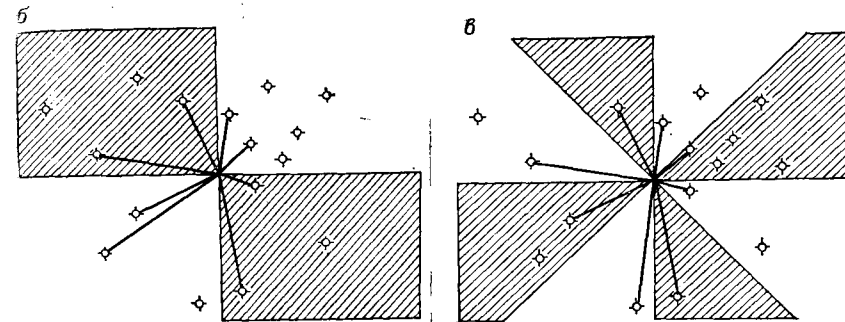
Рис. 5.57. (а) Метод поиска, локализирующий n ближайших соседей вокруг оцениваемого узла сети. На радиальное распределение контрольных точек не накладывается никаких ограничений. (б) Схема поиска по квадратам, используемая для установления истинного распределения контрольных точек вокруг оцениваемых узлов сети. (в) Октантный вариант схемы поиска вокруг оцениваемых узлов сети
