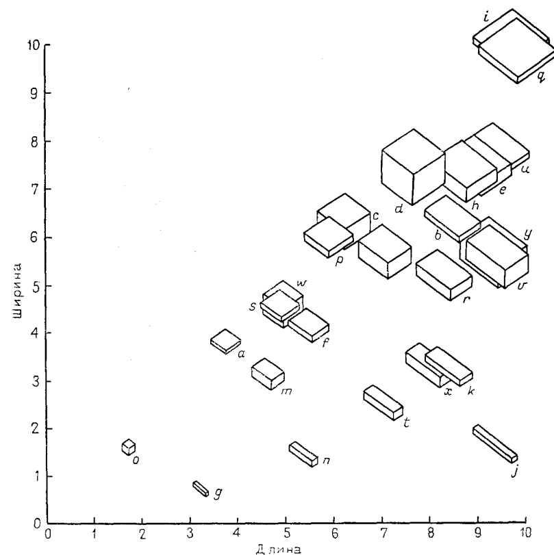
Рис. 6.17. Представление зависимости ширины случайных блоков от их длины. Так как ширина меньше длины, то все блоки расположены в нижней части диаграммы под диагональю. Такое положение соответствует корреляции r=0,58 между длиной и шириной. Длина и ширина приведены в произвольных единицах
