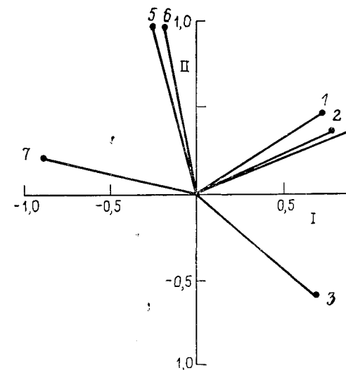
Рис. 6.36. Графическое представление нагрузок на два фактора для необработанных данных по 25 случайным блокам.
