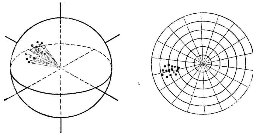
Рис. 5.33. Векторы внутри единичной сферы и их проекции на равноплощадную полярную диаграмму
