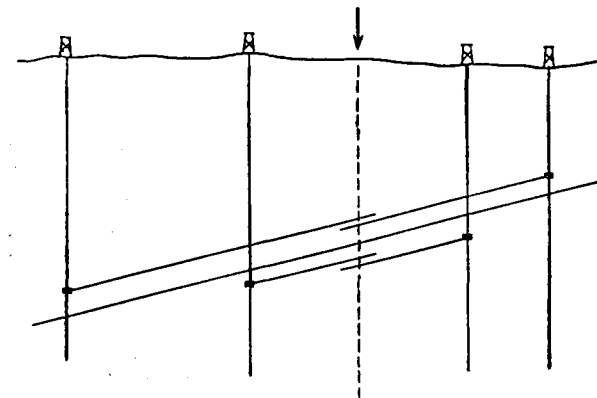
Рис. 5.54. Вид разреза, на котором представлены контрольные точки (скважины) с известными отметками поверхности (кровли формации).
