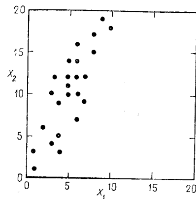
Рис. 6.33. Множество данных по стандартизации. Необработанные данные имеют средние значения \bar{X}_1=5 и \bar{X}_2=10
