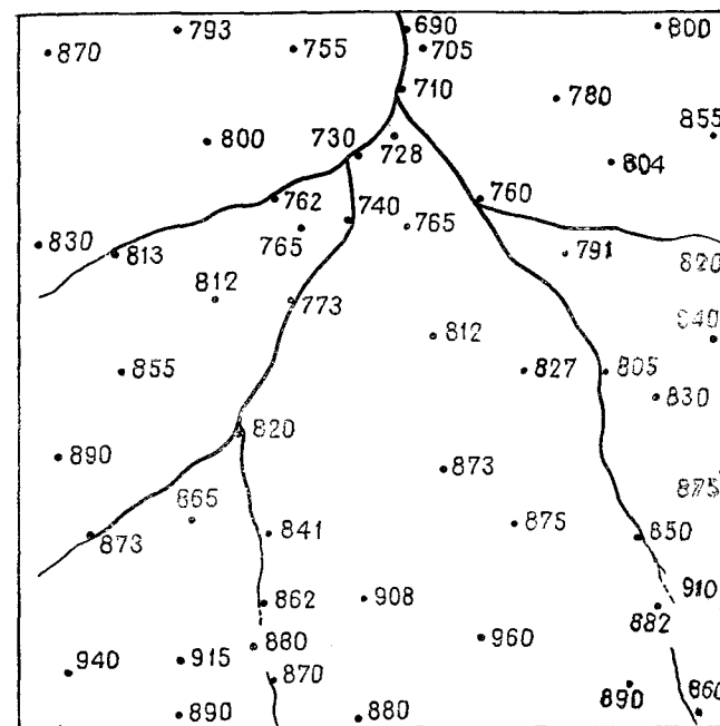
Рис. 5.49. Изображение контрольных точек для задачи топографического картирования.
