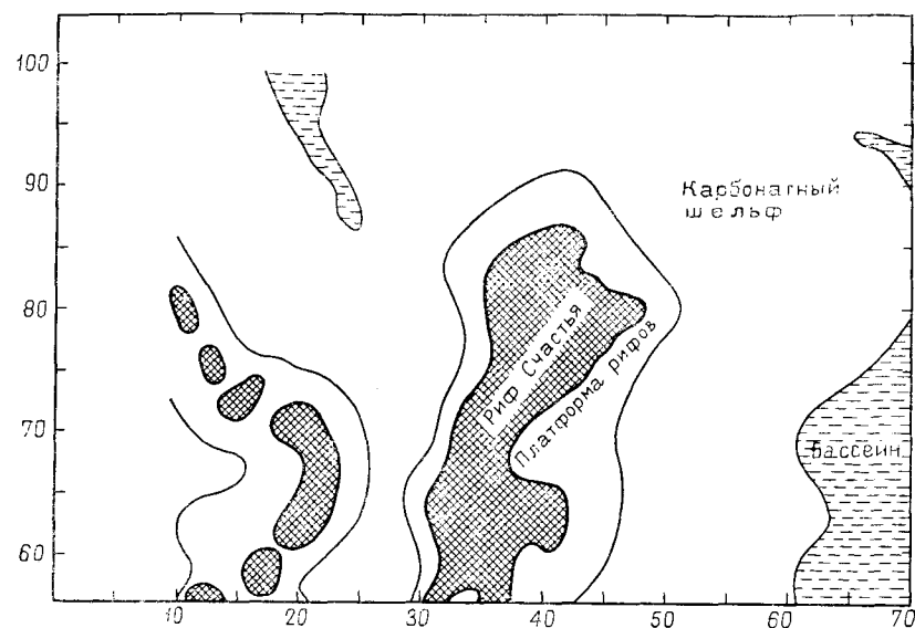
Рис. 5.80. Палеогеографическая карта верхнего девона рифов Ледука, развитых на карбонатной платформе вдоль западного побережья Девонского моря
