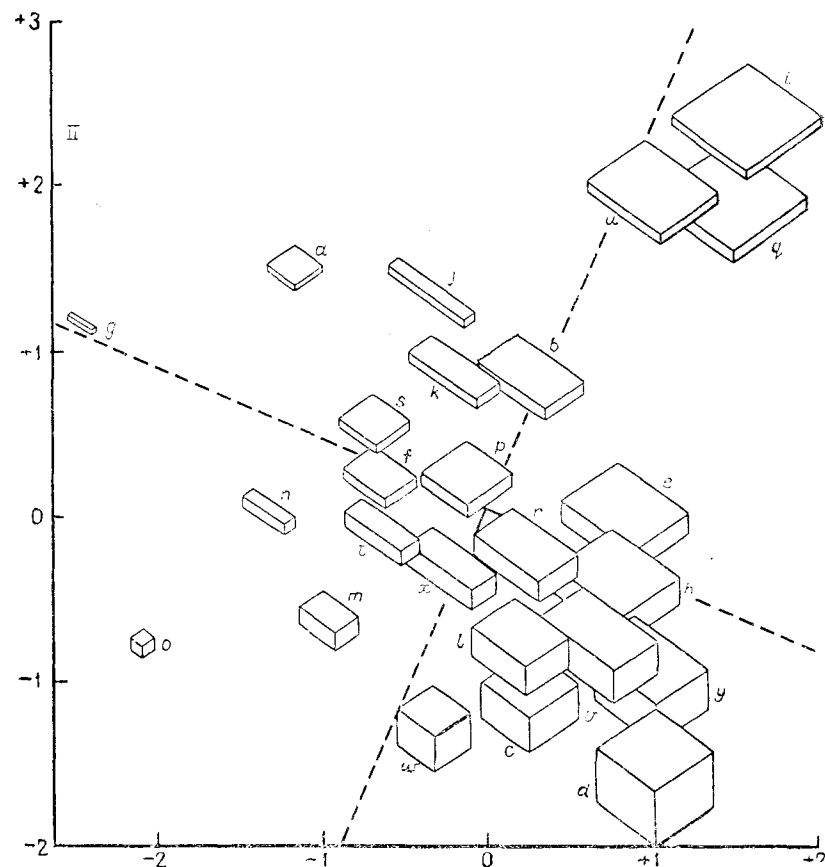
Рис. 6.38. Графическое представление факторных меток данных по случайным блокам для первых двух факторов (I и II).
