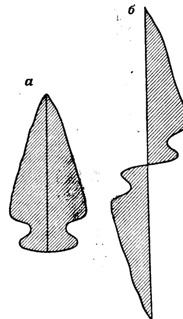
Рис. 5.43. Контур наконечника кремневой стрелы позднего палеолита:
