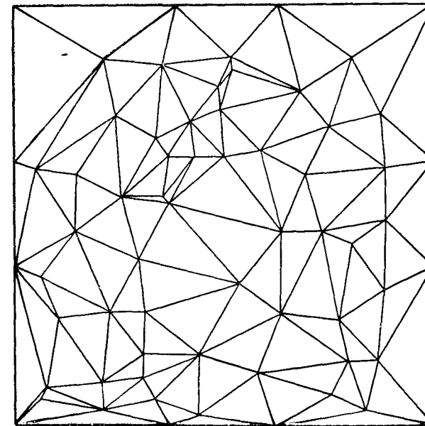
Рис. 5.50. Треугольная сеть Делоне для контрольных точек, изображенных на рис. 5.49. Добавлены ложные точки по краю карты
