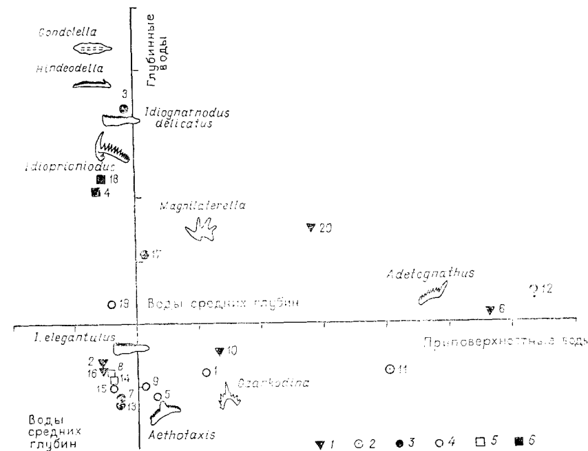
Рис. 6.44. Представление факторных нагрузок метода соответствия для данных по распространенности конodontов, представленных в табл. 6.37.
