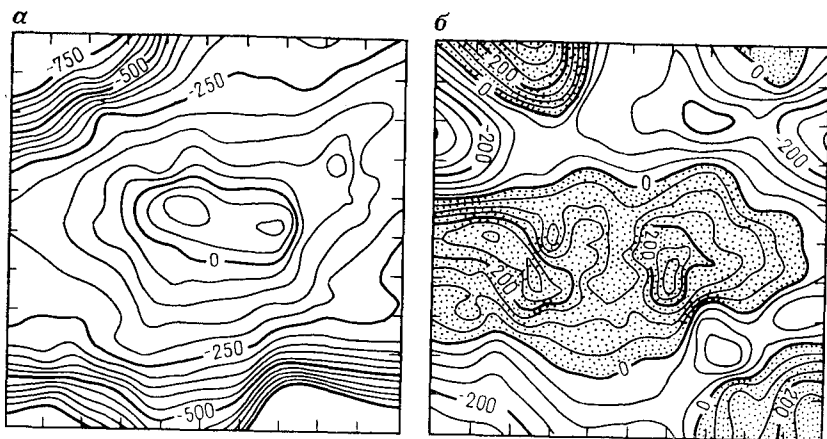
Рис. 5.101. Структурная карта, полученная на основании сейсмических данных (а) и карта разностей отметок изолиний карты «а» и структурной карты рис. 5.100 (б). Заштрихованы площадки, на которых предсказанные значения положительных отклонений ниже истинных.
