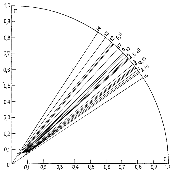
Рис. 6.41. Графическое изображение факторных нагрузок в Q-методе для 20 проб изверженных пород (см. рис. 6.42)
