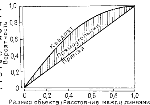
Рис. 5.6. Вероятность обнаружения линейного объекта равномерной схемой, изменяющейся от поиска множеством квадратов до поиска множеством параллельных линий.
