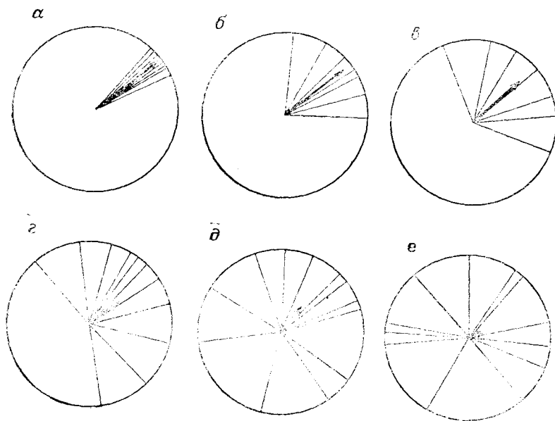
Рис. 5.22. Множества единичных векторов, иллюстрирующие значение, получаемое при различном расположении векторов во всех примерах, среднее направление — 52^\circ :
