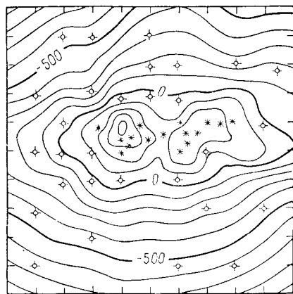
Рис. 5.100. Структурная карта кровли отражающего горизонта, построенная по данным бурения.
