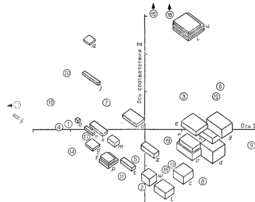
Рис. 6.47. Представление нагрузок R - и Q -методов на первые две оси соответствия для данных по блокам в порядке возрастания их объемов.
