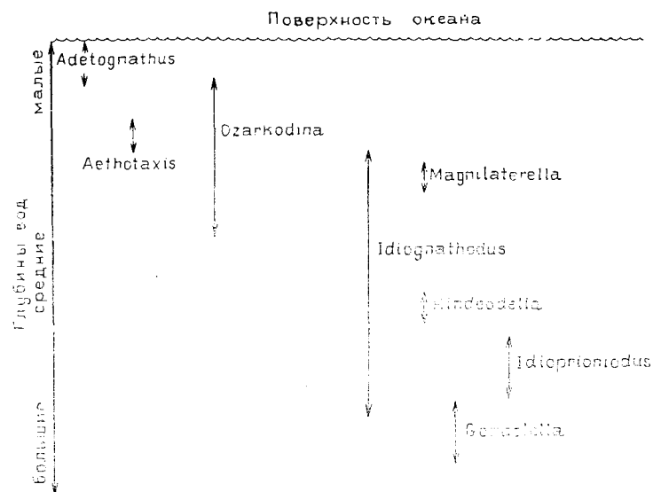
Рис. 6.45. Области значений относительных глубин для конодентов из Миссиссиппийской стратиграфической последовательности
