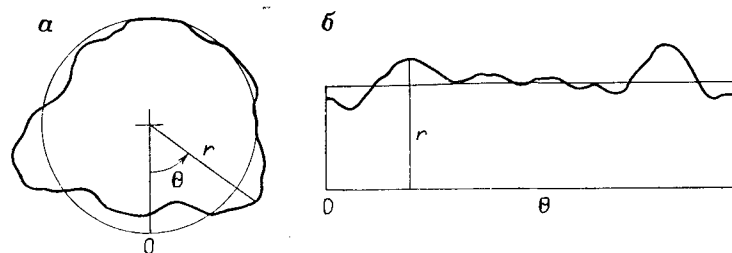
Рис. 5.37. Эквивалентность между полярными и декартовыми представлениями координат:
