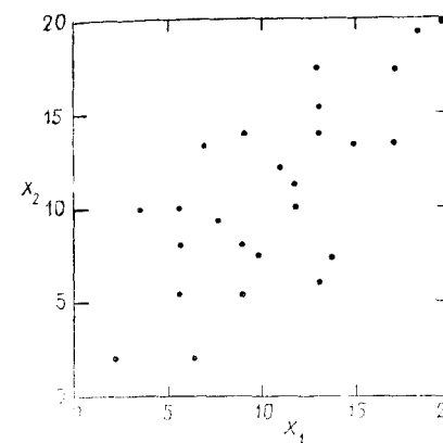
Рис. 6.18. Диаграмма рассеяния двухмерных данных табл. 6.19
