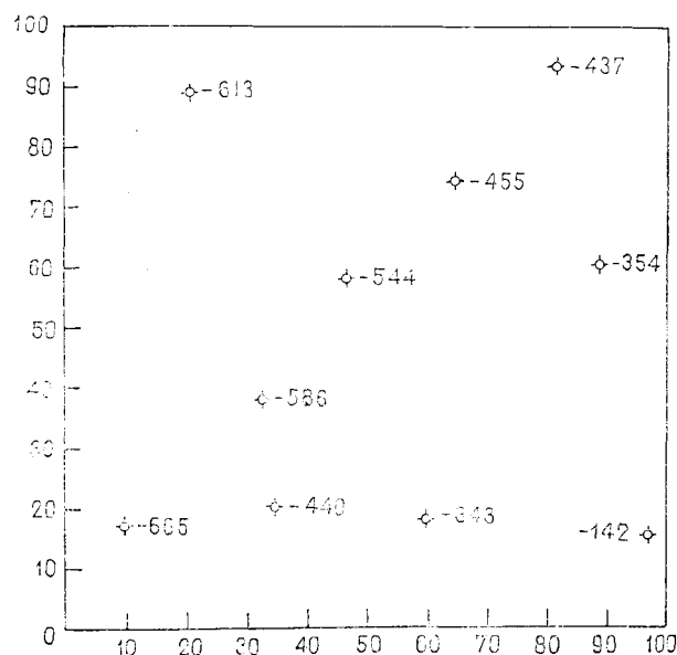
Рис. 5.73. Карта расположения скважин и абсолютных отметок подошвы меловых отложений в Северо-Восточной Африке. По данным нефтяной компании Англо-Баррен Ойл Кампани.
