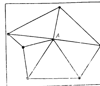
Рис. 5.46. Сеть треугольников Делоне вокруг точки A.
