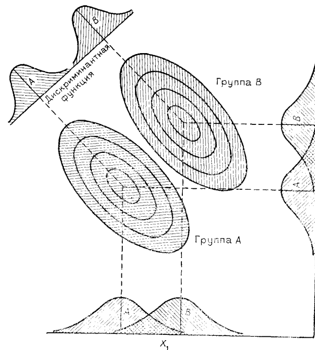
Рис. 6.2. Графическое представление двух двумерных распределений. Указаны перекрытия распределений для групп А и В по осям X_1 и X_2 ; проектирование на дискриминантную линию позволяет различить две группы
