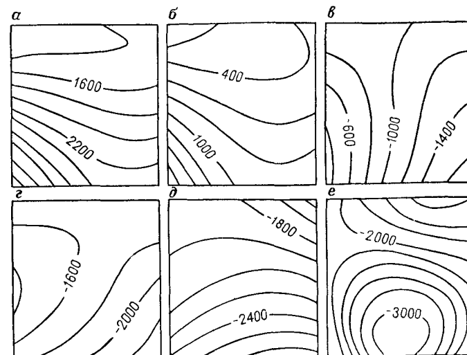
Рис. 5.107. Поверхности тренда третьей степени для стратиграфических формаций в Северо-Западном Канзасе [57].
