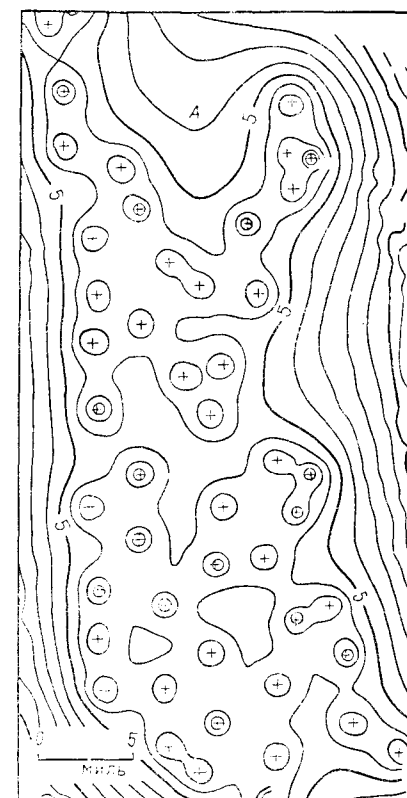
Рис. 5.68. На карте представлена стандартная ошибка оценок уровней воды в Экус Бедз.
