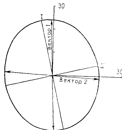
Рис. 6.26. Близкий к окружности эллипс, определенный векторами дисперсий и ковариаций для рандомизированных данных рис. 6.15.
