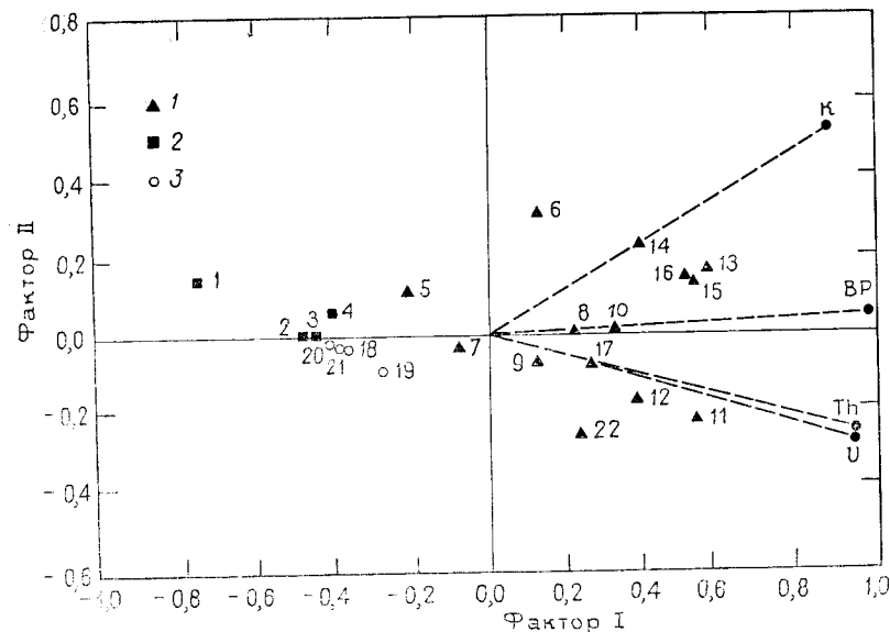
Рис. 6.50. Представление нагрузок R- и Q-методов на две первые факторные оси для данных Берса, вычисленных из ковариационной матрицы (см. табл. 6.42) [65].
