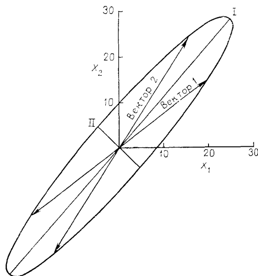
Рис. 6.20. Эллипс, определенный дисперсиями и ковариациями данных табл. 6.19 для ореола точек, представленных на рис. 6.18.
