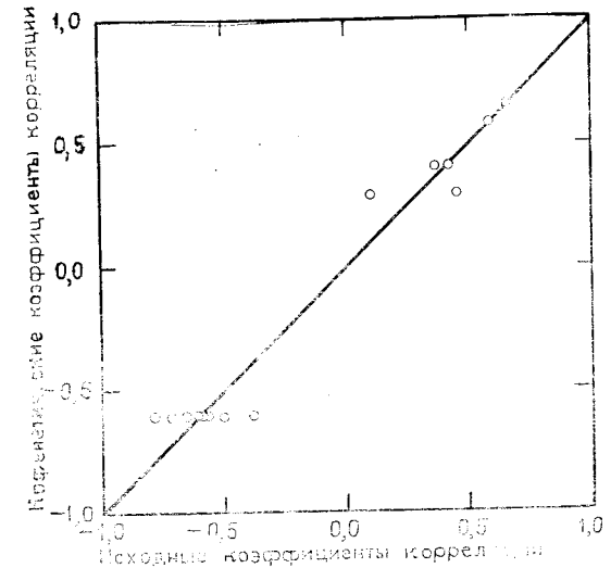
Рис. 6.7. Графическое представление зависимости кофенетических коэффициентов корреляции для дендрограммы, представленной на рис. 6.6, от эквивалентных им исходных коэффициентов корреляции, значения которых приведены в табл. 6.11.
