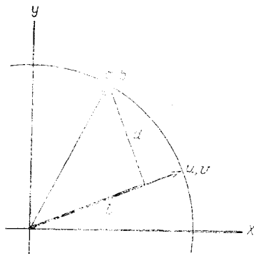
Рис. 5.29. Проекция вектора a, b на вектор u, v .
