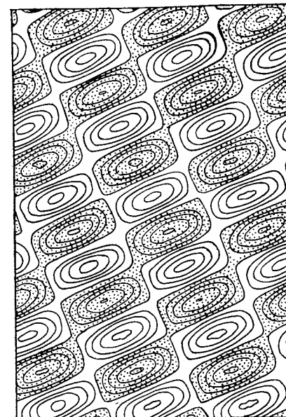
Рис. 5.96. Реконструкция изолиний двух доминирующих волновых форм для волноприбойных знаков.
