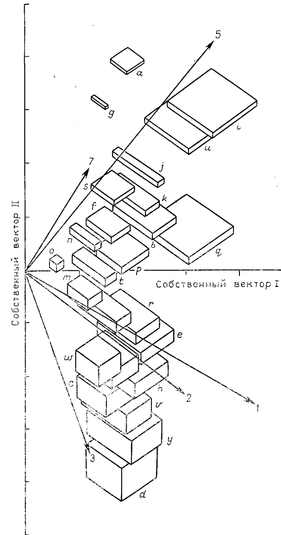
Рис. 6.48. Представление нагрузок R - и Q -методов на две первые факторные оси для данных по блокам, вычисленных для матрицы необработанных сумм квадратов и попарных произведений [X][X] .
