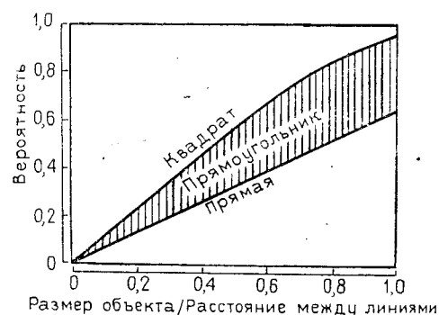
Рис. 5.5. Вероятность обнаружения кругового объекта с прямоугольной схемой поиска, изменяющейся от квадратной схемы до множества параллельных линий.
