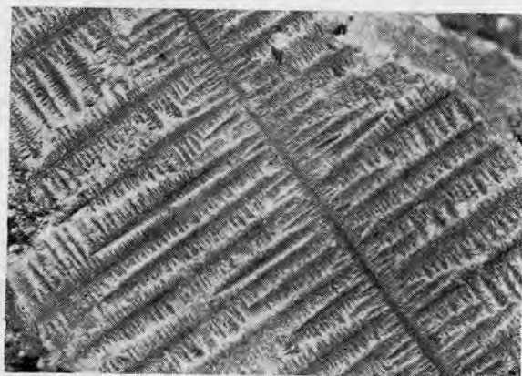
Рис. 27. Пустоты растворения от дендритов самородного серебра I в агрегате сафлорита и раммельсбергита ( \times 8 ).
