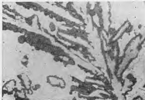
Рис. 17. Выделения настурана II вокруг дендритов никелина в массе раммельсбергита (микрофото; \times 70 ).
