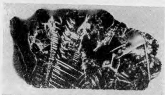
Рис. 13. Авторадиограмма настурана II, окружающего дендриты самородного висмута I ( \times 11 ).
