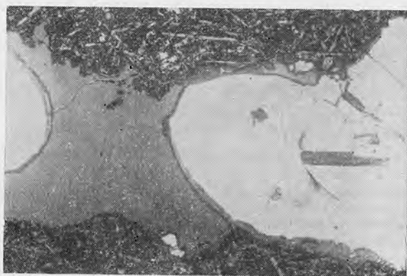
Рис. 2. Каплевидные выделения самородного висмута (белый) с включениями висмутина в кальцитовом прожилке (серый) из третичного базальта (микрофото; \times 70 ).
