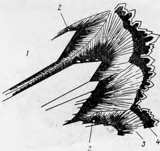
Рис. 35. Бариты поздних генераций: 1— барит II; 2— «присыпки» халькопирита; 3— барит III; 4— зонарные кристаллы барита IV.
