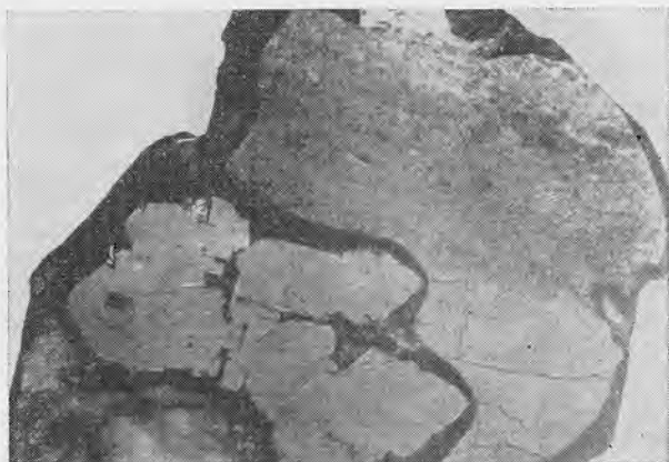
Рис. 3. Метакристаллы пирита в агрегате пирротина, заместившего биотитовый сланец. Вокруг кристаллов пирита кайма хлорита с редкими включениями халькопирита ( \times 1 ).
