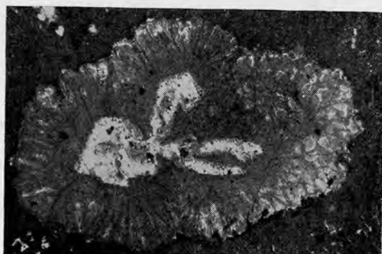
Рис. 19. Столбчатый настуран II вокруг кристалла самородного висмута I (микрофото аншлифа; \times 115 ).
