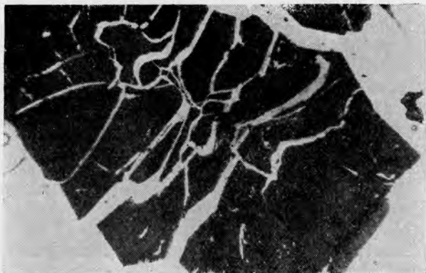
Рис. 23. Кристаллы настурана II в никелине (белый) (микрофото аншлифа; \times 450 ).
