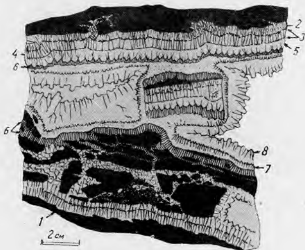
Рис. 34. Зарисовка штуфа из карбонатной жилы: 1 — углистый сланец; 2, 4, 5 — регенерированный доломит арсенидного парагенезиса с включениями полусфер гематита; 3 — гематит; 6 — сидерит; 7, 8 — поздний кальцит.
