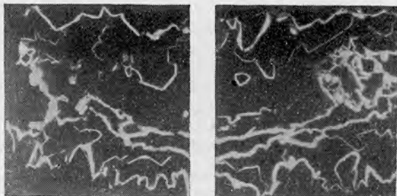
Рис. 7. Почковидные корки настурана вокруг скаленоэдрических кристаллов кальцита, нацело замещенного доломитом (авторадиограмма; \times 1 ).
