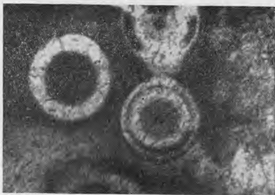
Рис. 10. Гало, образованные в результате пробега \alpha -частиц различных радиоактивных элементов в кристалле фиолетового флюорита (микрофото прозрачного шлифа, полученное на микроскопе МИМ-7 с зеркалом; \times 450 ).
