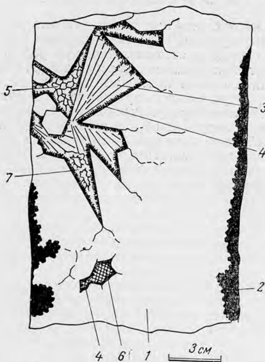
Рис. 37. Выполнение баритом пустот в агрегате скаленоэдрического кальцита:
