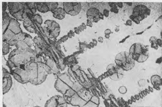
Рис. 16. Две генерации настурана II, отложившиеся на дендритах самородного серебра I и сцементированные раммельсбергитом (фото шлифа; \times 10 ).
