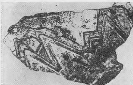
Рис. 8. Структура доломитовой жилы, образовавшейся в результате замещения кальцитовой жилы, иллюстрируется шлифовкой штуфа. Включения гаматита (темно-серое) подчеркивают зоны роста скаленоэдрических кристаллов (фото, \times 1,5 ).
