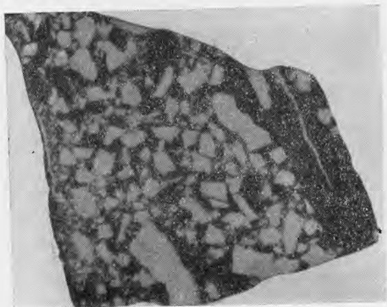
Рис. 31. Обломки выделений настурана I (белое), сцементированные поздним кальцитом (автордиограмма; \times 1 ).
