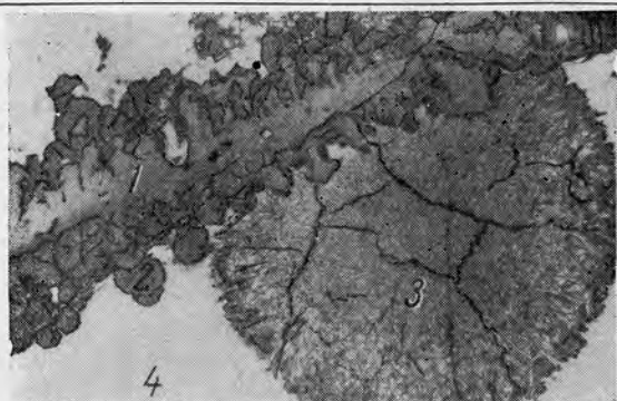
Рис. 21. Скелетные сферолиты пластинчатого настурана II:
