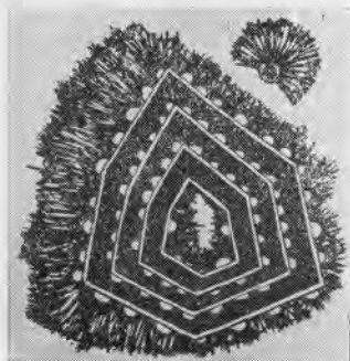
Рис. 25. Спекулярит, замещивший совместно с кварцем анкерит (?) по скаленоздрическому кальциту. Полусферы красного гематита сохранились при замещении и своим расположением подчеркивают скаленоздрическую форму исчезнувшего кристалла (незначительно увеличено).
