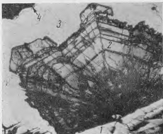
Рис. 18. Выделения никелина (2) на скуттерудите (1), покрытые последовательно коркой раммельсбергита (3) и настурана II (4) (микрофото; \times 89 ).
