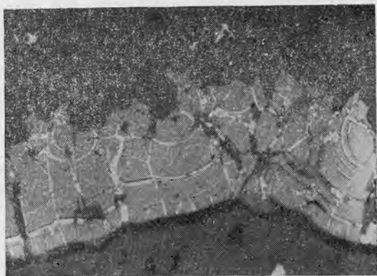
Рис. 5. Колломорфная почковидная корка настурана с прожилками халькозина и кальцита на гребенчатом кварце (микрофото аншлифа; \times 70 ).
