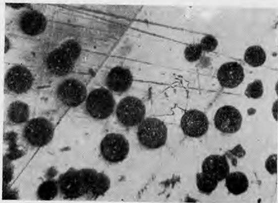
Рис. 32. Сферолиты настурана II в клаусталите (микрофото шлифа; \times 450 ).
