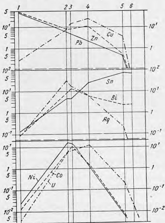
Рис. 36. Относительное содержание металлов в рудогорских гранитах (по Эльснеру):
