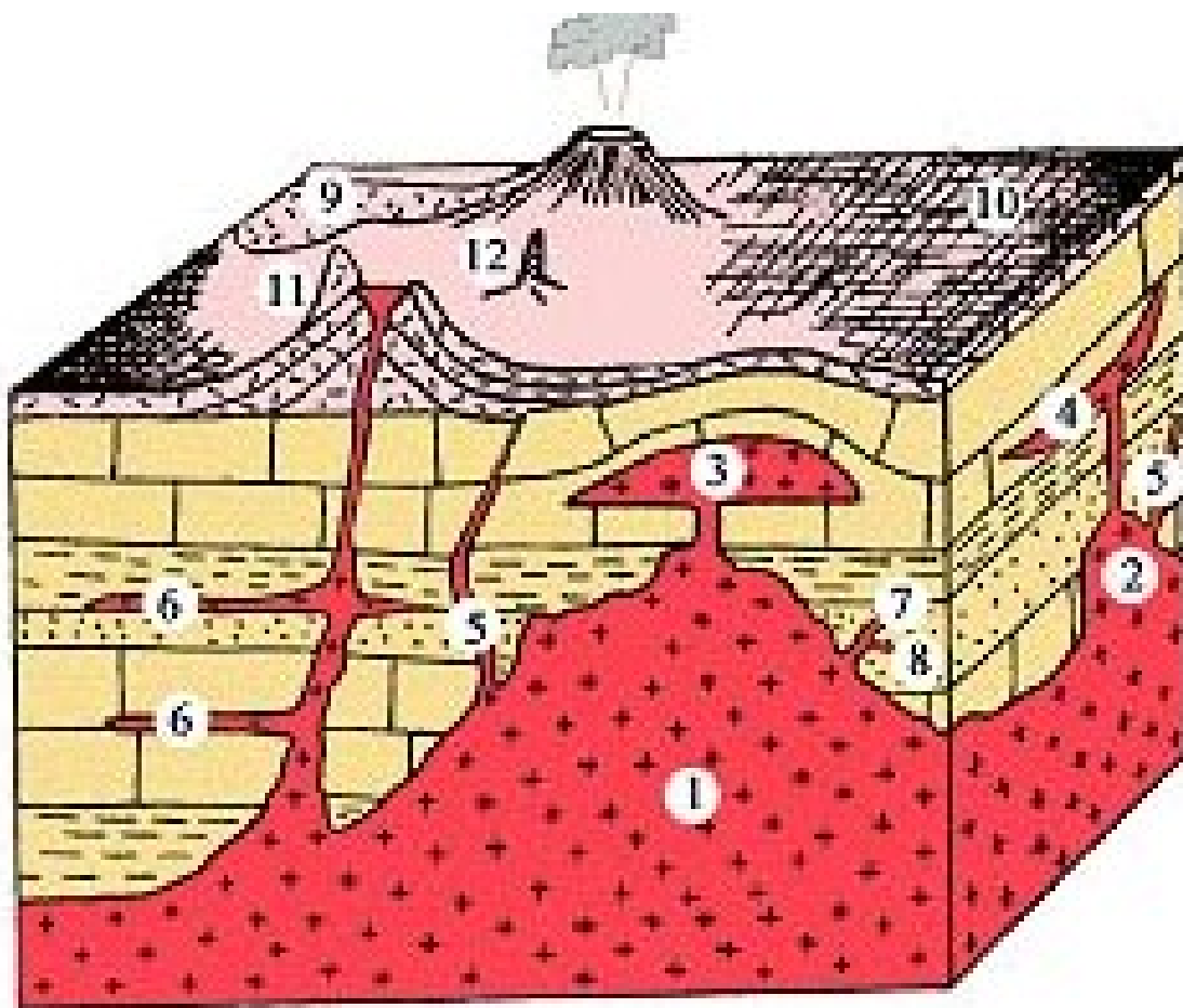
Рис. 31. Формы залегания магматических тел
