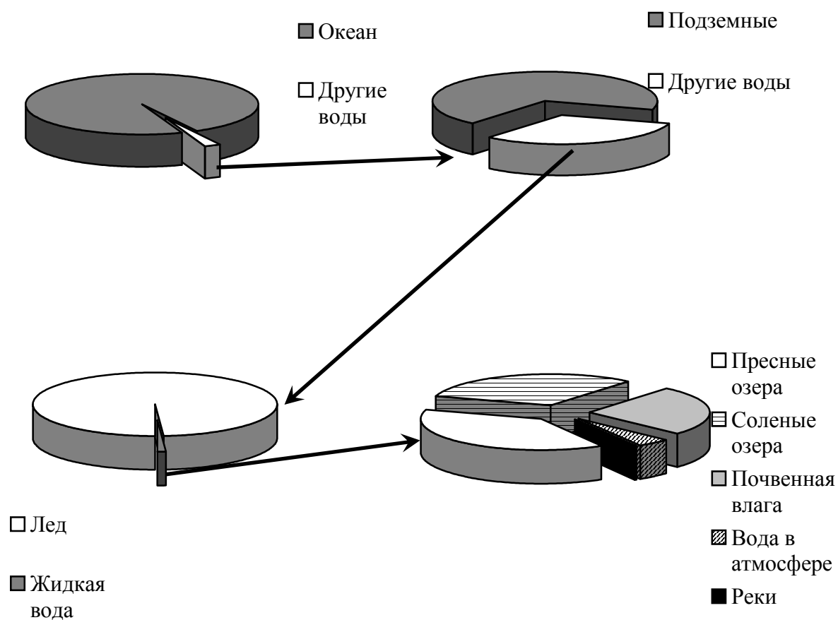
Рис. 8. Состав гидросферы по классам вод
