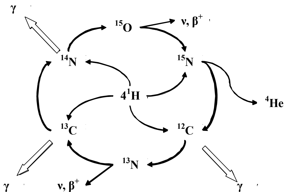
Рис. 2. Углеродный цикл Бете–фон Вайцзекера
