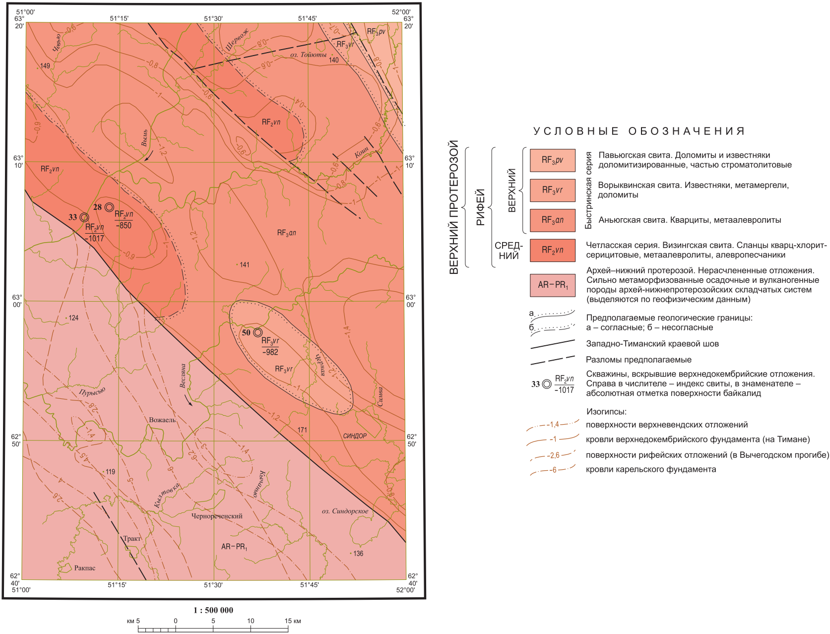
СХЕМА ГЕОЛОГИЧЕСКОГО СТРОЕНИЯ ФУНДАМЕНТА
