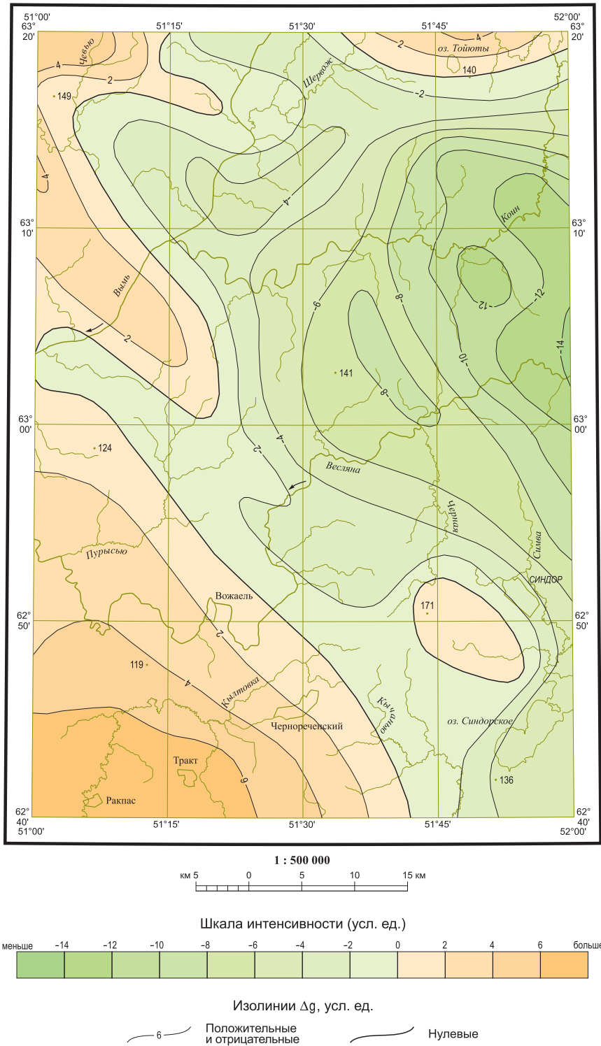
СХЕМА ГРАВИТАЦИОННЫХ АНОМАЛИЙ
