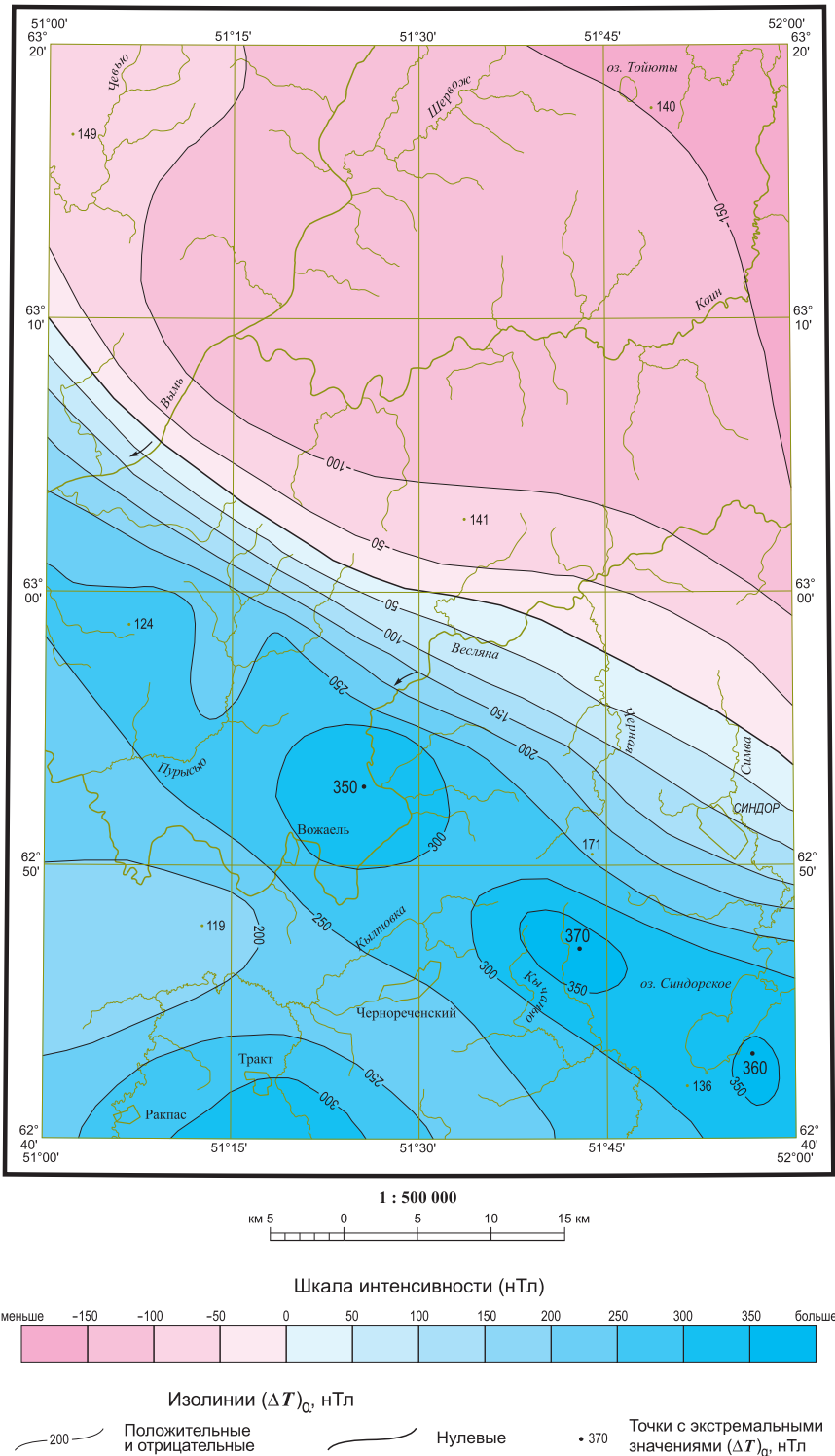
КАРТА АНОМАЛЬНОГО МАГНИТНОГО ПОЛЯ
