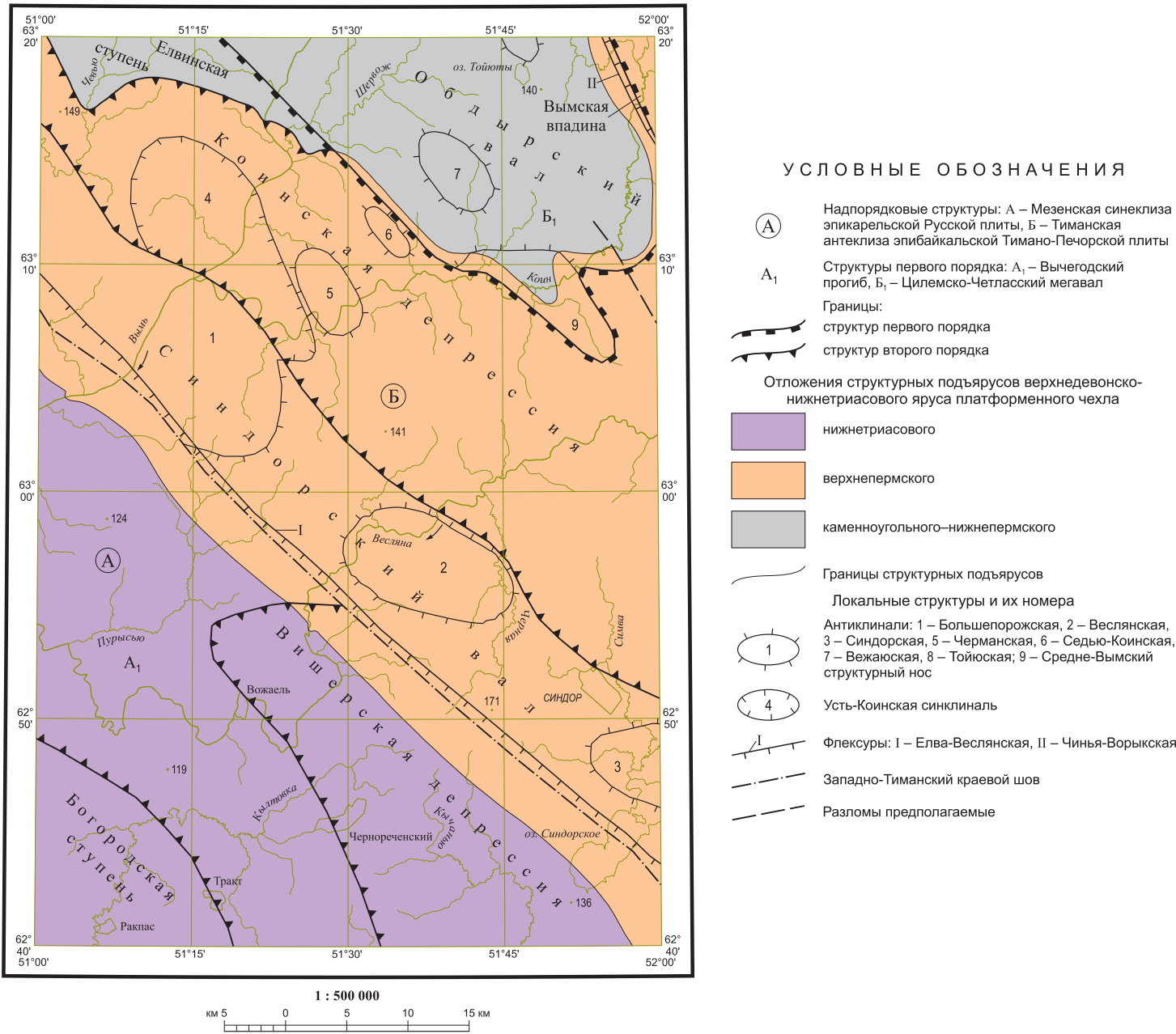
ТЕКТОНИЧЕСКАЯ СХЕМА
