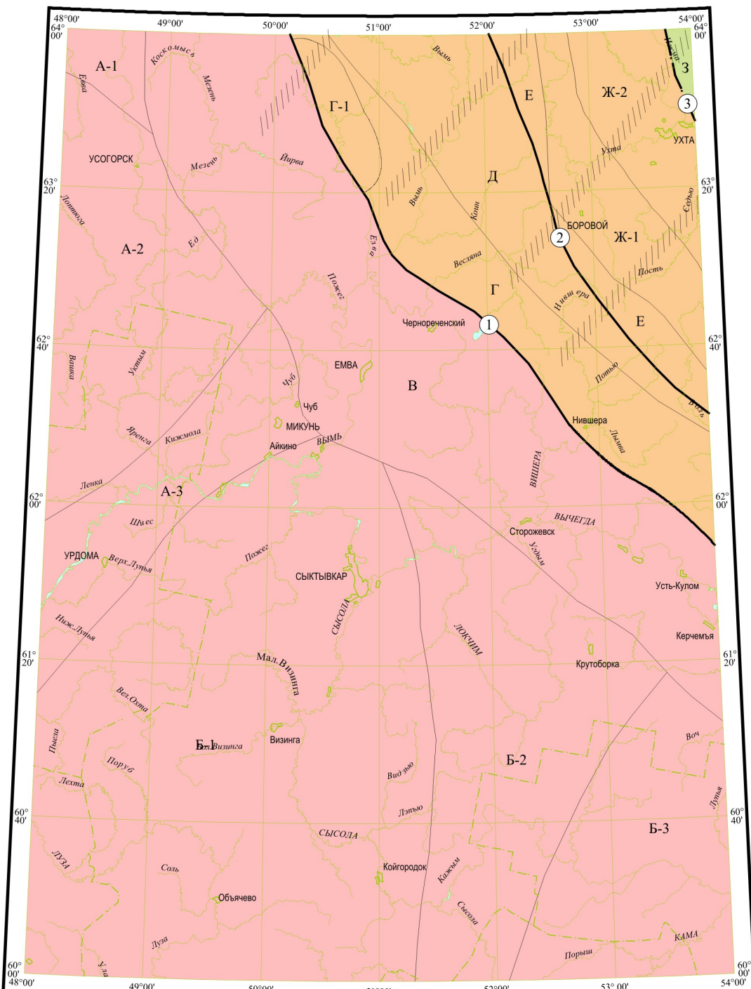
ТЕКТОНИЧЕСКАЯ СХЕМА ФУНДАМЕНТА Масштаб 1 : 2 500 000
