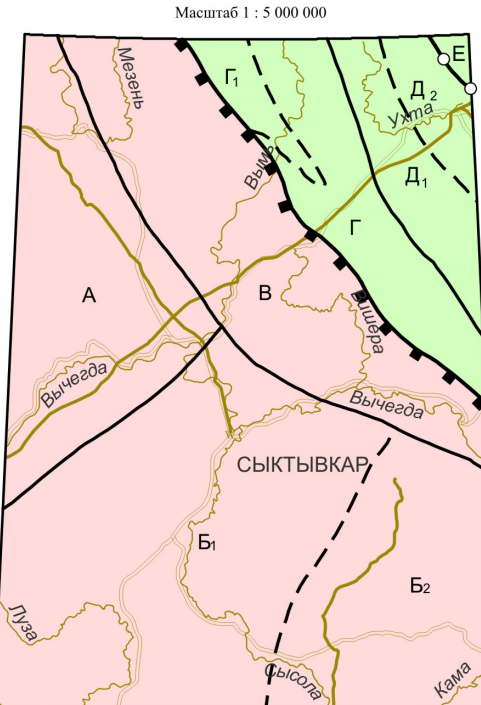
СХЕМА ТЕКТОНИЧЕСКОГО РАЙОНИРОВАНИЯ Масштаб 1 : 5 000 000
