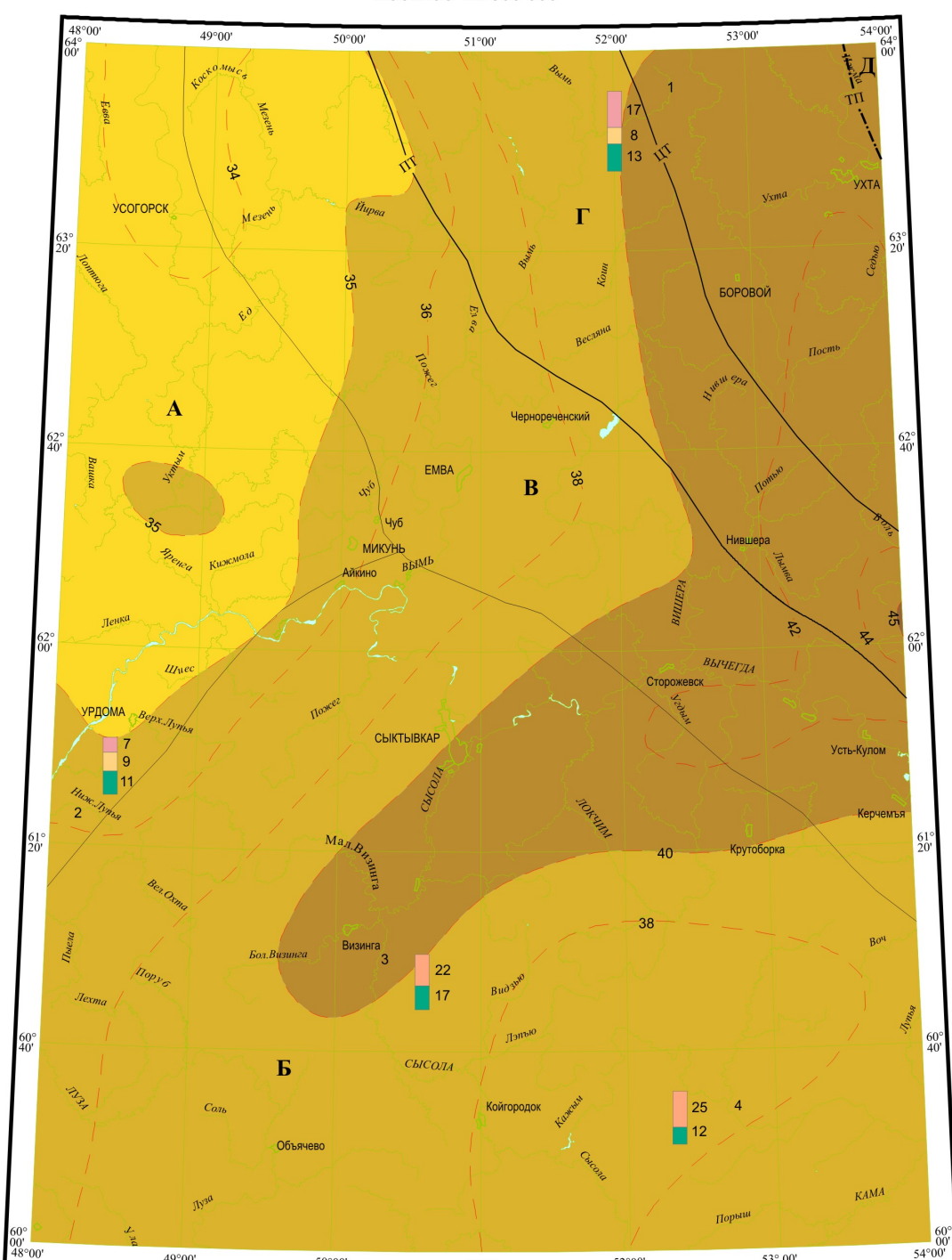
СХЕМА ГЛУБИННОГО СТРОЕНИЯ Масштаб 1:2 500 000
