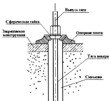
Рисунок 3.2 – Конструкция оголовка анкера
