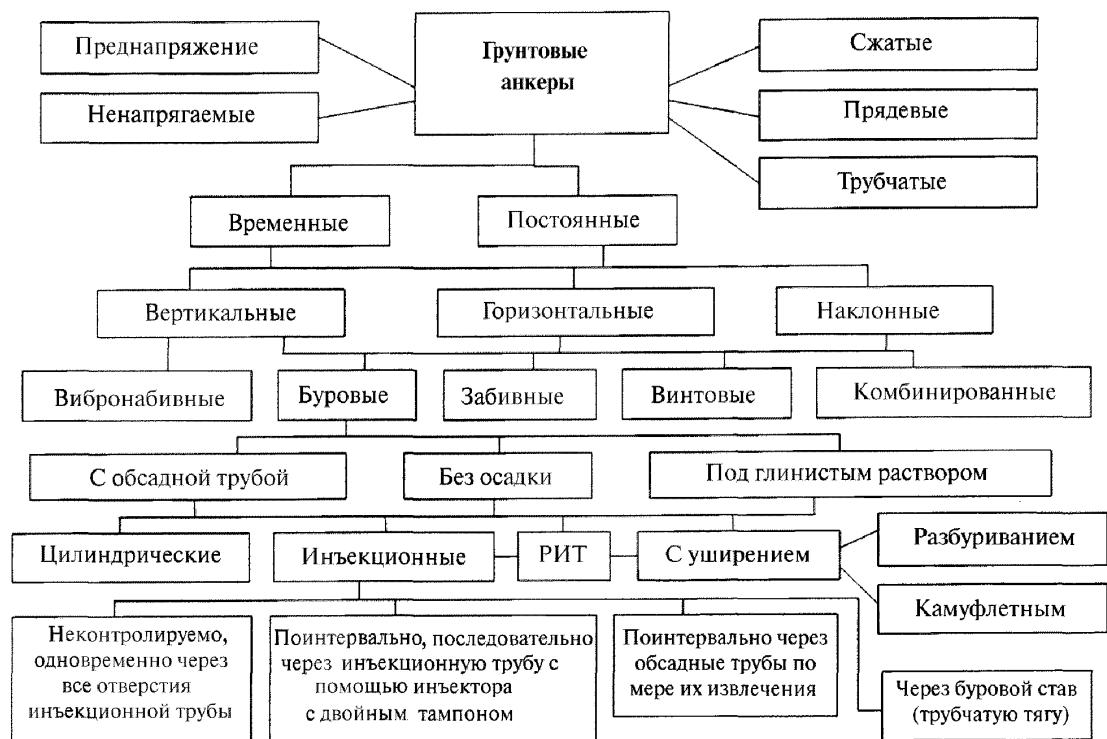
Рисунок А.1 – Схема классификации грунтовых анкеров
