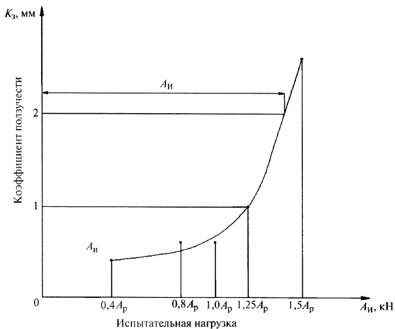
Рисунок Т.2 – Графическое определение предельной нагрузки A_{и} по изменению коэффициента ползучести K_z
