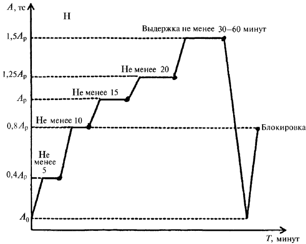
Рисунок 11.5 – Программа контрольных испытаний
