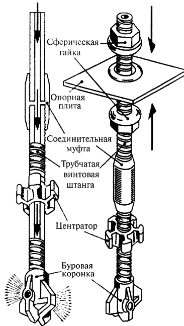
Рисунок 9.1 – Конструкция анкера (микросваи) из трубчатой винтовой штанги
