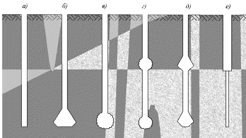
а) – цилиндрическая; б) – с разбуhrенным основанием; в) – с пятой, уширенной трамбованием или инъекцией; г) – с промежуточными инъекционными уширениями; д) – с промежуточными расширениями, образуемыми разбуhrиванием; е) – телескопическая
