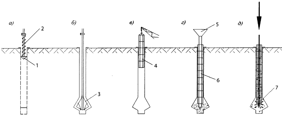
а) – проходка скважины; б) – устройство уширения механическим способом (при необходимости); в) – погружение армокаркаса; г) – заполнение скважины; д) – опрессовка ствола; 1 – буровая коронка; 2 – шнек; 3 – опускной механический расширитель; 4 – армокаркас; 5 – приемная воронка; 6 – бетонолитная труба; 7 – опускной иньектор
