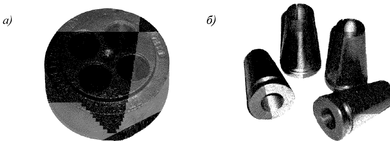
а) – инвентарная обойма под тягу из четырех арматурных канатов; б) – заклинивающие трехлепестковые конусы
