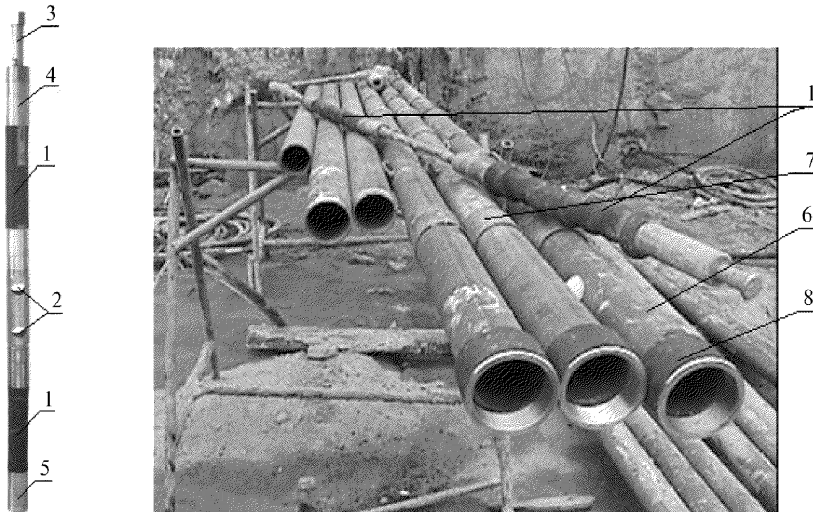
Рисунок 10.10 – Иньектор с двойным уплотнительным тампоном*
