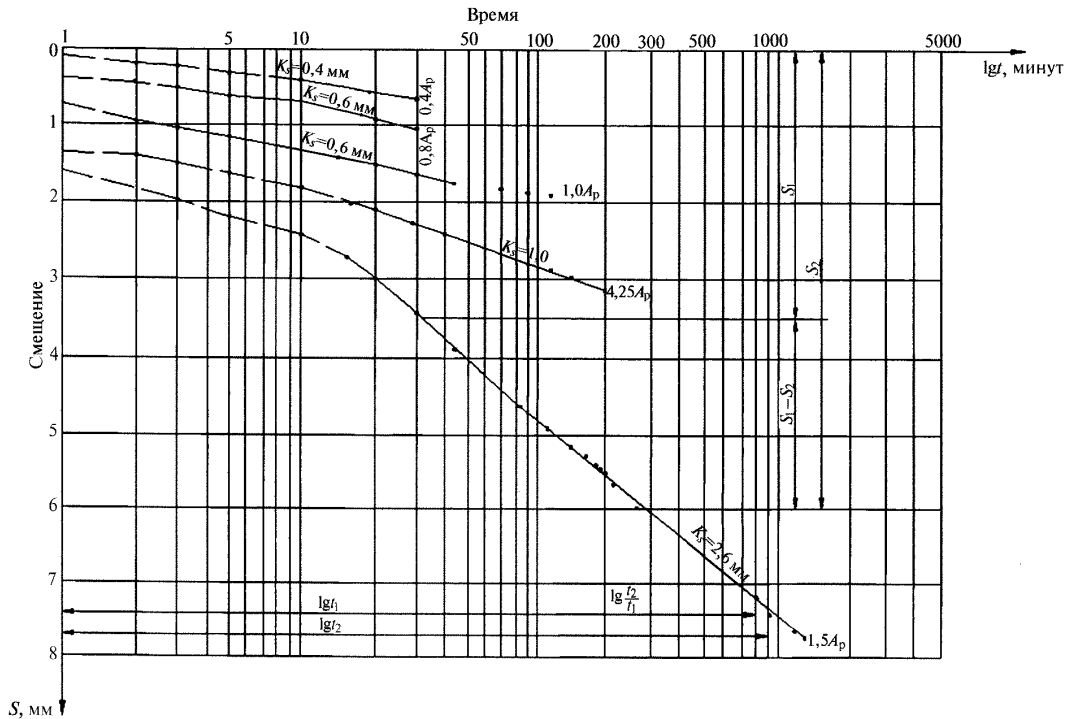
Рисунок Т.1 – Графики зависимости смещений во времени S = f(\lg t) для определения коэффициента ползучести
