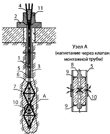
Рисунок 7.3 – Типовая конструкция временного инъекционного анкера с манжетной трубой при наружном расположении арматурных канатов (прядей)
