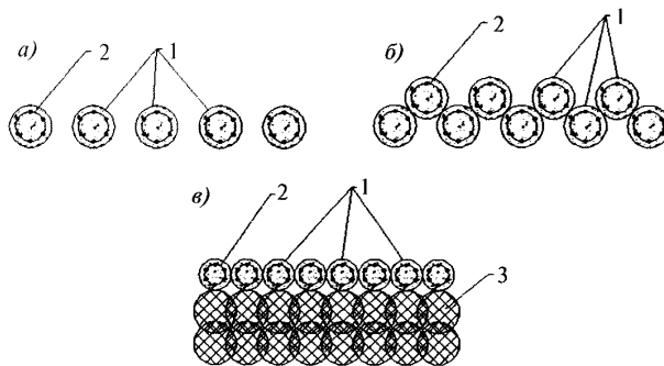
а) – стена из микросвай прерывистого расположения; б) – размещение микросвай в несколько рядов в шахматном порядке; в) – размещение касательных микросвай в один ряд с противофильтрационной стенкой из ГЦС;
