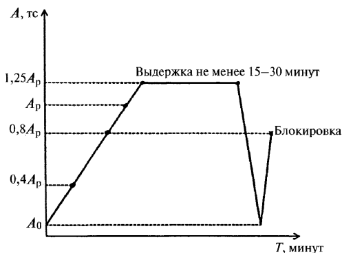
Рисунок 11.6 – Программа приемочных испытаний
