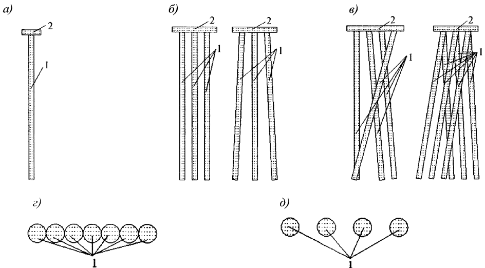
а) – одиночная микросваля; б) – группа (куст) микросвай; в) – сетка из микросвай; г) – стена из микросвай касательного расположения; д) – стена из микросвай прерывистого расположения;
