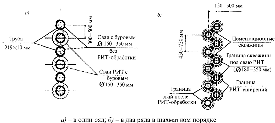
Рисунок 7.11 – Варианты расположения микросвай РИТ в подпорной стенке*
