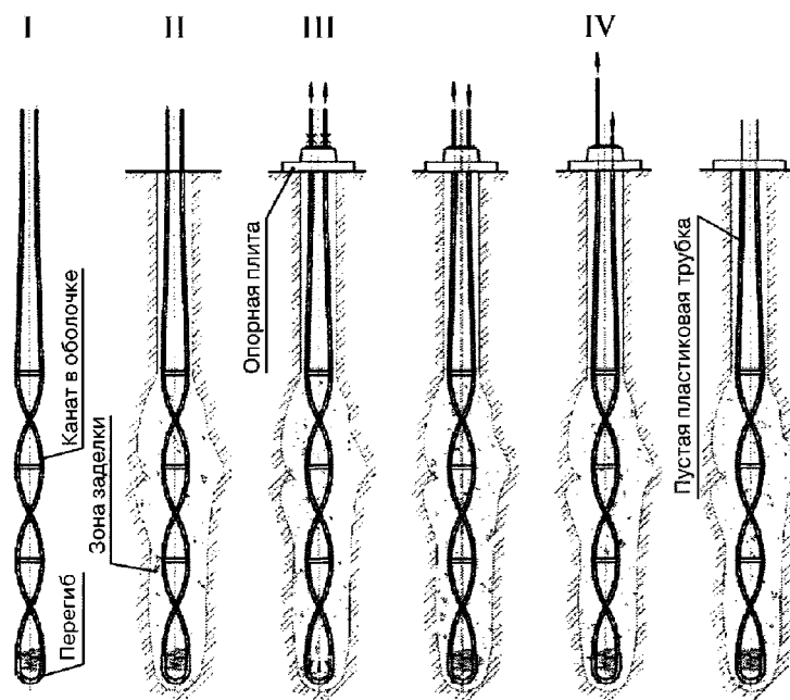
I – анкер перед установкой; II – установка и инъектирование; III – натяжение; IV – извлечение
