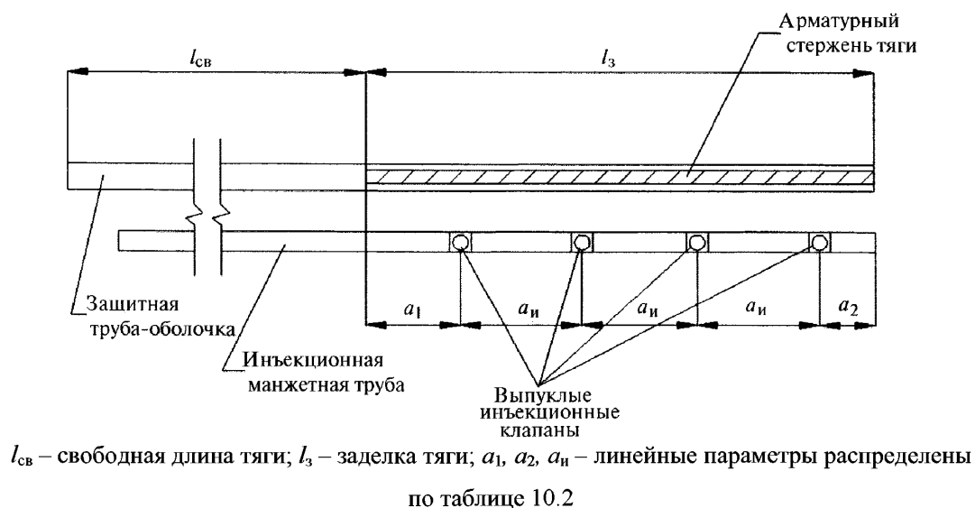
Рисунок 10.3 – Распределение выпускных клапанов по длине инъекционной трубы
