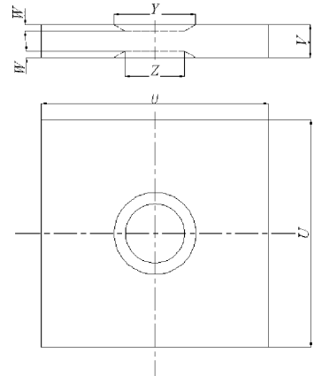
Рисунок Л.3 – Опорная плита
