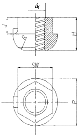
Рисунок Л.1 – Фиксирующая шаровая гайка. Тип 1
