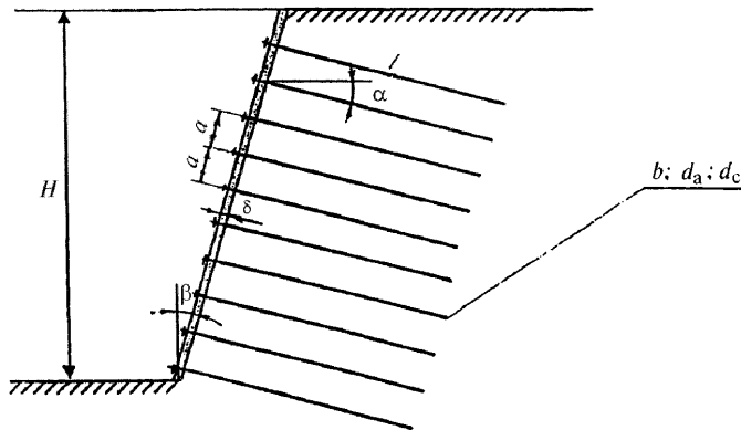
Рисунок 6.1 – Основные конструктивные параметры нагельного крепления
