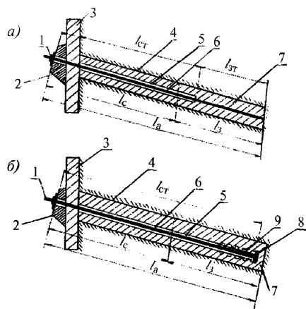
Рисунок 3.1 – Основные элементы грунтового анкера
