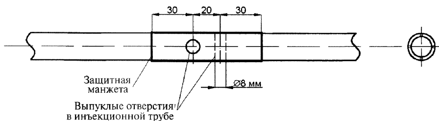
Рисунок 10.4 – Схема расположения выпускных отверстий в инъекционной трубе
