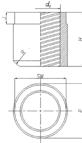
Рисунок Л.2 – Фиксирующая гайка. Тип 2
