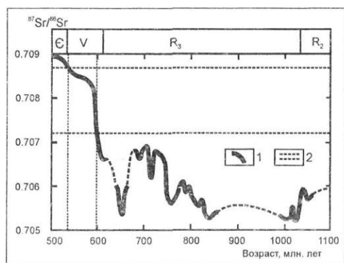
Рис. 9. Изотопный состав стронция в карбонатных отложениях боксонской и снисейской серий в сравнении с кривой эволюции ^{87}\text{Sr}/^{86}\text{Sr} в неопротерозойском океане [по Кузнецову и др., 2003].
