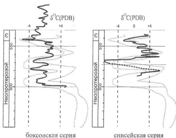
Рис. 10. Сопоставление изотопного состава углерода карбонатных отложений боксонской и снисейской серий с обобщенной кривой (Brasier et al., 2000; Jacobsen, Kaufman, 1999) вариации изотопного состава углерода в морской воде в венде-раннем кембрии
