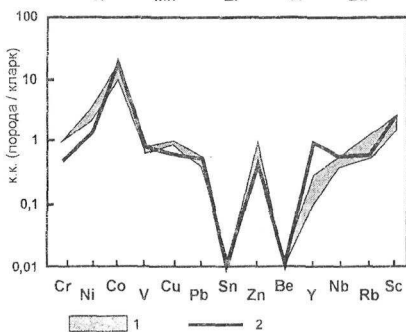
Рис. 19. Распределение основных типоморфных и примесных элементов в карбонатных отложениях задговых бассейнов (1) и одновозрастных сублатформенного типа (2).
