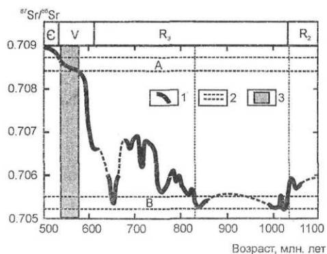
Рис. 6. Изотопный состав стронция в карбонатных отложениях байкальской серии (А) и иркутской и шунтарской свит (В) в сравнении с кривой эволюции ^{87}\text{Sr}/^{86}\text{Sr} в неопротерозойском океане [по Кузнецову и др., 2003].
