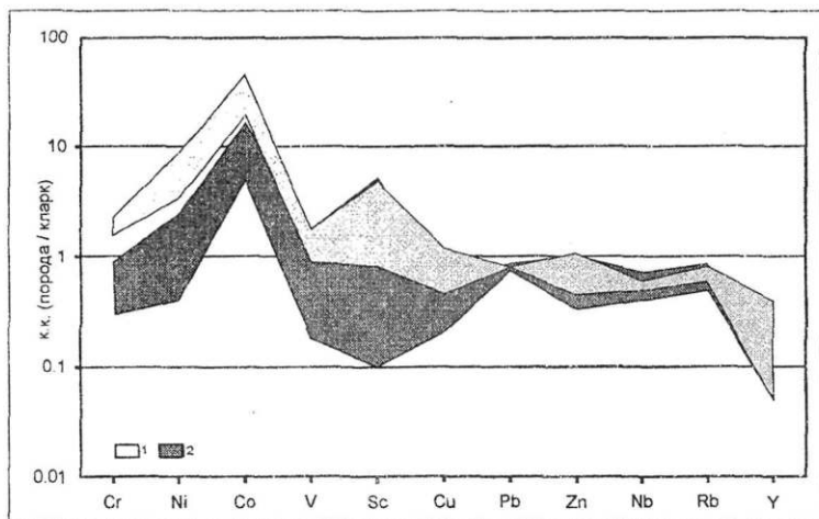
Рис.12. Распределение элементов примесей в шельфовых карбонатных отложениях Тувино-Монгольского микроконтинента, Амалатской глыбы и Батеневского кража. Усл. обозн. см.рис.11.
