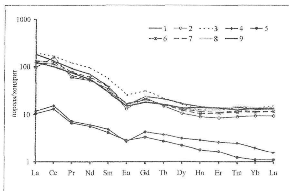
Рис. 2. Тренд распределения REE в породах байкальской серии, гнейсо-гранитов приморского комплекса и PAAS.
