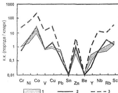
Рис. 20. Распределение основных типоморфных и примесных элементов в карбонатных отложениях задговых бассейнов (1) и мелководных (2) и глубоководных (3) карбонатных породах океанических островов.
