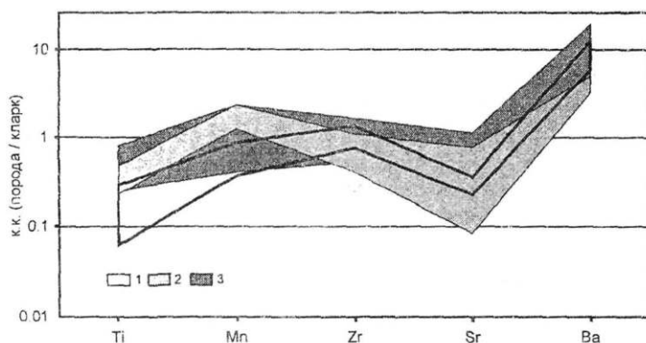
Рис.7. Распределение основных типоморфных элементов в карбонатных отложениях древних континентальных блоков: 1 - байкальская серия (97 проб), 2 - иркутская свита (109 проб), 3 - шунтарская свита (96 проб).
