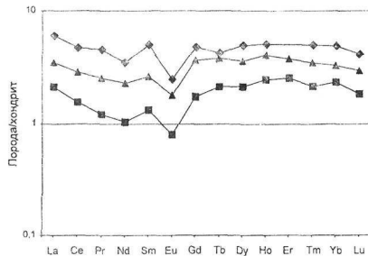
Рис. 22. Редкоземельный спектр хемогенных карбонатных отложений улунтуйской свиты, отражающий значительный вклад в его формирование морской воды.
