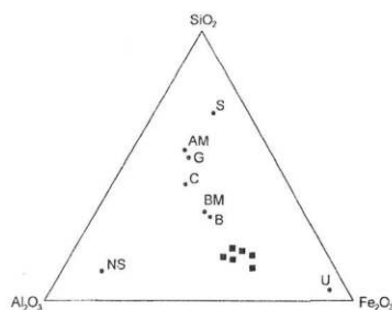
Рис. 13. Диаграмма средних составов бокситов, развивающихся по различным типам пород [Schellmann, 1986] и бокситов боксонской серии.
