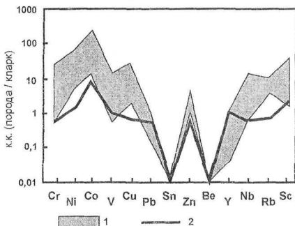
Рис. 21. Распределение основных типоморфных и примесных элементов в карбонатных отложениях океанических островов (1) и одновозрастных отложений сублатформенного типа (2).
