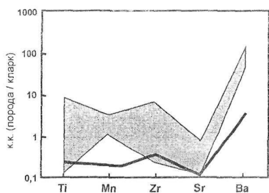
Рис. 19. Распределение основных типоморфных и примесных элементов в карбонатных отложениях задговых бассейнов (1) и одновозрастных сублатформенного типа (2).
