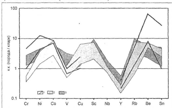
Рис.8. Распределение элементов-примесей в карбонатных отложениях древних континентальных блоков. Усл. обозн. см. рис.7.
