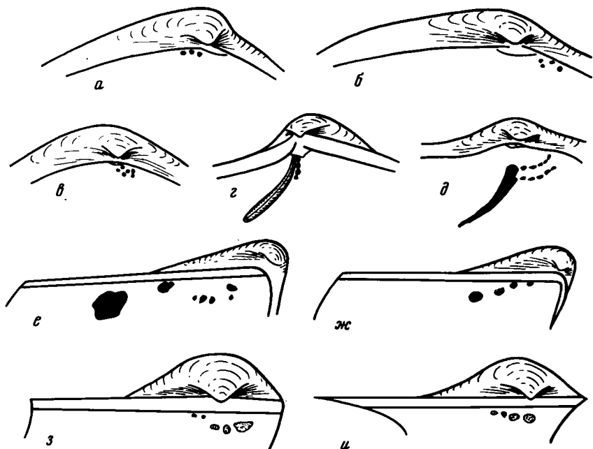
Р и с. 12. Отпечатки висцеральных мускулов Palaeonucula (а), Malletia (б), Prosoleptus (в), Dacryomya (г), Lapteviella (д), Myalina (е), Promyalina (ж), Bakevellia (з) и Hoernesia (и)
