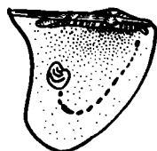
Р и с. 19. Схематический рисунок левой створки Bakevellia (Maizuria) reticularis (Popov) (*2)
