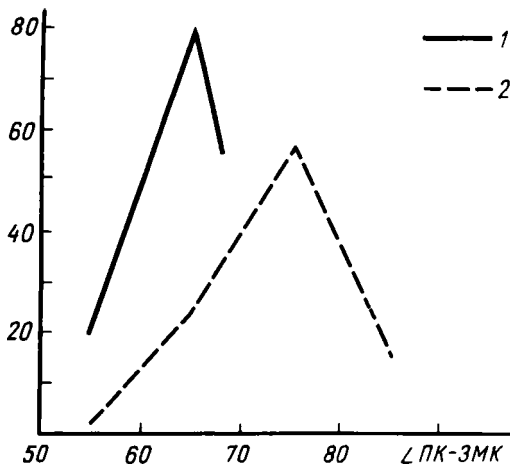
Р и с. 24. Индивидуальная изменчивость Bakevellia ( Maizuria ?) czezanowski Kur. из двух выборок верхнеанизийского подъяруса (1 — гора Туора-Хаята, 2 — мыс Аиркат)
