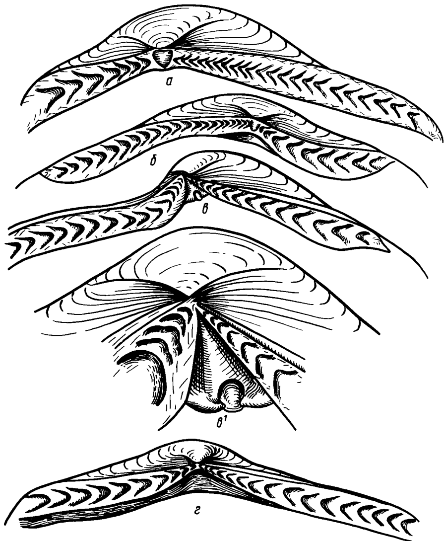
Р и с. 6. Строение замочного аппарата Taimyrodon (а), Lapteviella (б), Dacryomya (в), (а1 — ложечка) и Sarepta (г)
