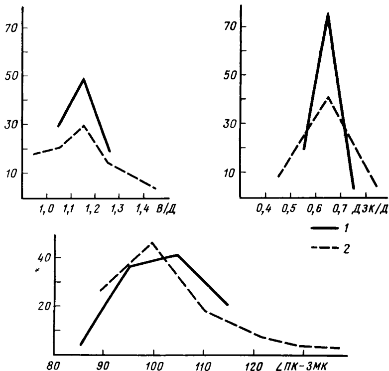
Р и с. 17. Индивидуальная изменчивость Promyalina schamarae (Bittner) из двух выборок индского яруса (1 — р. Даркы, 2 — р. Эбитием)
