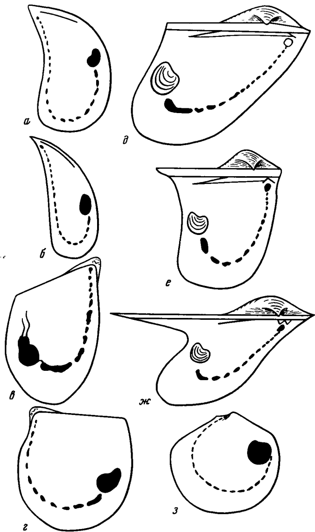
Р и с. 11. Мантийная линия и мускульные отпечатки Mytilus (а), Falcimytilus (б), Myalina (в), Promyalina (г), Bakevellia ( Maizuria ) (д), Bakevellia ( Boreiobakevellia ) (е), Hoernesia (ж) и Plagiostoma (з)
