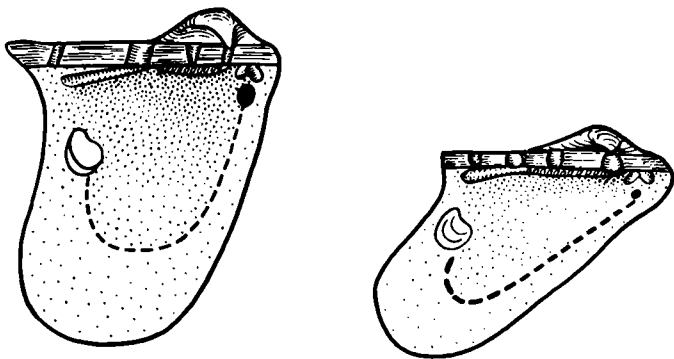
Р и с. 26. Схематический рисунок правой створки Bakevellia (Boreiobakevellia) prima Kug. (*2)
