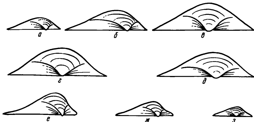
Р и с. 4. Макушки представителей рода Bakevellia (а—д — виды подрода Maizuria ):
