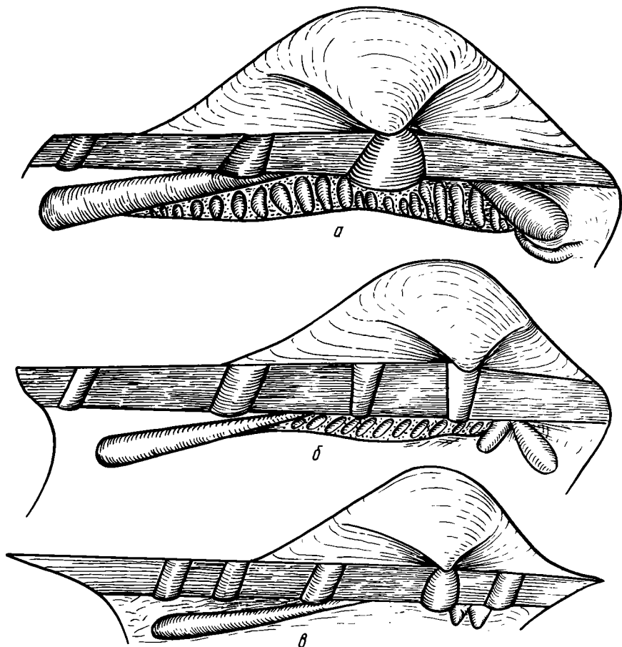
Р и с. 8. Строение замочного аппарата Bakevellia ( Maizuria ) (а), B. (Boreiobakevellia) (б) и Hoernesia (в)
