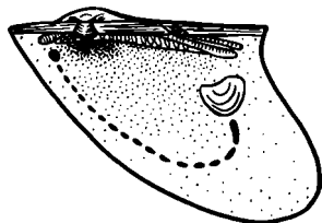
Рис. 22. Схематический рисунок правой створки Bakevella (Maizuria) lapteviciensis Kur. (*2)
