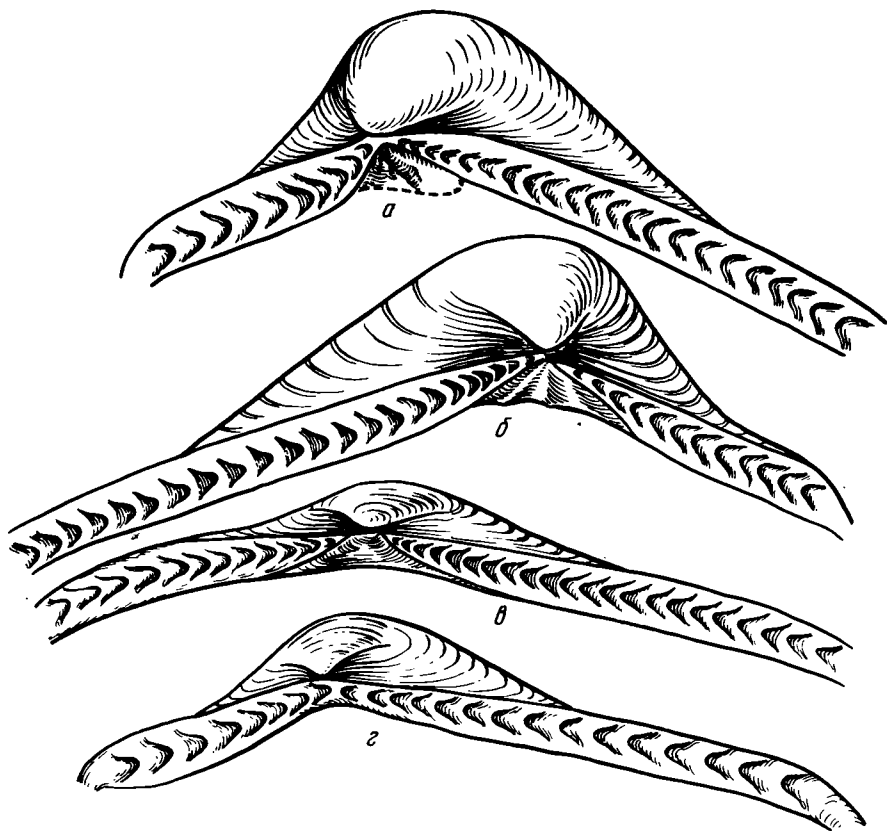
Р и с. 5. Строение замочного аппарата Nuculoma (а), Palaeonucula (б), Malletia (в) и Prosopleptus (г)
