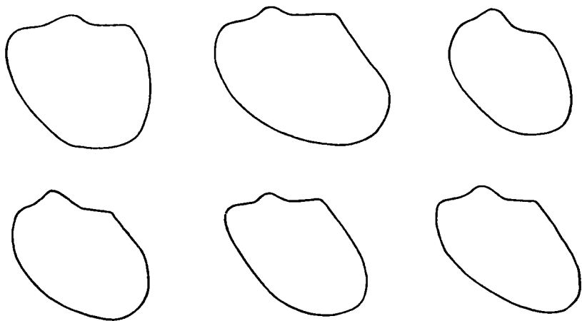
Р и с. 3. Изменчивость формы раковин вида Bakevellia (Maizuria) arctica (Kipar.), происходящих из одной выборки (Восточный Таймыр, мыс Цветкова, обн. 2, пачка 28, слой 40)
