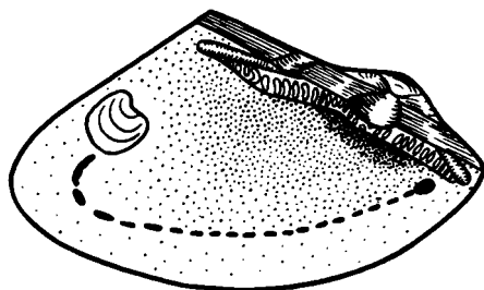
Р и с. 25. Схематический рисунок левой створки Bakevellia (Maizuria) ladinica Kur.
