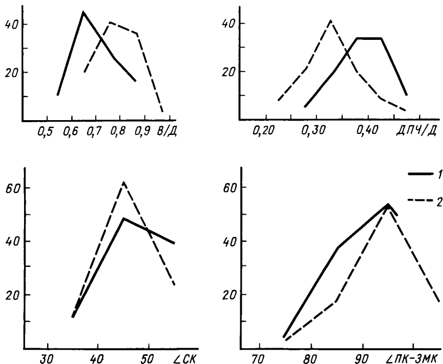
Р и с. 21. Индивидуальная изменчивость Bakevella (Maizuria) varians Kur. из двух выборок оленекского яруса (1 — рч. Менгилех, зона Olenekites spiniplicatus , 2 — р. Ныыкаабыт, зона Dienericeras demokidovi )
