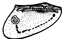
Р и с. 20. Схематический рисунок левой створки bakevella ( Maizuria ) varians Kur. (*2)
