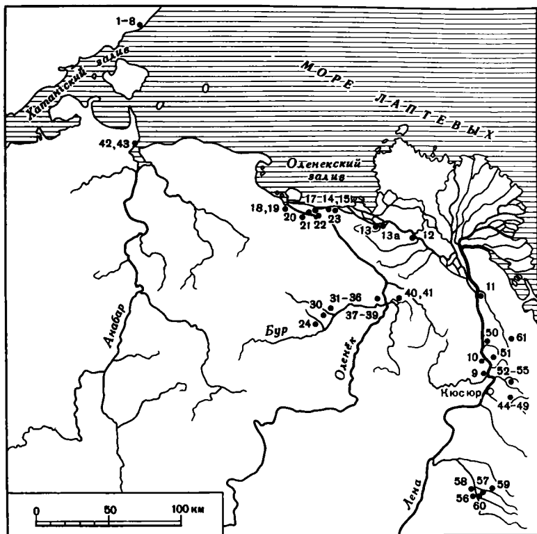
Р и с 1. Обзорная карта местонахождения триасовых брахиопод и двустворчатых моллюсков на севере Средней Сибири
