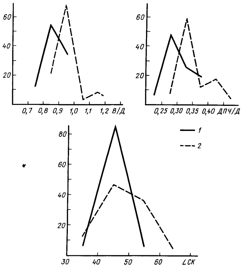
Р и с. 18. Индивидуальная изменчивость Bakevella (Maizuria) arctica (Kipar.) из двух выборок анизийского яруса мыса Цветкова (1 — зона Grambergia taimyrensis , 2 — зона Gymnotoceras rotelliforme )
