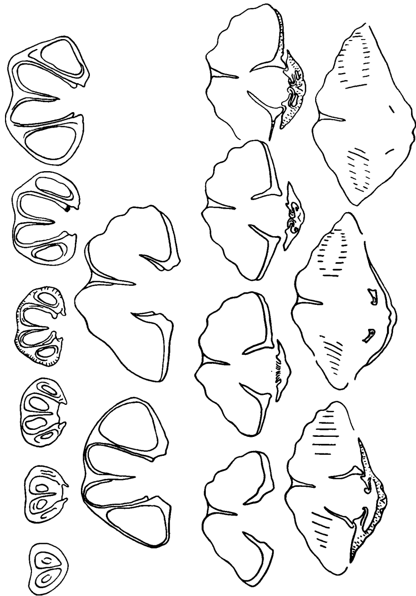
Р и с. 15. Серия поперечных срезов через раковину Costispiriferina taskrestensis sp. nov. Дельта р. Лены, Оленская протока, рч. Таас-Крест; средний аннзий
