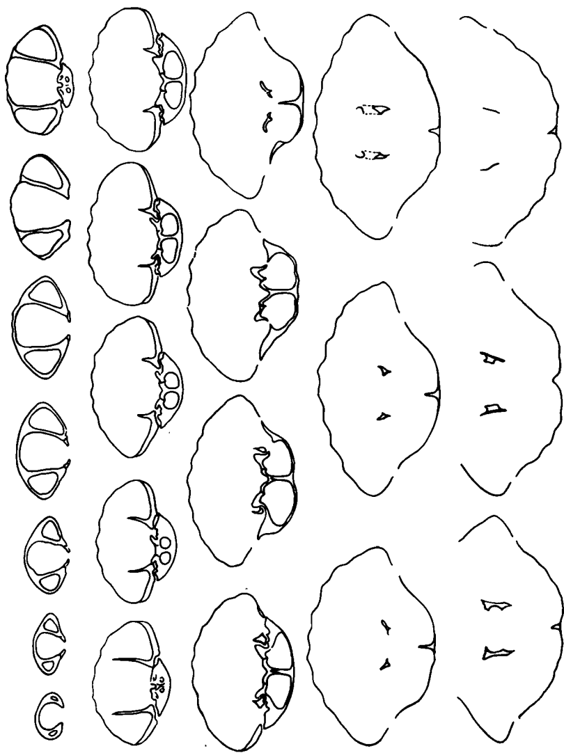
Р и с. 14. Серия поперечных срезов через раковину Sakawaihyunghia olsenkensis Dagus. Восточный Таймыр, мыс Цветкова; карнийский ярус
