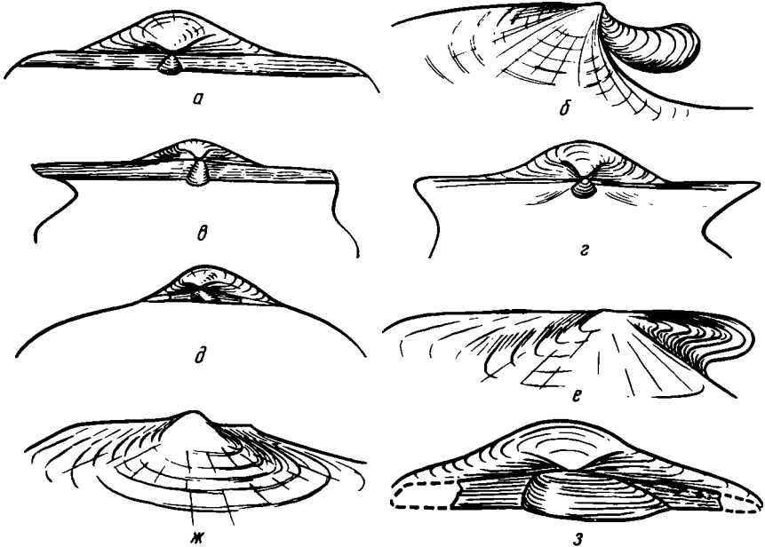
Р и с. 9. Строение замочного аппарата Streblopteria (а), (б — ушко правой створки), Leptochondria (в), Janorecten (г), Otapiria (д), (е — правая створка, ж — левая створка) и Plagiostoma (з)
