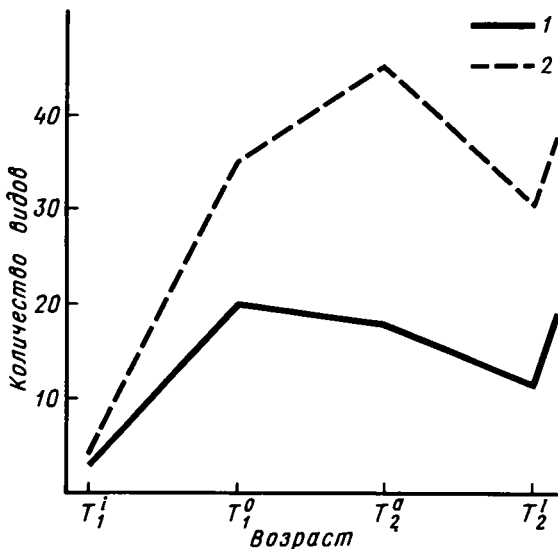
Р и с. 2. Степень изученности среднесибирских двустворчатых моллюсков нижнего и среднего триаса
