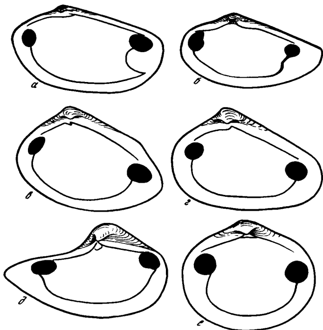
Р и с. 10. Мантийная линия и мускульные отпечатки Malletia (а), Lapteviella (б), Nuculoma (в), Palaeonucula (г), Dacryomya (д) и Sarepta (е)
