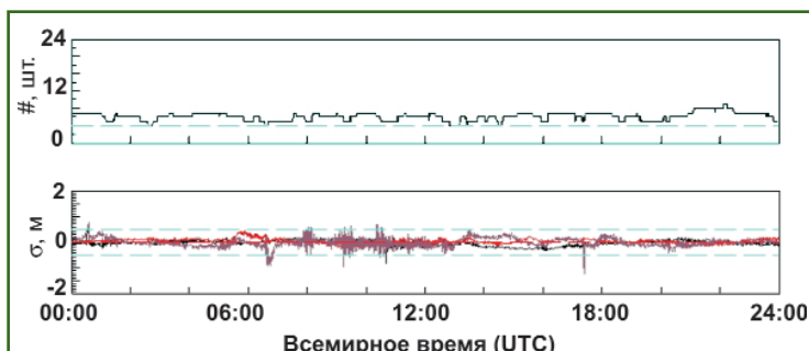
Рис. 7 Результаты точного позиционирования (сервис PPP) с использованием только системы ГЛОНАСС (11 мая 2009 г.)
