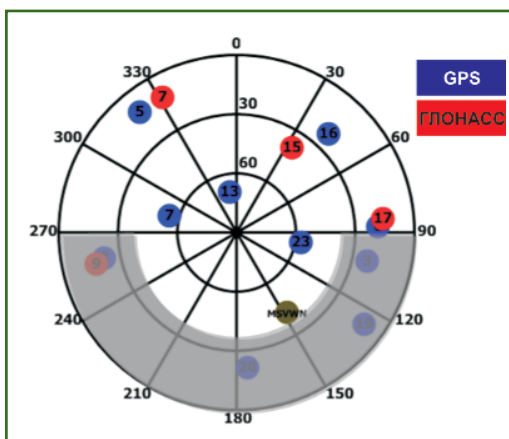
Рис. 9 Модель блокировки спутников GPS и ГЛОНАСС в южном полушарии
