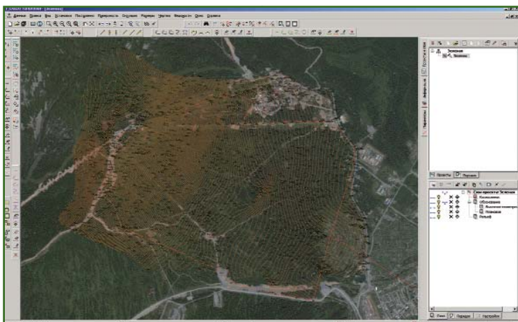
Рис. 5 Сеть планово-высотного обоснования и поверхность рельефа, нанесенные на космический снимок
