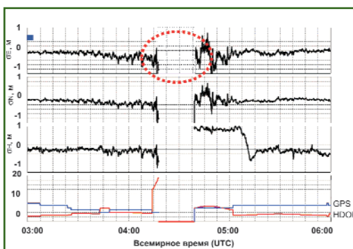
Рис. 10 Результаты позиционирования с помощью GPS при блокировке спутников в южном полушарии
