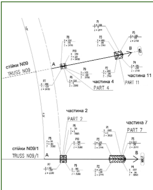
Рис. 8 Базисные линии (А-В)
