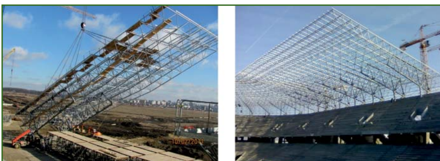
Рис. 9 Установка секции крыши и готовая крыша
