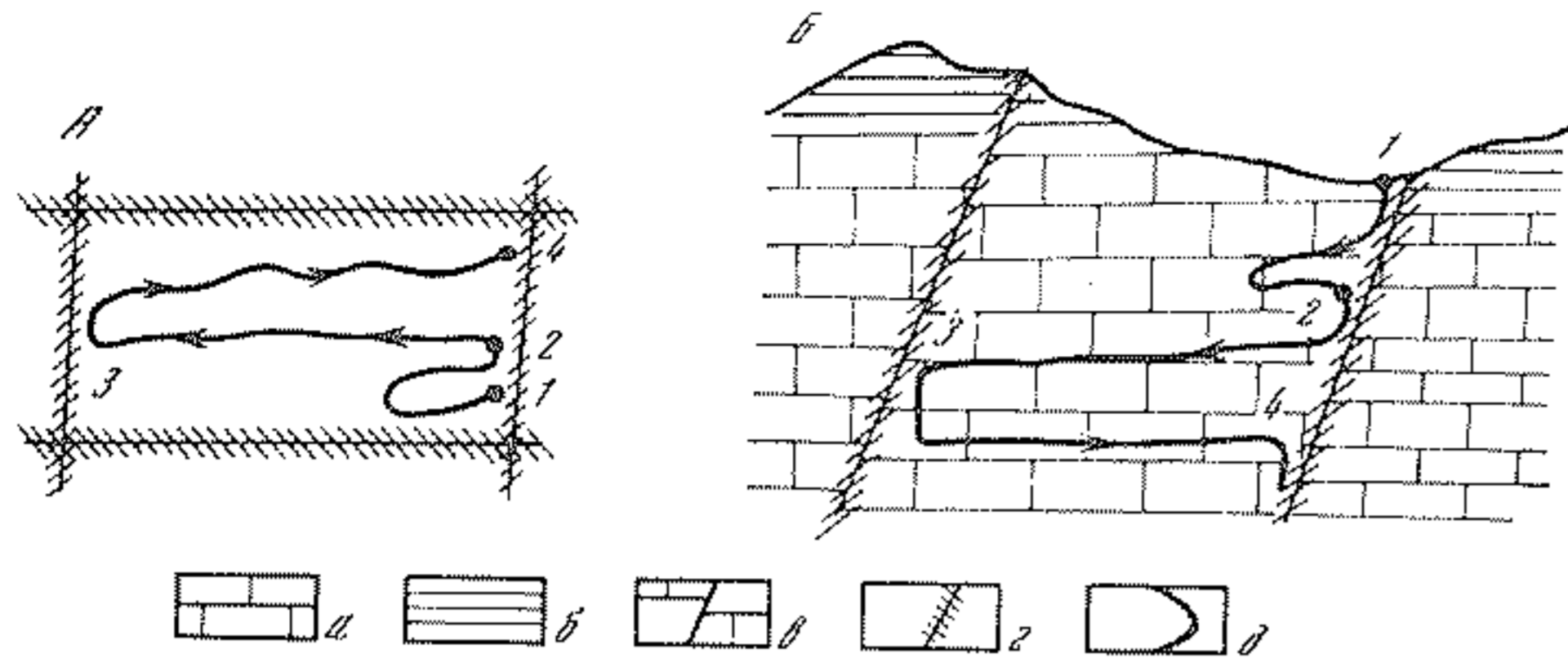
Р и с. 5. Заложение карстовой полости у разрывного нарушения (А — в плане, Б — в разрезе)
