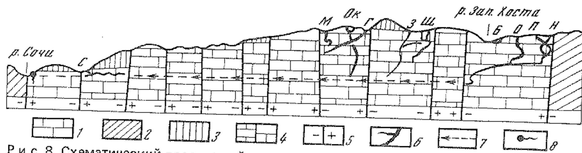
Р и с. 8. Схематический продольный разрез через массив Алек 1 — верхнеюрские известняки; 2, 3 — некарстующиеся породы: 2 — мел-палеогена, 3 — палеогена; 4 — тектонические нарушения; 5 — относительное положение блоков у тектонических нарушений; 6 — карстовые полости; 7 — направления движения подземных вод; 8 — источник на р. Сочи. Шахты-поноры: Н — Назаровская, П — Примусная, О — Осенняя; Б — Барибана; Ш — Школьная; З — Заблудших; Г — Гигантов; Ок — Октябрьская; М — Медвежья. С — пещера-источник Соколова
