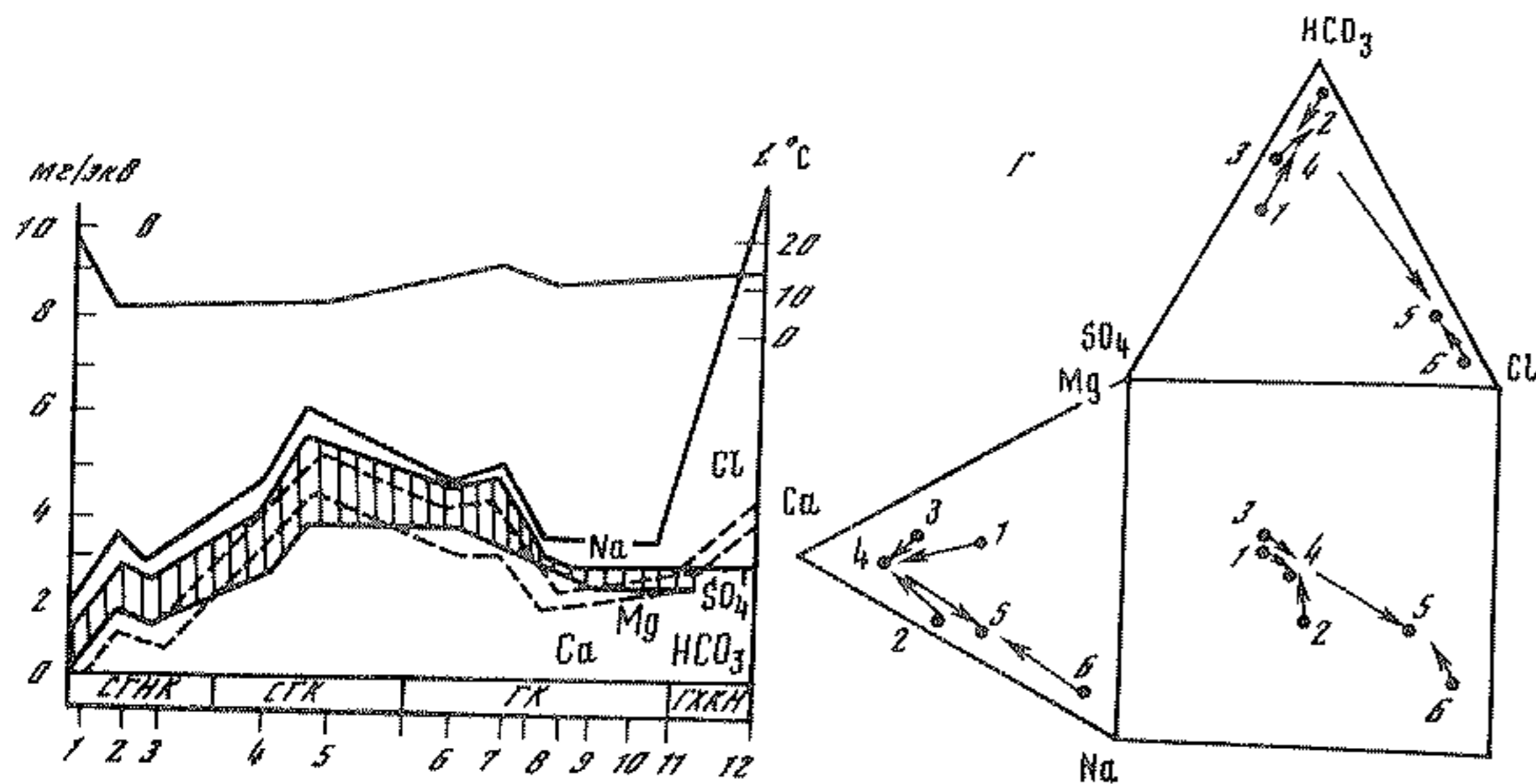
Рис. 24. Метаморфизация карстовых вод вниз по потоку А — Горный Крым, Красная пещера; Б — Западный Кавказ, массив Алек (шахты-поноры: Гф — Географическая, Д — Девичья, Н — Назаровская, О — Октябрьская; С — вскрытая пещера Соколова; цифры у точек — минерализация воды, мг/л); В — Г — Абхазия, Гумишхинский массив; В — изменения химического состава и температуры воды в источниках в сентябре 1974 г. (график Бродского). Водопункты: 1 — дождевые воды; 2—3 — шахта-понор Снежная на глубине 590 и 720 м; 4—7 — поверхностный сток, поглопители; 4 — на р. Аапсте; 5 — на р. Цкваре; 6, 7 — на р. Мсре; 8—10 — Новоафонская пещера; 11—12 — р. Мааниквара: 11 — правобережный вклюд, 12 —
