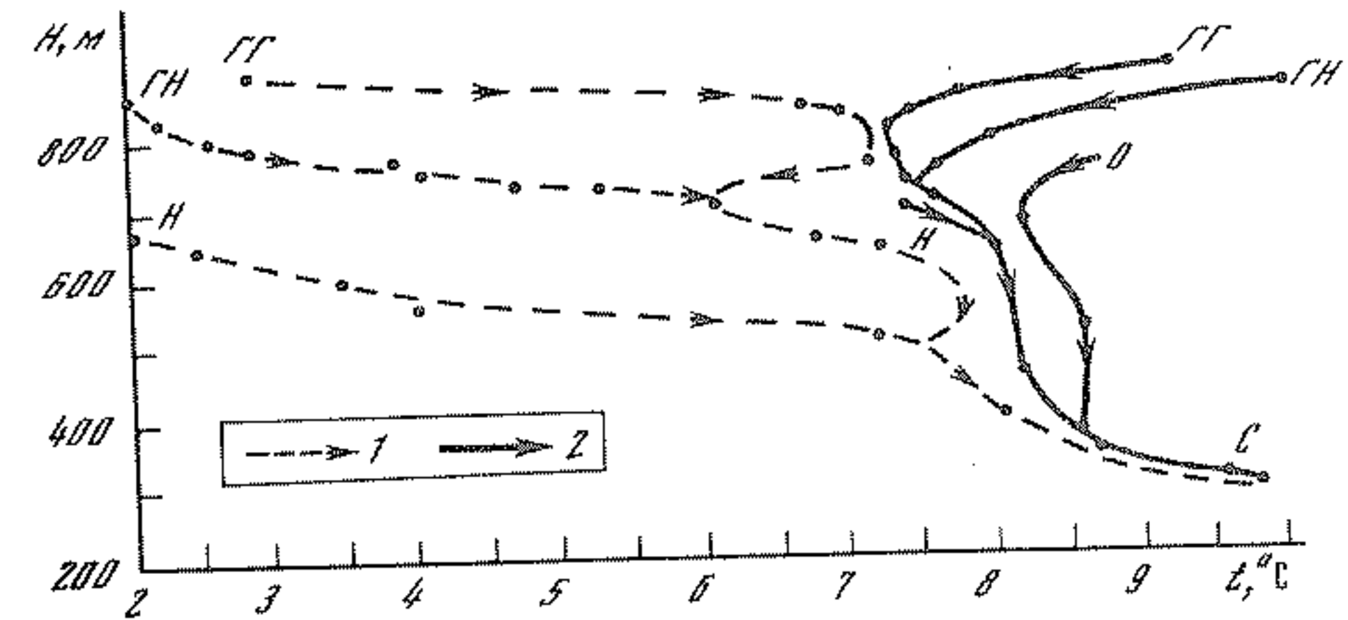
Р и с. 21. Схема формирования температуры подземных потоков массива Алек 1 — холодный период; 2 — теплый период. Шахты и пещеры: ГН — Географическая, Нудный ход; ГГ — Географическая, Главный ход; Н — Назаровская; О — Октябрьская; С — Соколова
