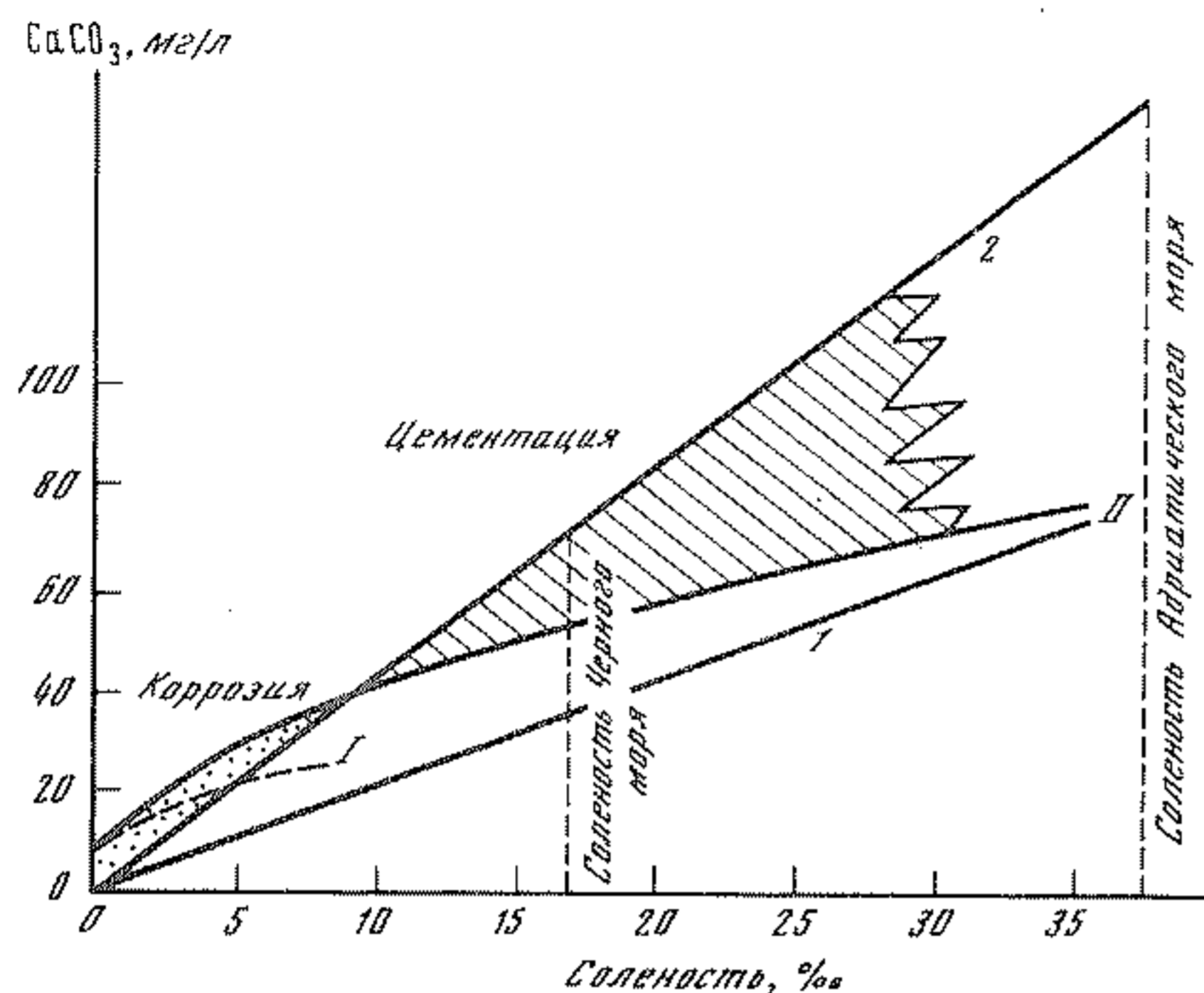
Р и с. 25. Химическая эволюция карстовых вод морских побережий [151] I, II — кривые растворения \text{CaCO}_3 в минерализованной воде: I — по Дебаю—Гюккелю, II — по Эдмонду—Гескесу. 1, 2 — линии смешивания пресных карстовых вод с морскими при насыщении (1) и двукратном пересыщении \text{CaCO}_3 (2)
