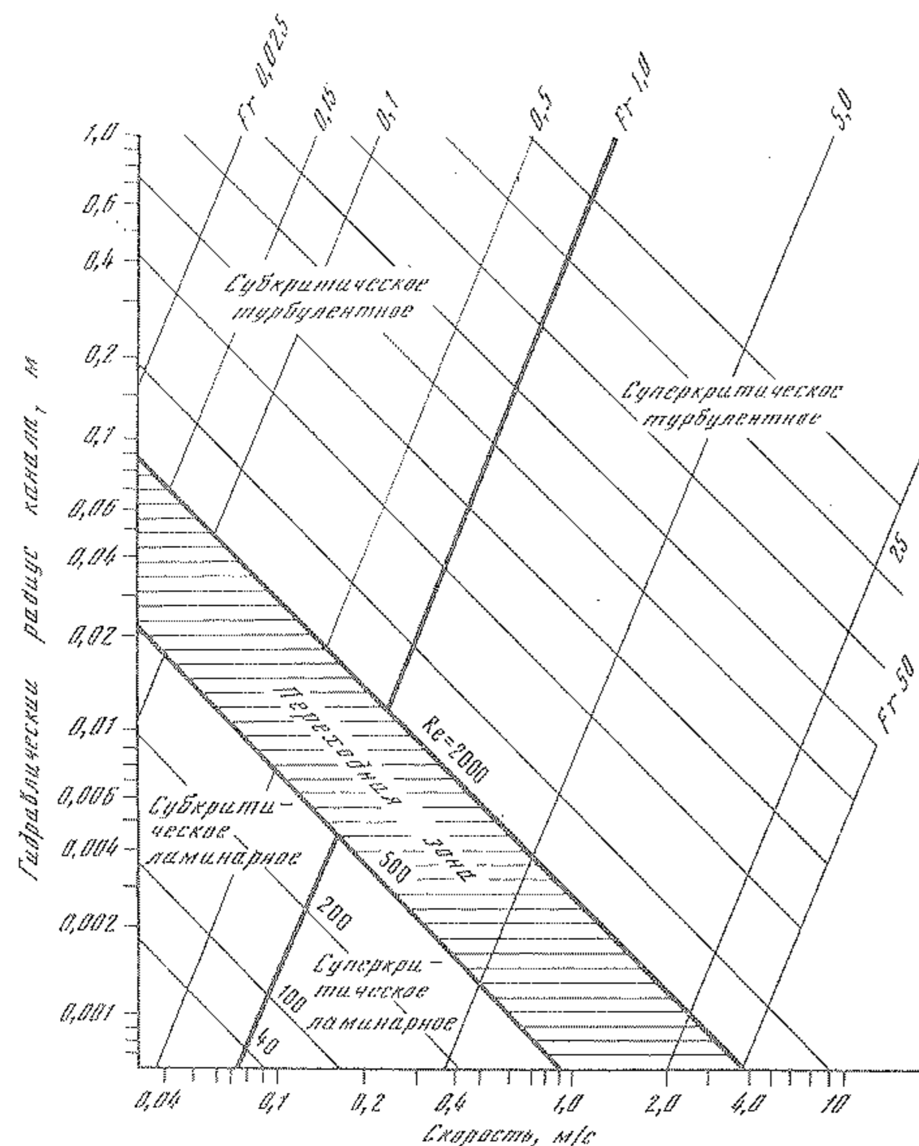
Р и с. 17. Характер движения воды в карстовых каналах при 10°С [108]
