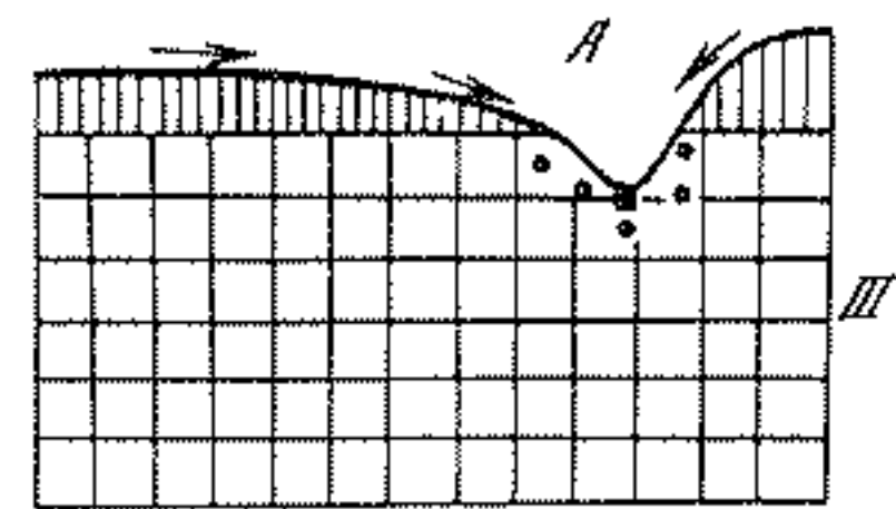
Р и с. 32. Изменения в положении гидродинамических зон в горном массиве при его поднятии
