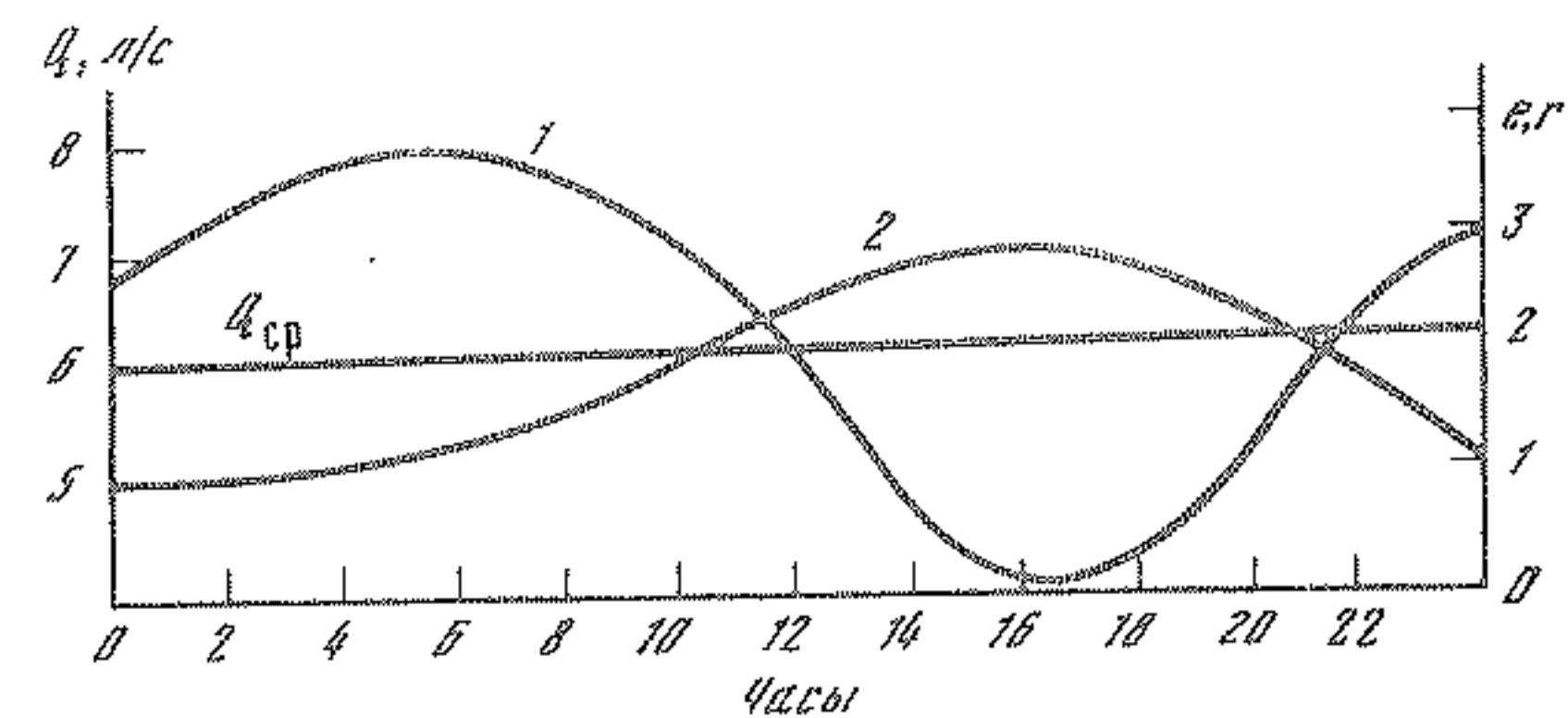
Р и с. 27. Внутрисуточный ход расхода р. Краснопещерной при Q_{ср} = 6 л/с (1) и ход конденсации в зоне аэрации Долгоруковского массива (2)
