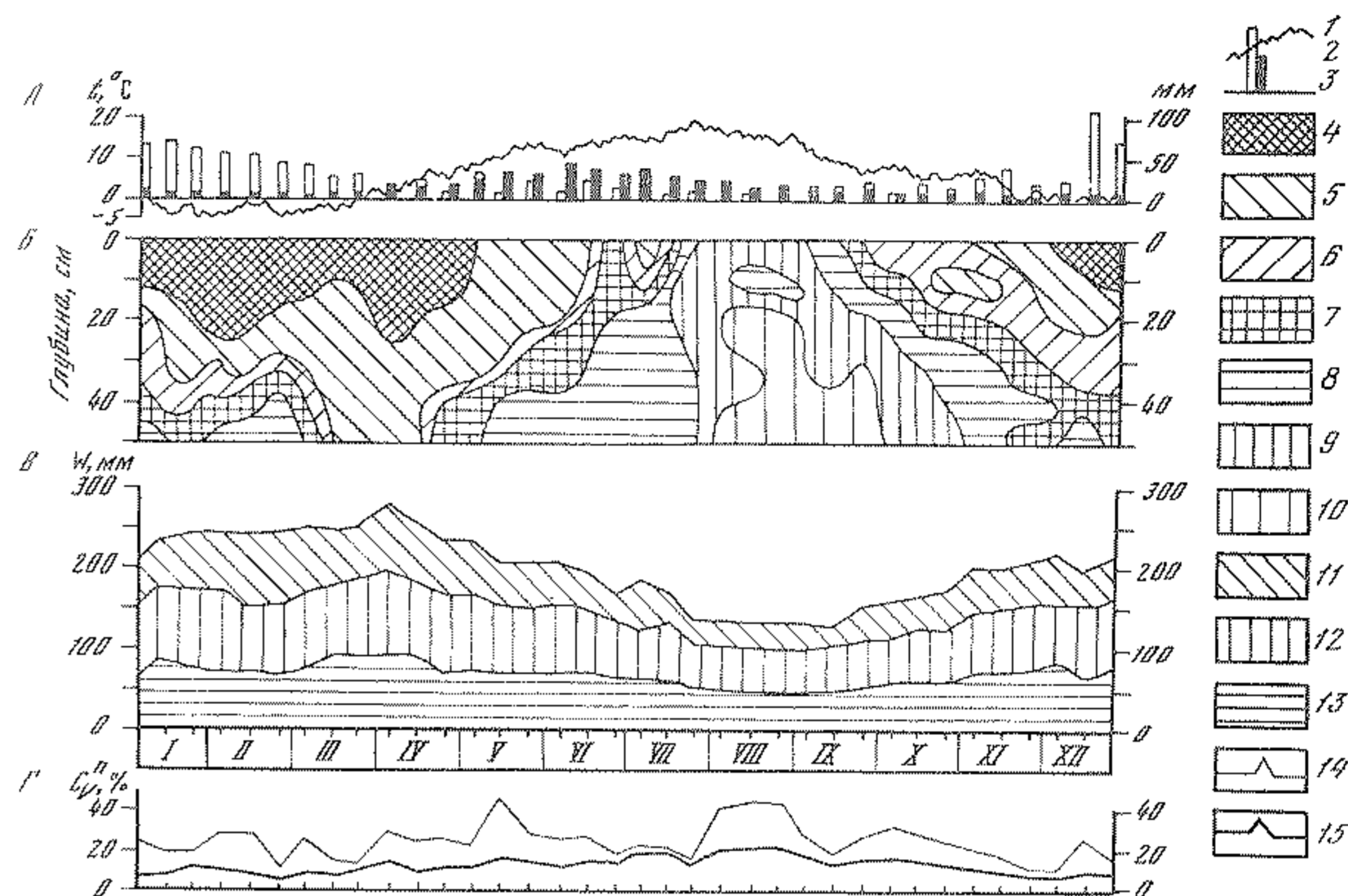
Р и с. 6. Водный режим почво-грунта Ай-Петринского массива (среднедекадные значения за 1957–1964 гг.)
