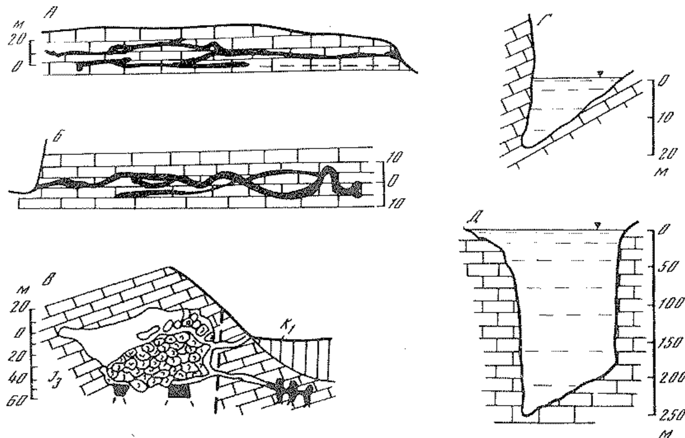
Р и с. 18. Разрезы пещер-источников Альпийской складчатой области юга СССР А — Джур-Джур (Крым); Б — Подземная Хоста (Кавказ, южный склон); В — Скельская (Крым); Г — Голубое озеро (Кавказ, южный склон); Д — Озеро Церик-Кель (Кавказ, северный склон)
