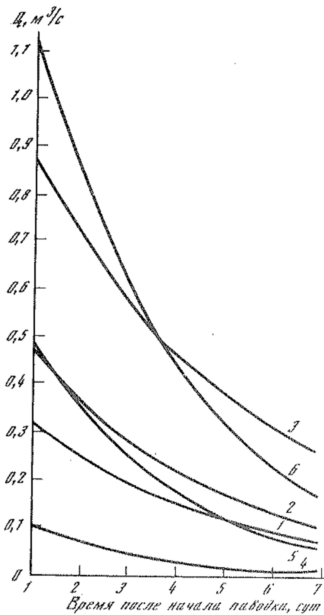
Р и с. 26. Типовые графики спада расхода р. Краснопещерной (рассчитано на ЭВМ) Условия питания: 1 — снеготаяние, 2 — снеготаяние и дождь на протяжении 1 сут, 3 — снеготаяние и дождь на протяжении 2 сут; дождь: 4 — 1–2 дня (менее 30 мм); 5 — 2–4 дня (20–40 мм); 6 — более 4 дней (более 40 мм)
