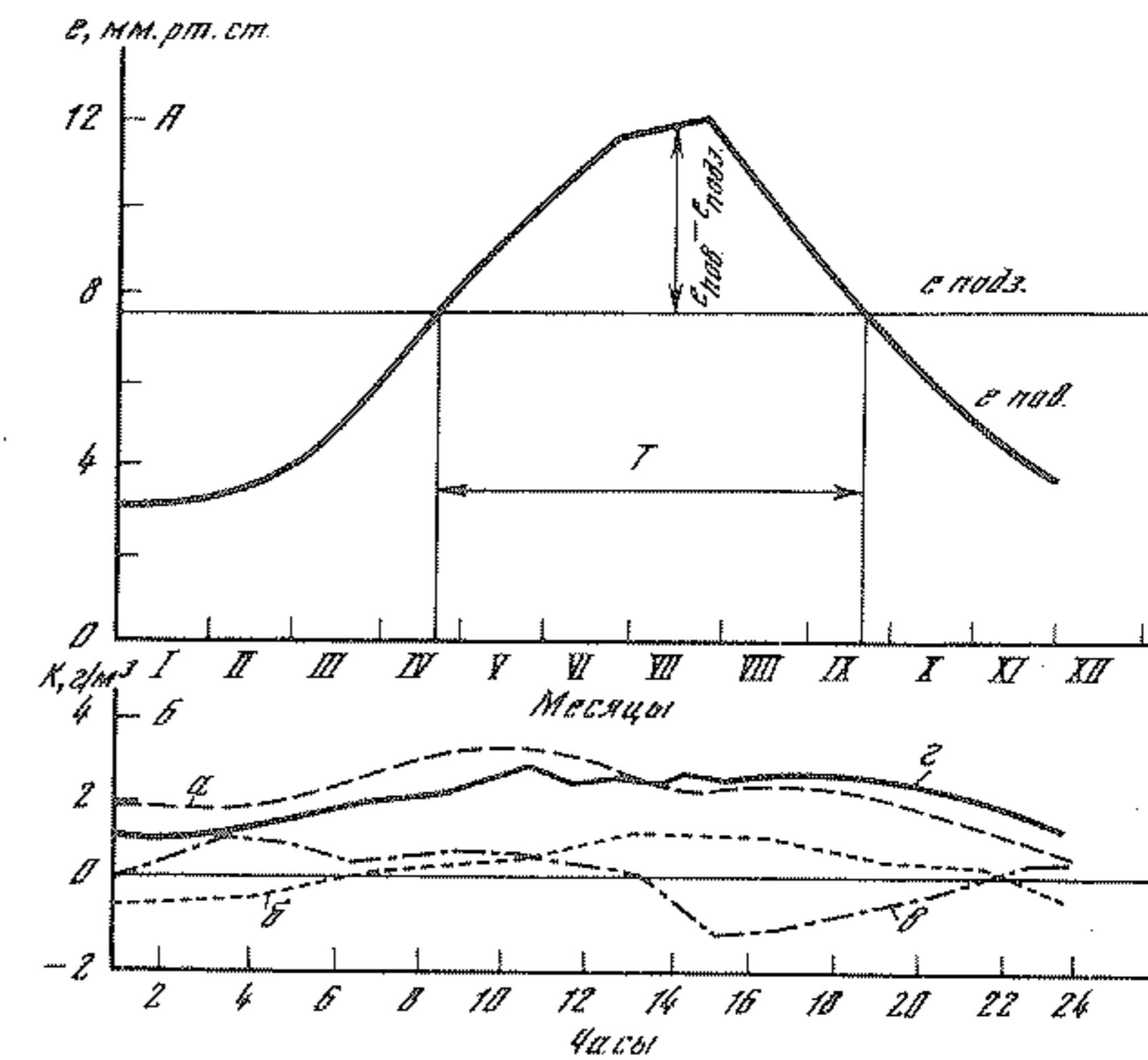
Р и с. 10. Годовой (А) и суточный (Б) ход процессов конденсации
