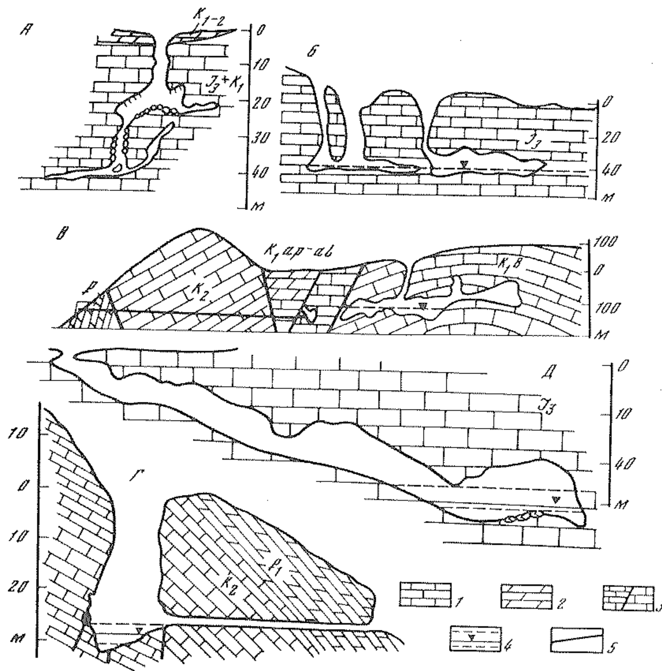
Р и с. 12. Вскрытые пещеры Альпийской складчатой области юга СССР А — Дружба (Восточные Карпаты); Б — реликтовая водоносная система Эгиз-Тинах (Горный Крым); В — Новофонская (Кавказ, южный склон); Г — Провал (Кавказ, северный склон); Д — Бахарденская (Копетдаг) 1 — известняки; 2 — мергели; 3 — тектонические нарушения; 4 — уровни воды и амплитуда их колебаний; 5 — проекция железнодорожного тоннеля
