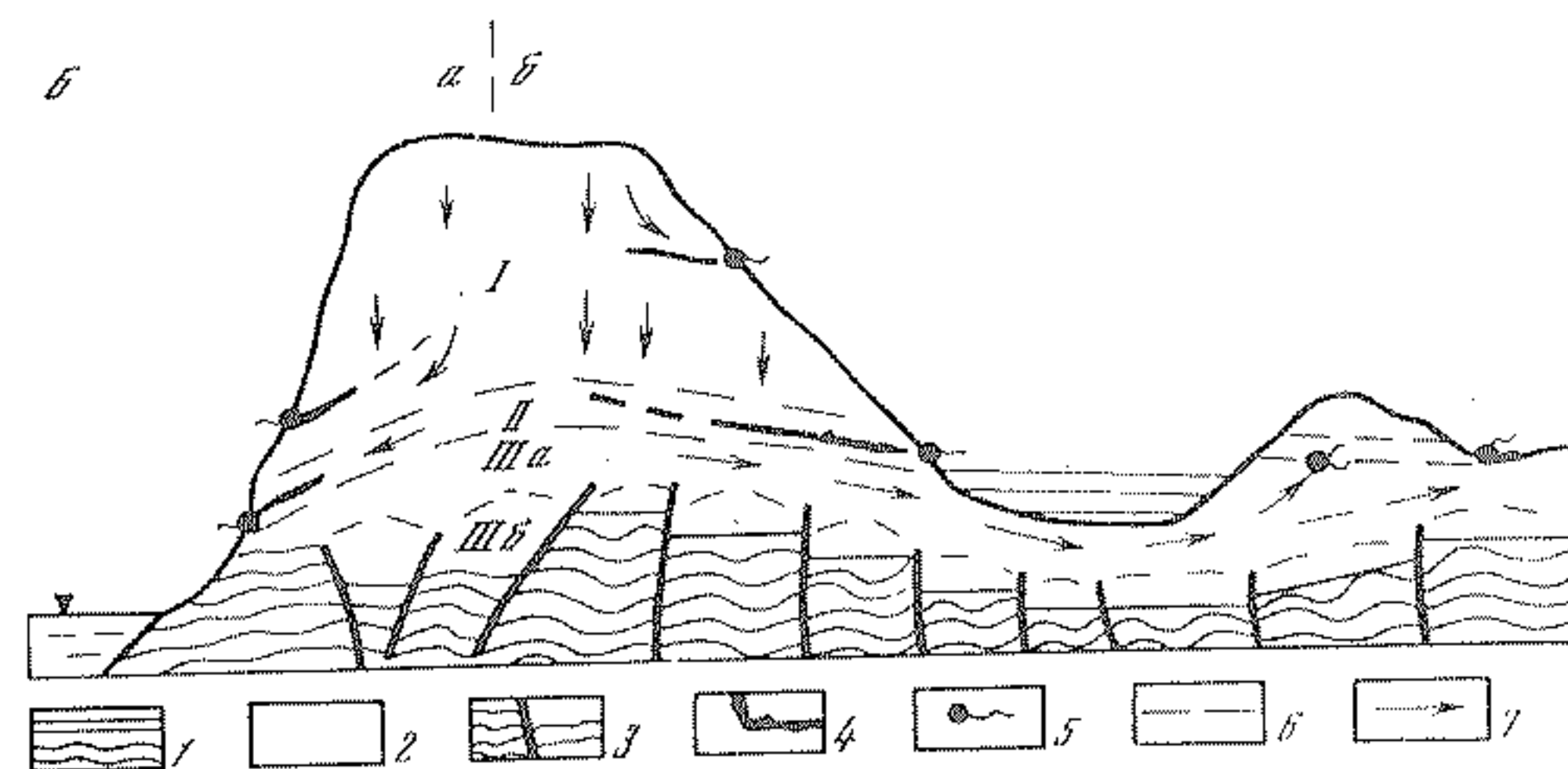
Рис. 11. Схема гидродинамической зональности карстовых вод А — Западная Грузия (по [16]). Гидродинамические зоны: I — гравитационной циркуляции, II — относительно затрудненной циркуляции, III — весьма замедленной циркуляции и относительного застоя, IV — застоя; подзоны: Iа — периодической циркуляции, Iб — подземной вертикальной нисходящей и наклонной циркуляции, Iв — подземной нисходящей наклонной и субгоризонтальной циркуляции, Iг — подземной субгоризонтальной циркуляции, Iд — подземной нисходящей наклонной или субгоризонтальной циркуляции подвешенных водотоков, IIа — подрусловой циркуляции без напора или с относительным напором, IIб — сифонной циркуляции с напором Б — Горный Крым (по [13]). а — цокольные приморские, б — склоновые континентальные массивы. Гидродинамические зоны: I — аэрации, II — сезонных колебаний уровней, III — полного насыщения; подзоны: IIIа — интенсивной фильтрации, IIIб — замедленной фильтрации 1 — водоупорные породы; 2 — карстующиеся породы; 3 — тектонические нарушения; 4 — современные и древние карстовые водоносные системы; 5 — карстовые источники; 6 — границы гидродинамических зон; 7 — направления движения подземных вод
