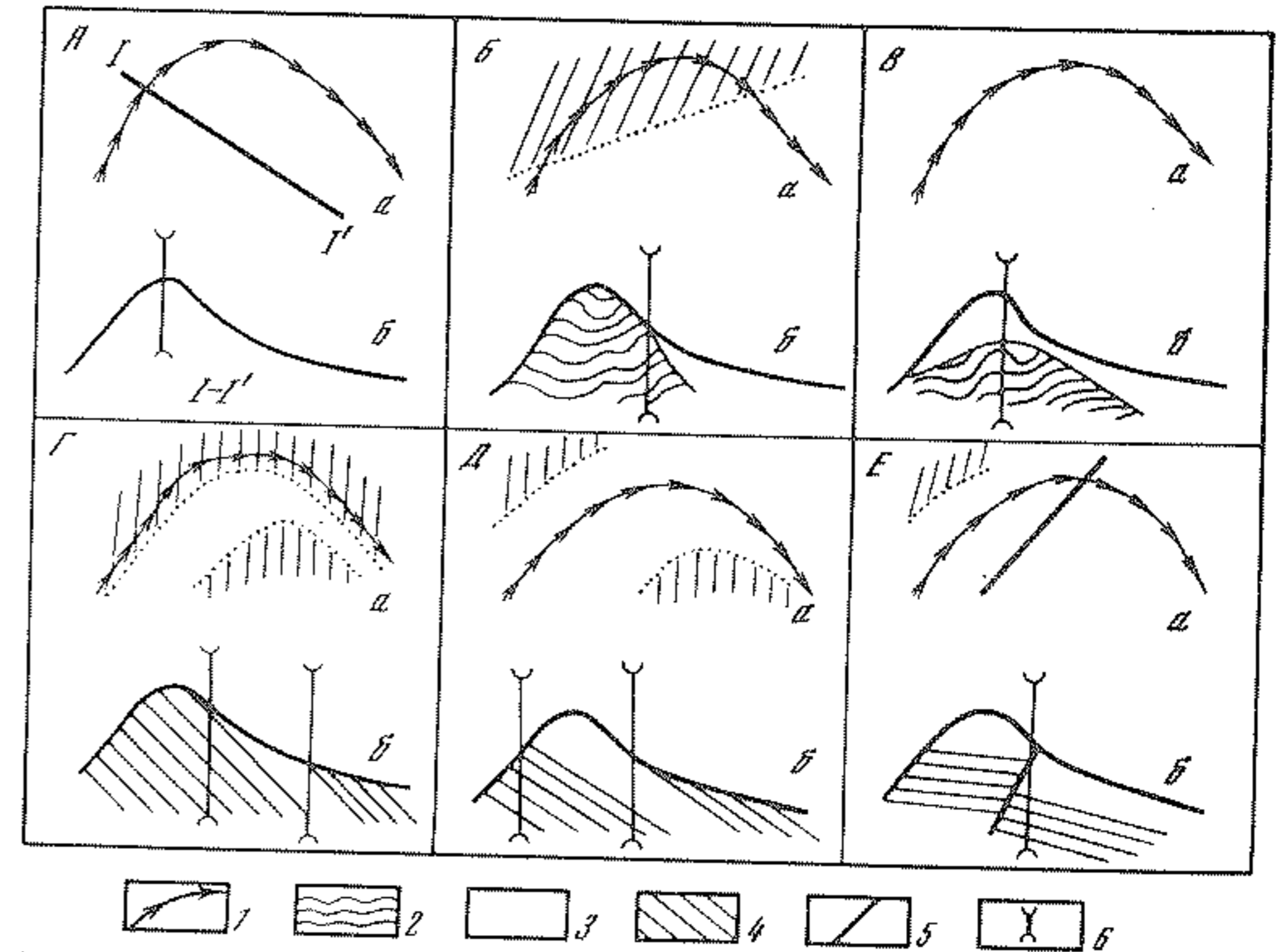
Р и с. 3. Принципы проведения границ гидрогеологических регионов на закарстованных территориях (а — план; б — разрез по линии I—I')
