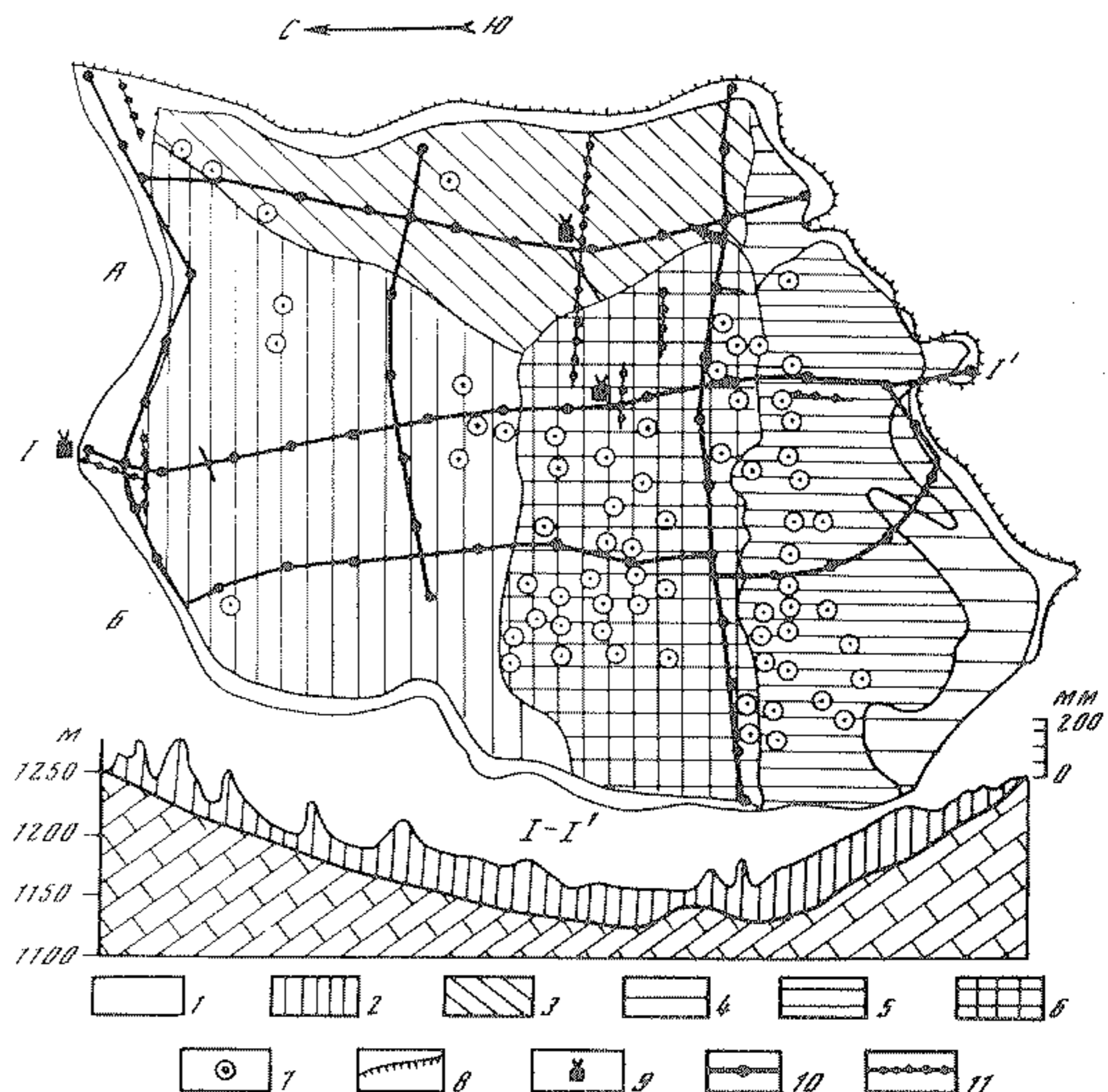
Рис. 7. Расположение снегомерных маршрутов в Приайпетринской котловине
