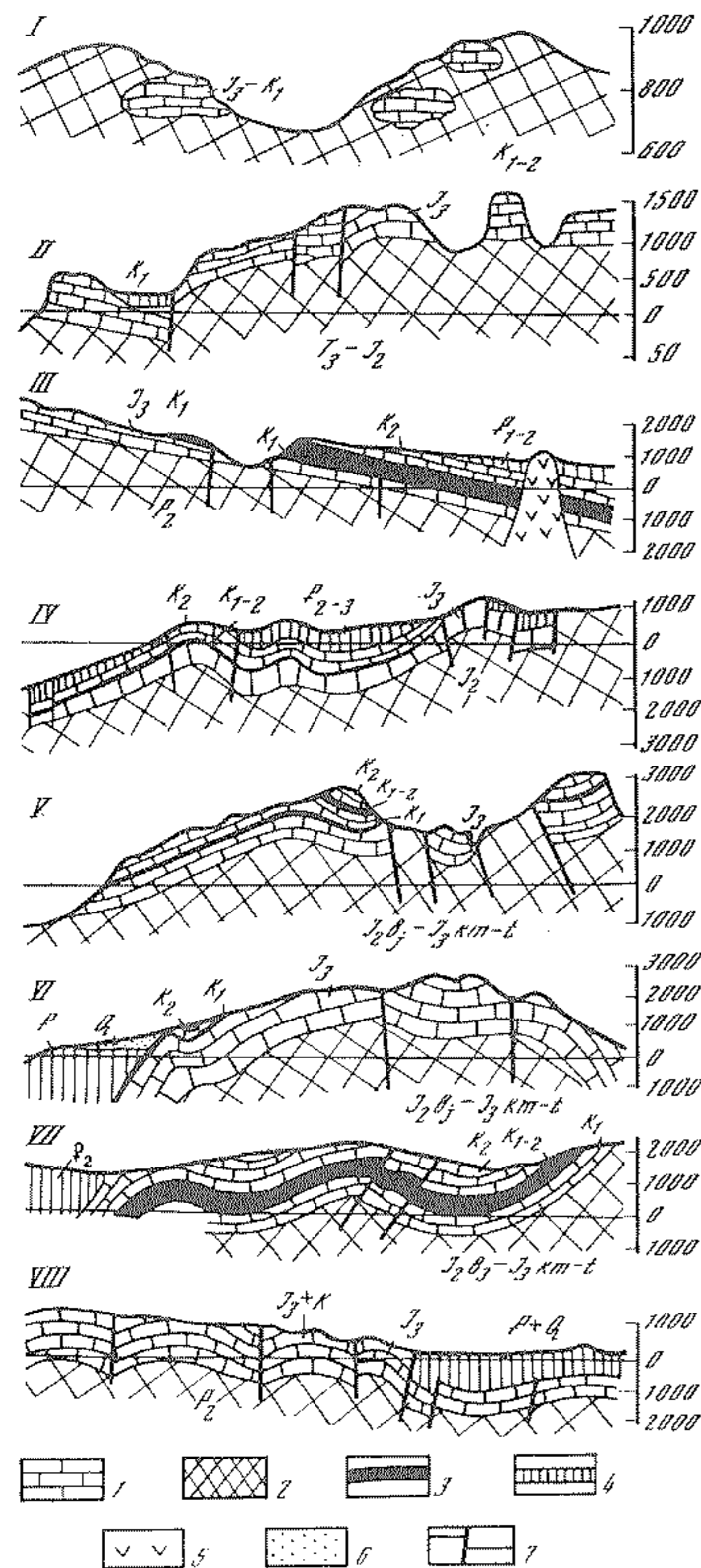
Р и с. 2. Структурно-гидрогеологические условия развития карста в Альпийской складчатой области юга СССР
