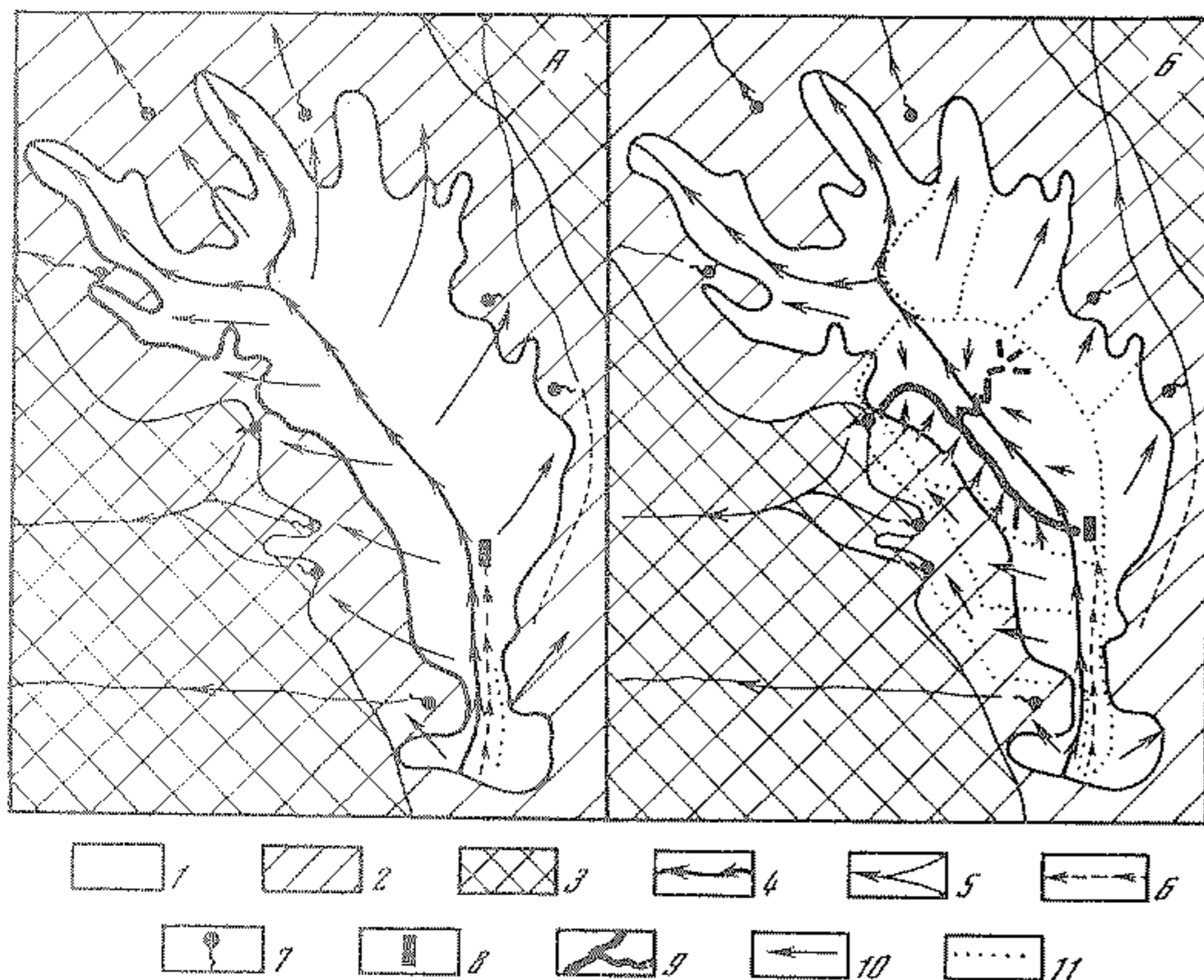
Р и с. 16. Схема движения подземных вод на Долгоруковском массиве (А — по Е.А. Зубровой [104]; Б — по В.Н. Дублянскому [13])
