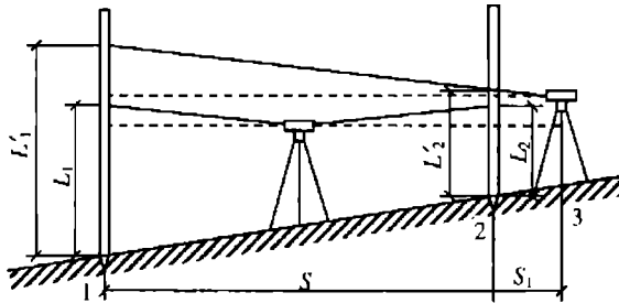
Рис. 4.6. Определение угла i по способу (б) — нивелирование из середины в сочетании с нивелированием вперед
