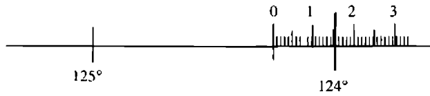
Рис. 3.2. Отсчет по шкаловому микроскопу: O = 124^\circ + 15,4' = 124^\circ 15'24''
