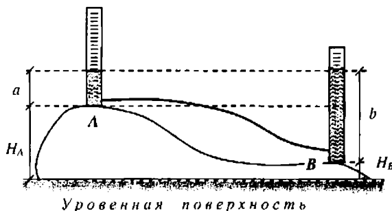
Рис. 4.1. Измерение превышения между точками А и В гидростатическим нивелиром
