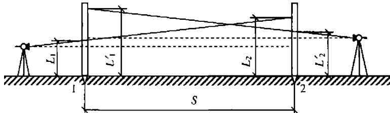
Рис. 4.7. Определение угла i по способу (в): нивелирование с разными плечами
