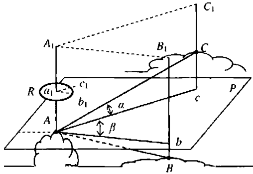
Рис. 3.3. Схема измерения горизонтального угла \beta
