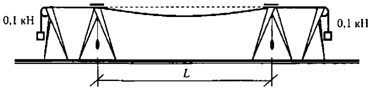
Рис. 2.1. Схема установки подвешенного прибора, подготовленного для снятия отсчета по измерению пролета L
