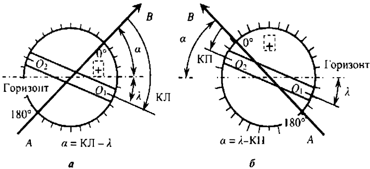
Рис. 3.5. Два положения визирной оси АВ при наведении трубы на точку а а – при «круге лево», б – при «круге право»
