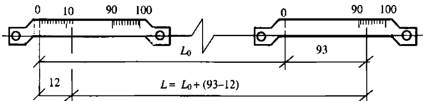
Рис. 2.2. Длина пролета L при одностороннем положении нулевых штрихов (в начале шкал, по ходу измерения)
