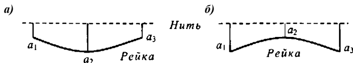
Рис. 4.9. Определение стрелки прогиба рейки
