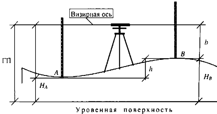
Рис. 4.3. Измерение нивелиром превышения h между точками А и В
