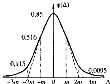
Рис. 5.1. Кривая Гаусса
