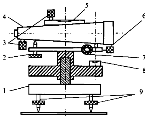
Рис. 4.2. Схема устройства и составные части нивелира: 1 – подставка, 2 – винт элевационный, 3 – винты-шпильки, 4 – зрительная труба, 5 – уровень цилиндрический, 6 – винт закрепительный, 7 – винт наводящий, 8 – уровень круглый, 9 – подъемные винты подставки
