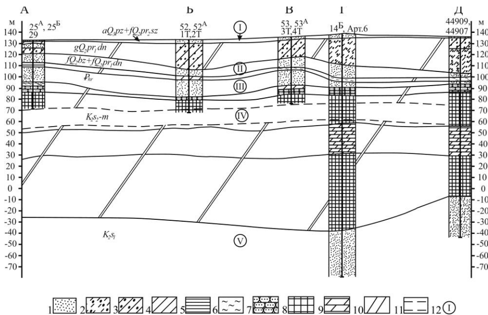
Рис. 2. Схематический геолого-гидрогеологический разрез. Обозначения: 1 – песок, 2 – супесь моренная, 3 – суглинок моренный, 4 – суглинок, 5 – глина, 6 – алеврит, 7 – песчаник, 8 – мел, 9 – мергель, 10 – слабопроницаемые отложения, 11 – ориентировочное положение водоносного горизонта, 12 – водоносные горизонты: I – грунтовый, II – межморенный, III – палеогеновый, IV – нижнемеловой (верхний сеноман-маастрихт), V – нижнемеловой (нижнесеноманский).
