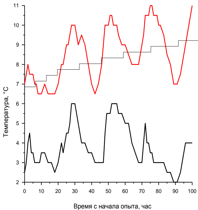
Рис. 1. График изменения температуры при обратной схеме циркуляции и расходе воды 10 \text{ м}^3/\text{час} в СТО, скважина Людвигинская 1Т. Обозначения: Температура воды на входе в кольцевое пространство (нижняя кривая), на выходе из НКТ (верхняя кривая) при работе СТО. Ступенчатой линией отмечена тенденция роста температуры на выходе из СТО.
