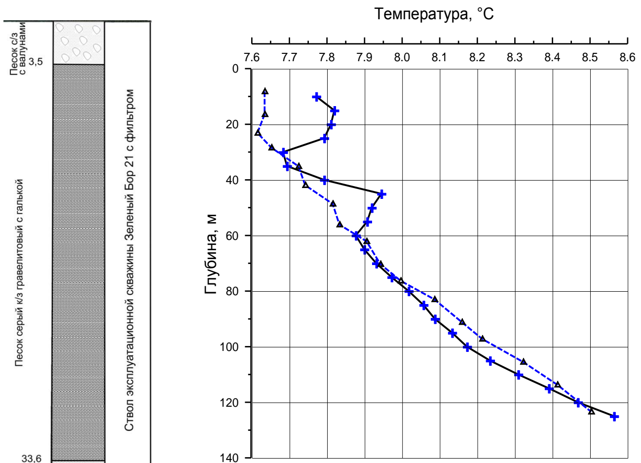
Рис. 2. Термограммы наблюдательной скважины 138 (справа) и геологическая колонка эксплуатационной скважины 21 (слева) водозабора «Зеленый Бор». Точки измерений обозначены: треугольниками (термограмма 1998 г. терморезистор) и крестиками (термограмма май 2013 г. цифровой) термометры.
