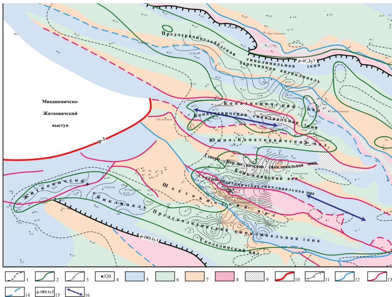
Рис. 1. Схематическая структурная карта по подошве калийного горизонта IV-п юго-западной части центральной зоны Припятского прогиба (совмещена со схемой структурного районирования межсолевого комплекса)
