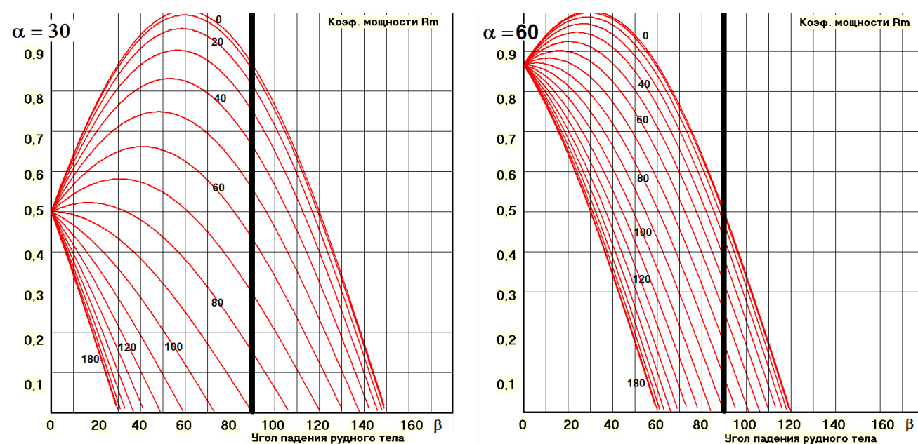
Рис. 2. Номограммы определения коэффициента мощности R_m для углов наклона скважины 30^\circ (слева) и 60^\circ (справа). Значения угла \gamma между горизонтальной проекцией скважины и направлением падения рудного пласта указаны на линиях номограмм
