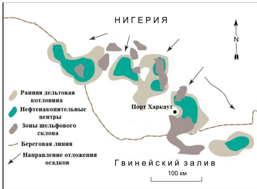
Рис. 1. Схематическое изображение местонахождения котловин ранней дельты Нигера, центров нефтеаккумуляции и зоны шельфового склона [Bustin, 1988]
