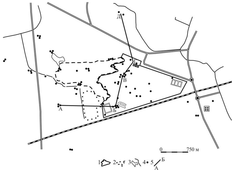
Рис. 1. Схема сети мониторинга подземных вод Гомельского химического завода. Обозначения: 1 – производственная зона ОАО «Гомельский химический завод», 2 – контуры размещения отходов производства, 3 – водоемы и водотоки, 4 – скважины режимной сети мониторинга, 5 – линия геолого-гидрогеологического разреза.
