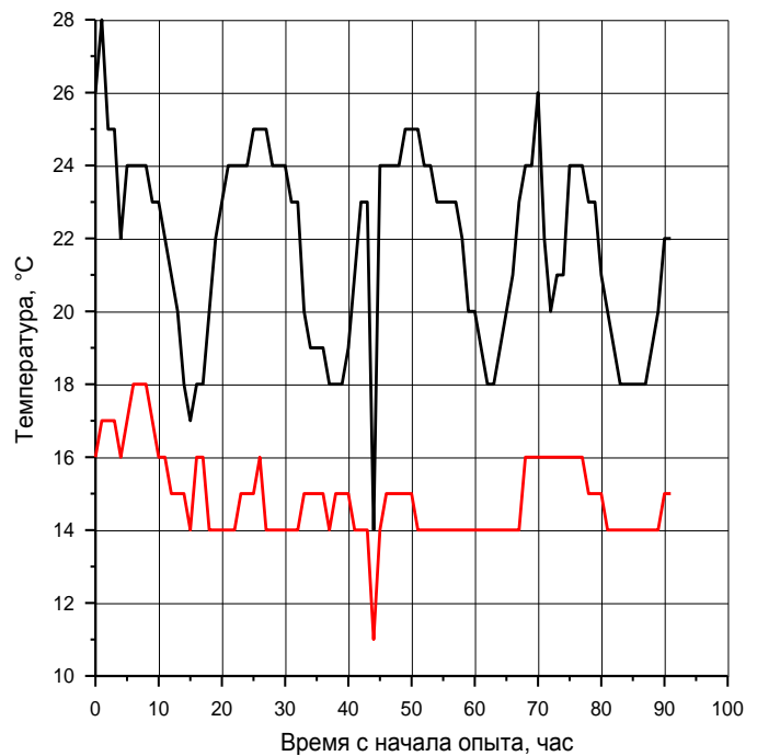
Рис. 2. Изменение температуры при расходе воды 20 \text{ м}^3/\text{час} и обратной схеме циркуляции в СТО скважины Ново-Ельская 43Т. Обозначения: Температура воды на входе в кольцевое пространство СТО верхняя кривая; на выходе из НКТ – нижняя кривая при ее прокачке через СТО.
