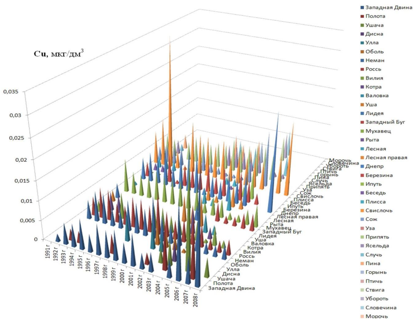
Рис. 1. Распределение растворённого Си в водах рек Беларуси в период 1991-2008 гг. (среднегодовое), мкг/дм 3 (составлено по данным [Состояние..., 1992, 1993, 1995а, 1995б, 1996, 1997, 1998, 1999, 2000, 2001, 2002, 2003, 2005, 2006, 2007, 2008])
