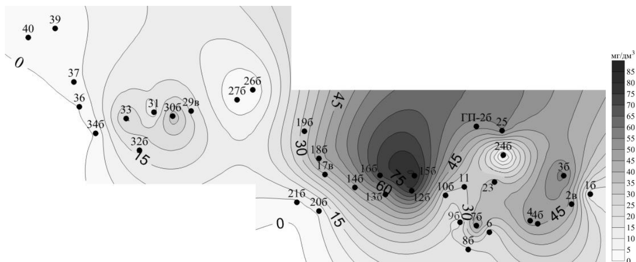
Рис. 1. Карта-схема распространения нитратов ( \text{NO}_3^- ) в водах днепровско-сожского водно-ледникового горизонта на водозаборе «Новинки» (составлена автором по материалам Государственного предприятия «НПЦ по геологии»)
