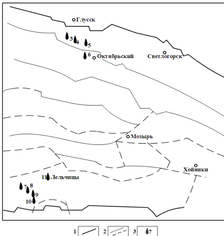
Рис. 1. Схема расположения рудопроявлений урана в юго-западной части Припятского прогиба (Масштаб 1:1 000 000). Условные обозначения: 1 – разломы, проникающие в чехол и ограничивающие Припятский прогиб; 2 – прочие разломы, проникающие в чехол; 3 - рудопроявления урана (3 – Малиновское; 4 – Заречное; 5 – Журавлиное; 6 - Октябрьское; 7 – Боровое; 8 – Юбилейное; 9 – Калиновское; 10 – Болотницкое; 11 – Лельчицкое).
