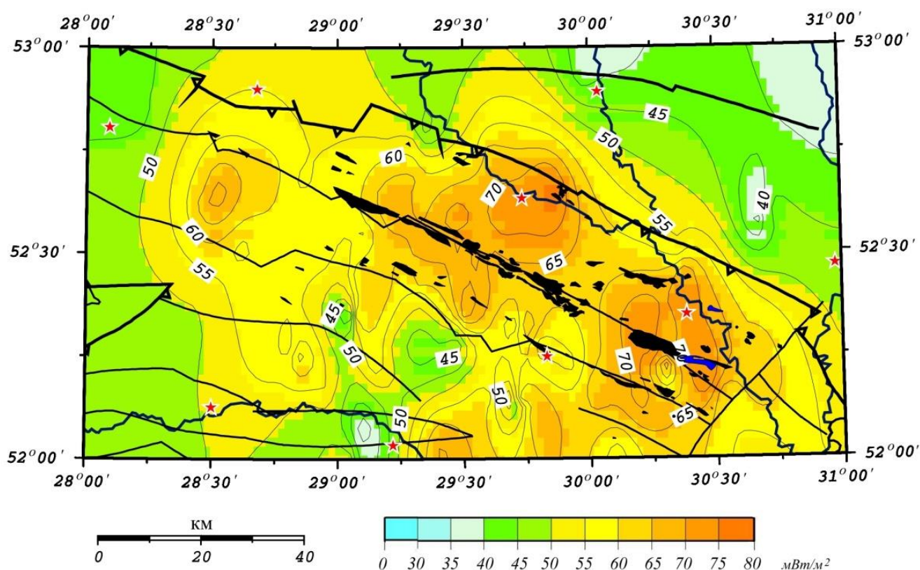
Рис. 3. Положение залежей углеводородов в Припятском прогибе на фоне распределения плотности теплового потока ( \text{мВт}/\text{м}^2 ) [Зуй, 2013].
