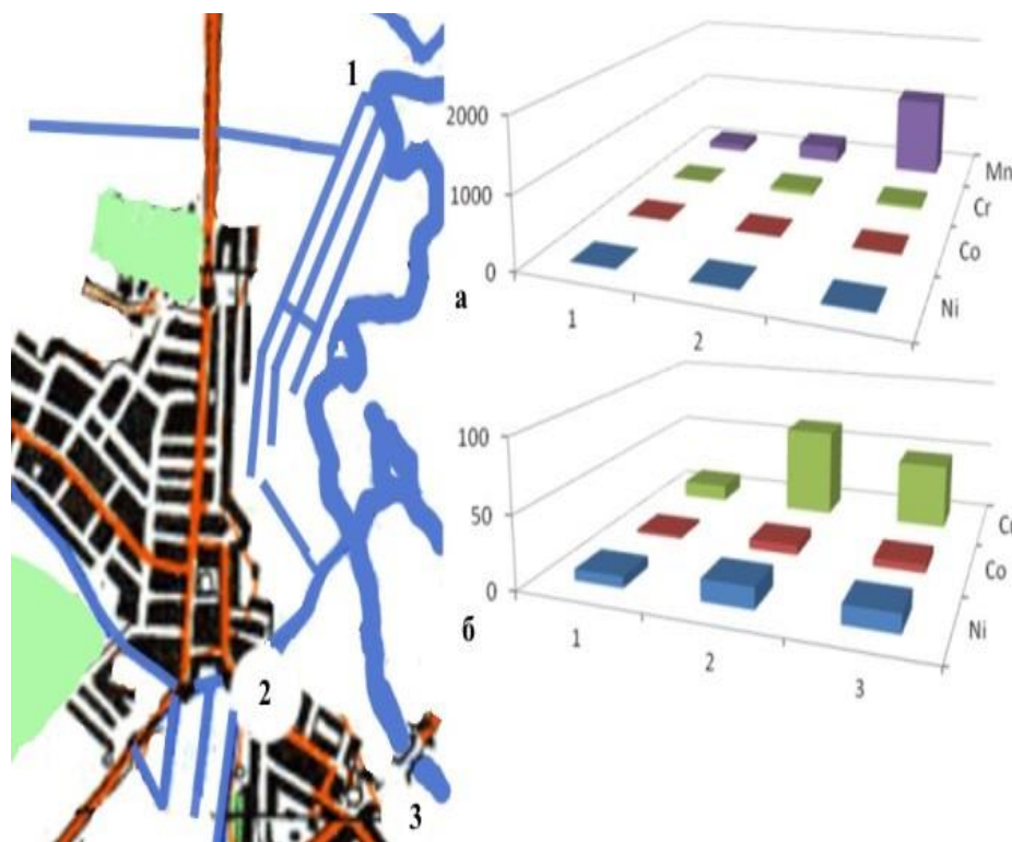
Рис. 1. Территория изучаемого региона (слева) и валовое содержание Mn, Ni, Co и Cr в донных отложениях р. Птичь и её притоков в п.г.т. Глуск, мг/кг сухого вещества (справа). Обозначения: 1 - р. Птичь ниже д. Калатичи, 2 - приток р. Птичь, техногенный ил, п. г. т. Глуск, 3 - р. Птичь ниже п. г. т. Глуск.
