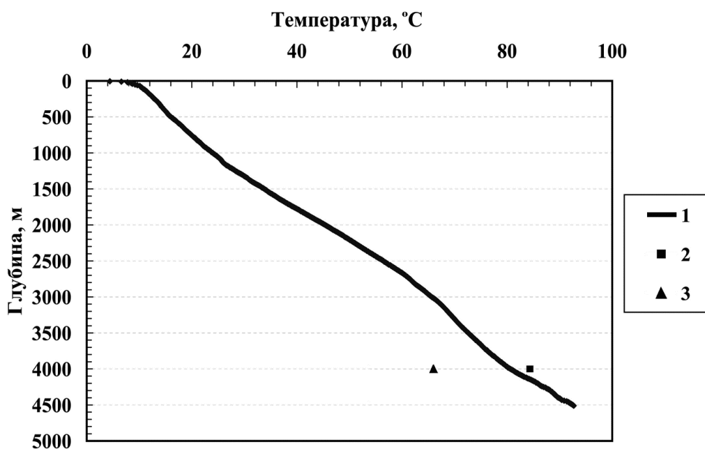
Рис. 1. Проверка предложенного метода расчета глубинных температур. \Обозначения: 1 — термограмма скважины Леузинская-1; 2 — температура на глубине 4000 м, рассчитанная по исправленному на влияние палеоклимата значению плотности теплового потока (50 мВт/м 2 ); 3 —
