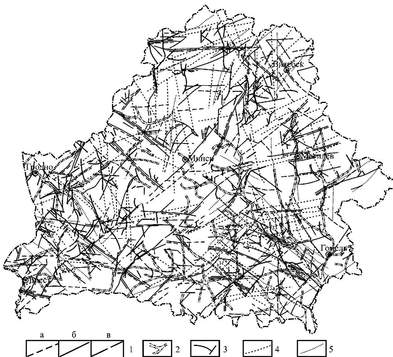
Рис. 1 – Геоактивные зоны на территории Беларуси:
