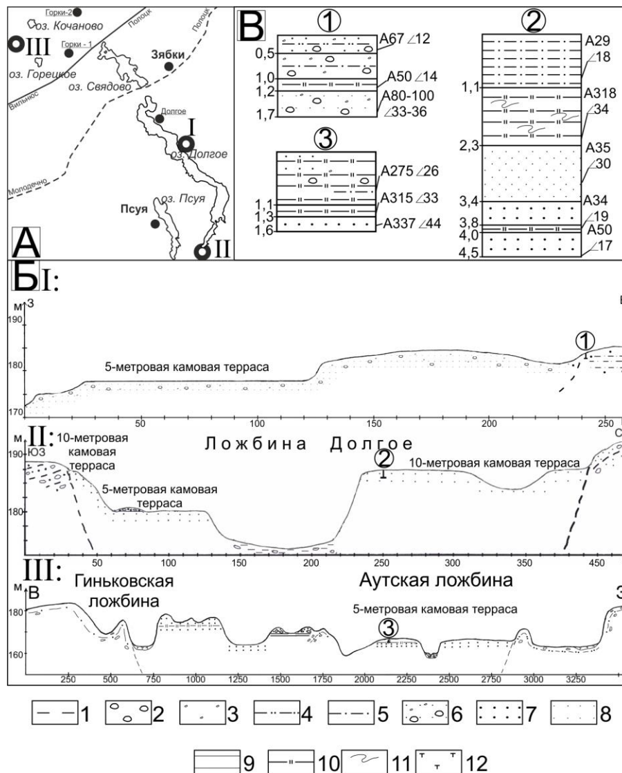
Рис. 1. Расположение и структура камовых террас в пределах ледниковой ложбины оз. Долгое и Аутской ледниковой ложбины: А – схема расположения камовых террас; Б – геолого-геоморфологические поперечные профили: I – восточного склона ложбины Долгое; II – южной части ложбины Долгое; III – Аутской ложбины, В – геологические разрезы камовых террас; 1 – граница бортов ложбин; 2 – гравий и мелкие валуны; 3 – галька; 4 – суглинок; 5 – супесь; 6 – песчано-гравийная смесь; 7 – песок мелкозернистый; 8 – песок тонкозернистый; 9 – глина; 10 – алеврит; 11 – знаки ряби; 12 – торф; элементы залегания: 337^\circ \angle 44^\circ – азимут простирания и угол падения слоев. Цифрами 1-3 в кружках на врезках Б и В показаны геологические обнажения террас.
