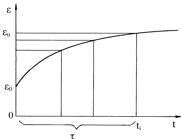
Рис. 5.10. Процесс деформирования твердого тела, имеющего предысторию
