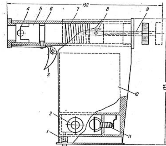
Рис. 4.42. Прибор Вильямса для испытания прочности бетона: 1 – выключатель; 2 – микрошкала; 3 – спусковой крючок; 4 – стальной шарик; 5 – боек; 6 – ствол; 7 – пружина; 8 – указатель; 9 – винт; Рис. 4.42. Прибор Вильямса для испытания прочности бетона: 1 – выключатель; 2 – микрошкала; 3 – спусковой крючок; 4 – стальной шарик; 5 – боек; 6 – ствол; 7 – пружина; 8 – указатель; 9 – винт; 10 – батарея; 11 – электрическая лампочка
