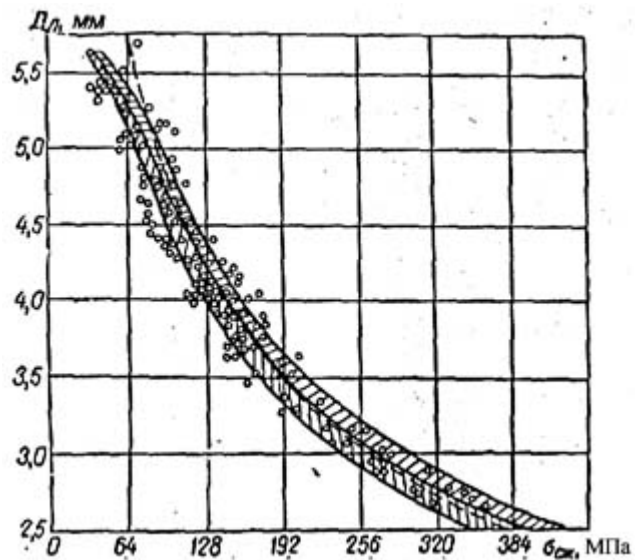
Рис. 4.43. Кривая зависимости между прочностью бетона на сжатие и диаметром лунок при оценке прочности с помощью пружинного пистолета
