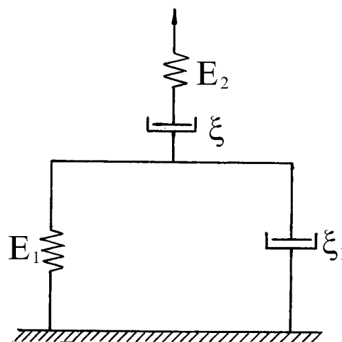
Рис. 5.9. Модель Бюргерса или компаунд-
