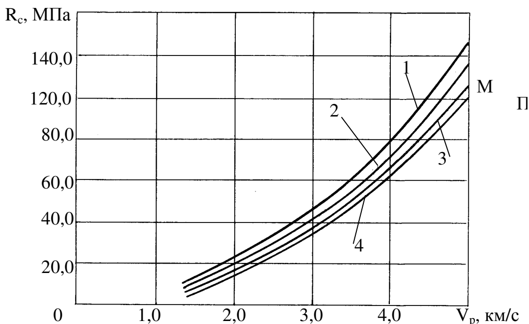
Рис.8.13. Связь акустических и прочностных свойств для алевролитов (1 – R_c=59,6 V_p^2 ; 2 – R_c=52,0 V_p^2 ; 3 – R_c=48,9 V_p^2 ; 4 – R_c=47,1 V_p^2 ).
