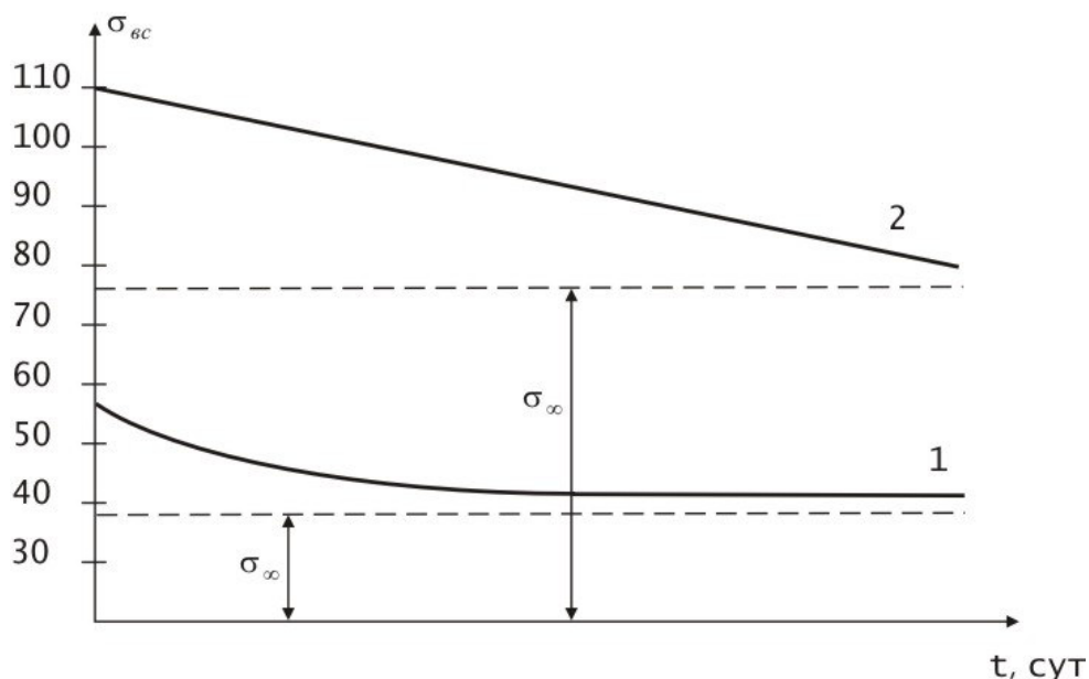
Рис. 4.17. Кривые длительной прочности песчанистого сланца Донбасса (1) и известняка (2)
