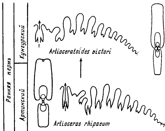
Рис. 17. Филогенетические связи в подсемействе Artioceratinae
