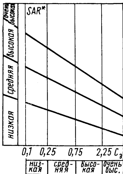
Рис. 61. Диаграмма для определения качества оросительной воды в зависимости от SAR^* и удельной электропроводности C_s в мСм; 1 \text{ мСм} = 10^{-3} (\text{Ом} \cdot \text{см})^{-1} [32]
