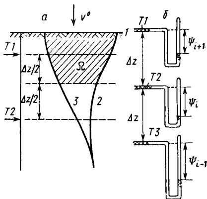
Рис. 68. Схема опыта для определения параметров влагопереноса:
