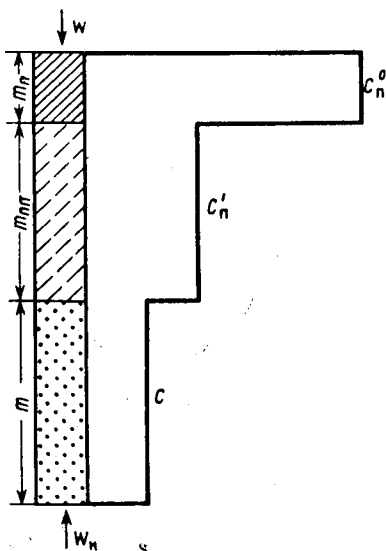
Рис. 58. Выделение зон (почвенной, подпочвенного покрова и водоносного пласта) с эпюрой исходной минерализации почвенных и грунтовых вод
