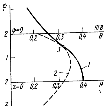
Рис. 72. График для определения водораздельного сечения восходящего и нисходящего влагопереносов (1 — кривая зависимости \psi(\theta) , 2 — замеренная кривая распределения влажности по высоте, 3 — водораздельная точка)
