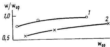
Рис. 32. Относительное ирригационное питание при различной удельной водоподаче оросительной воды w_{ор} в л/(с·га) при зимних (1) и летних (2) промывках [2]
