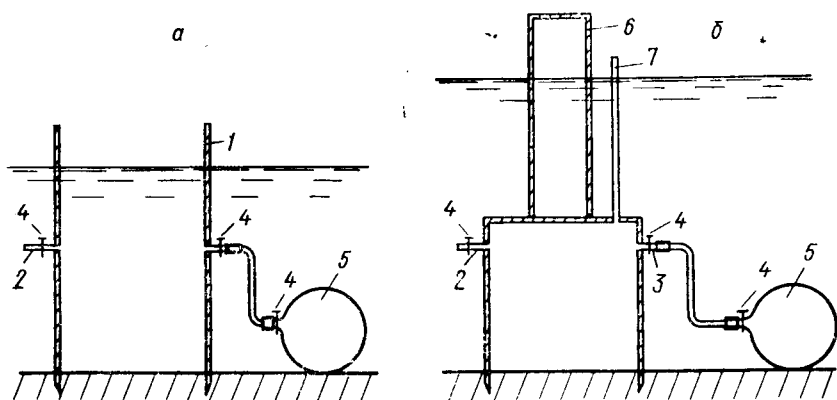
Рис. 84. Фильтромеры закрытого типа (по И. С. Теплицкому): а и б — для водотоков небольшой (а) и значительной (б) глубины (1 — задавливаемый стакан, 2 и 3 — патрубки, 4 — краны, 5 — резиновая камера, 6 — штанга, 7 — выводная трубка)
