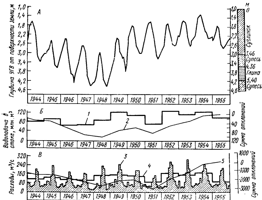
Рис. 27. Многолетние колебания уровня грунтовых вод при резко изменяющейся водоподаче на орошение. Субаральная дельта р. Зеравшана в Бухарском оазисе (по Д. М. Кацу):
