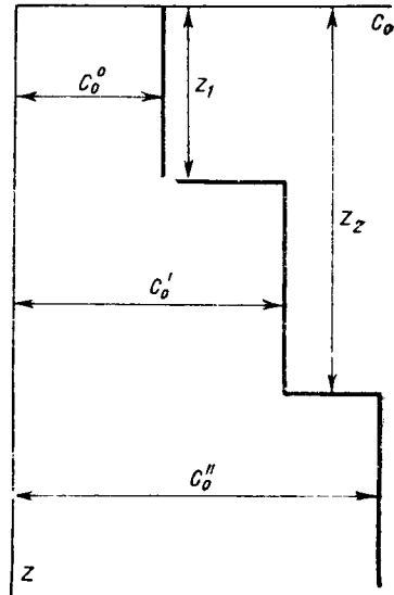
Рис. 56. Ступенчатый график начального распределения концентрации солей
