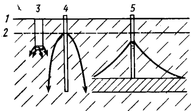
Рис. 62. Опытные опробования в зоне аэрации:
