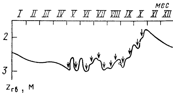
Рис. 47. Данные примера расчетов изменения глубины залегания среднего на междуренье уровня грунтовых вод при поливах. Стрелкой обозначено время поливов
