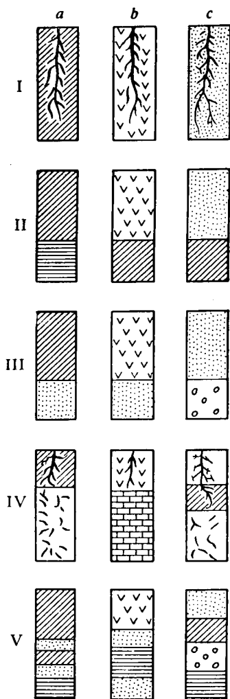
Рис. 22. Основные схемы (I—V) геологического строения осушаемых земель (на схемах I и IV показаны корни растений) (по Б. С. Маслову).
