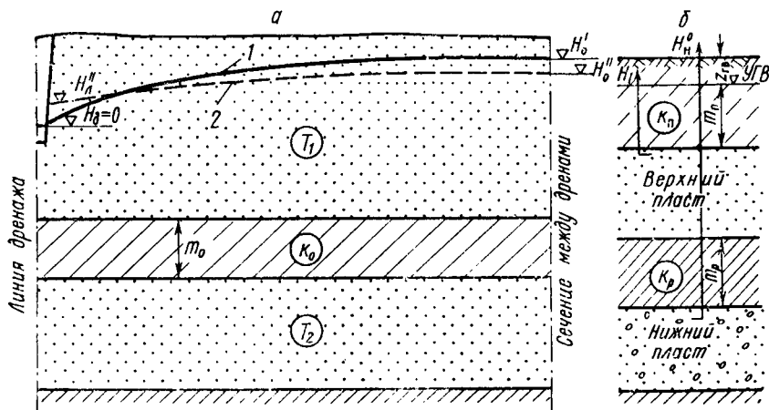
Рис. 48. Линейный дренаж в двухпластовой системе:
