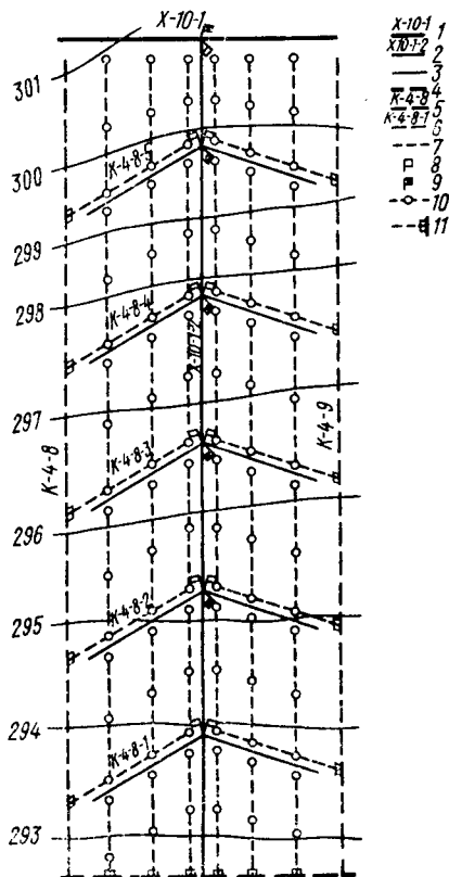
Рис. 2. Схема внутрихозяйственной оросительной и дренажной сети («Практикум по сельскохозяйственным мелиорациям», 1980):
