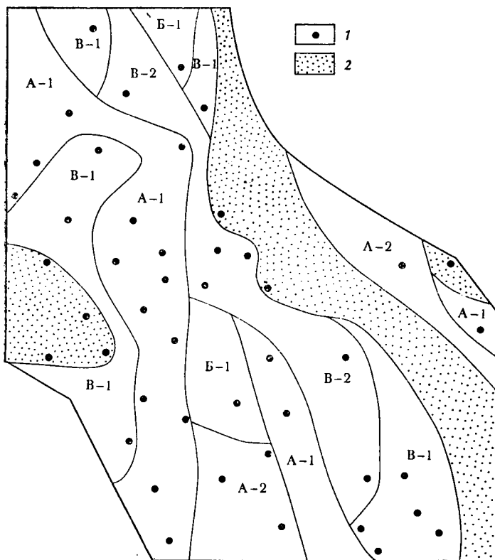
Рис. 55. Пример картирования покровных отложений по условиям применения горизонтального дренажа в Каршинской степи (по А. М. Соيفеру): 1 — разведочные скважины, 2 — область, где отсутствуют покровные отложения и песчаный пласт залегает на поверхности земли
