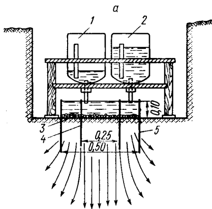
Рис. 63. Схема налива в инфильтрометр:
