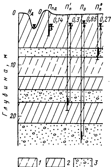
Рис. 80. Разрез по кусту пьезометрических скважин вблизи открытой дрены на территории Чуйской впадины (по данным М. И. Гоголева): 1 — супесь; 2 — суглинок; 3 — песок с гравием
