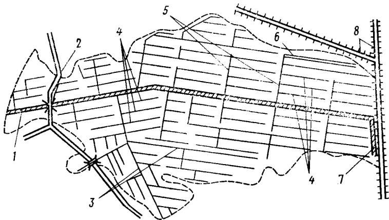
Рис. 11. Схема осушительной системы:
