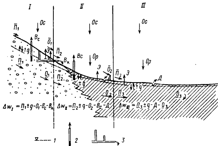
Рис. 17. Схема водного баланса Ширванской равнины:
