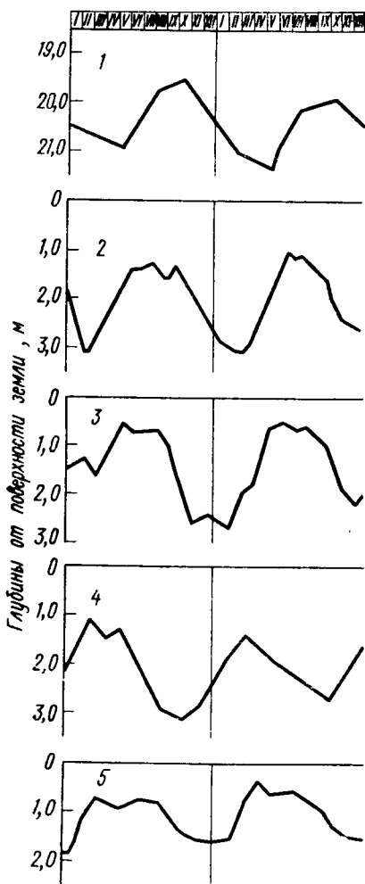
Рис. 25. Типовые графики сезонных колебаний уровня грунтовых вод в орошаемых районах разной естественной дренированности (по среднемесячным данным).
