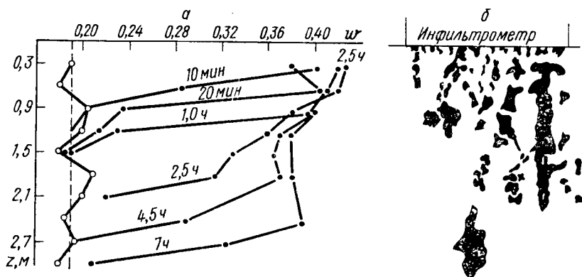
Рис. 64. Динамика увлажнения лёссовидных суглинков при наливе в шурф: а — эпюра влажности под шурфом (по данным В. В. Бадова); б — зарисовка распространения красителя под шурфом в разрезе по диаметральному сечению (по данным Е. К. Широковой)
