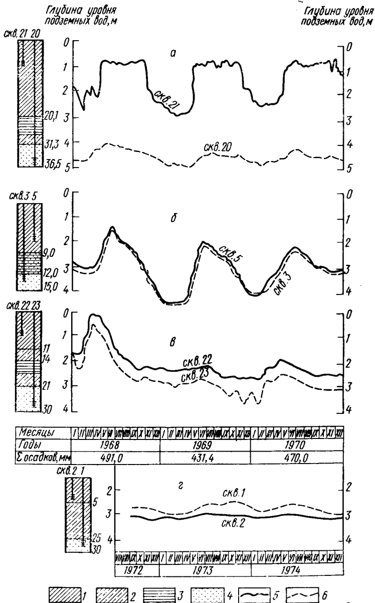
Рис. 29. Графики режима уровней подземных вод Багаевско-Садковской оросительной системы (по В. А. Васильченко, 1974):
