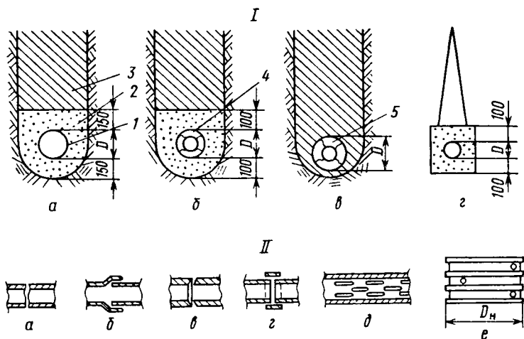
Рис. 3. Конструкции горизонтального дренажа: I — конструкция дренажа при механизированном способе строительства: а — с круговым песчано-гравийным фильтром; б — то же с дополнительным применением стеклохолста; в — с круговым фильтром из искусственных волокнистых материалов; г — с песчано-гравийным фильтром при бестраншейном способе строительства; II — типы дренажных труб: керамические трубы, фильтрующие через стык, — гладкие (а), раструбные (б), фасонные (в), муфтовые (г); фильтрующие через тело труб (трубофильтры) гладкие с дырчатой или шелевой перфорацией (д); полимерные гофрированные трубы (е)
