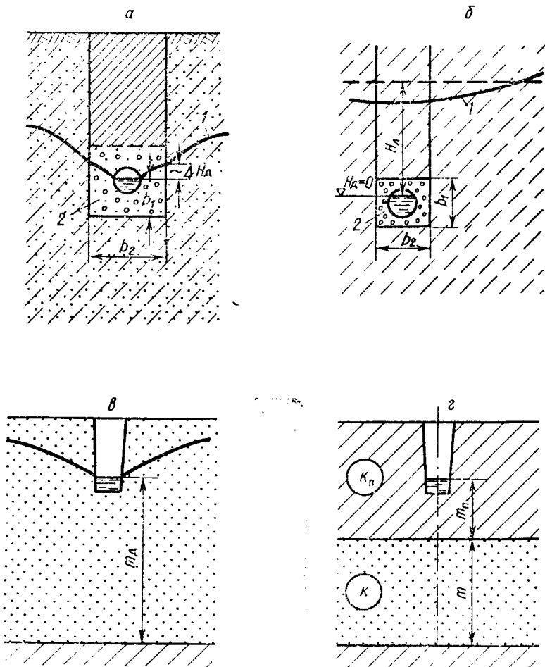
Рис. 43. Сечение горизонтальных дрен:
