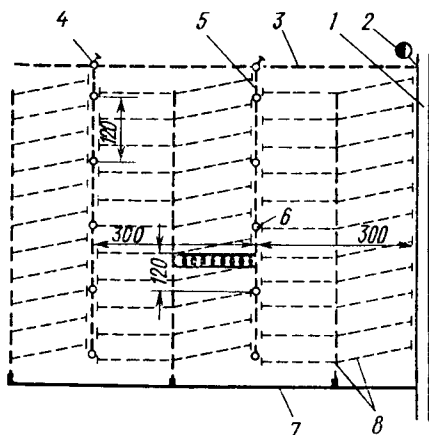
Рис. 14. Схема осушительно-увлажнительной системы с закрытым дренажем и поливом установкой УДС-25 (по Б. С. Маслову, В. С. Станкевичу, В. Я. Черненко, 1981):
