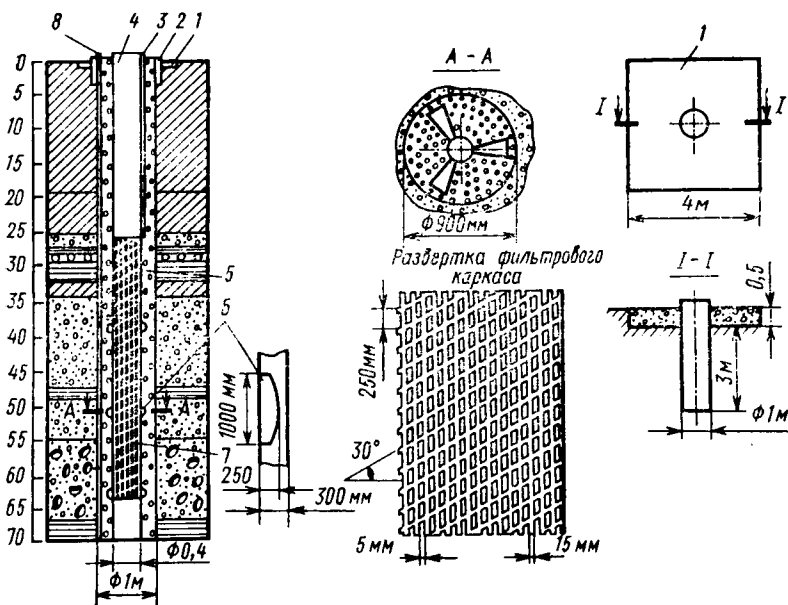
Рис. 5. Конструкция скважин вертикального дренажа в совхозе «Социализм» в Голодной степи (по Н. М. Решеткиной, Х. И. Якубову, 1978): 1 — бетонная плита для крепления кондуктора; 2 — кондуктор; 3 — труба для замера уровня воды в скважине; 4 — глухая часть фильтрового каркаса; 5 — перфорированная часть фильтрового каркаса, скважность 20%; 6 — направляющие фонари из стали толщиной 10 мм; 7 — гравийная обсыпка, размер фракций 1—10 мм; 8 — затрубный пьезометр, скважность фильтра 15%
