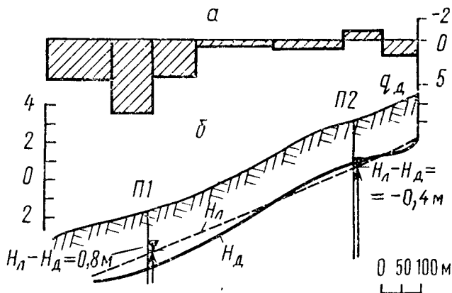
Рис. 81. Характеристики дренажного стока по данным гидродинамической съемки на участке закрытой горизонтальной дрены в Чуйской впадине (по данным М. И. Гоголева): а — распределение удельного притока к дрене; б — напоры H_n и H_d на линии дрены
