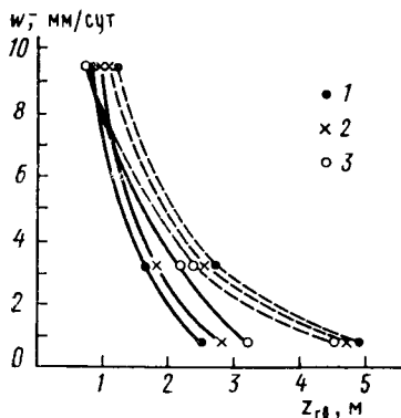
Рис. 36. Расчетные графики зависимости интенсивности испарения w^- от глубины залегания грунтовых вод z_{гв} и изменения коэффициента фильтрации \kappa_\phi зоны аэрации при задании \kappa(\psi) по (4.6 в): сплошные линии при m=3 и a=40 \text{ м}^{-3} , пунктир при m=2 и a=20 \text{ м}^{-2} ; 1 — \kappa_\phi=0,3 \text{ м/сут} , 2 — \kappa_\phi=0,5 \text{ м/сут} , 3 — \kappa_\phi=1 \text{ м/сут}
