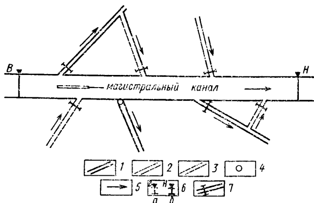
Рис. 82. Гидрографическая схема участка магистрального канала: 1 — оросительные каналы; 2 — дренажи; 3 — сбросные коллекторы; 4 — насосная станция; 5 — направление движения воды в каналах; 6 — гидрометрические створы, ограничивающие расчетный участок (В — верхний, Н — нижний по течению); 7 — гидрометрические створы
