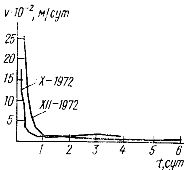
Рис. 33. Изменение во времени скорости просачивания v_n (средней в пределах поля) при промывках на опытном участке в Джизакской степи [21]
