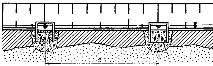
Рис. 7. Горизонтальные дрены с колодцами-усилителями
