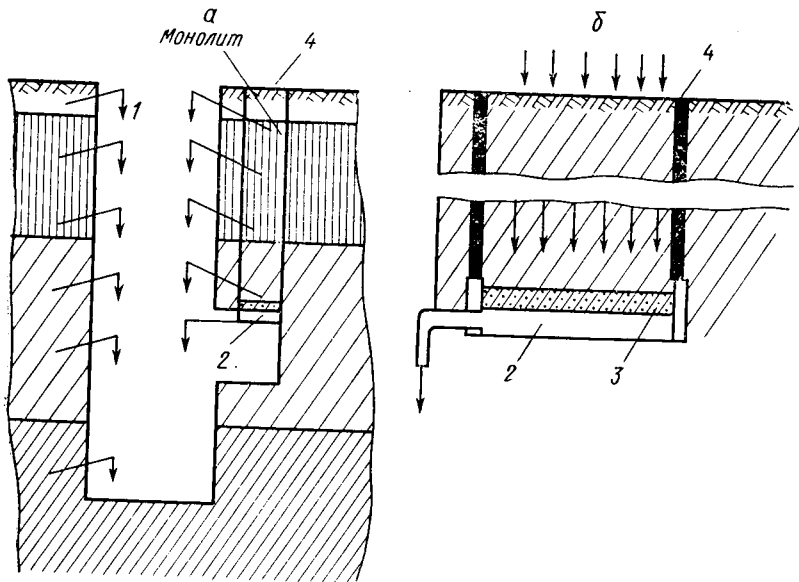
Рис. 70. Шурф, оборудованный балансометром:
