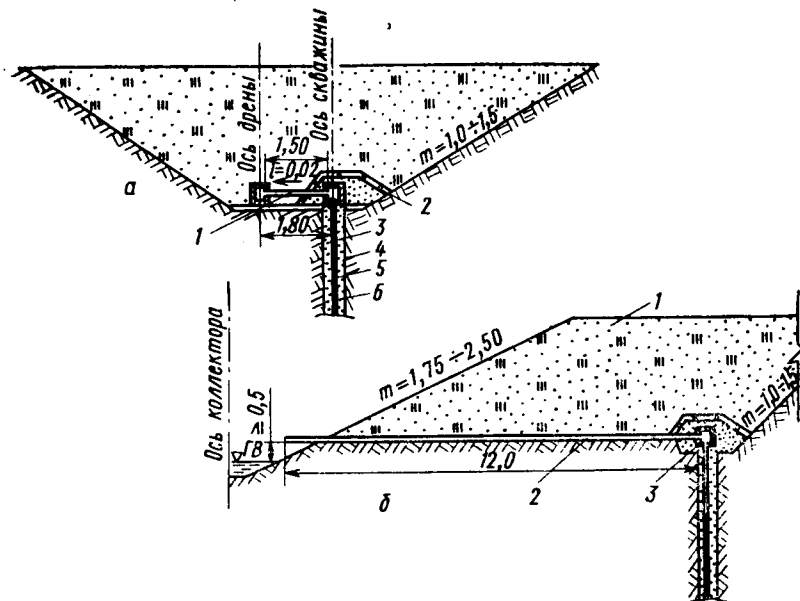
Рис. 6. Комбинированный дренаж:
