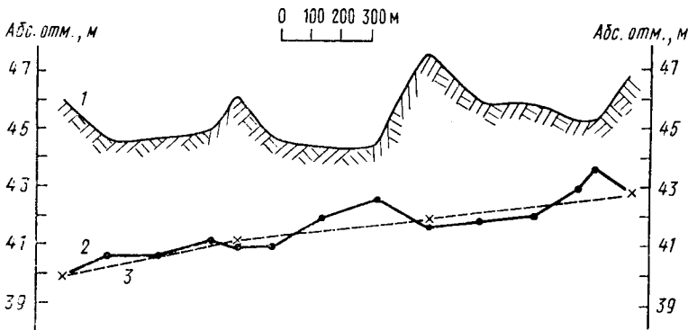
Рис. 78. Данные гидродинамической съемки в Куйбышевском Поволжье: 1 — поверхность земли; 2 и 3 — уровни воды в покровных отложениях и водоносном пласте
