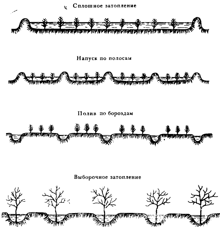
Рис. 8. Классификация поверхностных способов полива (по Б. Г. Штепе)
