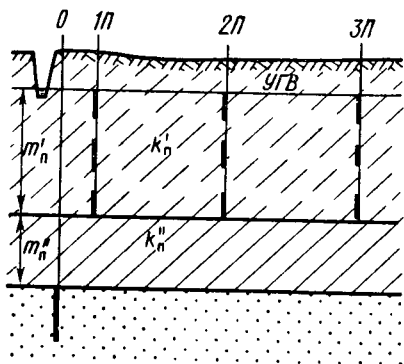
Рис. 79. Схема размещения пьезометров вблизи дрены в вертикальном сечении покровных отложений при наличии в их подошве экранирующего слоя
