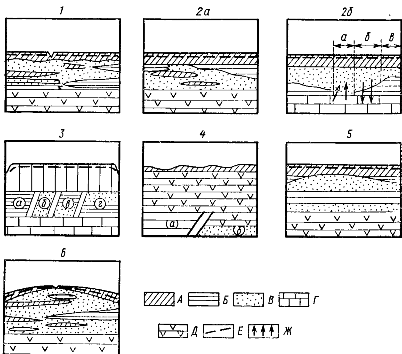
Рис. 20. Типы гидрогеологических условий орошаемых районов платформенной группы (по Д. М. Кацу):
