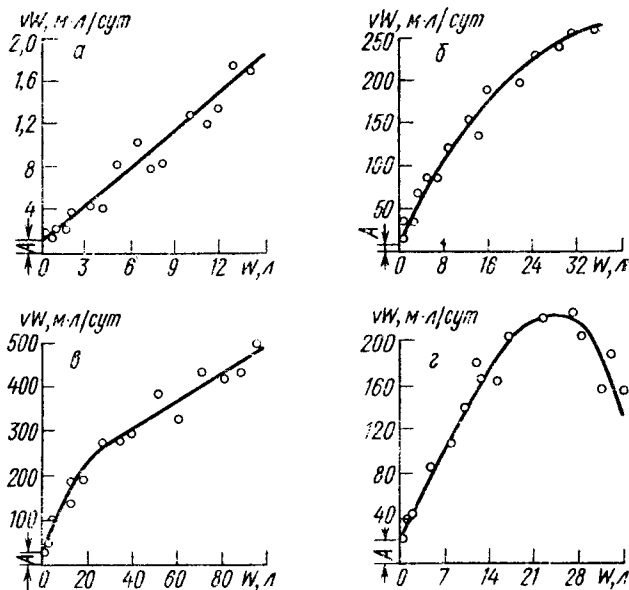
Рис. 65. Типичные графики зависимости v — w по данным наливов в эолово-делювиальных суглинках [4]: a — однородная толща; б — постепенное уменьшение проницаемости по глубине; в — двухслойное строение фильтрующих пород; г — однородный слой с постепенным переходом к уменьшающейся по глубине проницаемостью
