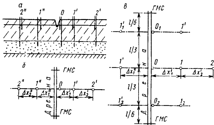
Рис. 76. Схема размещения пьезометрической сети ОФА на междуренье: а — вертикальное сечение при двухслойном строении дренируемого потока; б и в — расположение створов пьезометров в плане между гидрометрическими створами (ГМС)
