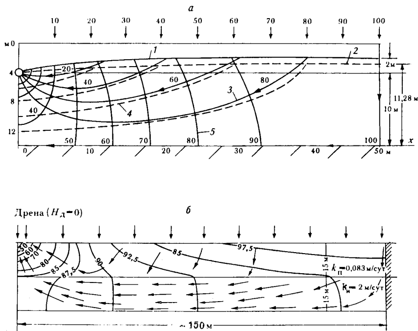
Рис. 42. Модельные гидродинамические сетки между горизонтальными дренами при инфильтрационном питании:
