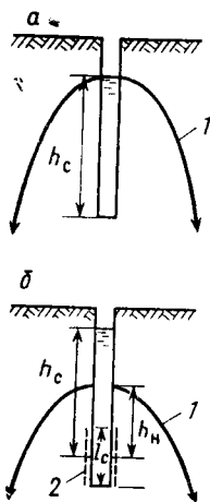
Рис. 67. Наливы в сухие скважины при однородном строении: а и б — открытая и фильтровая скважины (1 — свободная поверхность, 2 — фильтр)
