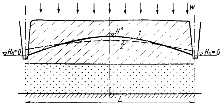
Рис. 45. Систематический горизонтальный дренаж в однопластовой системе: 1 — уровни свободной поверхности; 2 — напоры в основном пласте
