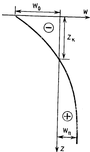
Рис. 31. Типичный график зависимости интенсивности результирующего ирригационного питания w от глубины залегания уровня грунтовых вод z
