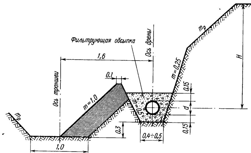
Рис. 4. Схема дренажа, сооружаемого методом «полки» (размеры в метрах) (по В. А. Духовному и др., 1979)
