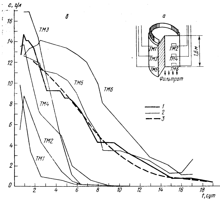
Рис. 57. Опытная промывка монолита: а — схема оборудования монолита (ТМ — тензиометрические датчики; в рассматриваемом монолите датчики ТМ1 и ТМ2 установлены на глубине 0,5 м, ТМ3 и ТМ4 — на глубине 1 м, ТМ5 и ТМ6 — на глубине 1,5 м от поверхности монолита); б — данные изменения концентрации хлор-нона во время промывки (1 — в фильтрате, 2 — в пробах, отбираемых из тензиометров, 3 — расчетная выходная кривая)
