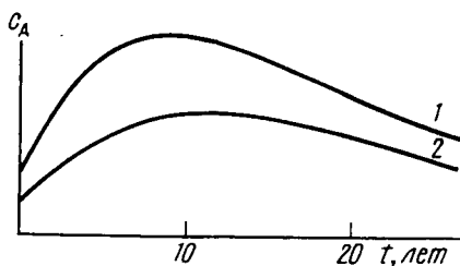
Рис. 59. Типичные графики минерализации пластовых (1) и дренажных (2) вод после промывок и поливов на фоне вертикального дренажа (по С. Я. Соيفер [25])
