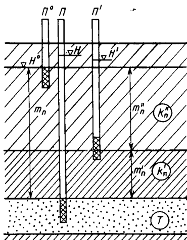
Рис. 77. Расположение этажных пьезометров в покровном пласте
