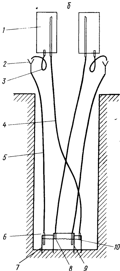
Рис. 63. Схема налива в инфильтрометр:
