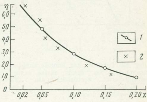
Рис. 80. График для оценки поправочного множителя \eta > 1,0 при малой глубине эрозионного среза оловянных проявлений Кавалеровского района. По А. П. Соловову и П. А. Куршеву.
