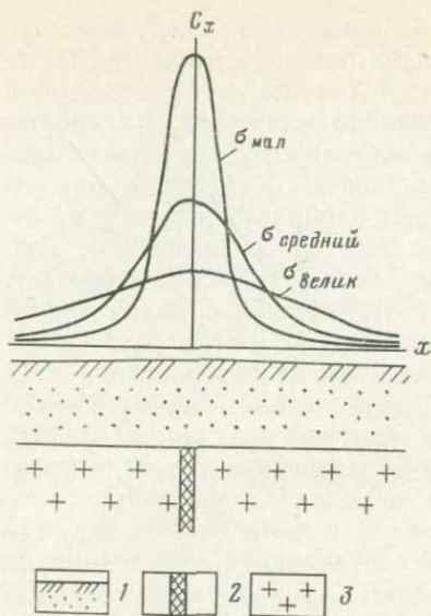
Рис. 34. Графики вторичных остаточных ореолов рассеяния рудной жилы для различных значений коэффициента рассеяния \sigma .
