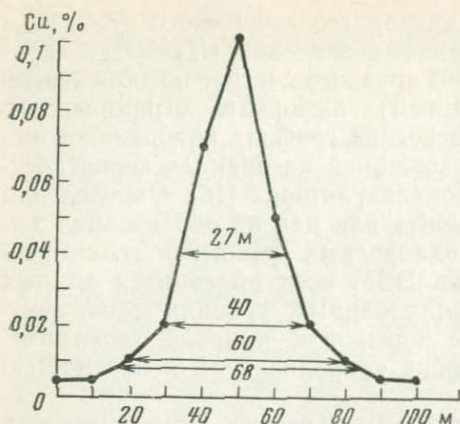
Рис. 6. График изменения эффективной (наблюдаемой) ширины геохимической аномалии в зависимости от чувствительности анализа проб и выбора нижнего аномального содержания меди
