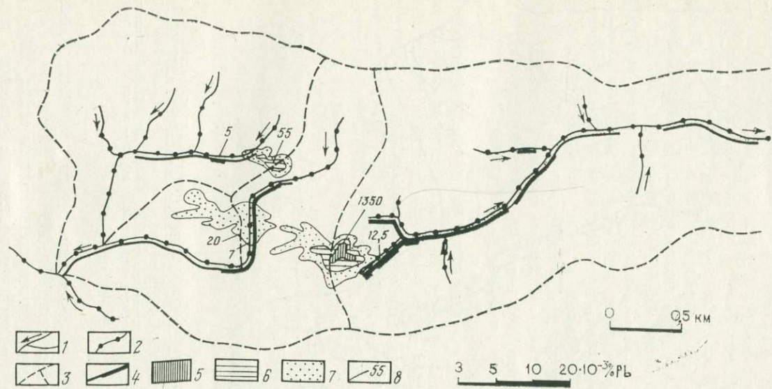
Рис. 98. Вторичные ореолы и потоки рассеяния свинца. Участок Тыкжол Джунгарский Ала-тау. По С. А. Миляеву.
