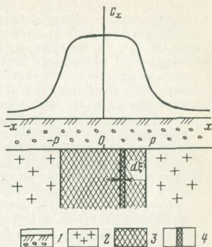
Рис. 35. График остаточного ореола рассеяния C_x = f(x) над мощным рудным телом.
