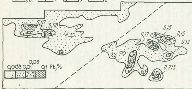
Рис. 111. Геологическая схема и вторичные ореолы рассеяния полиметаллического рудопоявления Левобержное. По Р. А. Дегтяреву и С. А. Миляеву.
