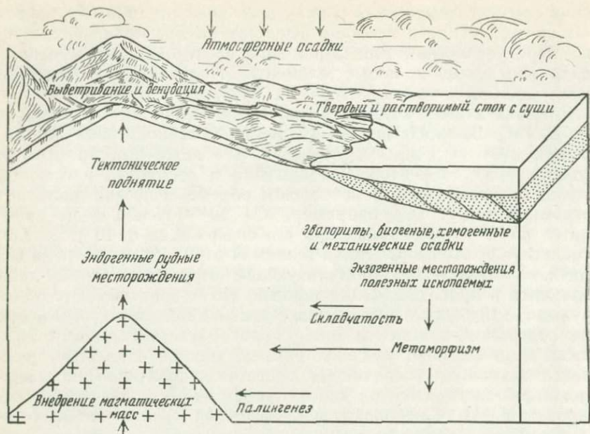
Рис. 2. Схема геологического цикла миграции химических элементов
