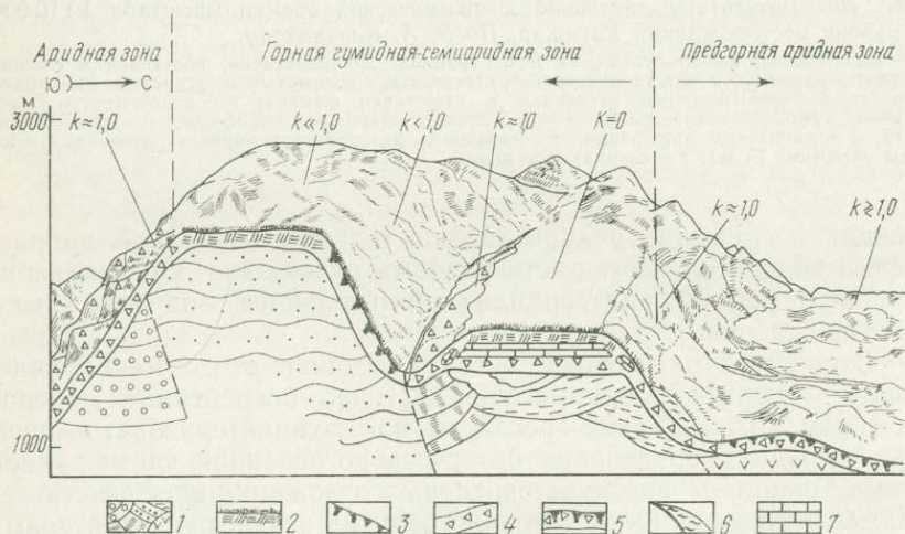
Рис. 109. Схема развития вторичных ореолов рассеяния свинца для Текелайской группы месторождений [25].
