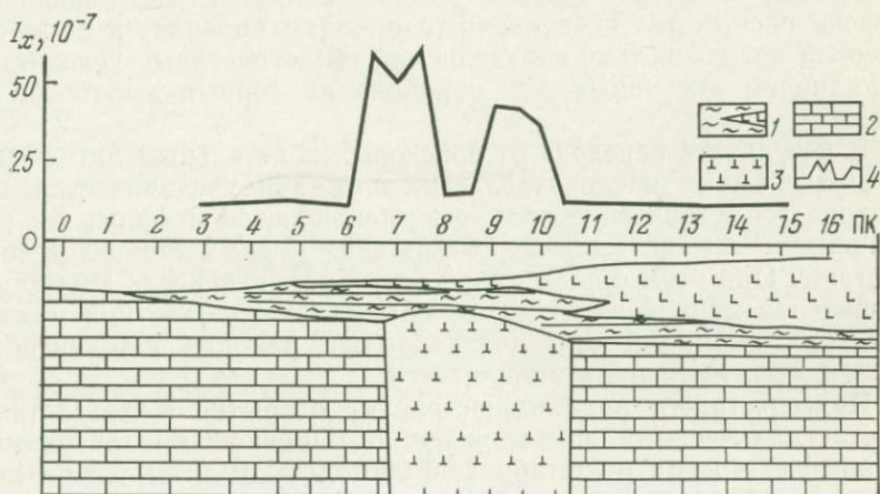
Рис. 107. Результаты наземной литохимической съемки над кимберлитовой трубкой. По С. А. Воробьеву.
