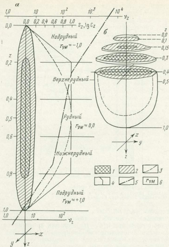
Рис. 78. Модель рудной линзы:
