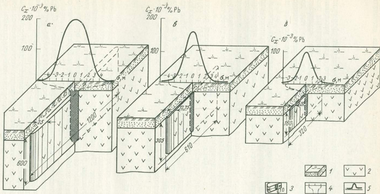
Рис. 51. Решение прямой задачи для крупного (а), среднего (б) и мелкого (в) месторождений свинцовых руд в ландшафтах выровненных водоразделов Заилийского Алатау [25].
