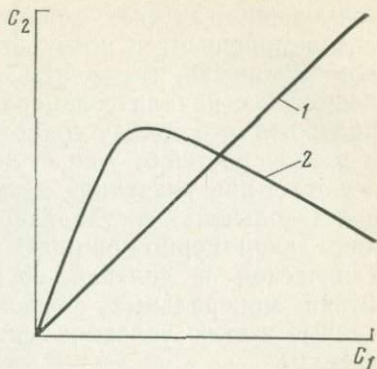
Рис. 93. Графики зависимостей содержания рудных элементов в золе растений ( C_2 ) от их содержания в почве ( C_1 ).
