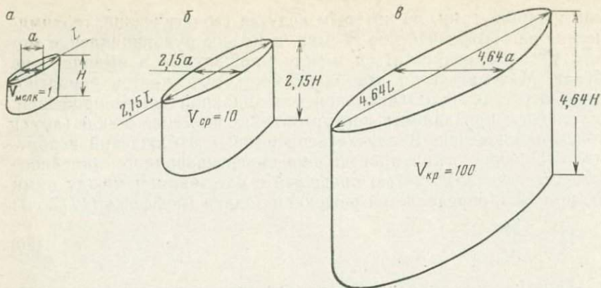
Рис. 9. Линейные и площадные размеры фигур подобия при соотношении объемов ( a : b : v ) 1 : 10 : 100
