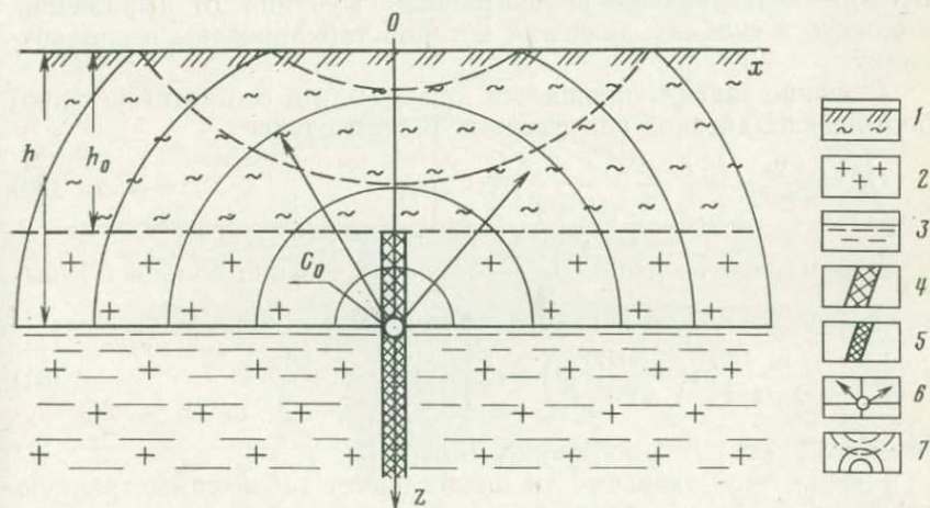
Рис. 45. Модель формирования наложенного диффузионного ореола рассеяния.
