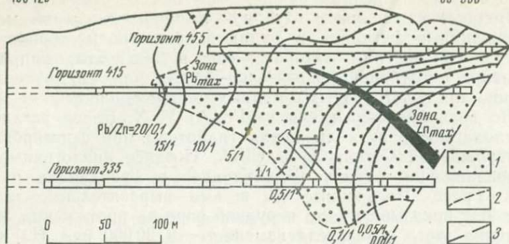
Рис. 63. Продольный вертикальный разрез рудника Блайклиппен с изолиниями v = \text{Pb}/\text{Zn} .
