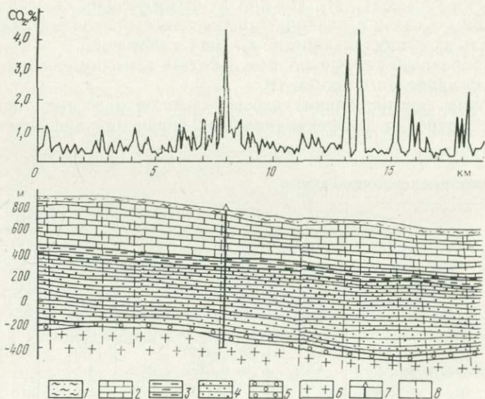
Рис. 90. График содержаний CO 2 и геологический разрез по профилю Боргустан — Эссентуки. По А. И. Фридману.
