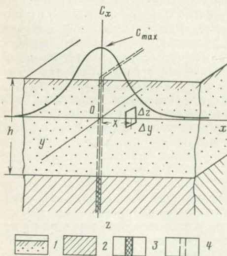
Рис. 33. К выводу уравнения рассеяния. 1 — элювио-делювий; 2 — коренные породы; 3 — рудное тело; 4 — положение рудного тела до выветривания
