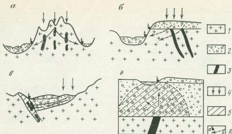
Рис. 83. Схемы В. И. Красикова для доказательства повышенной глубинности гидрохимических поисков.
