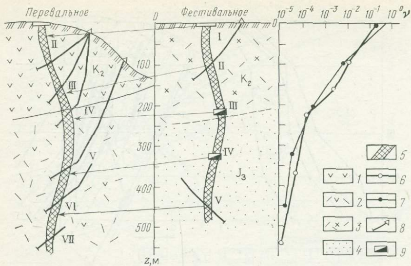
Рис. 74. Геологические разрезы двух оловорудных месторождений и графики общего для них геохимического показателя зональности v_z = \frac{\text{Bi}^2 \cdot \text{Ag}}{\text{Sn}^2 \cdot \text{W}} .
