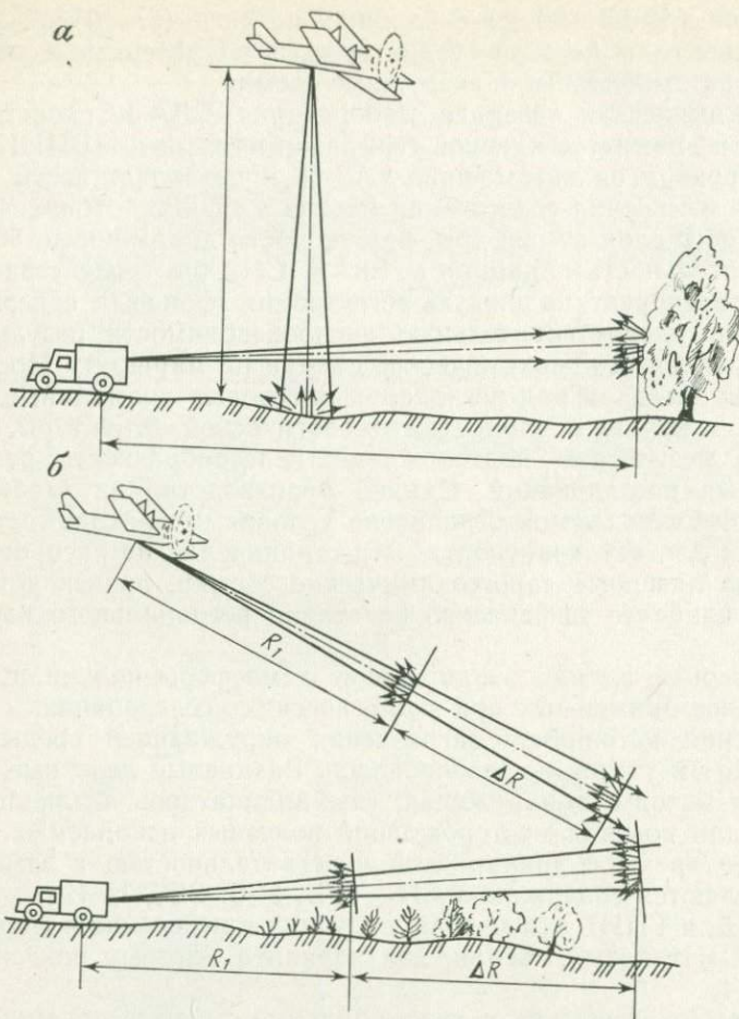
Рис. 114. Лазерная геохимическая съемка. По И. М. Назарову и др. а — с использованием топографических отражателей; б — с измерением рассеянного отражения
