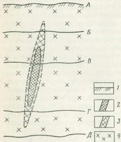
Рис. 4. Уровни денудационных срезов (Б—Д) крутопадающего рудного тела и его первичного ореола.
