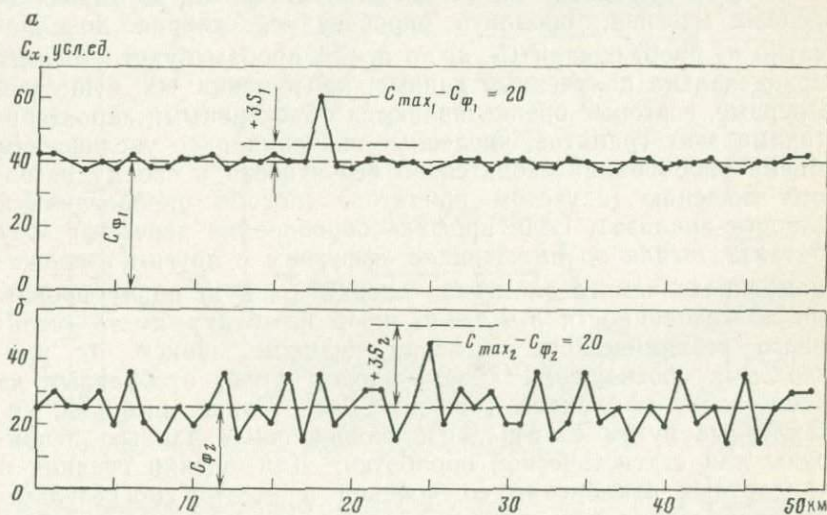
Рис. 7. Сравнение контрастности двух слабых аномалий при разных параметрах фона:
