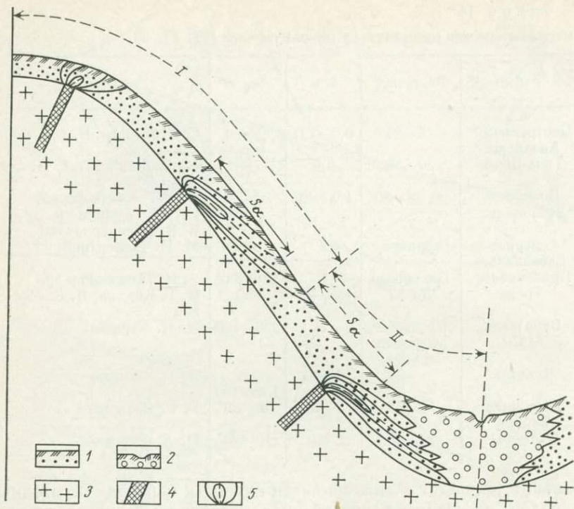
Рис. 44. Вторичные остаточные ореолы рассеяния на горном склоне. I — алувио-делювий; 2 — аллювий; 3 — рудовмещающие породы; 4 — рудное тело; 5 — вторичный ореол рассеяния, пунктиром показана ось ореола. Интервалы склона: I — ореолы открытого типа; II — ореол преимущественно закрытого типа
