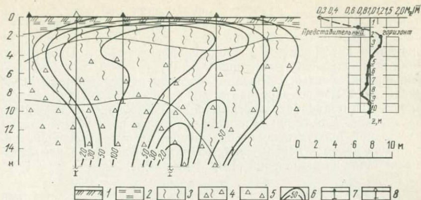
Рис. 40. Вертикальный разрез ореола рассеяния и график M_z/\bar{M} .
