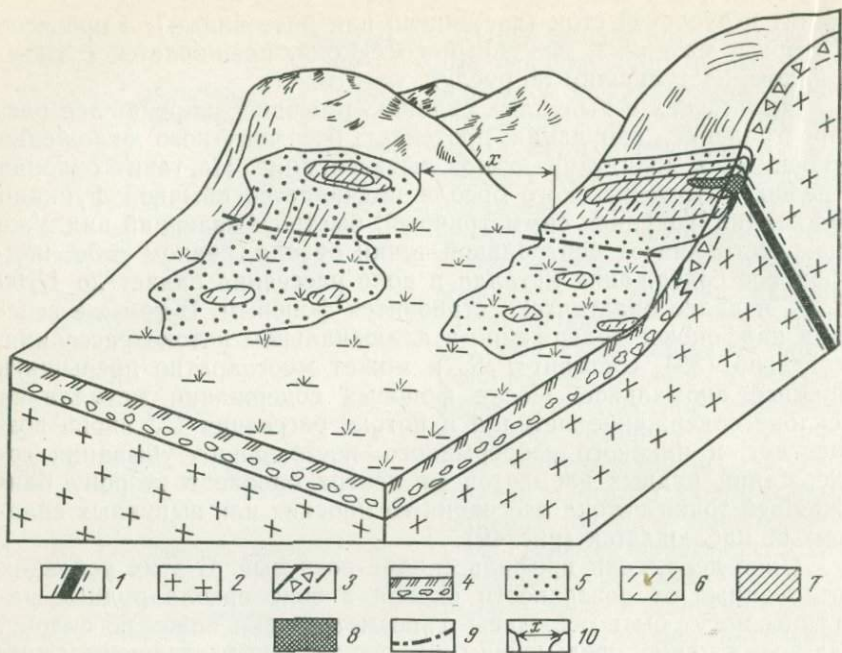
Рис. 50. Шлейфы ореолов рассеяния на вогнутом склоне.
