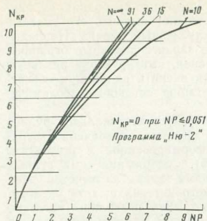
Рис. 68. Номограмма для оценки критического числа случайных показателей (95 %-ный доверительный предел). По Ю. В. Шварову.
