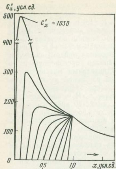
Рис. 15. Семейство кривых C'_x = f(x) для различных положений точки R_0 = 0,0; 0,1; 0,2; \dots 0,9 при C'_\phi = 0; P = 100; R = 1,0 и S_x = x^2 - \frac{1}{3}x^3 .
