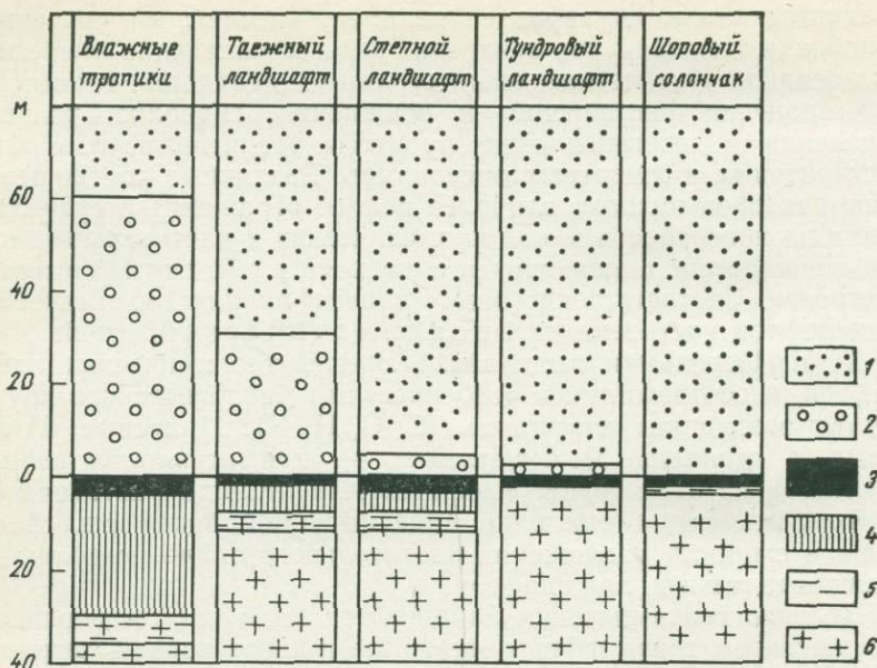
Рис. 12. Строение элементарных ландшафтов.
