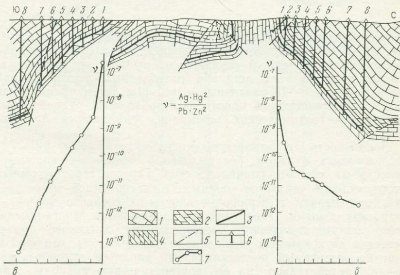
Рис. 73. Графики изменения показателя геохимической зональности с глубиной. Миргалимское месторождение.
