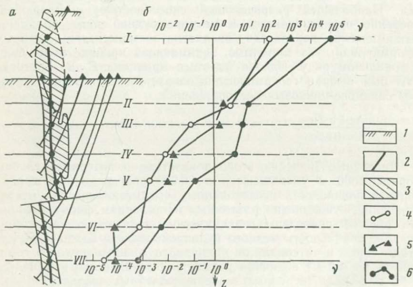
Рис. 64. Сводный профиль (а) и графики геохимических показателей зональности (б) медного рудопоявления.
