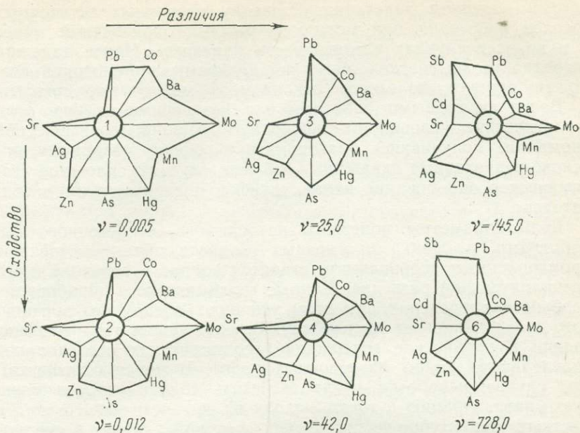
Рис. 112. Круговые геохимические спектры медных месторождений Спасской рудной зоны. Отношение средних содержаний 12 рудных элементов к содержаниям меди; диаметр круга равен \lg 10 . По И. А. Кошелевой.
