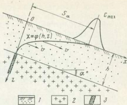
Рис. 42. Смещение остаточного литохимического ореола рассечения на плоском склоне.
