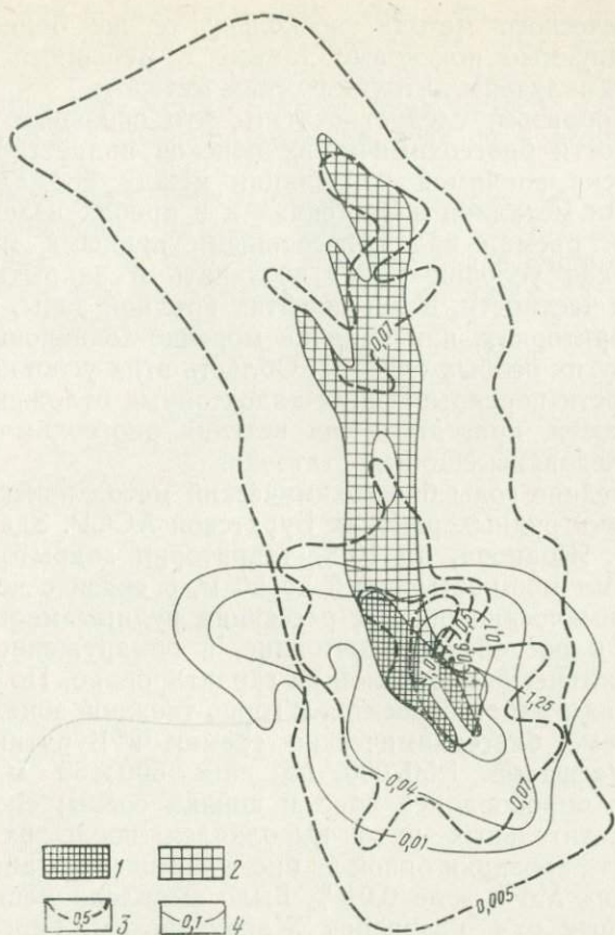
Рис. 94. Сравнительные результаты лито- и биогеохимических съемок на месторождении Узунжал. По В. О. Гетманчуку.
