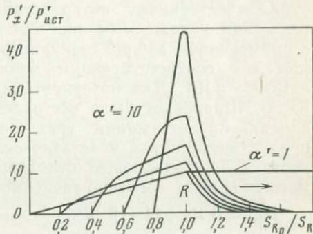
Рис. 17. Графики C'_x = f(S_x) и P'_x = f(S_x) истинной (при \alpha' = 1 ) и кажущейся (при \alpha' = 3 и \alpha' = 10 ) продуктивностей потоков рассеяния.
