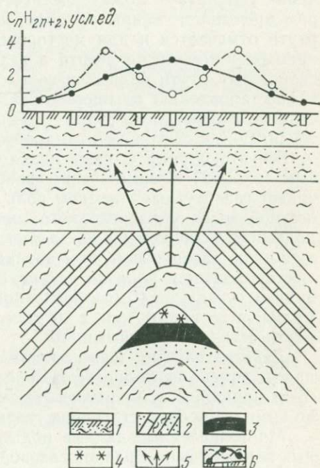
Рис. 87. Схема атмохимического ореола рассеяния газонефтяной залежи.
