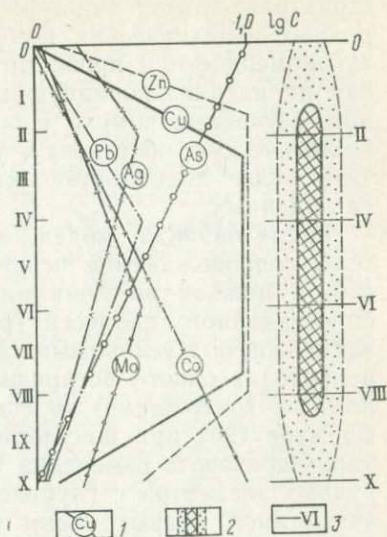
Рис. 69. Модель эндогенного оруденения (вертикальный разрез).
