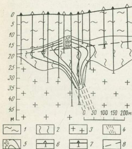
Рис. 29. Погребенный остаточный ореол рассеяния (Северный Казахстан). По А. Н. Еремеву и А. П. Соловову.
