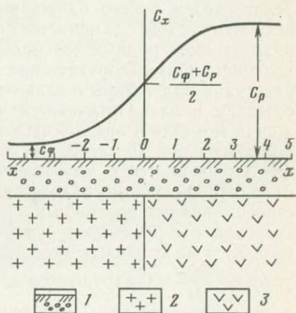
Рис. 36. График ореола рассеяния над контактом пород.
