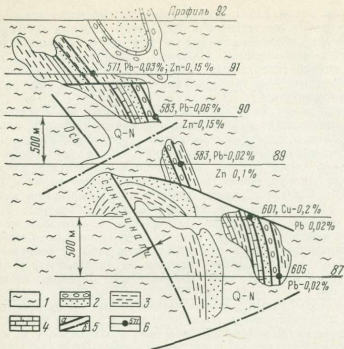
Рис. 101. Геологическая схема, составленная по результатам осмотра аномалии и дешифрирования аэрофотоснимков. По Л. М. Филинскому.
