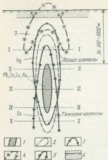
Рис. 57. Модель первичных ореолов гидротермального месторождения.
