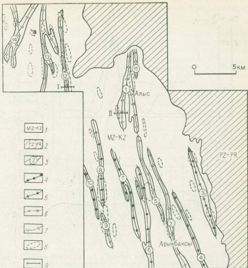
Рис. 103. Результаты атмосферической съемки масштаба 1:100 000. Тургайский прогиб. По Б. А. Досановой, В. Н. Колесникову, С. А. Воробьеву.
