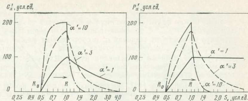
Рис. 17. Графики C'_x = f(S_x) и P'_x = f(S_x) истинной (при \alpha' = 1 ) и кажущейся (при \alpha' = 3 и \alpha' = 10 ) продуктивностей потоков рассеяния.
