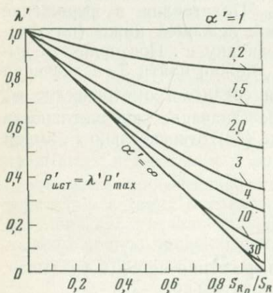
Рис. 19. Номограмма для оценки \lambda' по значениям \alpha' и S_{R_0}/S_R [43]
