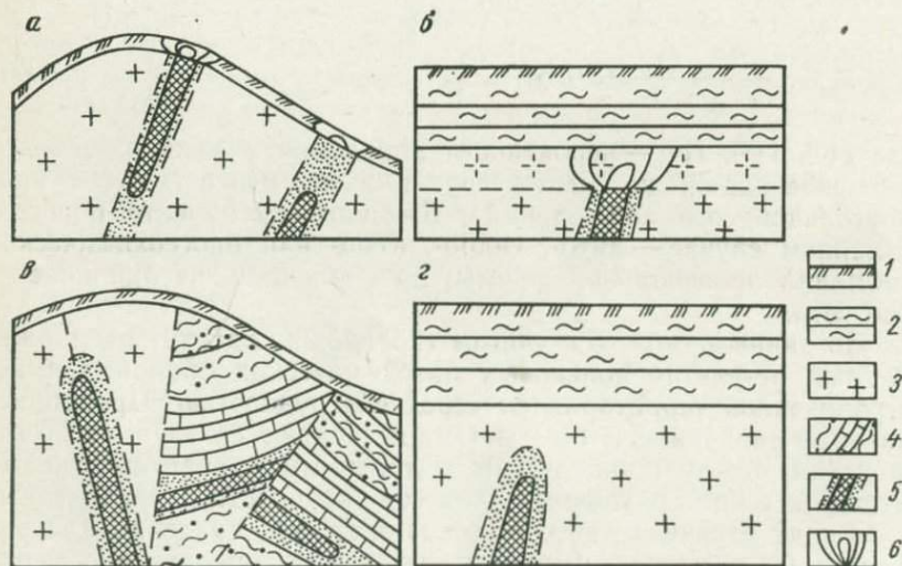
Рис. 10. Рудные месторождения в различных условиях залегания а — выходящие на поверхность; б — погребенные; в — слепые; г — слепые погребенные. 1 — современный элювио-делювий; 2 — дельтаприносные отложения; 3, 4 — рудовмещающие породы; 5 — рудные тела и их первичные ореолы (по основному рудному элементу); 6 — вторичные остаточные ореолы рассеяния
