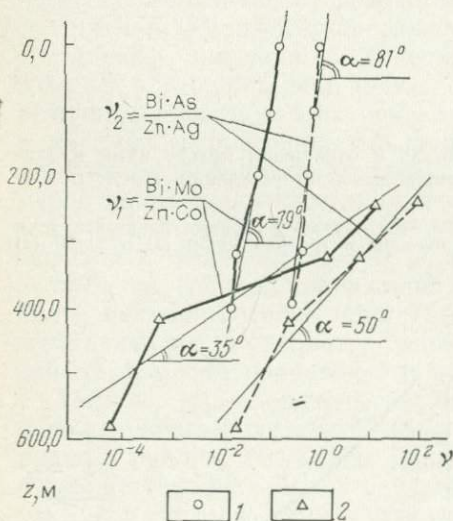
Рис. 81. Графики для оценки коэффициента подобия между двумя медно-порфировыми месторождениями. По А. А. Матвееву.
