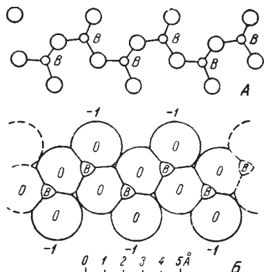
Рис. 268. Цепочки связанных комплексов \text{BO}_3 : a — положение центров ионов; b — вид цепочки в кристаллической структуре
