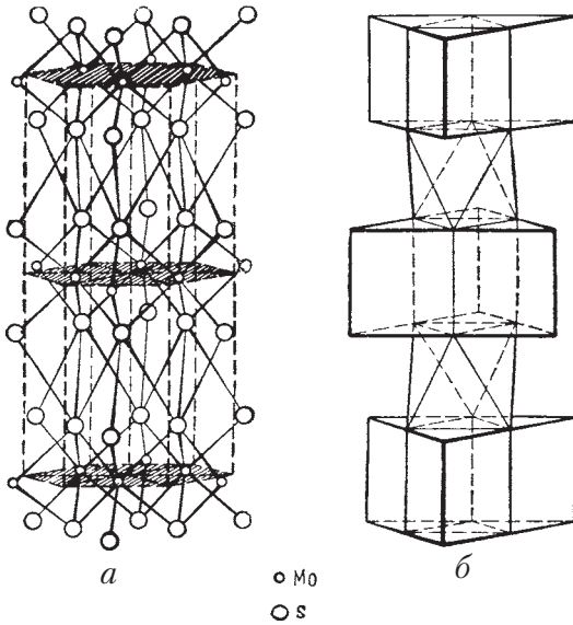
Рис. 112. Кристаллическая структура молибденита: a — расположение центров ионов (слои, содержащие ионы молибдена, заштрихованы); б — та же структура изображена по способу Н. В. Белова
