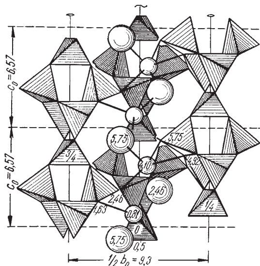
Рис. 364. Кристаллическая структура натролита.
