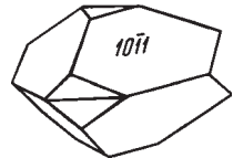
Рис. 214. Двойник кальцита по (0001)
