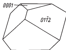
Рис. 249. Кристалл алунита
