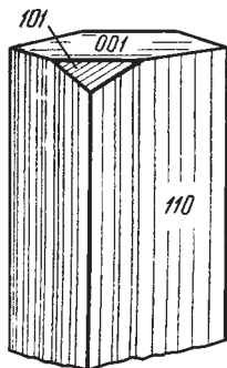
Рис. 205. Кристалл манганита
