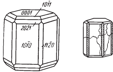
Рис. 359. Кристаллы нефелина
