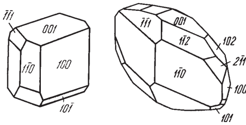
Рис. 304. Кристаллы алланита
