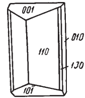
Рис. 351. Кристалл адуляра
