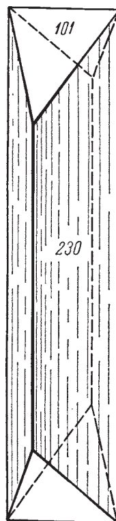
Рис. 126. Кристалл арсенопирита
