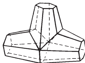
Рис. 101. Двойник пирротина
