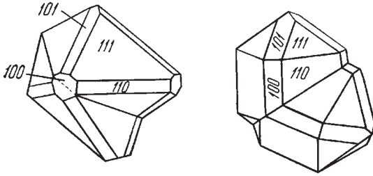
Рис. 166. Двойники касситерита
