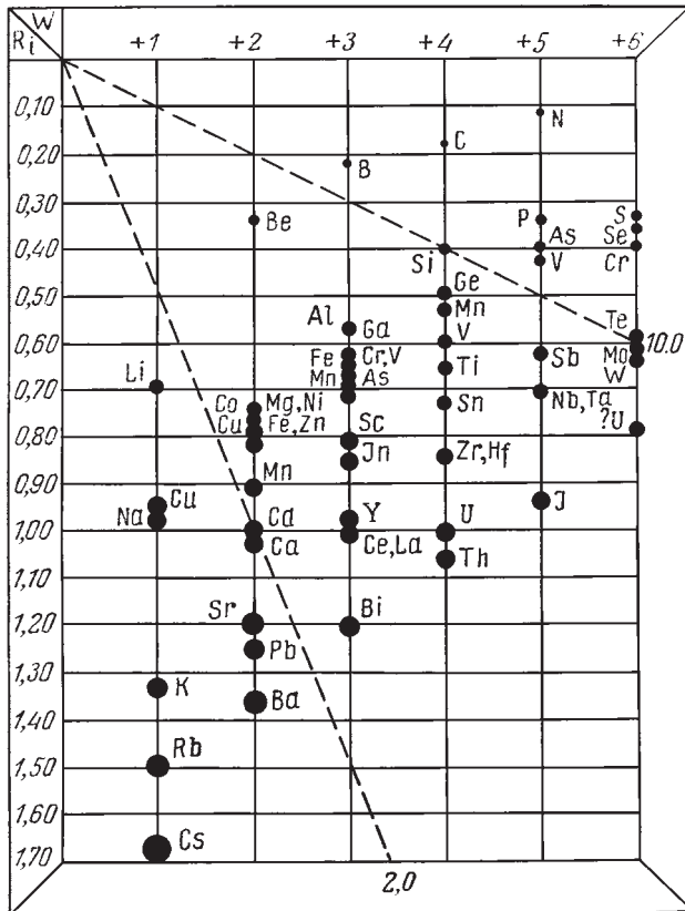
Рис. 206. Диаграмма главнейших катионов, распространенных в природных соединениях
