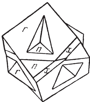
Рис. 98. Двойник киновари r \{10\bar{1}1\} , n \{20\bar{2}1\} , x \{42\bar{6}3\}
