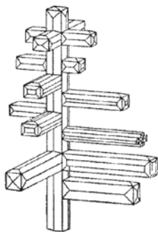
Рис. 20. Реберные скелетные кристаллы: а — нашатырь; б — галит
