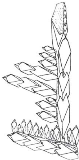
Рис. 69. Дендритовидный скелетный кристалл золота
