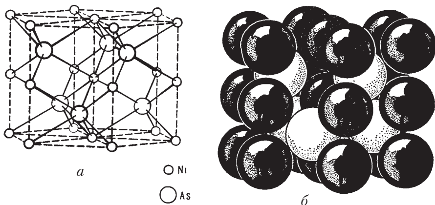
Рис. 102. Кристаллическая структура никелина.
