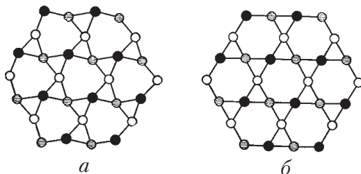
Рис. 184. Соотношения в кристаллических структурах \beta -кварца (а) и \alpha -кварца (б). Показаны только ионы кремния, высотное положение которых отмечено различной степенью затененности кружков
