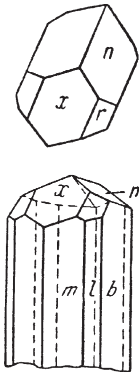
Рис. 108. Кристалл реальгара. Лухумское месторождение (по И. И. Шафрановскому): m \{110\} , l \{120\} , b \{010\} , n \{011\} , x \{\bar{1}01\} , r \{\bar{1}\bar{1}1\}
