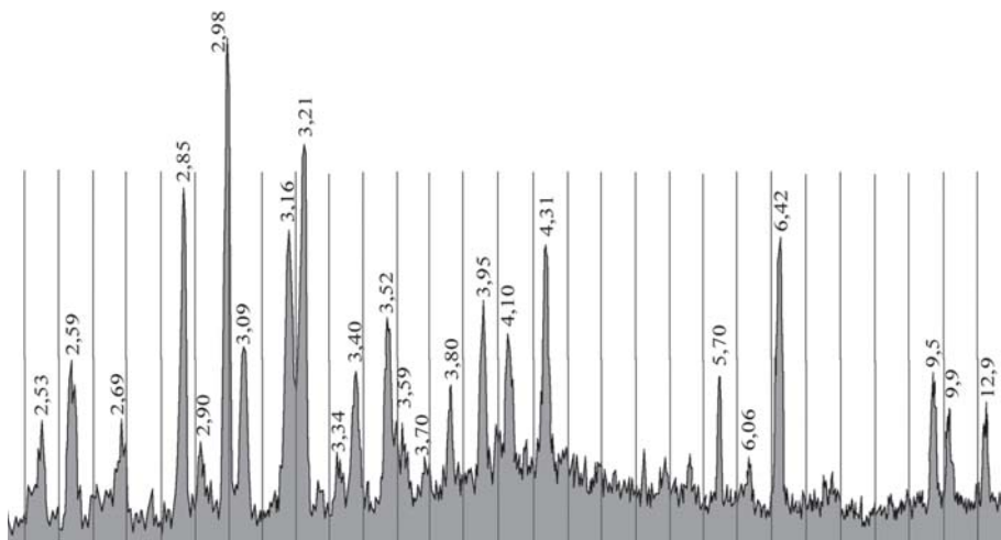
Рис. 33. Дифрактограмма эпидиота. Пики кривой соответствуют максимумам интенсивности излучения, дифрагированного на определенных семействах плоскостей решетки. Цифры у пиков выражают соответствующие межплоскостные расстояния в Å
