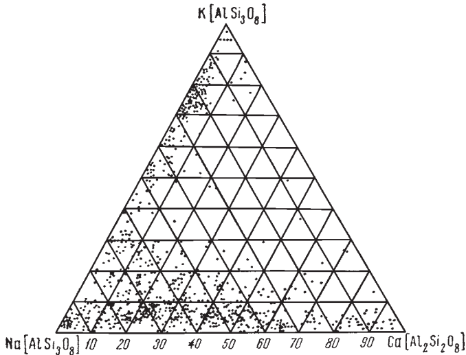
Рис. 346. Диаграмма колебаний химического состава полевых шпатов
