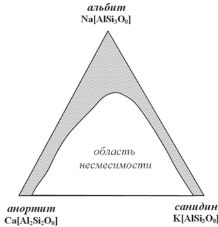
Рис. 8. Поле составов твердых растворов высокотемпературных полевых шпатов (выделено крапом)
