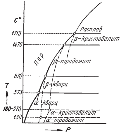
Рис. 180. Однокомпонентная система SiO 2 . Кривые упругости паров различных модификаций показаны схематически. При каждой данной температуре более устойчива та модификация, у которой упругость пара меньше (т. е. кривая ближе к оси ординат)
