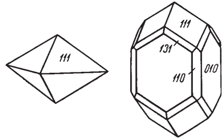
Рис. 277. Кристаллы торита
