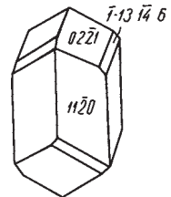
Рис. 309. Кристалл диоптаза
