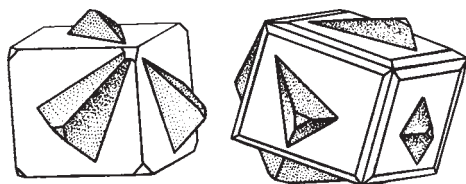
Рис. 174. Двойники лопарита
