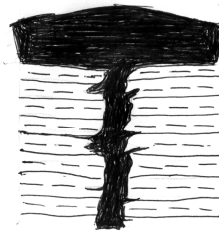
Рис. 2. Схема образования эффузивных пород
