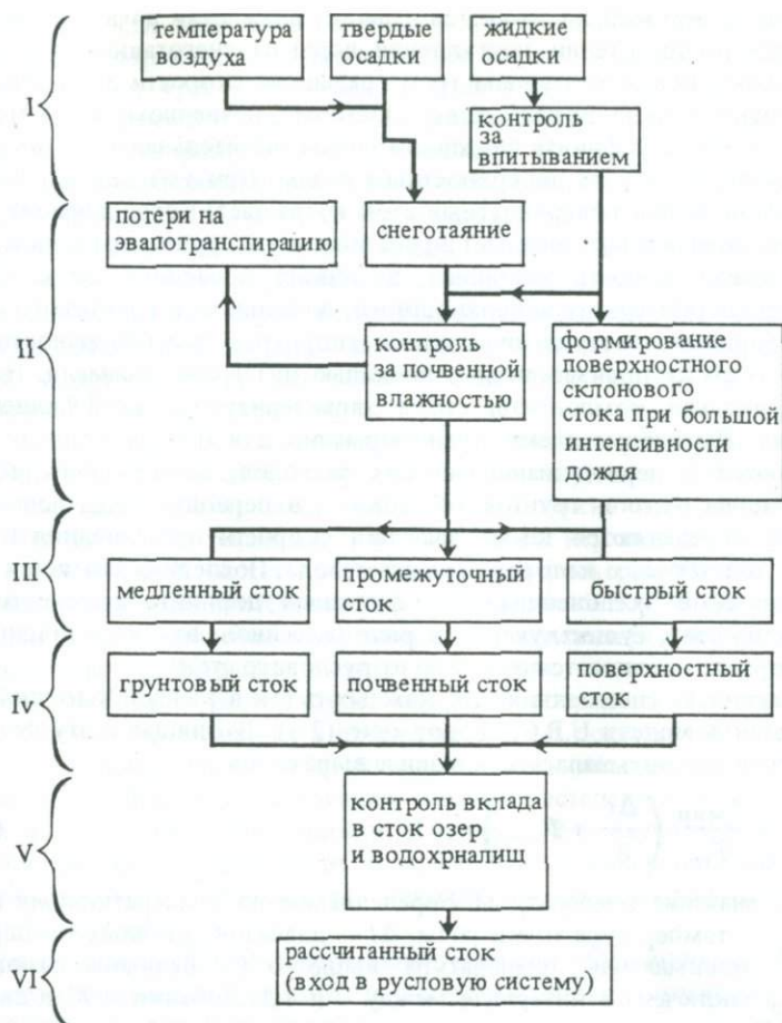
Рис. 5. Блок-схема модели U.V.C. [170]
