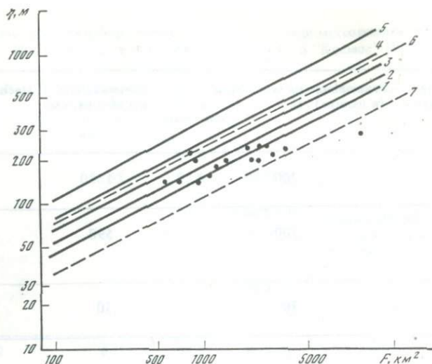
Рис. 1. Зависимости разрешающей способности ТВ информации \eta от площади горных водосборов F и степени их заснеженности при относительной ошибке определения заснеженности, равной 0,1, и разных значениях параметров a и b в формуле (1.15) [110]
