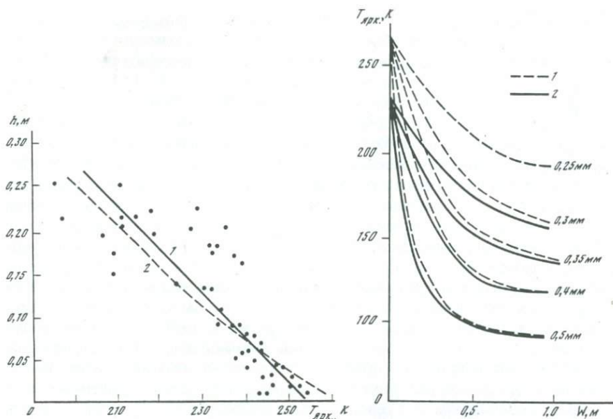
Рис. 2. Зависимости высоты снежного покрова h от радиояростной температуры T_{ярк} , определенной при микроволновом зондировании с ИСЗ "Nimbus-7" для южных степных районов СССР при вертикальной поляризации излучения с длиной волны \lambda = 0,81 см [147]
