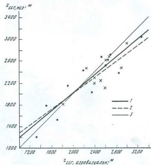
Рис. 20. Графики связи высоты сезонной снеговой границы, определенной по снимкам с ИСЗ и по данным аэровизуальных наблюдений, для бассейнов:
