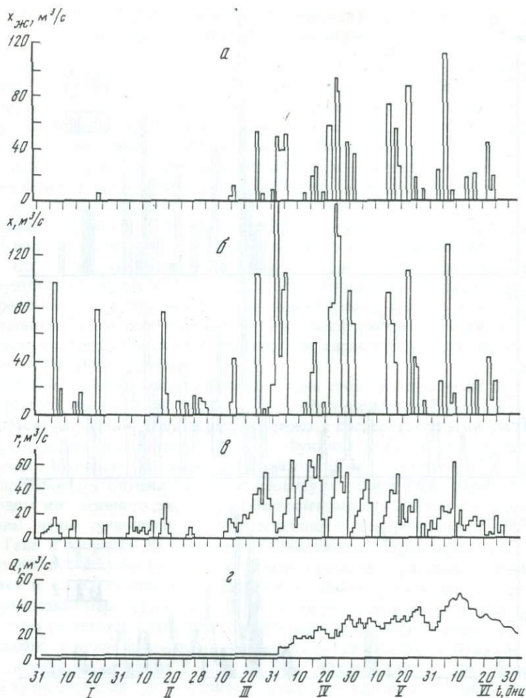
Рис. 11. Временной ход рассчитанных по модели значений x_{жж} — (а), x — (б), r — (в) и фактический гидрограф стока Q — (г) р. Гавасай — с. Гава для 1979 г.
