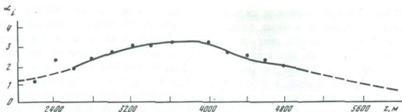
Рис. 4. Зависимость фактора орографического роста \alpha_i в формуле (2.25) от высоты водосбора z [132]
