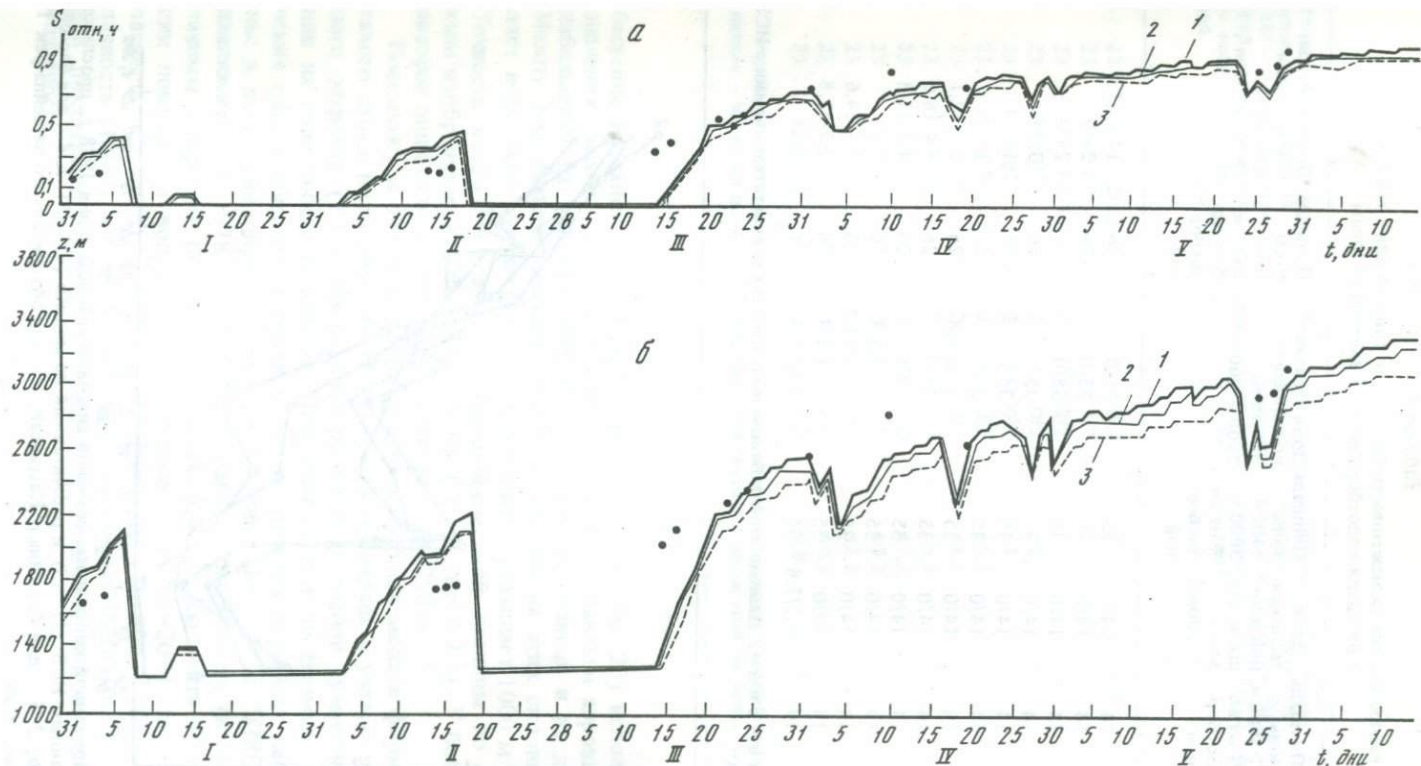
Рис. 17. Временной ход значений доли освободившейся от снега площади бассейна р. Кассансай S_{\text{отн.ч}} (а) и высотного положения снеговой линии z (б) для 1979 г.
