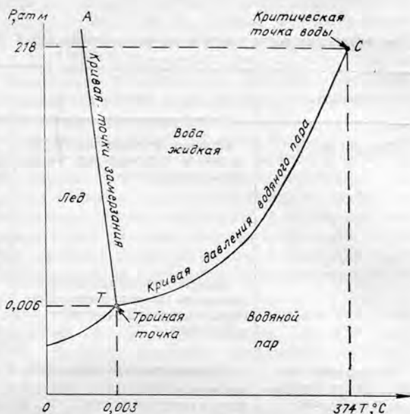
Рис. VI. 1. Диаграмма фазового состояния воды в зависимости от температуры и давления; по К. Краускоффу [1961].
