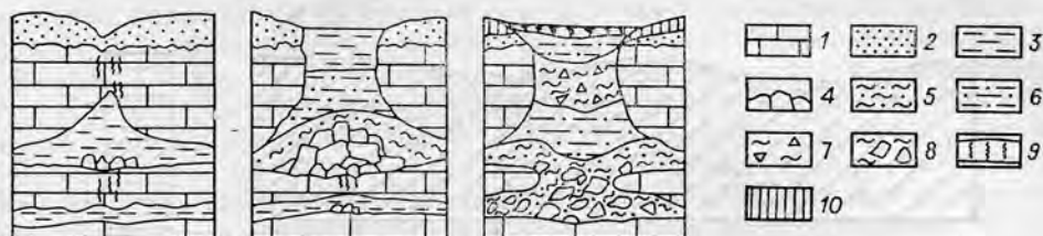
Рис. VIII.3. Стадии заполнения карстовой озерной ванны провального происхождения. 1 — карбонатные породы; 2 — пески; 3 — вода; 4 — коллювий обрушения; 5 — паттумы; 6 — алевроиты; 7 — суглинки с обломками; 8 — коллювий повторного обрушения; 9 — торф; 10 — покровные суглинки.
