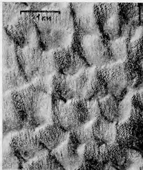
Рис. III.17. Барханоподобные драа (высотой ~50 м) [Wilson, 1972].
