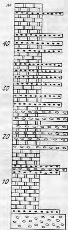
Рис. VII. 14. Разрез нижней части свиты буровой (рифей), р. Ниж. Тунгуска, Восточная Сибирь.
