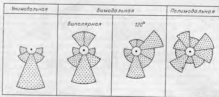
Рис. IX.3. Основные типы роз-диаграмм наклона косых слоев; по Ф. Петтиджону и др. [1967].
