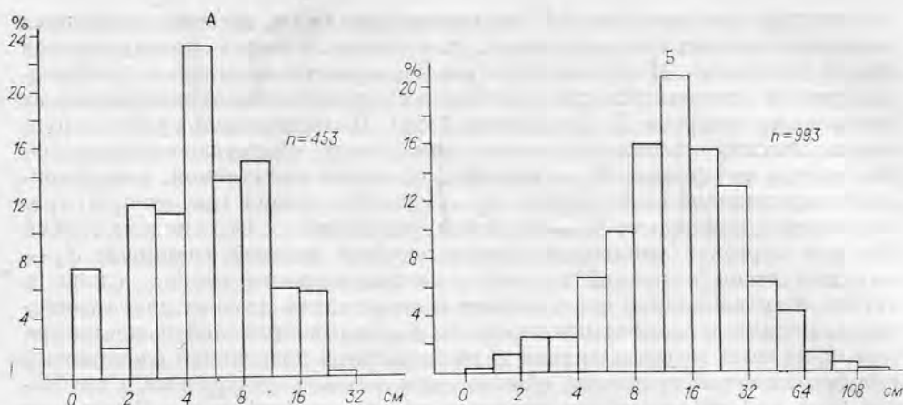
Рис. VII. 10. Распределение мощностей турбидитов одного гранулометрического класса (мелкозернистых T_3 ) в граувакковом флише. А — вендский флиш (рангская свита, Бол. Каратау); Б — верхнерифейский флиш (большекарройская свита, Мал. Каратау).
