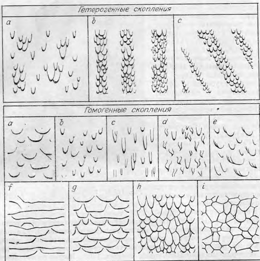
Рис. III.19. Типы скоплений и морфология слепков выемок [Allen, 1971].
