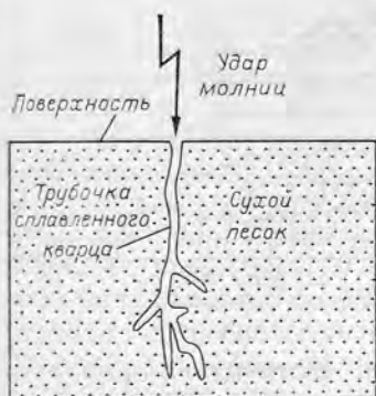
← Рис. III.48. Схема образования фульгурита [Шрок, 1950].
