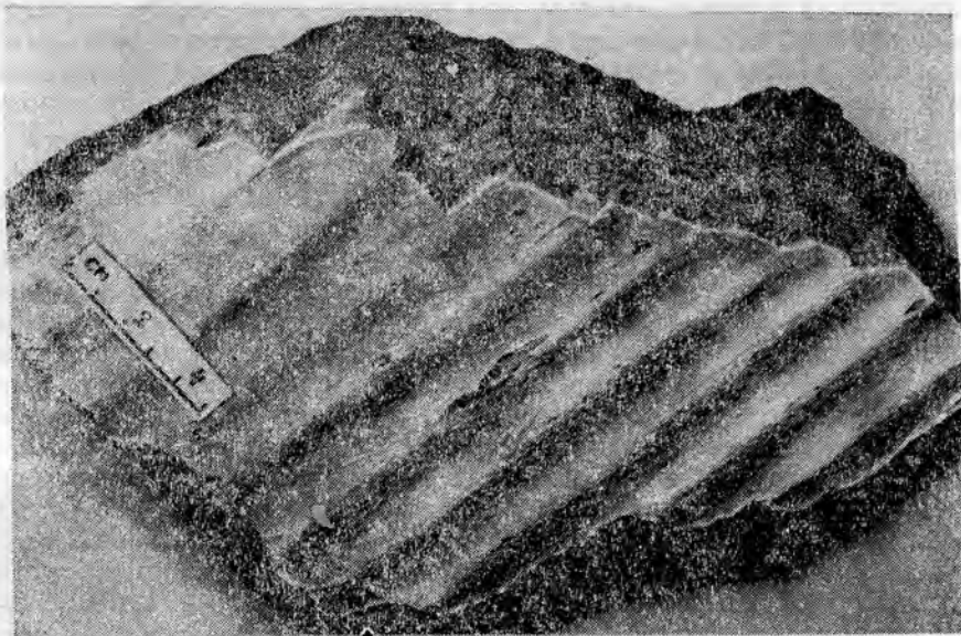
Рис. III.11. Прямолинейная мелкая рябь течения на поверхности мелкозернистого глинистого песчаника; Енисейский кряж, р. Енисей; верхний рифей, потоскуйская свита.
