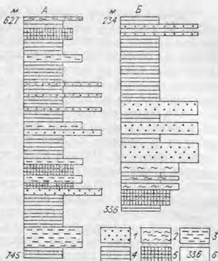
Рис. VII.8. Разрезы пестроцветной глинистой ассоциации (сеноман—турон).
