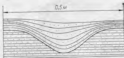
Рис. III.35. Косая слойчатость выполнения промоин; Восточная Сибирь, Енисейский край, р. Бол. Пит; верхний рифей, мелкозернистые глинисто-известковые песчаники нижнеангарской свиты.
