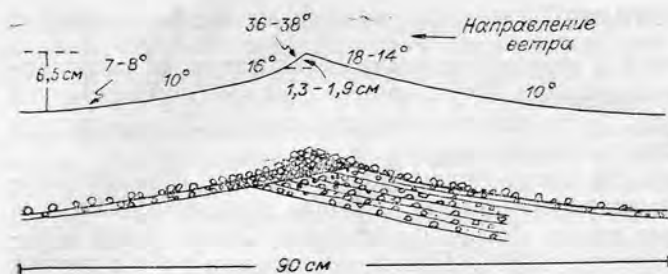
Рис. III.15. Гранулярная рябь; наличие чередовых слоев, падающих в противоположных направлениях, связано с изменением направления ветра; по Р. Шарпу [Sharp, 1963], с изменениями.
