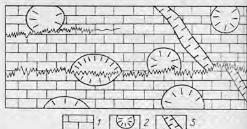
Рис. III.50. Стилолиты в известняке (1), пересекающие стебли кораллов (2) и прожилки кальцита (3); Крым; верхняя юра; по Г. И. Бушинскому [Справочник..., 1983].
