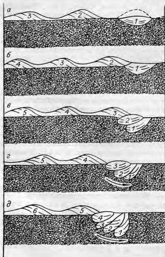
Рис. III.42. Схема развития знаков внедрения ряби; по С. Дзулинскому, И. Котларчику [Рейнек, Сингх, 1981].
