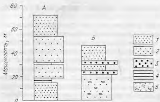
Рис. VII.1. Разрезы песчано-кварцевой ассоциации (верхний мел, сымская свита).
