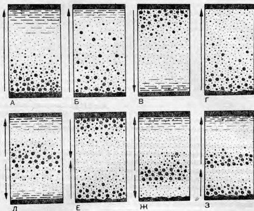
Рис. III.39. Типы градационной слоистости; по Ксеижкевичу [Седиментология, 1980]. А — Г — однократные, градуированные (А — с хорошим разделением, Б — с плохим разделением В — опрокинутые, Г — прерывистые, отсутствует мелкозернистая часть); Д — симметричные; Е — симметричные опрокинутые; Ж — несимметричные; З — двухкратные. Стрелки показывают на- правление уменьшения размера зерен.
