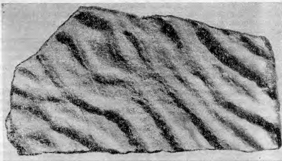
Рис. III.12. Волнистая мелкая рябь течения на поверхности мелкозернистого песчаника с раздваивающимися гребнями; Енисейский кряж, р. Бол. Пит; верхний рифей, киргитейская свита.
