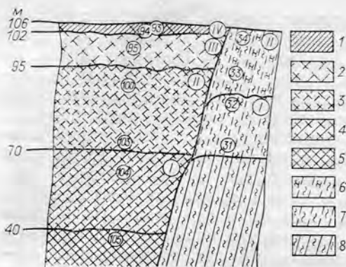
Рис. VII. 3. Схема вертикальной зональности коры выветривания железистых кварцитов и сланцев в северном борту Анновского карьера (Кривбасс, Украинский щит).
