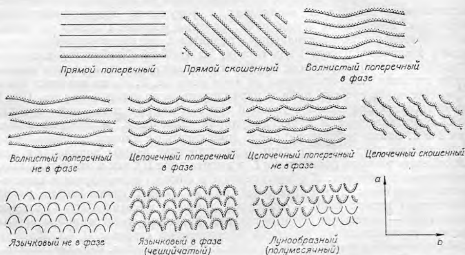
Рис. III.8. Классификация различных типов гребней ряби в плане; по Д. Аллену [Лидер, 1986].
