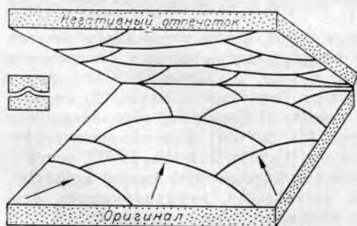
Рис. III.23. Следы прилива (знаки заплеска) [Шрок, 1950].
