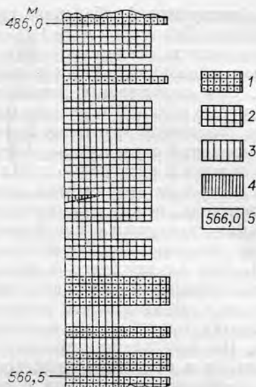
Рис. VII. 17. Разрез нижнего пласта калийных солей Старобинского месторождения; по А. А. Иванову, Ю. Ф. Левицкому [1960].
