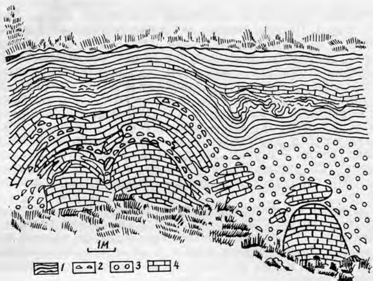
Рис. VII. 15. Онколито-строматолитовые биогермы. Зарисовка юго-западной стенки северного карьера на Южном Оленьем острове; по В. А. Соколову [1963].
