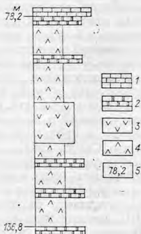
Рис. VII. 16. Разрез нижнепермских отложений в скв. 6, с. Порецкое, Русская платформа; по А. А. Иванову, Ю. Ф. Левицкому [1960].
