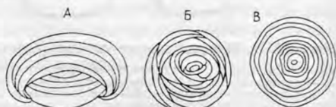
Рис. III.5. Классификация строматолитов, онколитов типа SS (spheroidal structure); по Б. Логану и др. [Седиментология, 1980].
