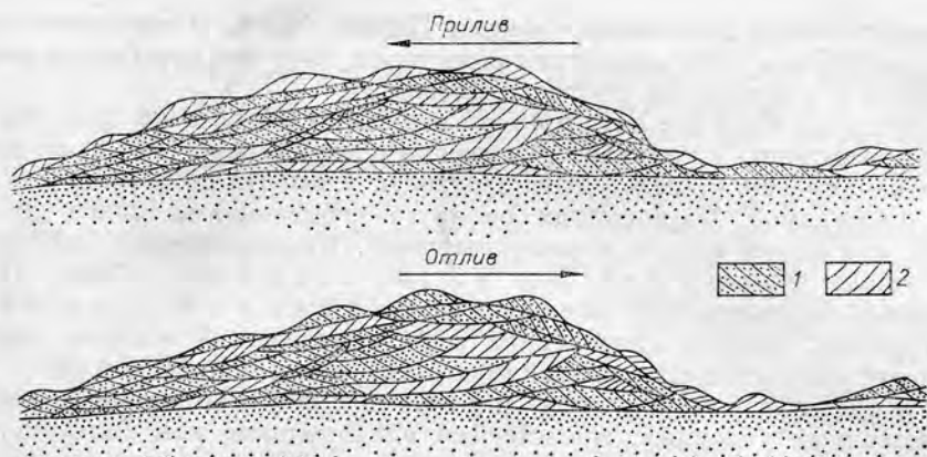
Рис. III.13. Внутреннее строение гигантской ряби [Рейнек, Сингх, 1981].
