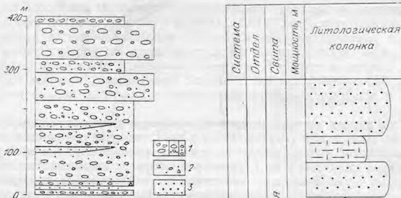
Рис. VII. 6. Разрез конгломератовой ассоциации в ордовикских отложениях, паразанская свита, р. Левый Каледом, Восточная Сибирь; по М. М. Оразовской [Булгакова, 1986], с изменениями.
