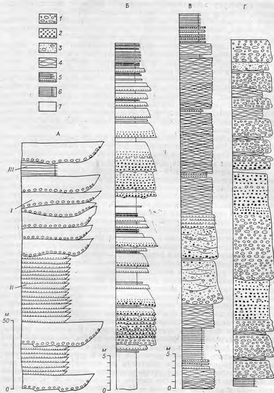
Рис. VII. 12. Массивно-линзовые и пластовые последовательности в граувакковом и карбонатном флишах.
