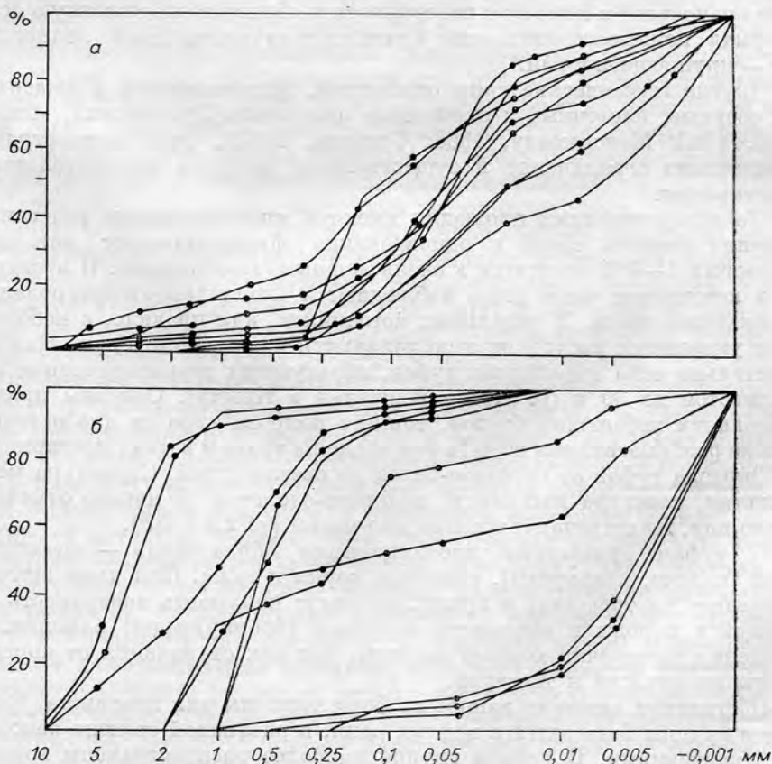
Рис. VIII.2. Куммулятивные графики инфлювия и аллювия.
