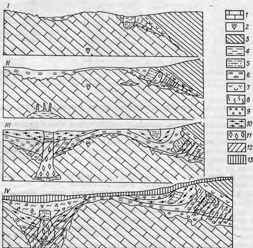
Рис. VIII.4. Схема формирования КСК.
