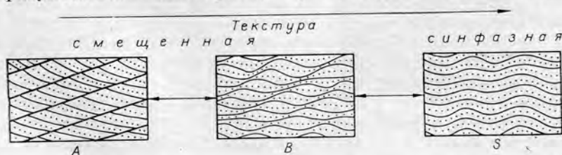
Рис. III.36. Три типа ( A , B , S ) слойчатых текстур восходящих знаков ряби. Стрелка над рисунком показывает увеличение отношения взвешенного материала (суспензии) к материалу твердого стока (влекомого по дну); по А. Джолингу, Р. Уолкеру [Jorling, Walker, 1968], с изменениями.
