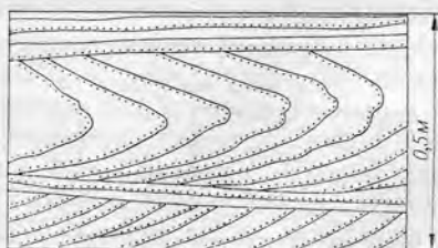
Рис. III.34. Опрокинутая косо́я сло́йчатость; Иркутское Присаянье, р. Иркут; венд, песчанки шамановской свиты (зарисовка с фотогра́фии).
