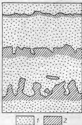
Рис. III.51. Поверхность палеокарста. 1 — известняк зеленовато-серый; 2 — кайма охристо-желтой окраски; по С. Г. Вишнякову, Р. Ф. Геккеру [Рухин, 1953].
