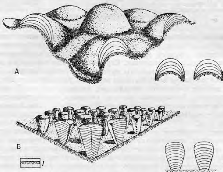
Рис. III.3. Классификация строматолитов типа SH (vertikal stacked hemispheroids); по Б. Логану и др. [Седиментология, 1980].
