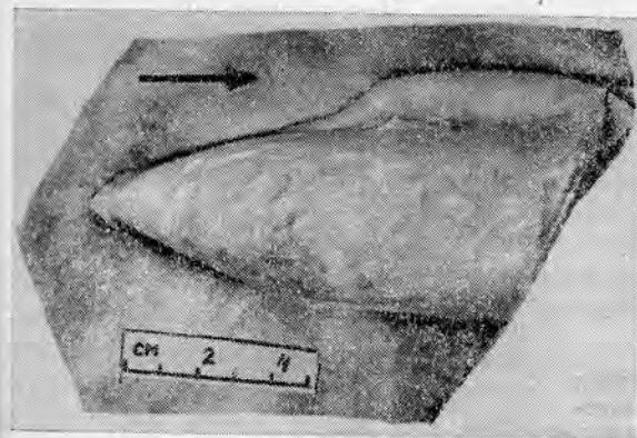
Рис. III.18. Слпок водоворотной ямки в подошве песчанистого микритового известняка; Евсейский краж, р. Каменка, верхний рифей, шунтарская свита; — образец С. В. Сараева.
