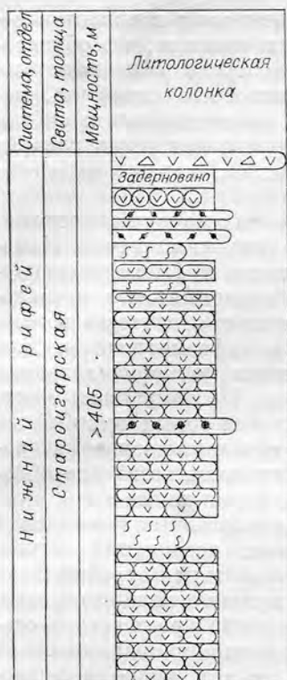
Рис. VII. 4. Разрез вулканокластической ассоциации (староигарская толща Игарского района, Восточная Сибирь); по Г. Г. Гелеяну [1970], с небольшими изменениями.
