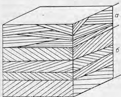
Рис. III.33. Перекрестная (а) и елочная (б) косо́я сло́йчатость.
