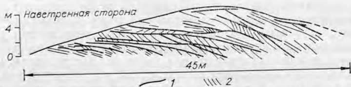
Рис. III.16. Внутреннее строение барханоподобной дюны [McKee, 1966].
