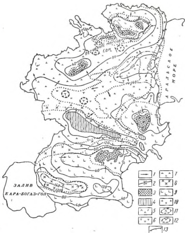
Рис. 29. Гидрогеологическая карта грунтовых вод неоген-четвертичных отложений плато Устьюрт. Составили В. Н. Соколов и А. С. Вишняков
